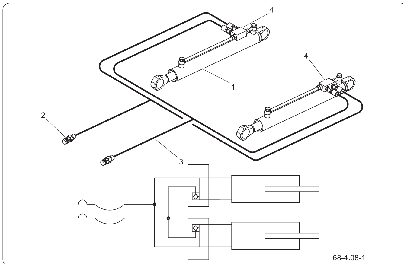
Rysunek 4.13 Budowa i schemat instalacji hydraulicznej klapy tylnej (SILO)
