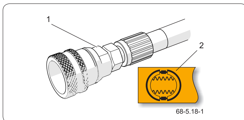
Rysunek 5.13 Przewód instalacji hamulcowej hydraulicznej
