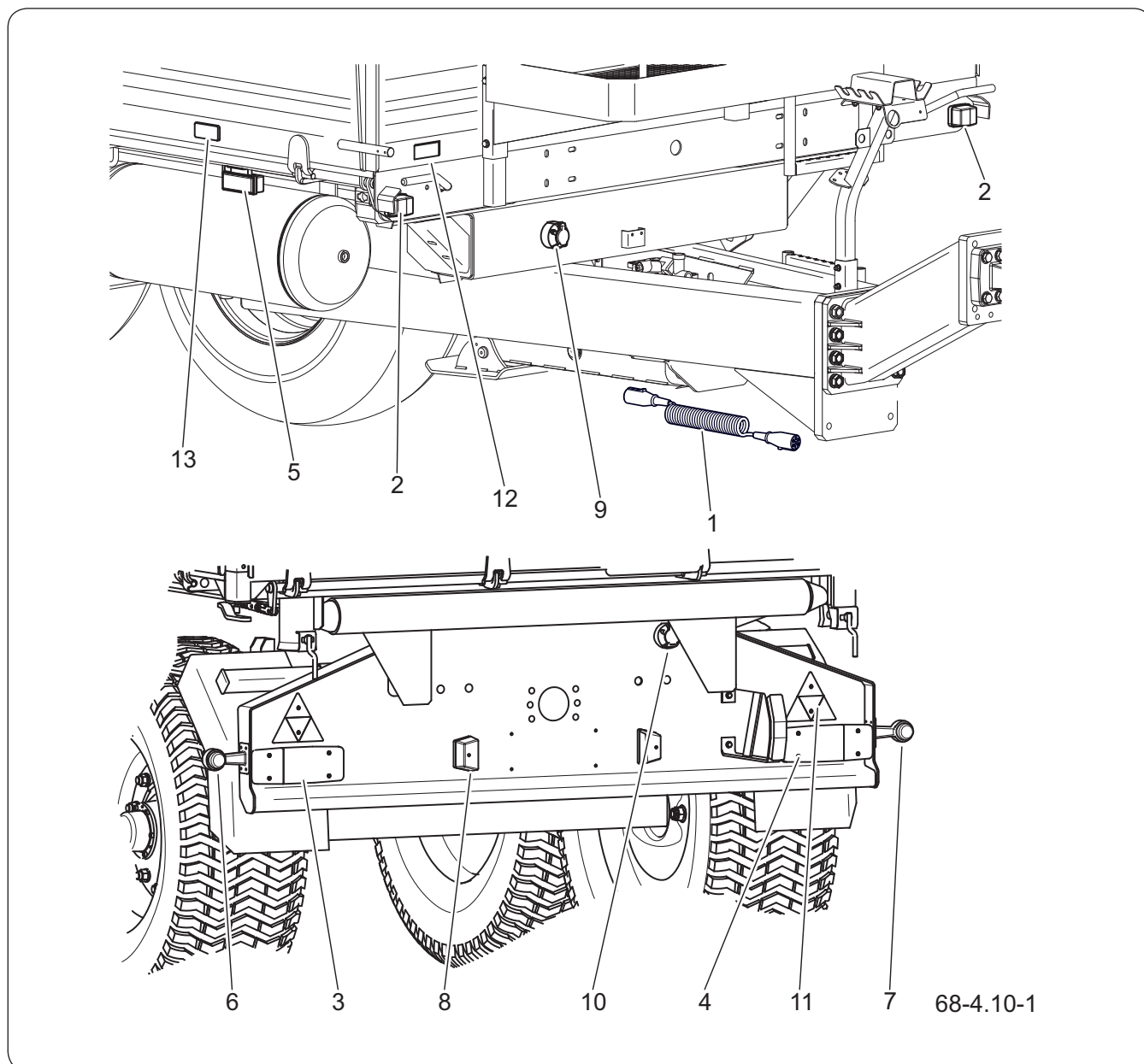
Rysunek 4.15 Rozmieszczenie elementów instalacji elektrycznej oraz elementów odblaskowych
