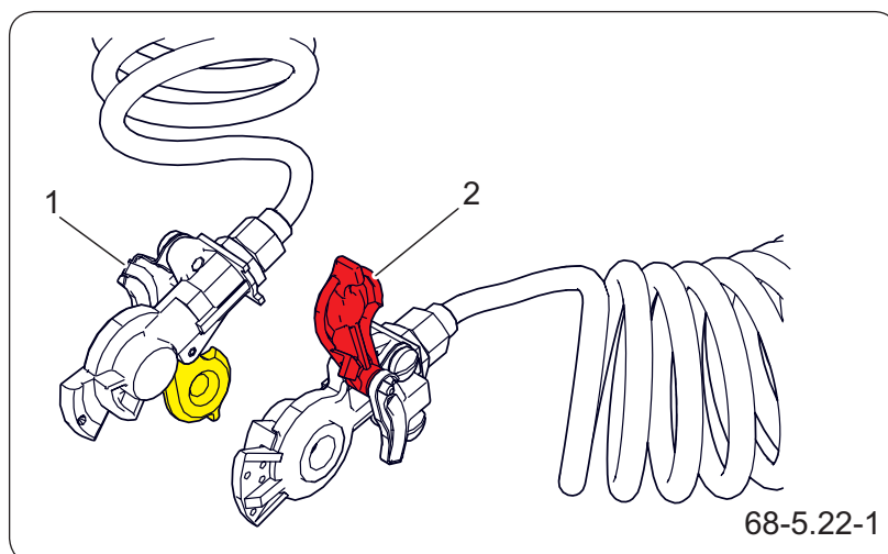
Rysunek 5.11 Instalacja hamulcowa dwuprzewodowa (1) wtyk żółty (2) wtyk czerwony
