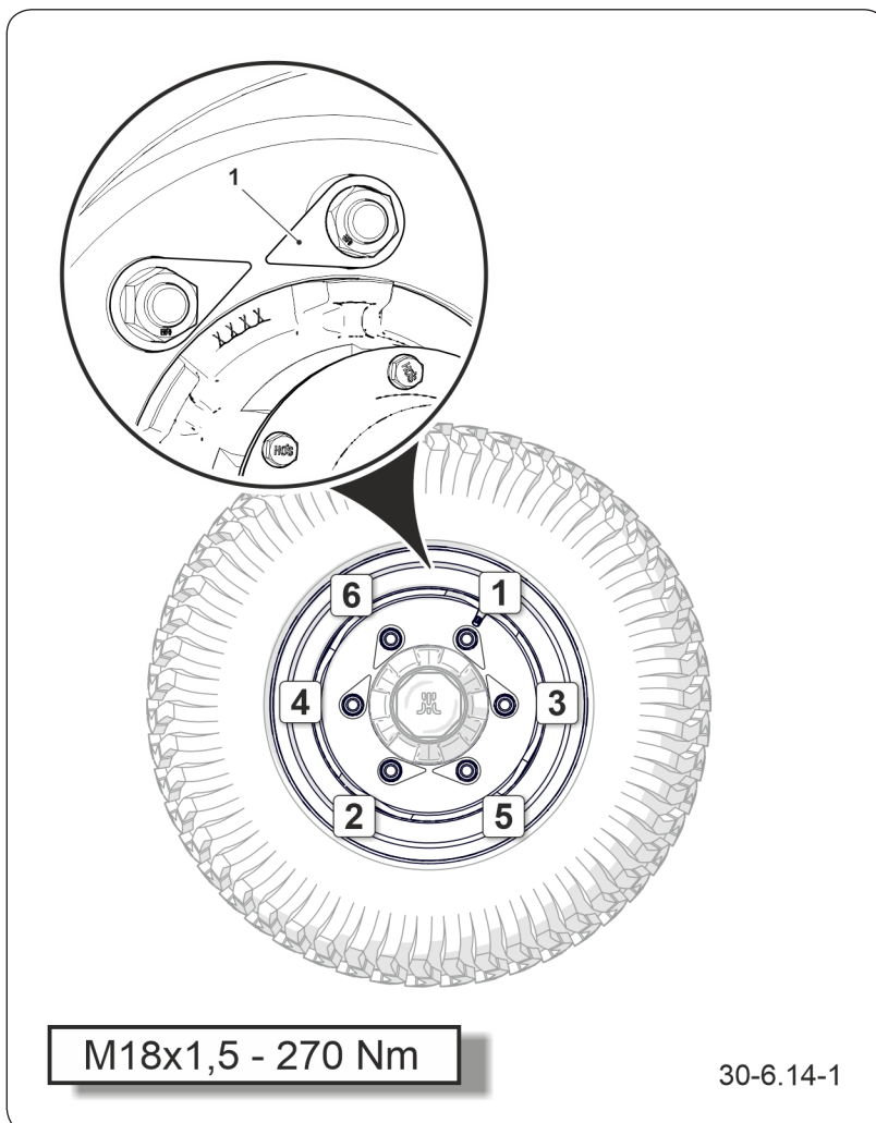
Rysunek 6.14 Kolejność dokręcania nakrętek (1) wskaźnik dokręcenia nakrętki
