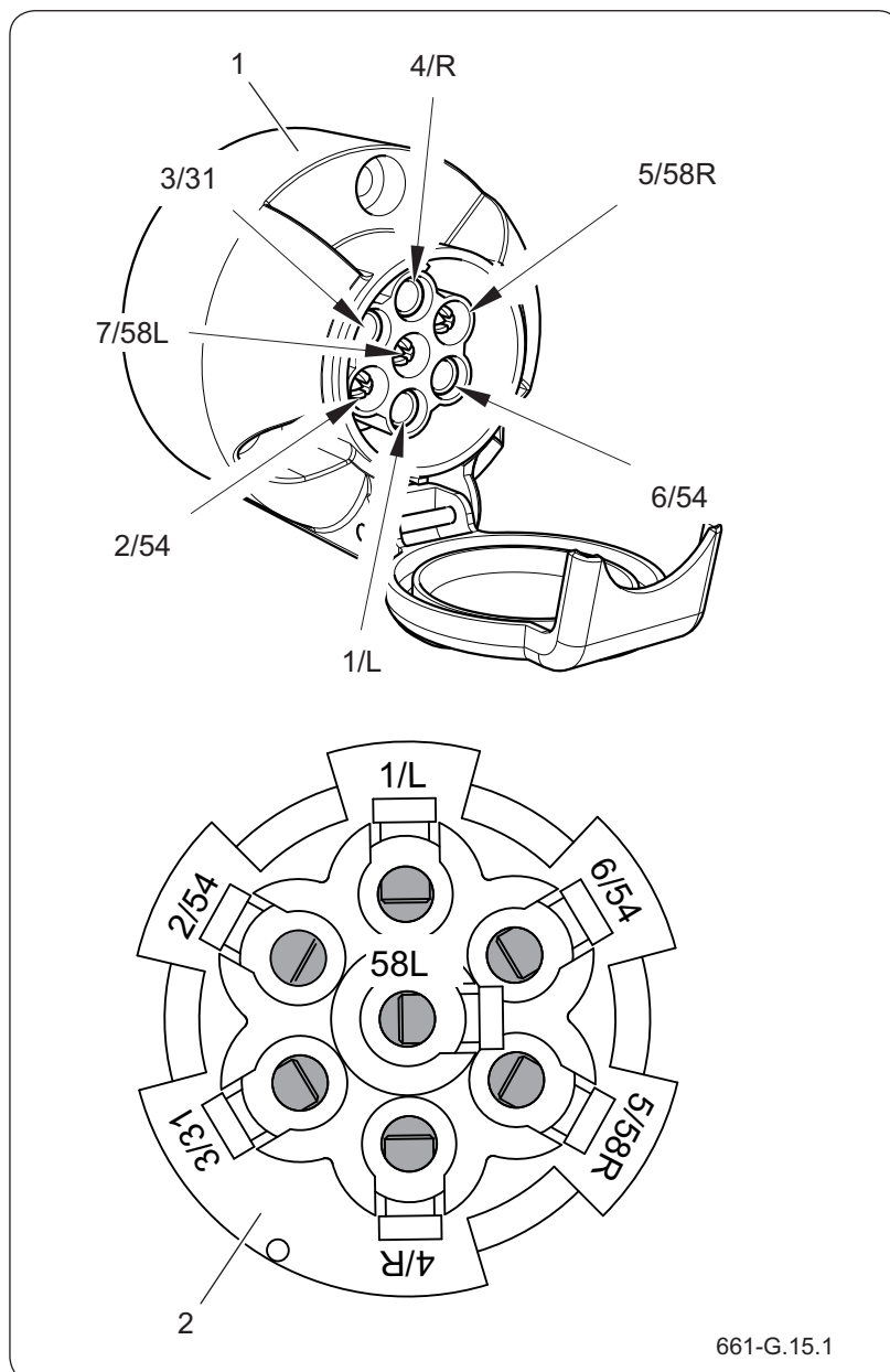
Rysunek 4.17 Gniazdo przyłączeniowe 7 pin
