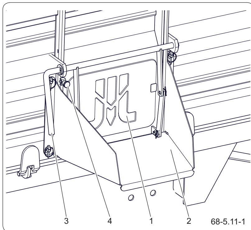
Rysunek 5.35 Szyber zsypowy
