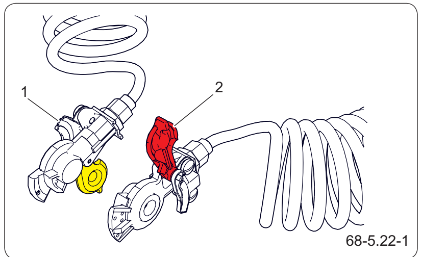
Abbildung 5.11 Z w e i l e i t u n g s - Druckluftbremsanlage (1) gelber Kupplungskopf (2) roter Kupplungskopf
