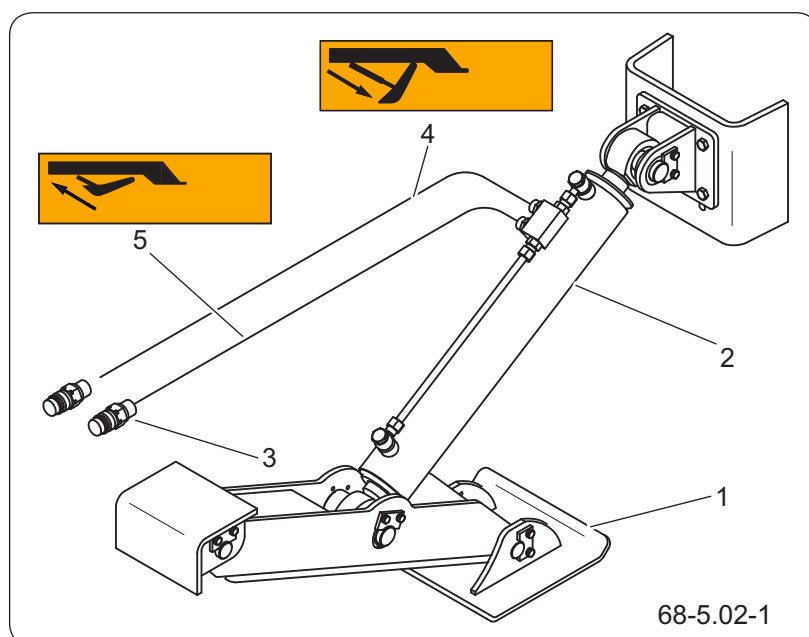
Abbildung 5.10 Scherenstützfuß
