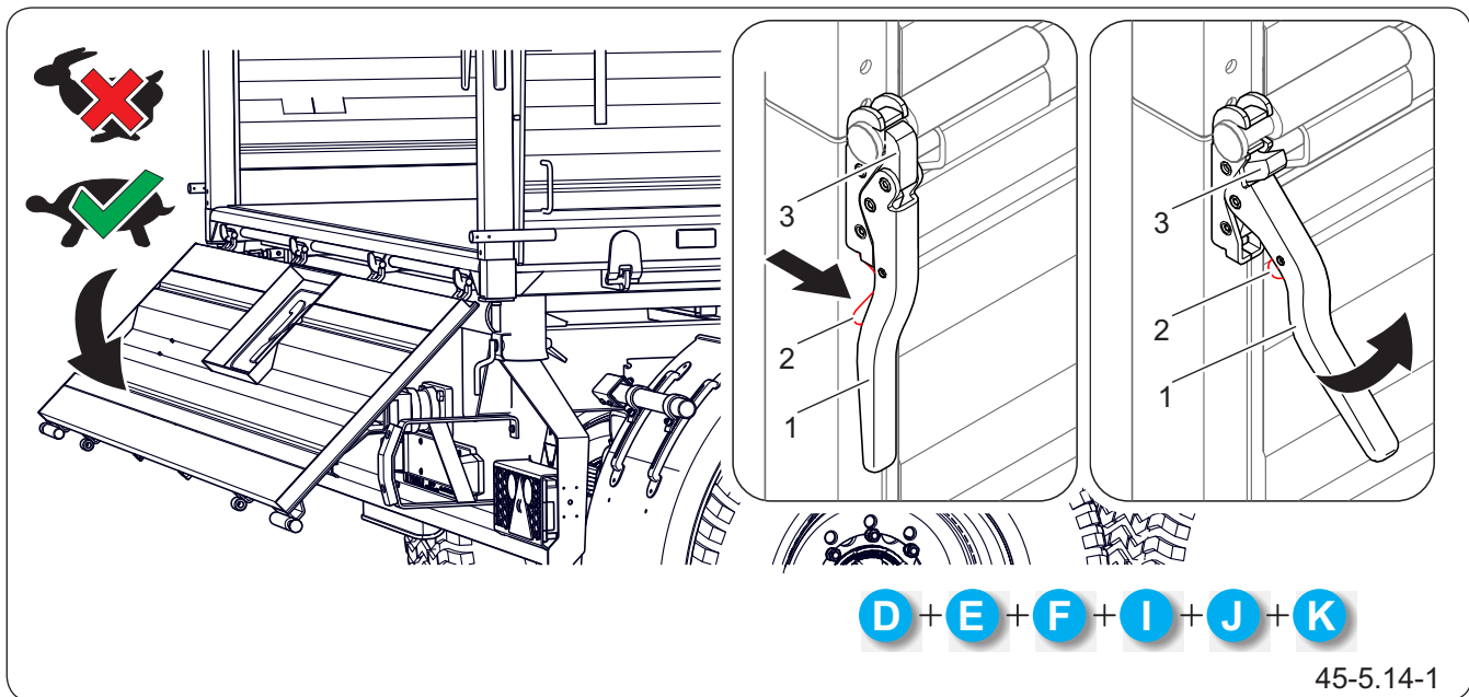
Abbildung 5.29 Bordwandverschluss
