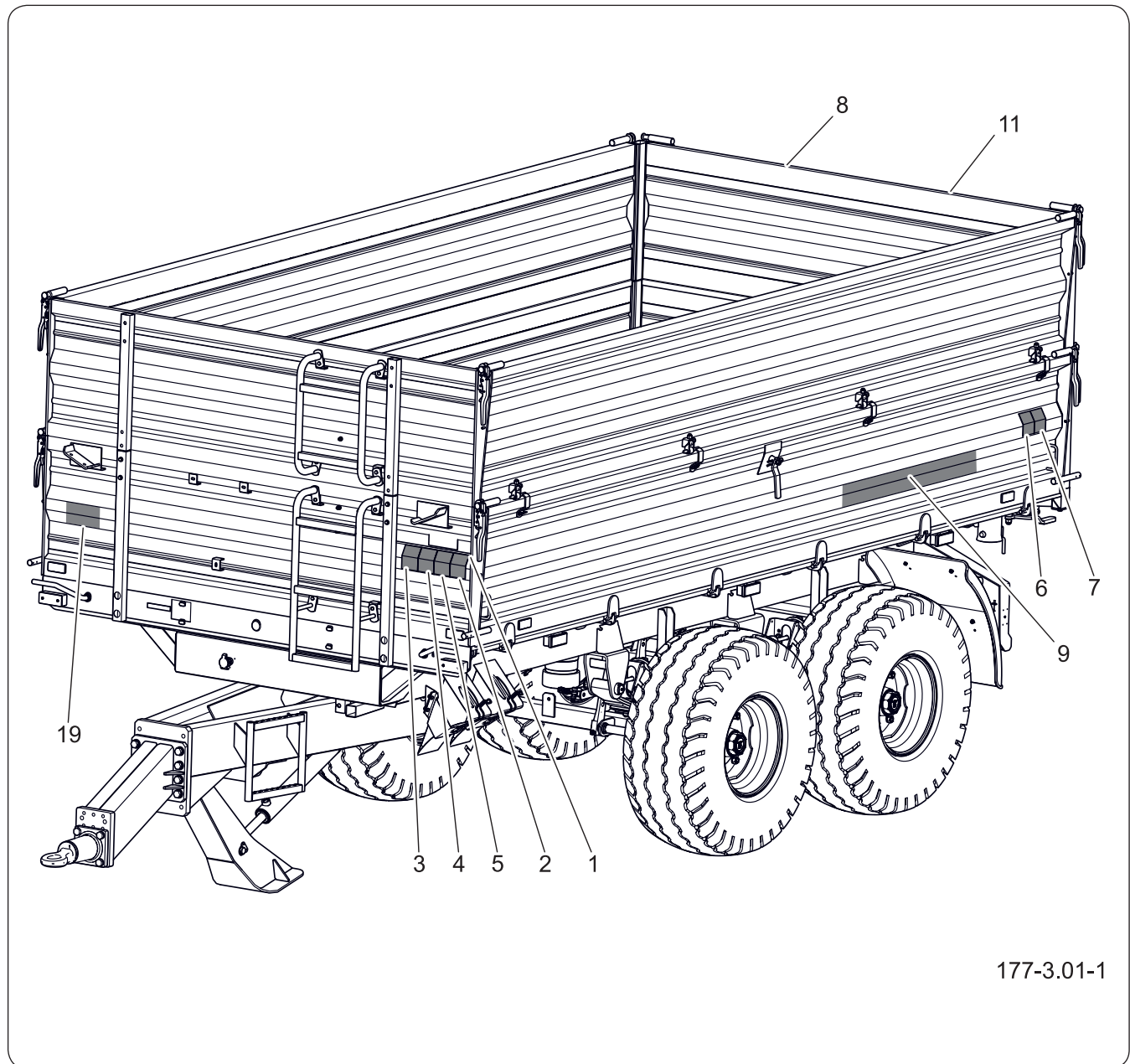
Abbildung 3.3 Anordnung der Hinweis- und Warnschilder den Hydraulikleitungen.
