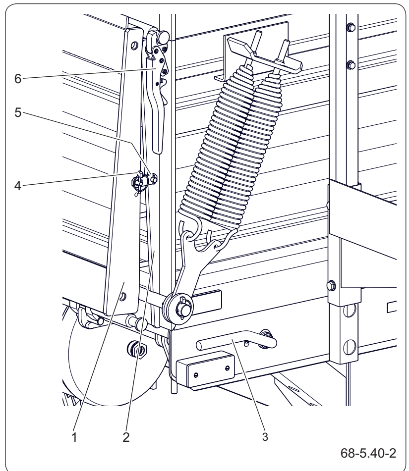
Abbildung 5.30 Zusammenklappen von Wand und Aufsatz
