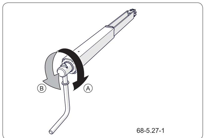
Abbildung 5.5 Feststellbremsmechanismus
