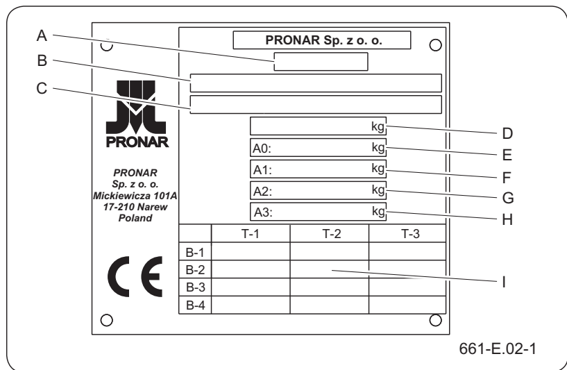
Abbildung 2.5 Typenschild EU
