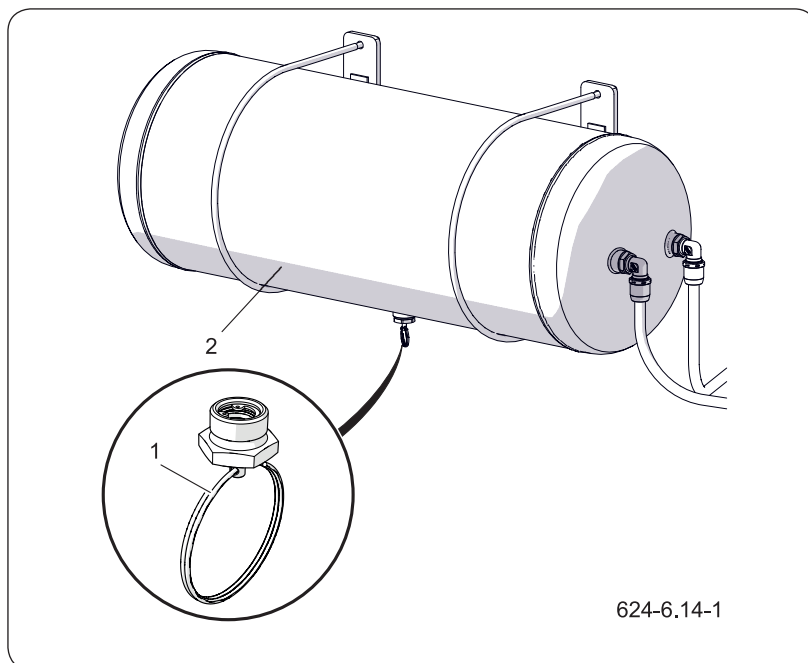
Abbildung 6.8 Druckluftbehälter
