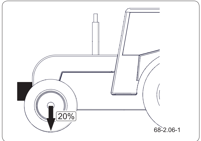
Abbildung 2.6 Mindestvorderachslast des Schleppers
