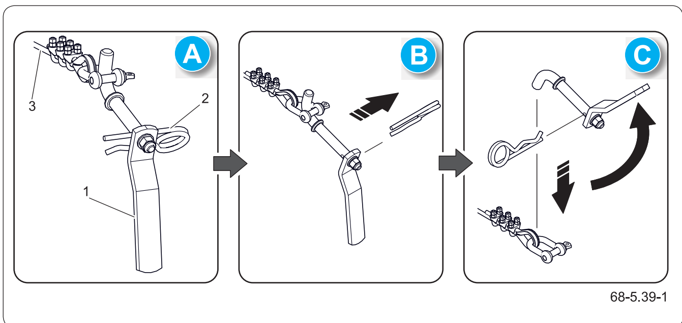
Abbildung 5.24 (3) Spannseil
