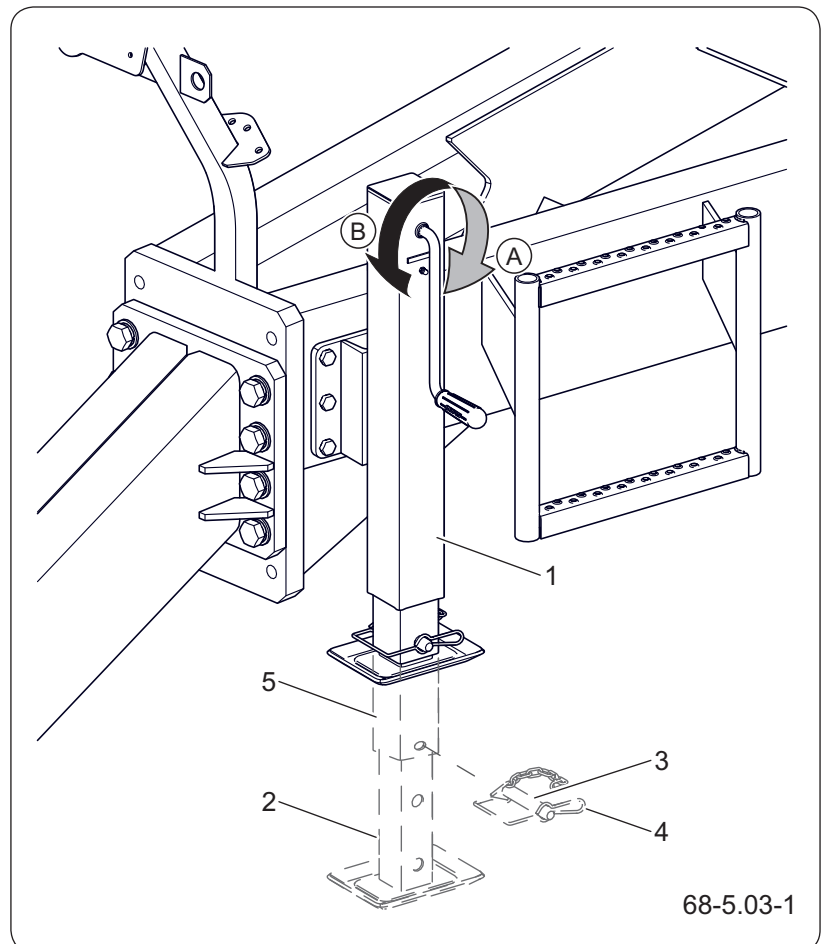
Abbildung 5.11 Mechanische Stütze
