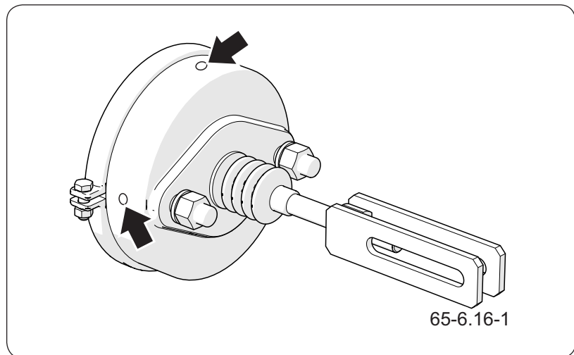
Abbildung 6.5 Bremszylinder
