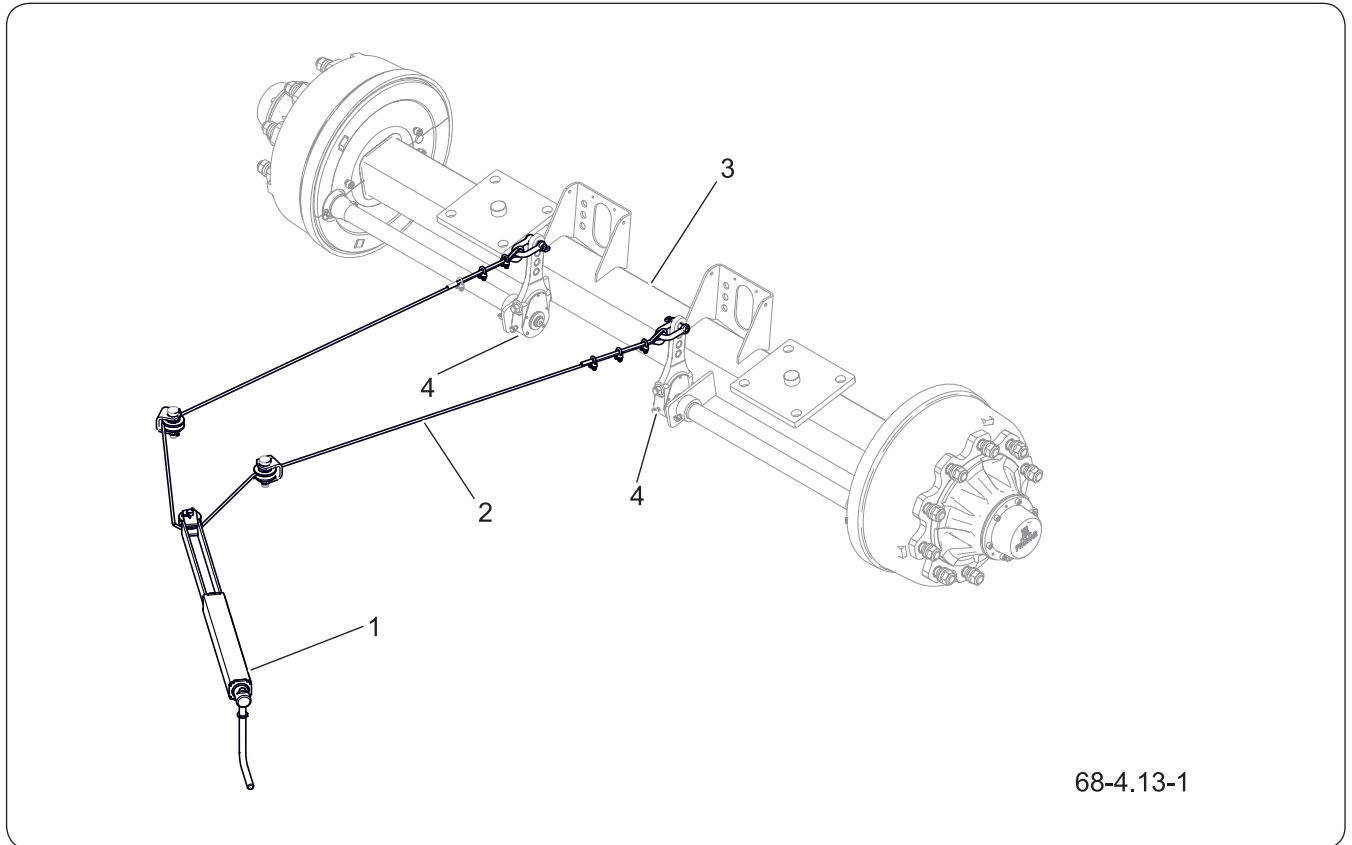
Abbildung 4.11 Aufbau der Feststellbremse
