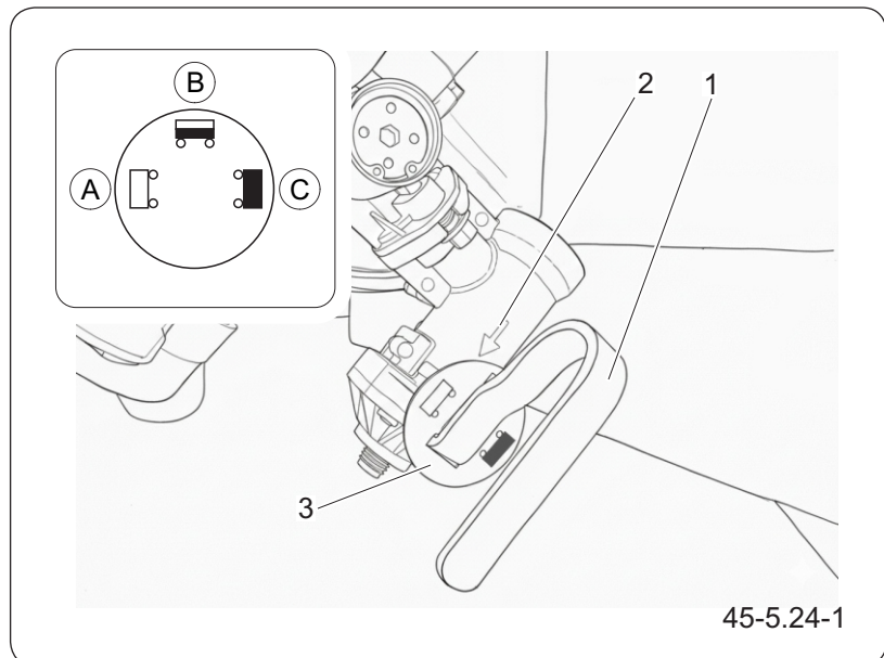
Abbildung 5.17 Bremskraftregler in der Druckluftanlage
