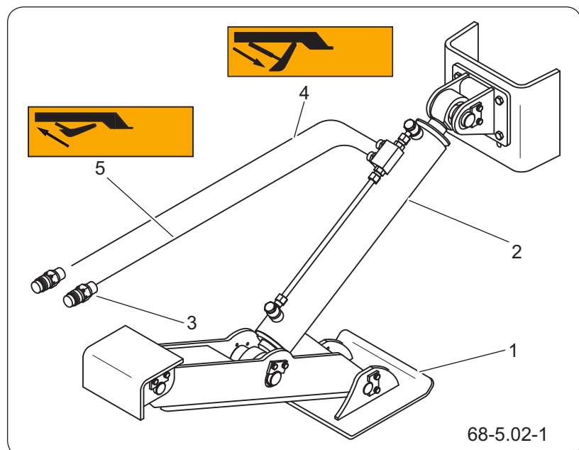
Abbildung 5.10 Scherenstützfuß
