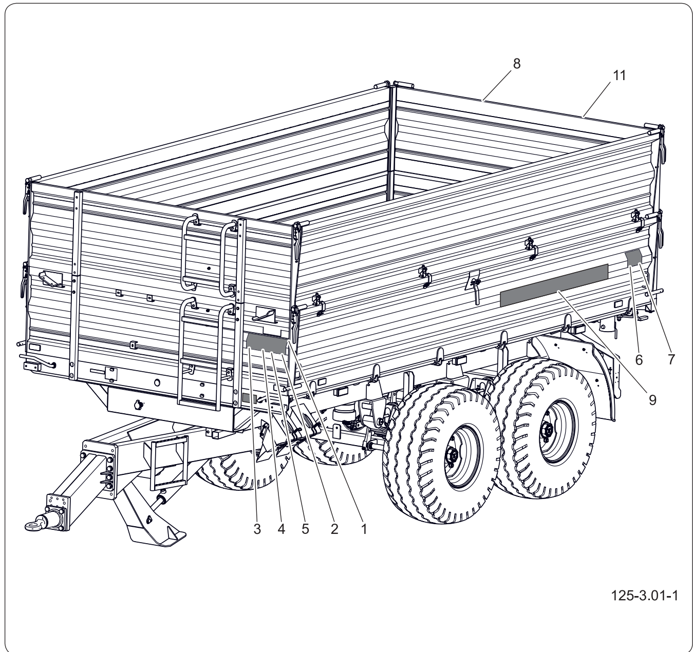
Abbildung 3.3 Anordnung der Hinweis- und Warnschilder
