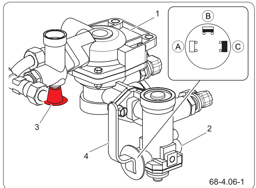
Abbildung 4.9 Steuerventil
