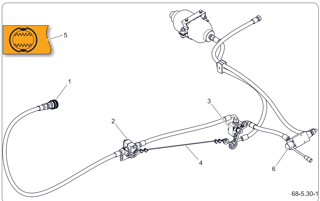
Abbildung 5.15 Bremsanlage
