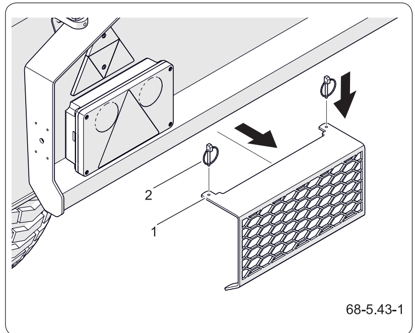
Abbildung 5.16 Lampenschutz
