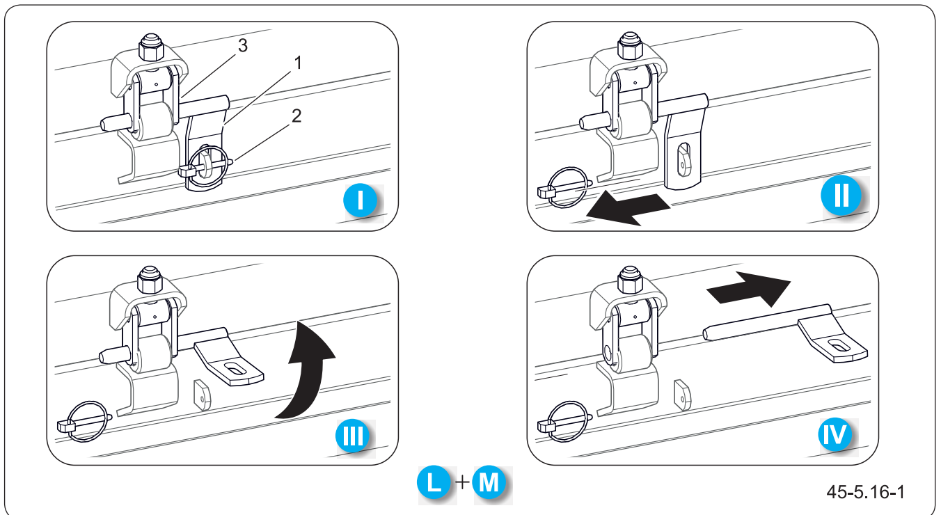
Abbildung 5.29 Heckscharnier
