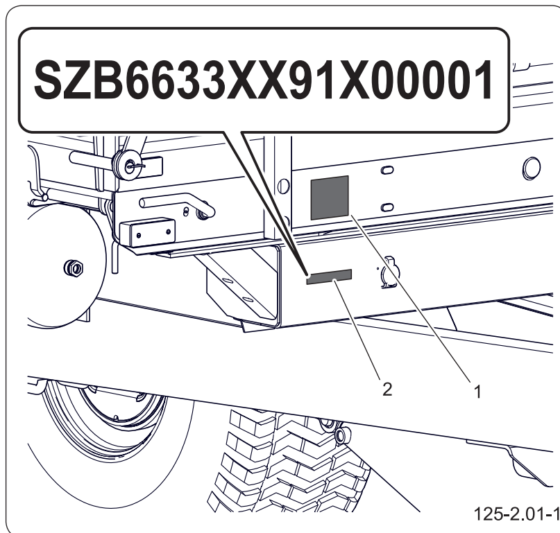
Abbildung 2.3 Identifikation des Anhängers
