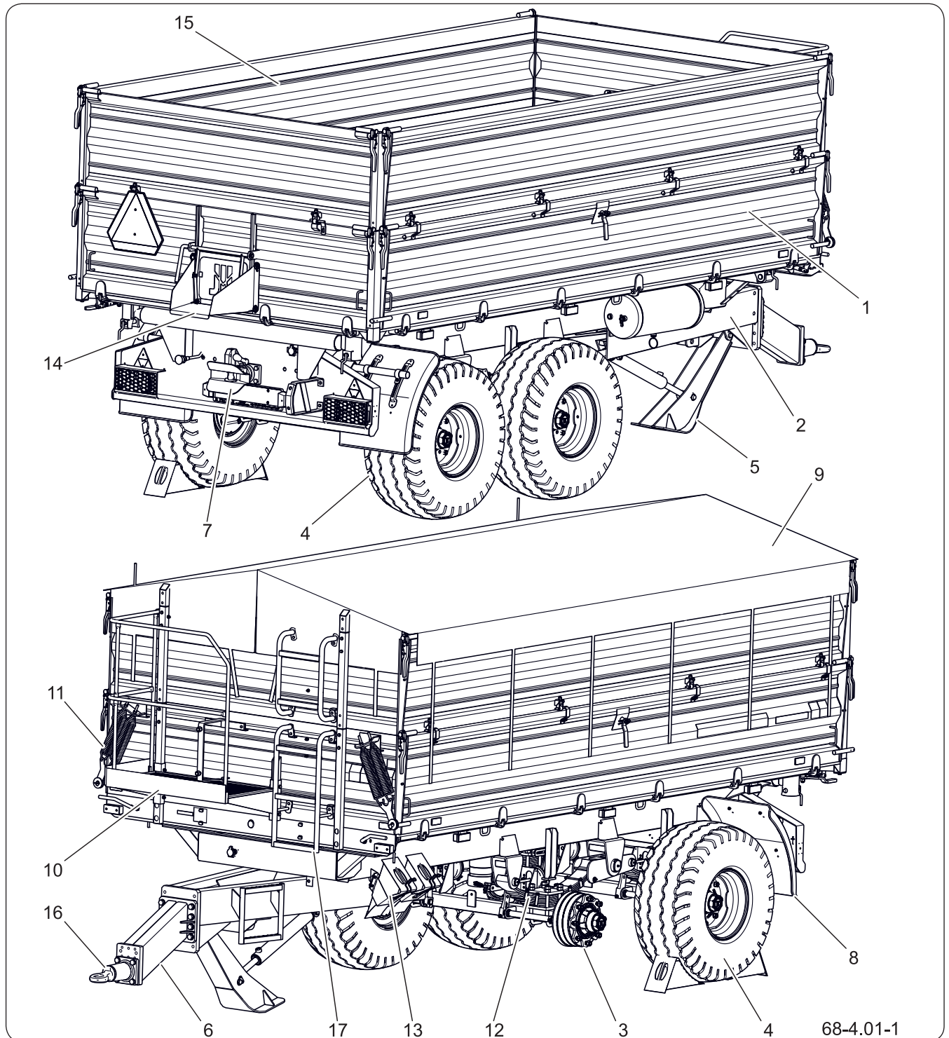
Abbildung 4.1 Aufbau des Anhängers
