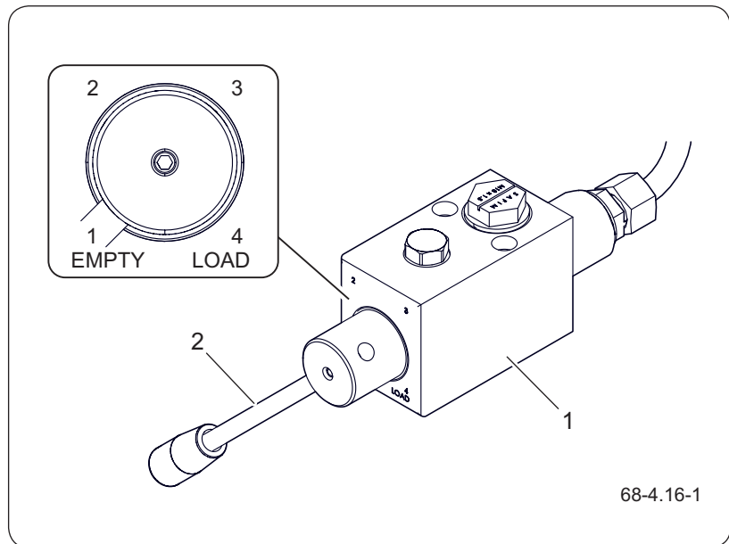
Abbildung 4.10 Bremskraftregler (1) Bremskraftregler (2) Hebel
