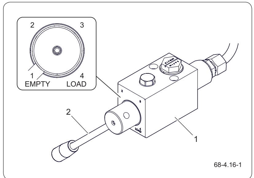
Abbildung 5.18 Bremskraftregler in der Hydraulikanlage
