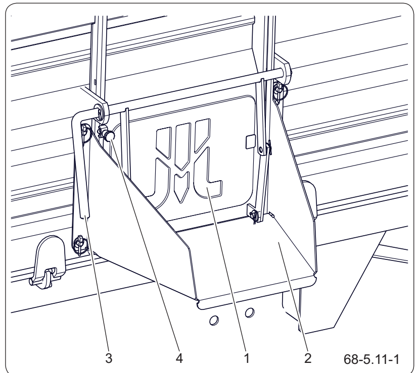
Abbildung 5.36 Kornschieber
