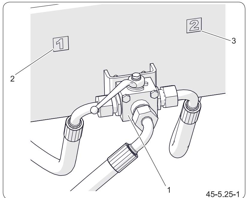
Abbildung 5.23 Hydraulikventil
