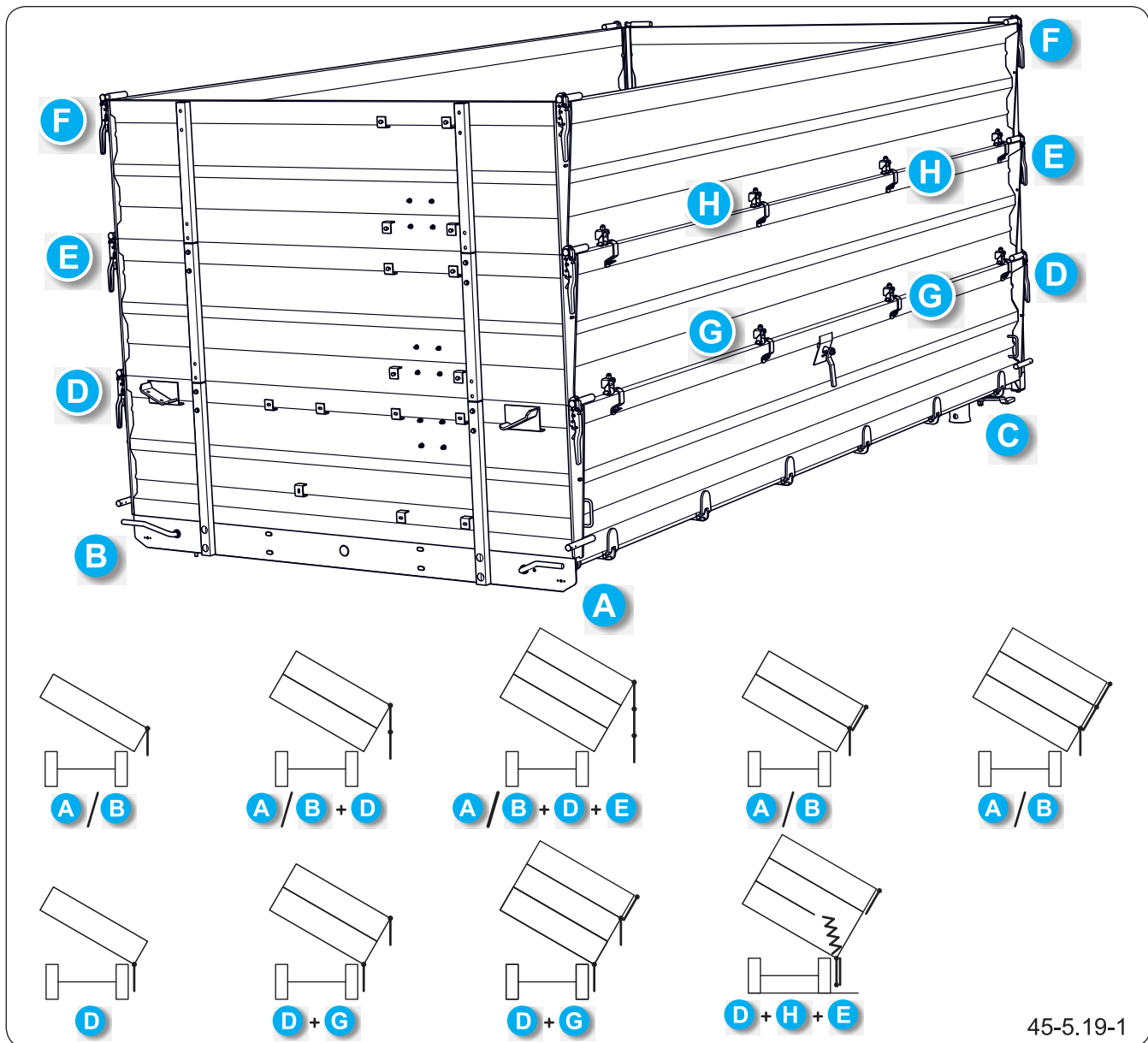
Abbildung 5.25 Varianten der Seitenbordwandöffnung
