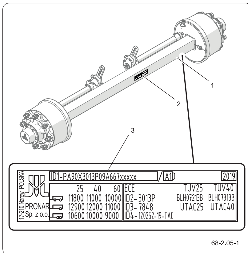
Abbildung 2.5 Identifizierung der Achsen
