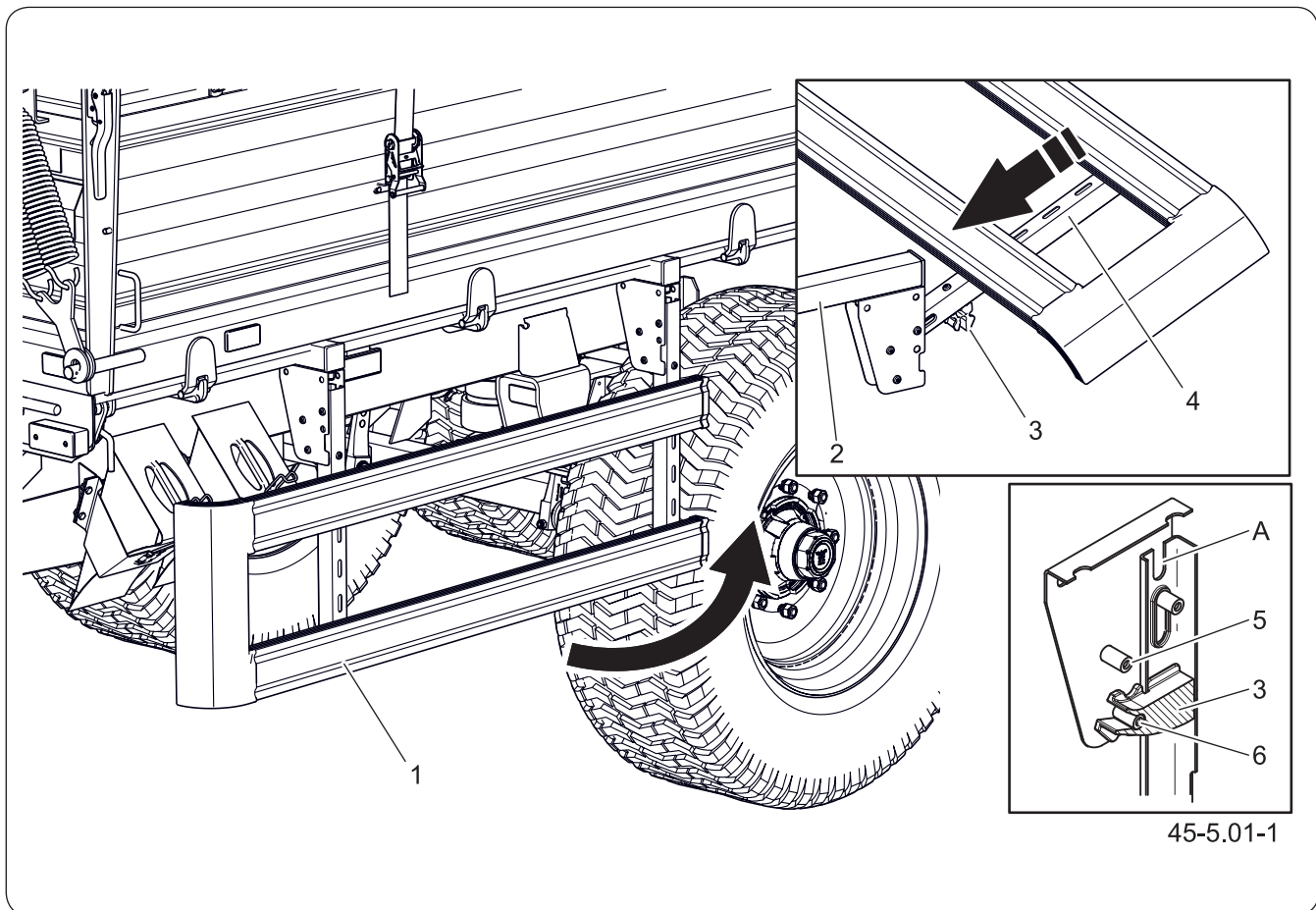
Abbildung 5.19 Bedienung des seitlichen Unterfahrschutzes
