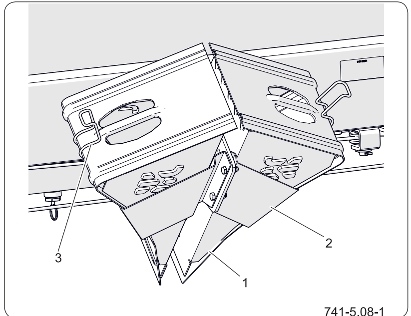
Rysunek 5.2 Gniazda odstawcze klinów
