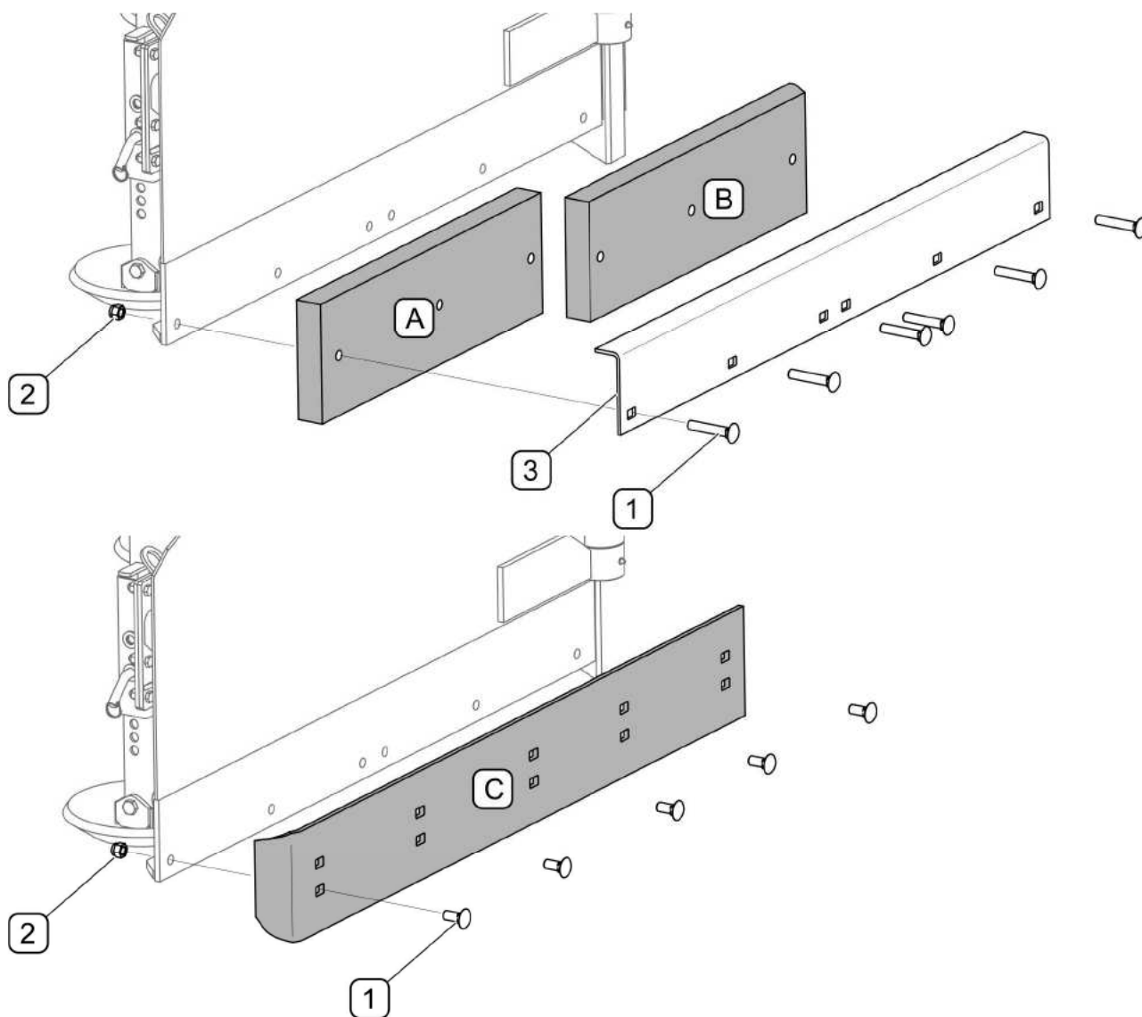
RYSUNEK 5.1 Wymiana listwy zgarniającej
