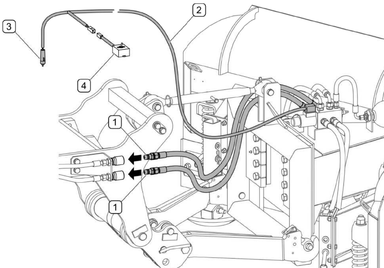
RYSUNEK 4.3 Podłączenie instalacji hydraulicznej i elektrycznej do ciągnika
