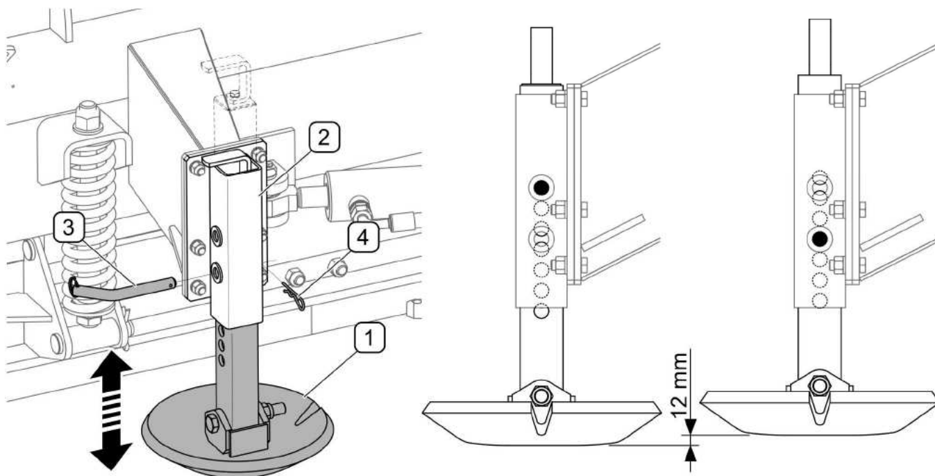
RYSUNEK 4.8 Regulacja wysokości pracy w pługach wyposażonych w ślizgi
