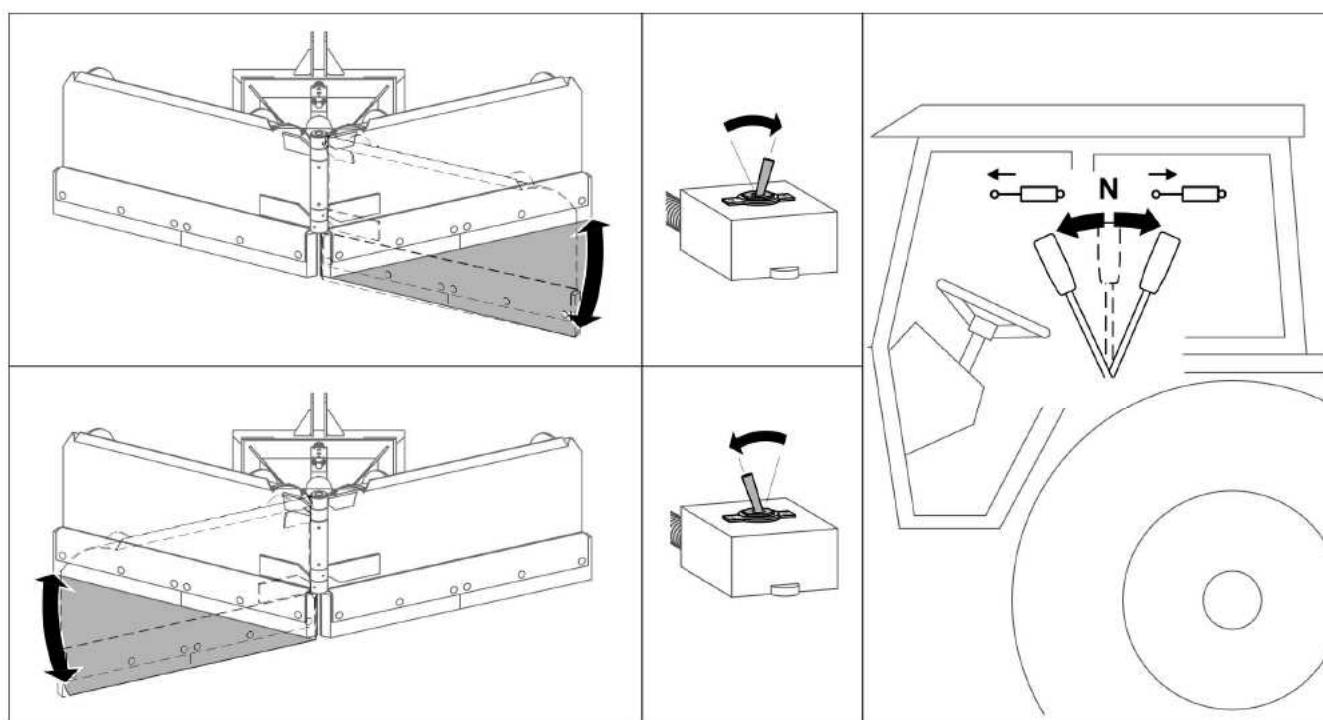
RYSUNEK 4.6 Zmiana pozycji roboczej
