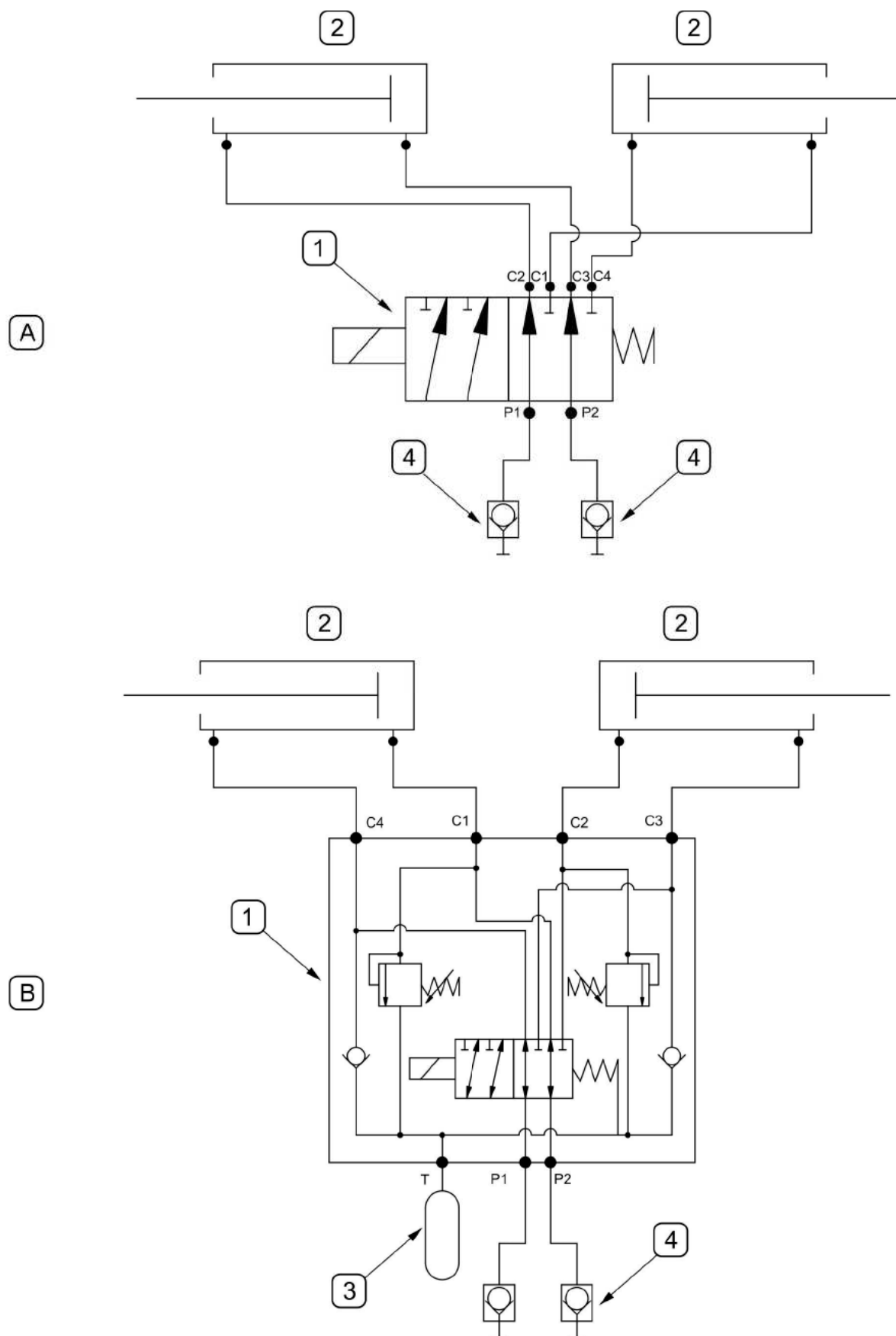
RYСУNEK 3.4 Schemat ideowy instalacji hydraulicznej
