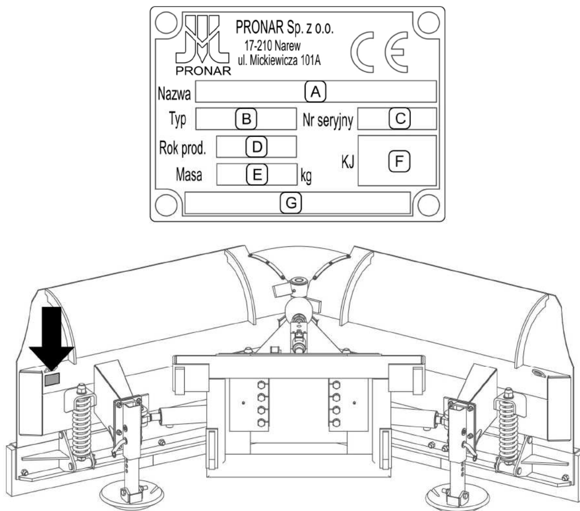
RYSUNEK 1.1 Miejsce umieszczenia tabliczki znamionowej
