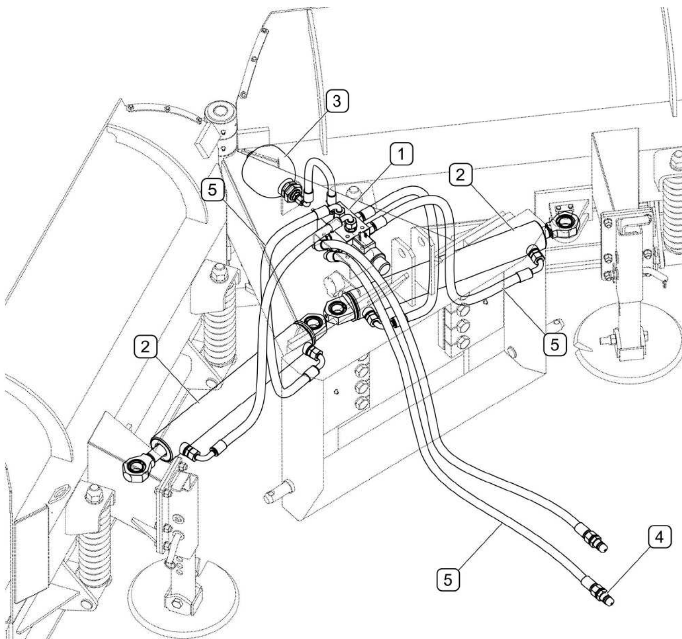
RYСУNEK 3.3 Budowa instalacji hydraulicznej
