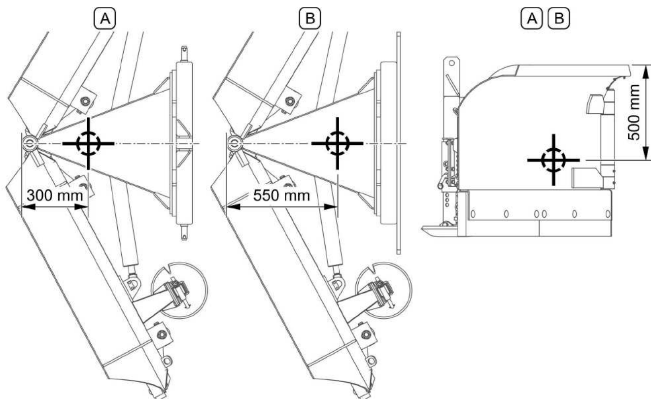
RYСУNEK 1.3 Położenie środka ciężkości
