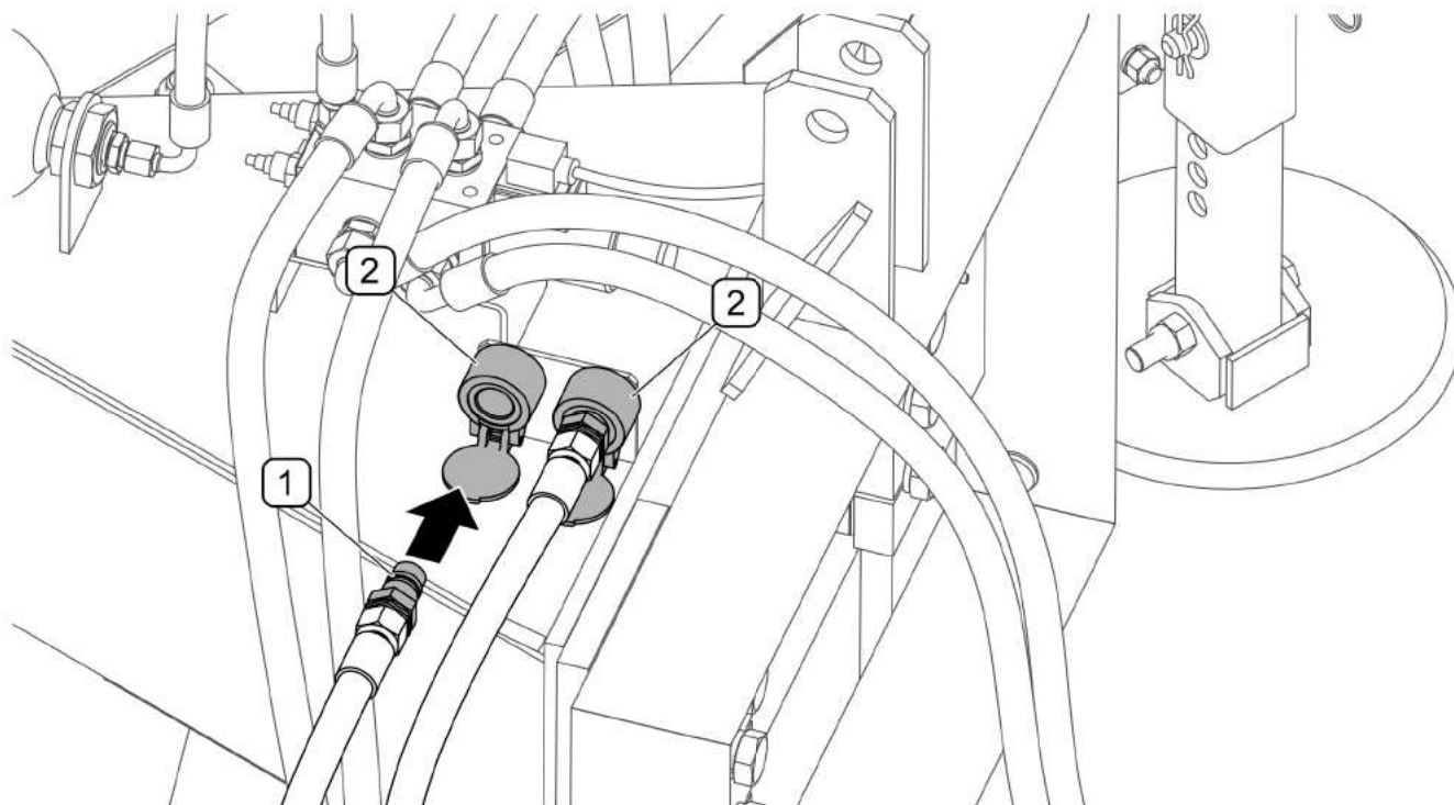
RYSUNEK 4.11 Zabezpieczenie wtyków gniazd hydraulicznych
