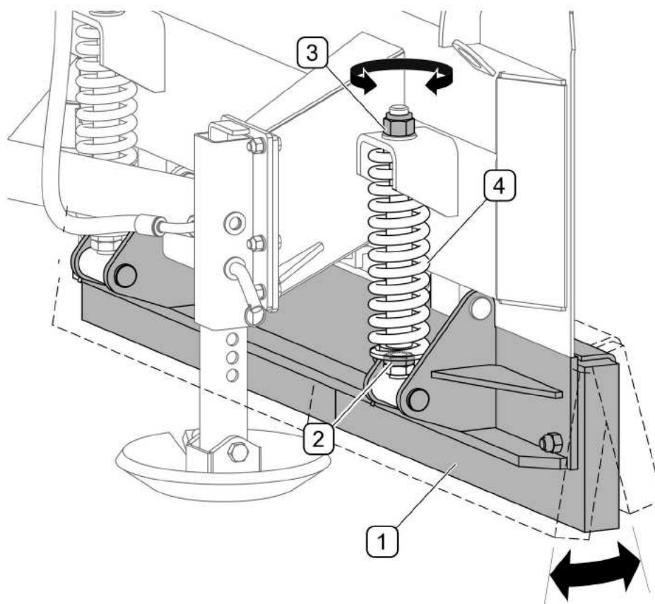
RYСУNEK 4.7 Ustawienie pochylenia listew zgarniających
