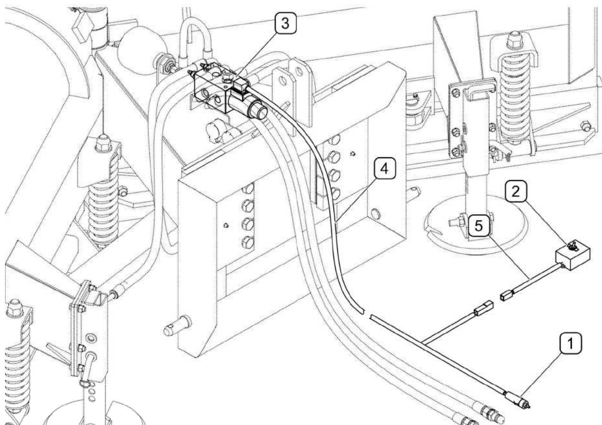
RYSUNEK 3.5 Budowa instalacji elektrycznej
