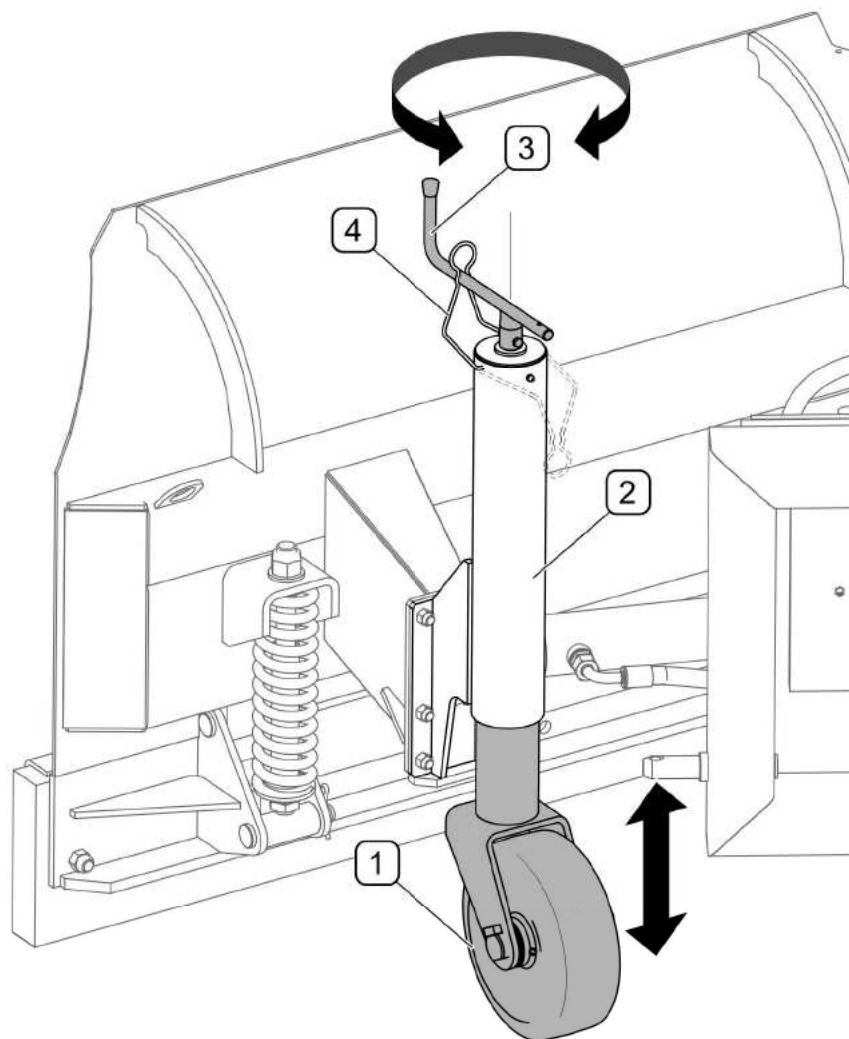
RYСУNEK 4.9 Regulacja wysokości pracy w pługach wyposażonych w kółka jezdne
