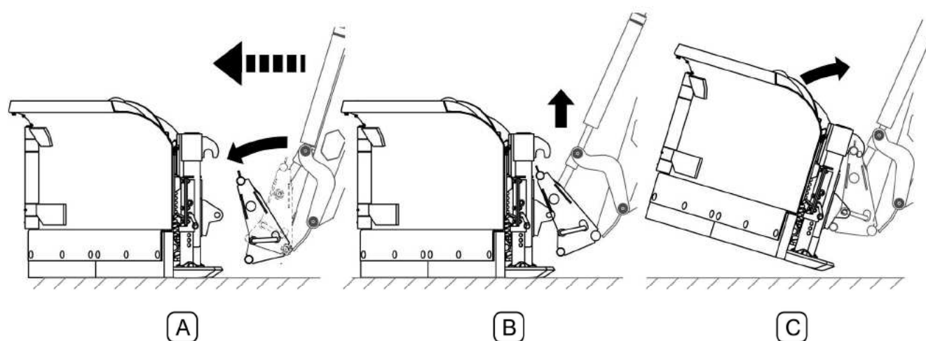
RYSUNEK 4.2 Łączenie z ładowaczem czołowym
