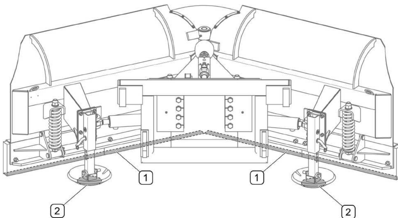
RYСУNEK 4.10 Pozycja pługa po odłączeniu od nośnika
