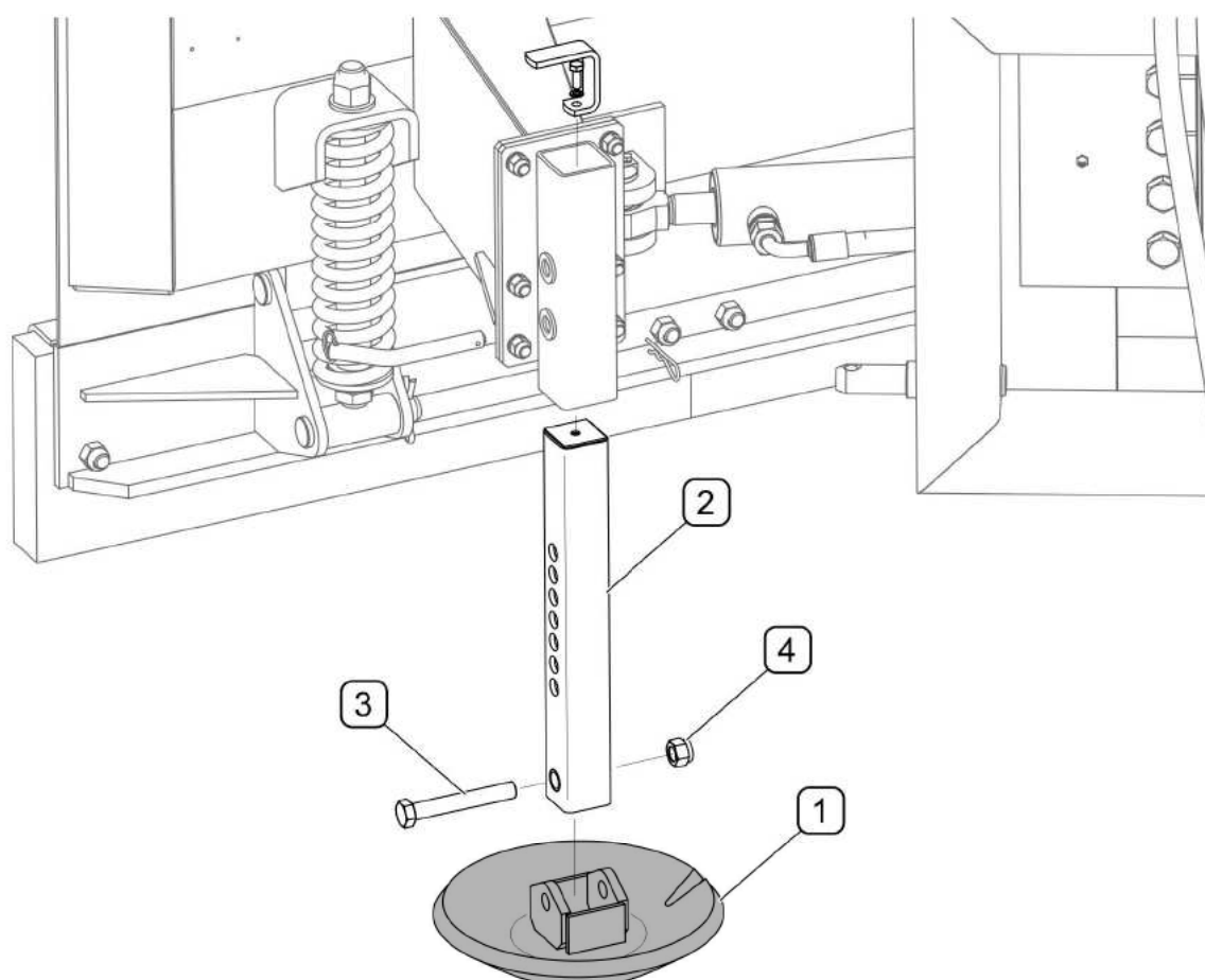
RYSUNEK 5.2 Wymiana ślizgu
