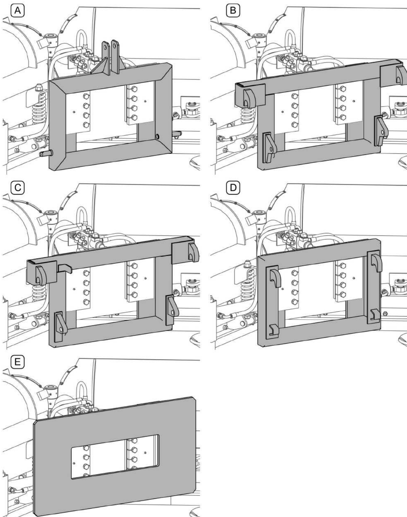
RYСУNEK 4.1 Rodzaje układów zawieszenia
