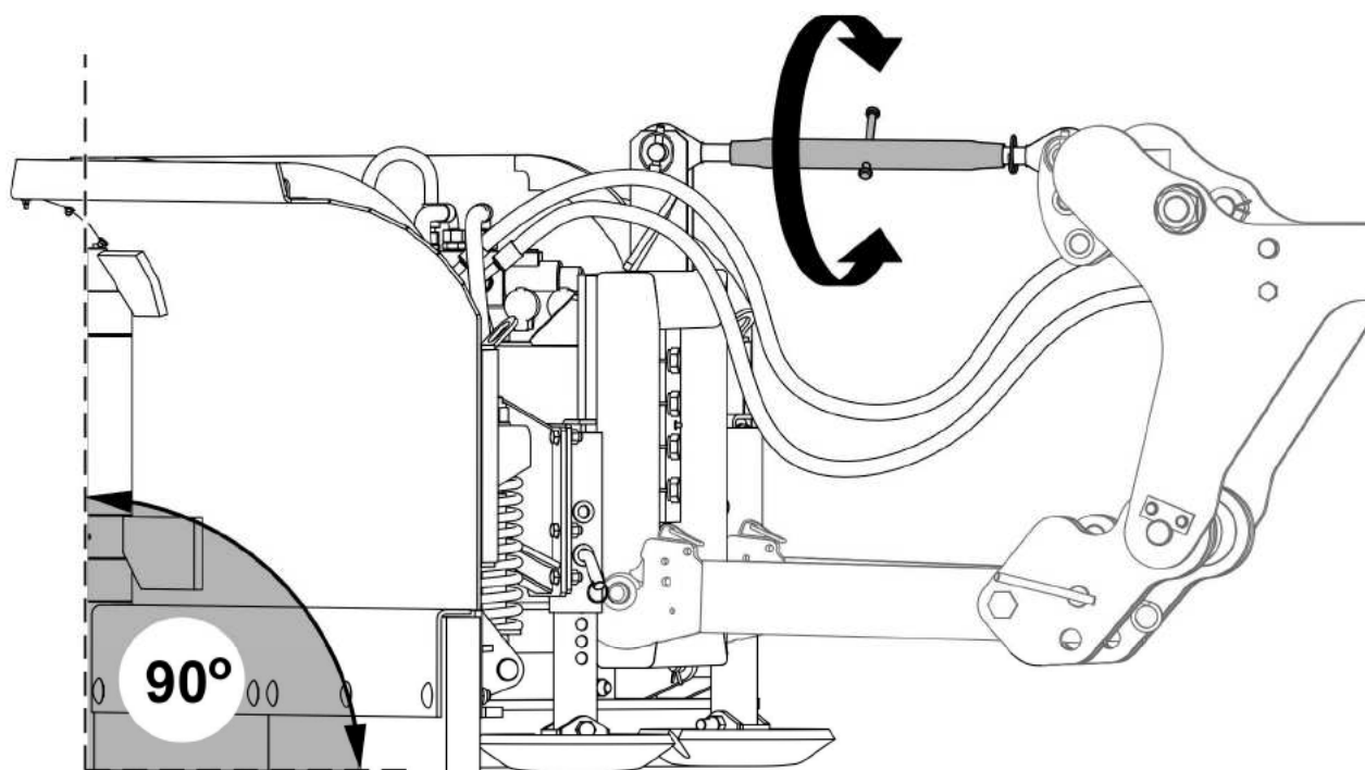
RYSUNEK 4.5 Poziomowanie korpusu pługa
