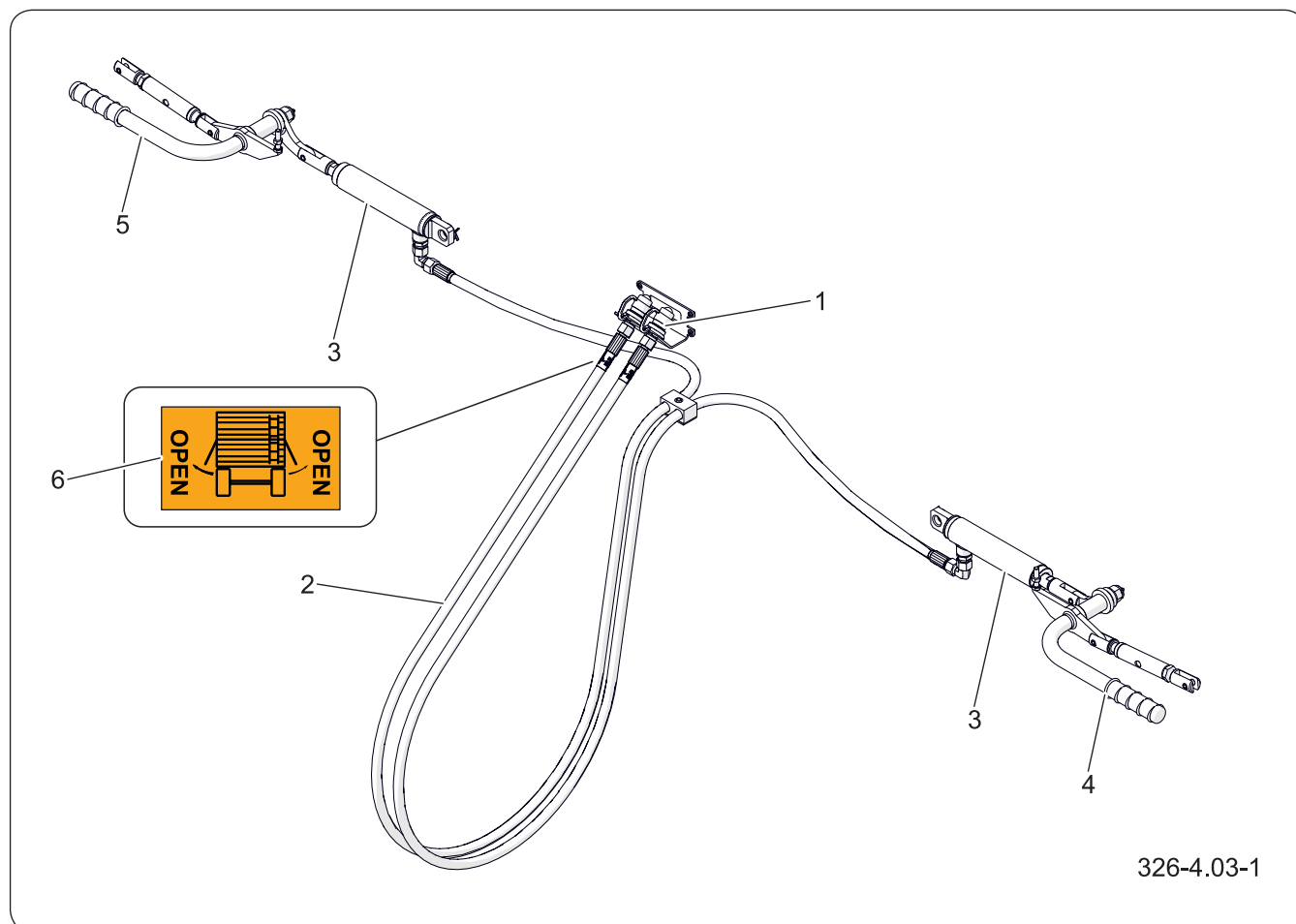
Rysunek 4.12 Budowa instalacji hydraulicznej rygłowania ścian bocznych.
