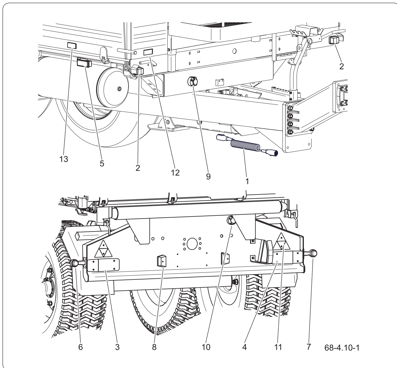
Rysunek 4.14 Rozmieszczenie elementów instalacji elektrycznej oraz elementów odblaskowych
