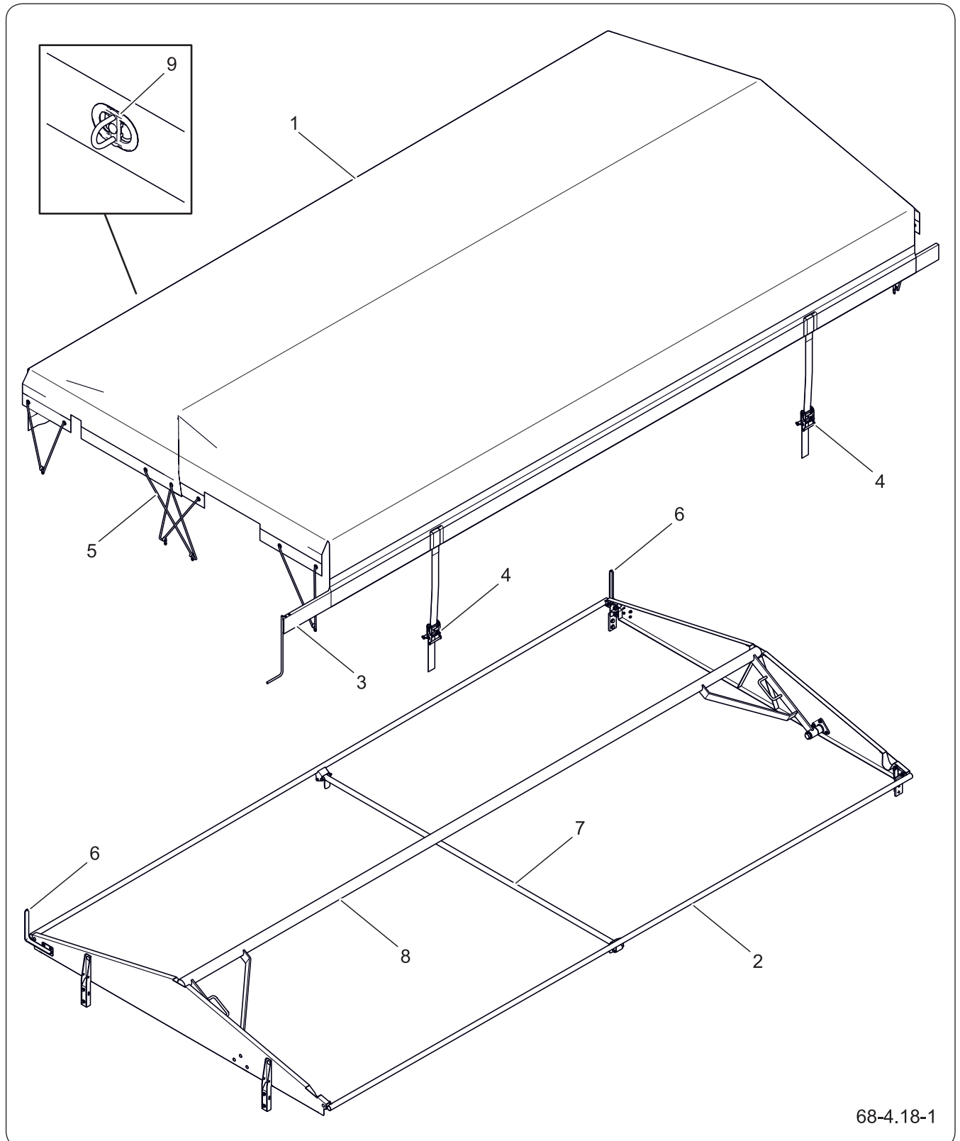
Rysunek 4.2 Budowa plandeki
