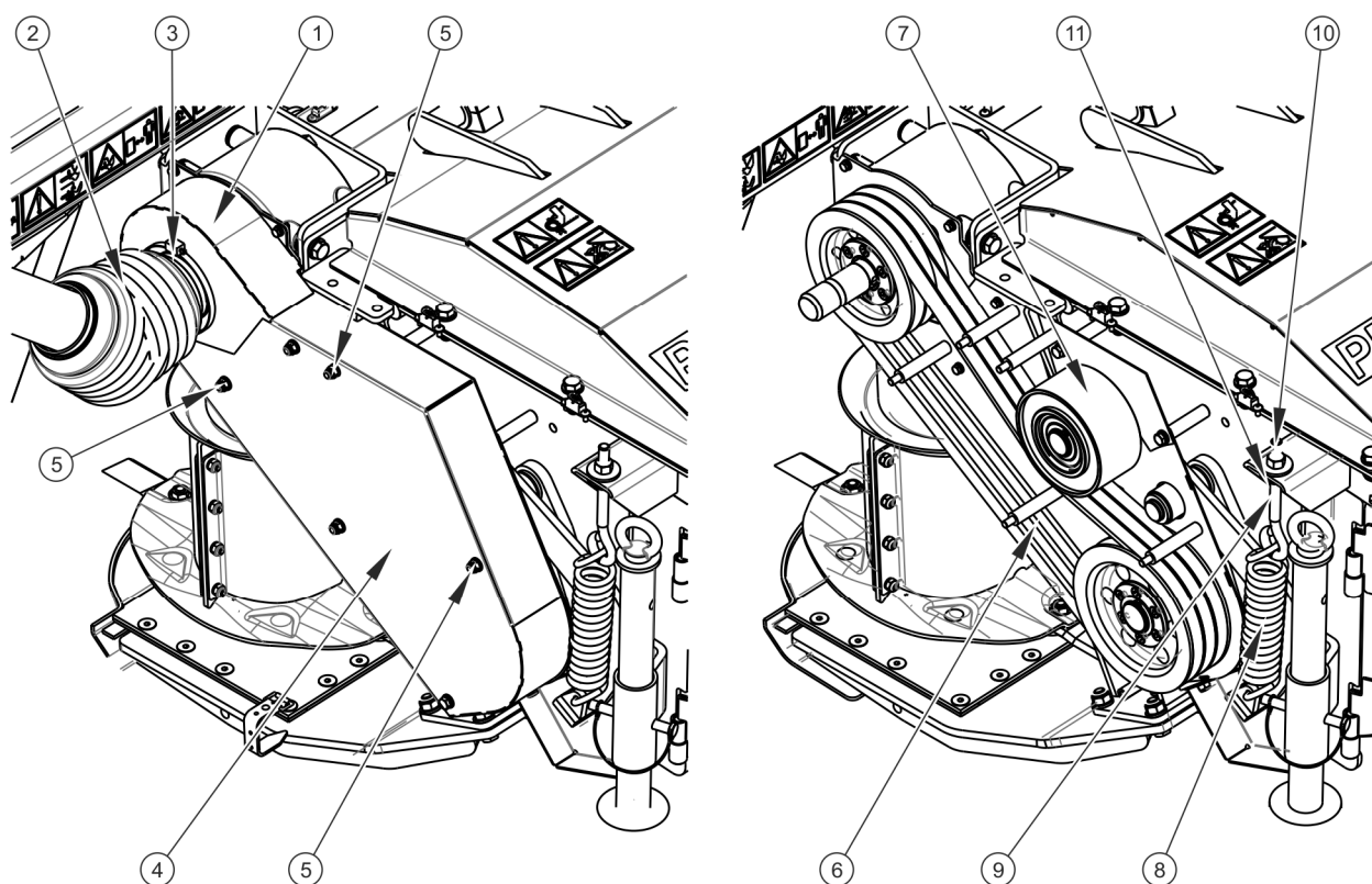
RYSUNEK 5.7 Regulacja napięcia przekładni pasowej kosiarek ze spulchniaczem
