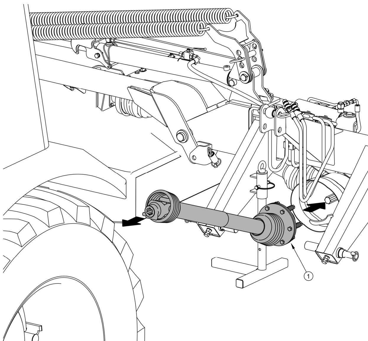
RYСУNEK 4.8 Podłączenie wału przegubowo teleskopowego
