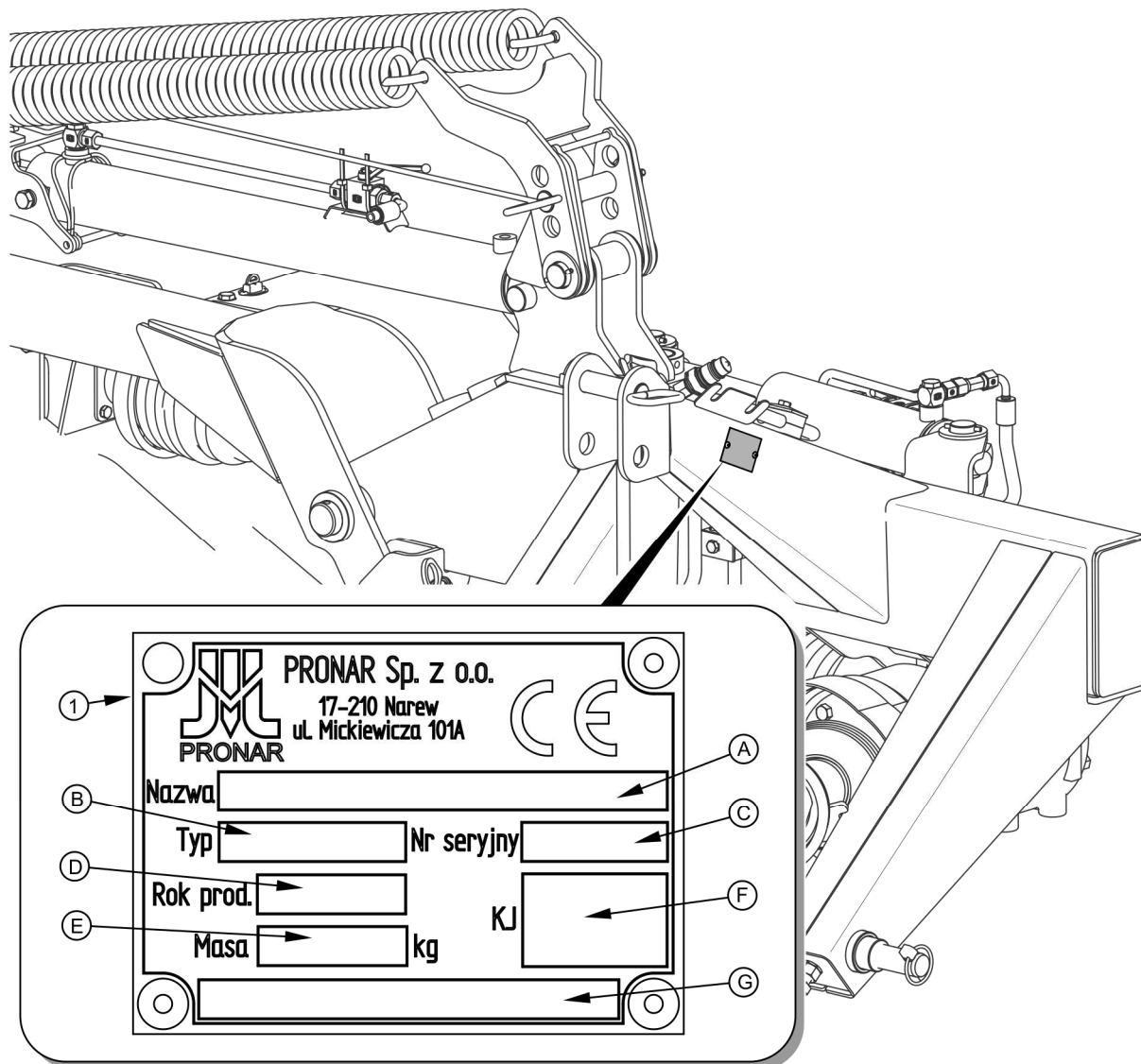
RYSUNEK 1.1 Miejsce umieszczenia tabliczki znamionowej
