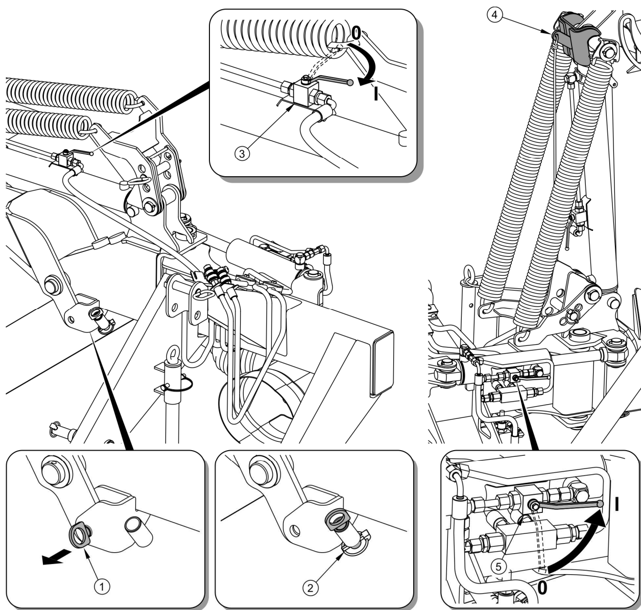
RYСУNEK 4.4 Ustawienie pozycji transportowej
