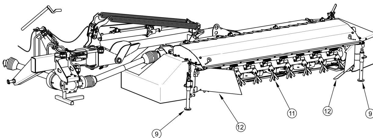
RYSUNEK 3.1 Budowa kosiarki
