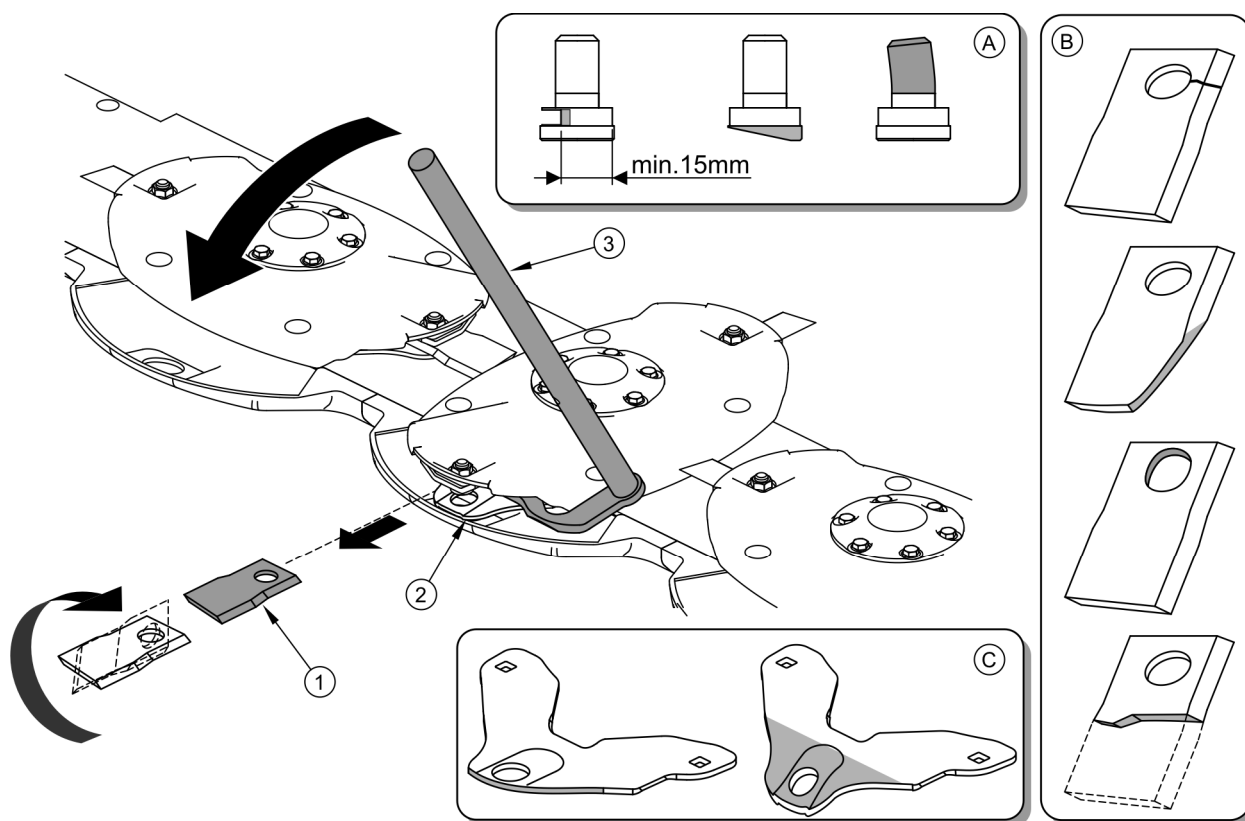
RYСУNEK 5.1 Wymiana noży listwy tnącej
