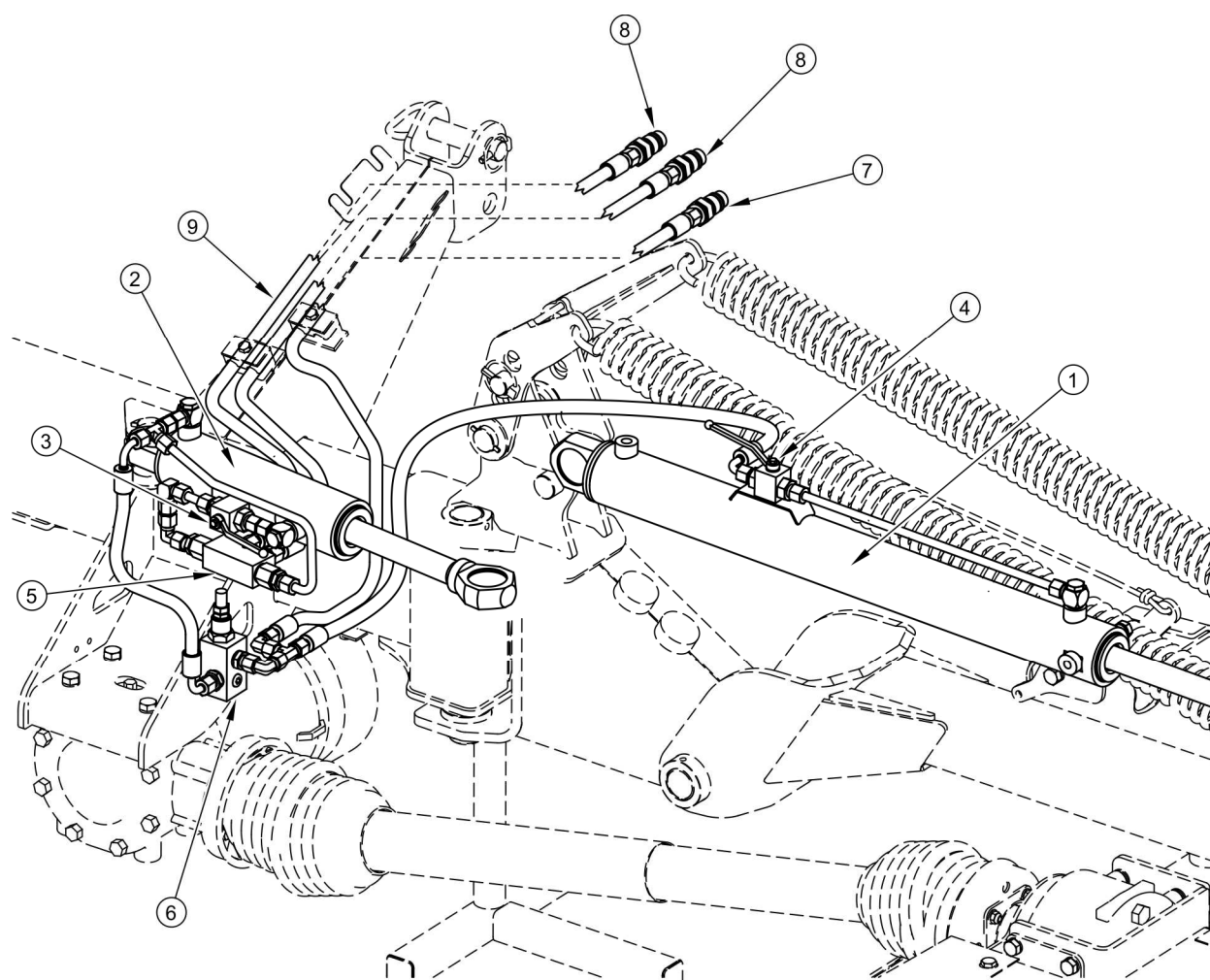
RYСУNEK 3.3 Budowa instalacji hydraulicznej
