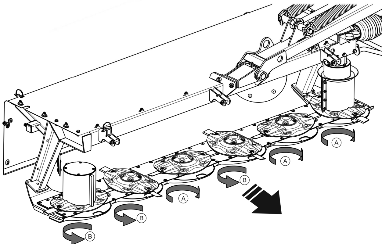
RYSUNEK 5.2 Rodzaje noży w zależności od kierunku obrotów dysków tnących
