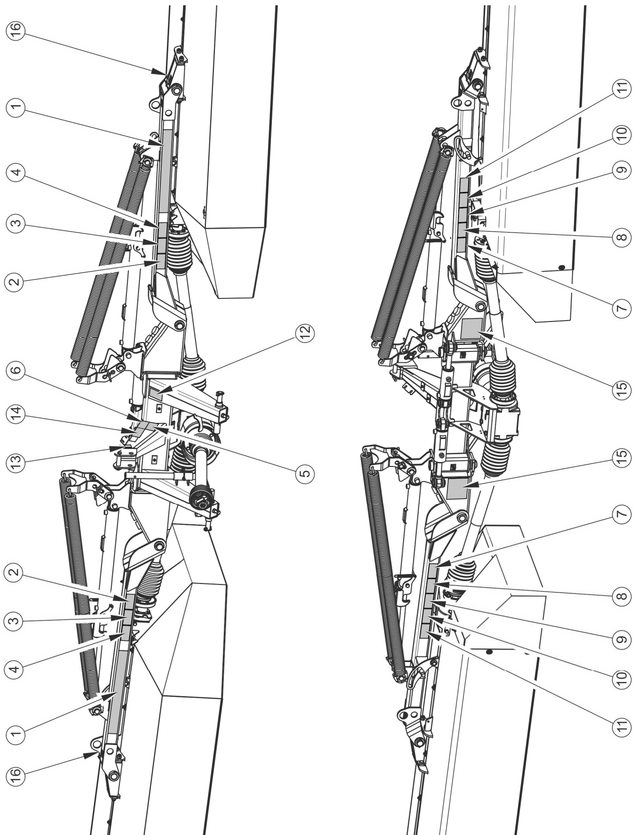
RYSUNEK 2.1 Rozmieszczenie naklejek informacyjnych i ostrzegawczych PDD830/ PDD830C
