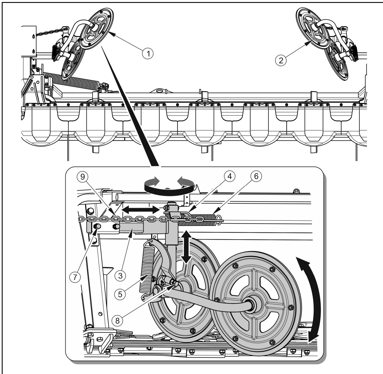
RYSUNEK 4.10 Ustawienie szerokości pokosu
