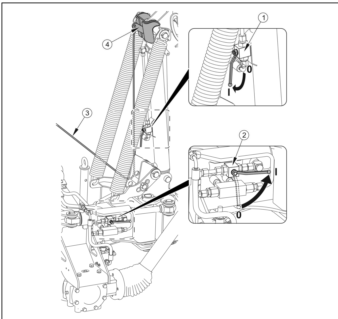
RYСУNEK 4.6 Ustawienie kosiarki do pozycji roboczej
