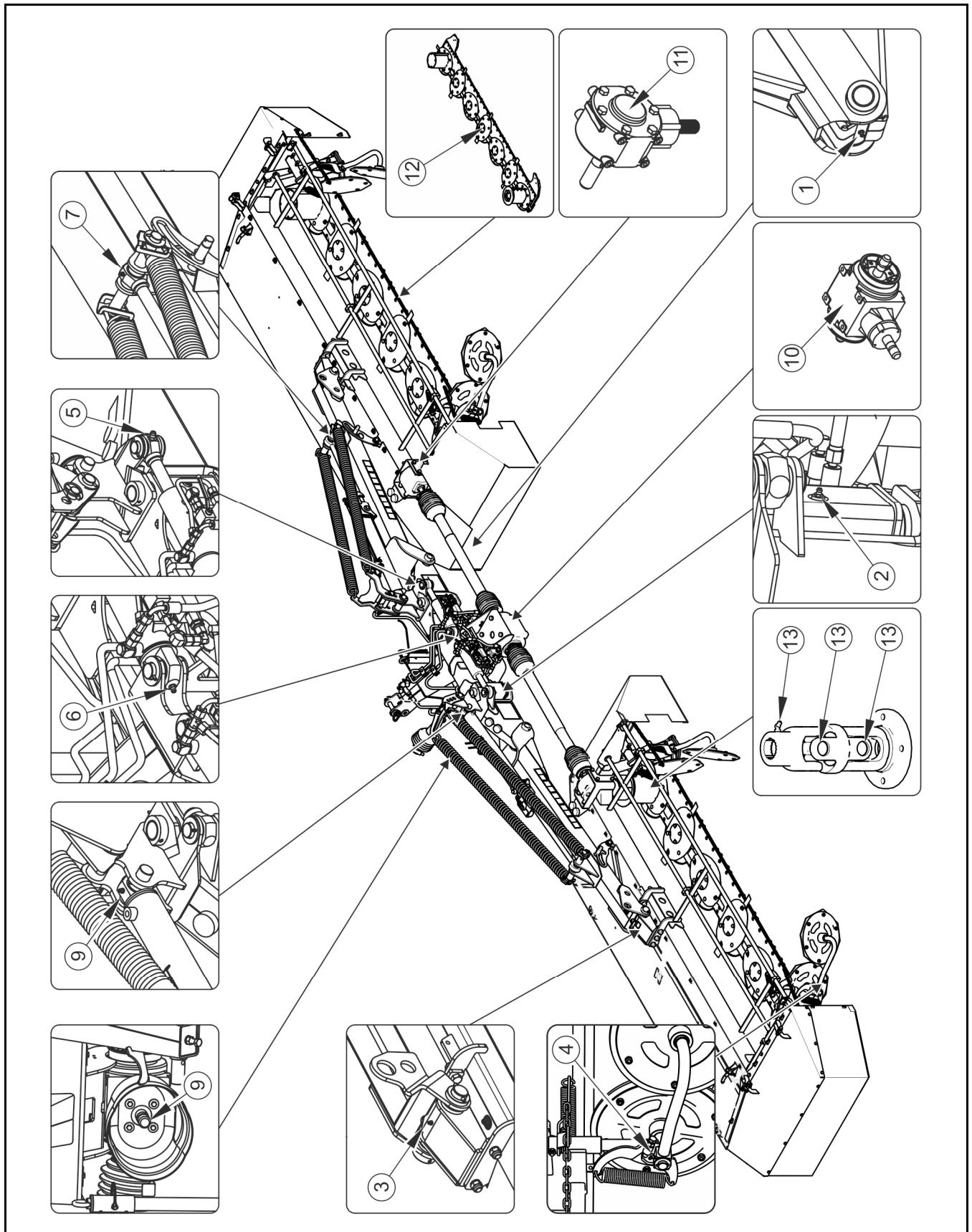
RYSUNEK 5.7 Punkty smarne kosiarki PDD830 / PDD830C
