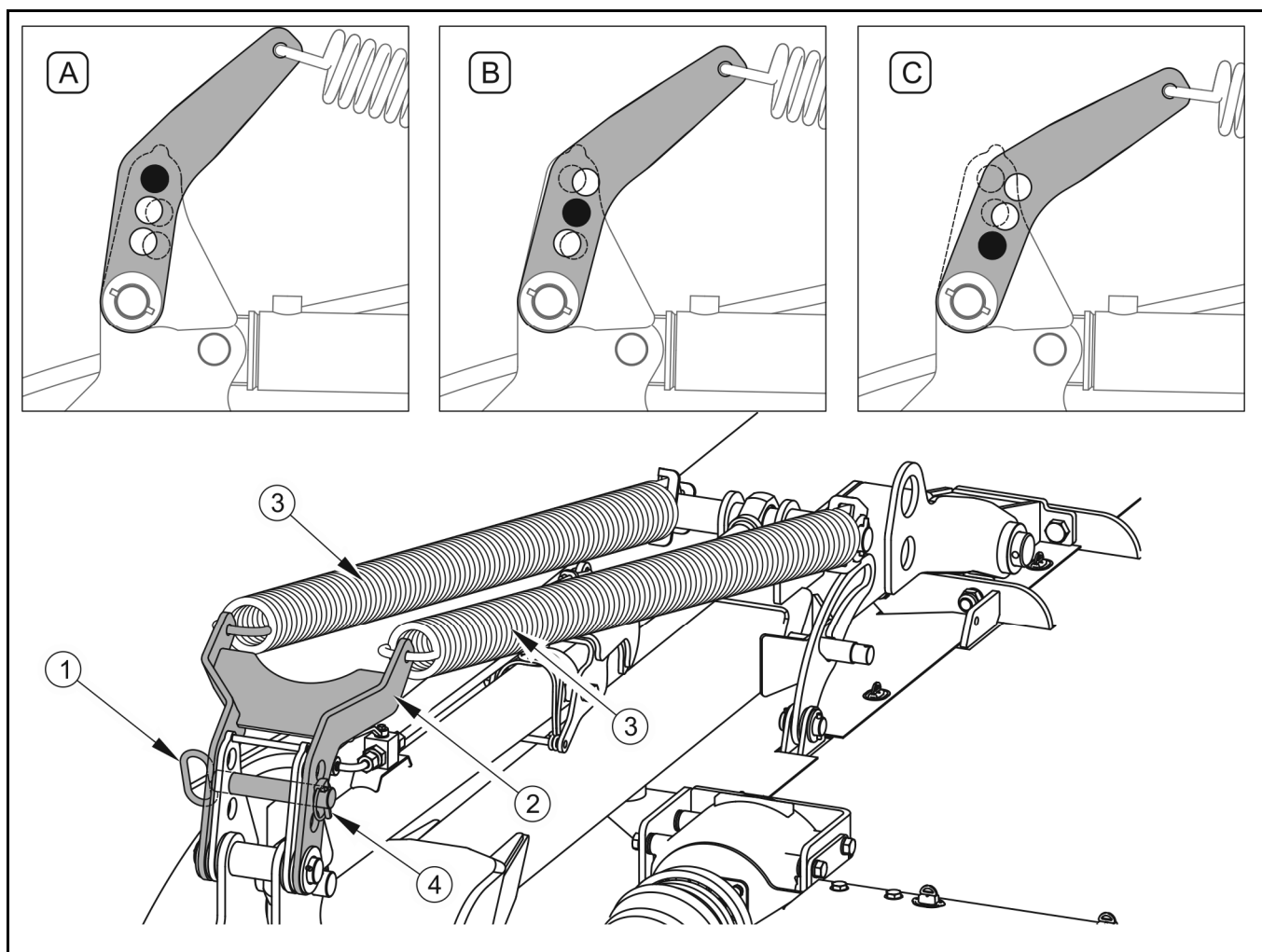
RYСУNEK 4.8 Regulacja nacisku listy tnącej
