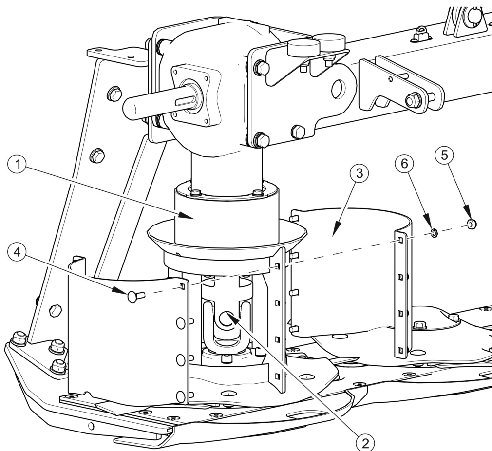
RYSUNEK 5.6 Czyszczenie i smarowanie dysku napędowego
