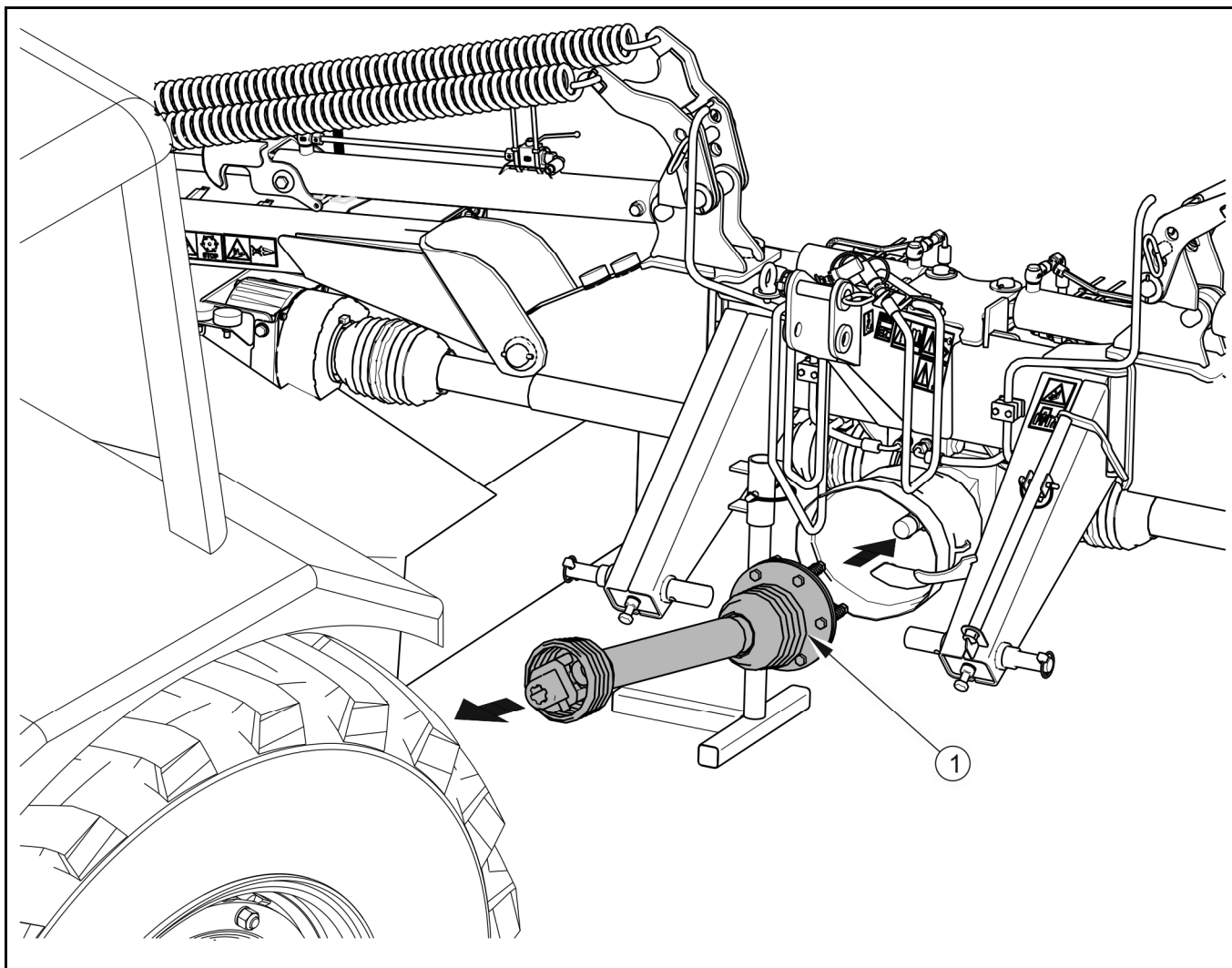
RYСУNEK 4.9 Podłączenie wału przegubowo-teleskopowego
