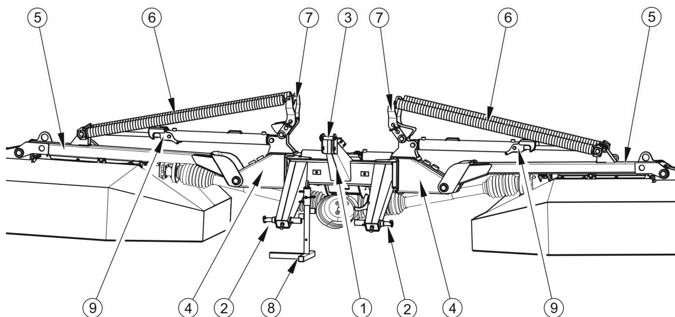
RYСУNEK 3.2 Układ zawieszenia
