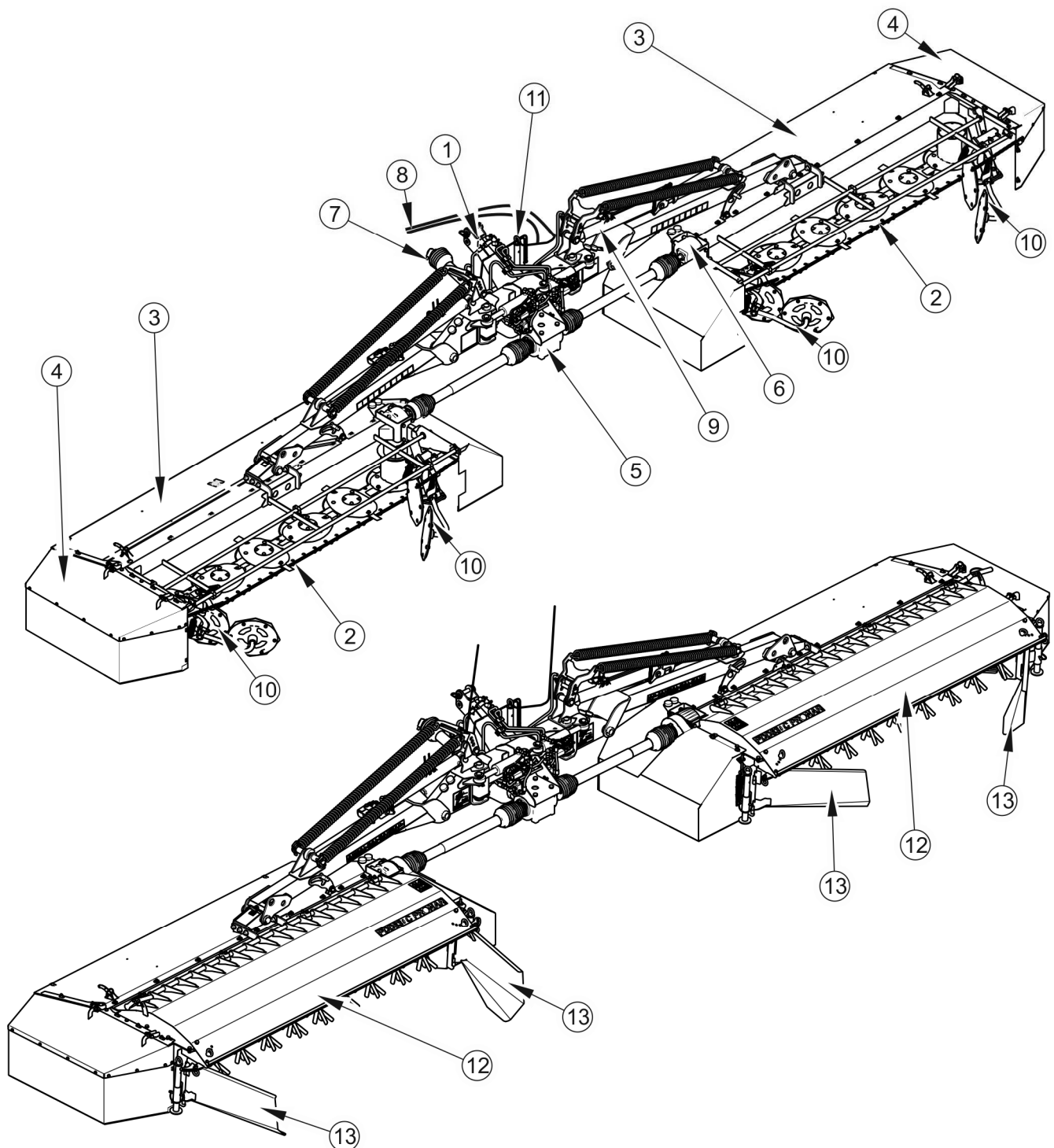
RYСУNEK 3.1 Budowa ogólna PDD830
