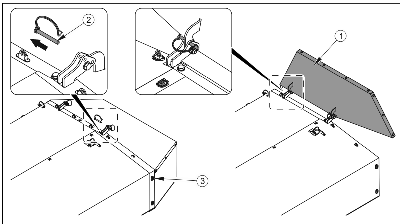
RYSUNEK 4.5 Podnoszenie osłon do transportu
