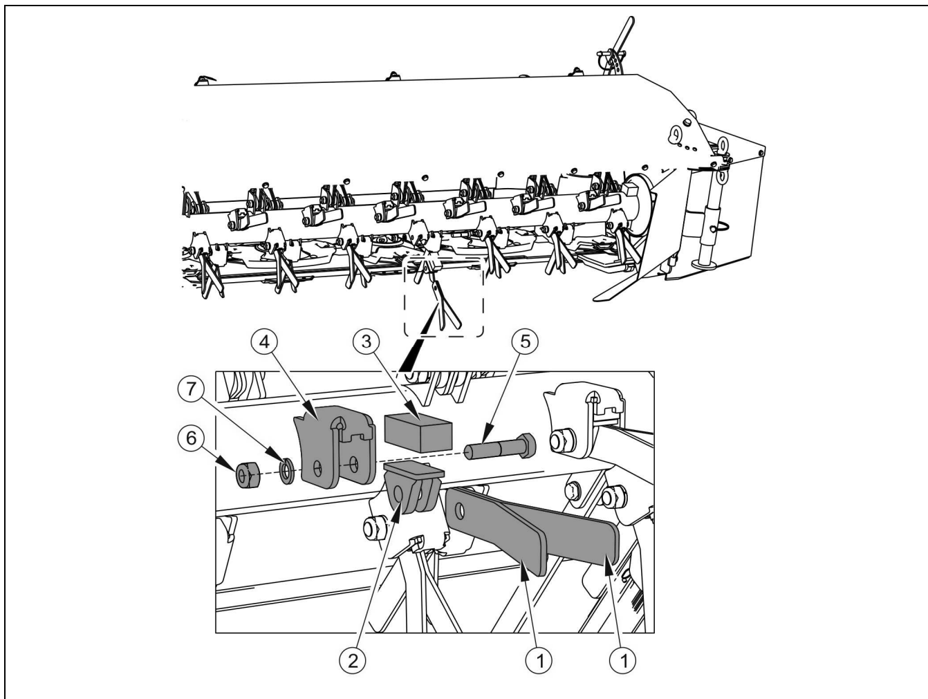
RYСУNEK 5.2 Wymiana noży bijakowych spulchniacza pokosów (PDD830C)
