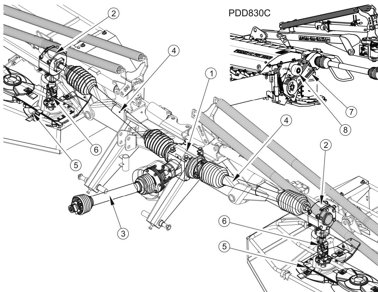
RYSUNEK 3.3 Mechanizm przeniesienia napędu
