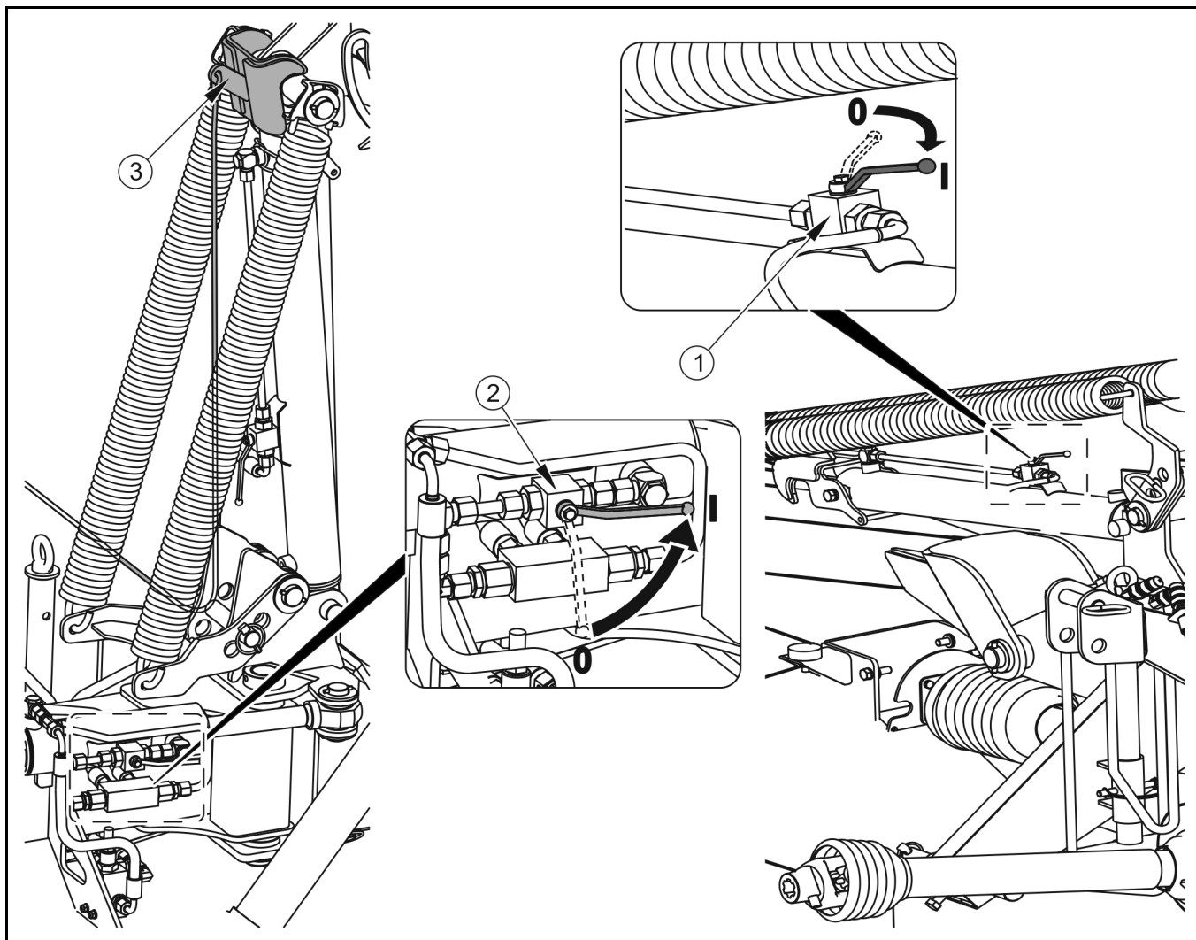
RYСУNEK 4.4 Ustawienie pozycji transportowej
