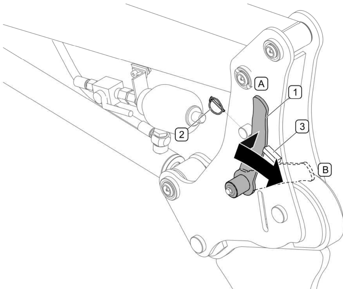
RYSUNEK 4.14 Odłączanie wysięgnika od ramy nośnej
