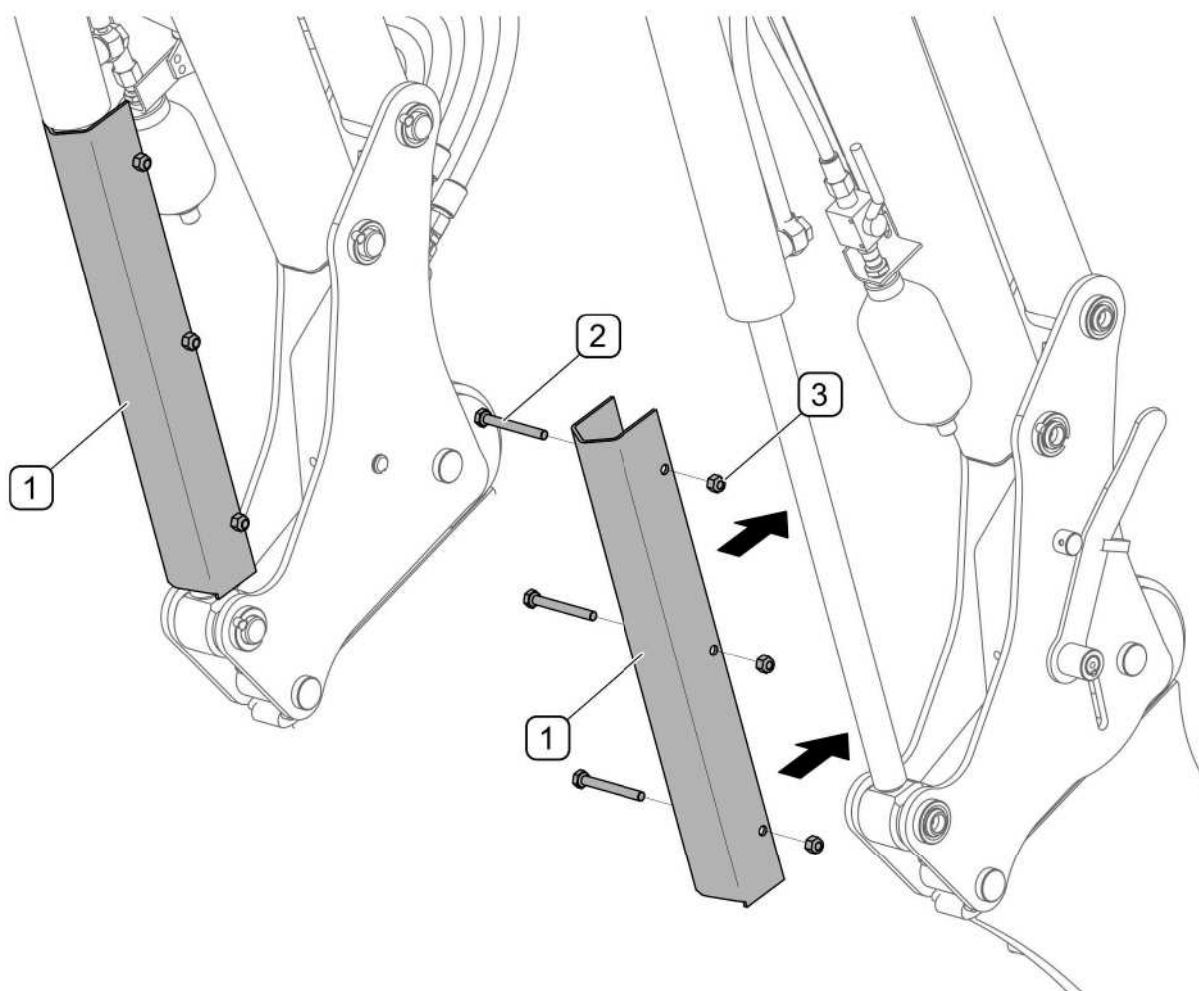
RYSUNEK 5.1 Blokady serwisowe
