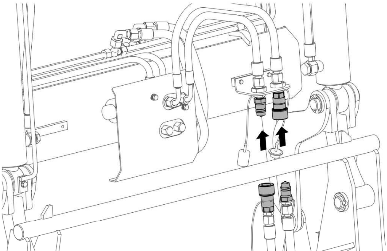
RYSUNEK 4.12 Podłączanie instalacji hydraulicznej osprzętu
