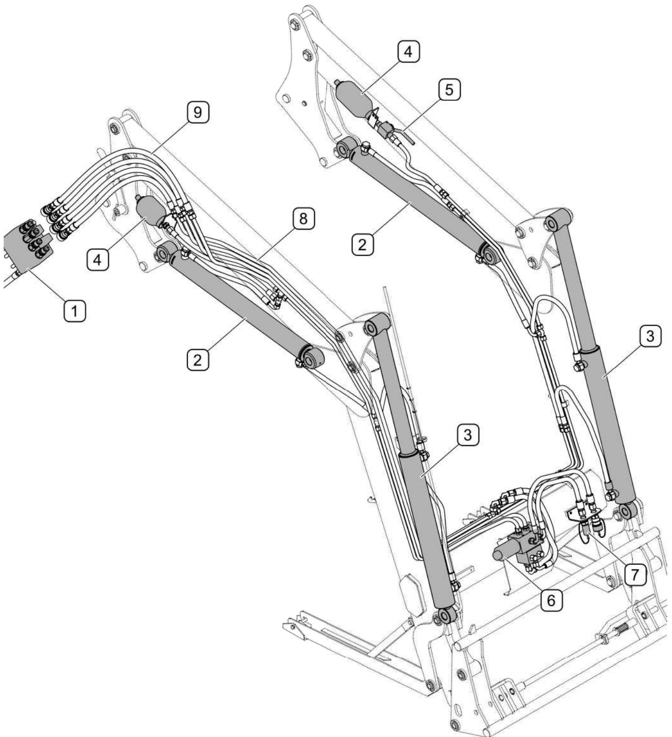
RYСУNEK 3.3 Budowa instalacji hydraulicznej
