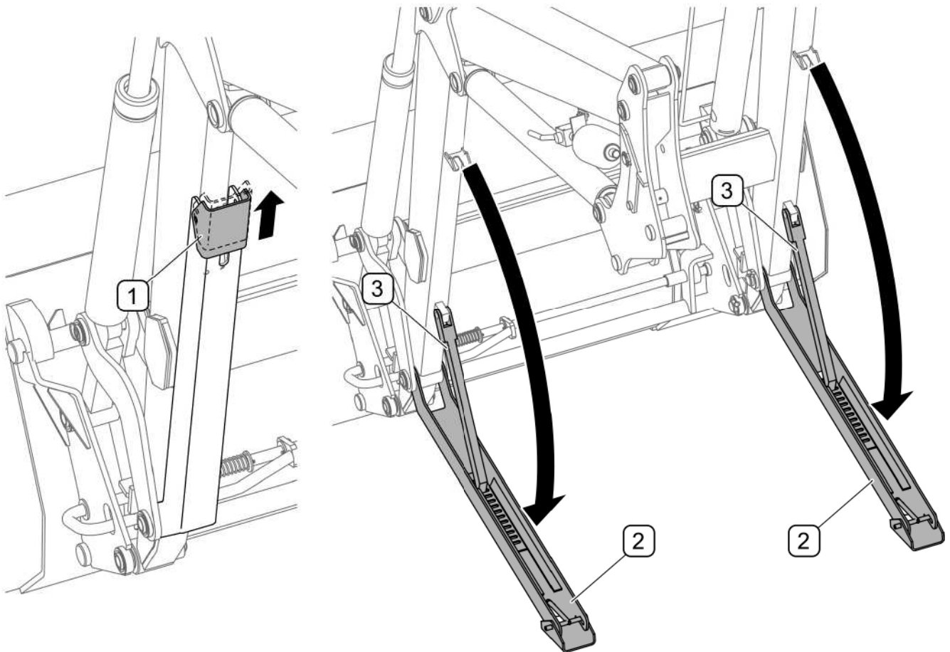
RYSUNEK 4.13 Podpory postojowe
