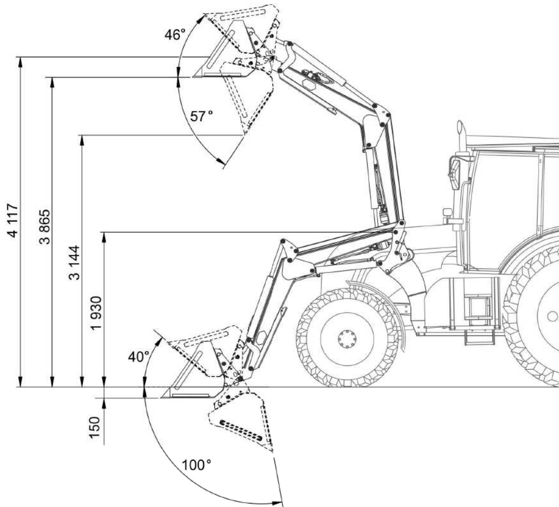
RYСУNEK 3.1 Zakres roboczy ładowacza LC4
