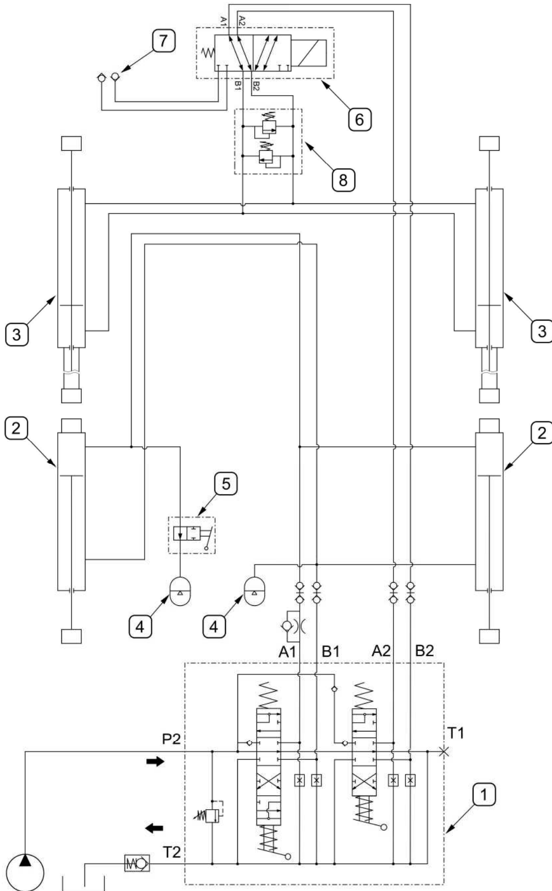
RYSUNEK 3.4 Schemat ideowy instalacji hydraulicznej ładowacza LC4
