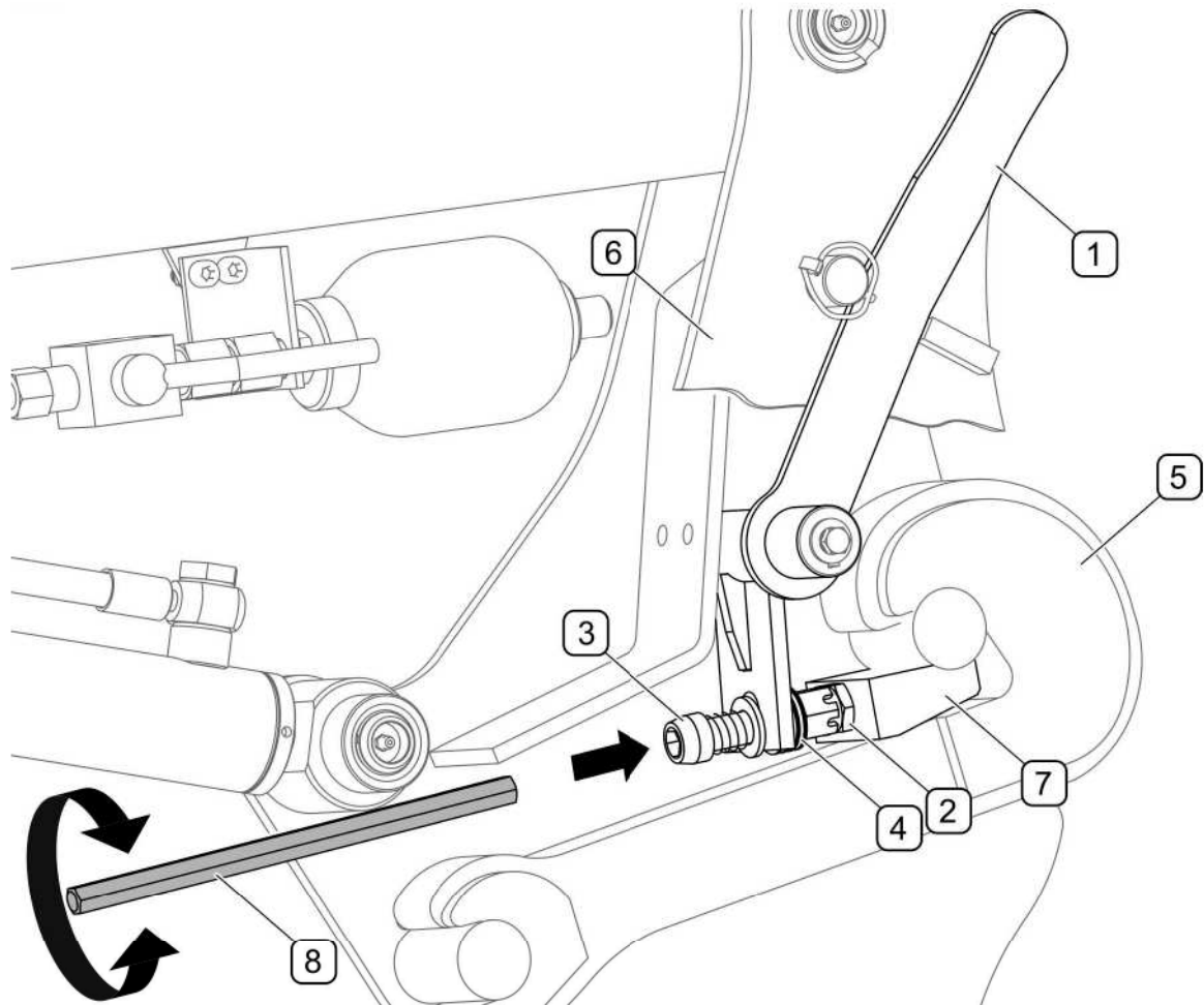
RYSUNEK 5.2 Regulacja zamków szybkosprzęgów
