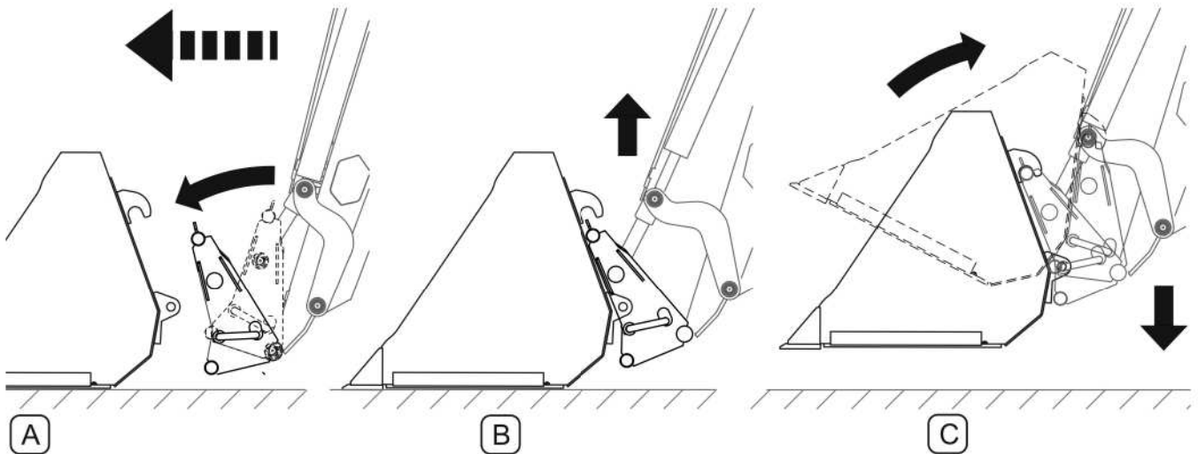
RYSUNEK 4.11 Montaż osprzętu roboczego
