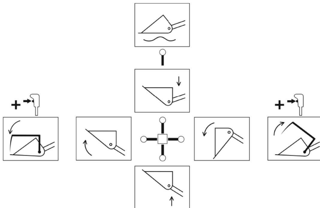
RYSUNEK 4.2 Schemat sterowania ładowaczem
