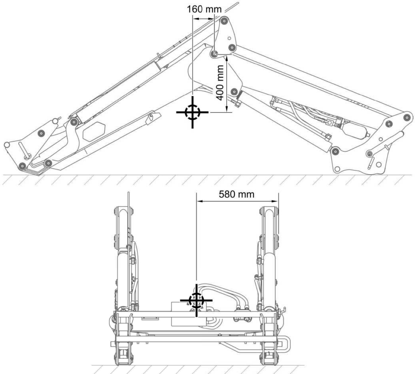
RYSUNEK 1.3 Położenie środka ciężkości wysięgnika ładowacza
