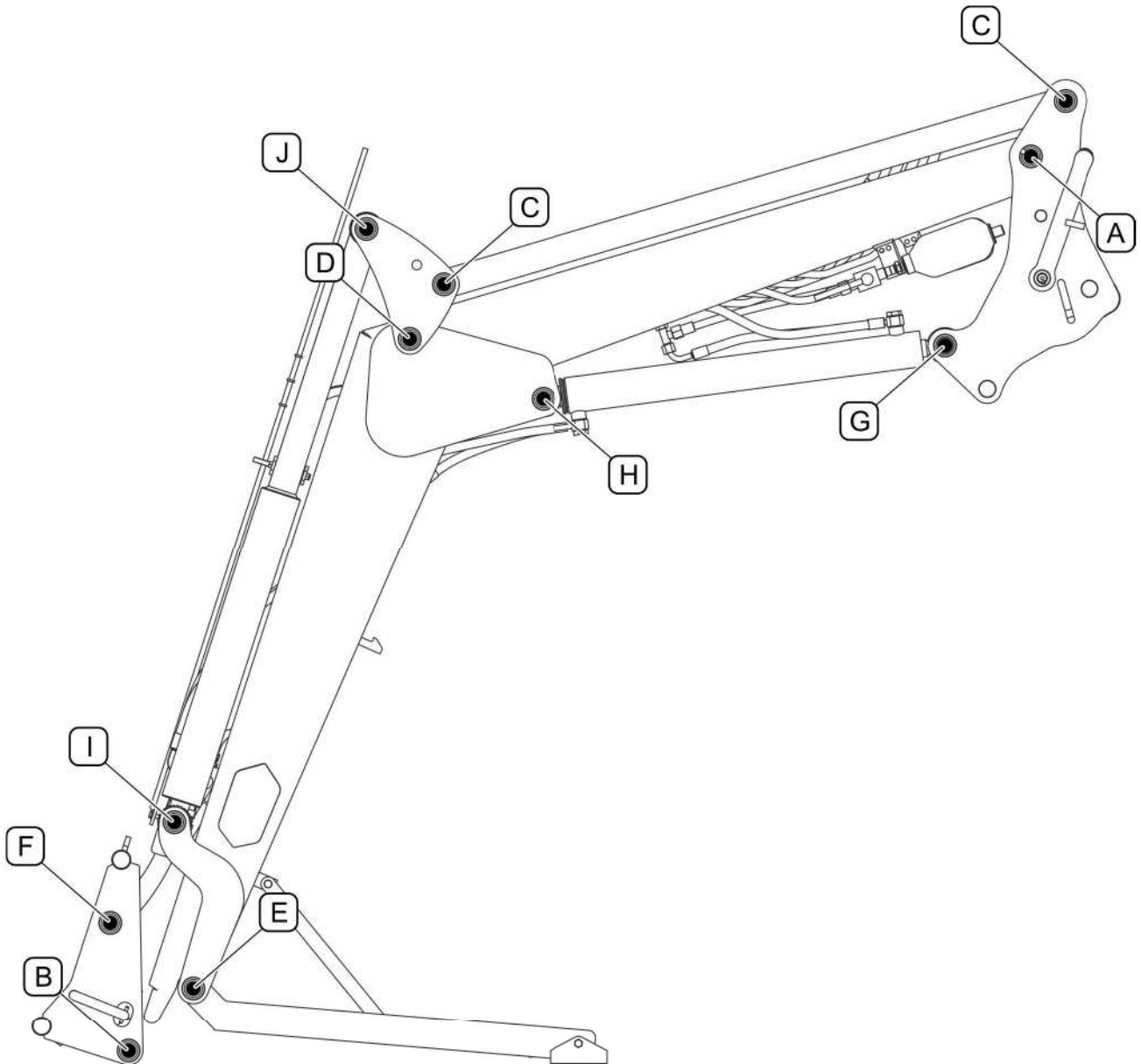
RYSunEK 5.4 Punkty smarowania
