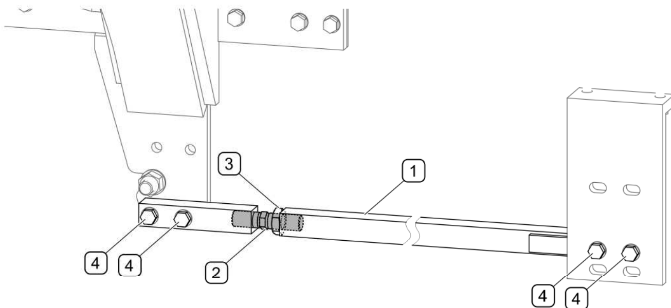
RYSUNEK 5.3 Napinanie podciągów rami nośnej ładowacza (w zależności od modelu ciągnika)
