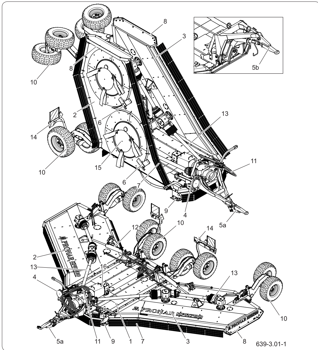
Рисунок 4.1 Конструкция машины
