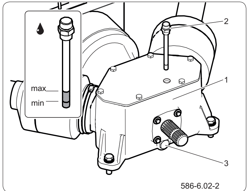
Рисунок 6.9 Проверка и замена масла в коробке передач
