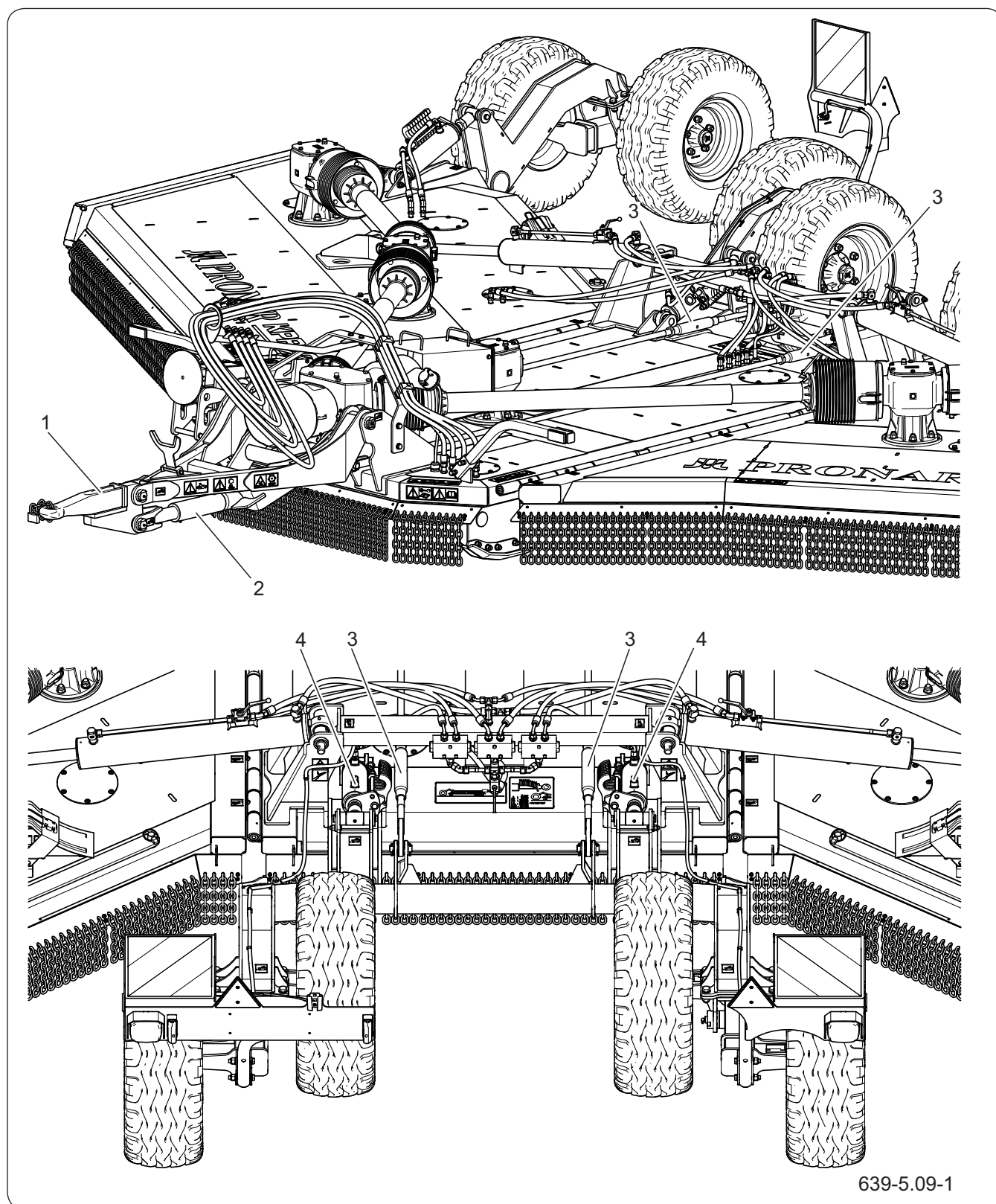
Рисунок 5.5 Регулировка положения машины
