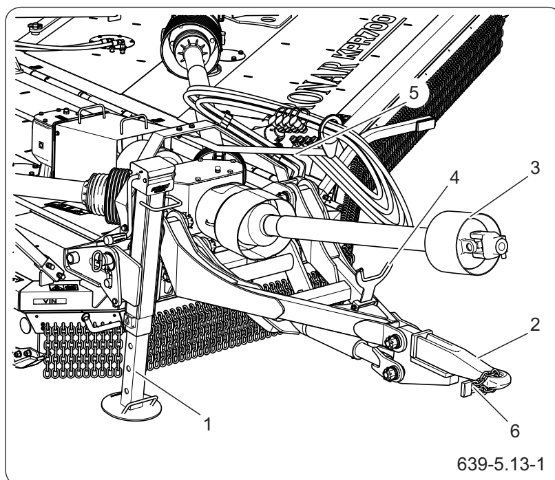
Рисунок 5.8 Подсоединение косилки к носителю (1) опорная ножка (2) нижняя сцепка (3) шарнирно-телескопический вал (ВПТ) (4) кронштейн ВПТ (5) кронштейн для проводов (6) предохранительное устройство
