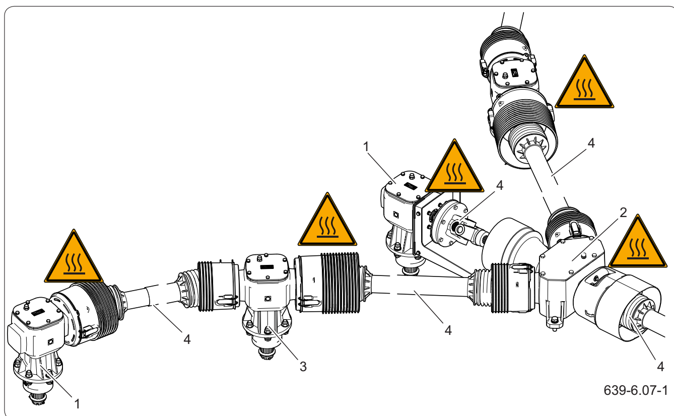
Рисунок 6.8 Проверка и замена масла в системе передачи привода
