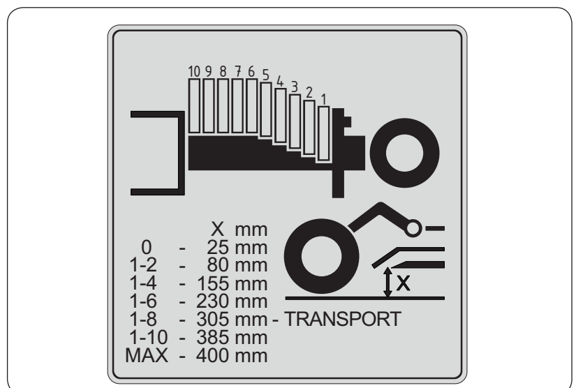
Рисунок 5.12 Высота среза
