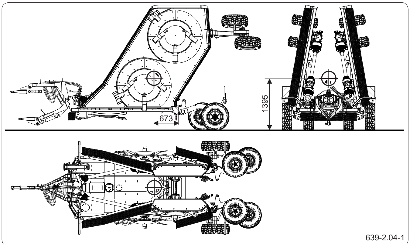
Рисунок 2.5 Расположение центра тяжести машины
