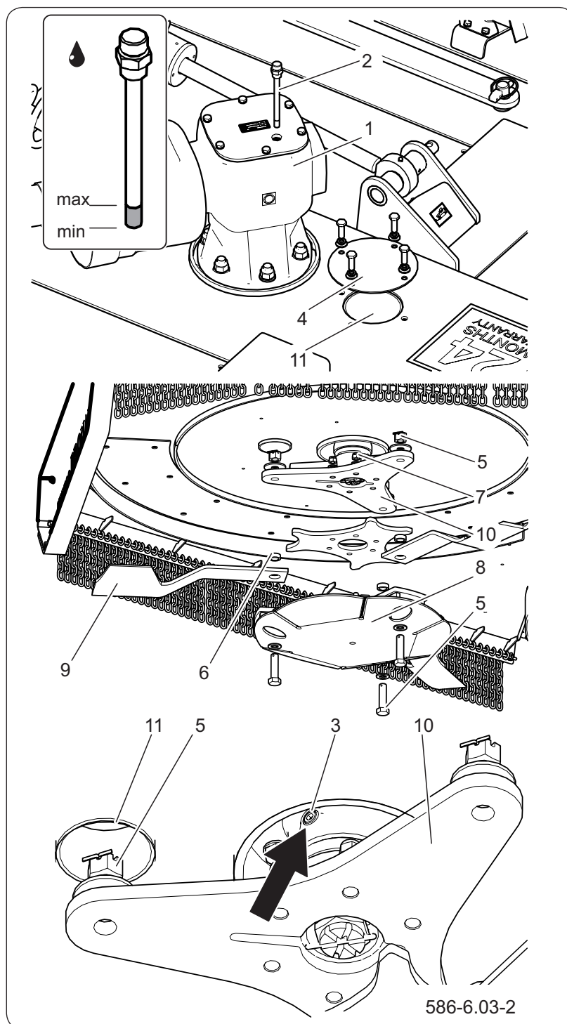
Рисунок 6.10 Проверка и замена масла в угловых передачах
