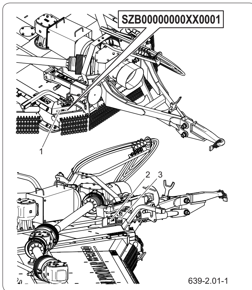
Рисунок 2.1 Идентификация машины
