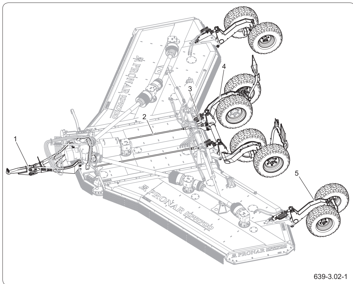
Рисунок 4.2 Конструкция системы подвески
