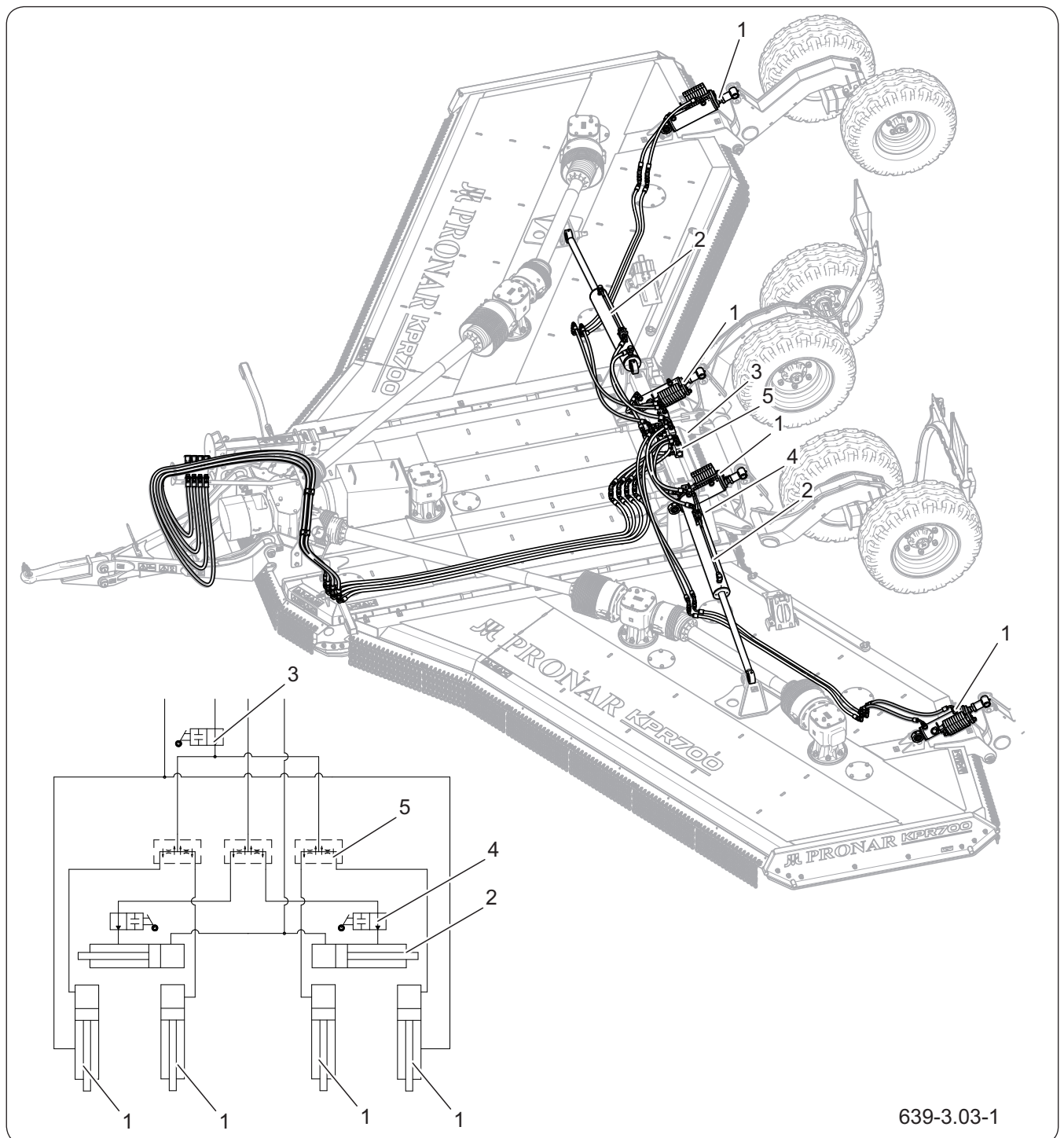
Рисунок 4.3 Конструкция гидравлической системы косилки KPR700
