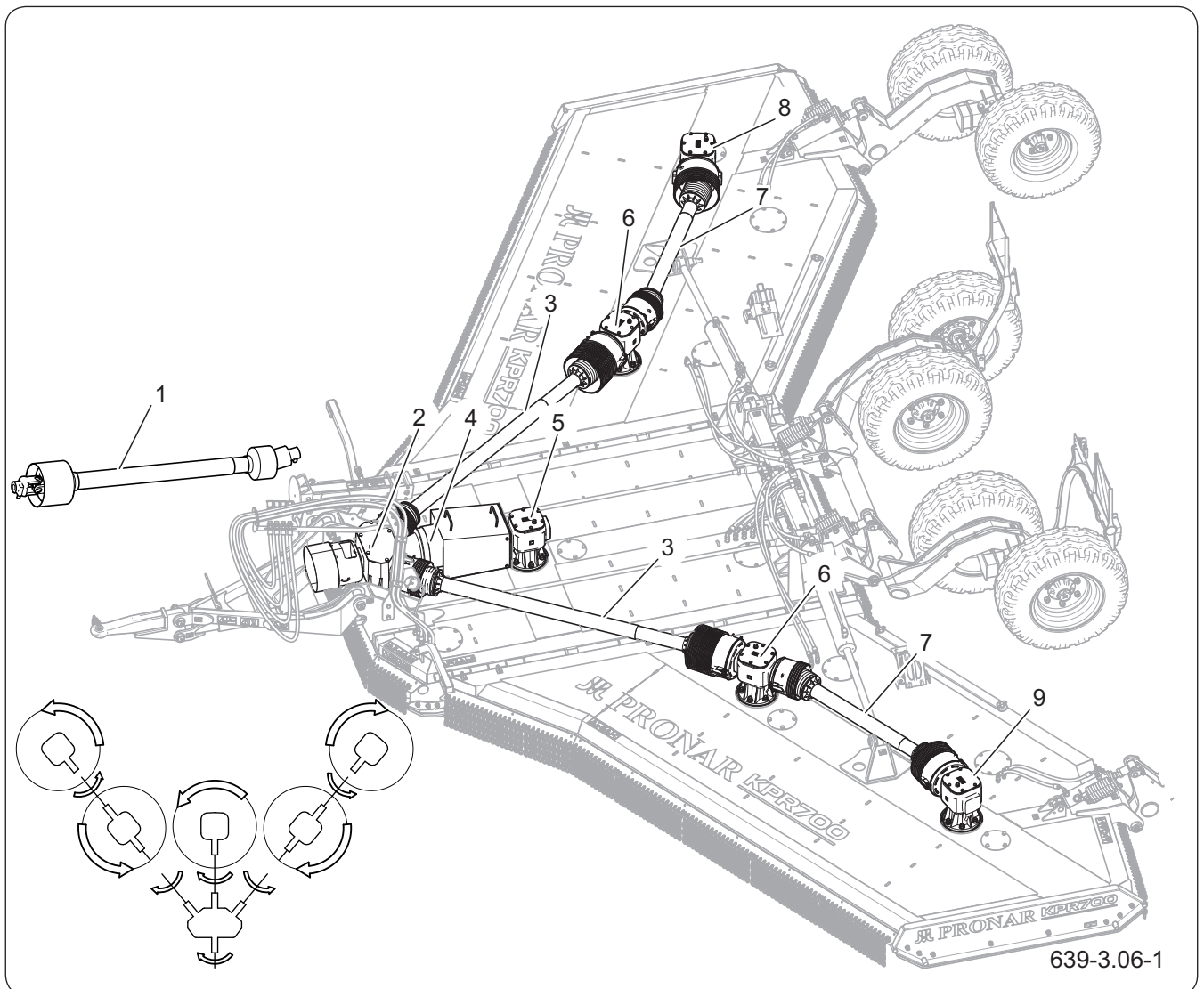
Рисунок 4.5 Конструкция приводной системы косилки KPR700
