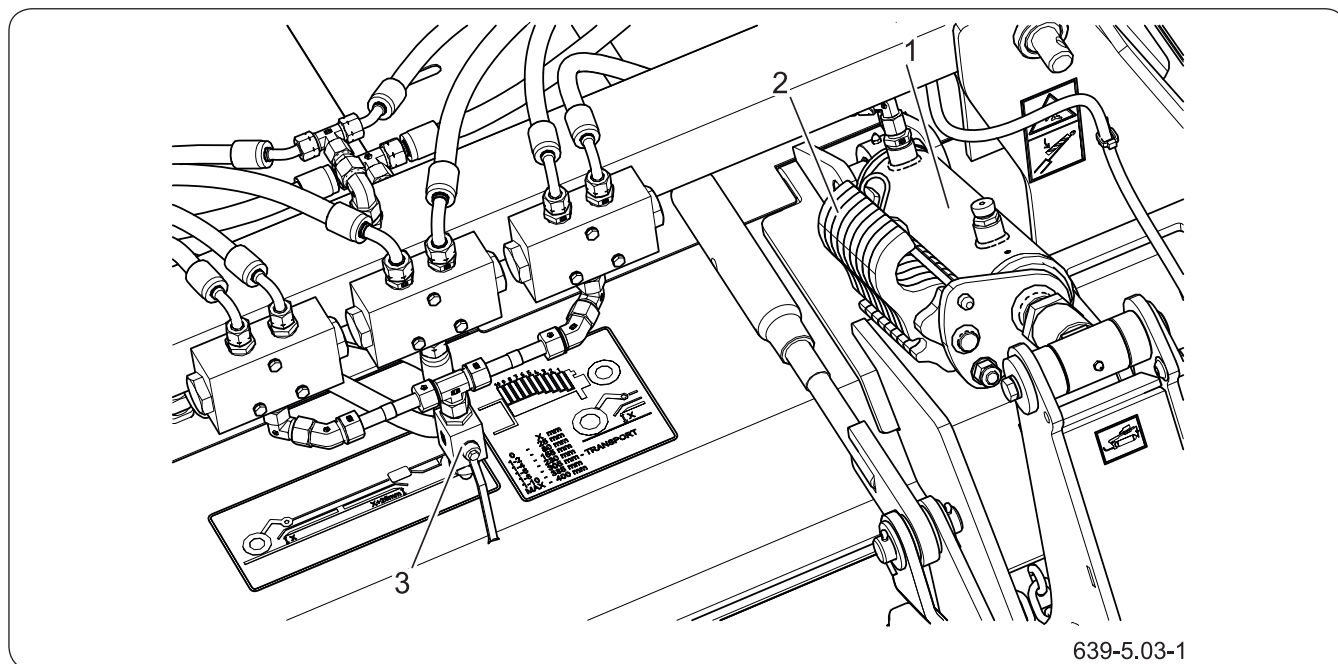
Рисунок 5.10 Транспортная блокировка II
