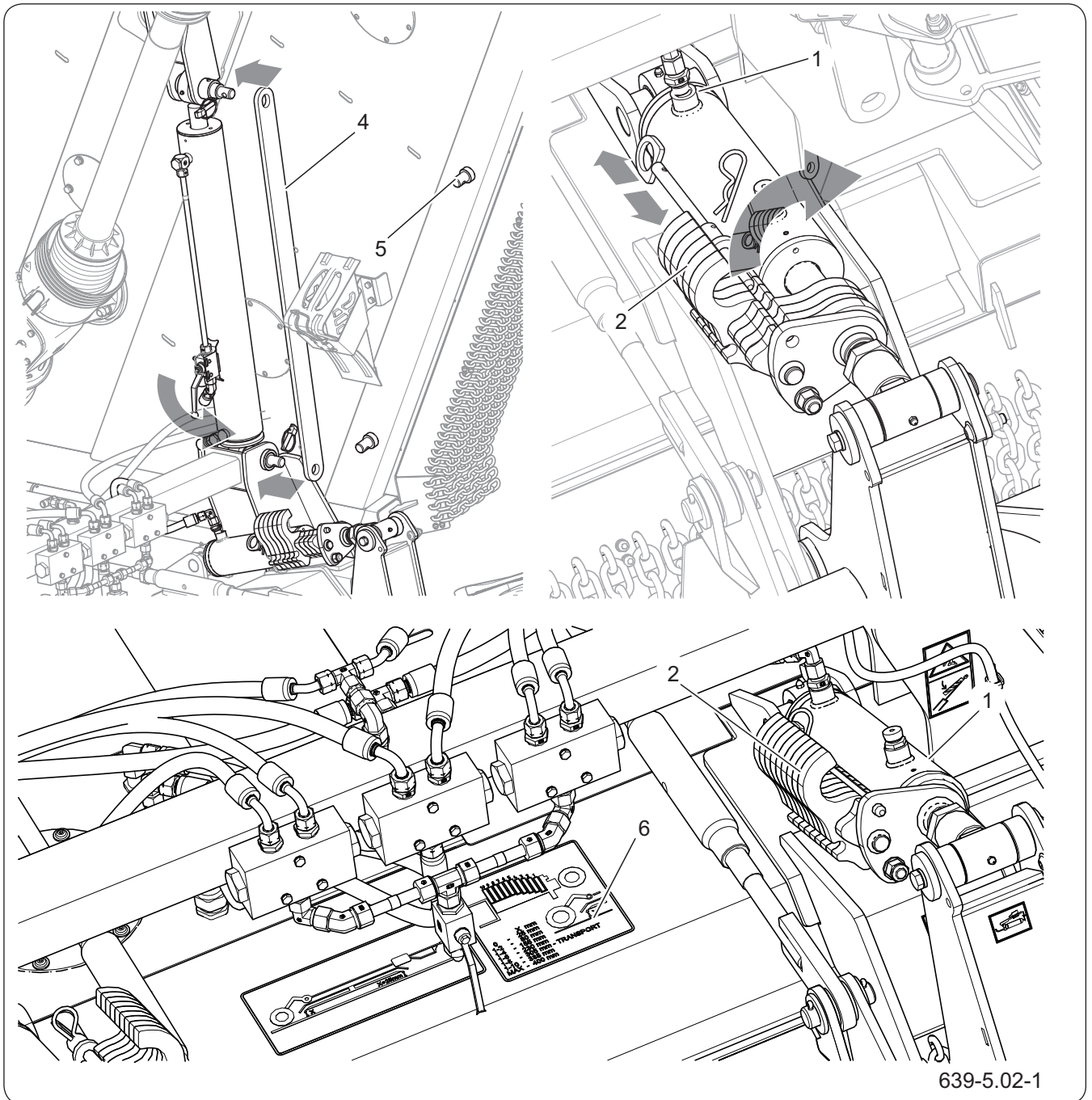
Рисунок 5.9 Транспортная блокировка
