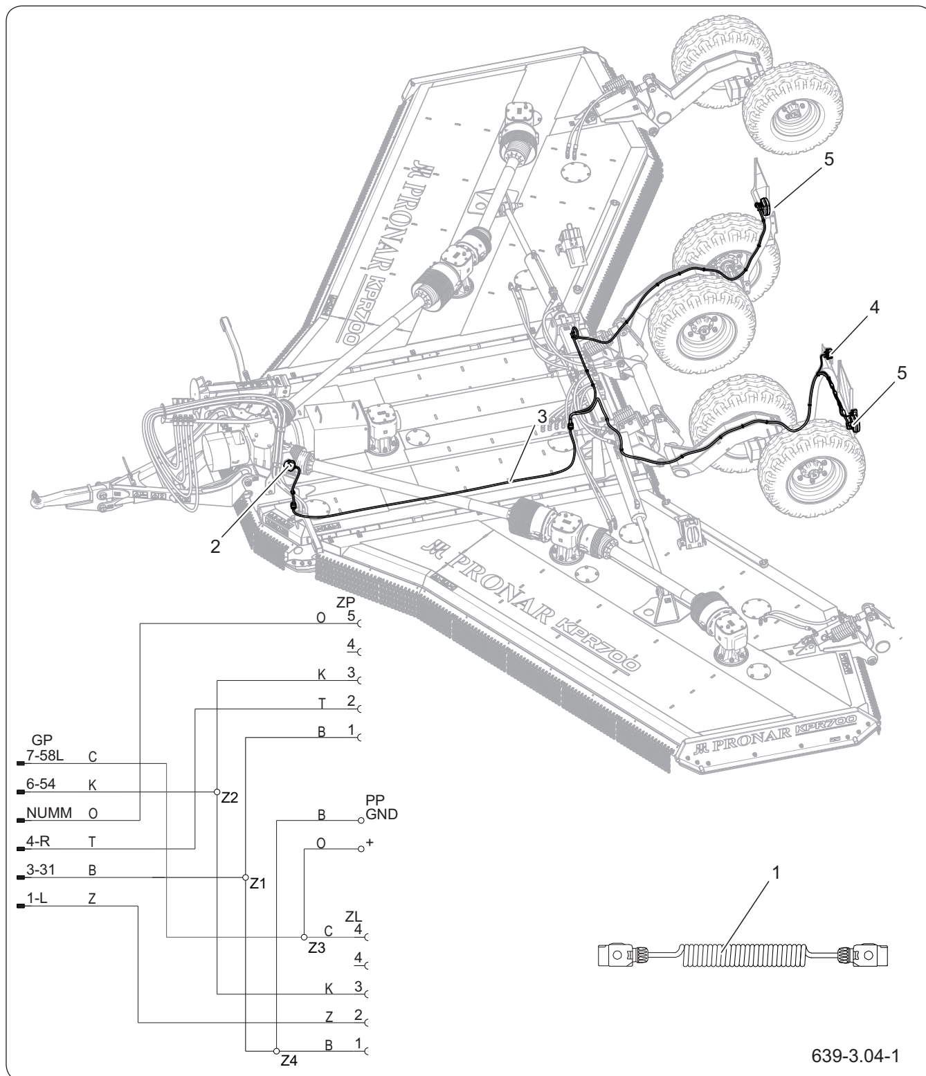
Рисунок 4.4 Конструкция электрической системы косилки KPR700
