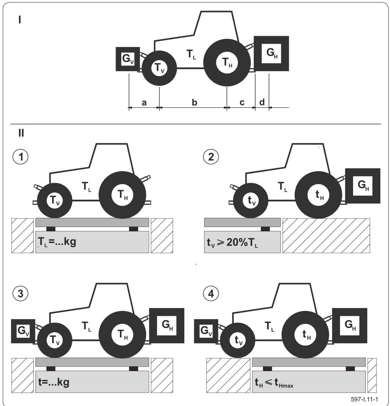
Рисунок 5.3 Утяжеление тягача
