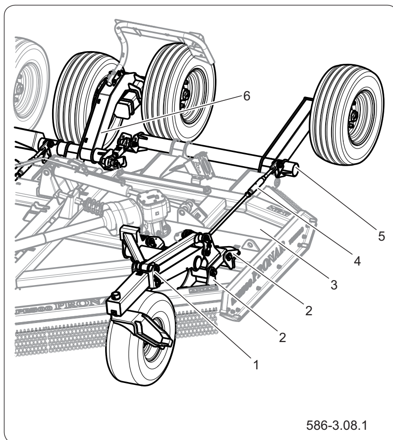
Rysunek 4.7 Przednie koła kopiujące
