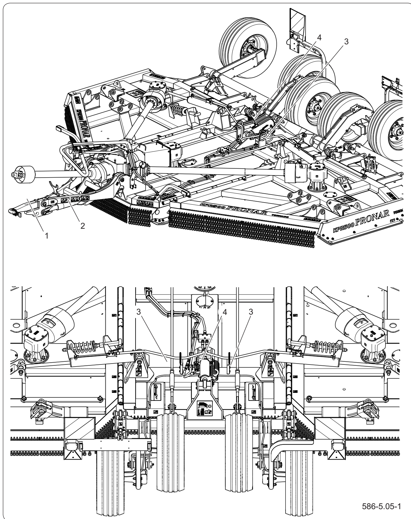
Rysunek 5.5 Regulacja położenia maszyny
