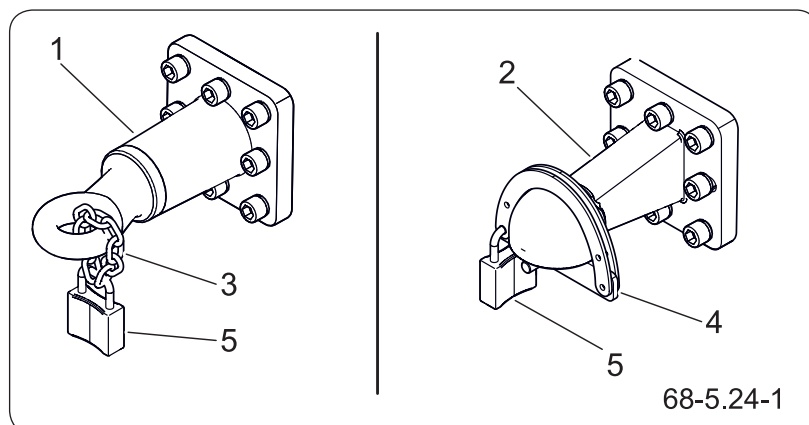
Rysunek 5.2 Zabezpieczenie ciągną dyszla
