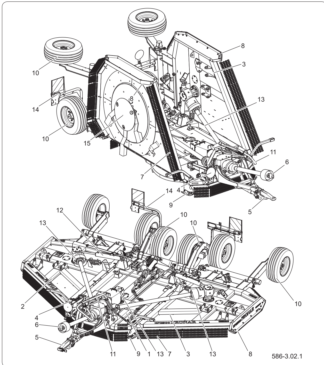
Rysunek 4.1 Budowa maszyny
