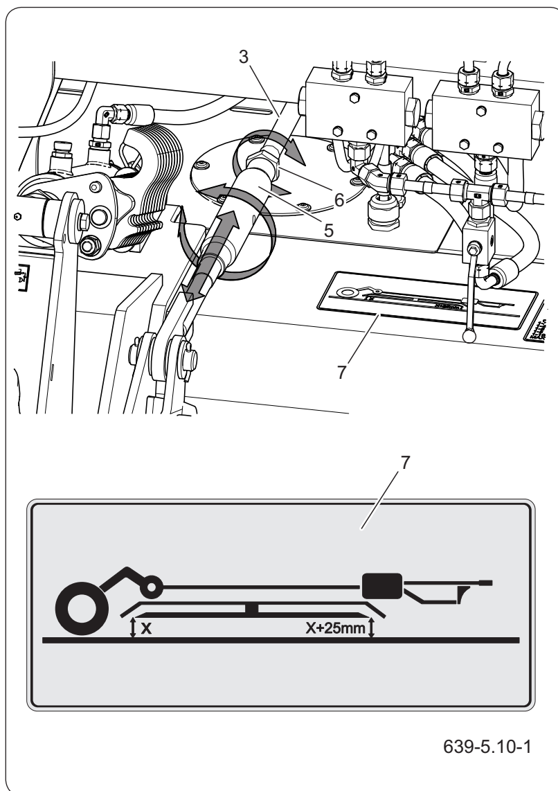
Rysunek 5.7 Regulacja pochylecia kosiarki
