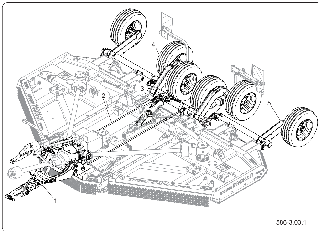
Rysunek 4.2 Budowa układu zawieszenia
