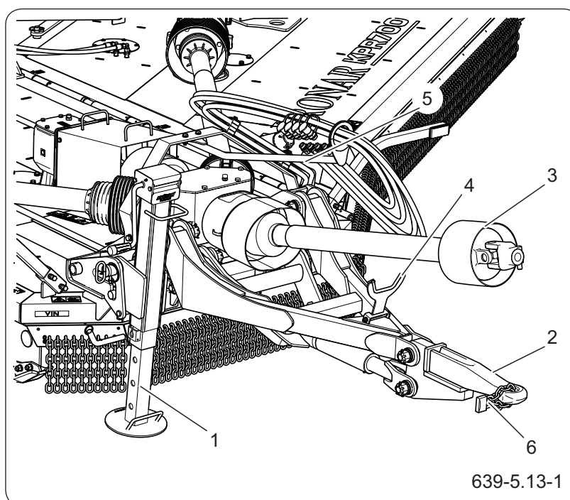
Rysunek 5.8 Łączenie kosiarki z nośnikiem
