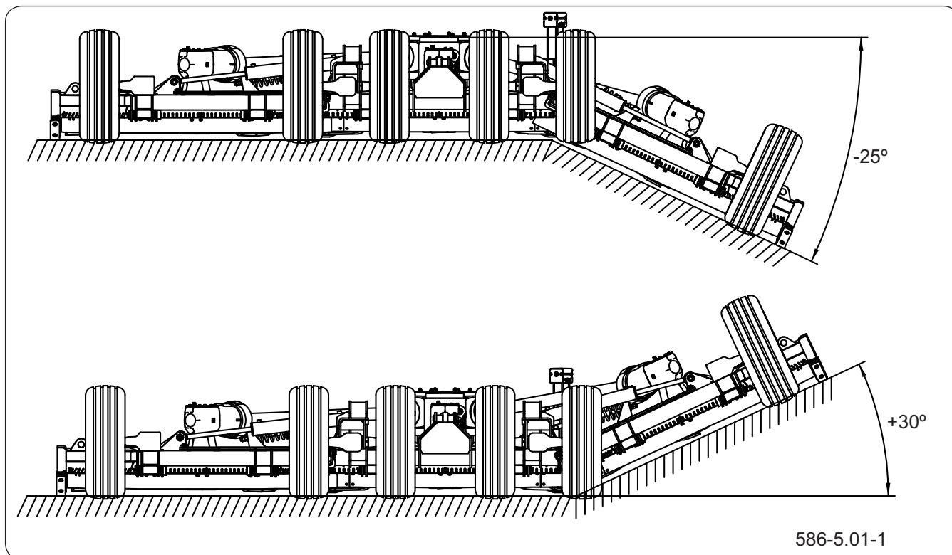
Rysunek 5.11 Praca kosiarką na pochyłości - kopiowanie terenu
