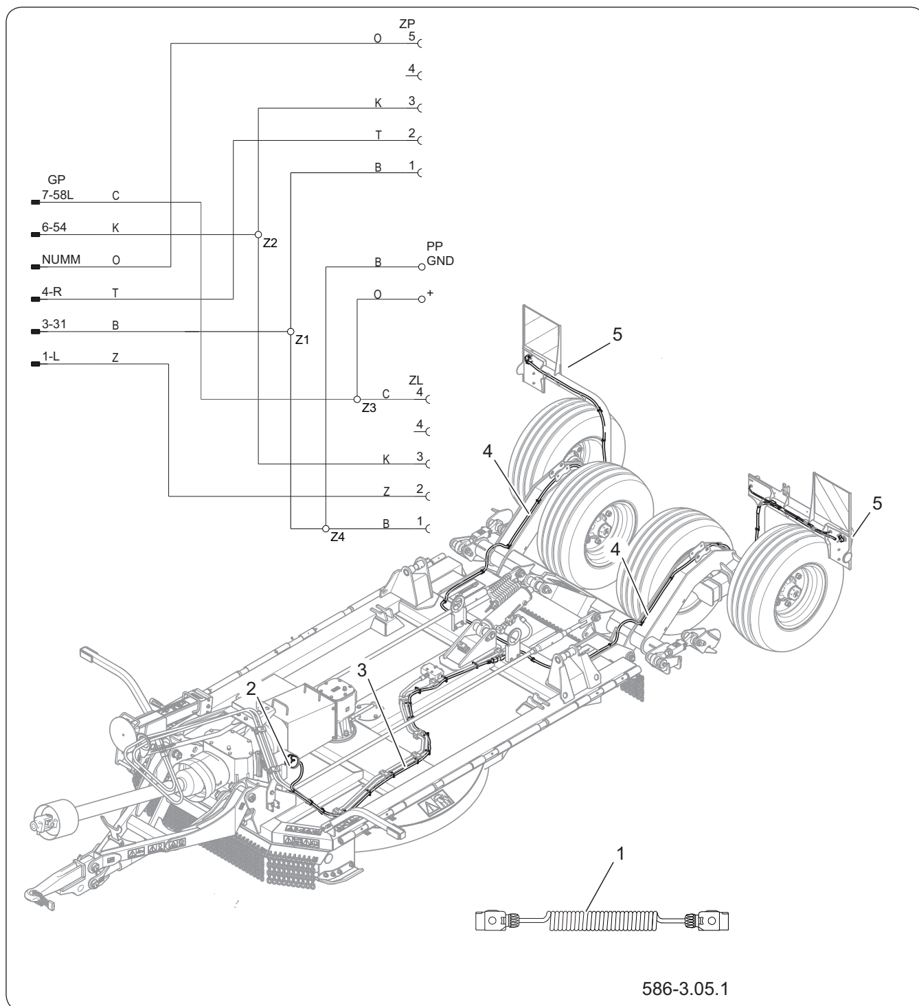
Rysunek 4.4 Budowa instalacji elektrycznej kosiarki KPR500
