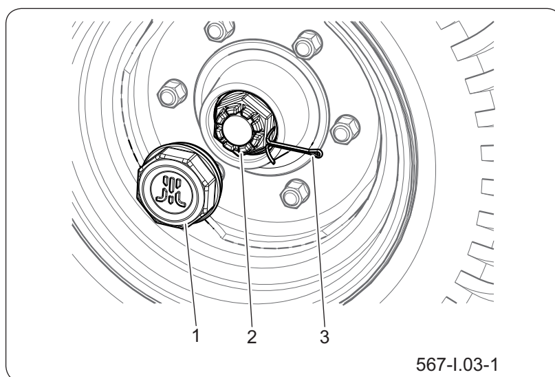
Rysunek 6.7 Regulacja luzu łożysk osi jezdnej (1) pokrywa piasty (2) nakrętka koronowa (3) zawleczka zabezpieczająca
