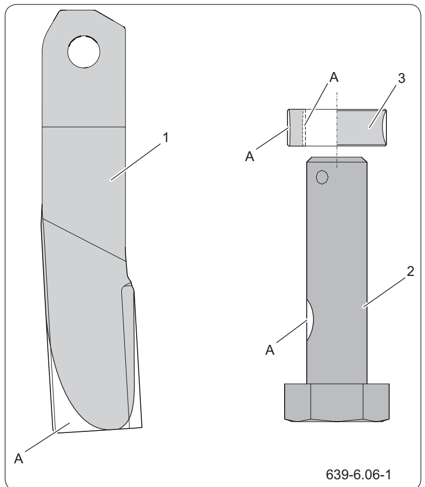
Rysunek 6.12 Potencjalne miejsca zużycia elementów głowicy
