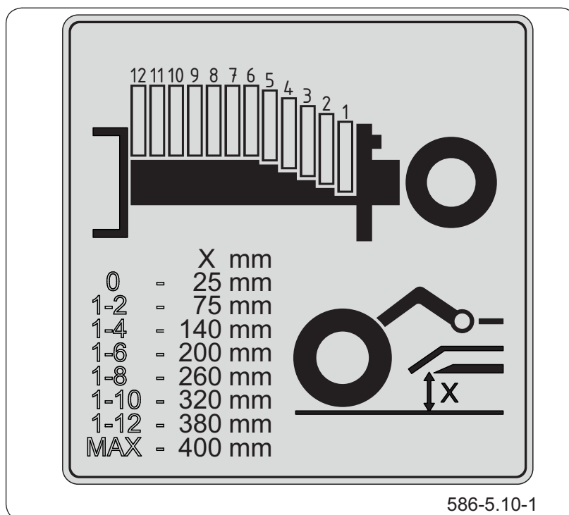
Rysunek 5.12 Wysokość koszenia
