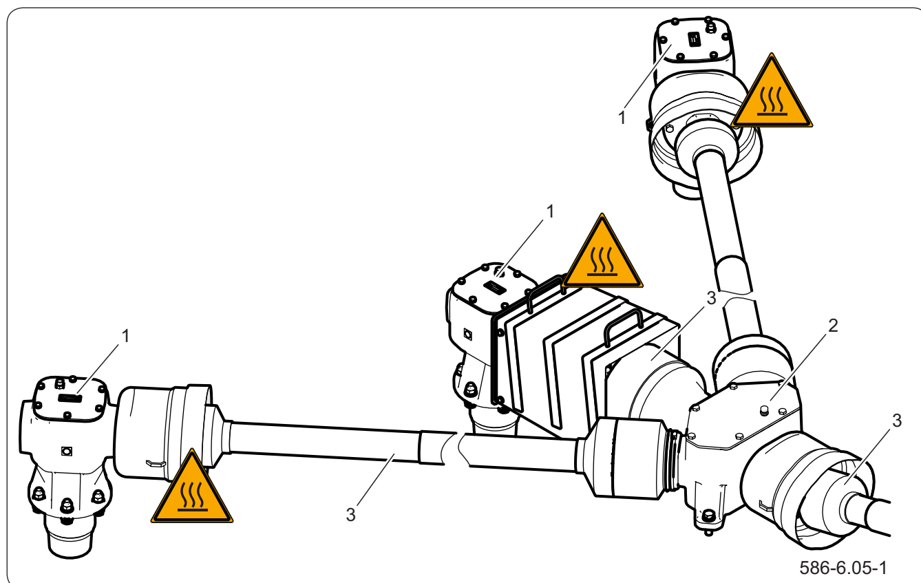
Rysunek 6.8 Kontrola i wymiana oleju w przekładni
