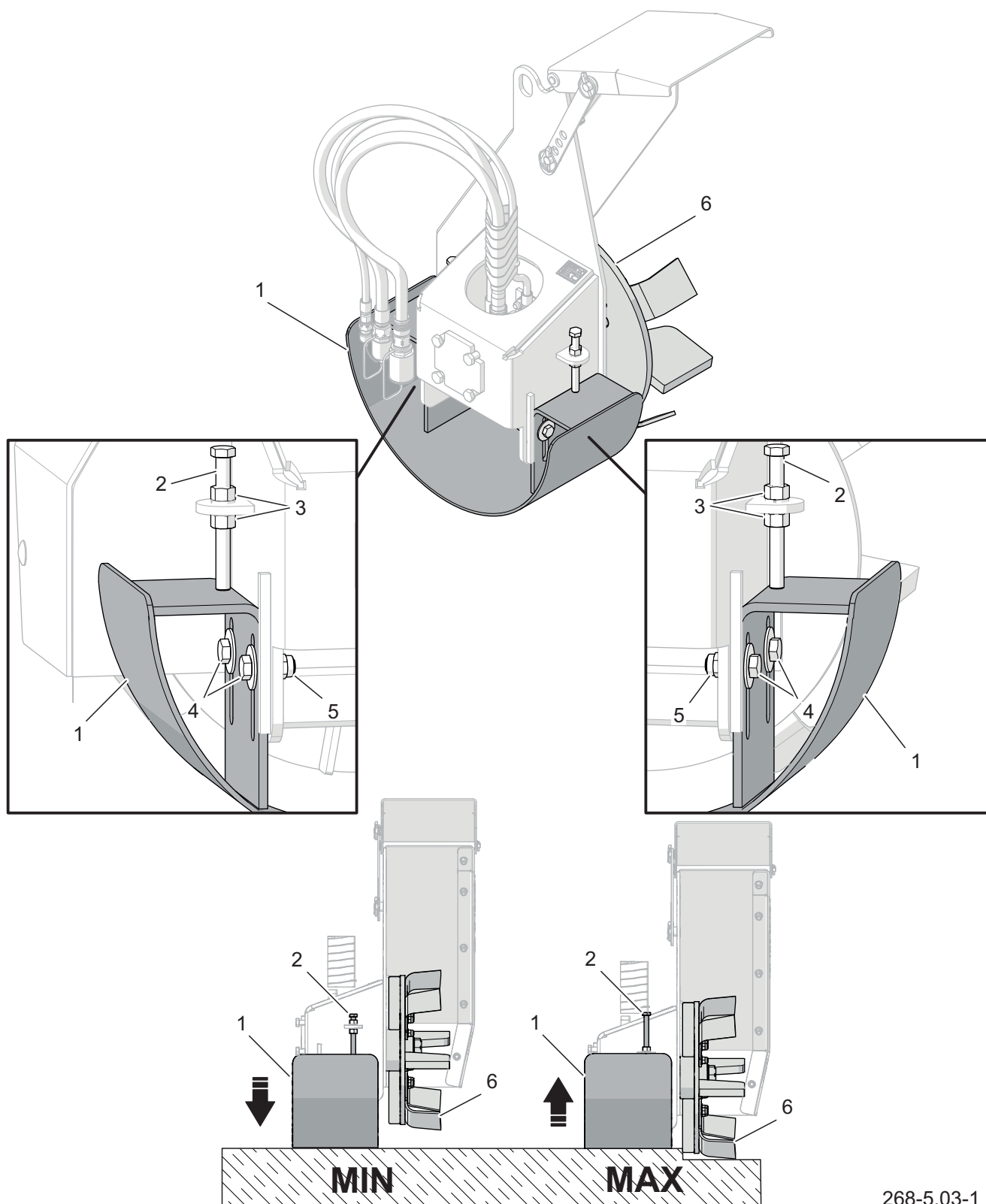
Rysunek 5.3 Ustawienie głębokości roboczej głowicy odmulającej
