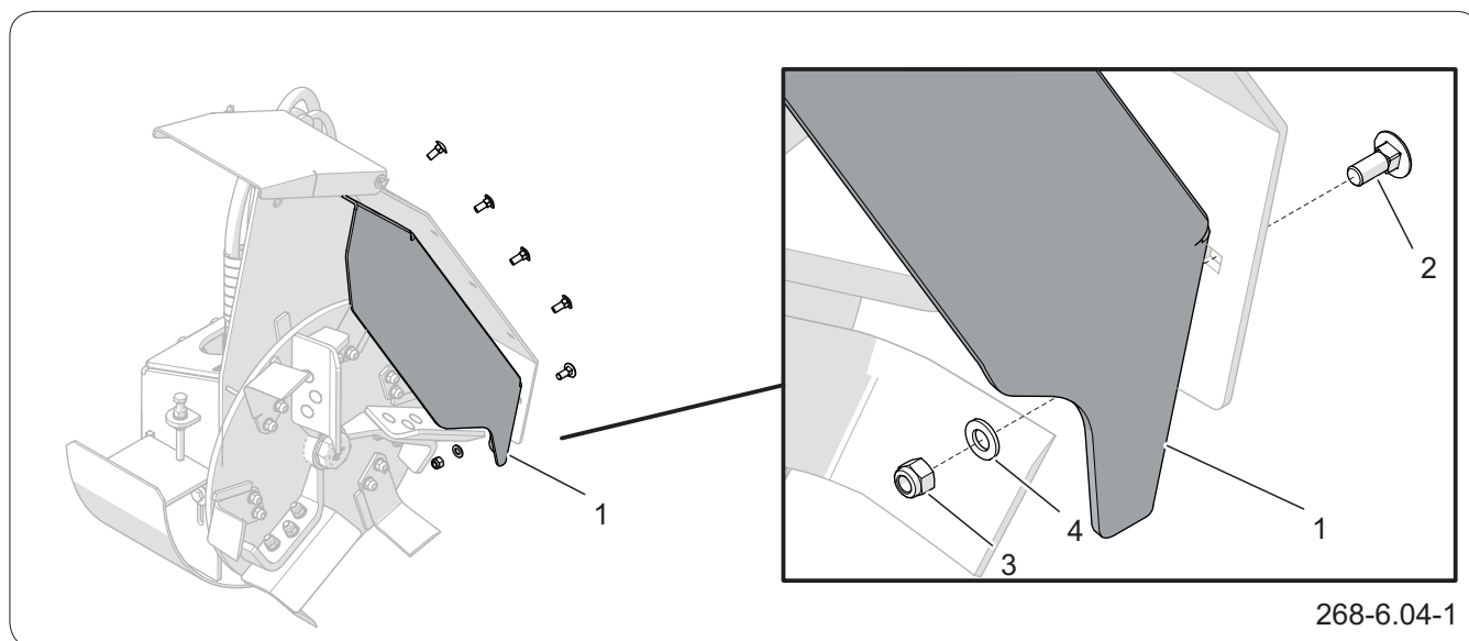
Rysunek 6.1 Demontaż osłony.
