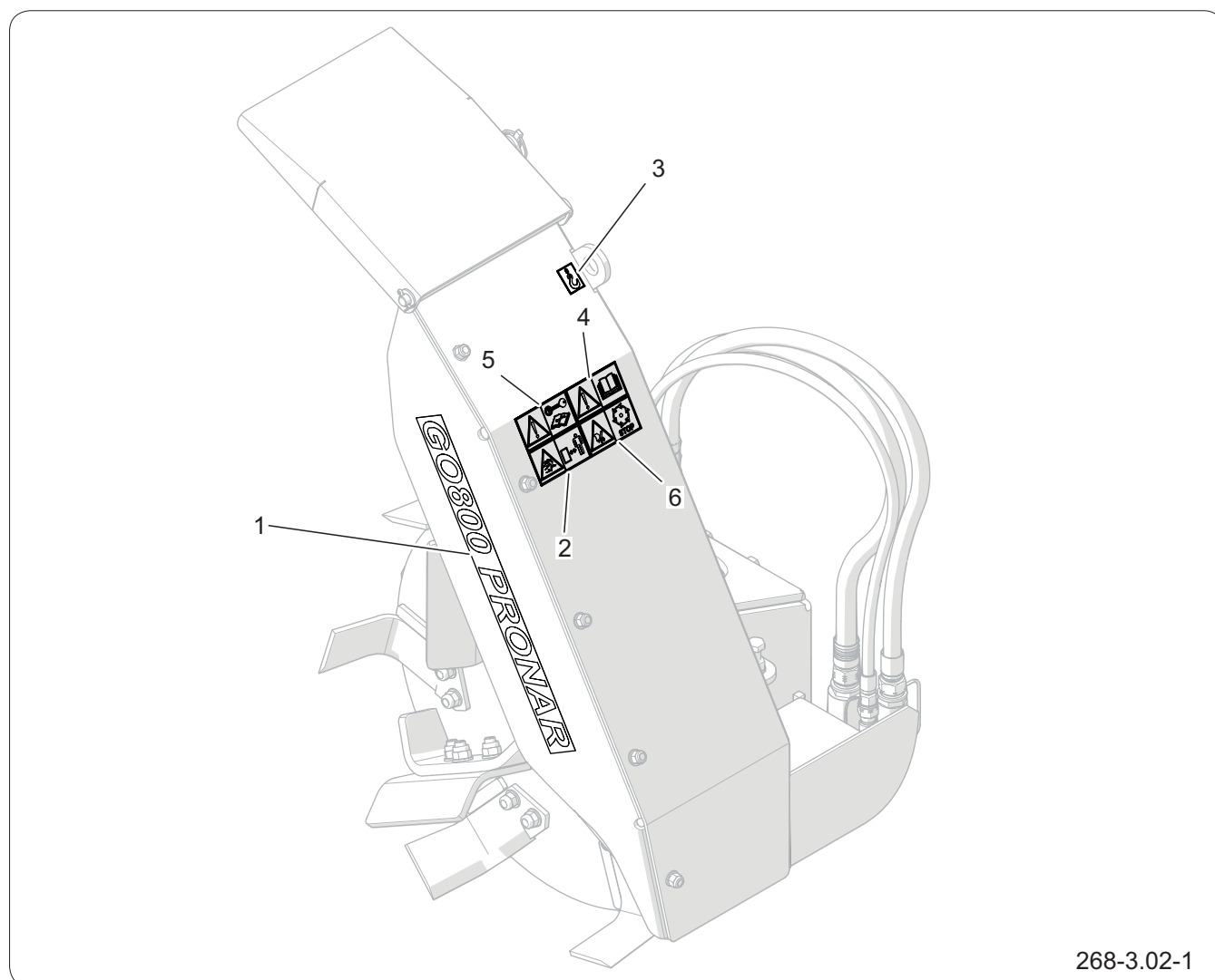
Rysunek 3.1 Rozmieszczenie nalepek informacyjnych i ostrzegawczych.
