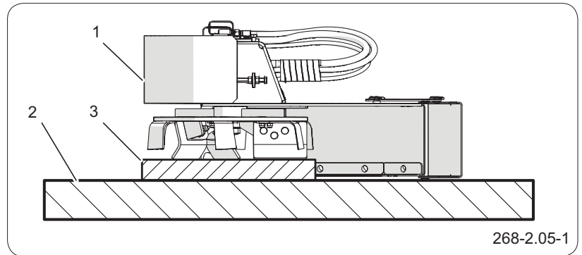
Rysunek 2.4 Sposób mocowania głowicy na paletce drewnianej
