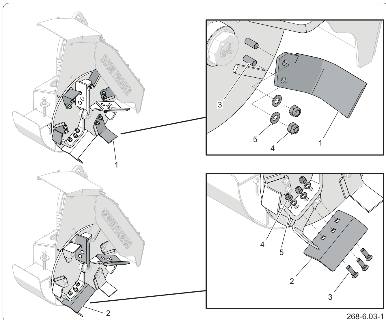
Rysunek 6.2 Wymiana noży i odrzutników.
