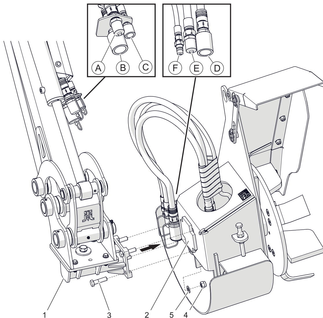
Rysunek 5.1 Łączenie z wisięgnikiem wielofunkcyjnym
