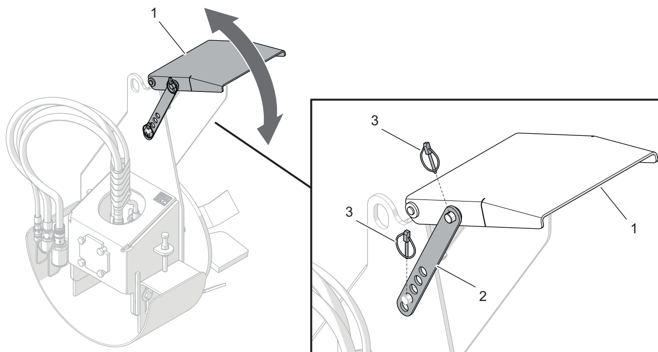
Rysunek 5.4 Regulacja kierownicy strumienia wyrzucanego materiału.
