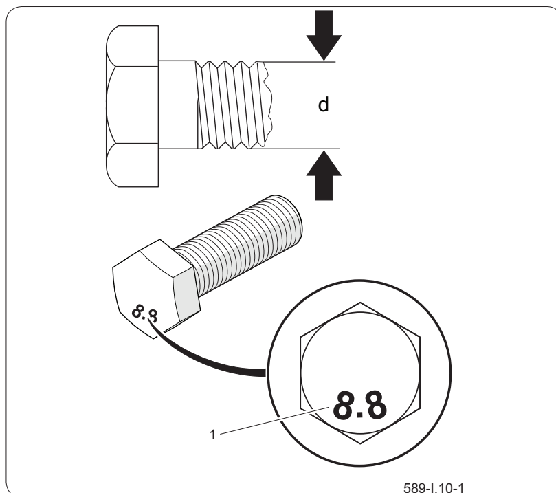
Rysunek 6.3 Śruba z gwintem metrycznym
