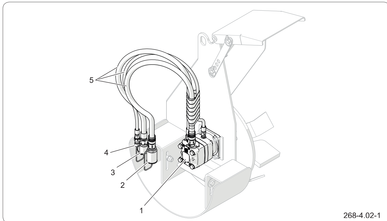
Rysunek 4.2 Budowa instalacji hydraulicznej napędu
