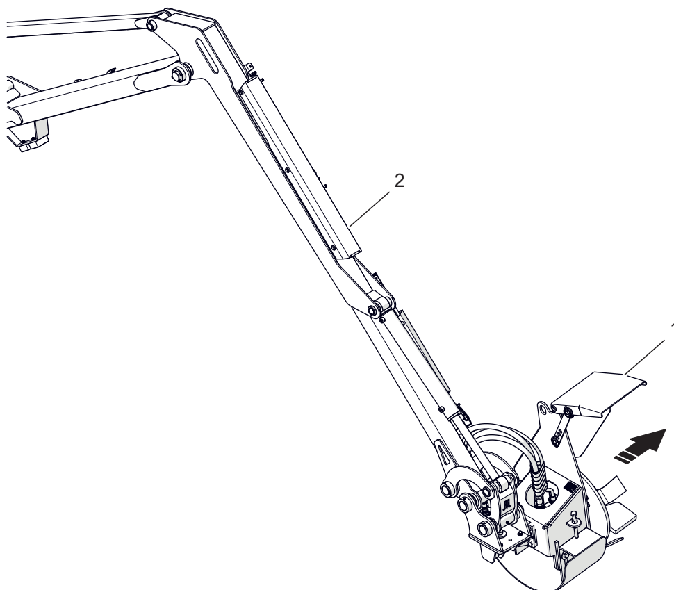
Rysunek 5.2 Pozycja robocza głowicy na wysięgniku wielofunkcyjnym (1) głowica w pozycji roboczej (2) ramię wysięgnika wielofunkcyjnego
