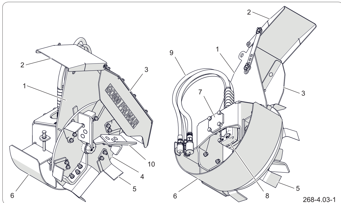
Rysunek 4.1 Budowa maszyny
