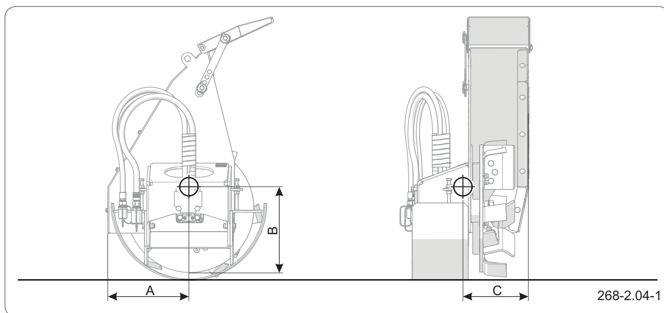
Rysunek 2.3 Położenie środka ciężkości maszyny
