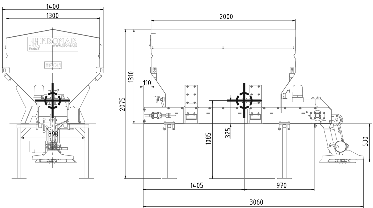
RYСУNEK 1.4 Położenie środka ciężkości EPT21
