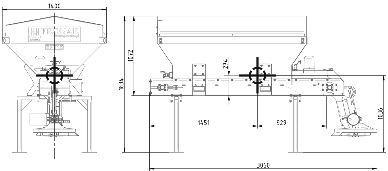
RYСУNEK 1.3 Położenie środka ciężkości EPT15
