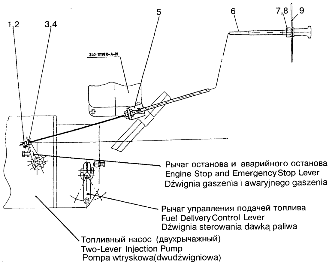
Rys. 24 Mechanizm zatrzymywania silnika (z 2-dźwigniową pompą wtryskową)
