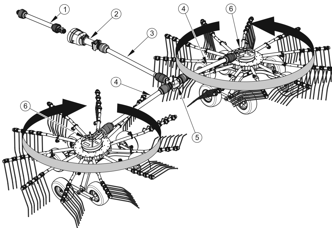
RYSUNEK 3.6 Budowa układu przeniesienia napędu
