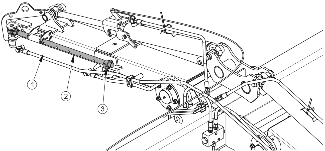
RYСУNEK 4.7 Ustawienie szerokości zgrabiarki (regulacja hydrauliczna)
