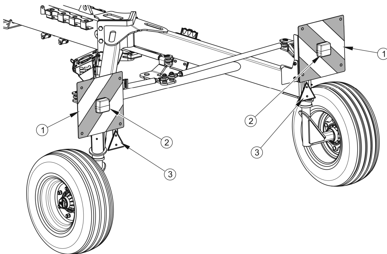
RYSUNEK 3.9 Rozmieszczenie elementów instalacji elektrycznej oraz elementów odblaskowych
