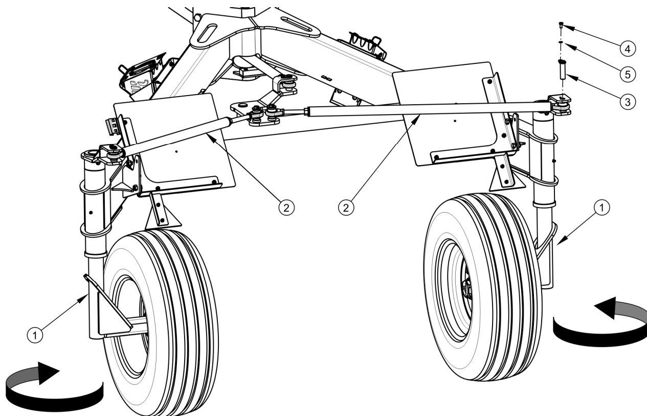
RYСУNEK A.1 Obrót kół
