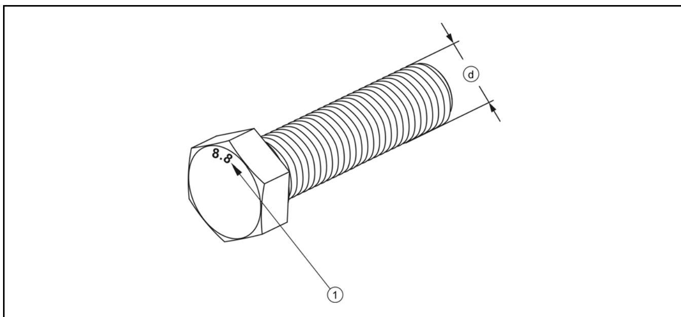
RYSUNEK 5.4A Śruba z gwintem metrycznym
