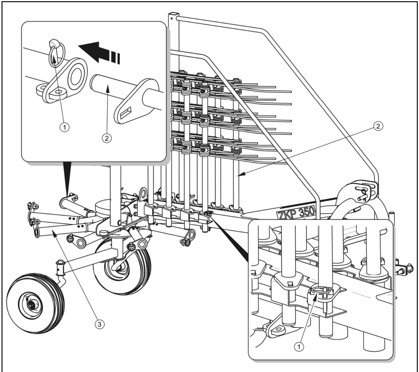
RYSUNEK 4.2A Montaż ramion
