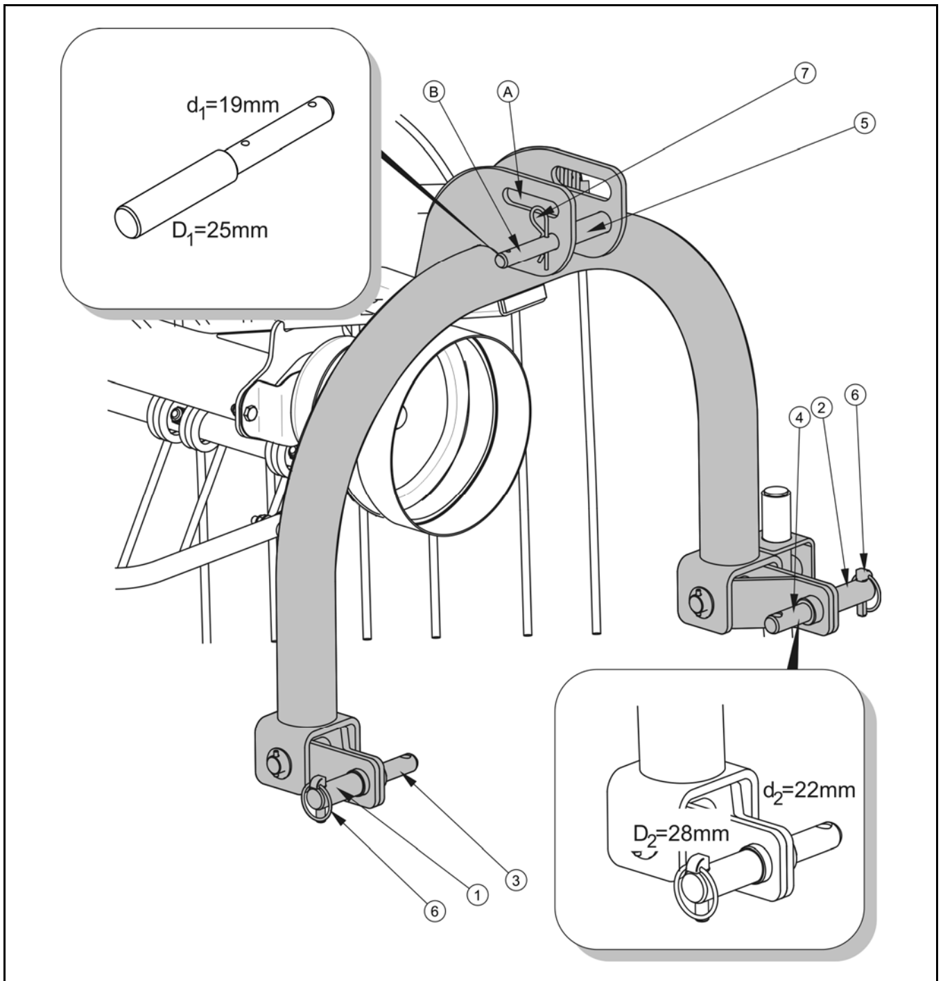
RYSUNEK 3.2A Układ zaczepowy
