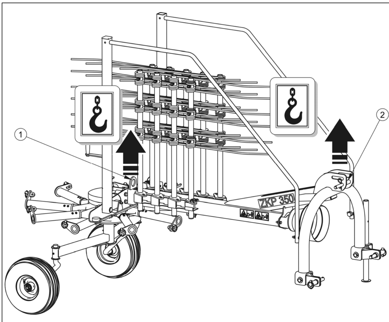
RYСУNEK 1.2A Miejsca podwieszania zgrabiarki
