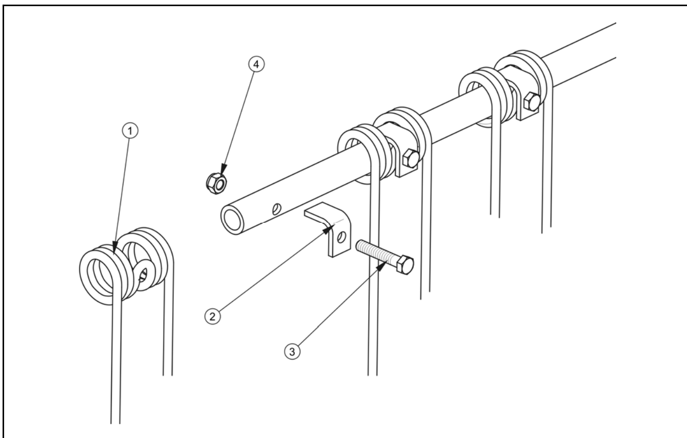
RYSUNEK 5.3A Wymiana zębów grabiących
