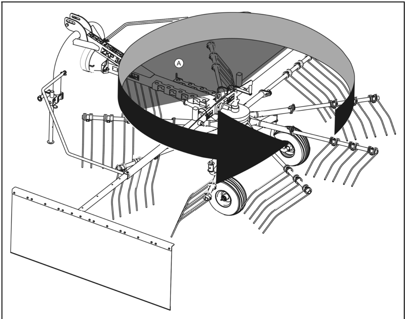
RYSUNEK 3.3A Zasada działania zgrabiarki
