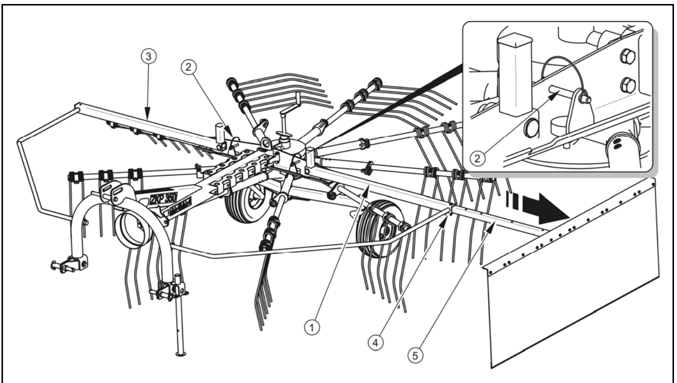
RYSUNEK 4.3A Ustawienie osłon bocznych
