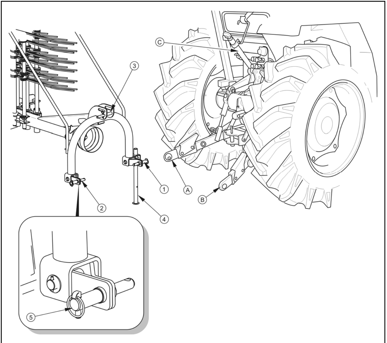
RYSUNEK 4.1A Łączenie zgrabiarki z ciągnikiem
