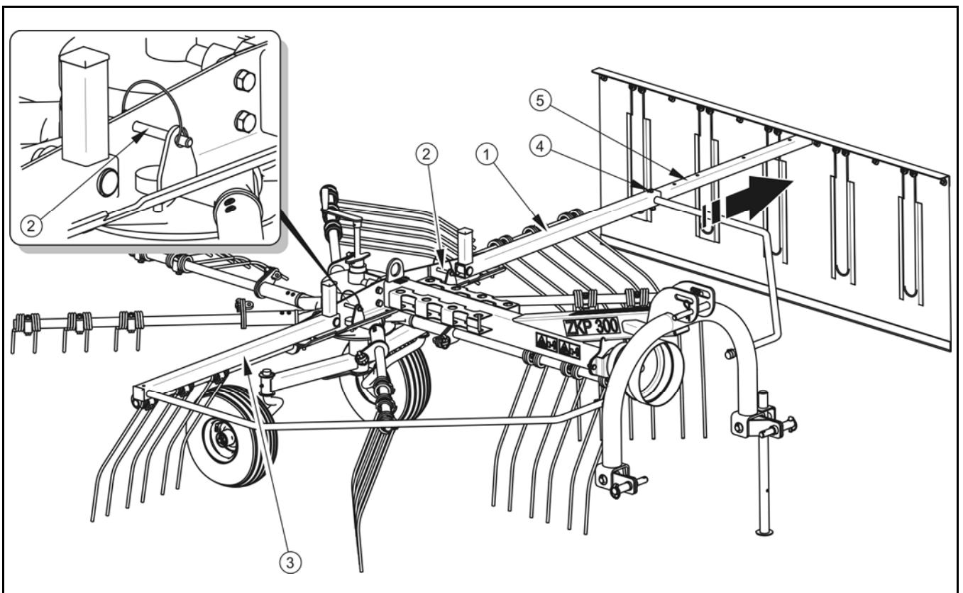
RYSUNEK 4.3A Ustawienie osłon bocznych
