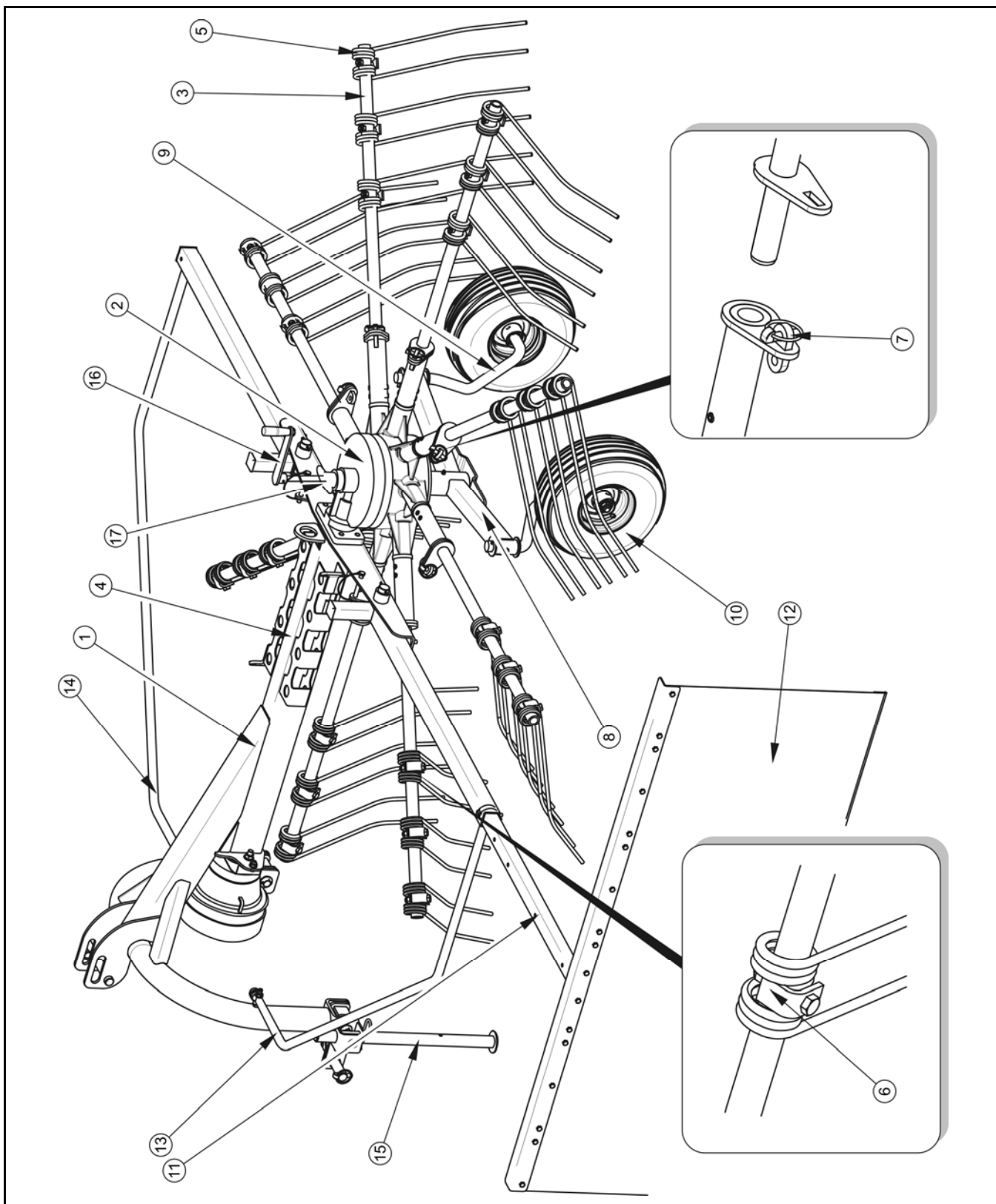
RYСУNEK 3.1A Budowa zgrabiarki karuzelowej
