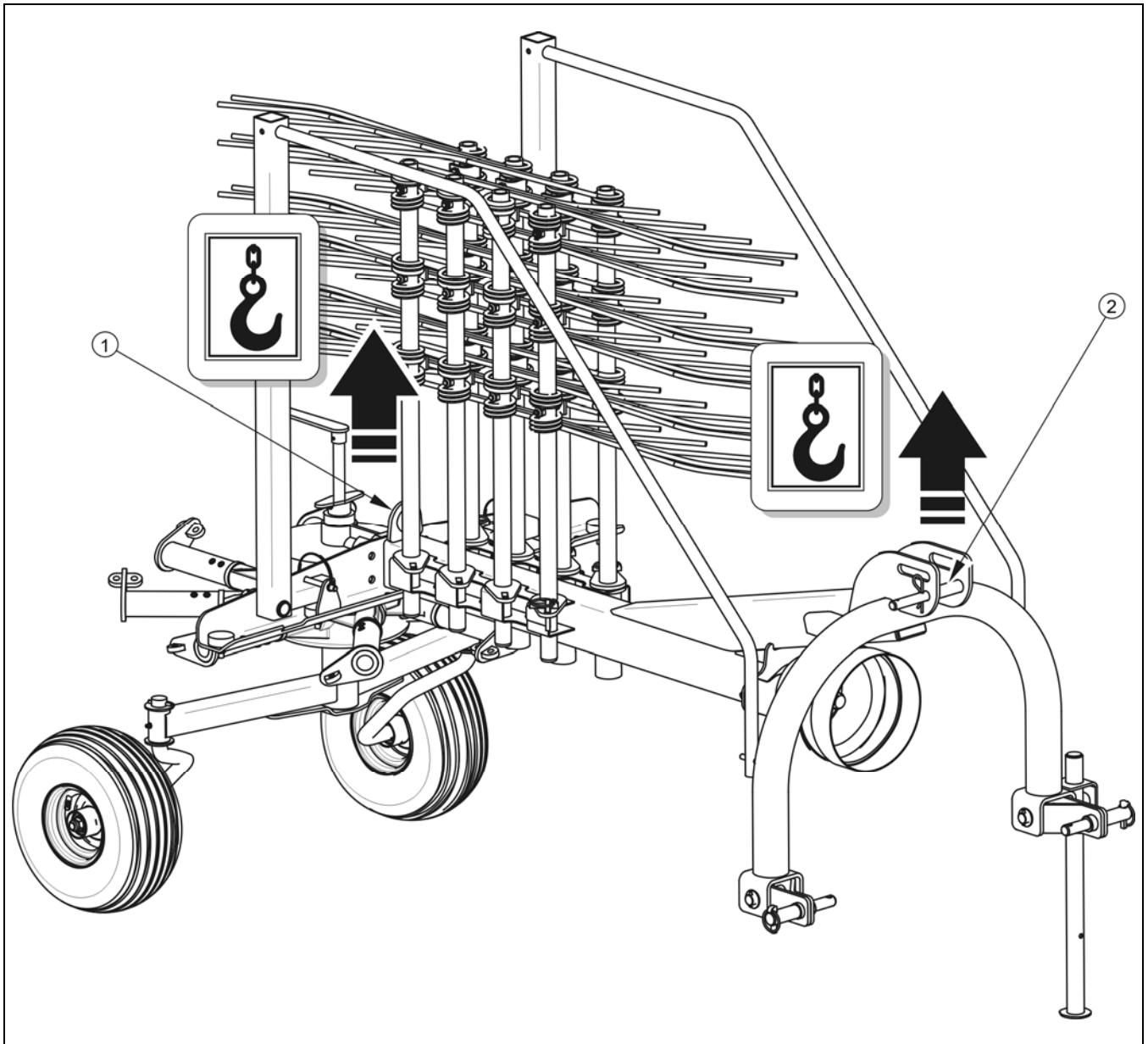
RYSUNEK 1.2A Miejsca podwieszania zgrabiarki
