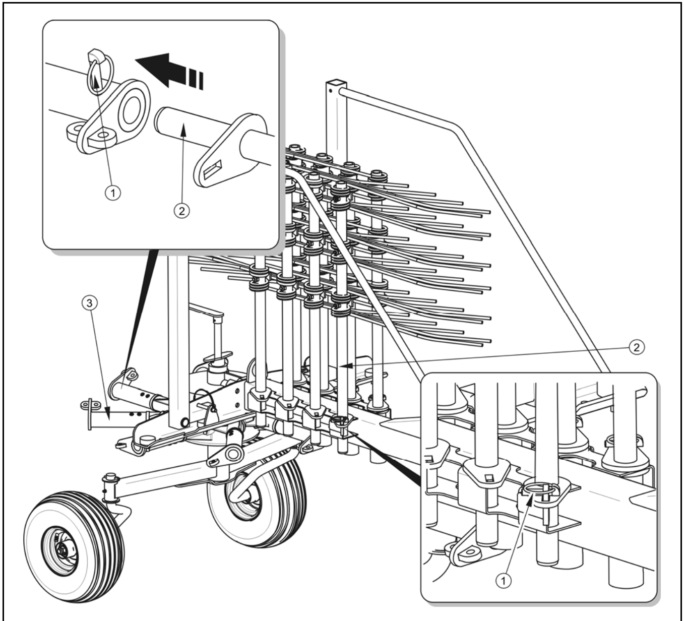
RYSUNEK 4.2A Montaż ramion
