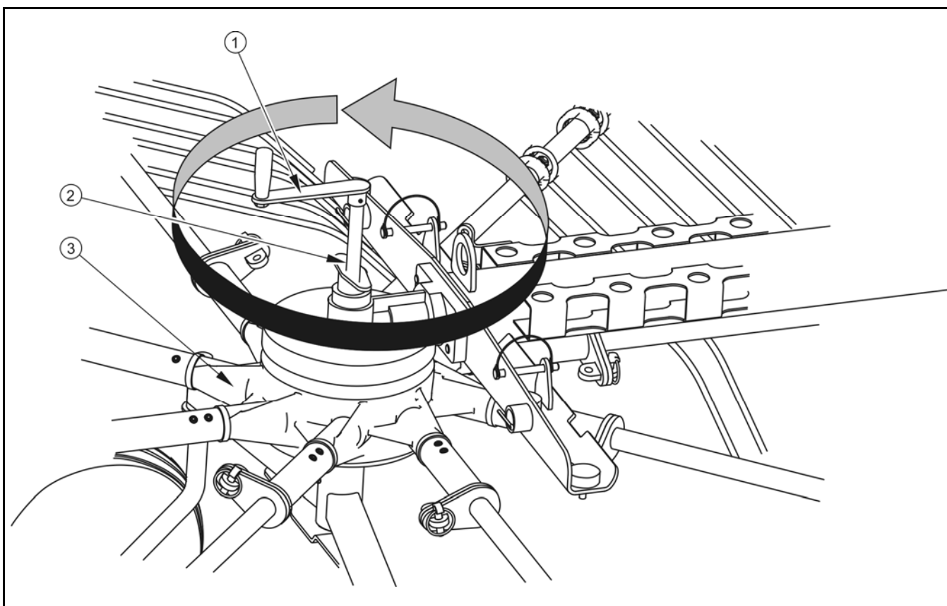
RYSUNEK 4.4A Regulacja wysokości roboczej
