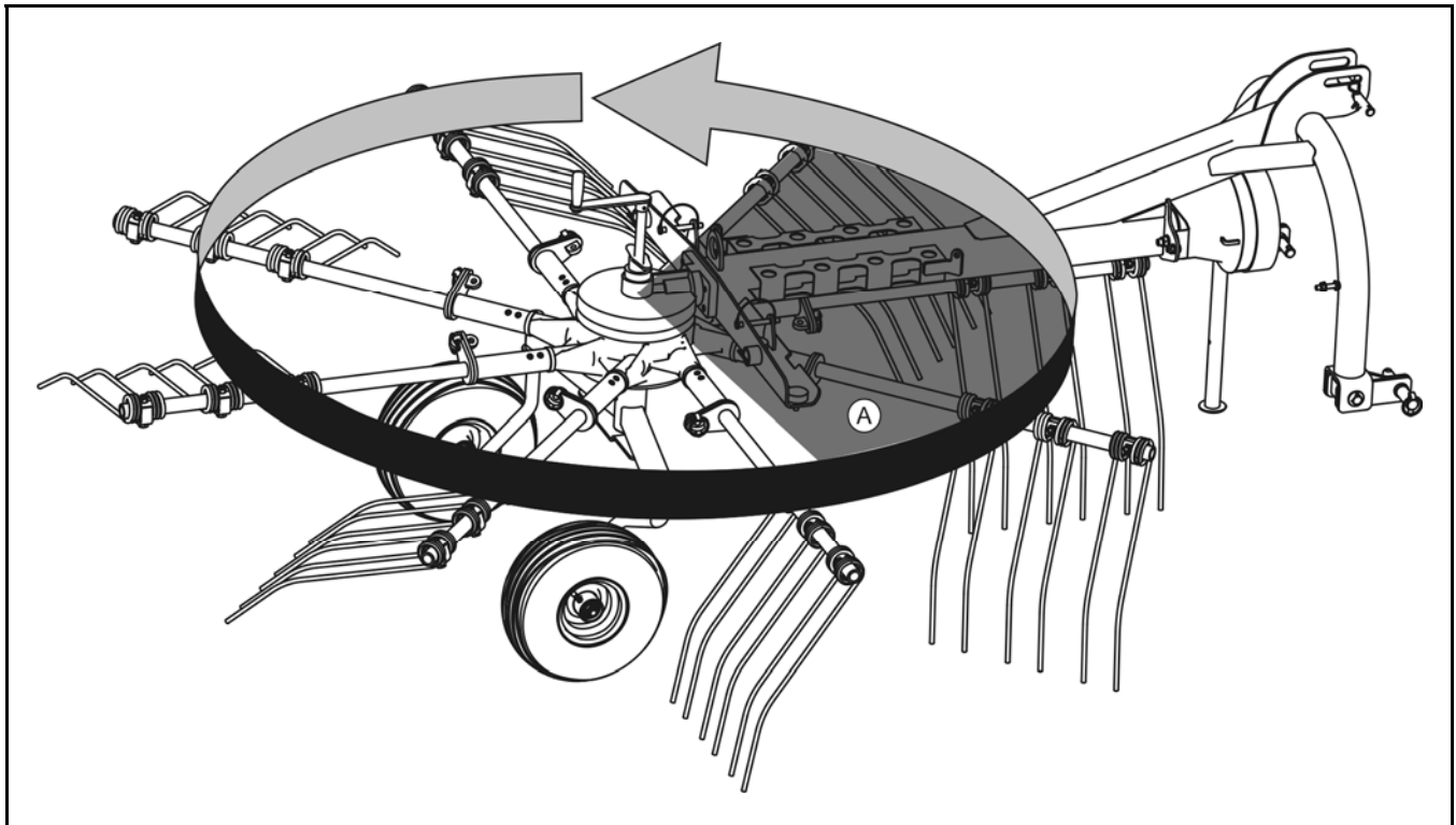
RYSUNEK 3.3A Zasada działania zgrabiarki
