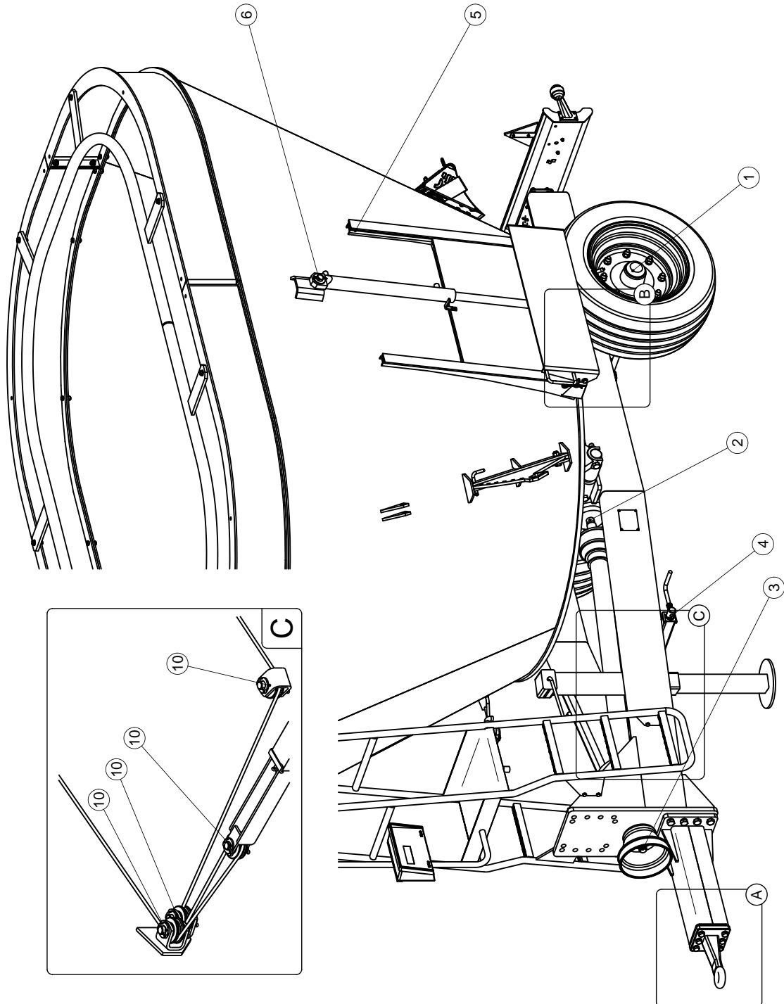
ABBILD 5.4A SCHMIERSTELLEN DES FUTTERWAGENS
