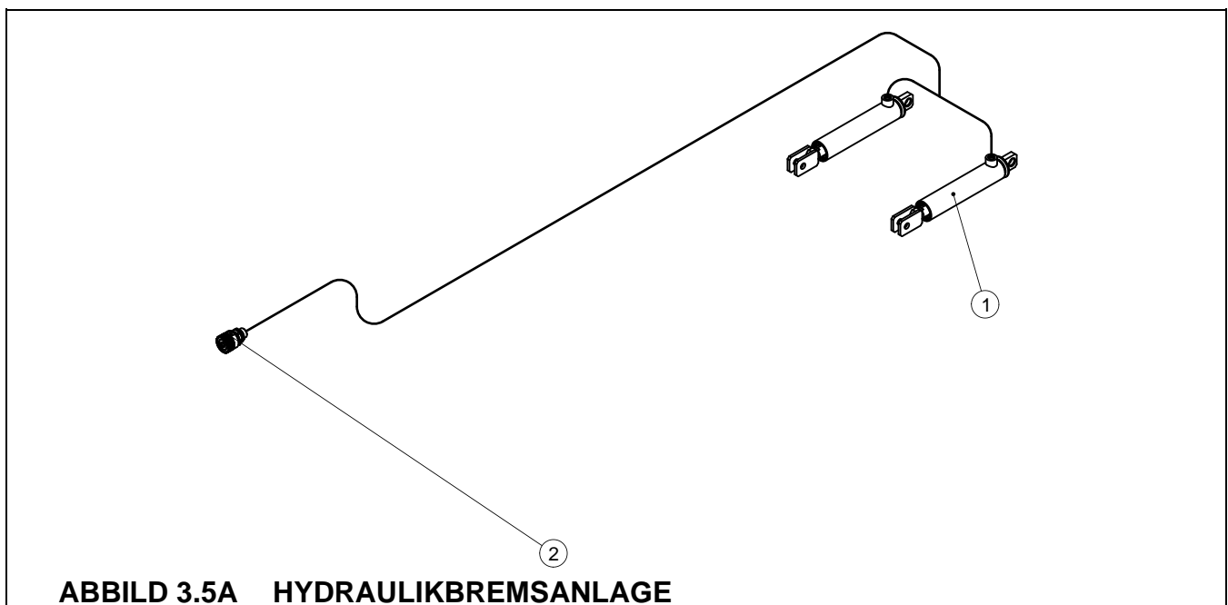
(1) Hydraulikbremszylinder, (2) Schnellverschluss
