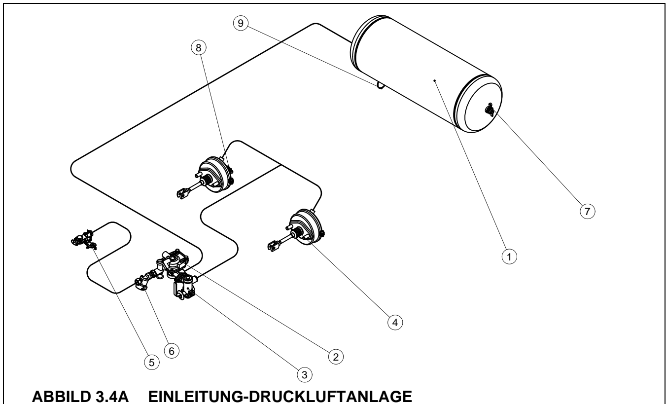
(1) Luftbehälter, (2) Steuerungsventil, (3) Bremskraftregler, (4) Druckluftzylinder, (5) Verbindung der Leitungen, (6) Luftfilter, (7) Prüfverbindung des Luftbehälters, (8) Prüfverbindung des Druckluftzylinders, (9) Entwässerungsventil
