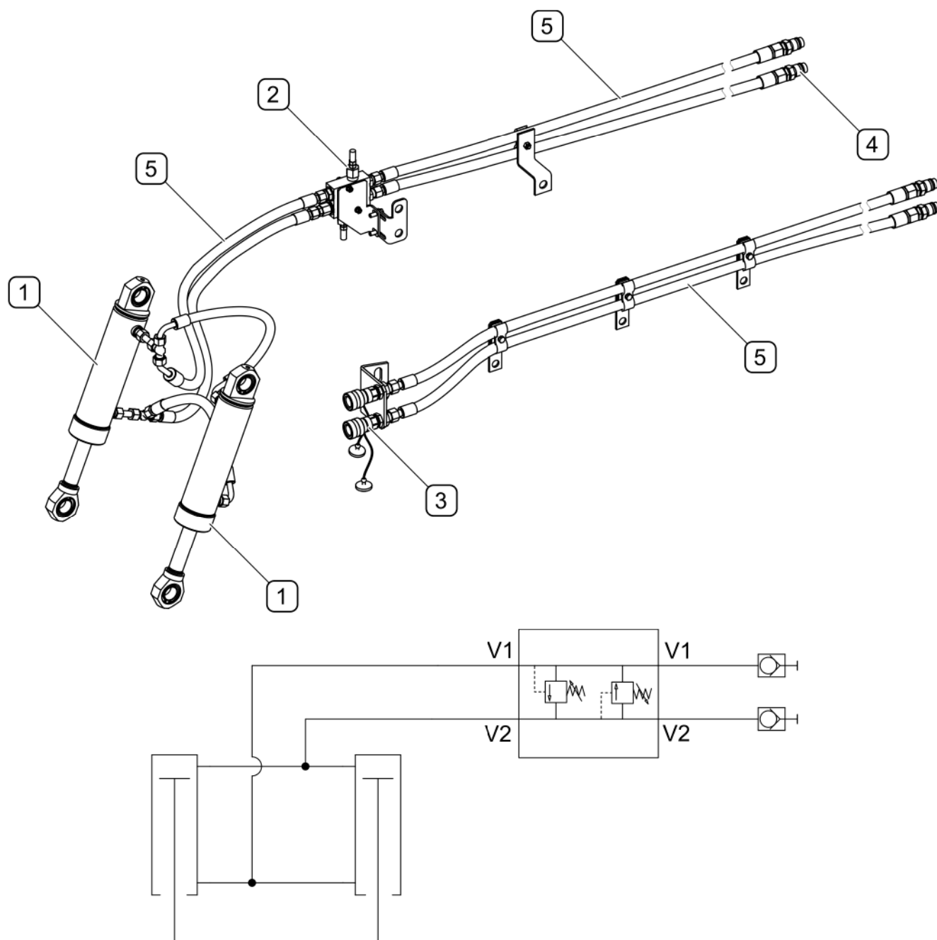
RYSUNEK 3.2 Budowa instalacji hydraulicznej przedniego TUZ
