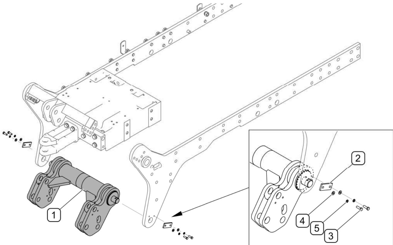
RYSUNEK 4.6 Montaż dźwigni
