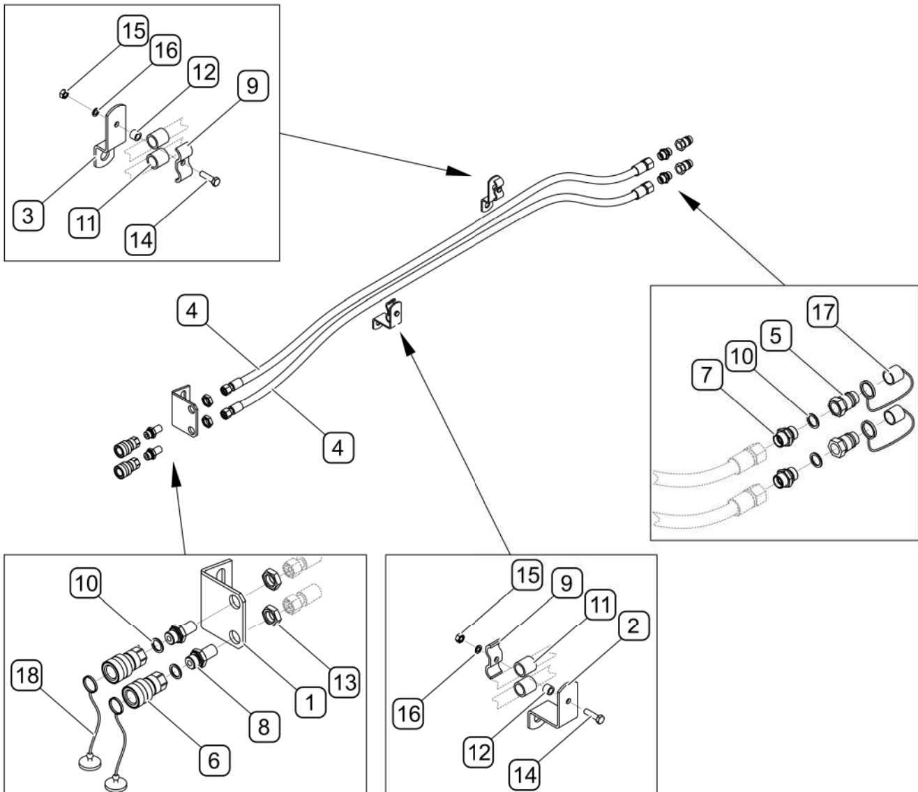
RYSUNEK 4.11 Montaż przednich szybkozłączy hydraulicznych TUZ
