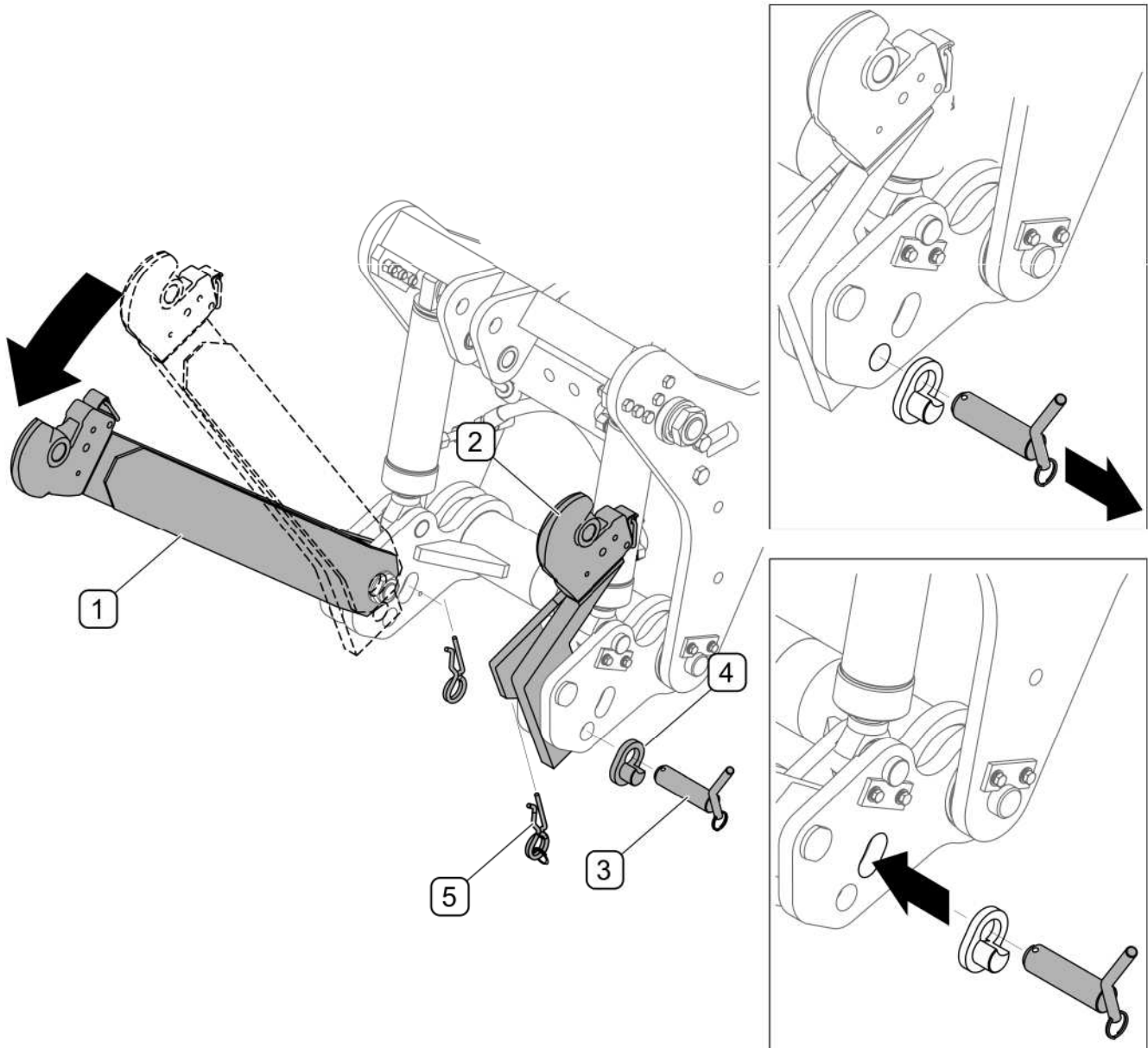
RYSUNEK 4.12 Ustawienie cięgieł dolnych do pozycji roboczej
