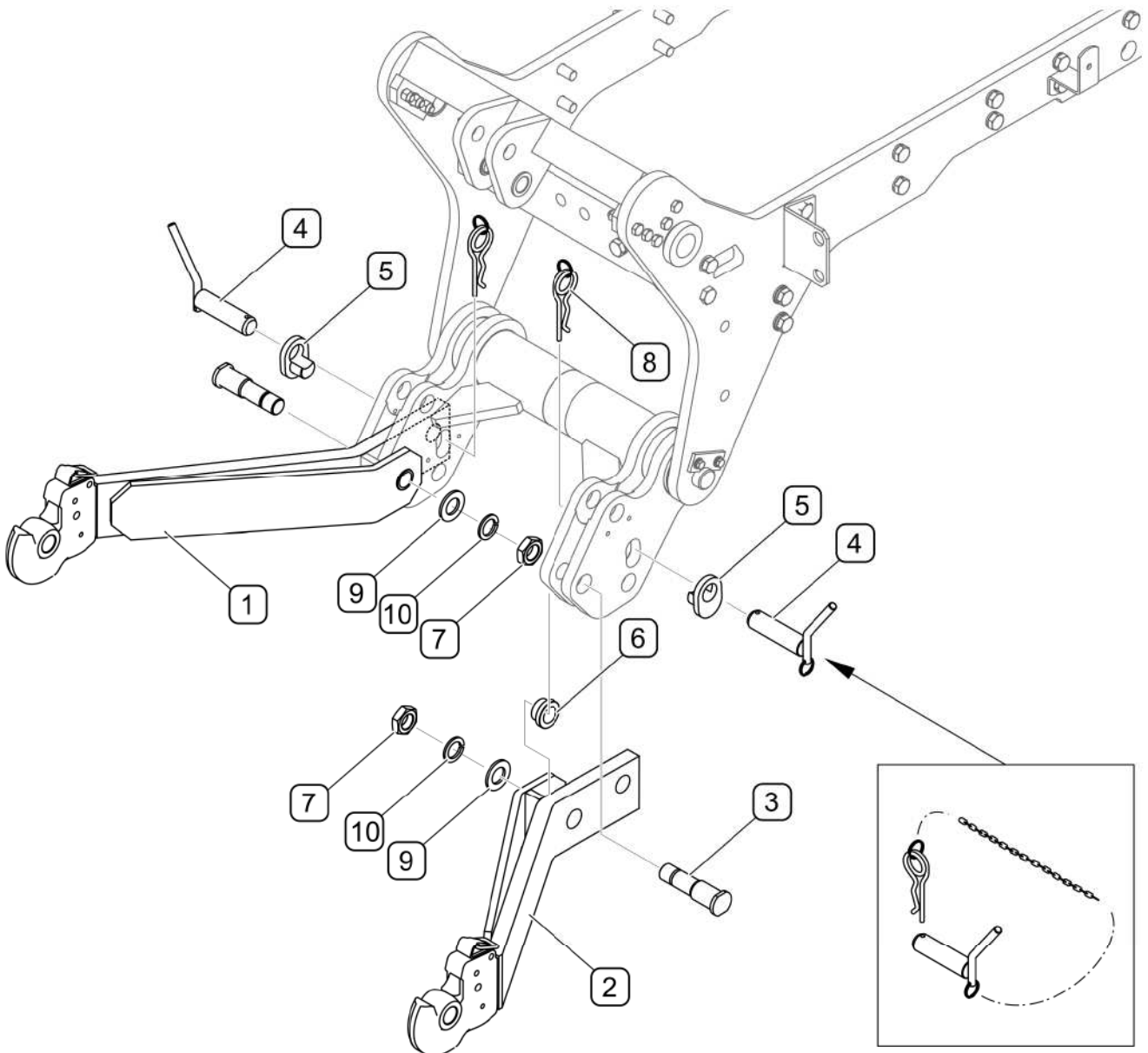
RYSUNEK 4.7 Montaż ramion cięgieł dolnych
