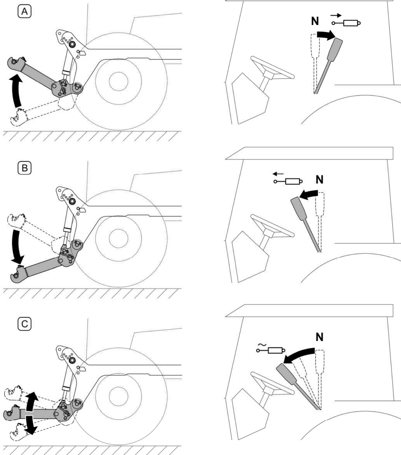
RYСУNEK 4.17 Sterowanie ramionami przedniego TУZ
