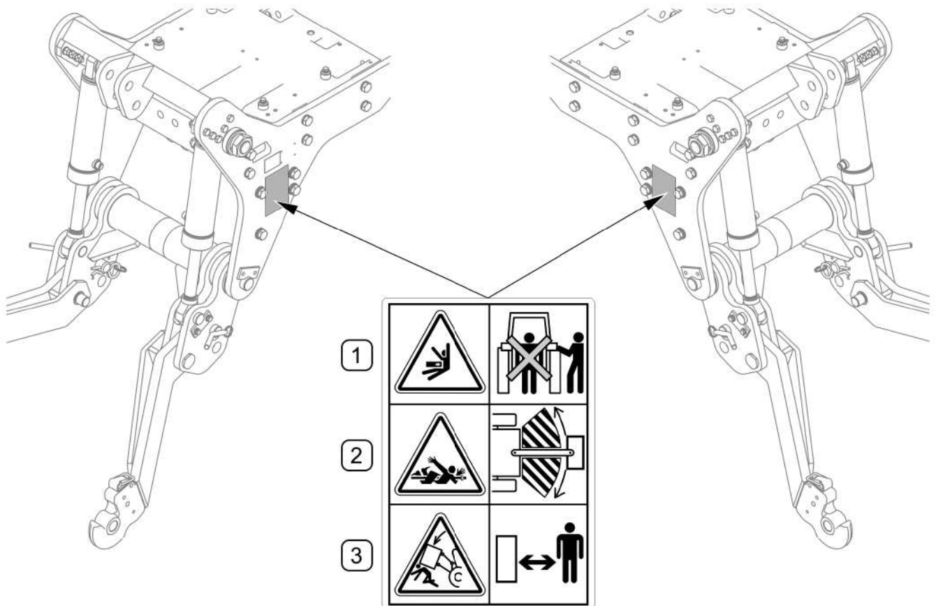
RYSUNEK 2.1 Rozmieszczenie naklejek informacyjnych i ostrzegawczych
