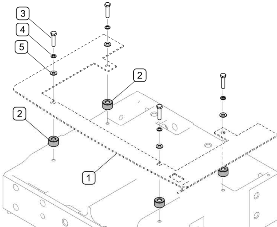
RYSUNEK 4.2 Montaż tulejek podstawy maski (Belarus)
