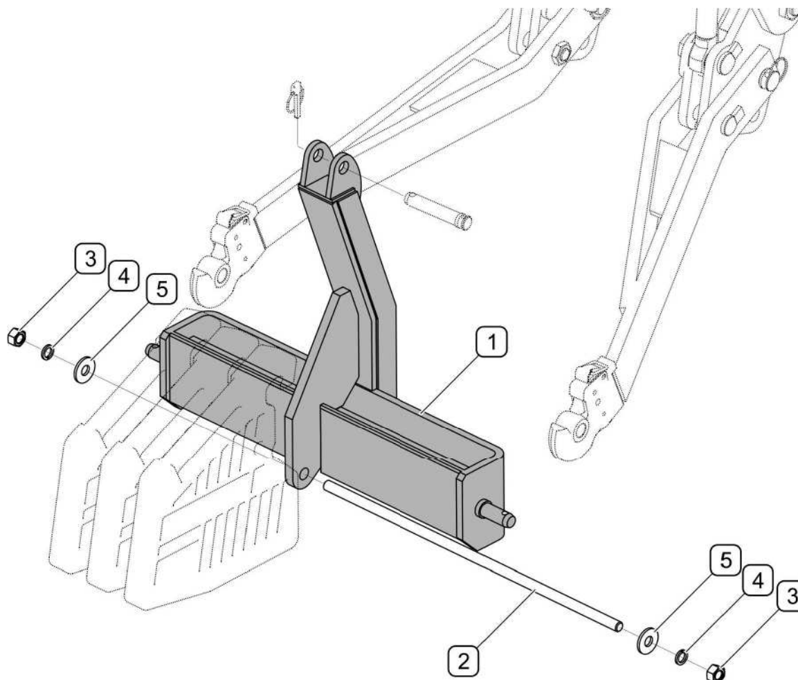
RYSUNEK 4.19 Wieszak obciążników (opcja)
