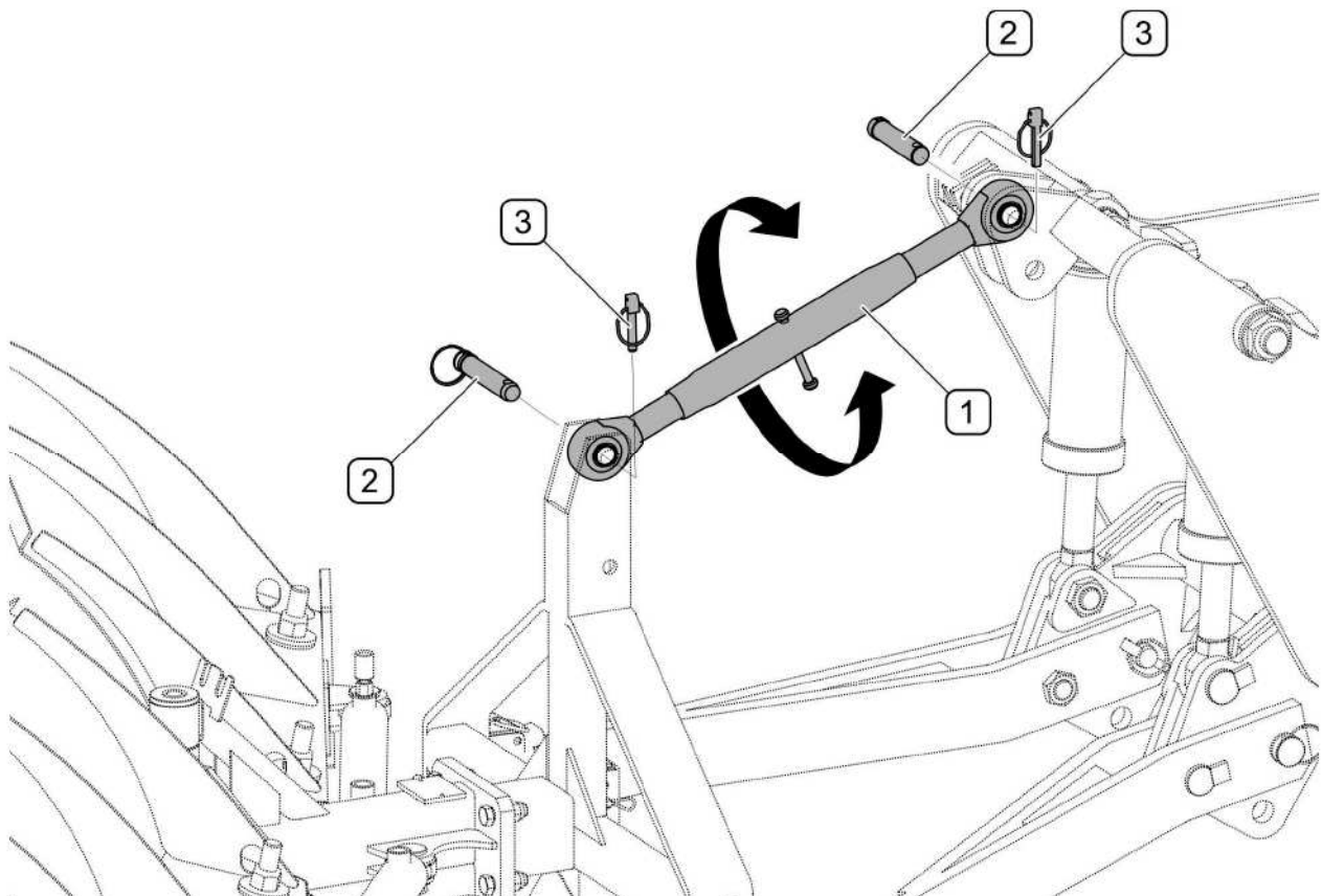
RYSUNEK 4.15 Łączenie cięgła górnego (rysunek przykładowy)
