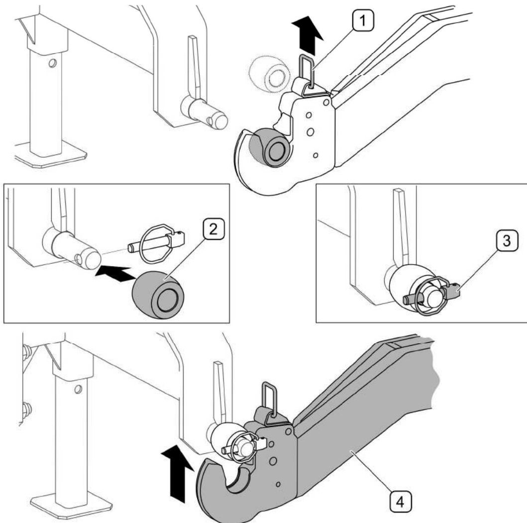
RYSUNEK 4.14 Łączenie cięgieł dolnych
