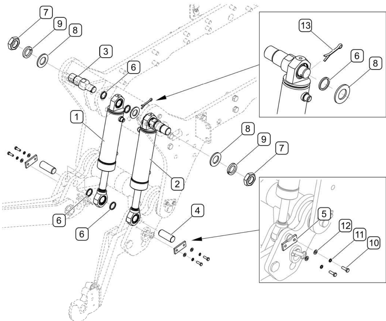
RYSUNEK 4.8 Montaż siłowników hydraulicznych
