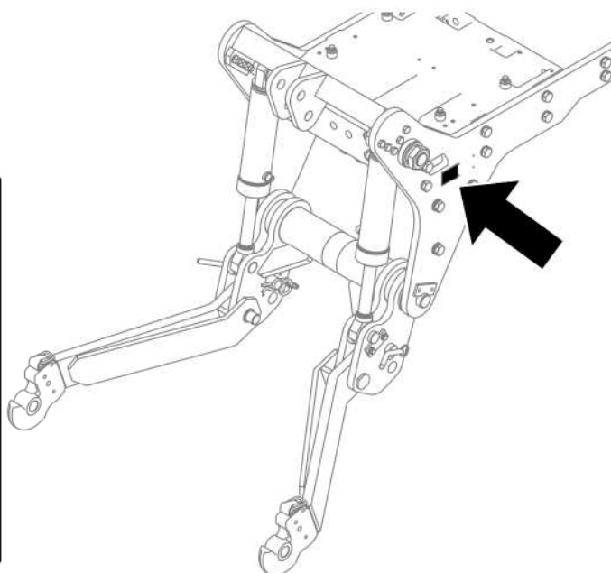
RYСУNEK 1.1 Miejsce umieszczenia tabliczki znamionowej
