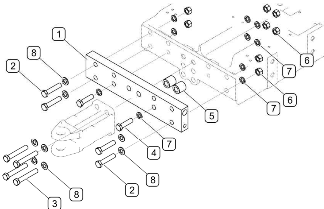
RYSUNEK 4.3 Montaż przedniego wspornika
