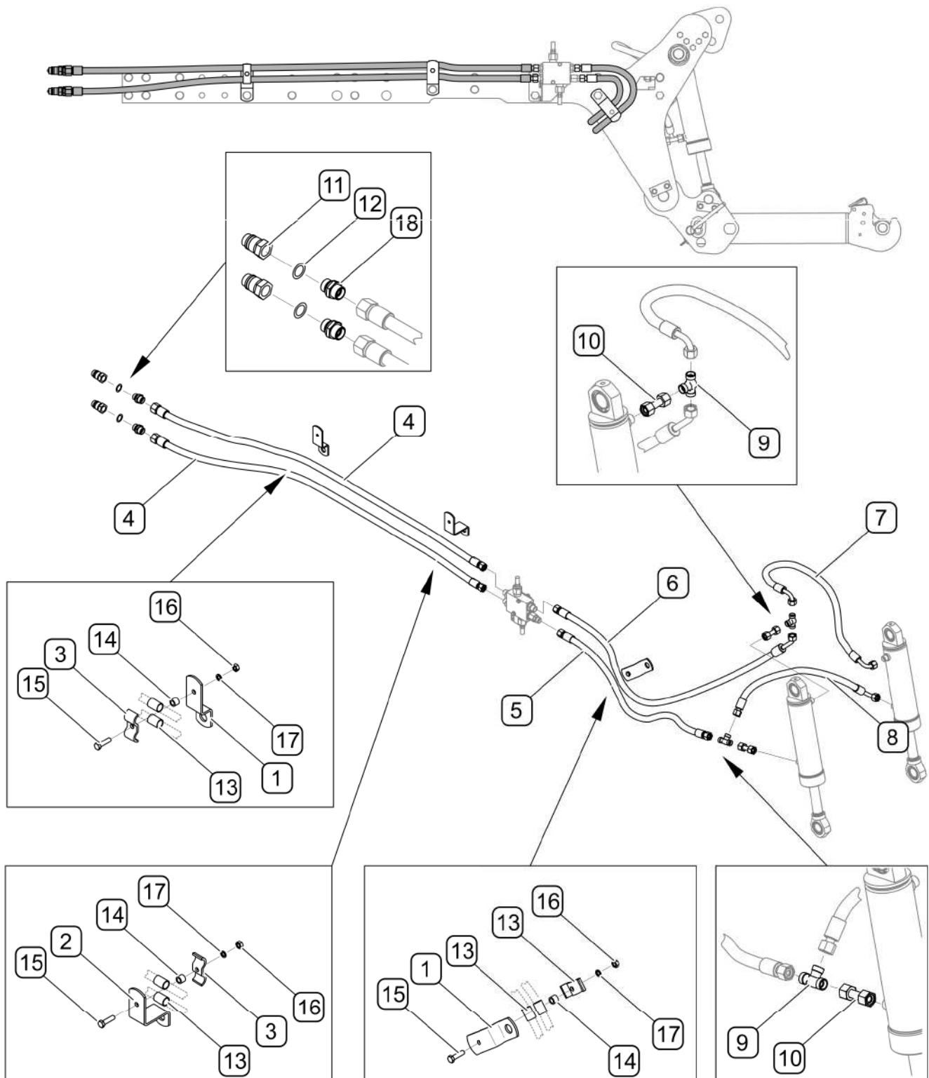
RYSUNEK 4.10 Montaż przewodów hydraulicznych zasilania TUZ
