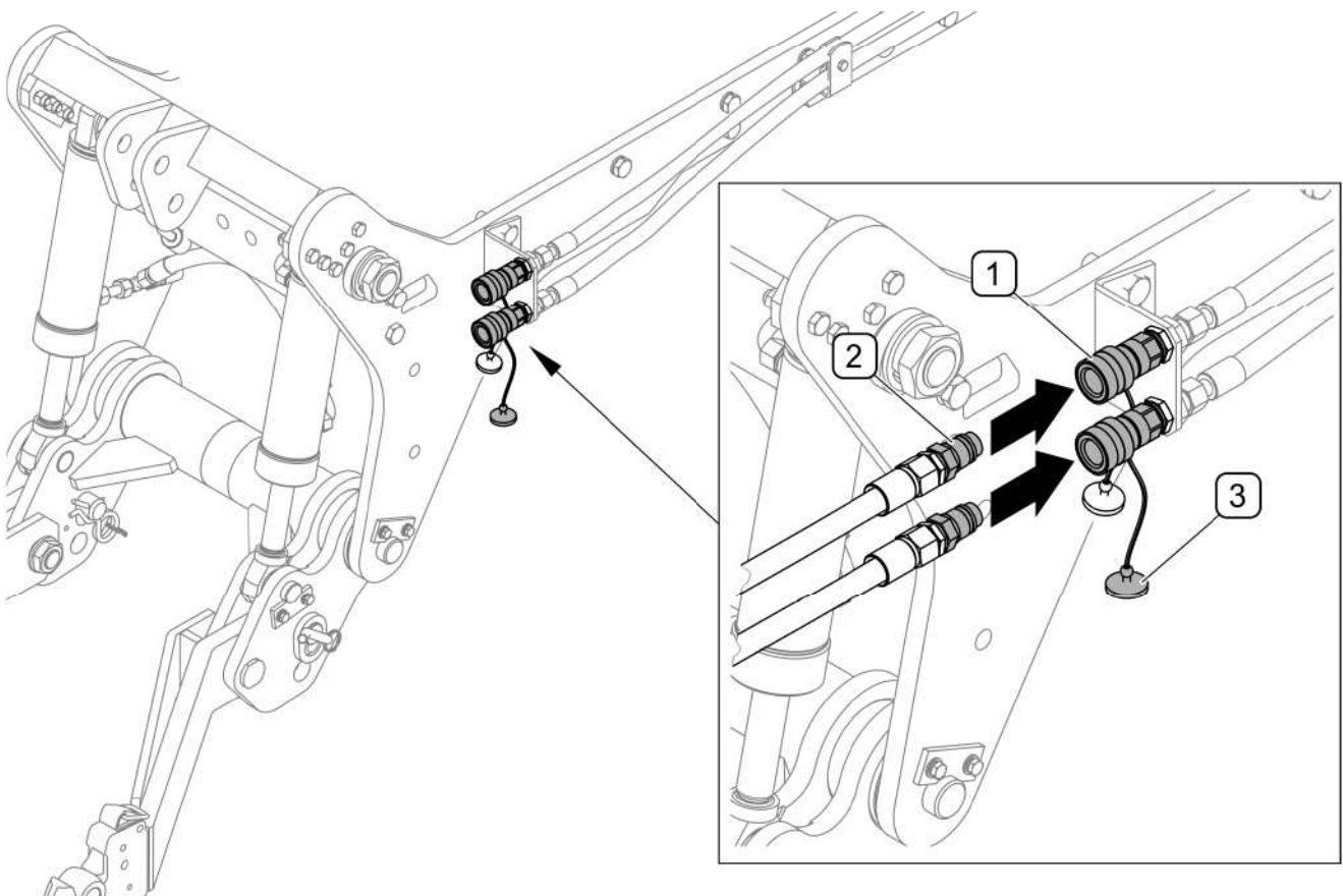
RYSUNEK 4.16 Podłączenie instalacji hydraulicznej maszyny
