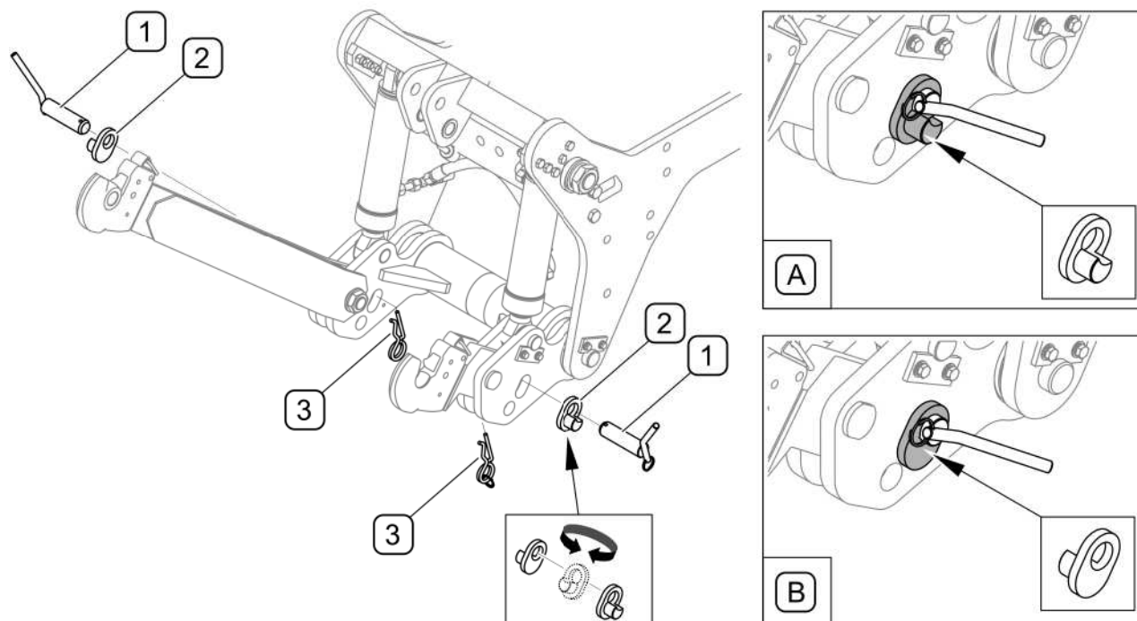
RYСУNEK 4.13 Pozycja pływająca cięgieł dolnych
