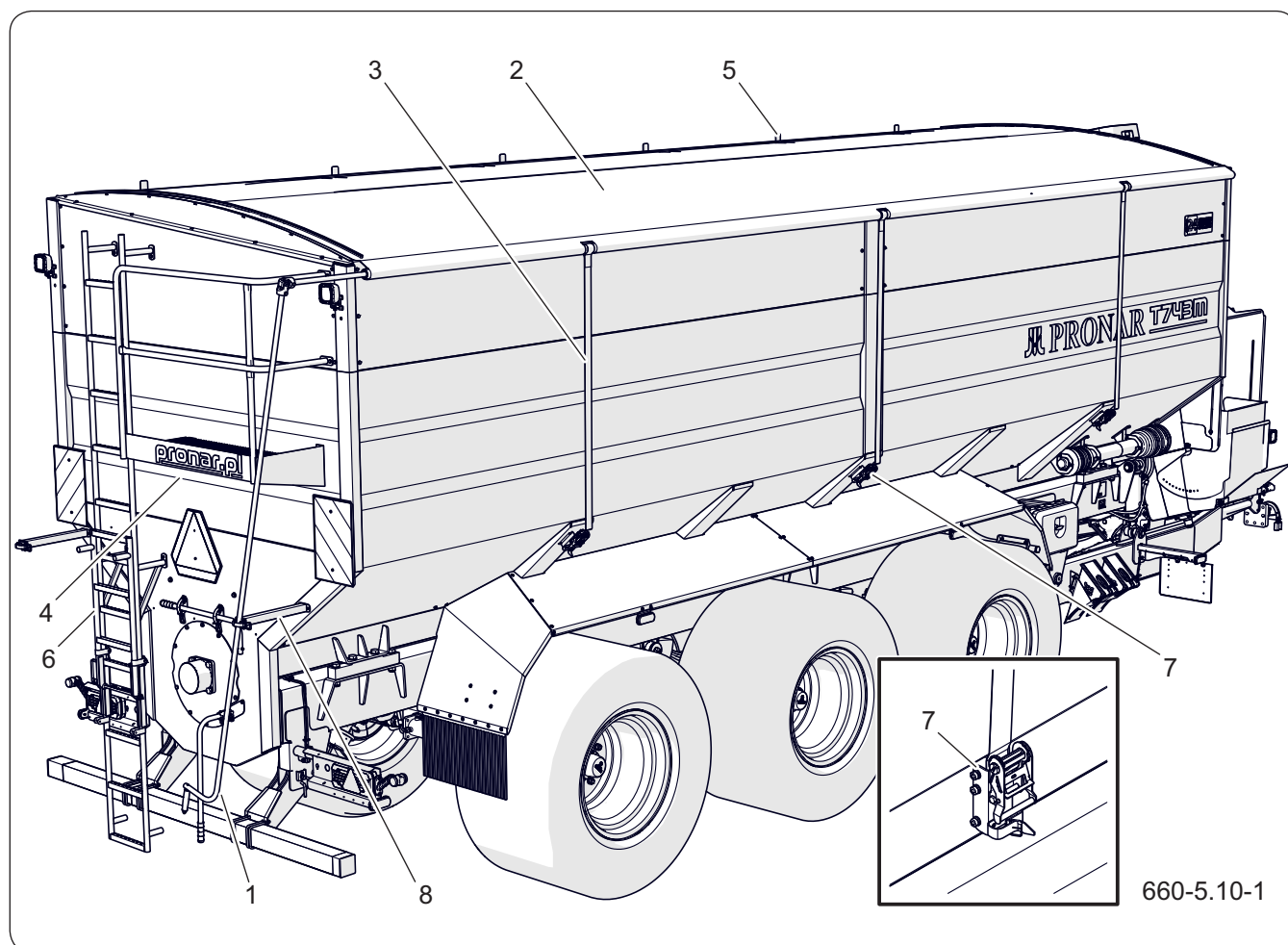
Рисунок 5.14 Работа с рулонным брезентом
