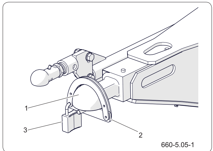
Рисунок 5.4 Защита тяги дышла
