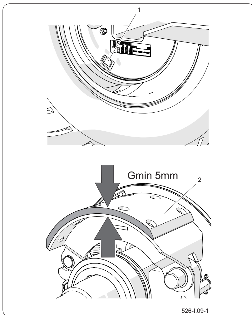
Рисунок 6.11 Проверка толщины тормозных накладок
