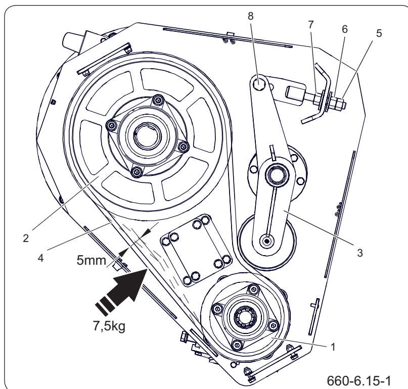
Рисунок 6.10 Ременная передача
