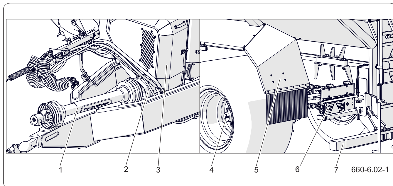
Рисунок 6.3 Крышки прицепа
