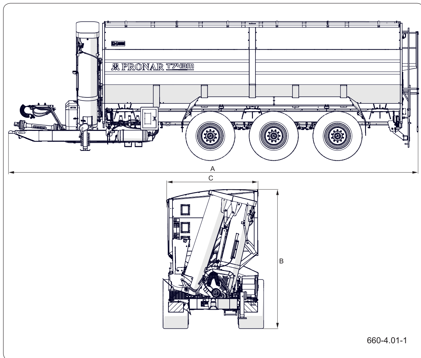
Рисунок 4.1 Основные размеры прицепа
