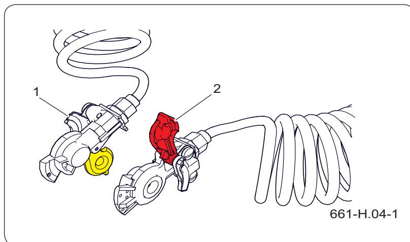
Рисунок 5.5 Линии пневматической тормозной системы
