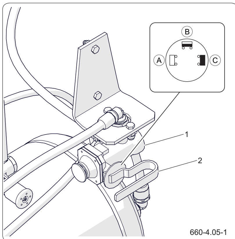
Рисунок 4.5 Ручной регулятор тормозного усилия (1) регулятор тормозных сил (2) рычаг
