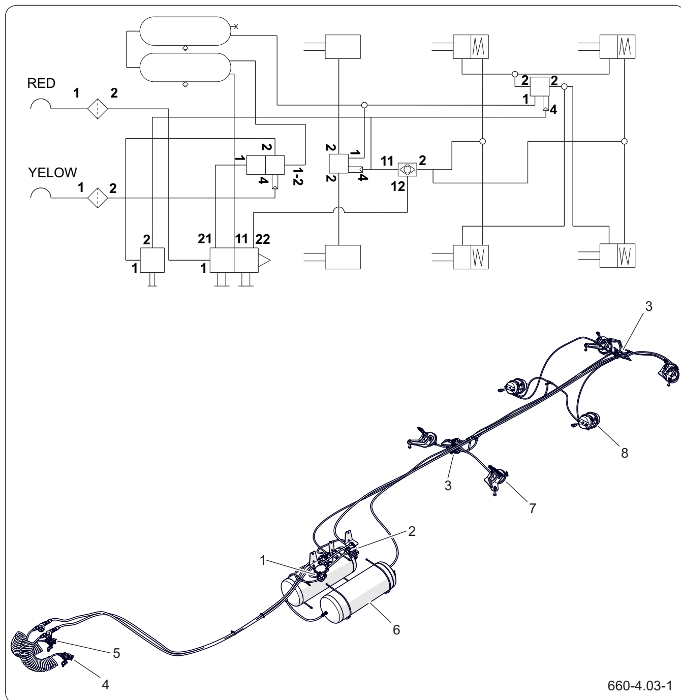
Рисунок 4.3 Схема и устройство пневматической тормозной системы с ручным регулятором тормозного усилия
