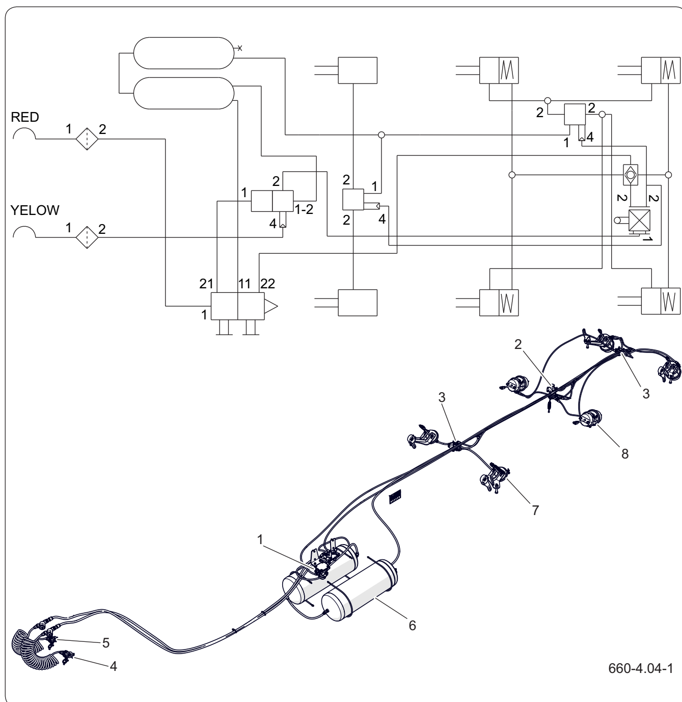
Рисунок 4.4 Схема и устройство пневматической тормозной системы с автоматическим регулятором тормозного усилия
