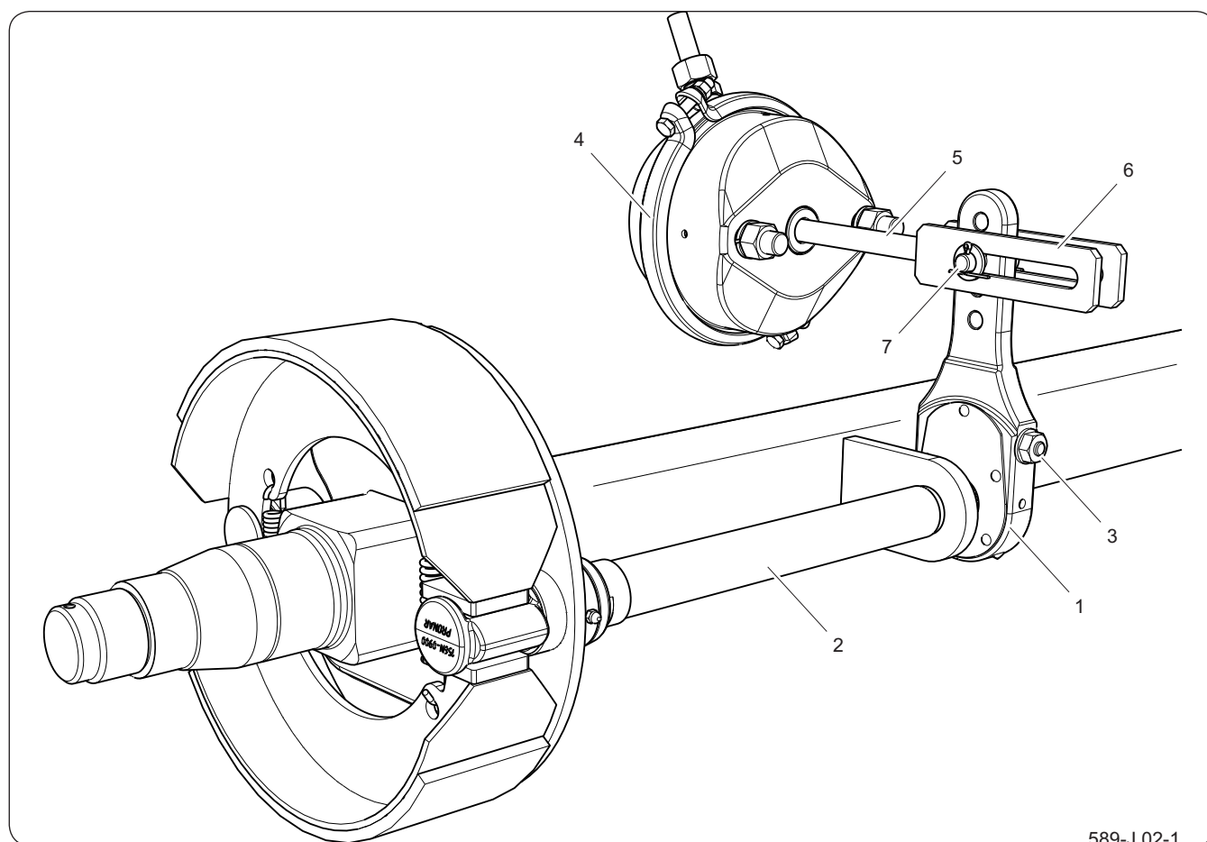
Рисунок 6.20 Конструкция пневматического тормоза ходовой оси
