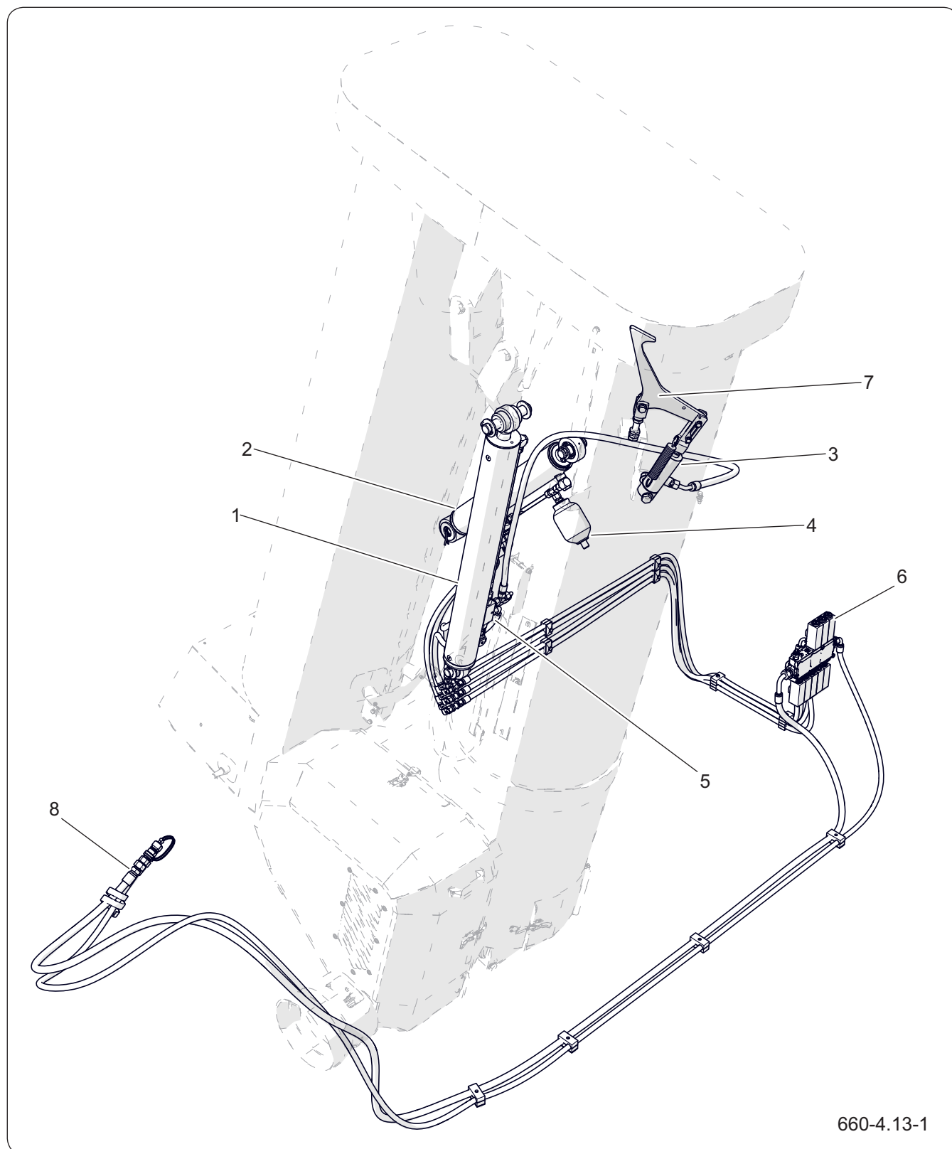
Рисунок 4.14 Конструкция гидравлической системы вертикального конвейера
