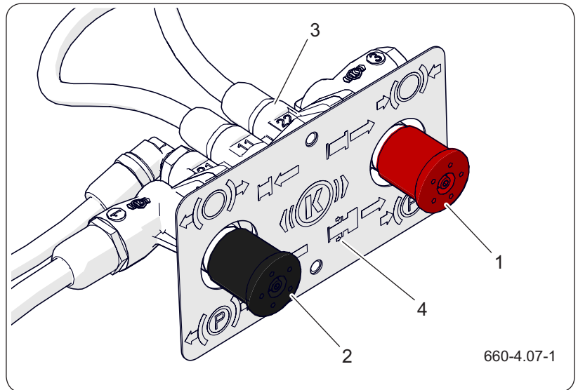
Рисунок 4.7 Выпускной и стояночный клапан
