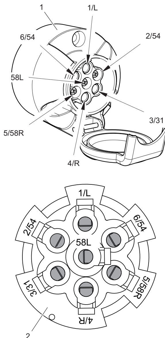
Рисунок 4.19 7-контактный разъем
