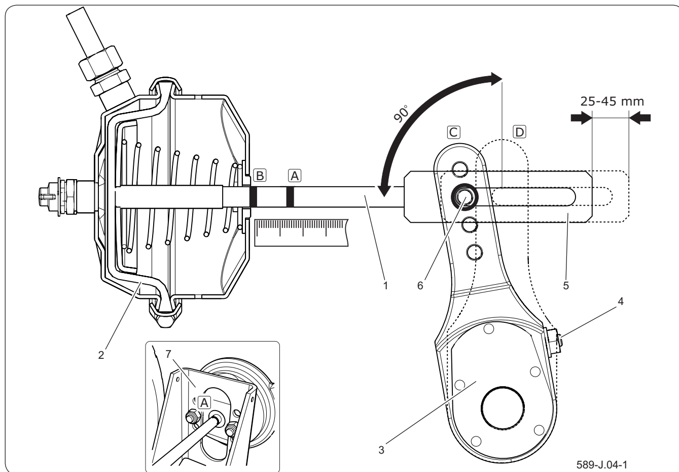
Рисунок 6.22 Принцип регулировки пневматического тормоза
