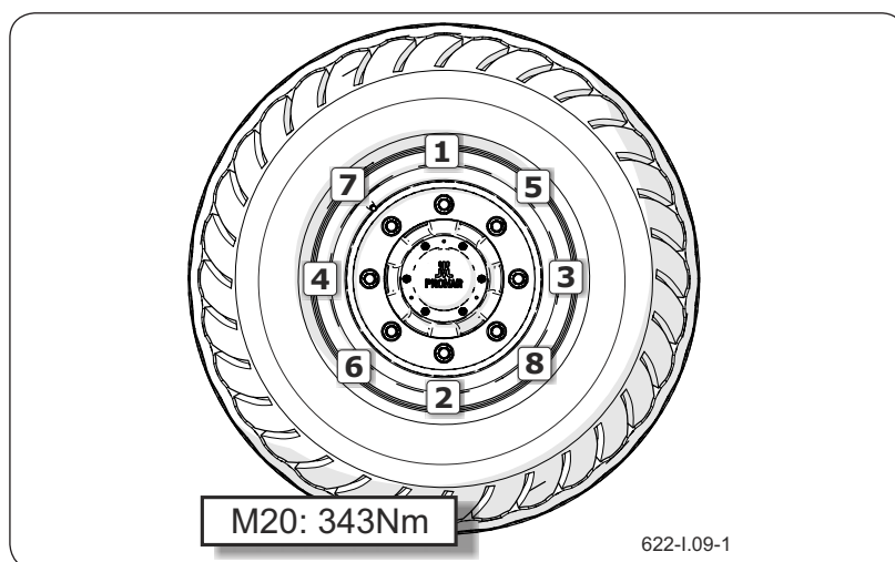
Рисунок 6.17 Очередность завинчивания гаек (8 штук)
