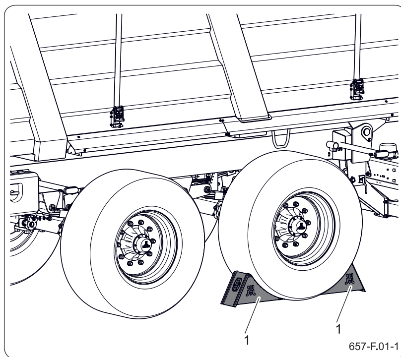
Рисунок 3.1 Положение блокирующих клиньев (1) упорный клин
