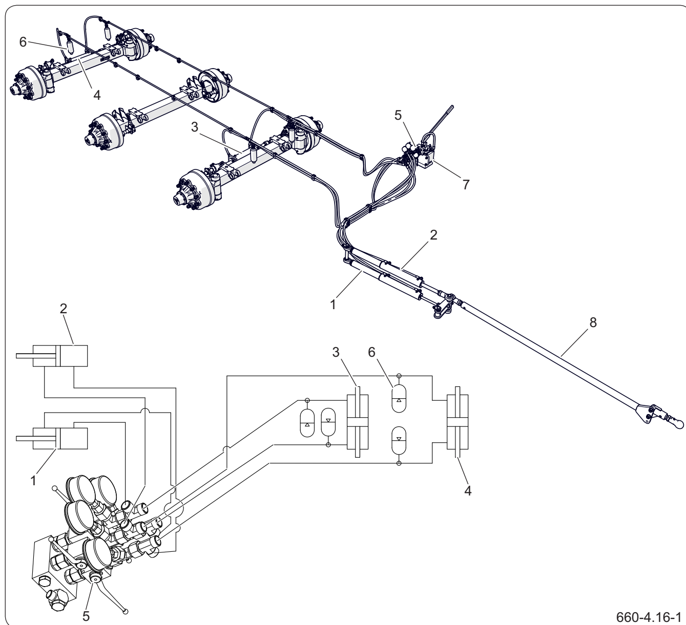
Рисунок 4.17 Конструкция и схема гидравлической установки управления
