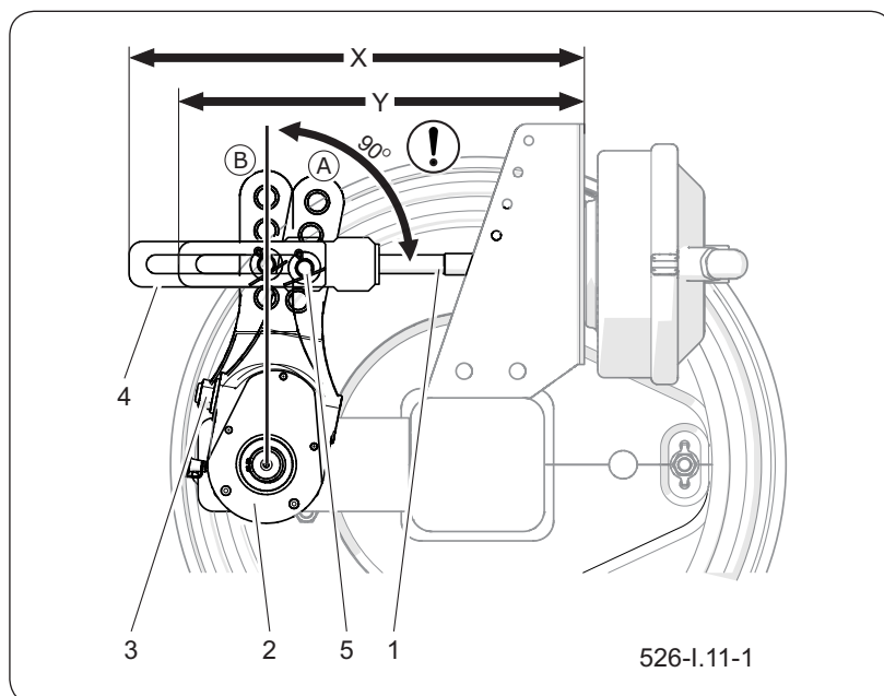
Рисунок 6.13 Проверка тормоза
