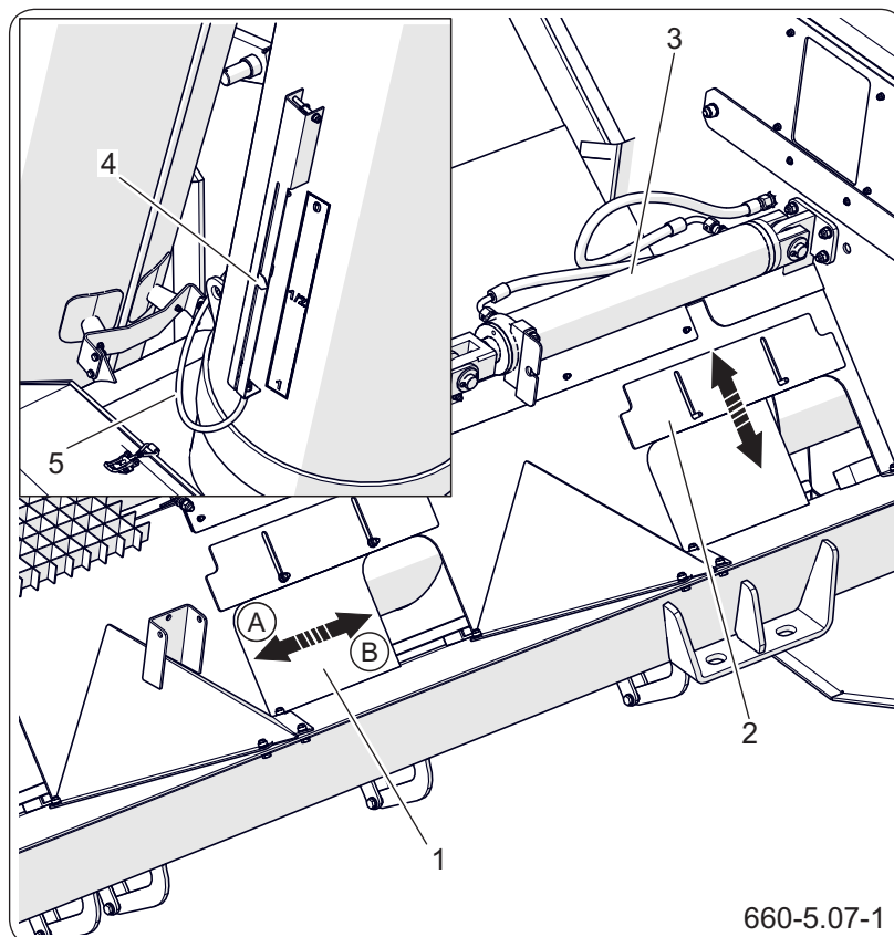
Рисунок 5.11 Затворы напольного конвейера
