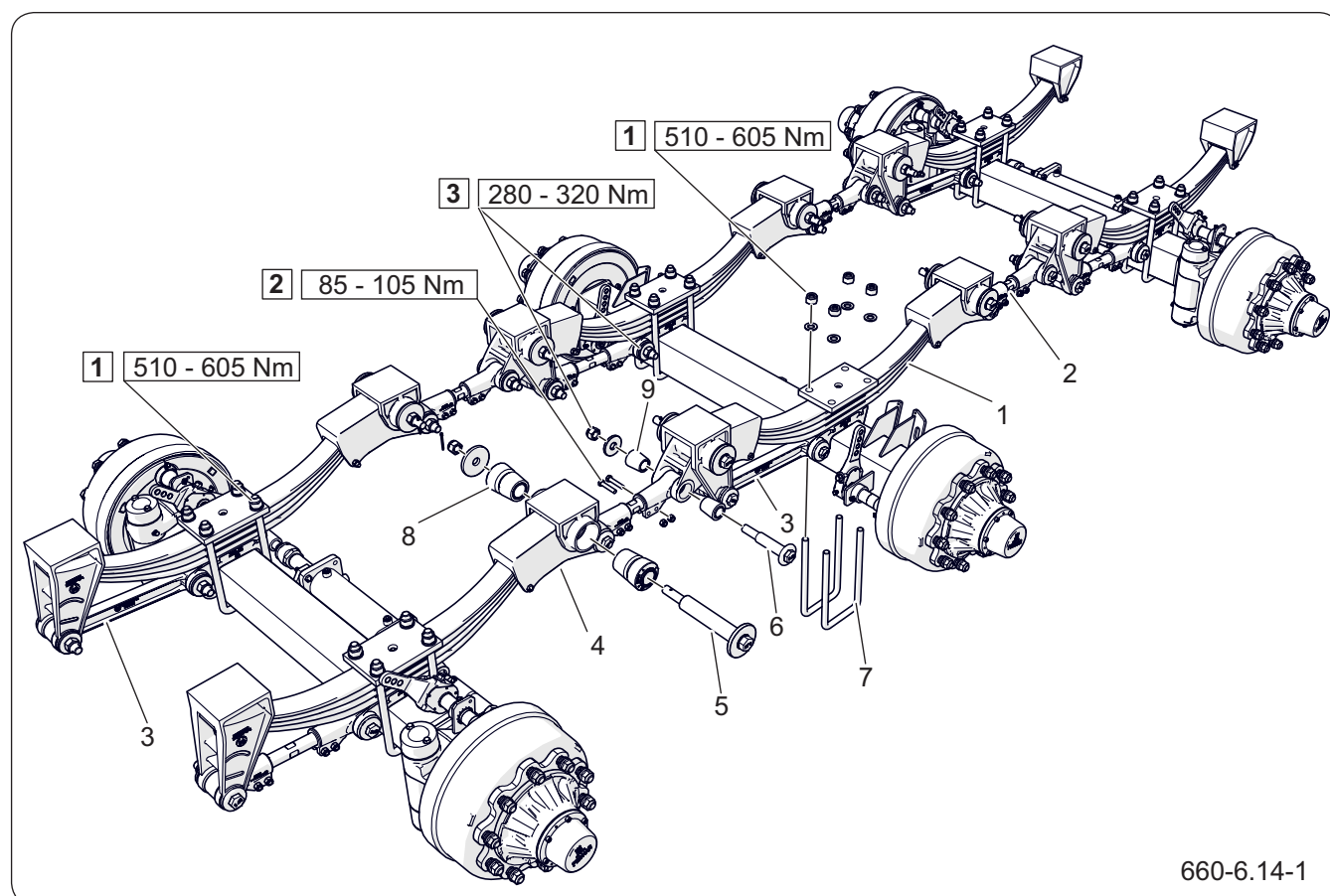
Рисунок 6.18 Работа механической подвески тридем, ось установлена под рессорой (1) ) пружина, (2) регулируемое соединение, (3) жесткое соединение, (4) рычаг, (5) «шпилька» подвески, (6) крепление рессоры, (7) винт крепления оси «U», (8) (9) металлорезиновая втулка
