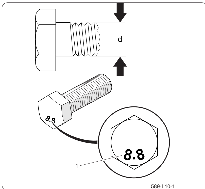
Рисунок 6.15 Болт с метрической резьбой (1) класс прочности, (d) диаметр резьбы
