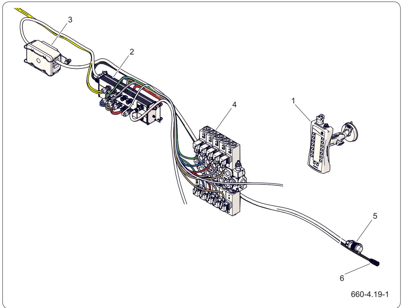
Рисунок 4.20 Элементы электрической установки управления
