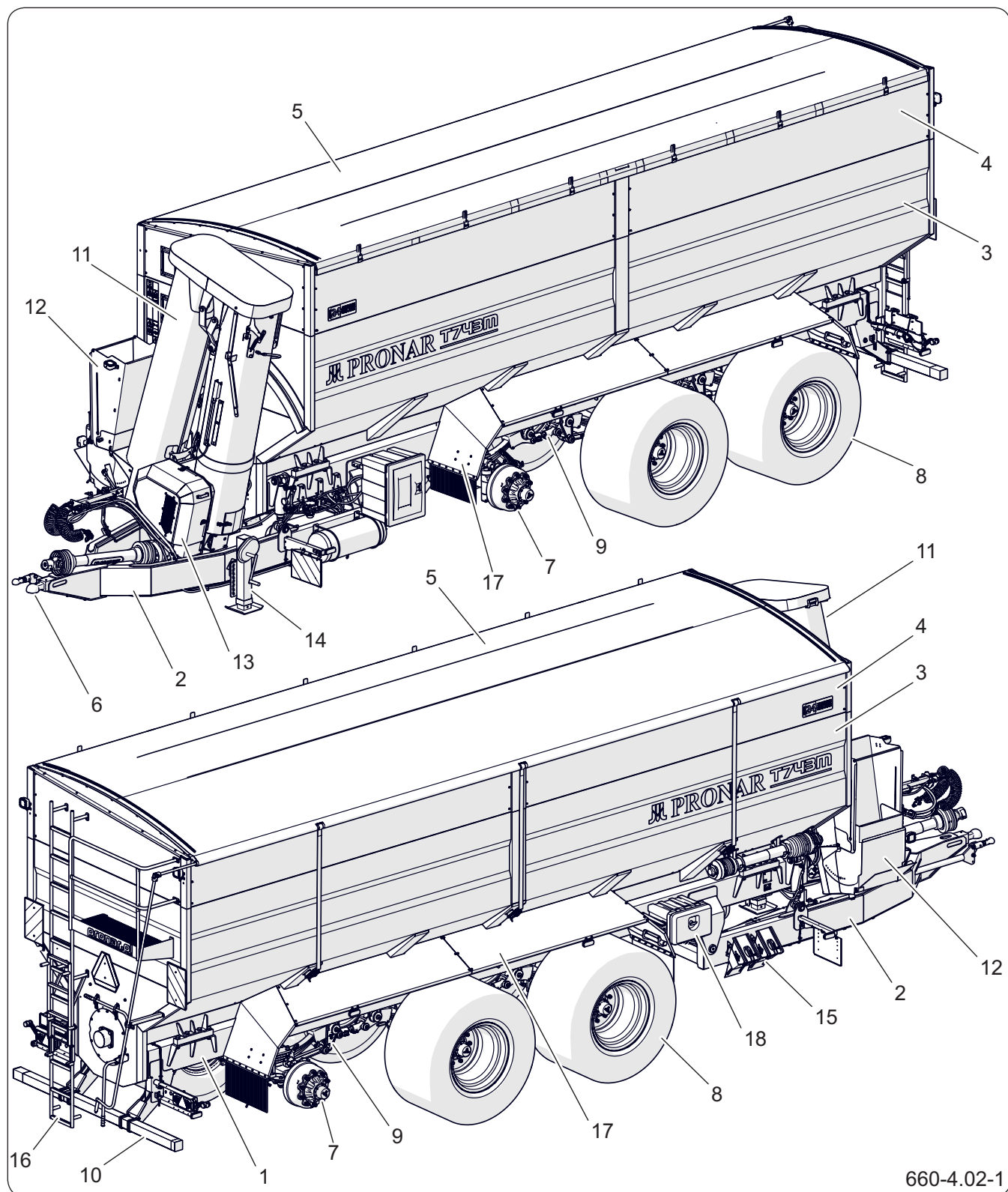
Рисунок 4.2 Конструкция воза-перегрузчика
