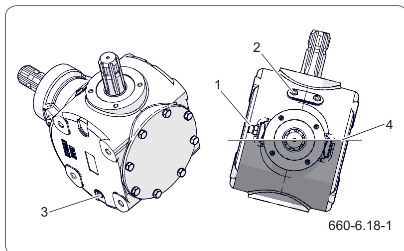
Рисунок 6.7 Коническая передача
