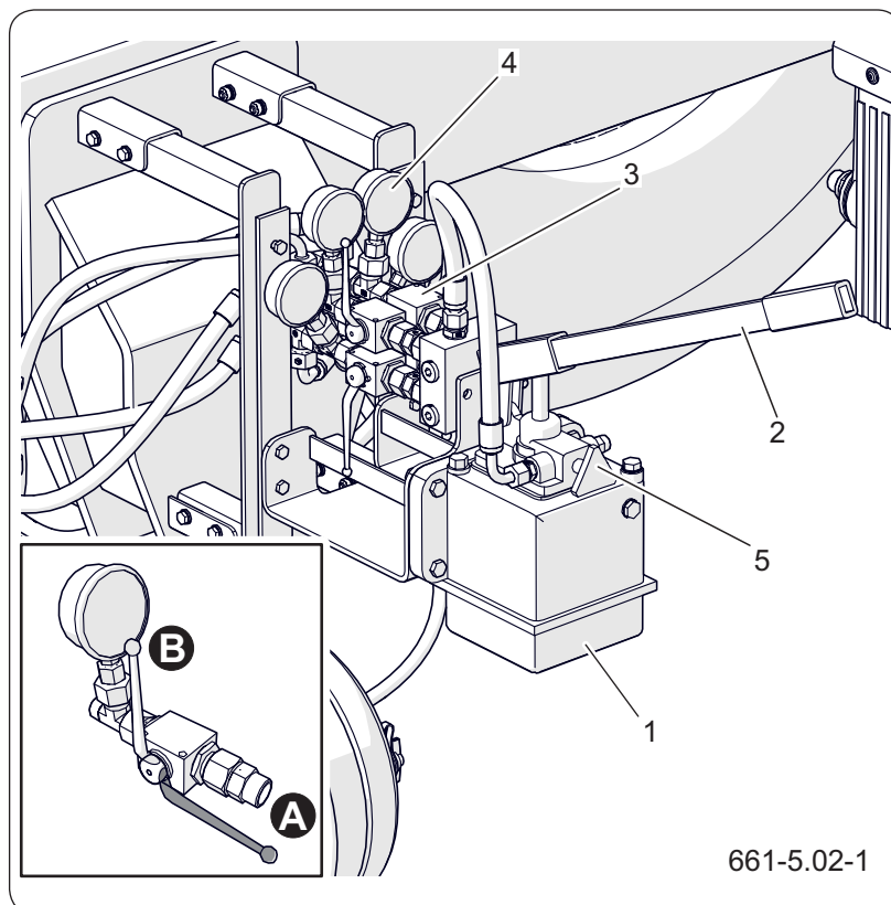
Рисунок 5.9 Настройка системы поворота оси
