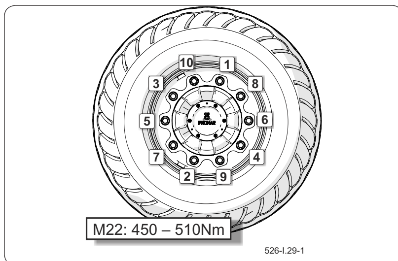
Рисунок 6.16 Очередность завинчивания гаек (10 штук)
