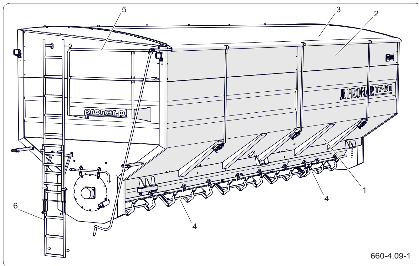
Рисунок 4.9 Грузовой контейнер
