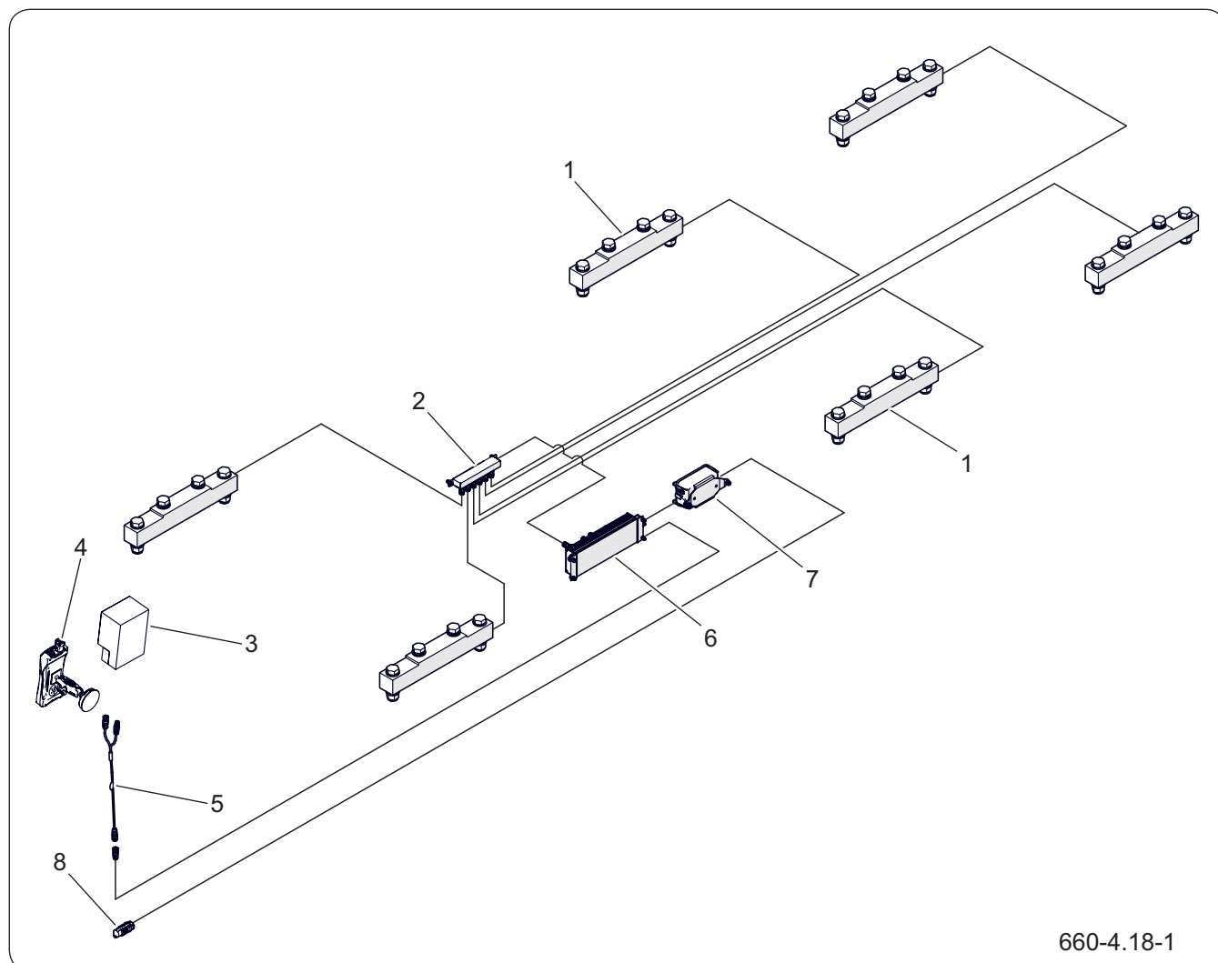
Рисунок 4.21 Весы с принтером
