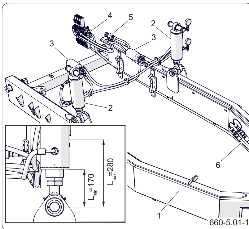
Рисунок 5.1 Регулировка высоты дышла
