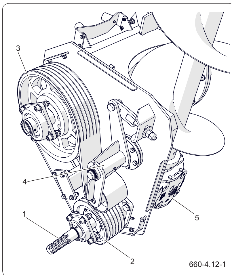
Рисунок 4.12 Главная передача
