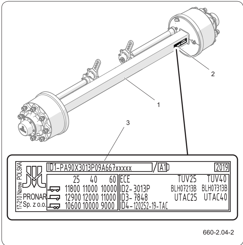
Рисунок 2.3 Идентификация оси
