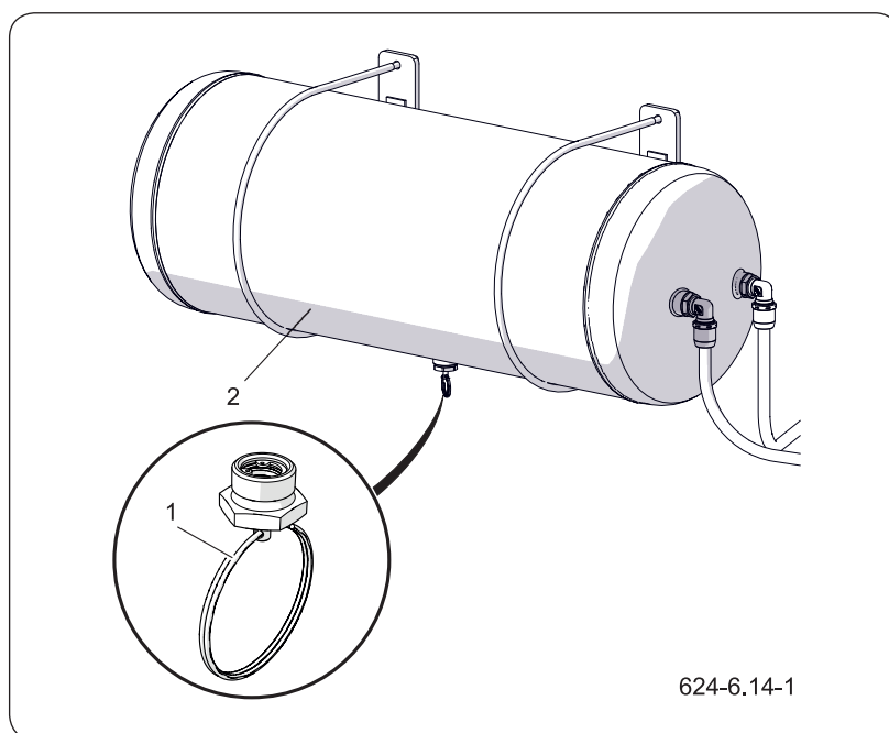
Рисунок 6.9 Емкость для сжатого воздуха (1) конденсатоотводящий клапан (2) бачок
