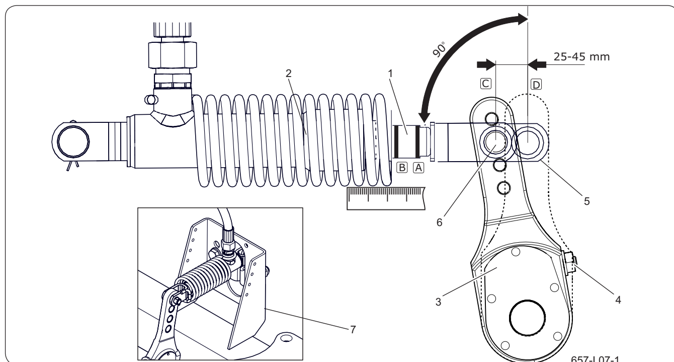
Рисунок 6.23 Принцип регулировки гидравлического тормоза
