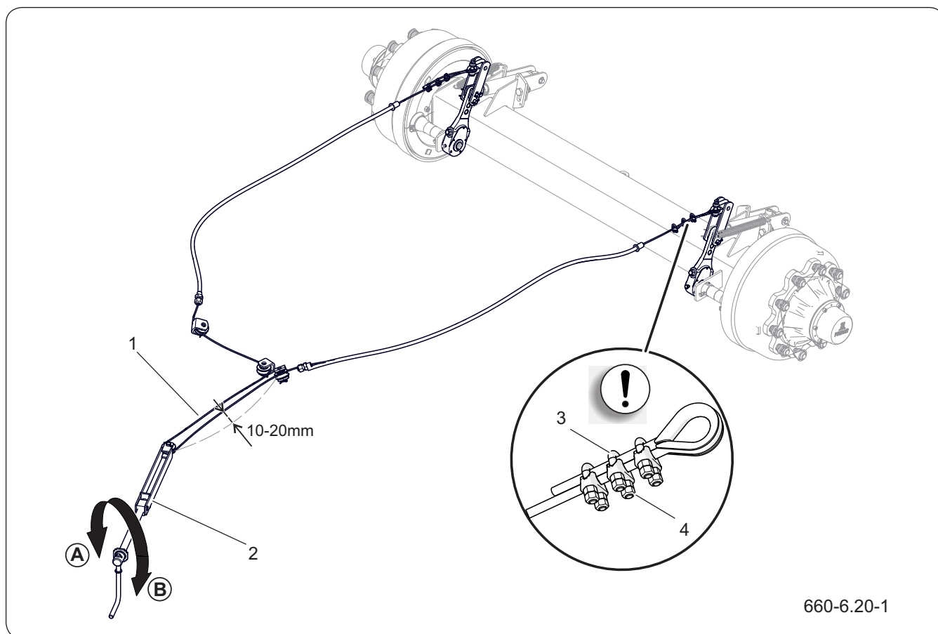
Рисунок 6.14 Проверка натяжения троса
