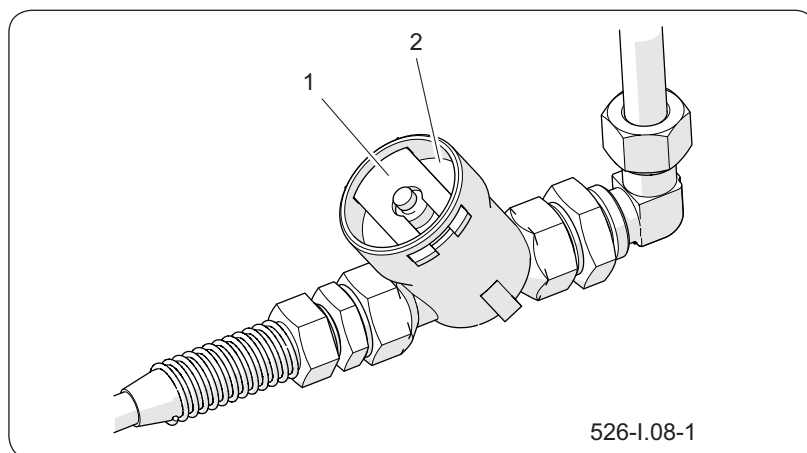
Рисунок 6.8 Воздушный фильтр
