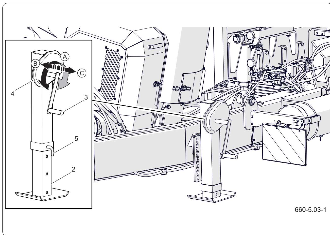
Рисунок 5.2 Телескопическая опора
