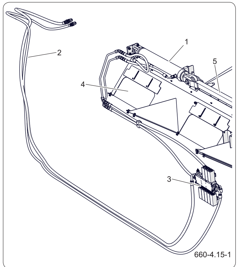
Рисунок 4.16 Гидравлическая установка задвижки
