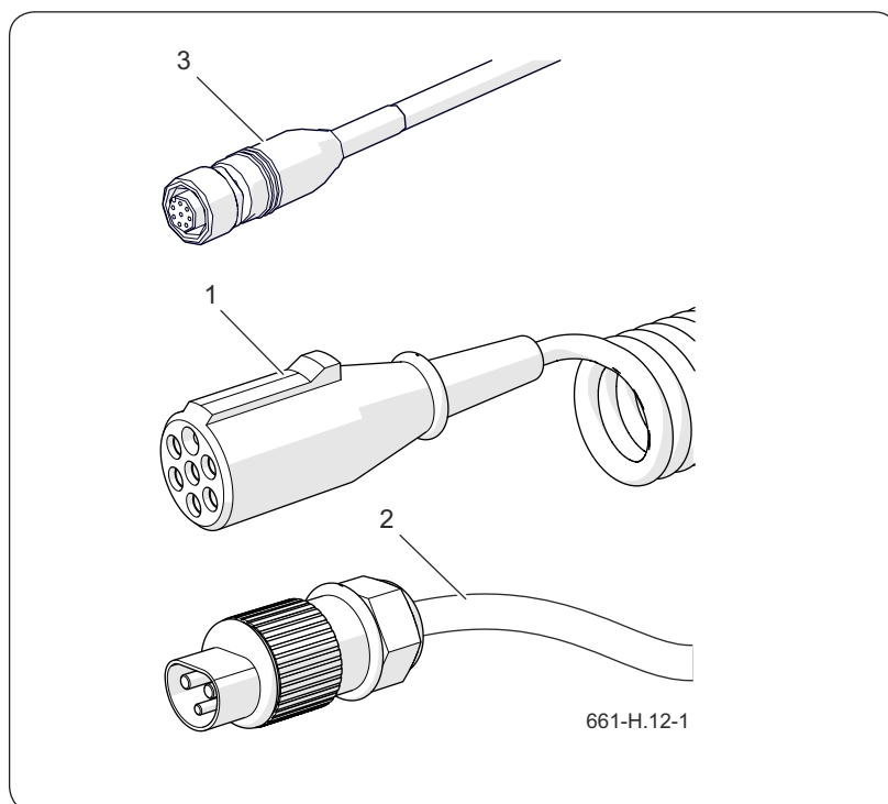
Рисунок 5.8 Электрические подключения (1) 7-контактный кабель (2) 3-контактный кабель (3) кабель пульта дистанционного управления
