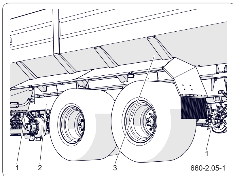
Рисунок 2.6 Точки крепления
