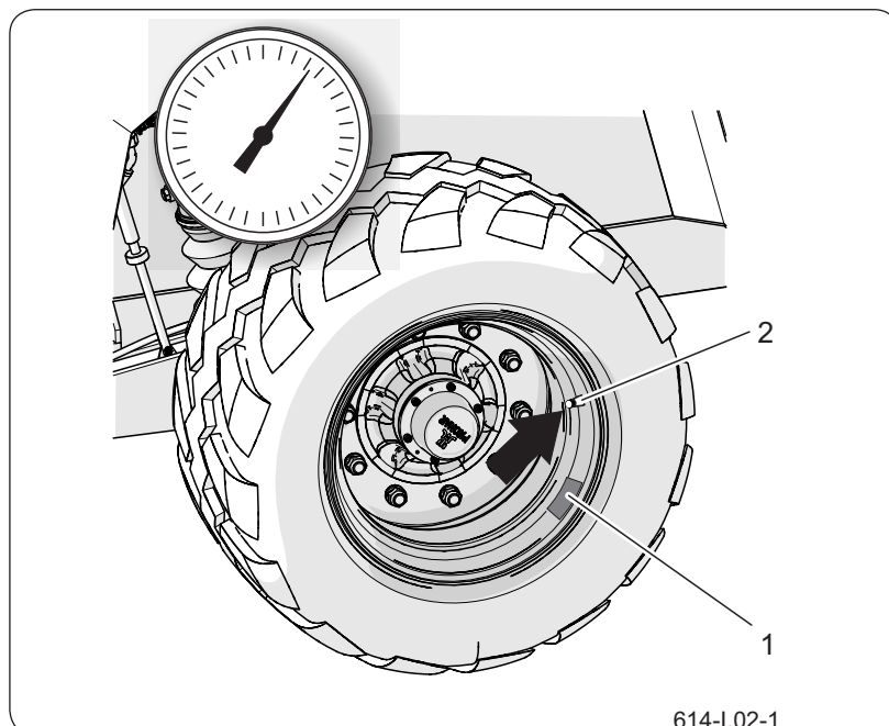
Рисунок 6.6 Колесо прицепа
