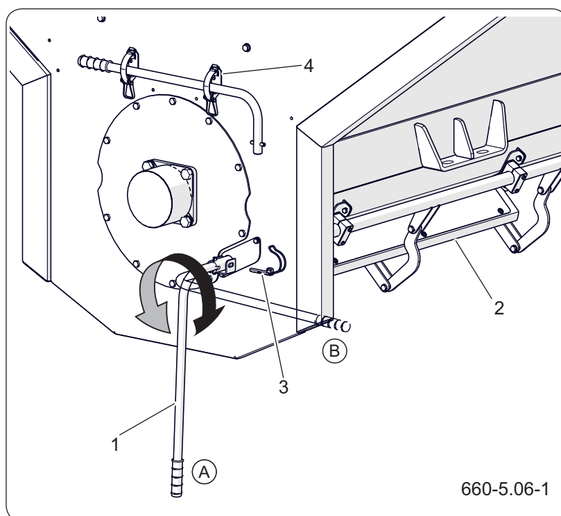
Рисунок 5.10 Сбрасывающие заслонки
