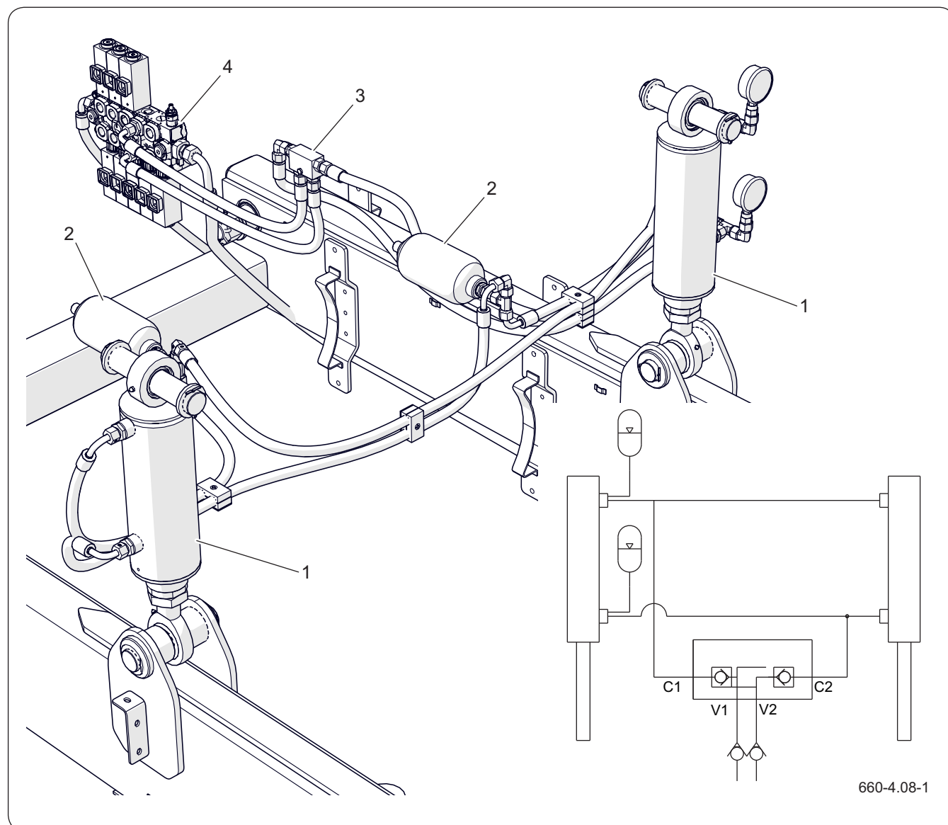
Рисунок 4.13 Конструкция и схема гидравлической установки дышла
