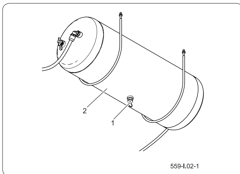
Рисунок 6.1 Емкость для сжатого воздуха
