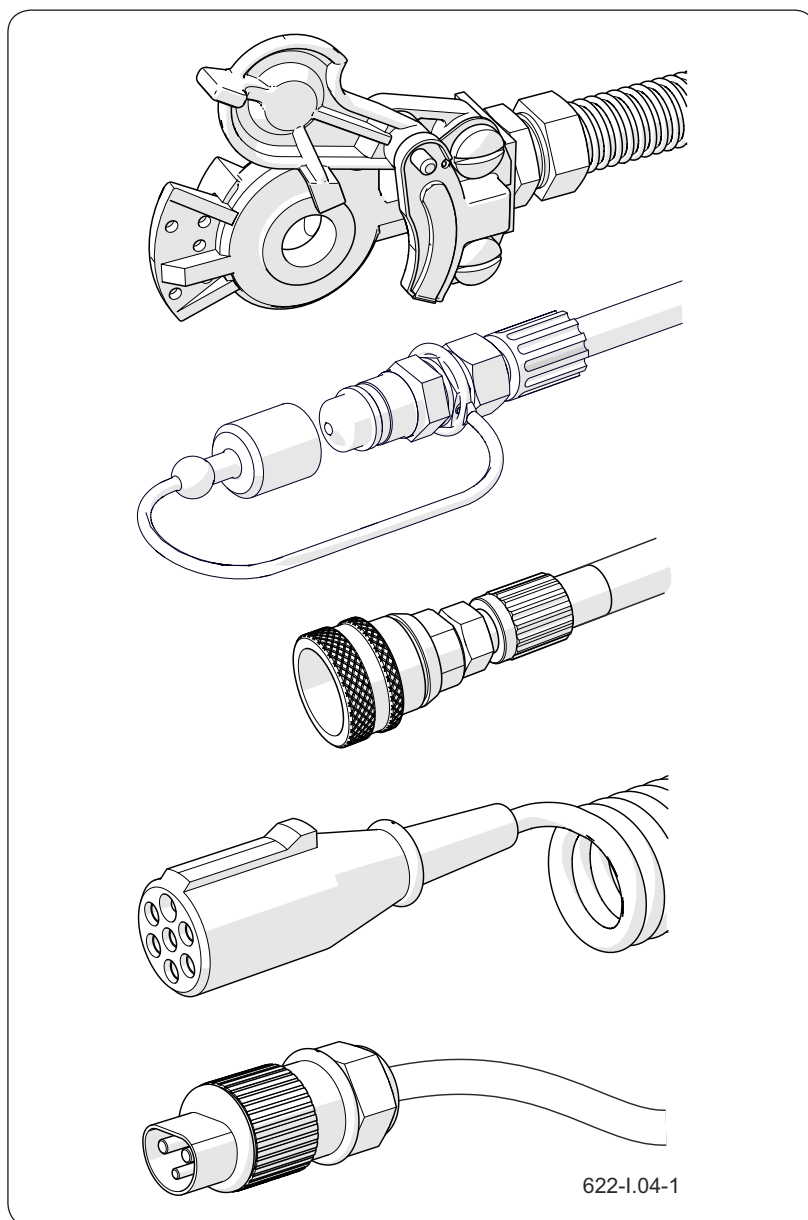
Рисунок 6.4 Примеры подсоединения прицепа
