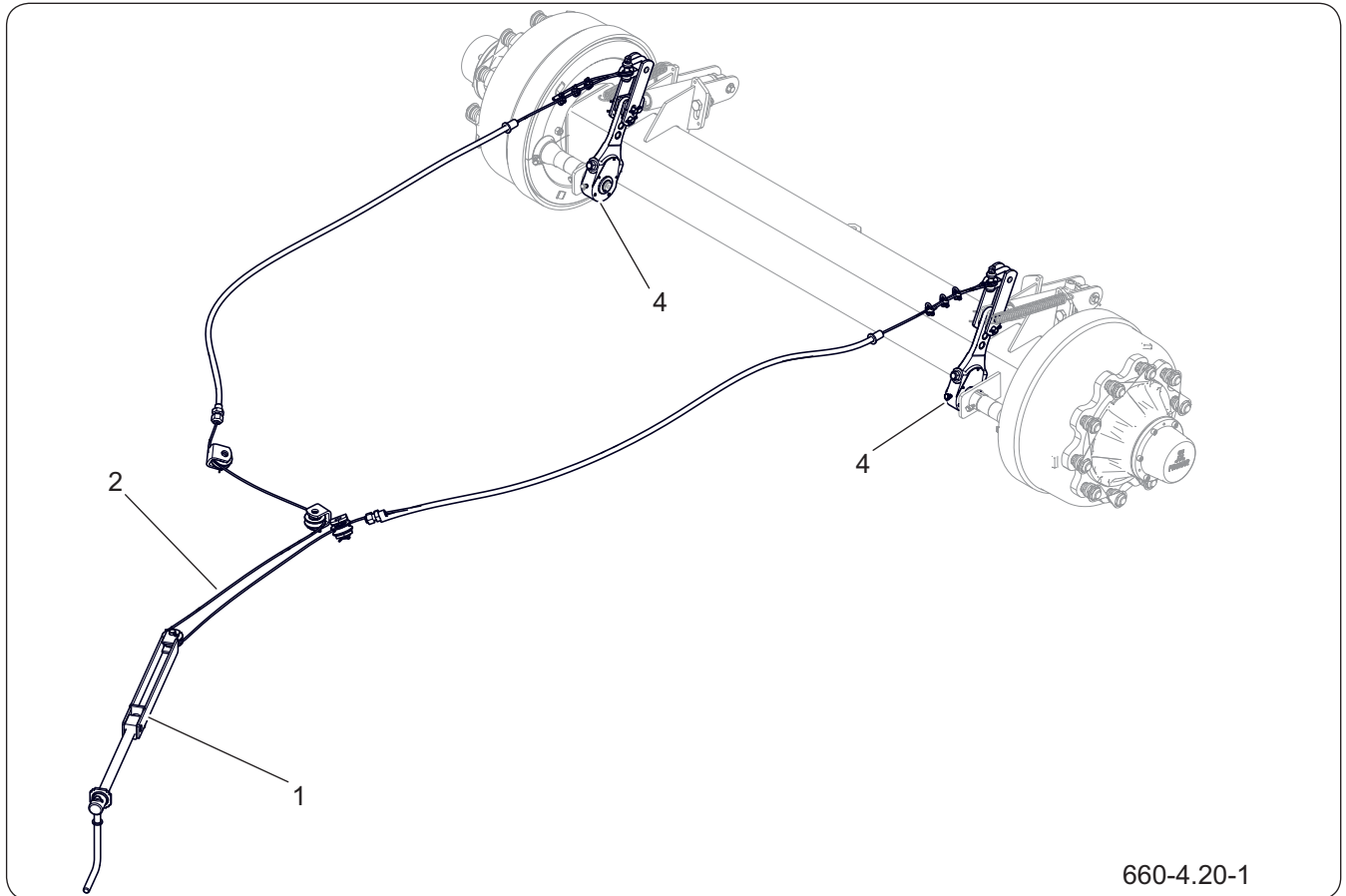
Рисунок 4.8 Конструкция стояночного тормоз
