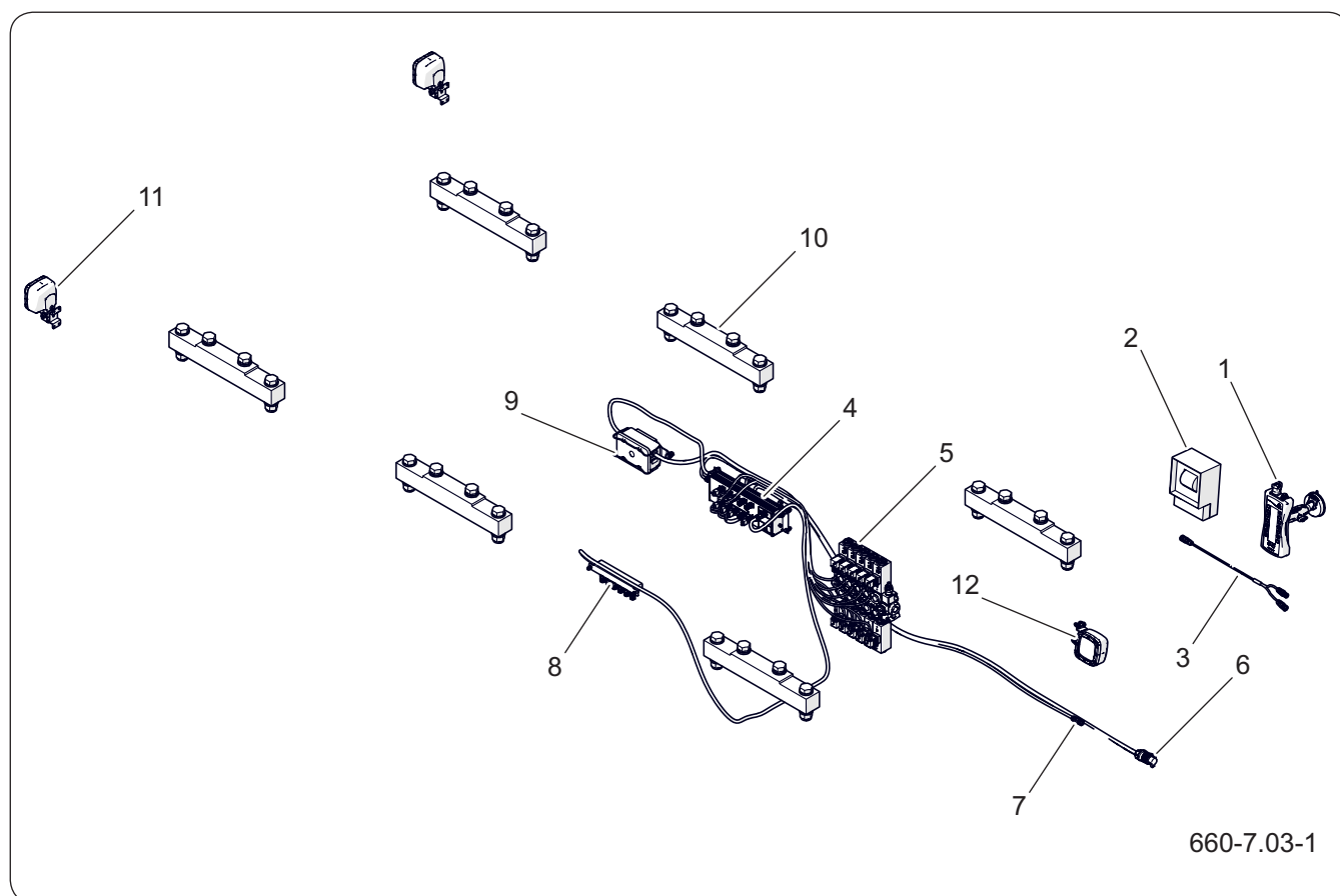
Рисунок 7.1 Элементы электрической установки управления
