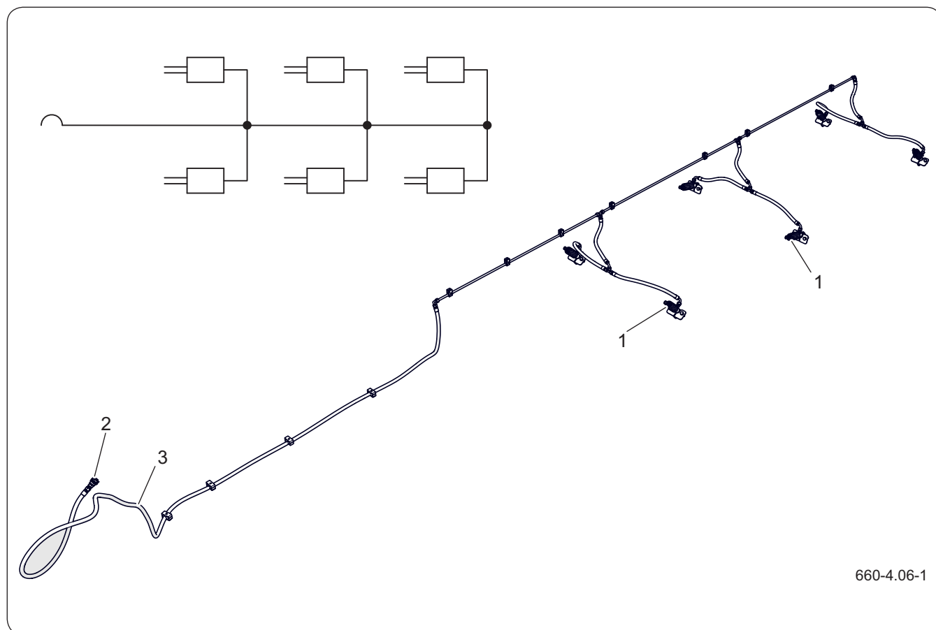
Рисунок 4.6 Схема и устройство гидравлической тормозной системы
