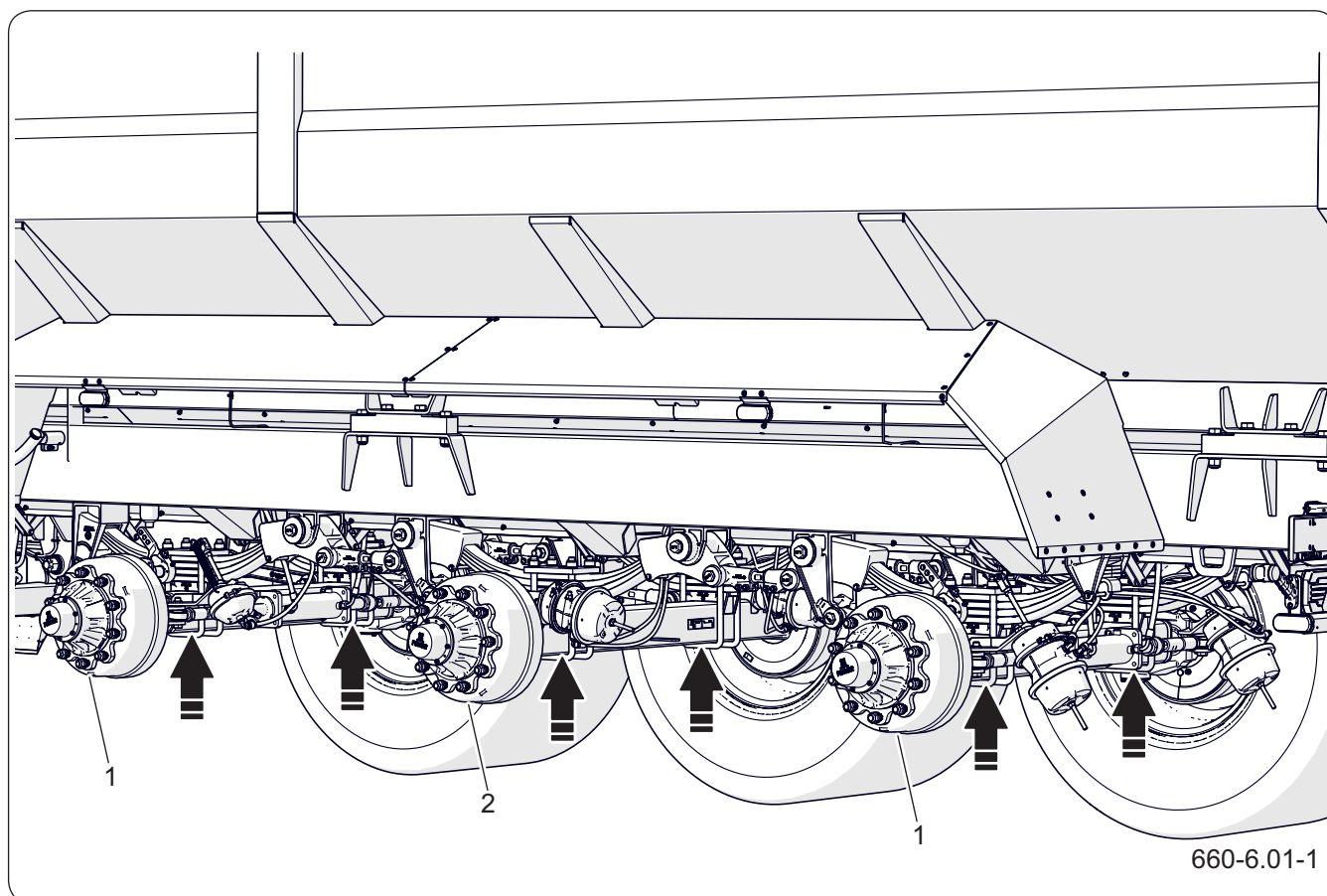
Рисунок 6.2 Рекомендуемые точки опоры прицепа
