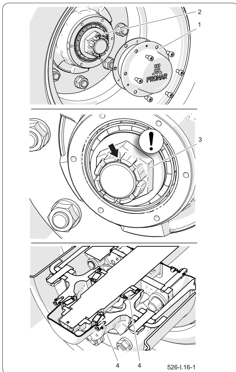
Рисунок 6.19 Правила регулировки зазора в подшипниках
