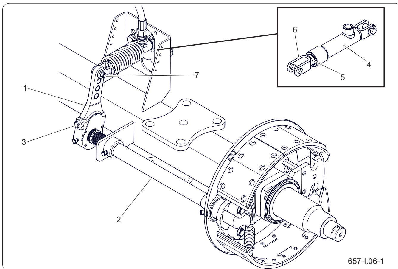
Рисунок 6.21 Конструкция гидравлического тормоза ходовой оси
