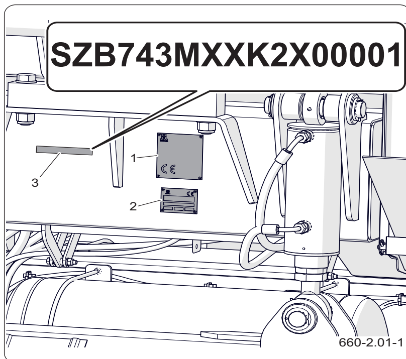
Рисунок 2.1 Идентификация прицепа
