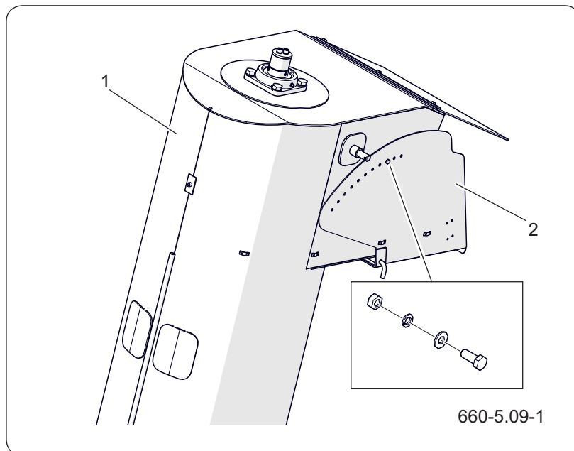
Рисунок 5.13 Желоб конвейера
