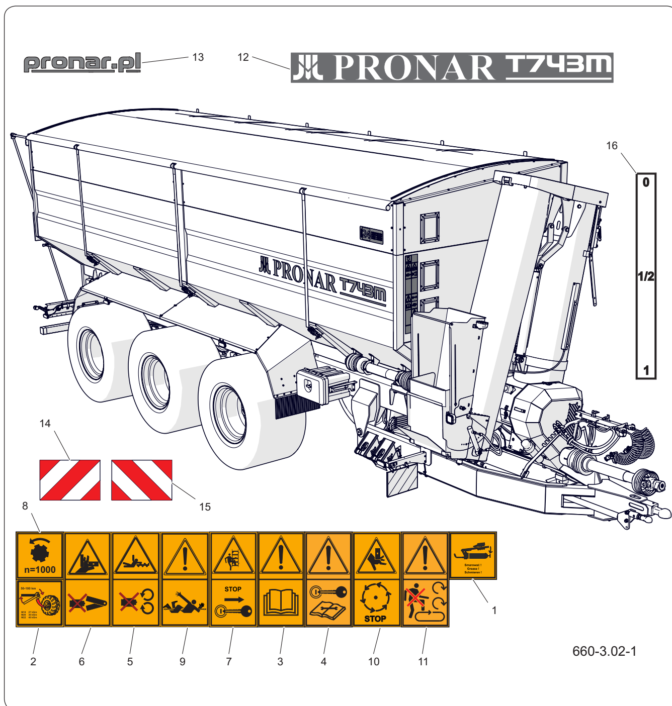
Рисунок 3.3 Расположение информационных и предупреждающих наклеек
