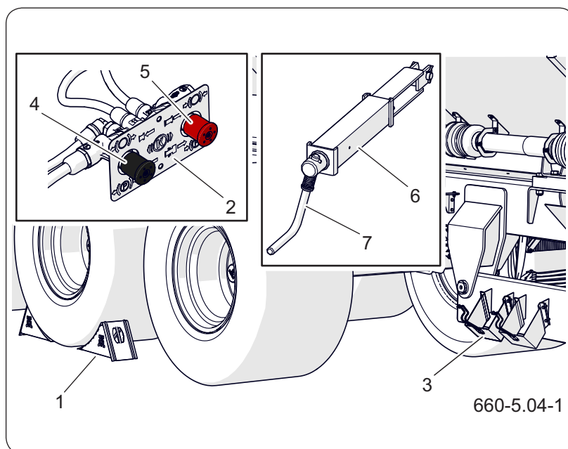
Рисунок 5.3 Стояночный тормоз
