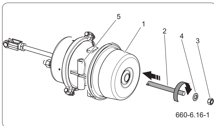
Рисунок 6.24 Аварийный выпуск тормозного цилиндра
