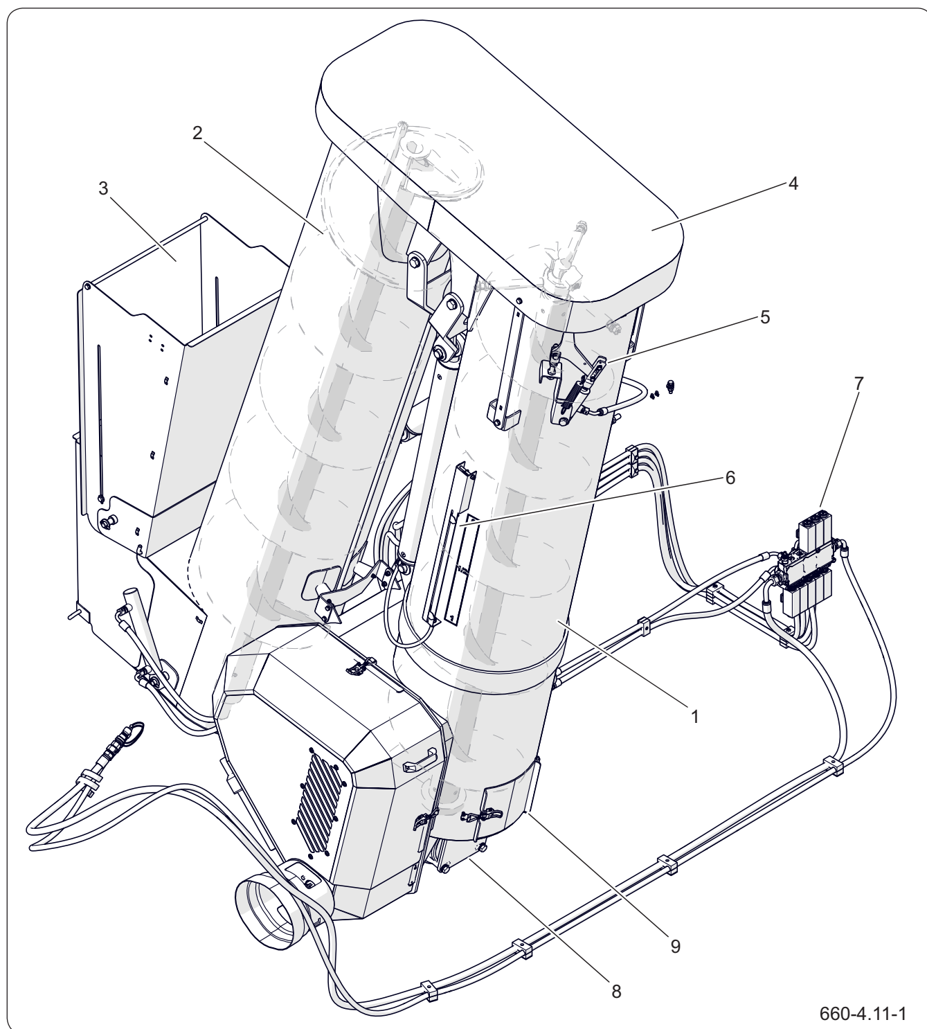
Рисунок 4.11 Передний конвейер
