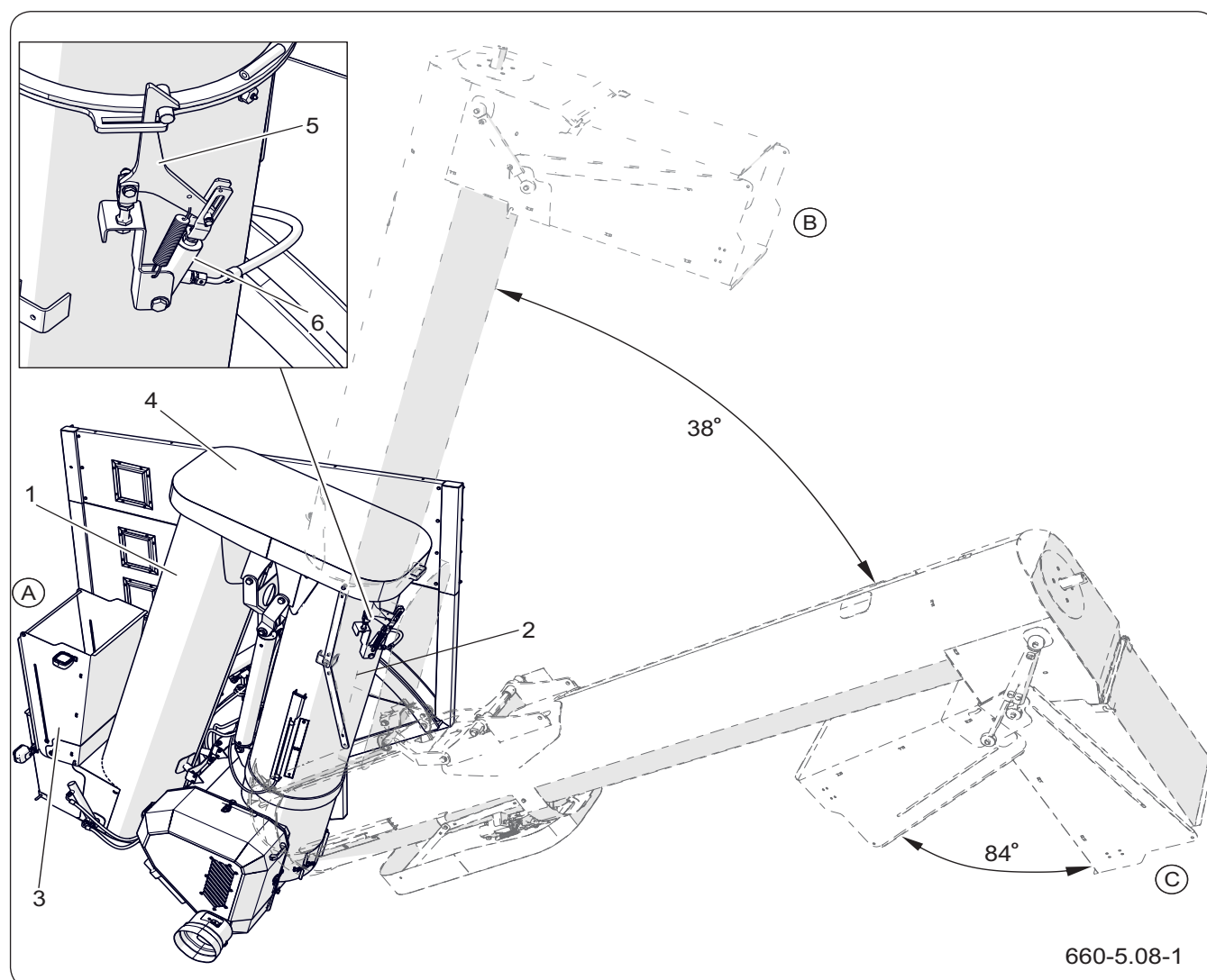
Рисунок 5.12 Вертикальный конвейер
