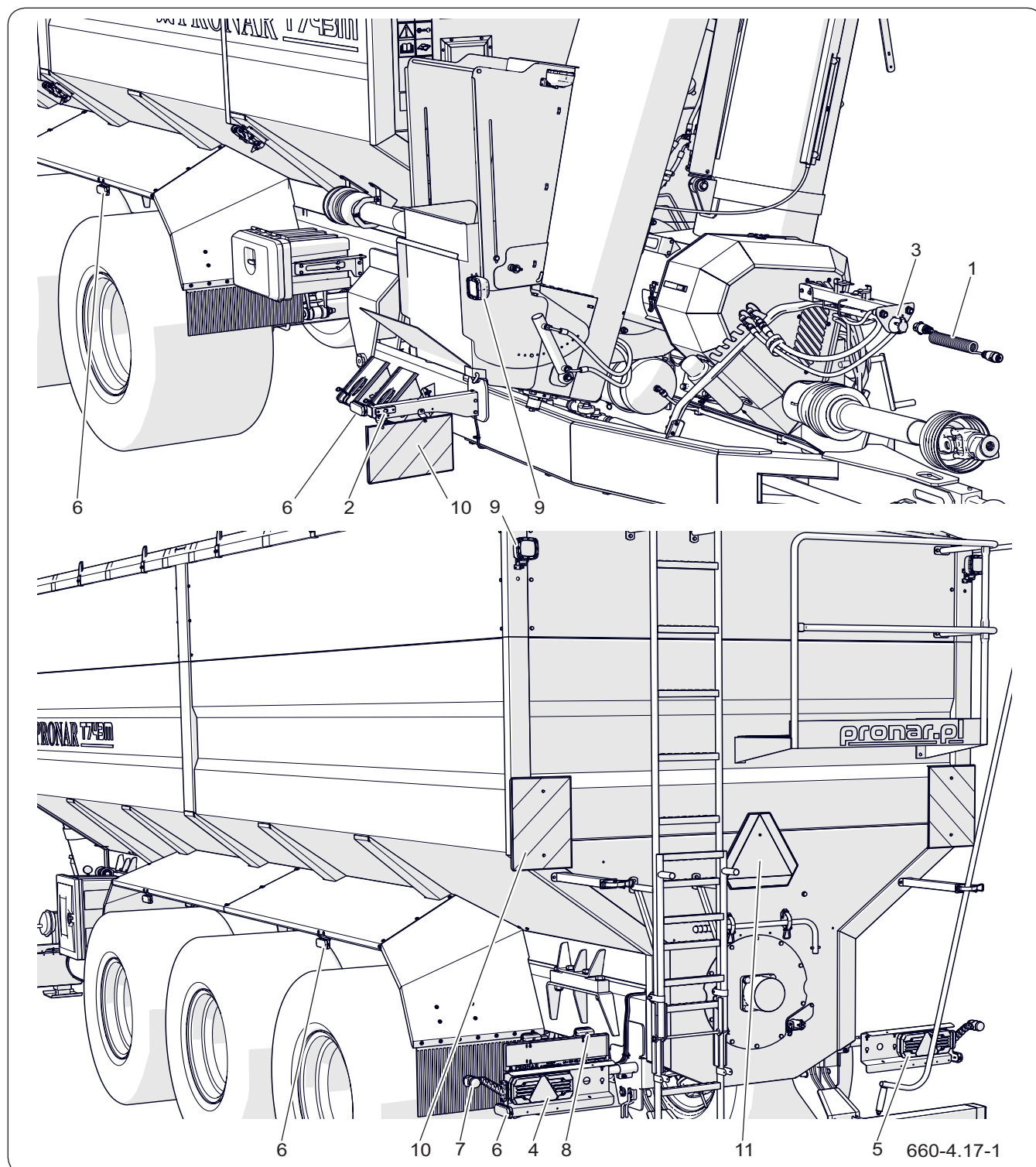
Рисунок 4.18 Расположение элементов электроустановки и светоотражающих элементов
