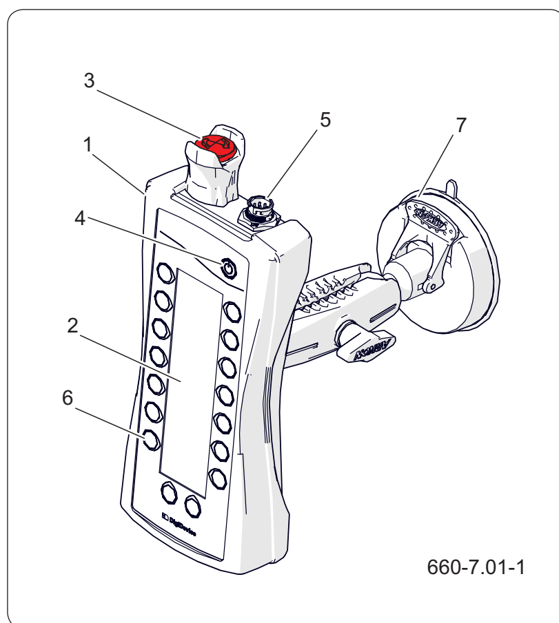
Рисунок 7.2 Пульт дистанционного управления (1) корпус (2) дисплей (3) кнопка безопасности (4) кнопка ВКЛ/ВЫКЛ (5) коммуникационный разъем (6) кнопки выбора (7) ручка
