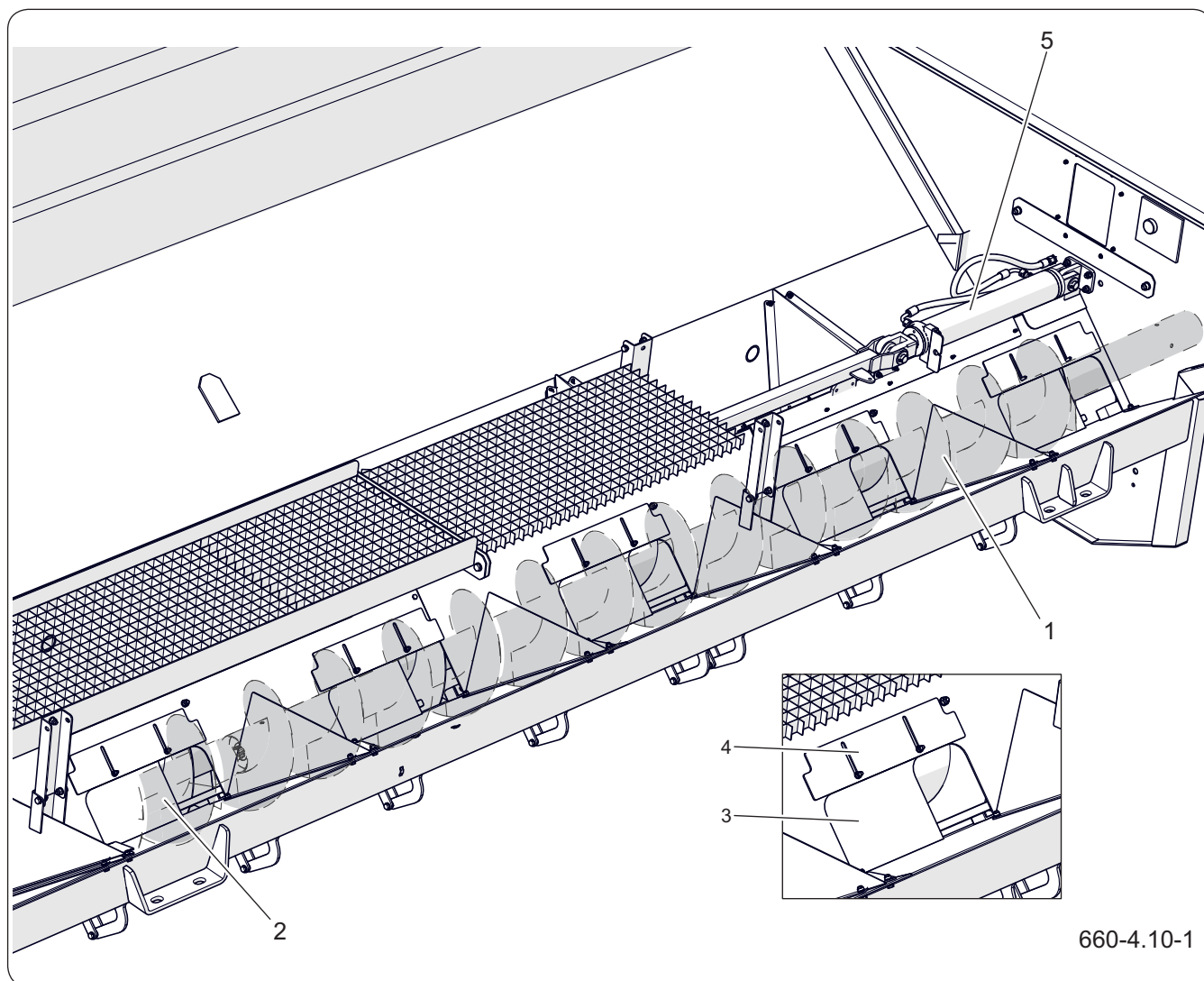
Рисунок 4.10 Напольный конвейер
