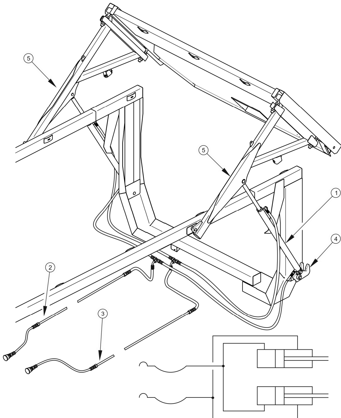
RYСУNEK 3.12 Budowa i schemat instalacji hydraulicznej klapy tylnej
