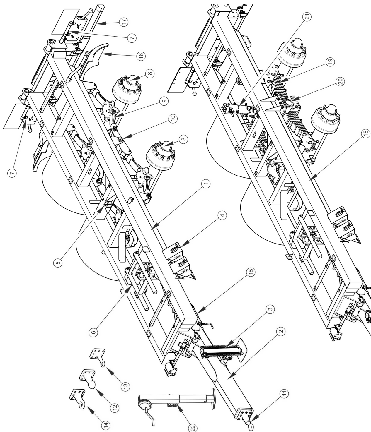
RYSUNEK 3.1 Podwozie przyczepy
