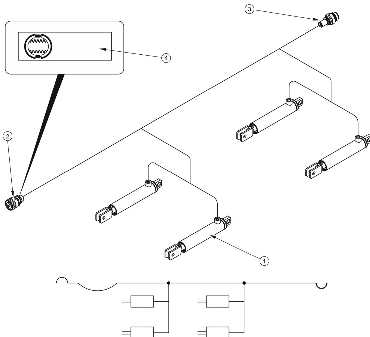
RYSUNEK 3.6 Budowa i schemat instalacji hamulcowej hydraulicznej
