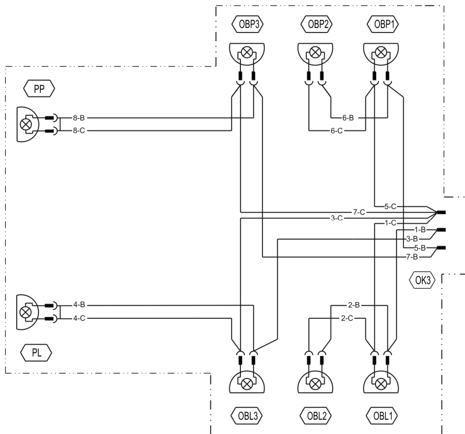
RYSUNEK 3.16 Schemat ideowy instalacji elektrycznej wiązki przedniej
