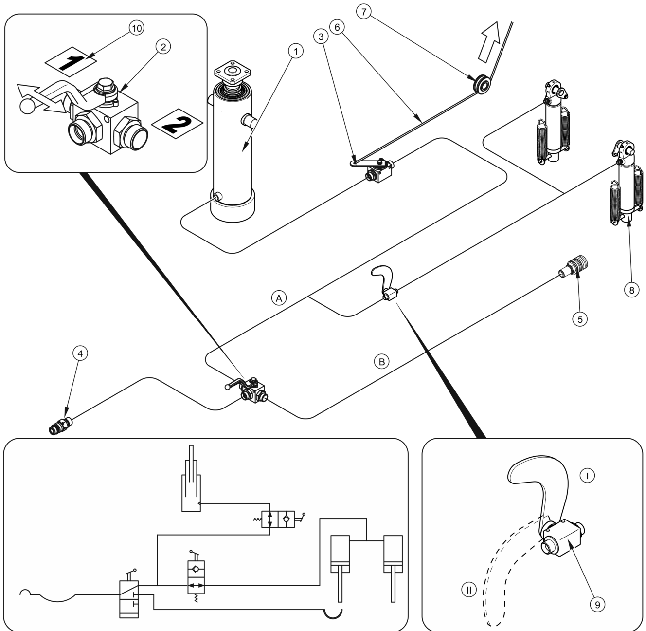
RYSUNEK 3.9 Budowa i schemat instalacji hydraulicznej wywrotu bogie
