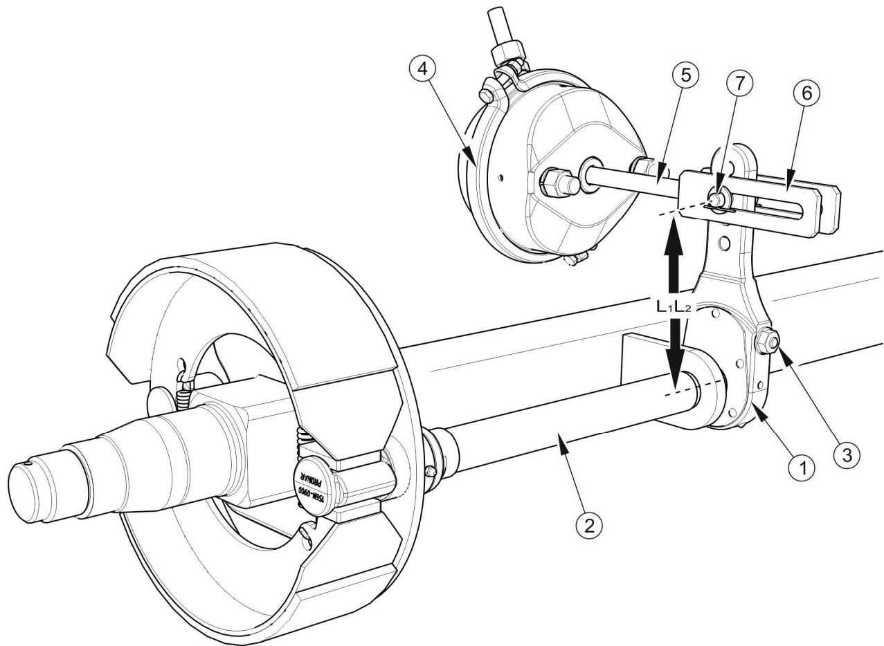
RYSUNEK 5.5 Regulacja hamulców mechanicznych osi jezdnych
