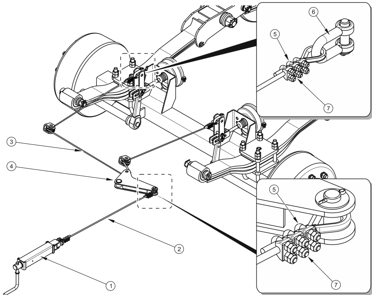
RYSUNEK 5.6 Regulacja napięcia linki hamulca postojowego
