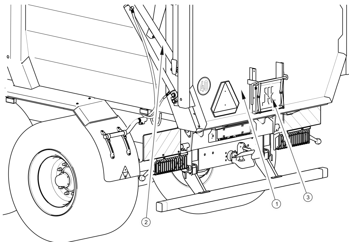
RYСУNEK 3.3 Kłapa tylna
