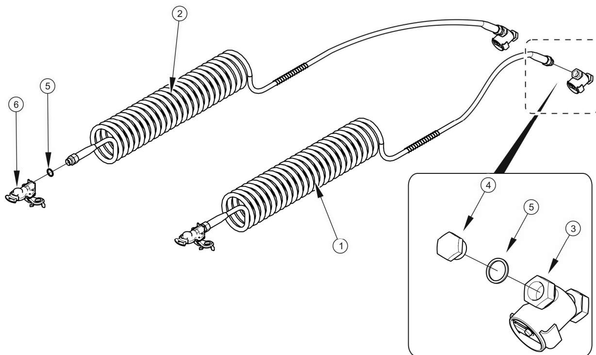
RYSUNEK 5.15 Dostosowanie instalacji dwuprzewodowej na jednoprzewodową
