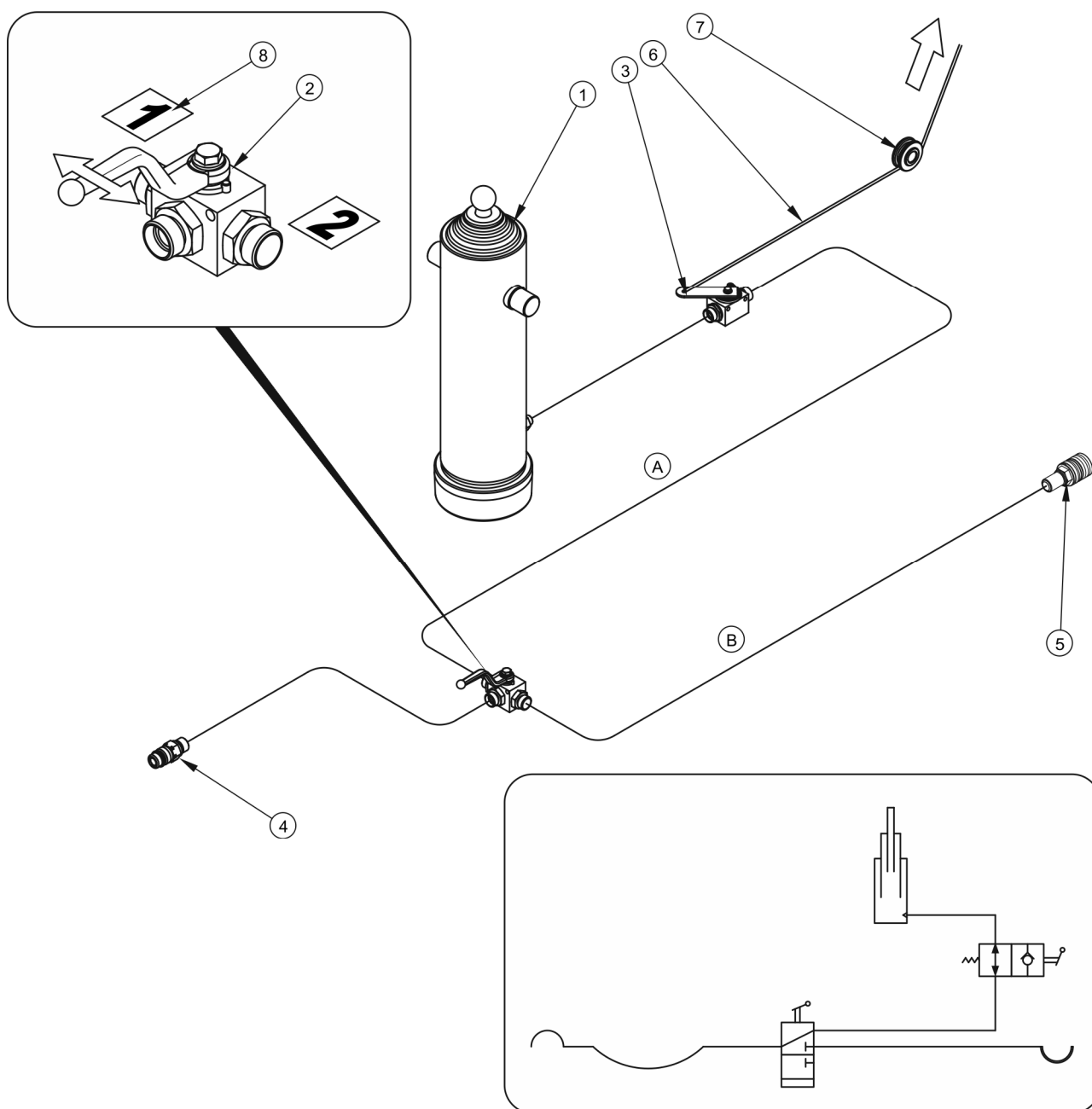
RYСУNEK 3.8 Budowa i schemat instalacji hydraulicznej wywrotu tandem
