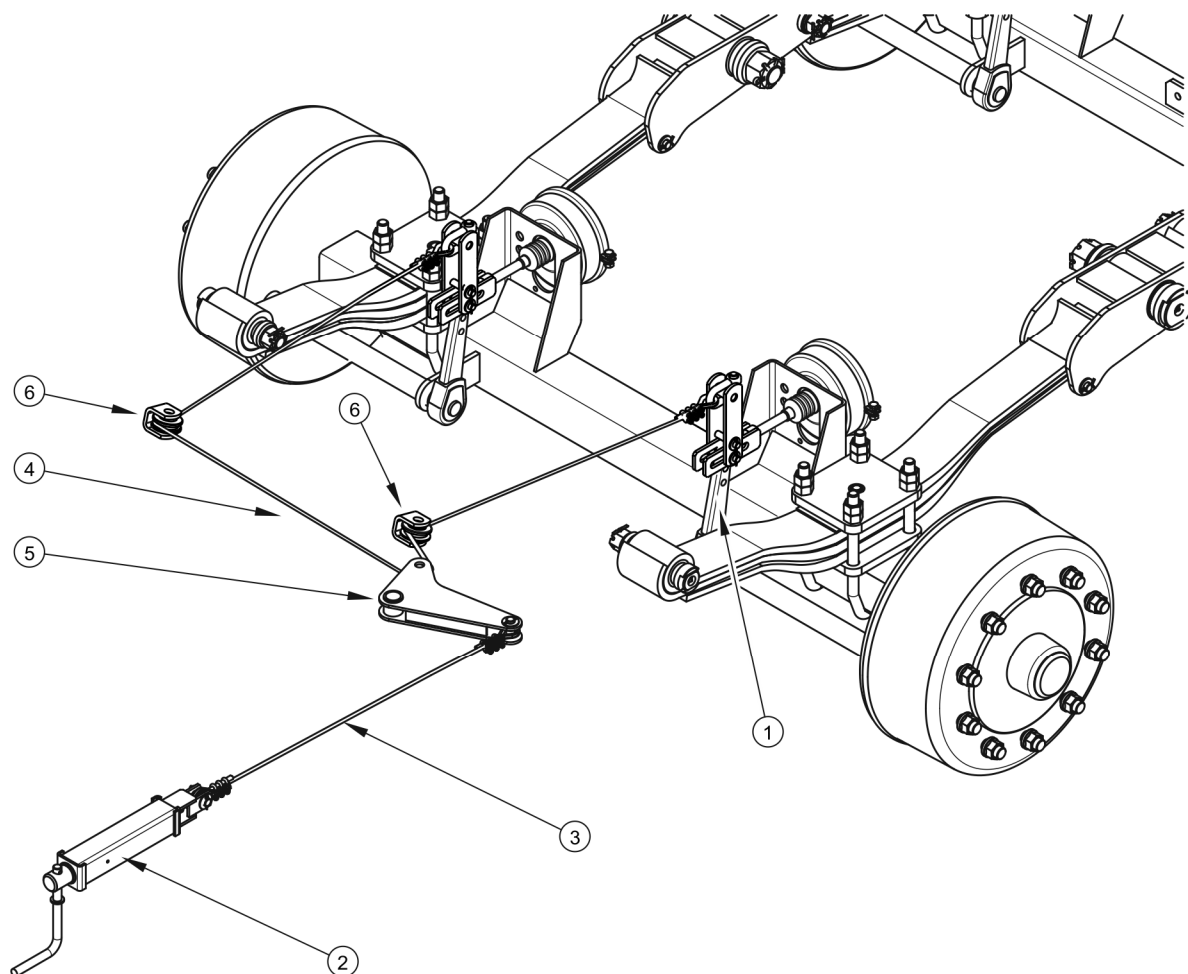
RYSUNEK 3.13 Budowa hamulca postojowego
