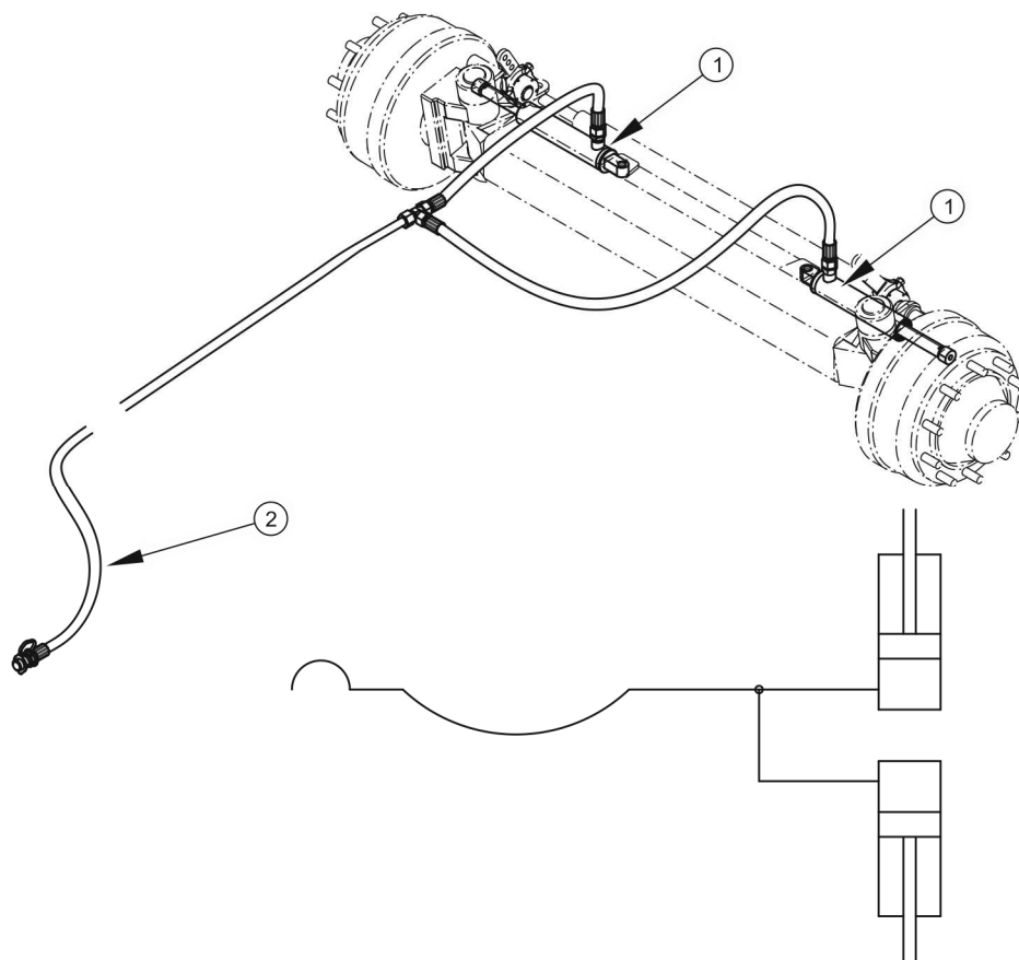
RYSUNEK 3.11 Budowa i schemat instalacji hydraulicznej blokady skrętu
