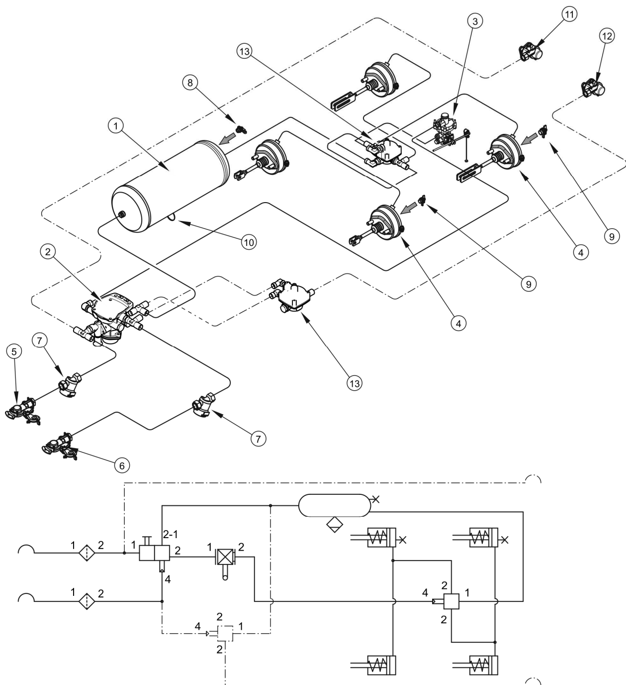
RYSUNEK 3.5 Budowa i schemat instalacji hamulcowej pneumatycznej dwuprzewodowej z regulatorem automatycznym
