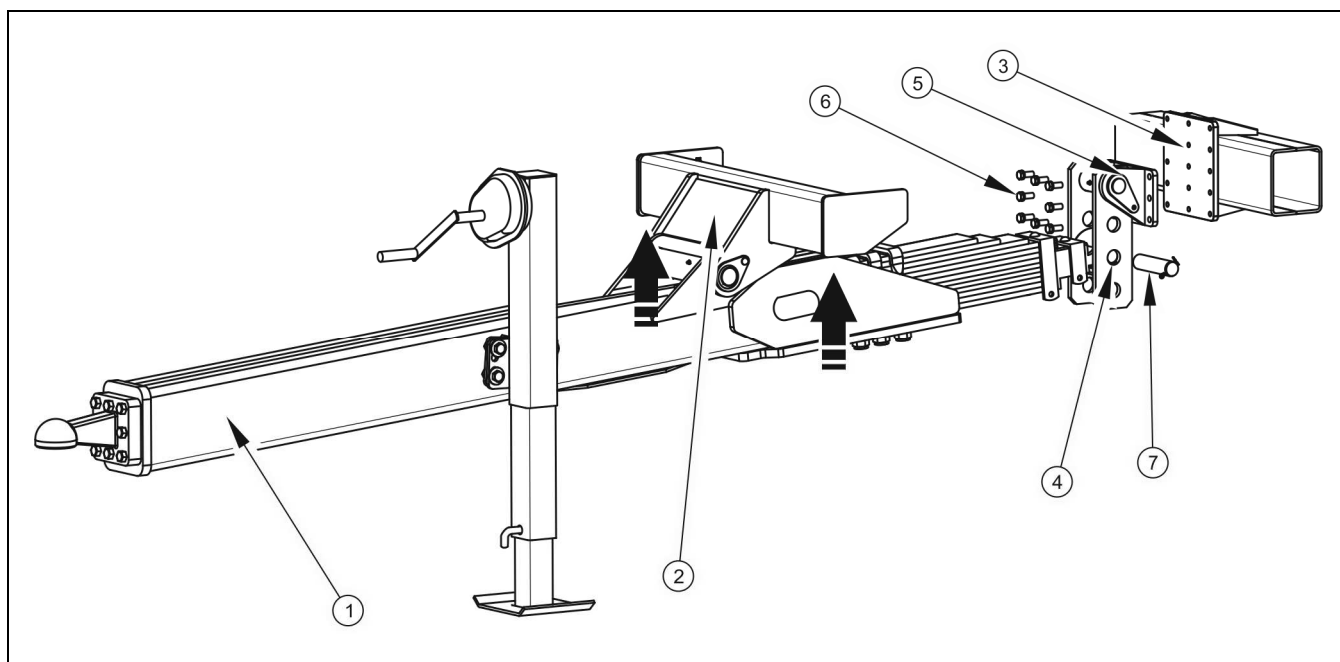
RYСУNEK 5.14 Ustawienie wysokości dyszla
