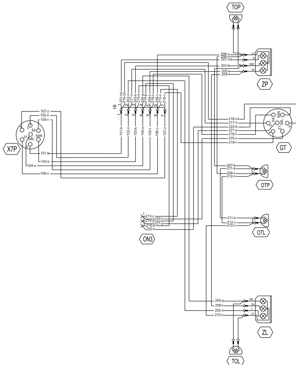
RYSUNEK 3.15 Schemat ideowy instalacji elektrycznej w wersji bez lamp bocznych
