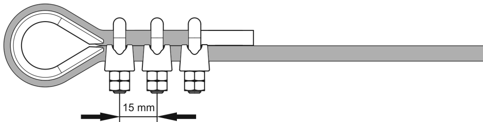
RYСУNEK 5.8 Montaż zacisków linki stalowej
