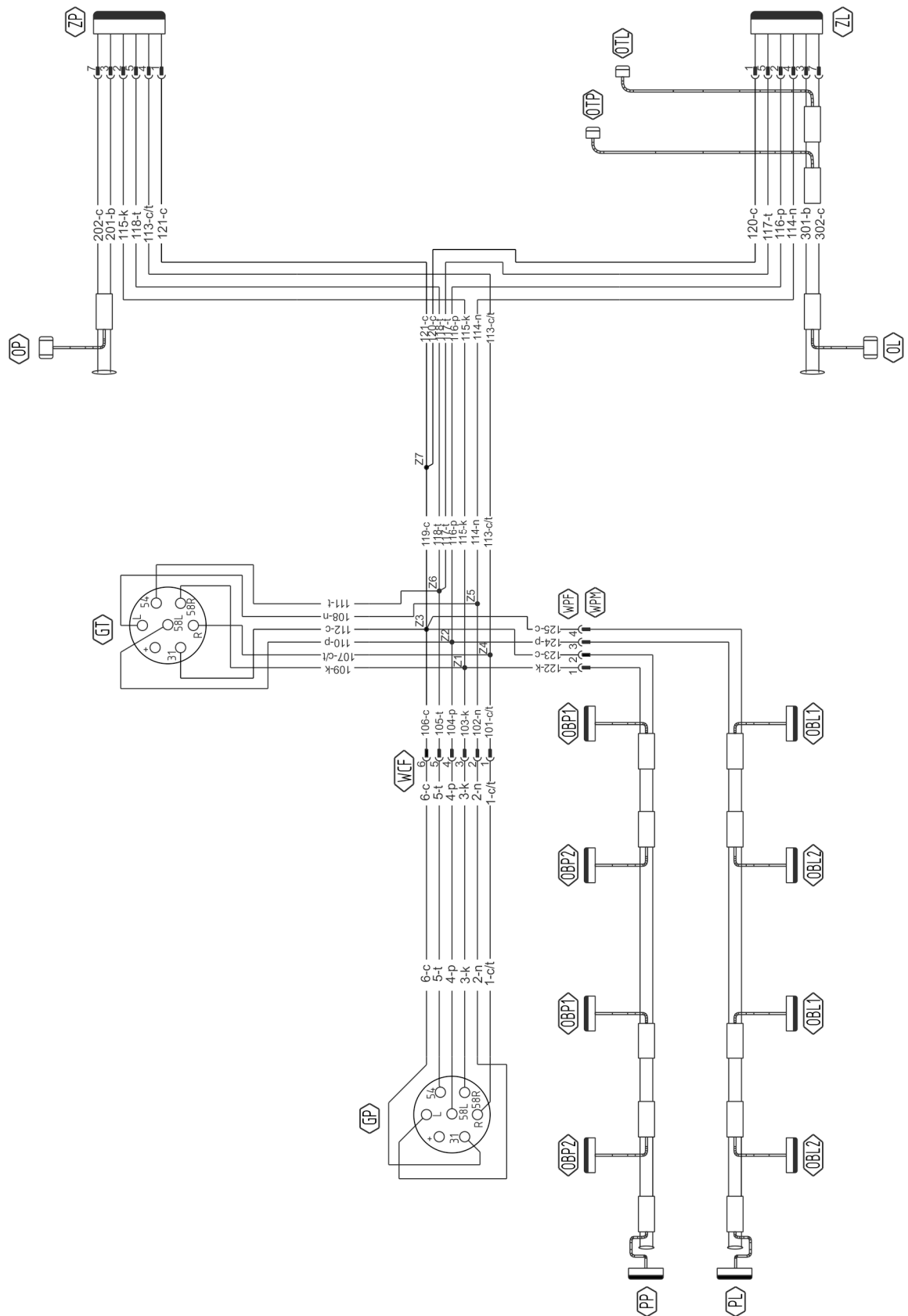
RYSUNEK 3.17 Schemat ideowy instalacji elektrycznej
