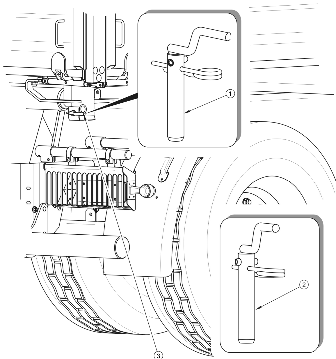
RYSUNEK 4.4 Ryglowanie sworzni wywrotu
