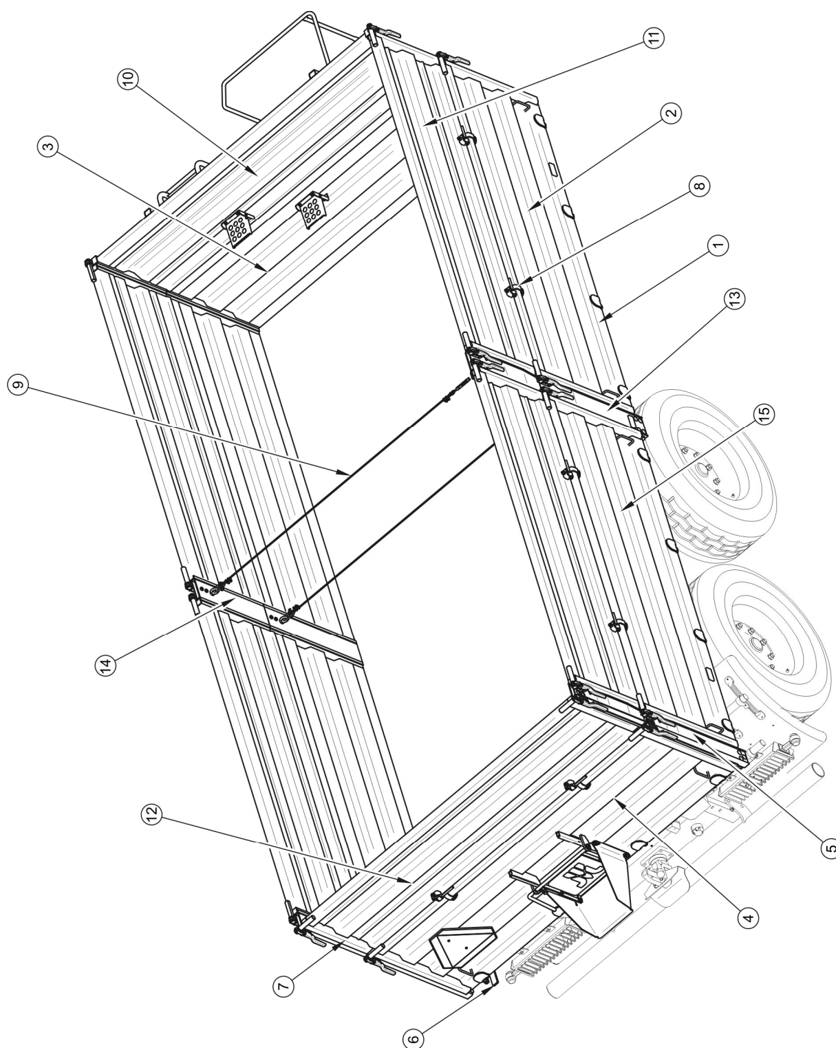
RYSUNEK 3.2 Skrzynia ładunkowa – widok z tyłu
