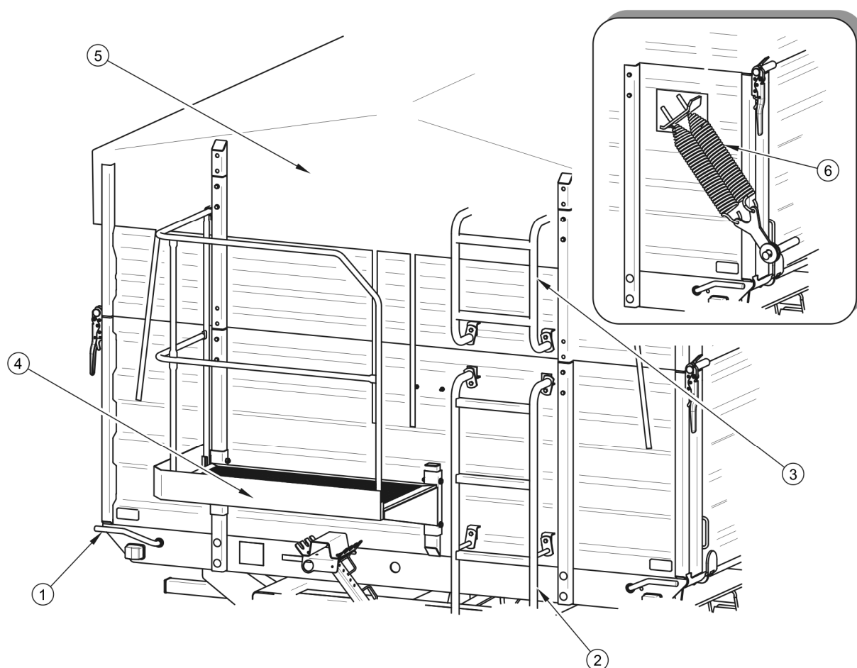
RYСУNEK 3.3 Skrzynia ładunkowa – widok z przodu
