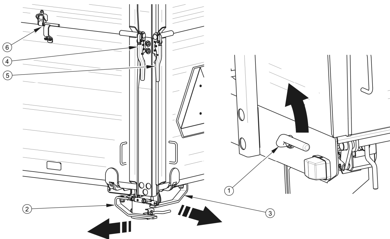
RYSUNEK 4.5 Zamki ścian i nadstaw skrzyniowych
