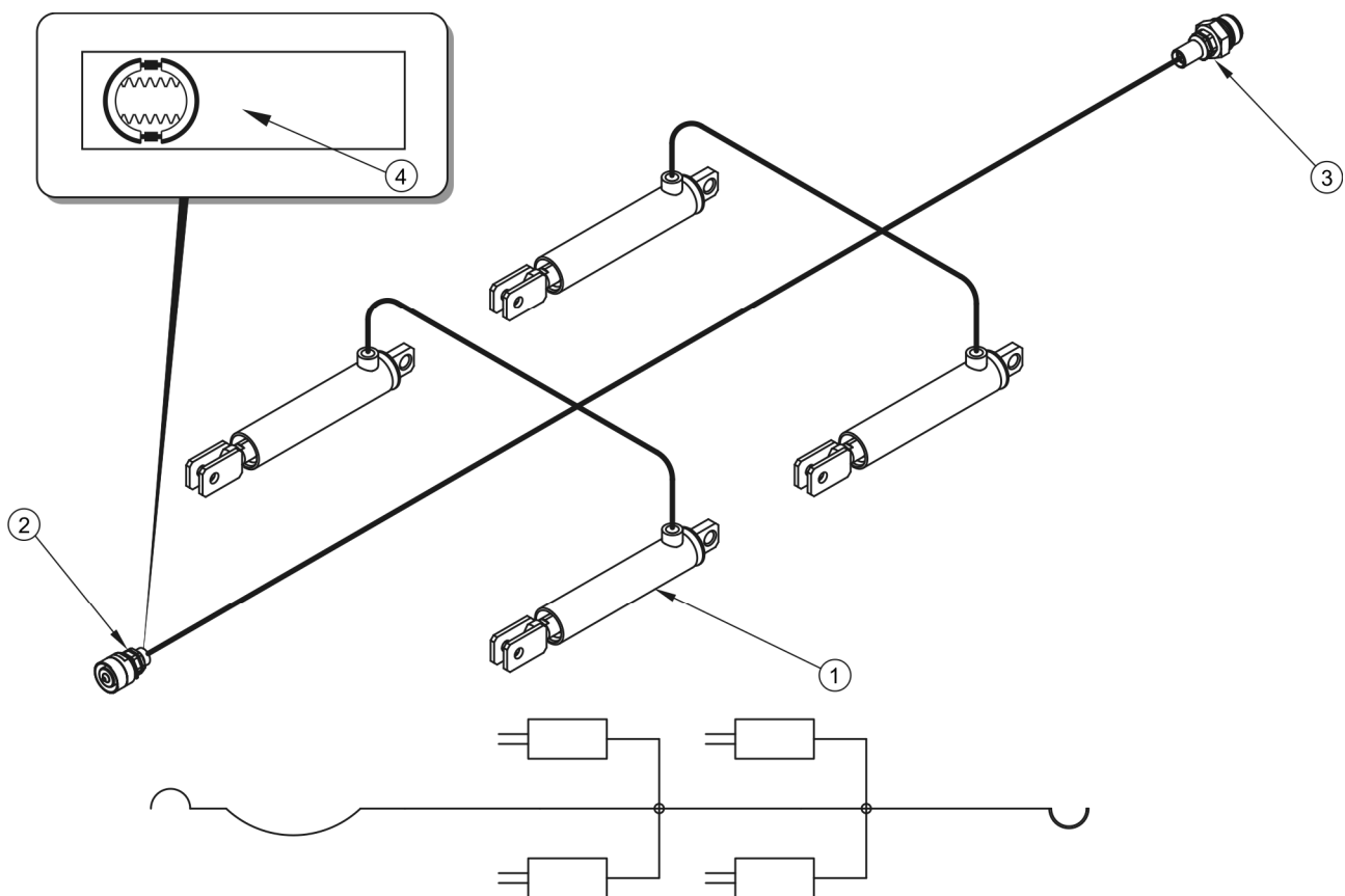
RYСУNEK 3.8 Budowa i schemat instalacji hamulcowej hydraulicznej
