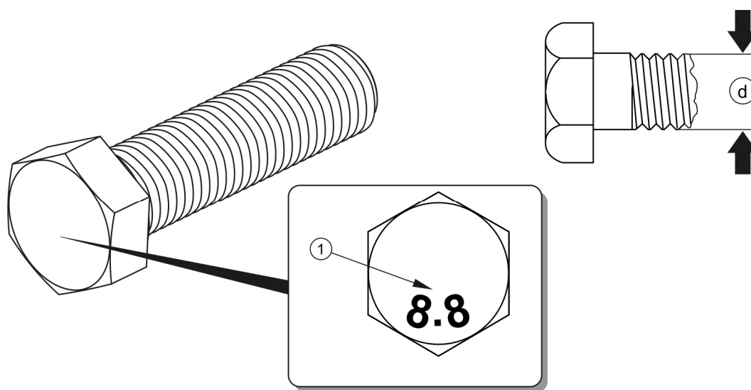
RYSUNEK 5.10 Śruba z gwintem metrycznym
