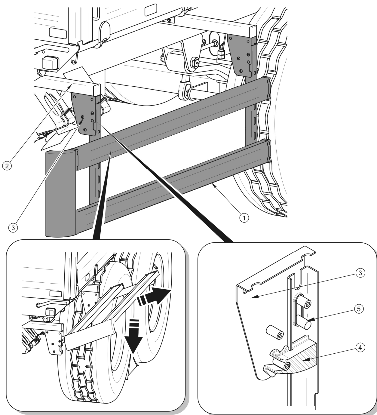
RYSUNEK 4.7 Osłona przeciwnajazdowa lewa
