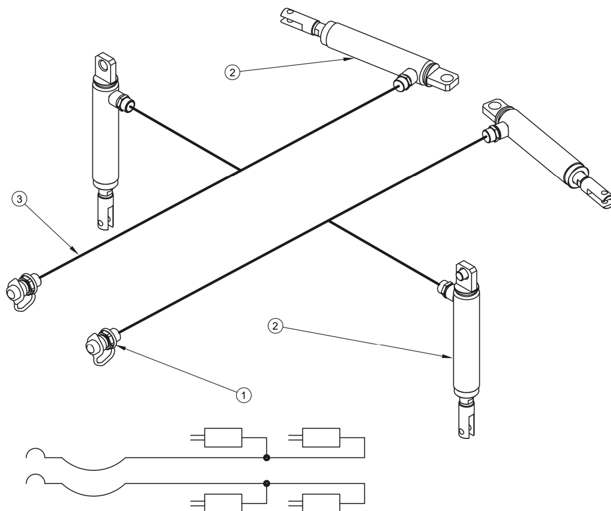
RYСУNEK 3.12 Budowa i schemat instalacji hydraulicznej otwierania burt
