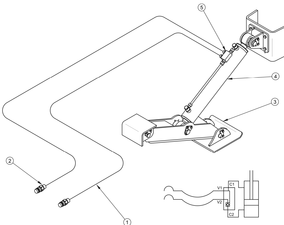
RYSUNEK 3.11 Budowa i schemat instalacji hydraulicznej podpory nożycowej
