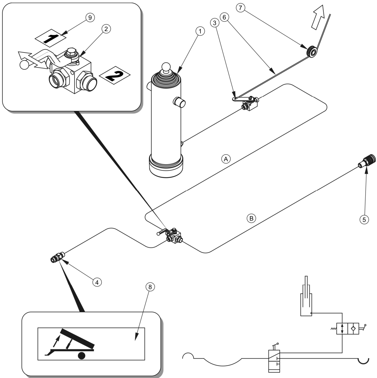
RYСУNEK 3.11 Budowa i schemat instalacji hydraulicznej wywrotu
