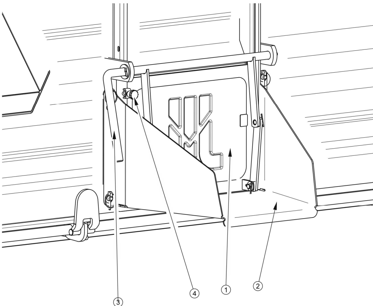
RYSUNEK 4.6 Zamki ścian i nadstaw skrzyniowych
