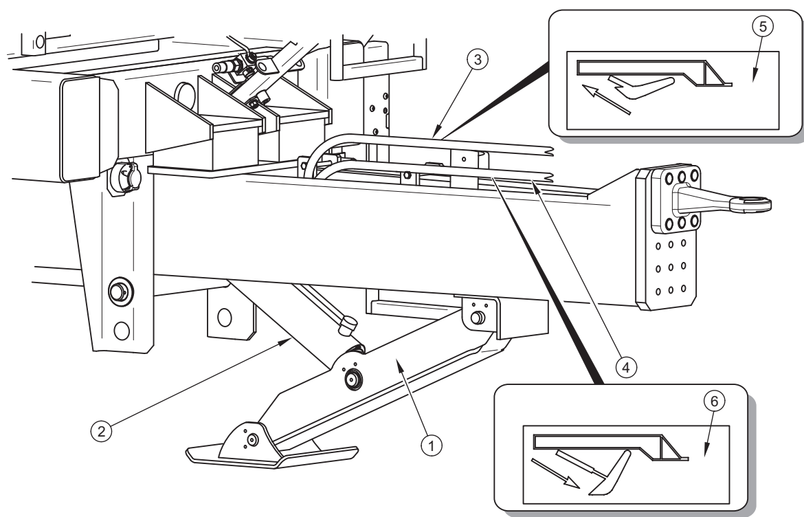
RYSUNEK 4.1 Podpora przyczepy
