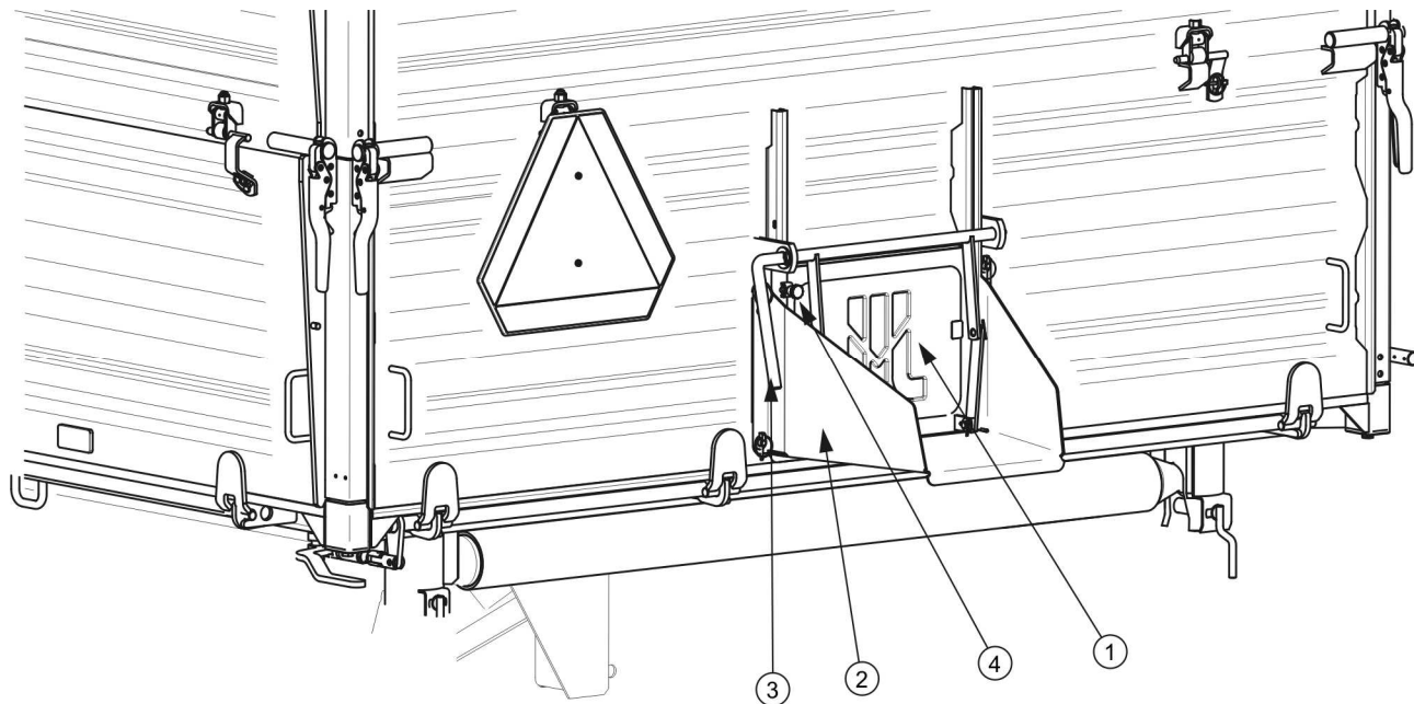
RYСУNEK 3.4 Ściana tylna
