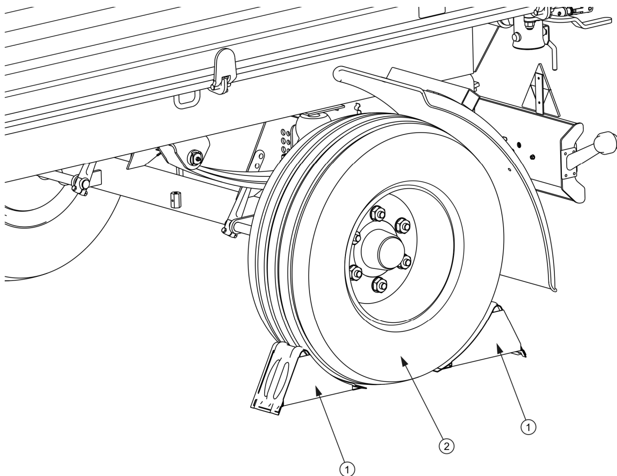
RYСУNEK 2.1 Sposób ustawiania klinów
