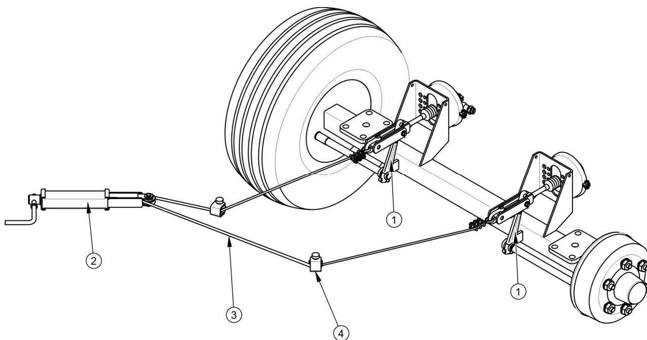
RYSUNEK 3.12 Budowa hamulca postojowego
