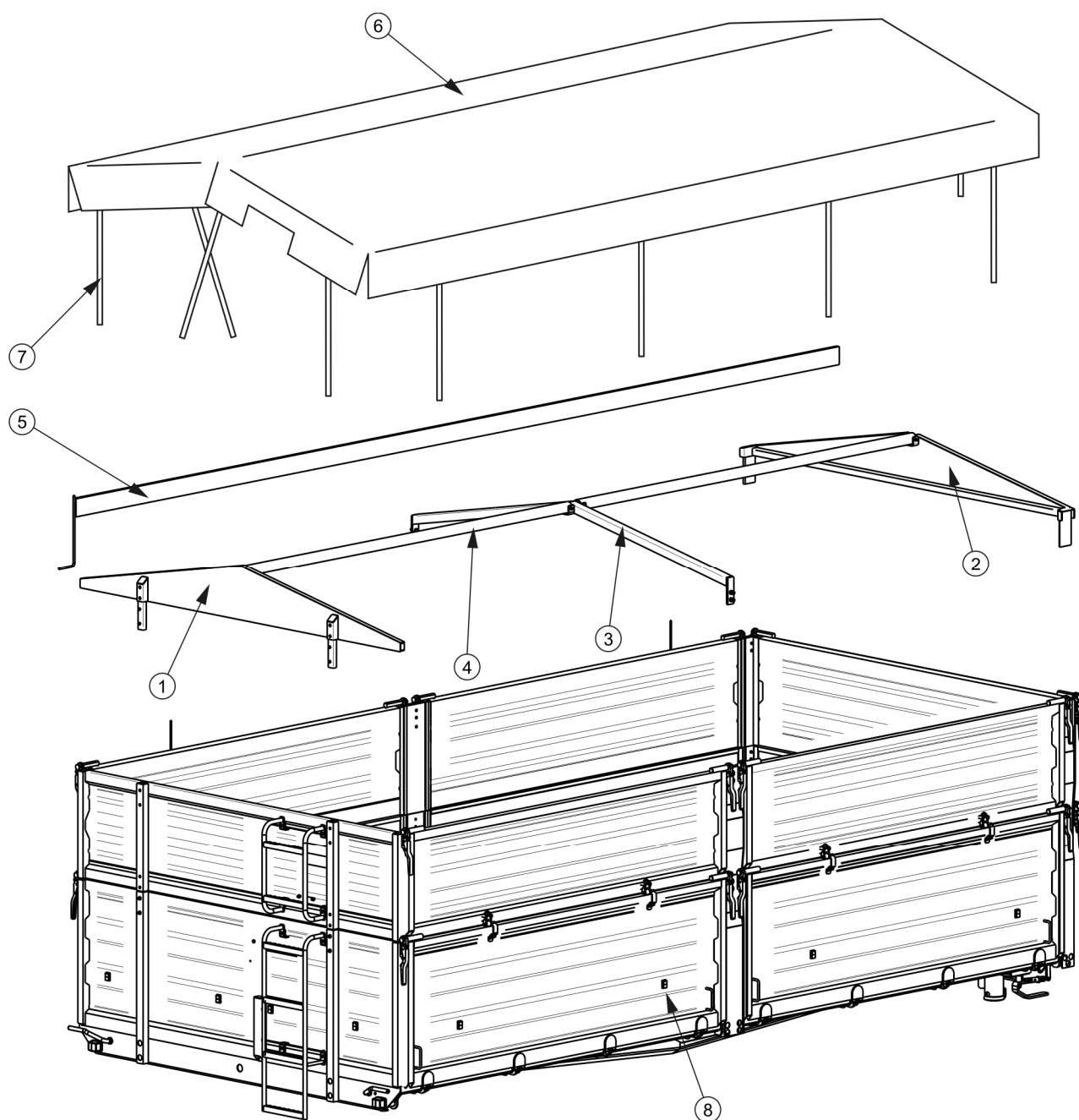
RYSUNEK 5.11 Stelaż z plandeką
