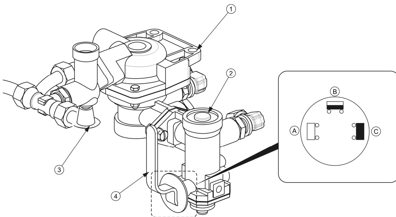
RYSUNEK 3.9 Zawór sterujący i regulator siły hamowania
