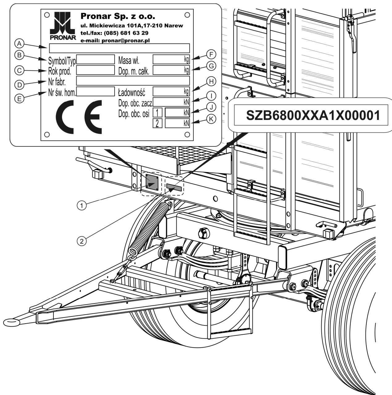
RYSUNEK 1.1 Miejsce umieszczenia tabliczki znamionowej i wybicia numeru fabrycznego
