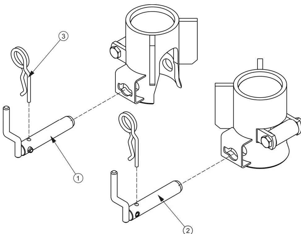
RYSUNEK 4.3 Ryglowanie sworzni wywrotu
