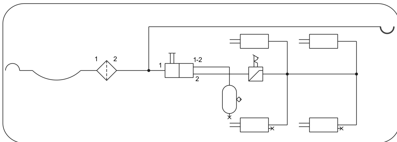
RYSUNEK 3.6 Budowa i schemat instalacji hamulcowej pneumatycznej jednoprzewodowej
