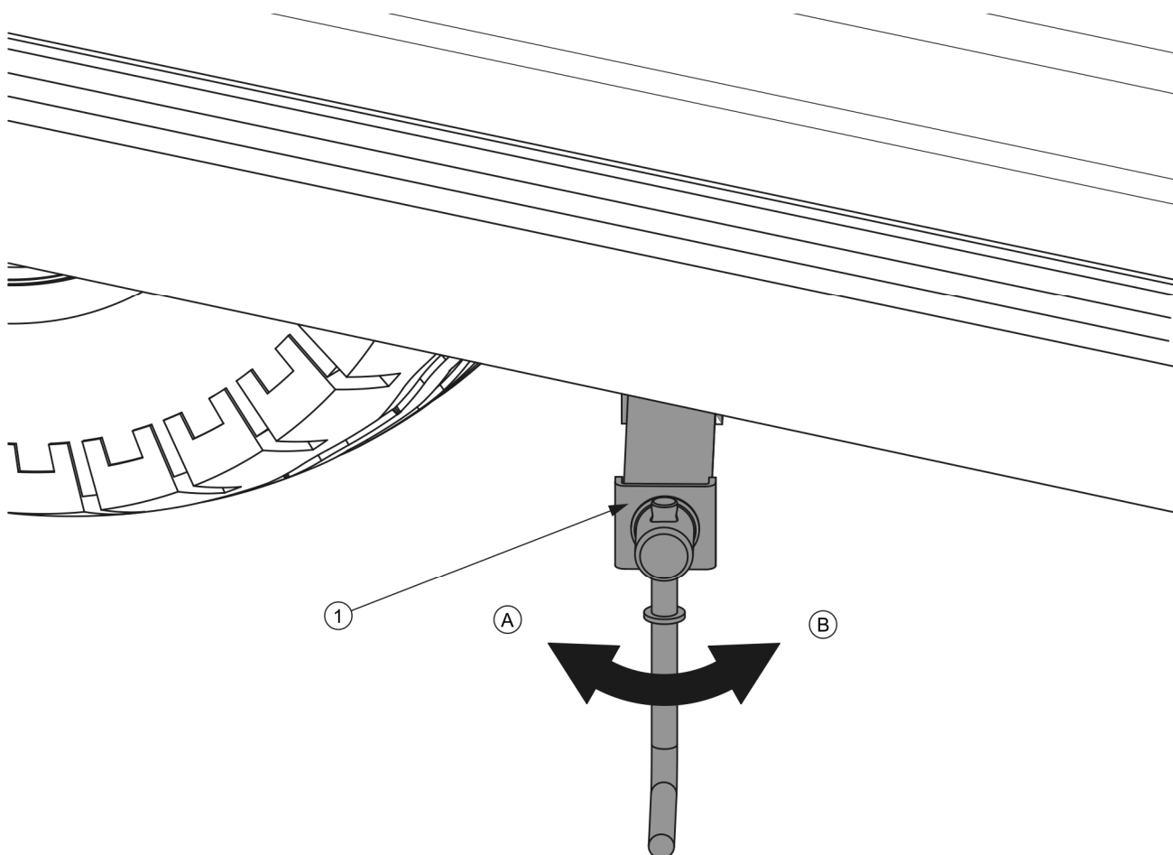
RYSUNEK 4.1 Hamulec postojowy
