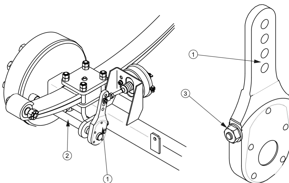
RYSUNEK 5.4 Regulacja hamulców mechanicznych osi jezdnych
