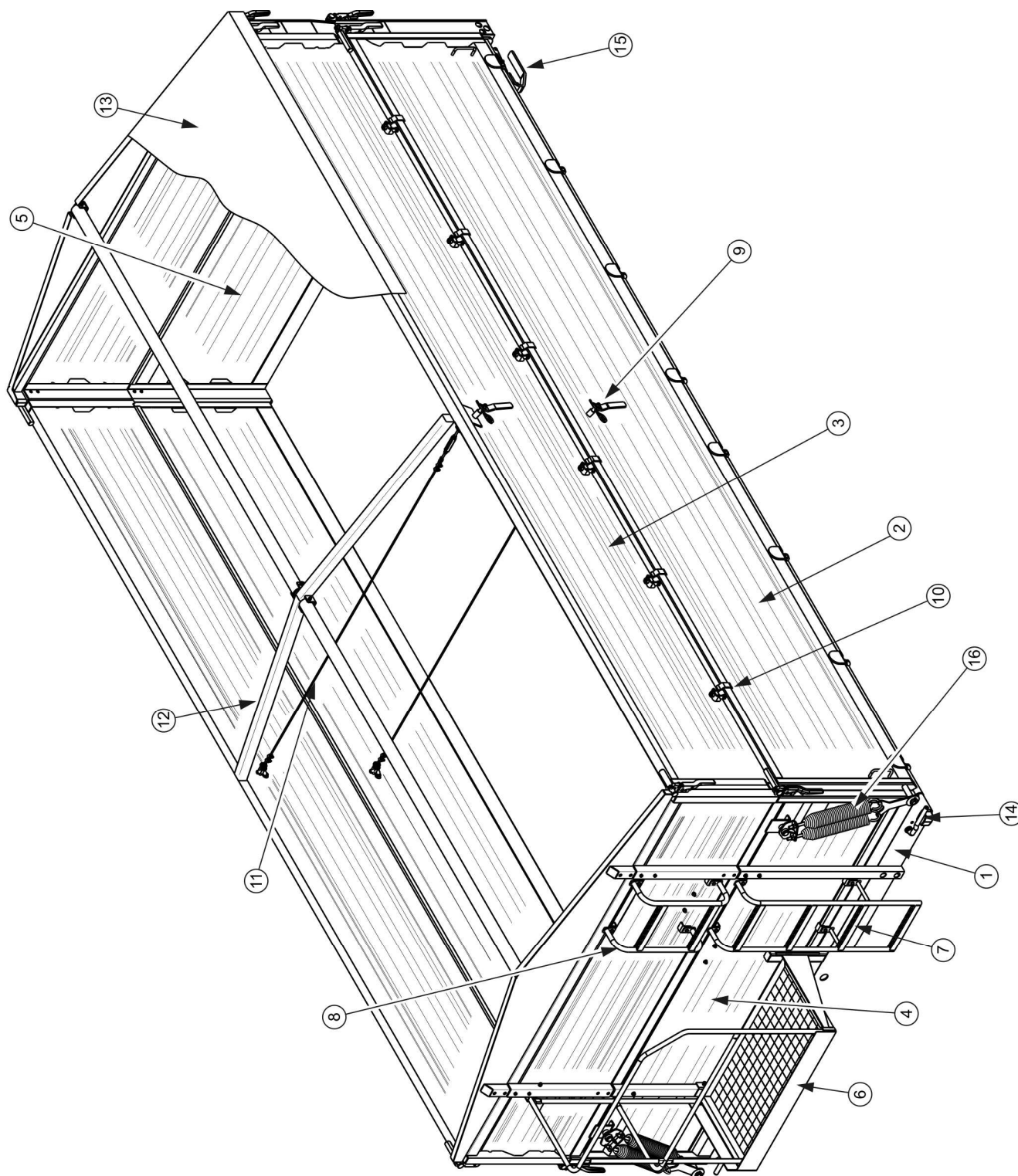
RYSUNEK 3.3 Skrzynia ładunkowa wersja ze ścianami nie dzielonymi
