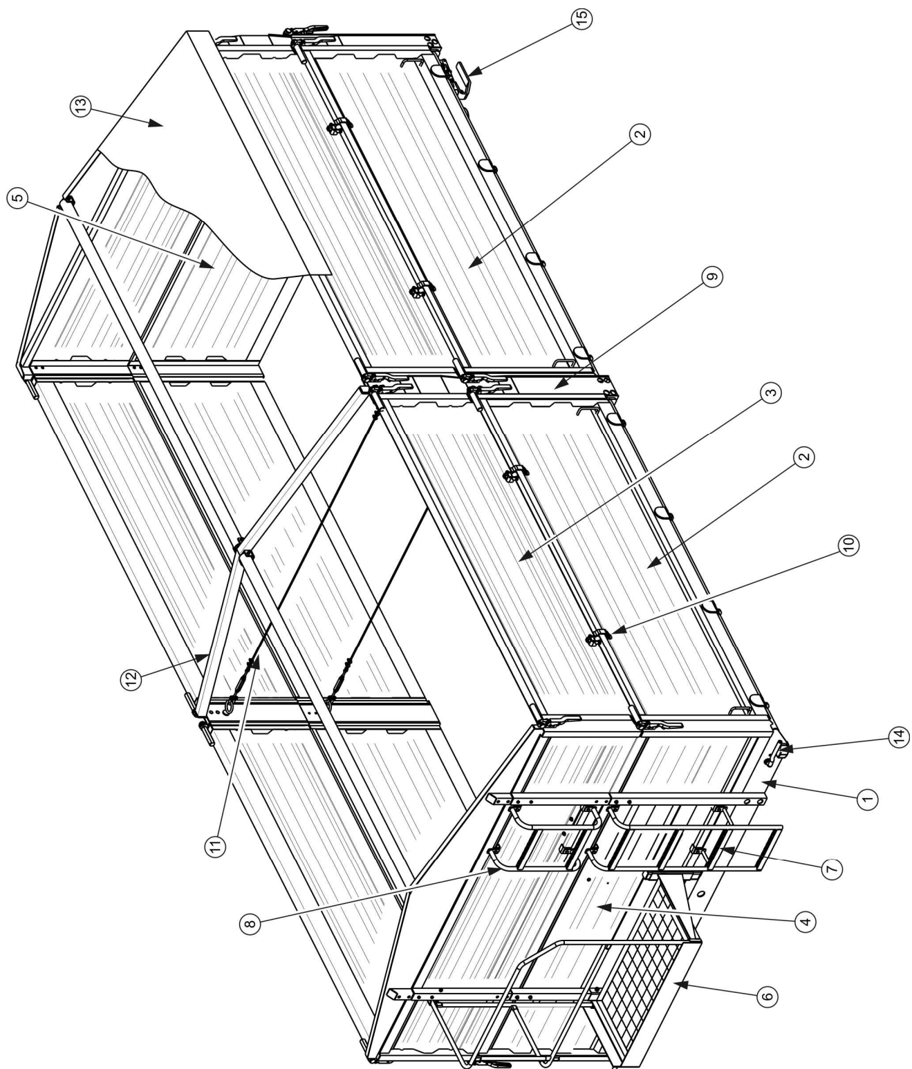
RYSUNEK 3.2 Skrzynia ładunkowa ze ścianami dzielonymi
