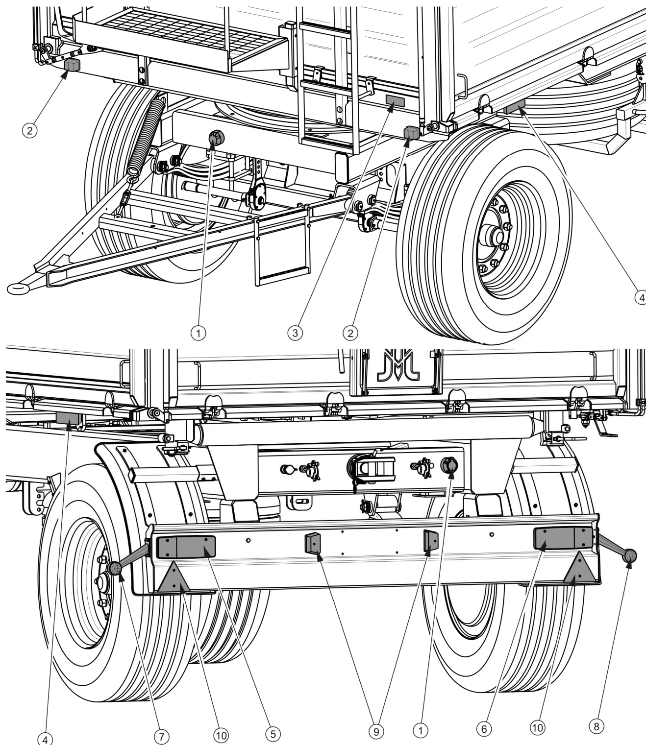
RYSUNEK 3.13 Rozmieszczenie elementów elektrycznych i odblaskowych
