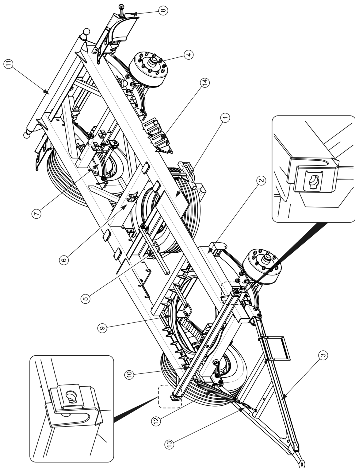
RYSUNEK 3.1 Podwozie przyczepy
