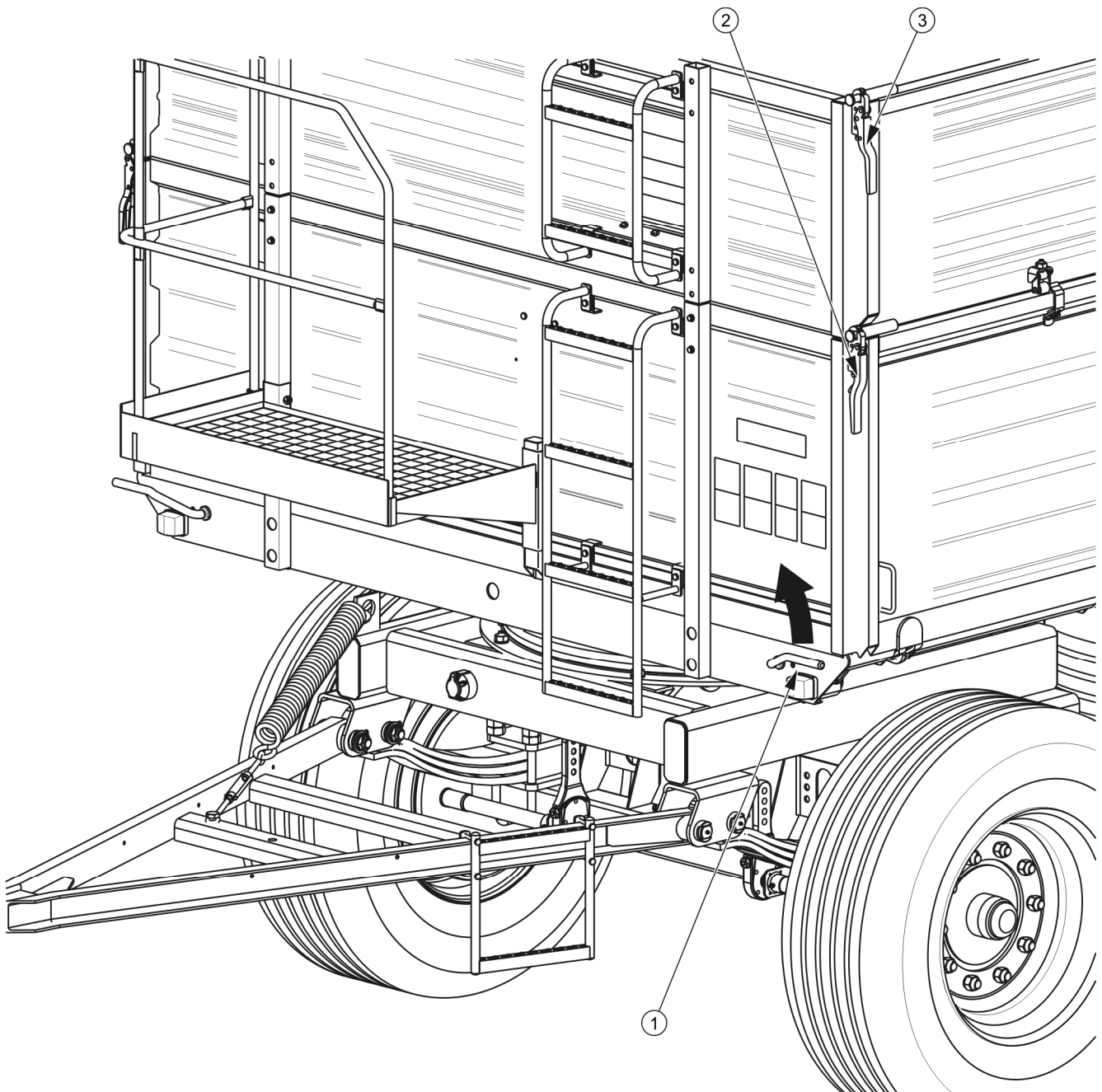
RYSUNEK 4.4 Zamki ścian i nadstaw skrzyniowych z przodu
