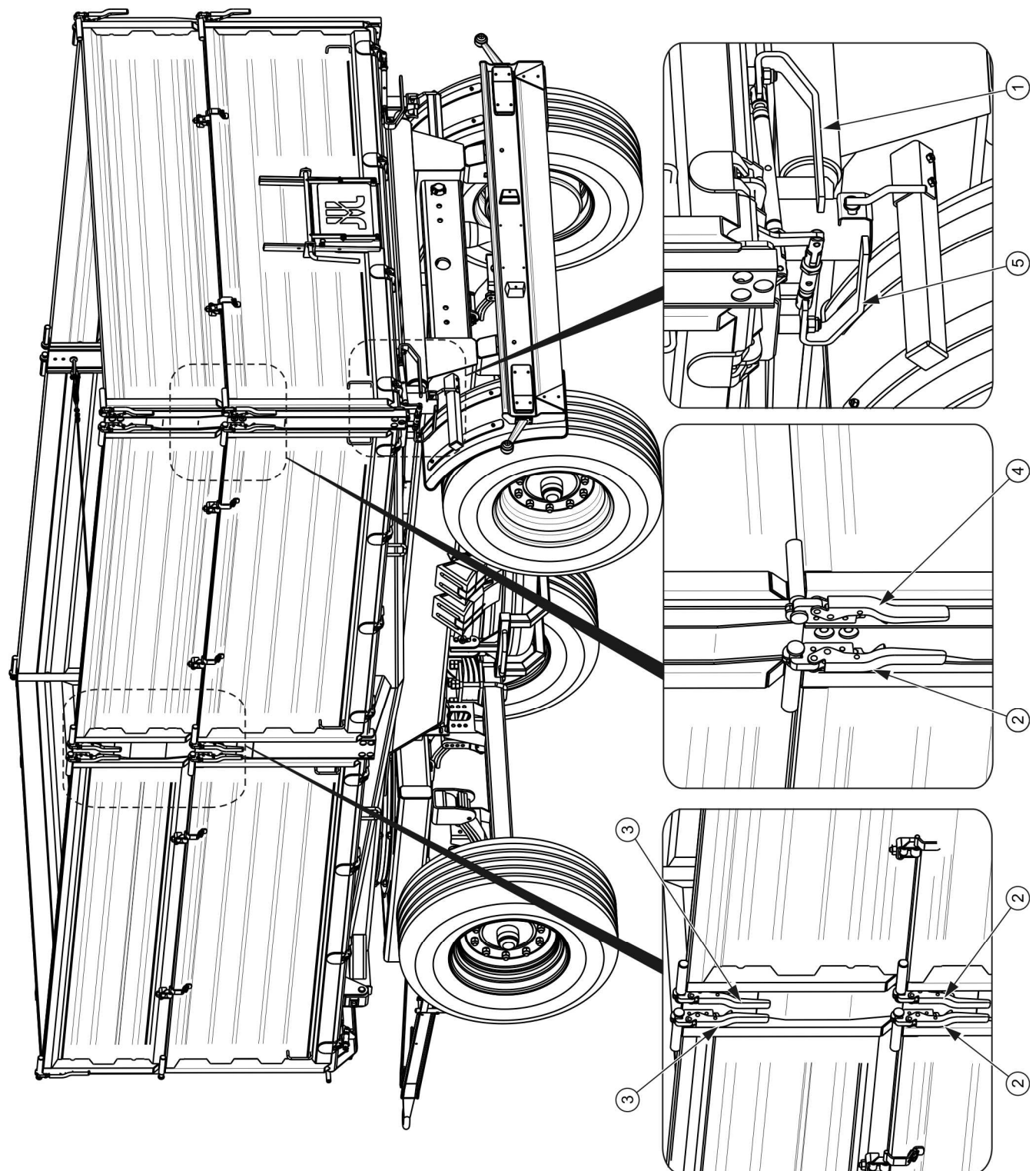
RYSUNEK 4.5 Zamki ścian i nadstaw skrzyniowych
