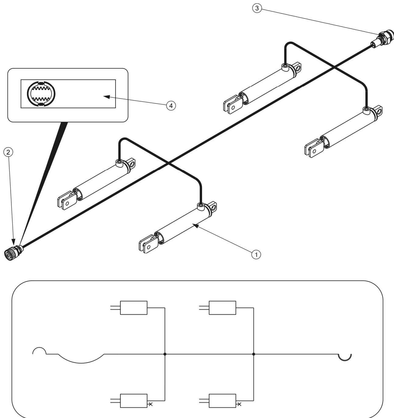
RYSUNEK 3.8 Budowa i schemat instalacji hamulcowej hydraulicznej
