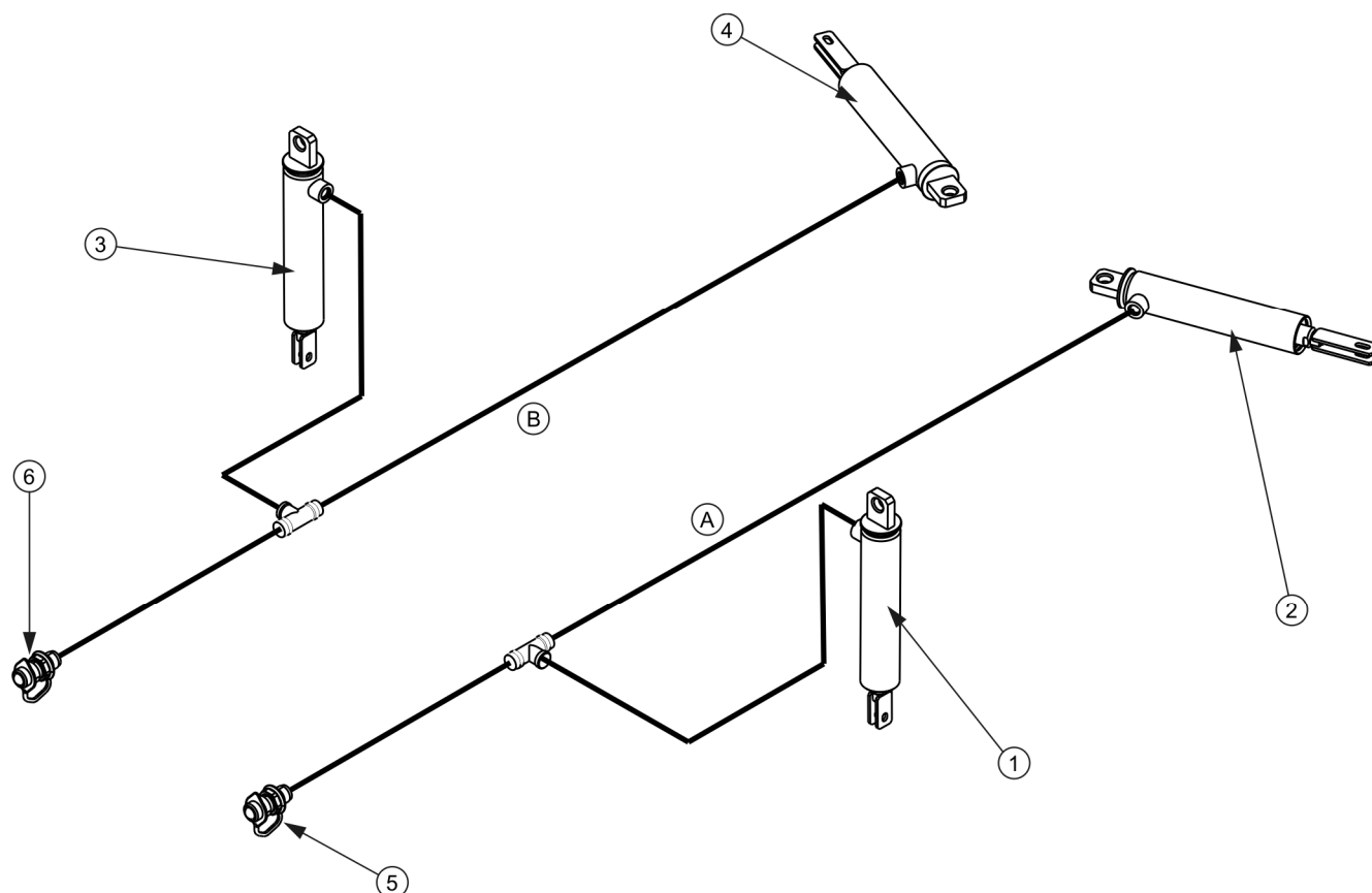
RYСУNEK 3.11 Instalacja hydraulicznego otwierania bort
