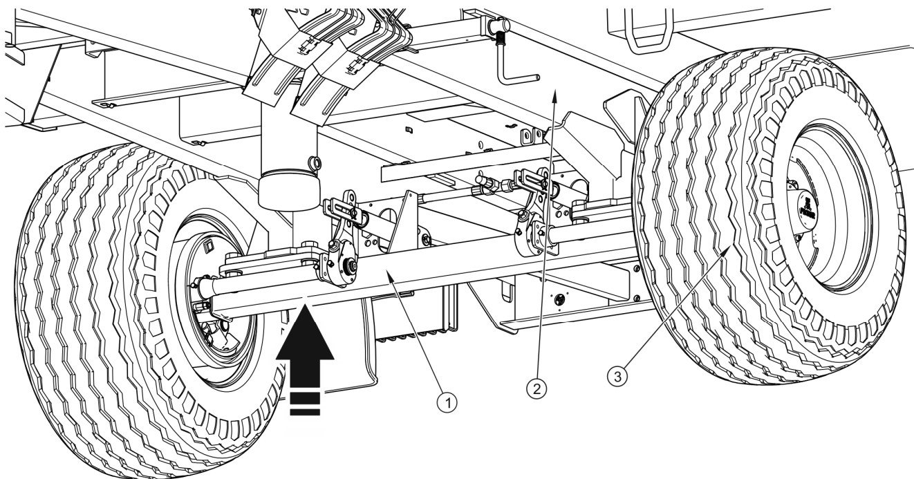
РИСУНОК 5.1 Точка поддомкрачивания
