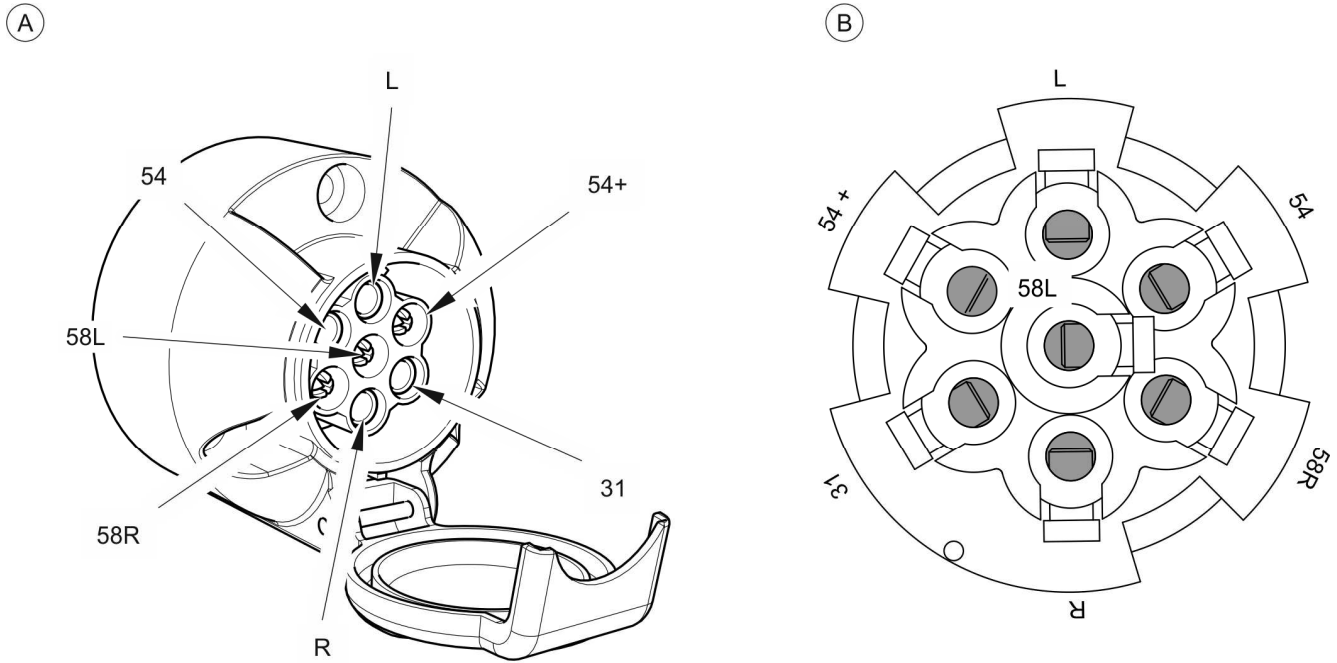
РИСУНОК 3.9 Разъем
