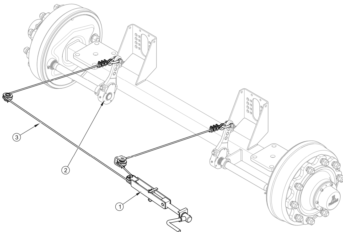
РИСУНОК 3.8 Устройство стояночного тормоза
