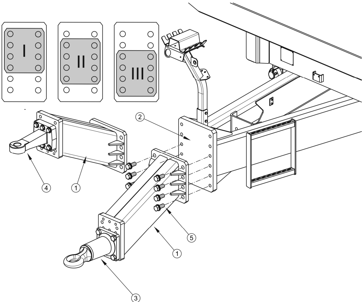
РИСУНОК 5.16 Регулирование положения дышла
