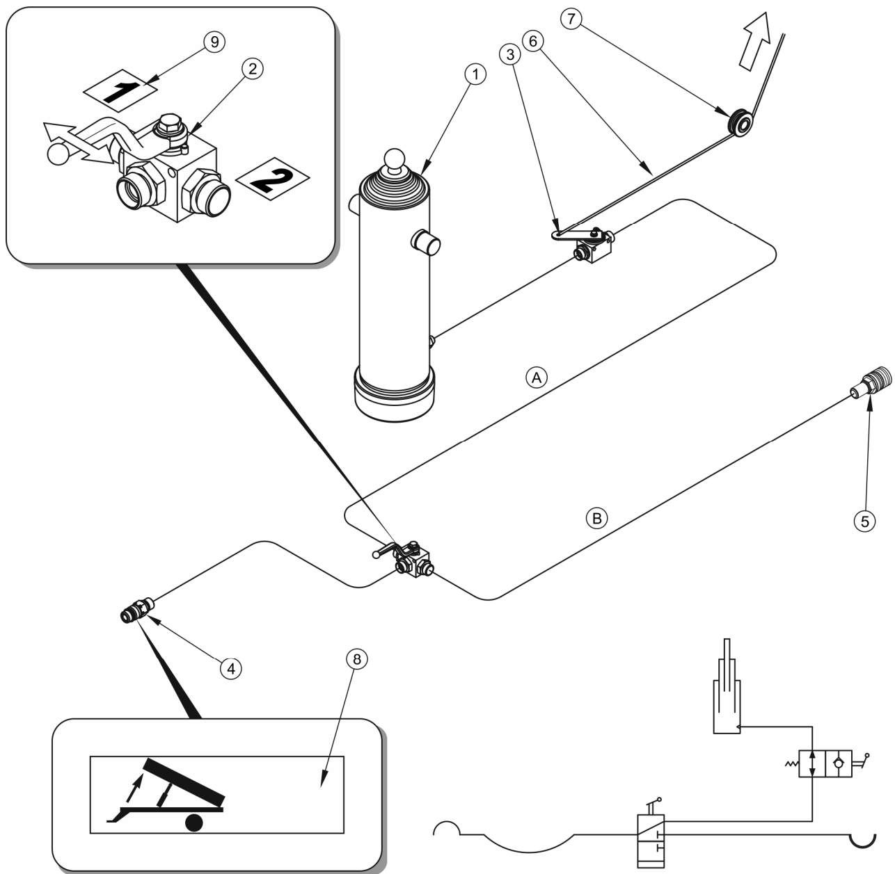
РИСУНОК 3.6 Устройство и схема гидравлической системы опрокидывания
