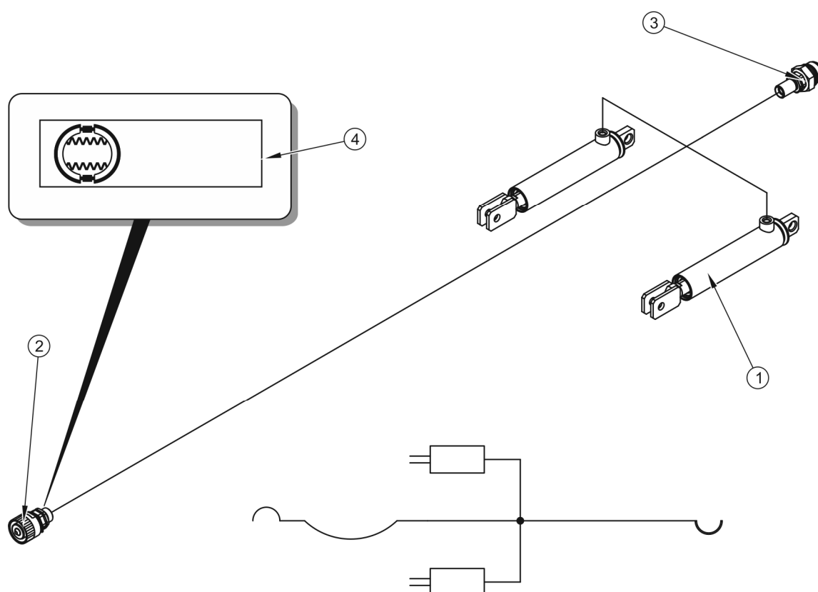
РИСУНОК 3.4 Устройство и схема гидравлической тормозной системы
