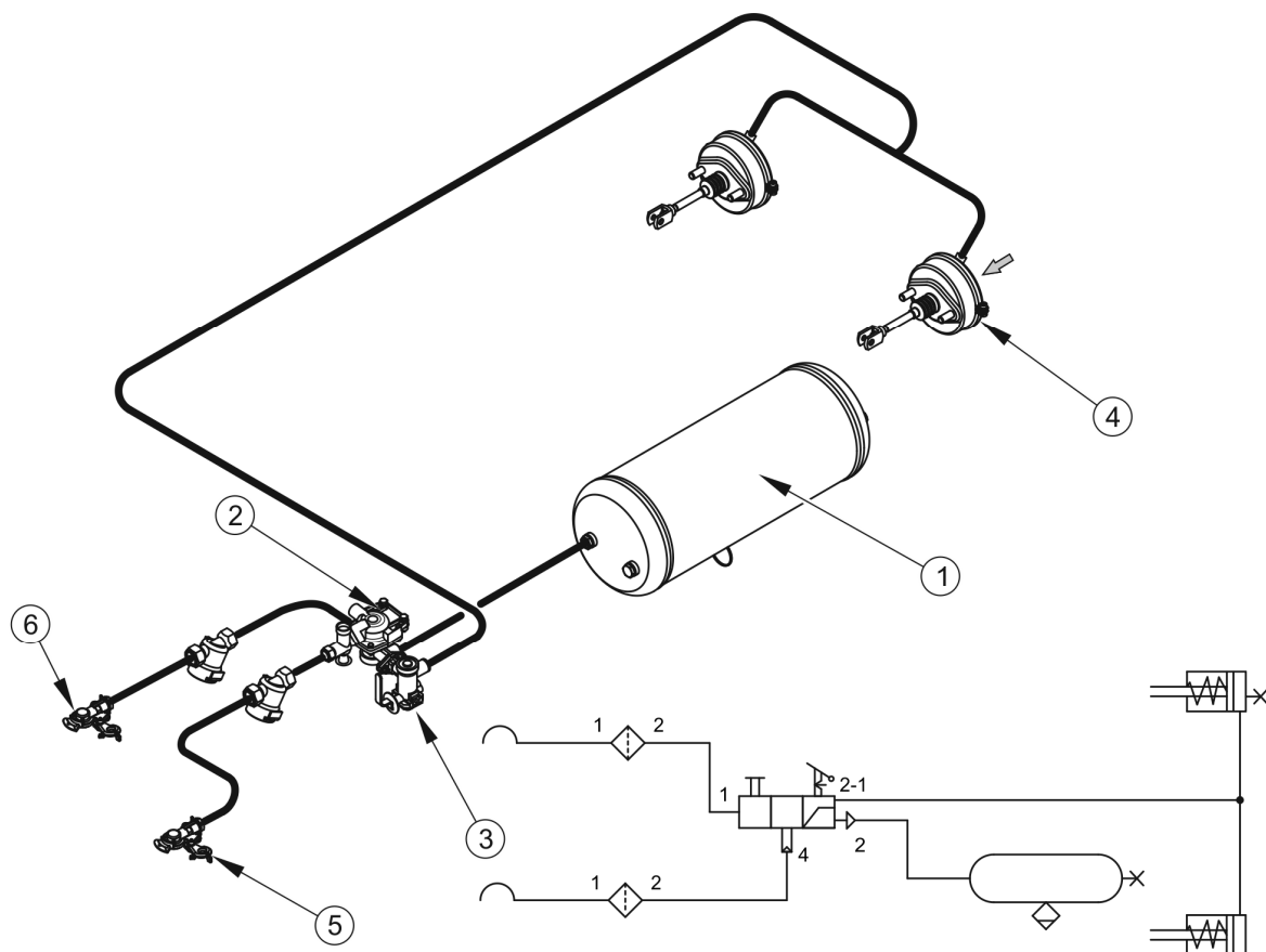
РИСУНОК 3.3 Устройство и схема пневматической тормозной системы
