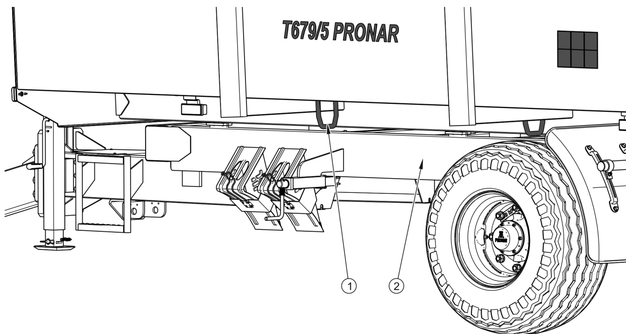
РИСУНОК 1.3 Транспортные захваты
