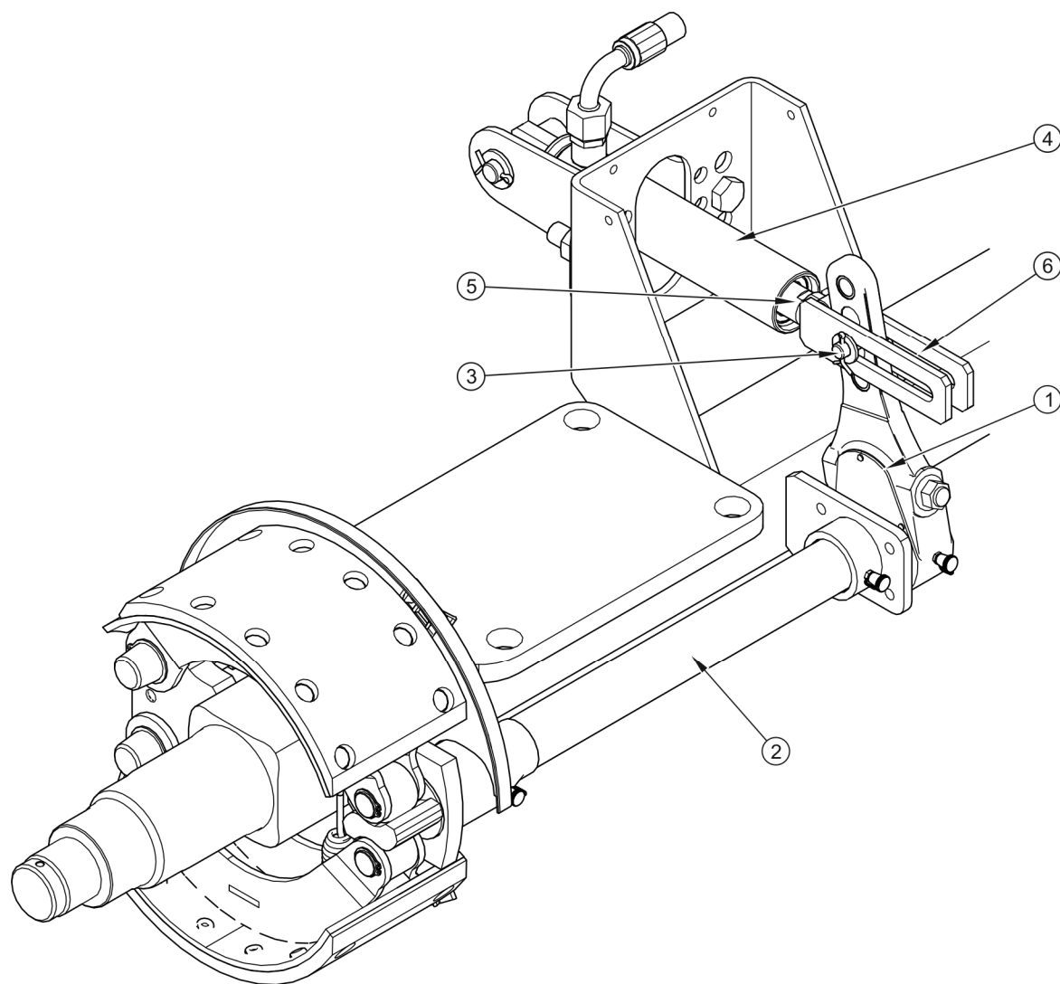
РИСУНОК 5.7 Устройство гидравлического тормоза ходовой оси
