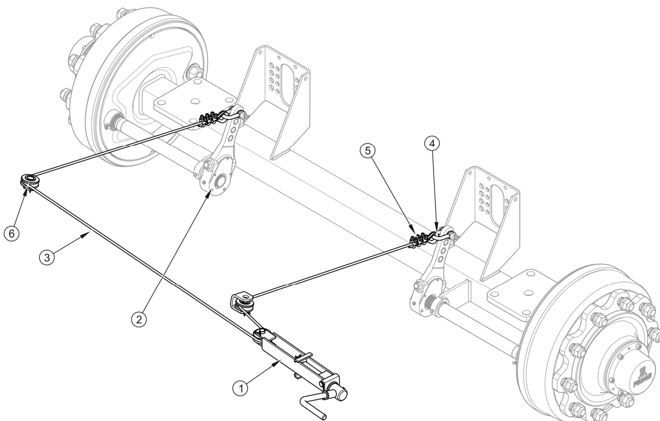
РИСУНОК 5.10 Стояночный тормоз
