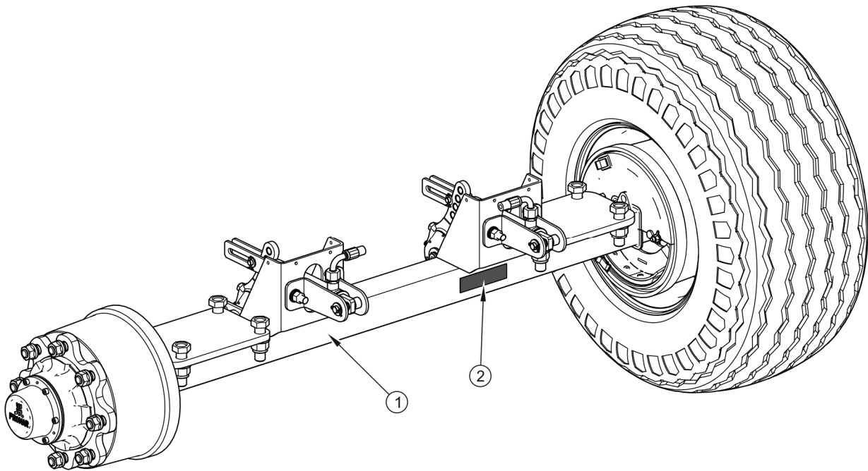
РИСУНОК 1.2 Размещение заводского щитка ходовой оси
