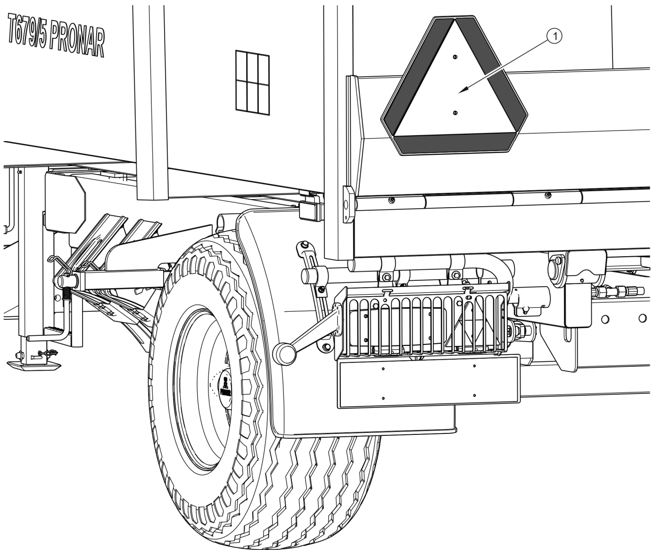
РИСУНОК 2.1 Место крепления знака
