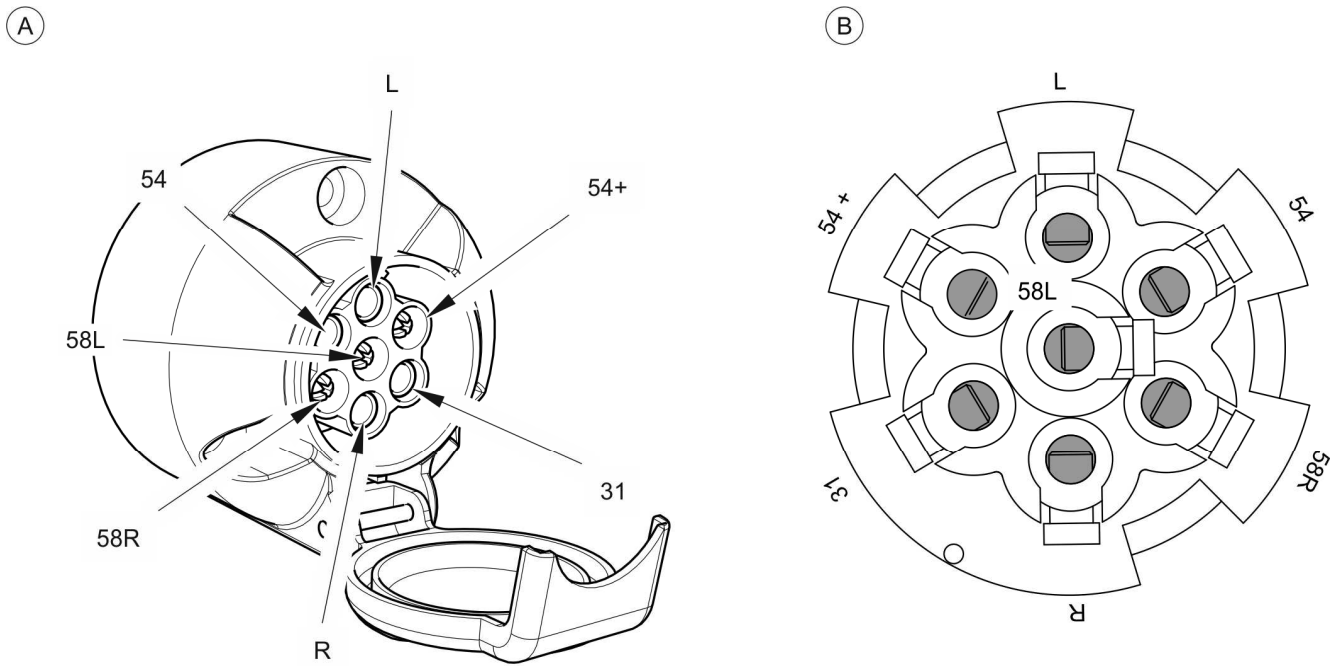
РИСУНОК 3.9 Разъем
