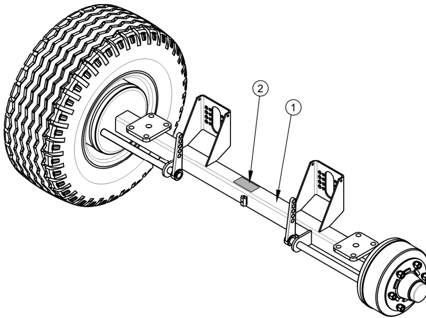
RYSUNEK 1.2 Miejsce umieszczenia tabliczki znamionowej osi jezdnej
