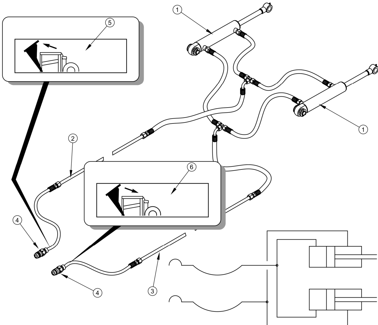
RYSunEK 3.11 Budowa i schemat instalacji hydraulicznej kłapy tylnej
