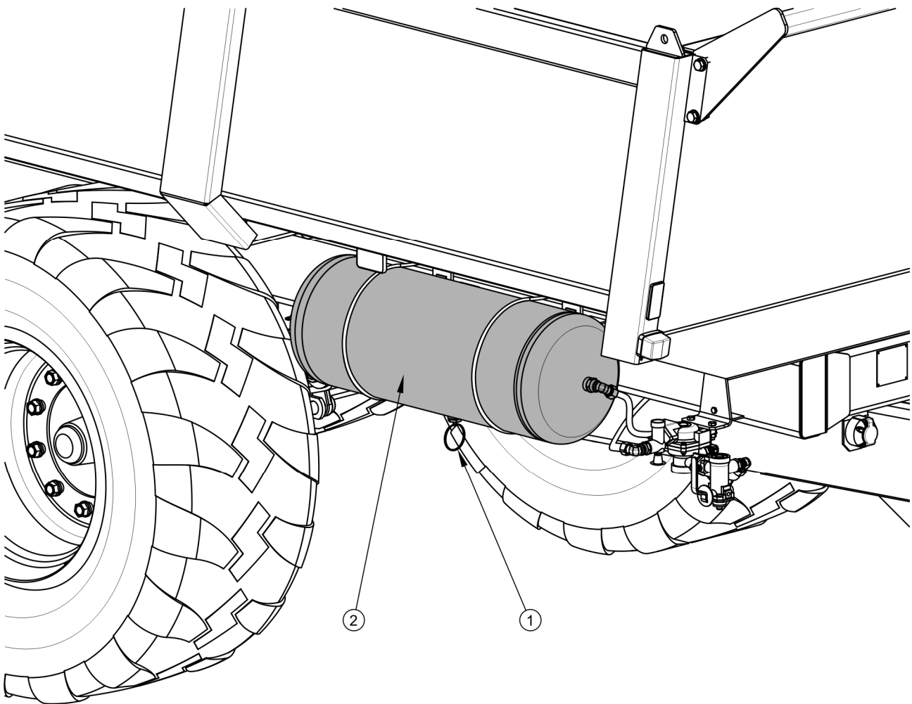
RYSUNEK 5.9 Odwadnianie zbiornika powietrza
