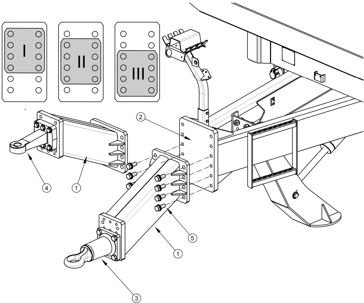
RYSUNEK 5.13 Regulacja położenia dyszla
