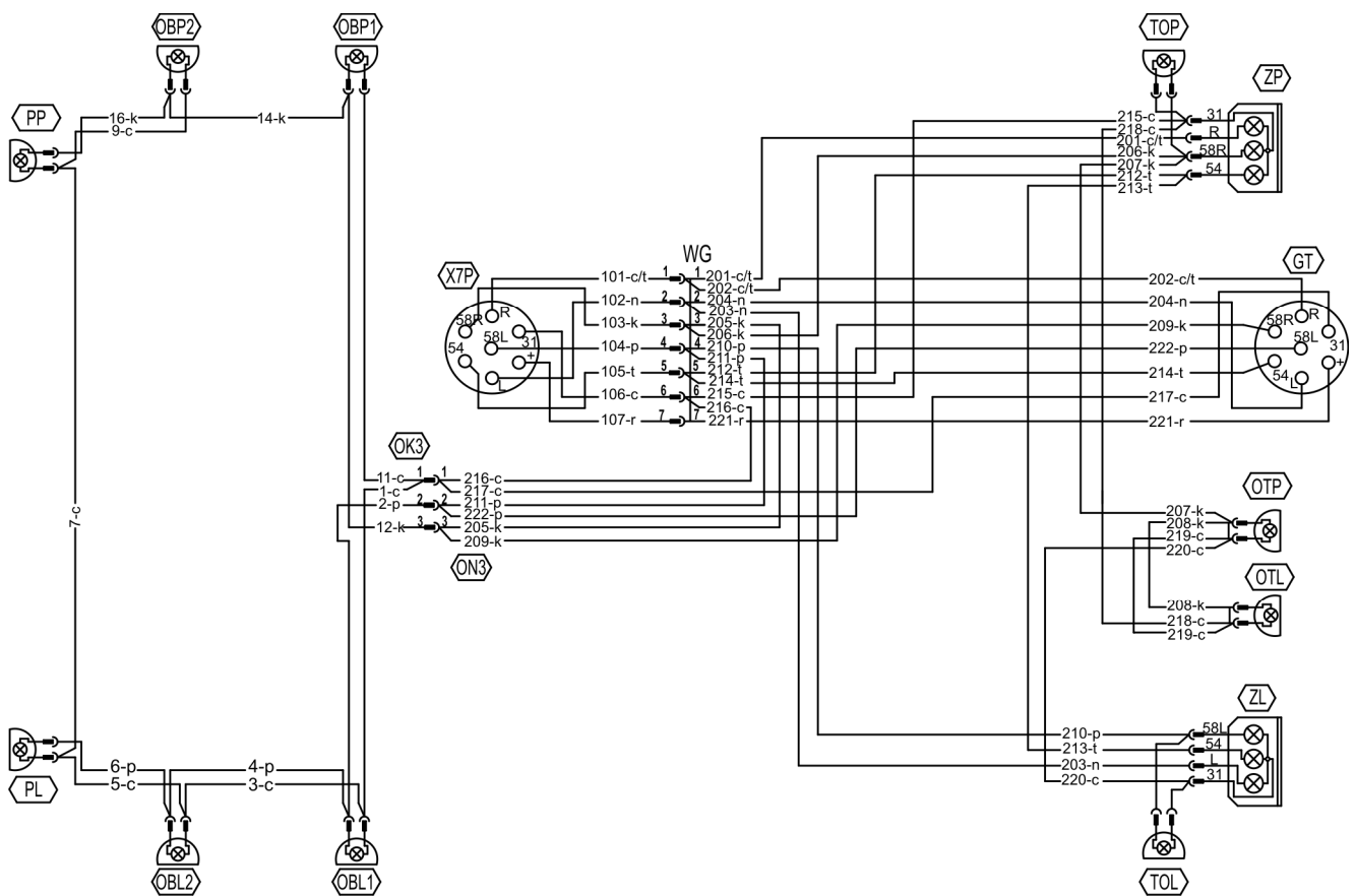
RYSUNEK 3.15 Schemat ideowy instalacji elektrycznej
