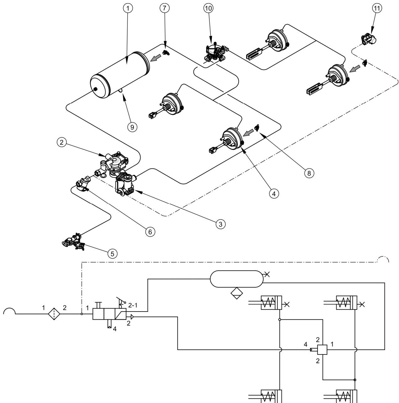
RYSUNEK 3.3 Budowa i schemat instalacji hamulcowej pneumatycznej jedнопrzewodowej
