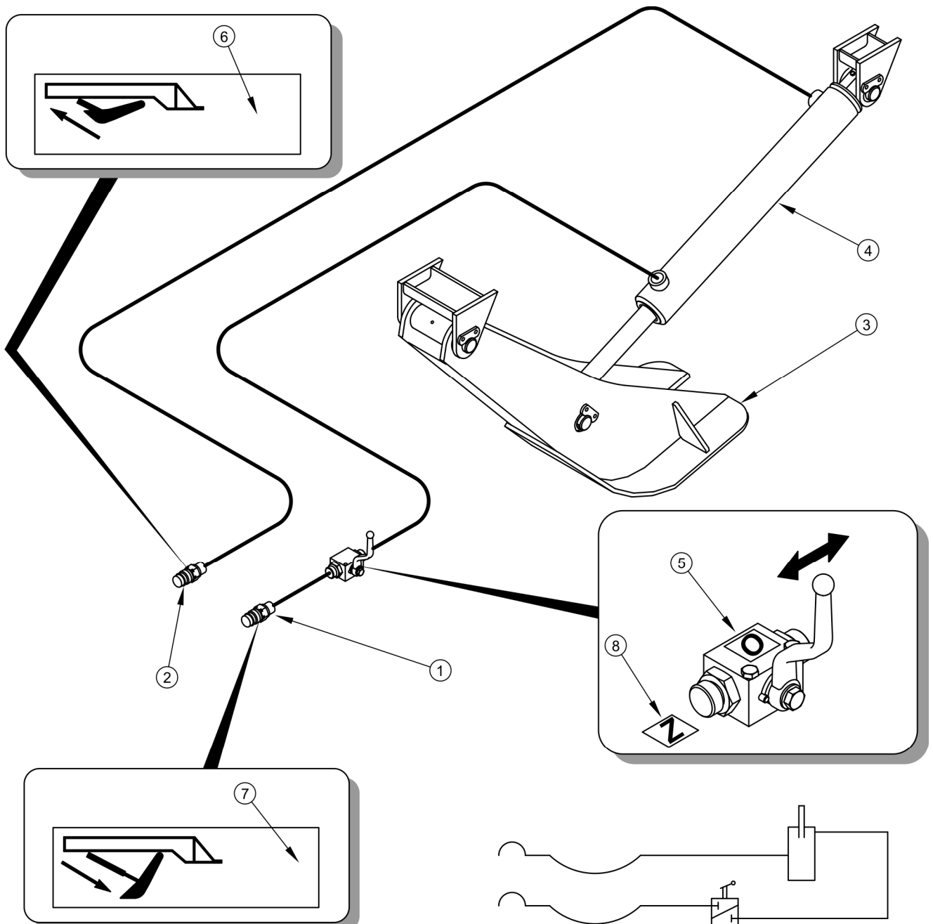
RYСУNEK 3.10 Budowa i schemat instalacji hydraulicznej podpory nożycowej
