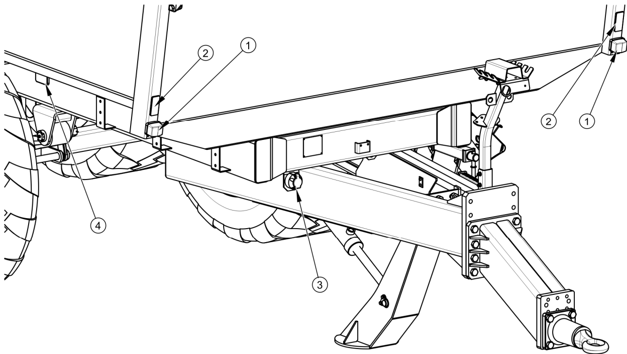
RYSUNEK 3.13 Rozmieszczenie elementów elektrycznych i odblaskowych z przodu
