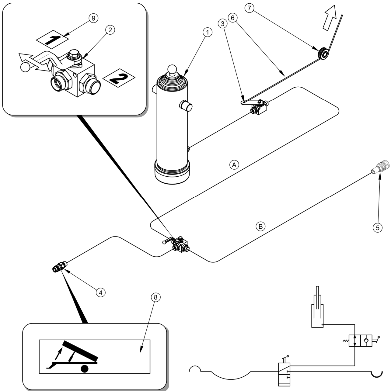
RYSUNEK 3.8 Budowa i schemat instalacji hydraulicznej wywrotu
