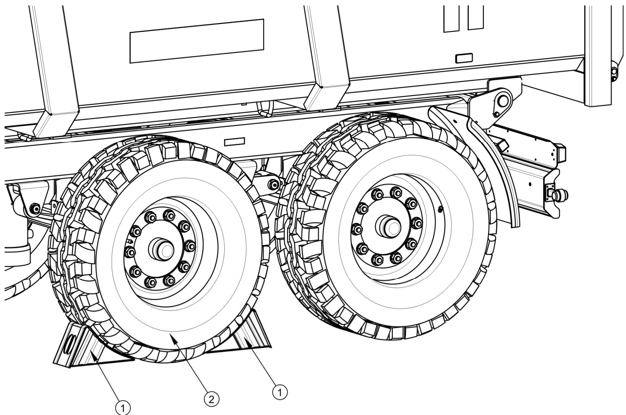
RYSUNEK 2.1 Sposób ustawiania klinów
