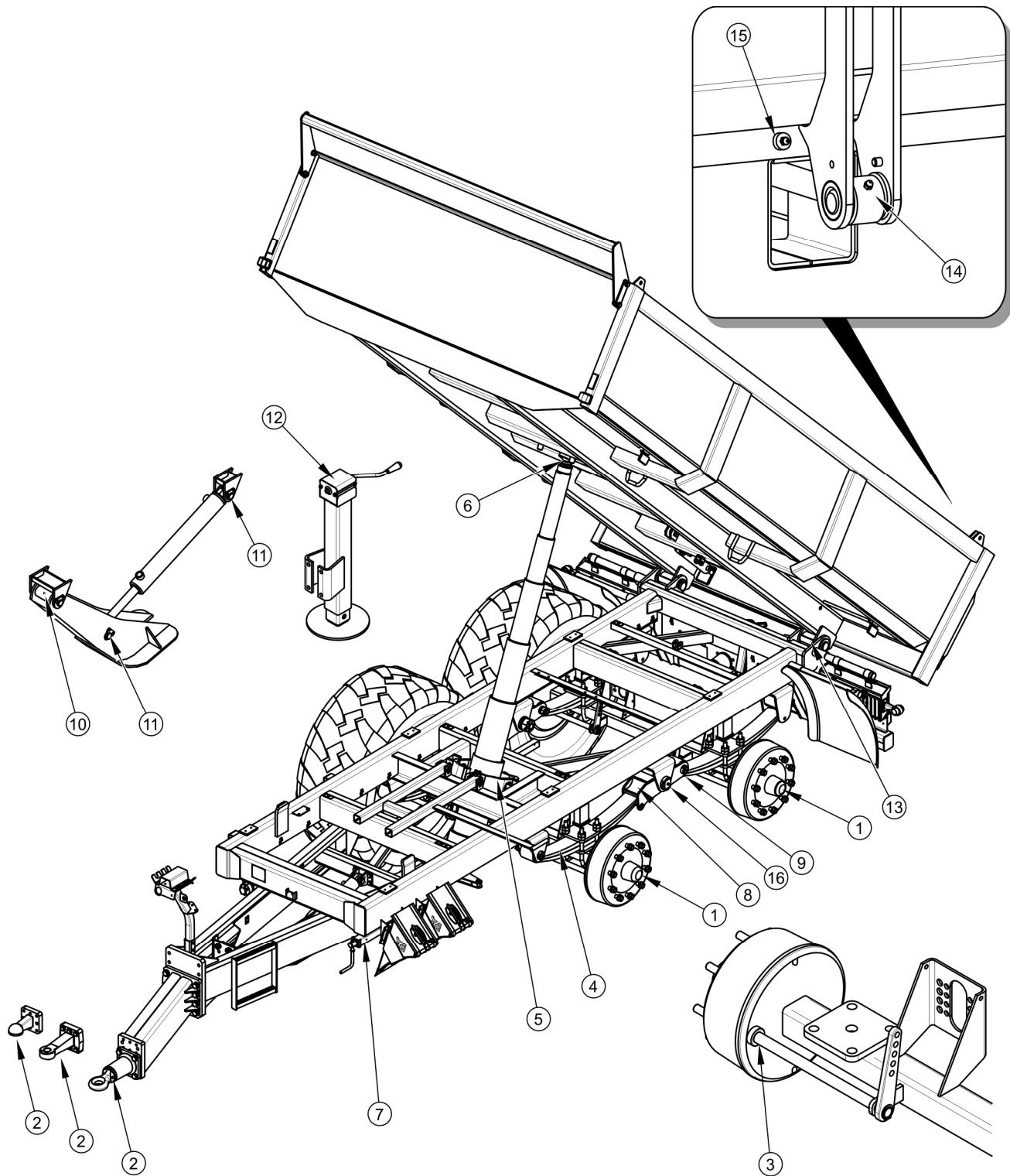
RYSUNEK 5.11 Punkty smarne przyczepy
