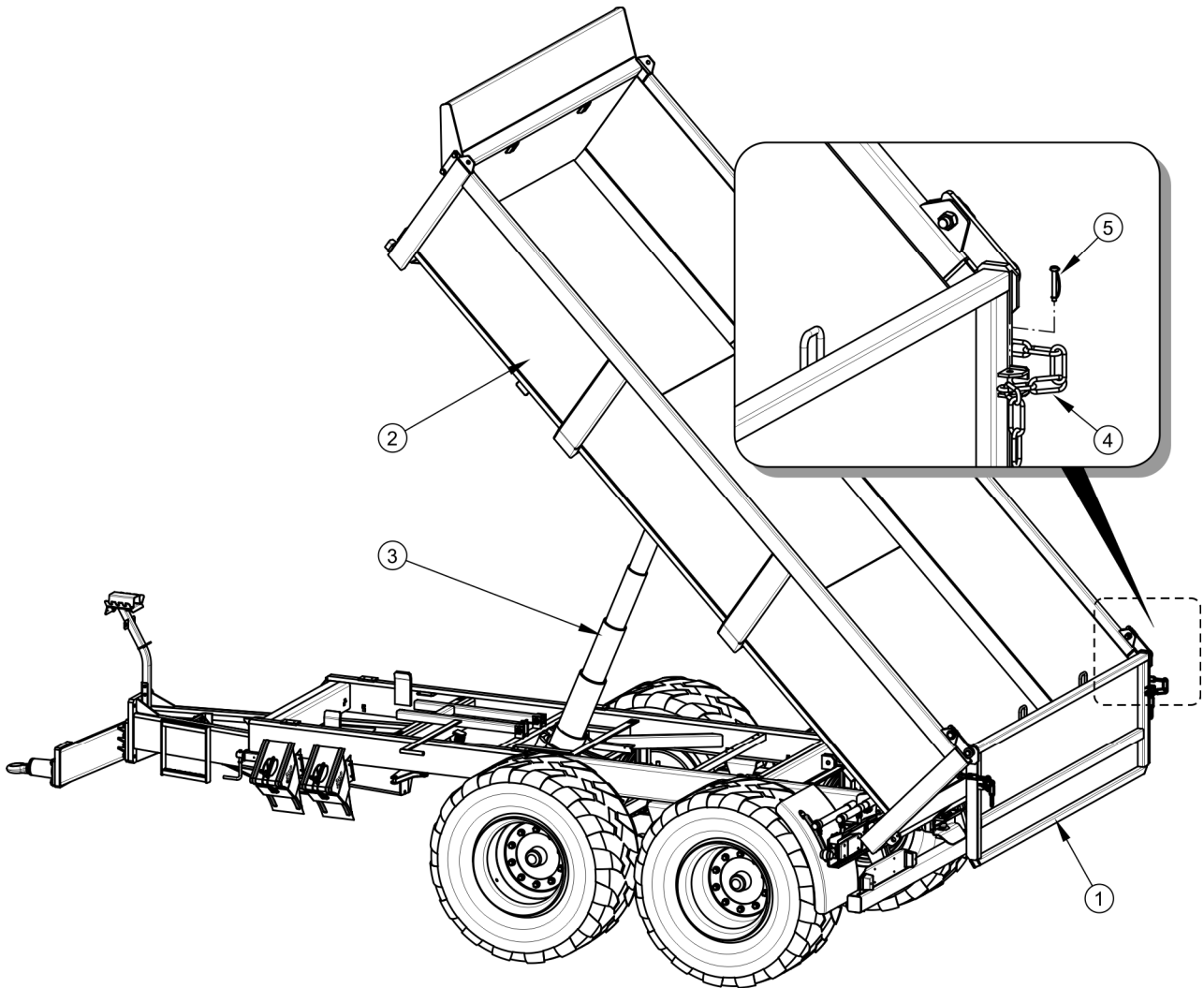
RYSUNEK 4.2 Rozładunek skrzyni ładunkowej z klapą uchylną
