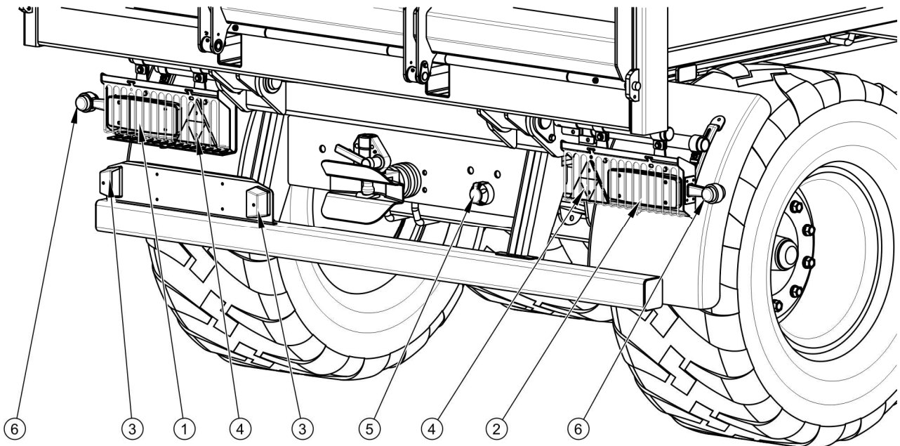
RYSUNEK 3.14 Rozmieszczenie elementów elektrycznych i odblaskowych z tyłu
