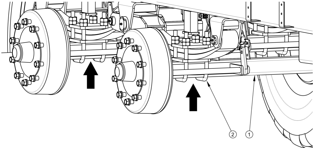
RYСУNEK 5.2 Punkt podparcia podnośnika
