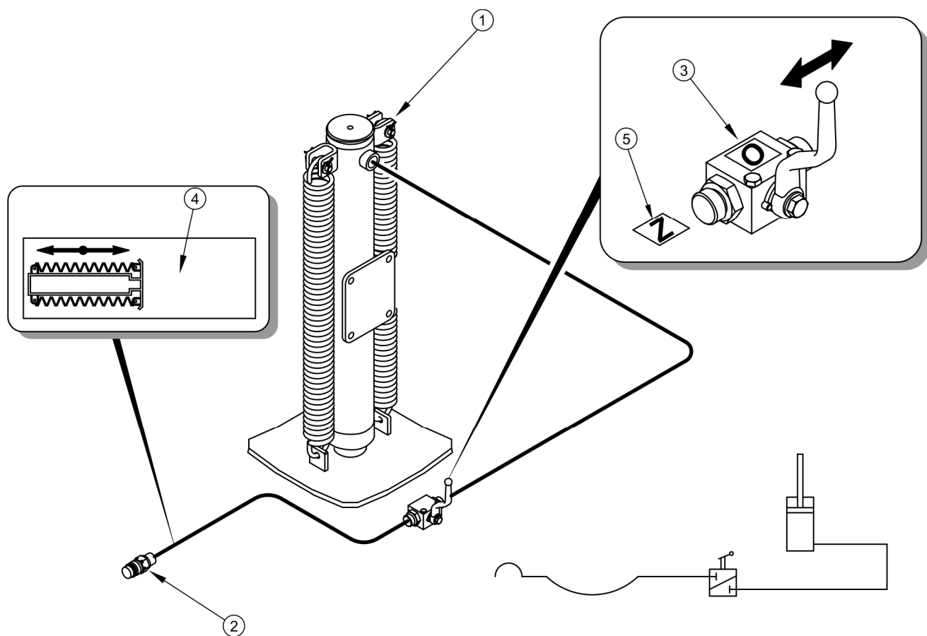
RYСУNEK 3.9 Budowa i schemat instalacji hydraulicznej podpory prostej
