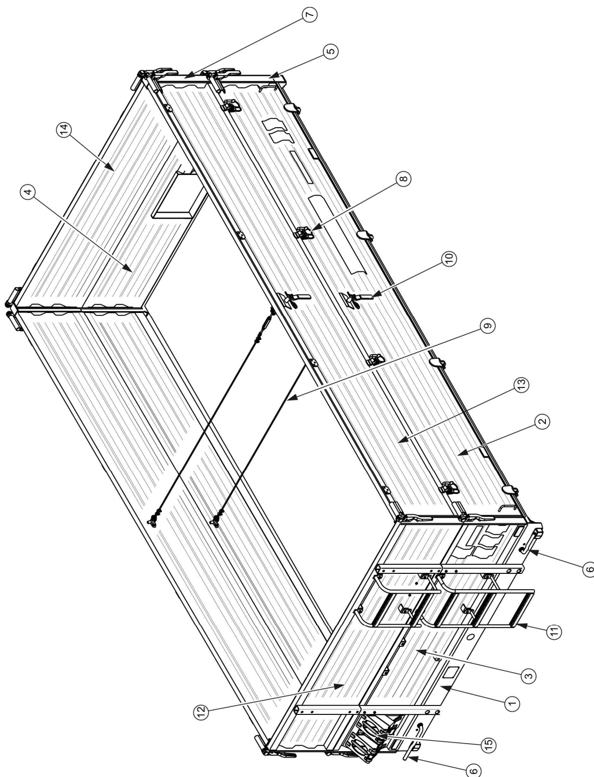
RYSUNEK 3.4 Skrzynia ładunkowa
