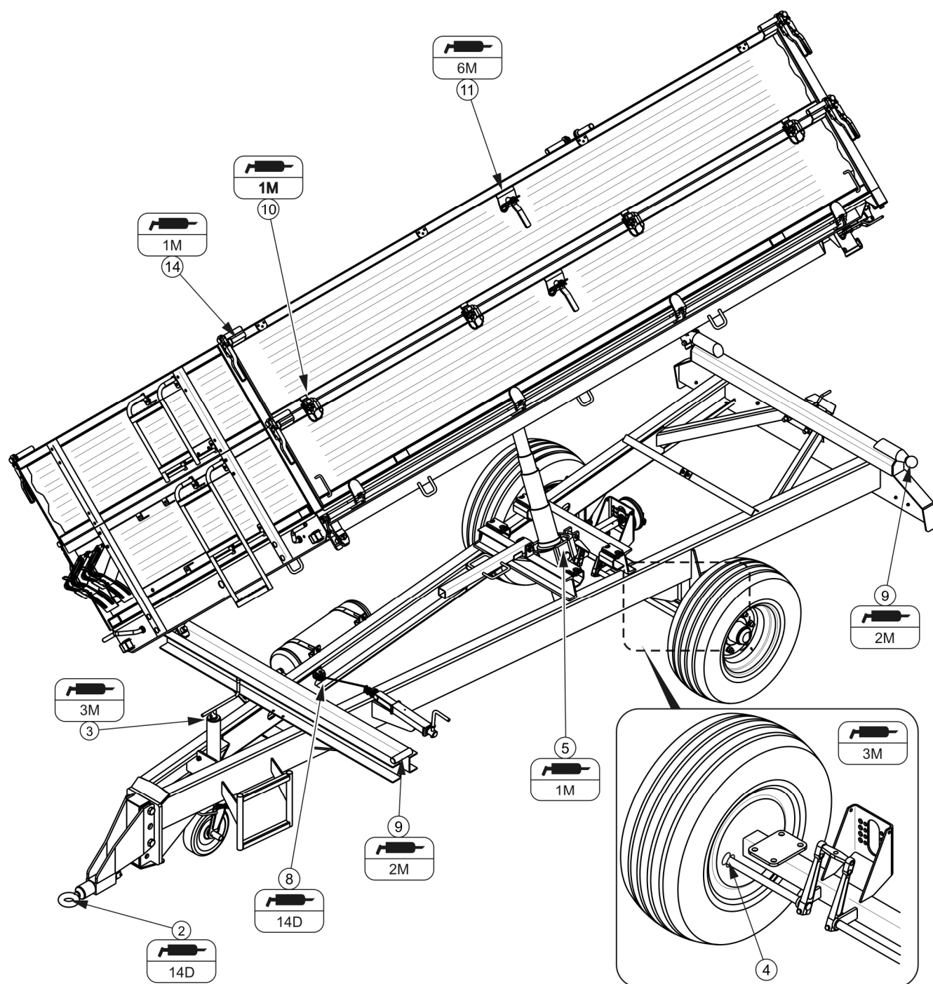
RYSUNEK 5.9 Punkty smarne przyczepy, część 1
