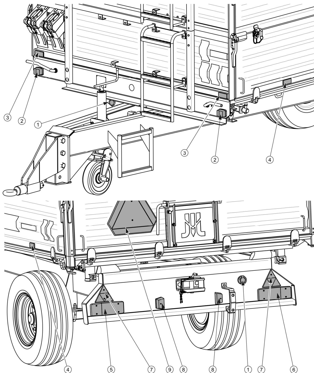
RYSUNEK 3.15 Rozmieszczenie elementów elektrycznych i odblaskowych
