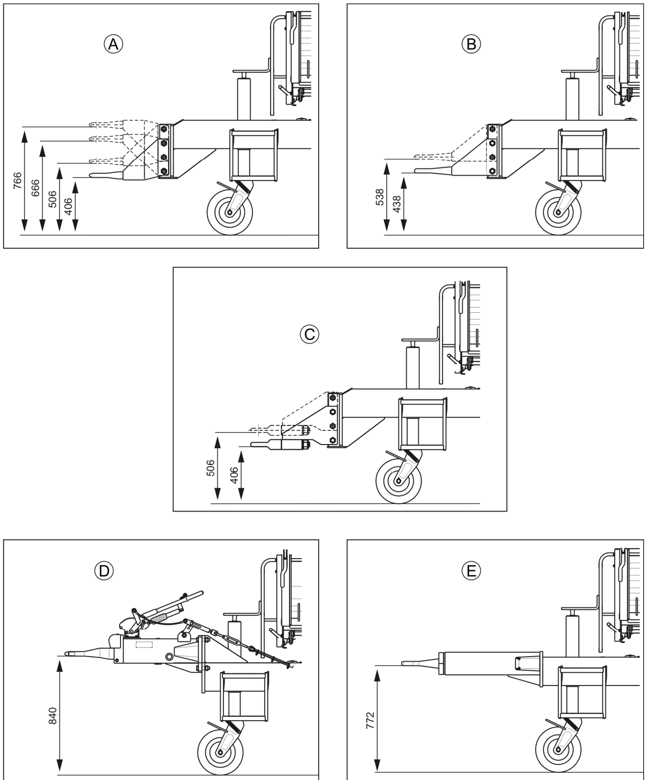
RYSUNEK 5.14 Zmiana wysokości położenia dyszli
