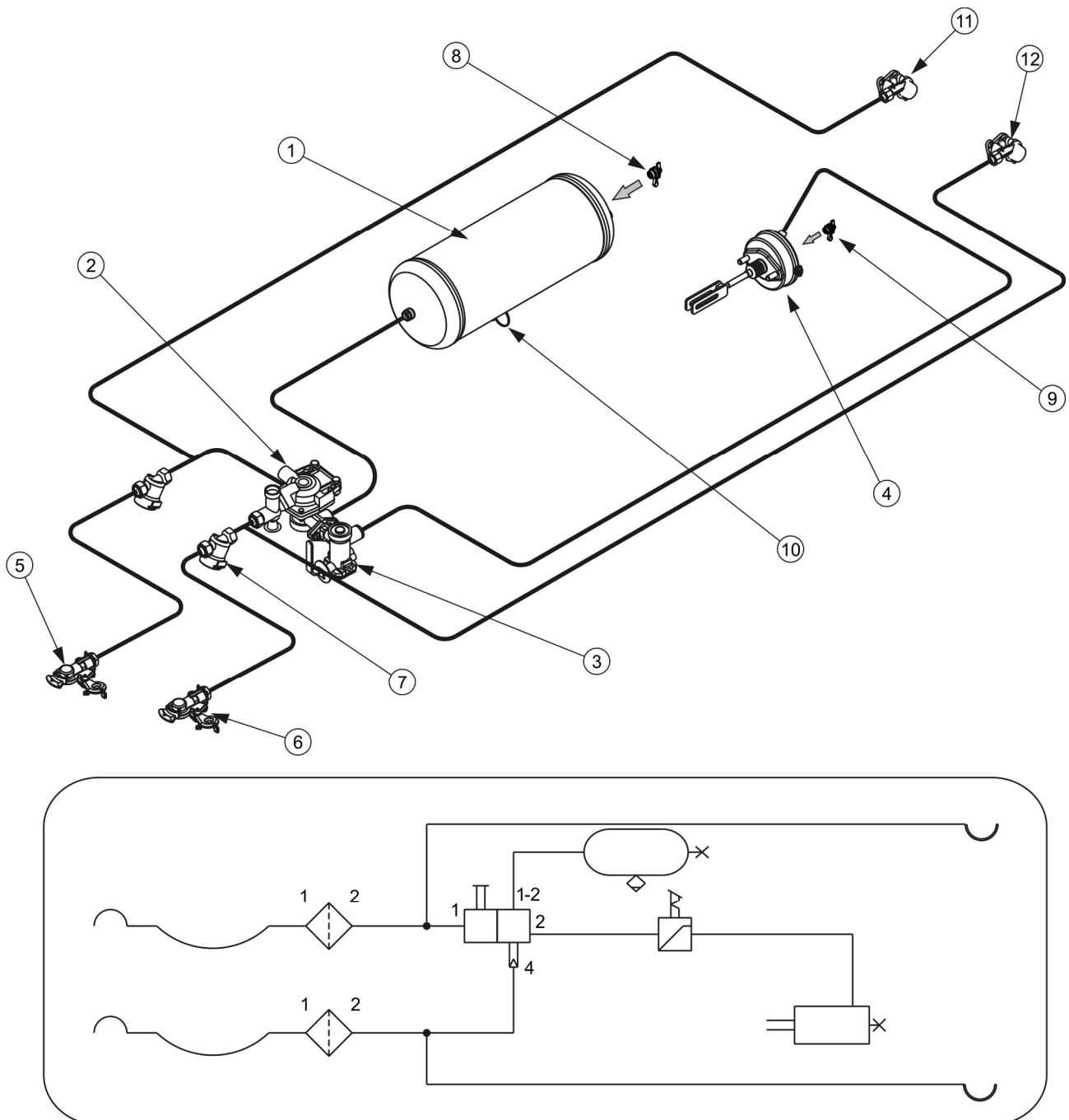
RYSUNEK 3.7 Budowa i schemat instalacji hamulcowej pneumatycznej dwuprzewodowej
