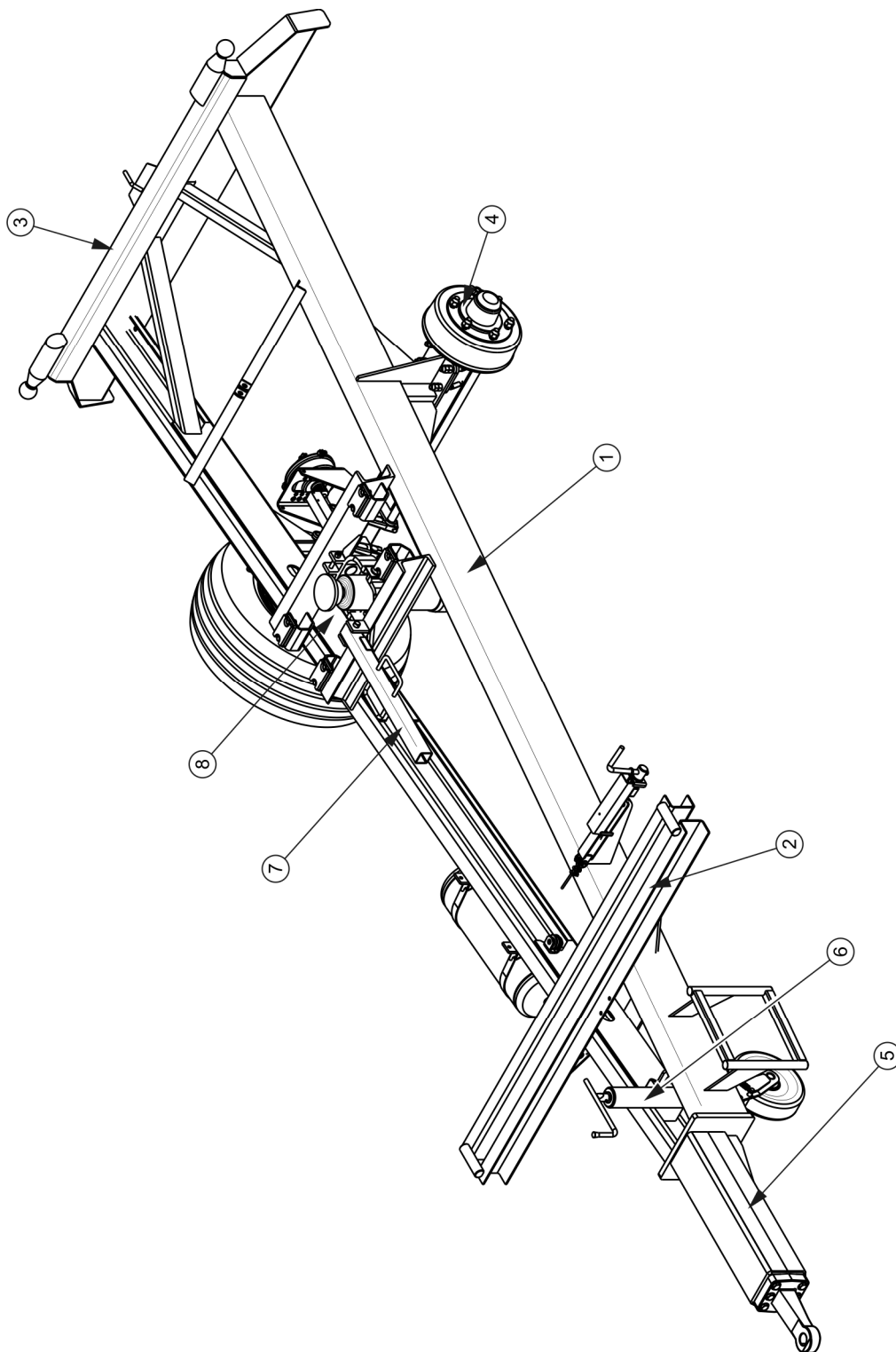
RYСУNEK 3.2 Podwozie przyczepy z dyszlem górnym
