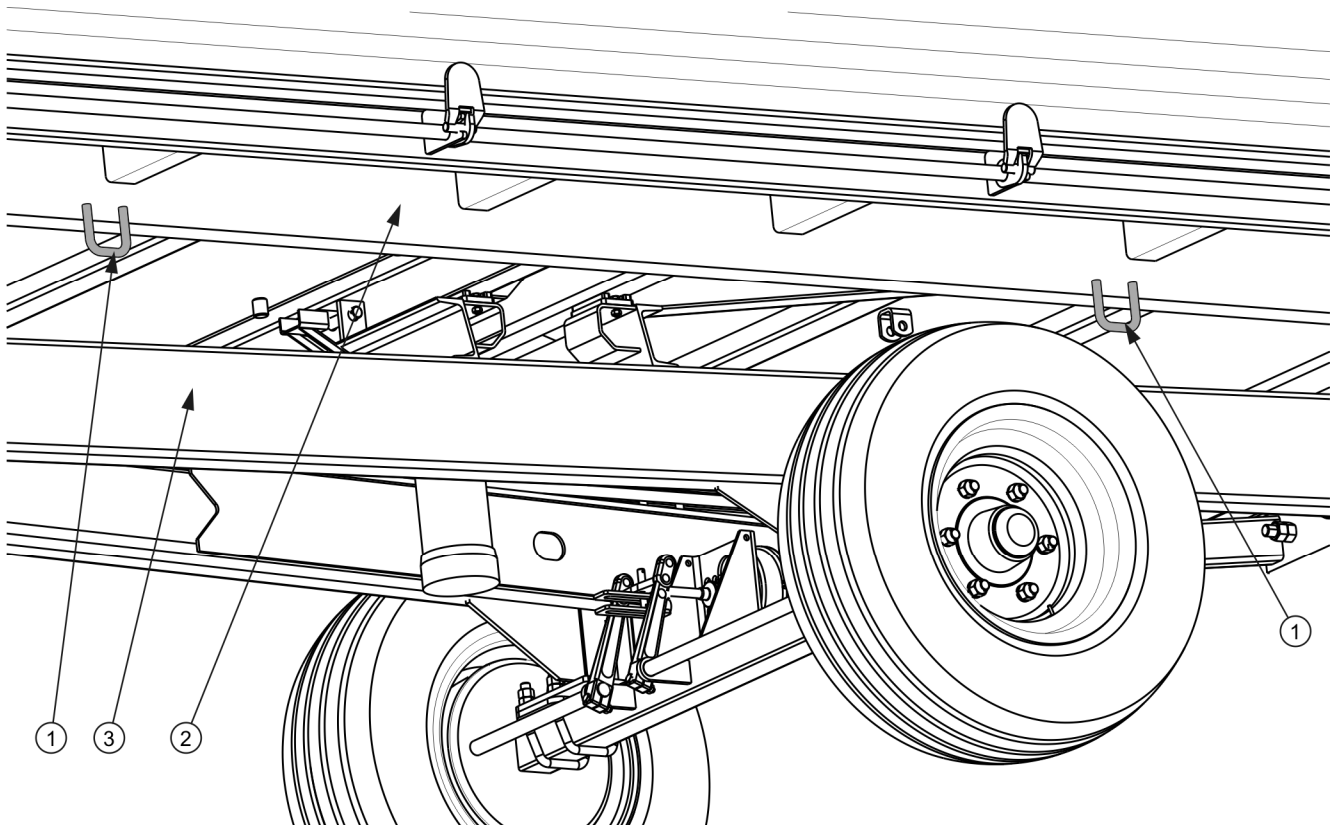
RYСУNEK 1.3 Rozmieszczenie uchwytów transportowych
