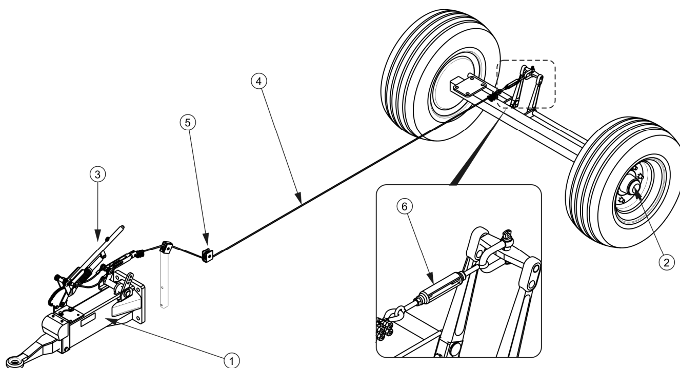
RYСУNEK 3.10 Hamulec najazdowy
