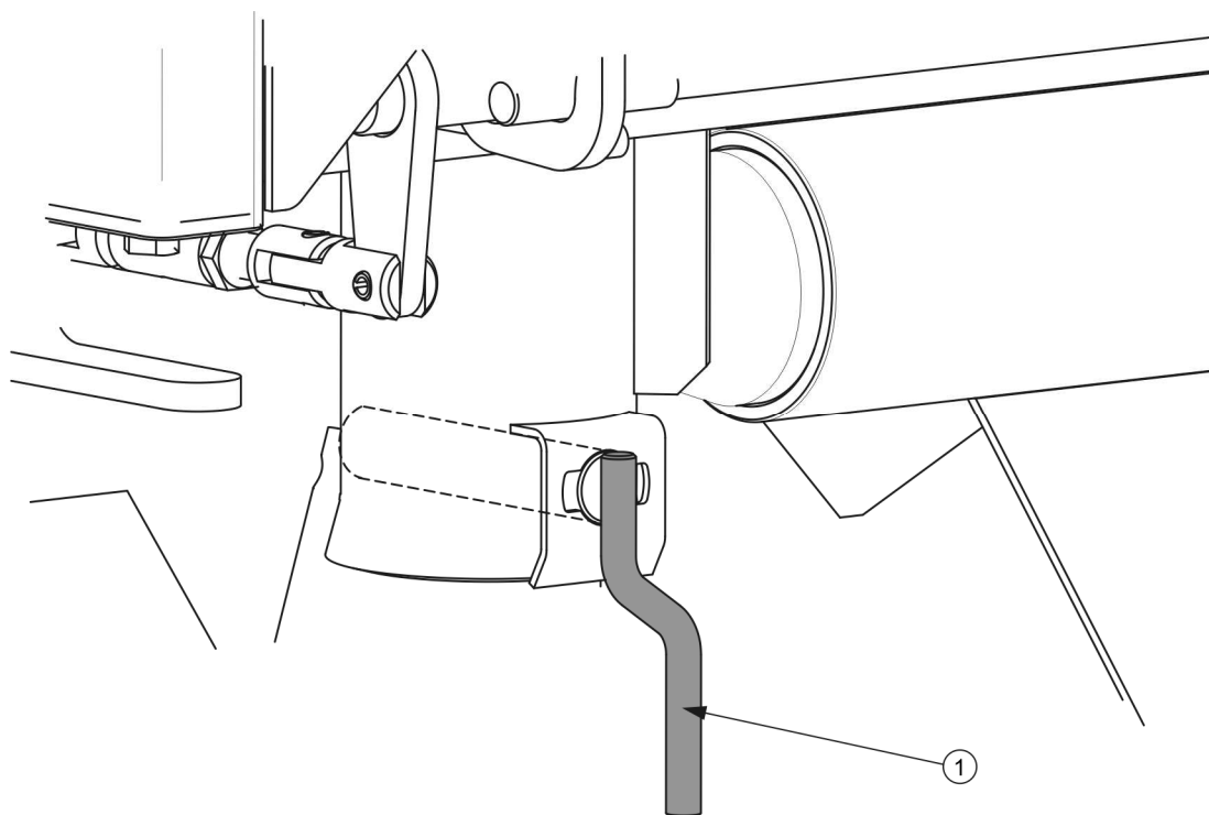
RYSUNEK 4.4 Ryglowanie sworzni wywrotu
