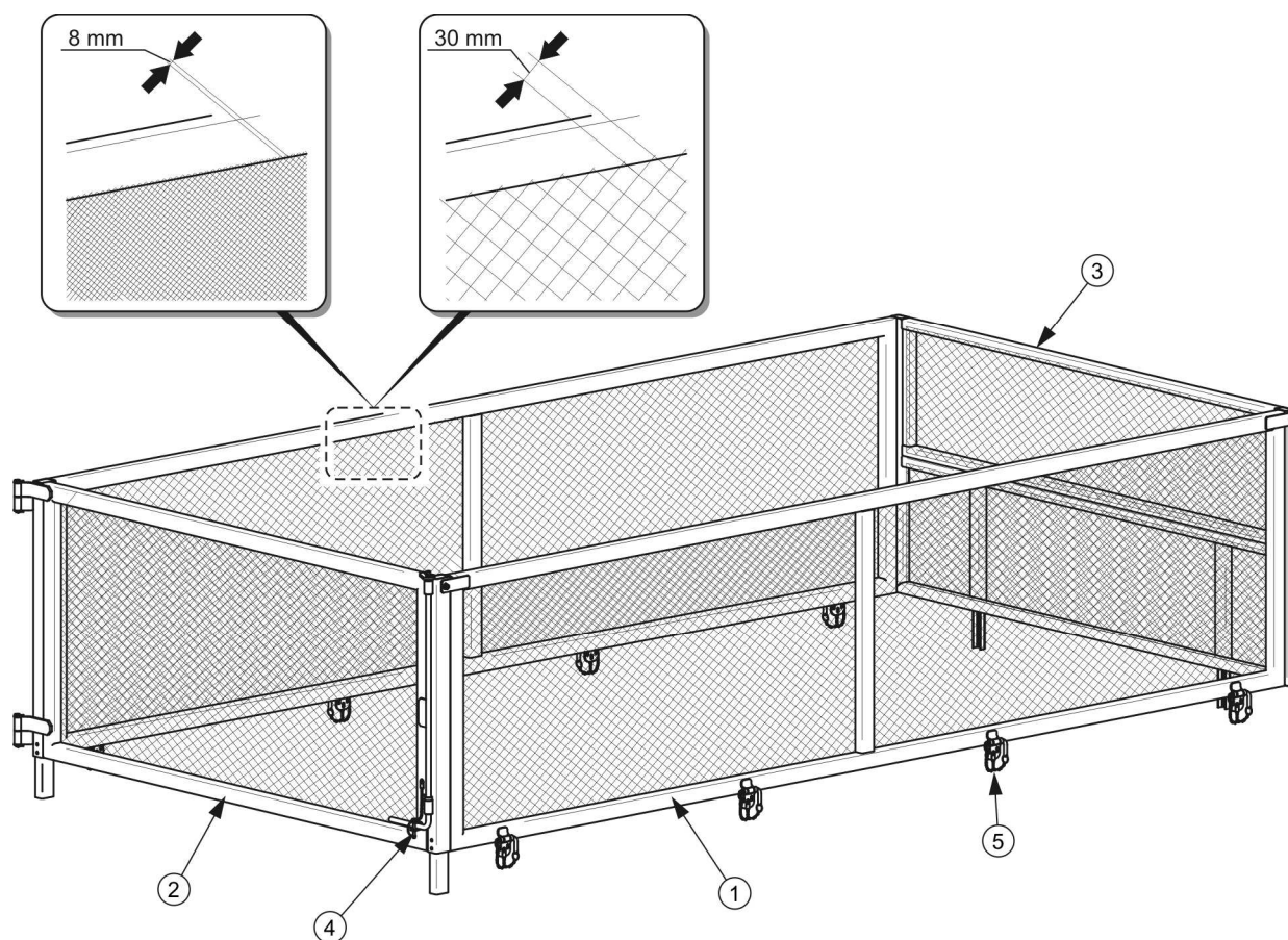
RYСУNEK 3.6 Nadstawy siatkowe 1 000 mm
