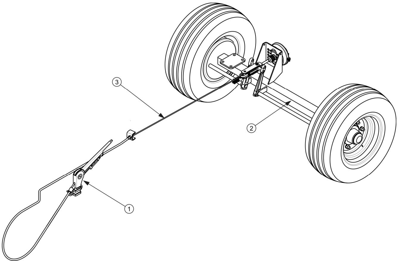
RYСУNEK 3.14 Hamulec ręczny dźwigniowy
