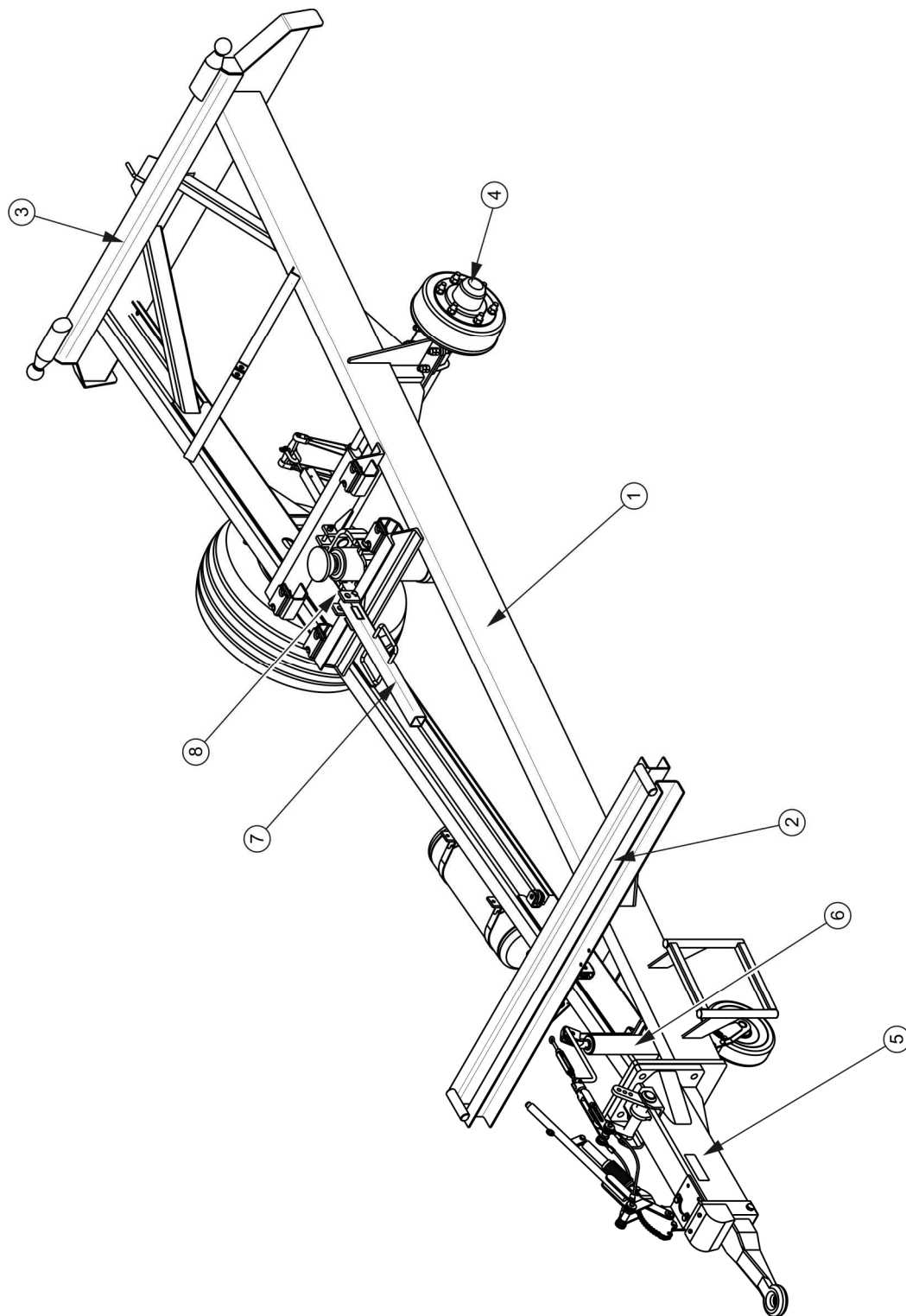
RYSUNEK 3.3 Podwozie przyczepy z dyszlem najazdowym
