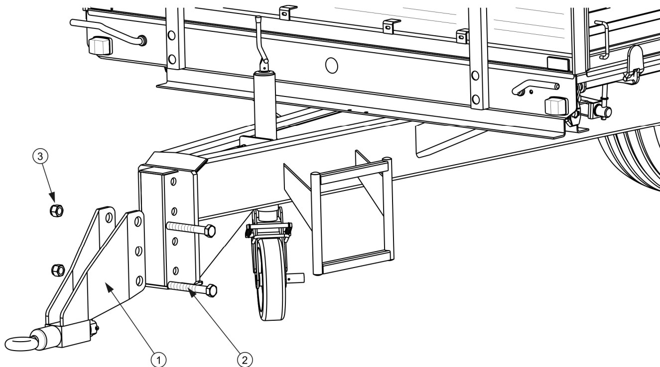
RYСУNEK 5.13 Regulacja położenia dyszla
