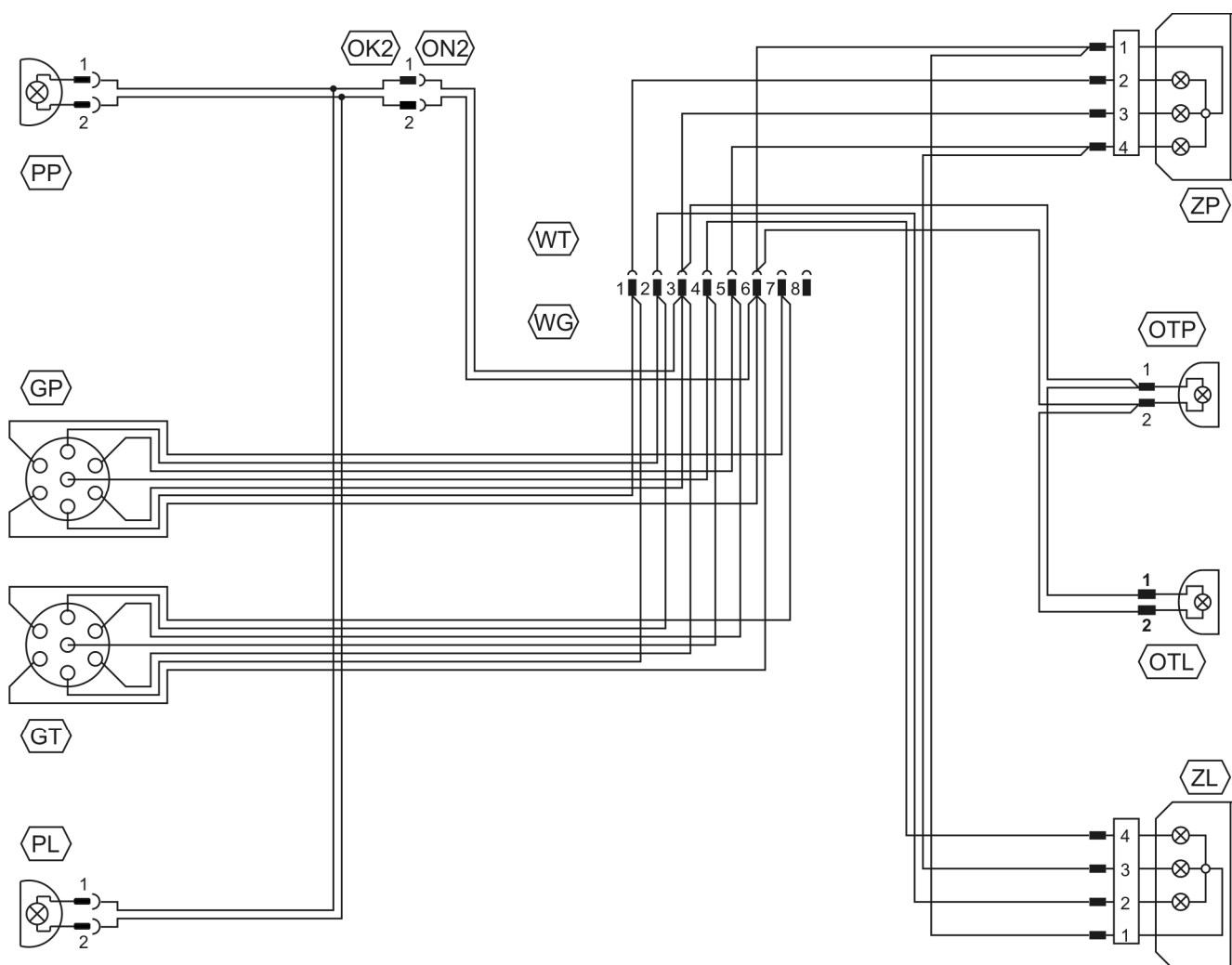
RYSUNEK 3.16 Schemat ideowy instalacji elektrycznej
