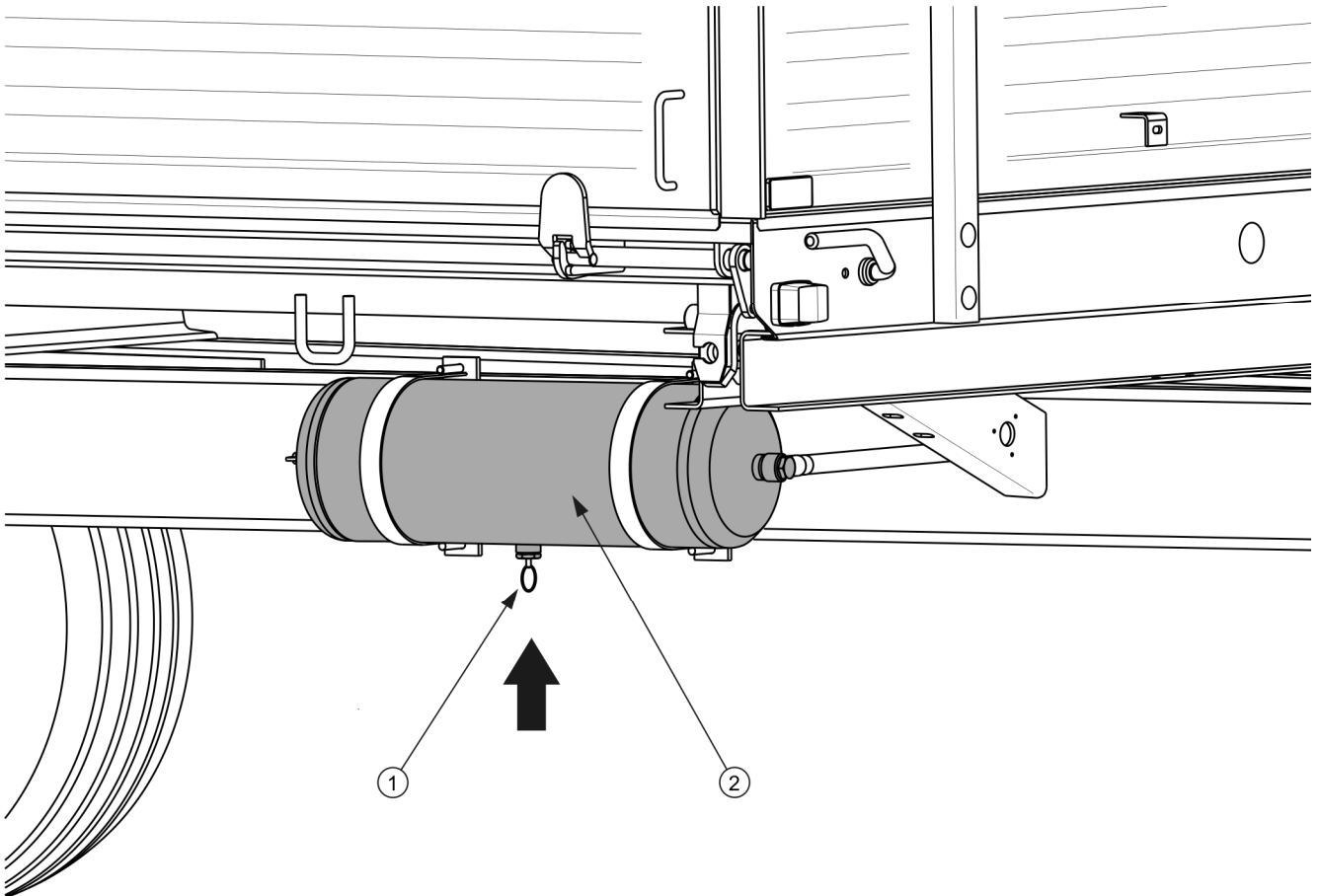
RYSUNEK 5.8 Odwadnianie zbiornika powietrza
