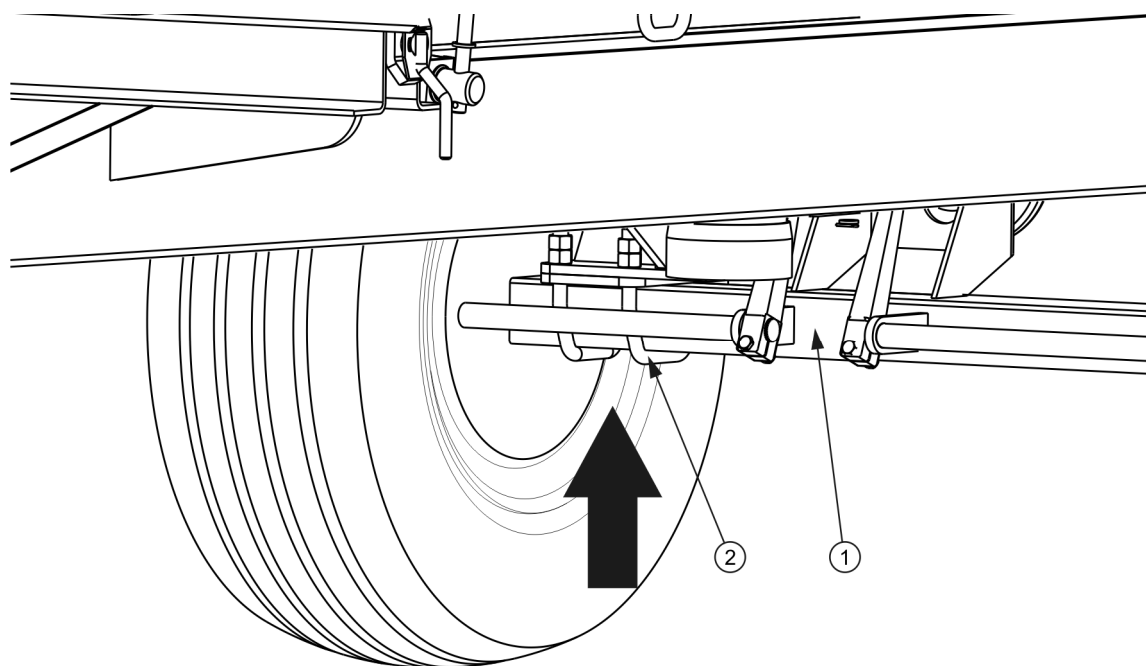
RYСУNEK 5.1 Punkt podparcia podnośnika
