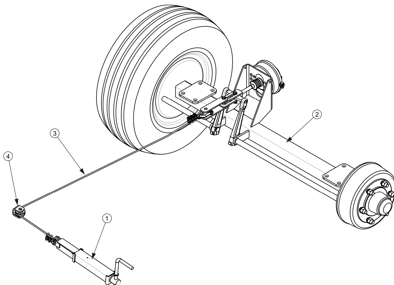
RYSUNEK 3.13 Hamulec ręczny korbowy
