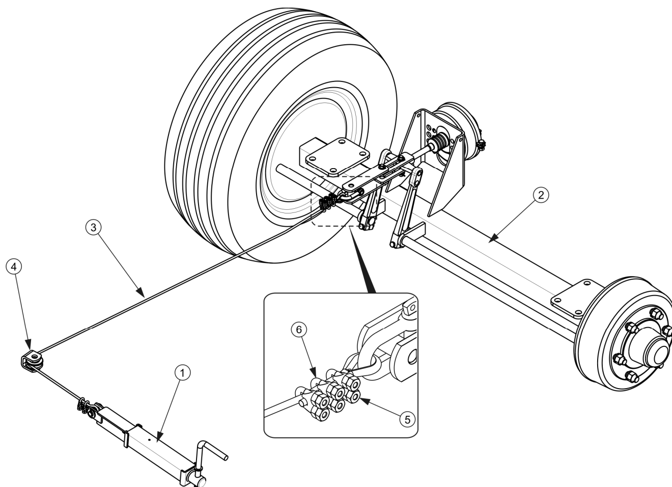
RYSUNEK 5.6 Regulacja napięcia linki hamulca postojowego
