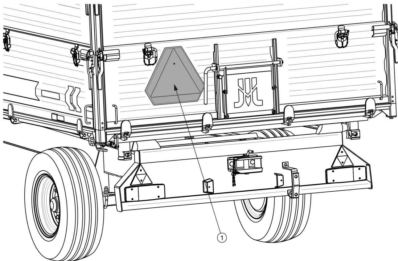
RYСУNEK 2.2 Miejsce montażu tablicy wyróżniającej pojazdy wolno poruszające się
