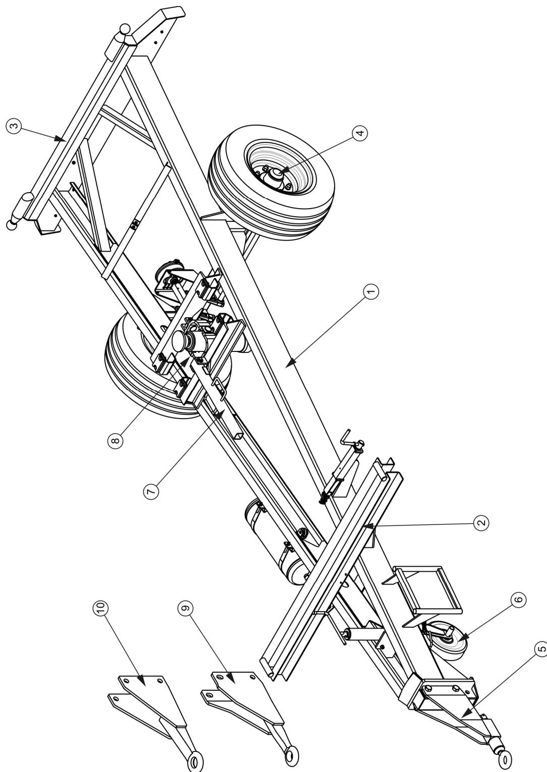
RYSUNEK 3.1 Podwozie przyczepy z dyszlem dolnym
