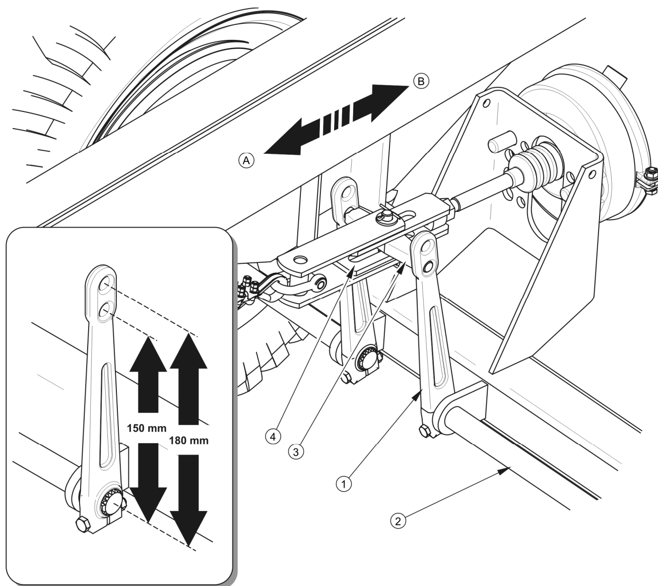
RYСУNEK 5.4 Regulacja hamulców mechanicznych osi jezdnych
