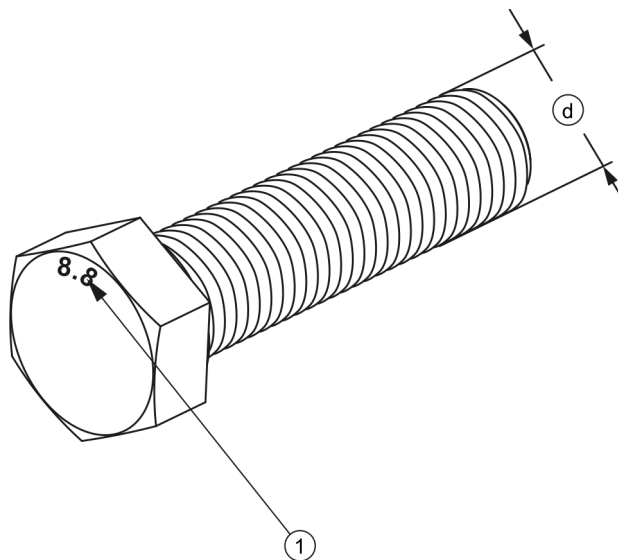
RYSUNEK 5.11 Śruba z gwintem metrycznym
