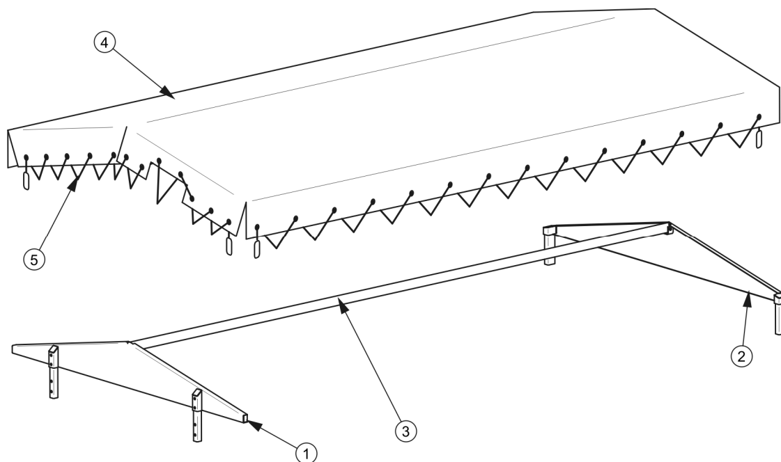
RYСУNEK 5.12 Stelaż z plandeką
