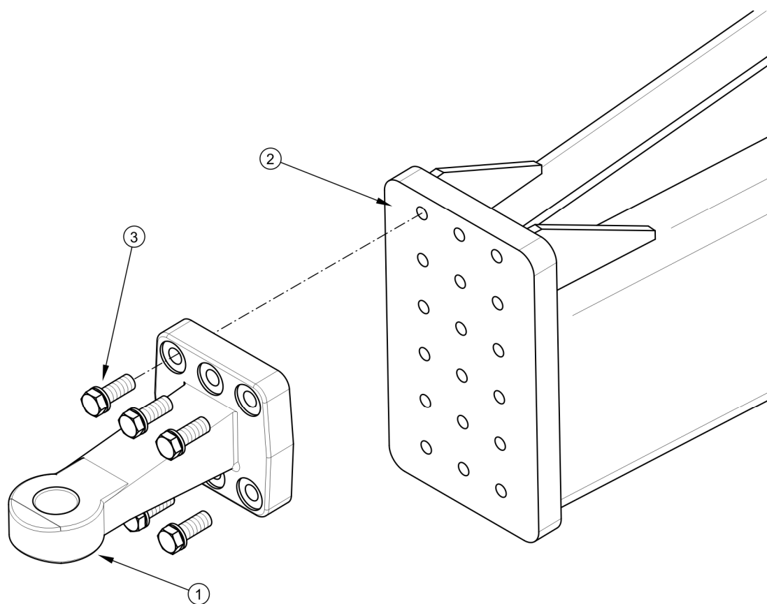
RYSUNEK 5.16 Regulacja położenia dyszla
