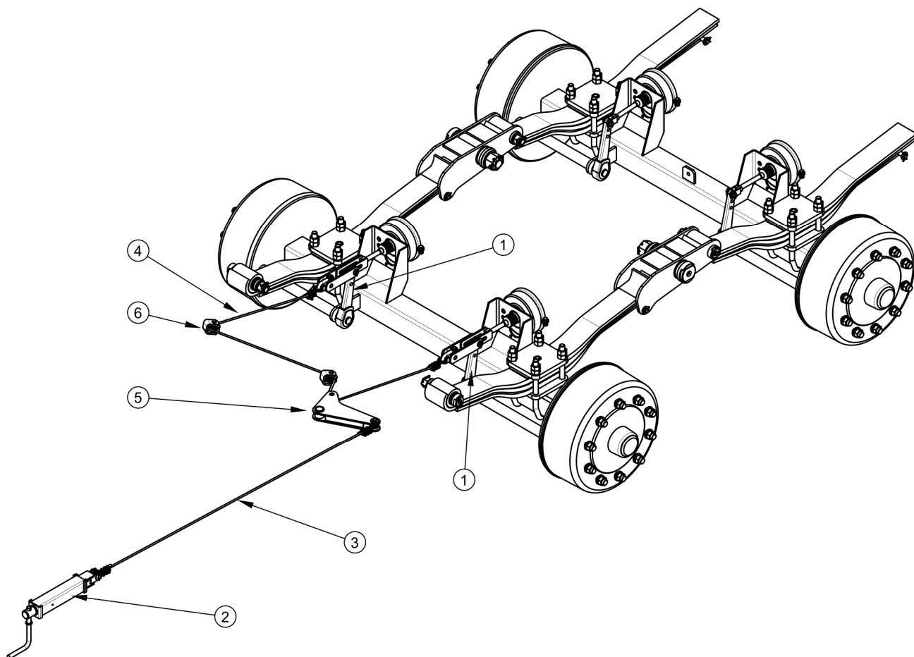
RYСУNEK 3.13 Budowa hamulca postojowego
