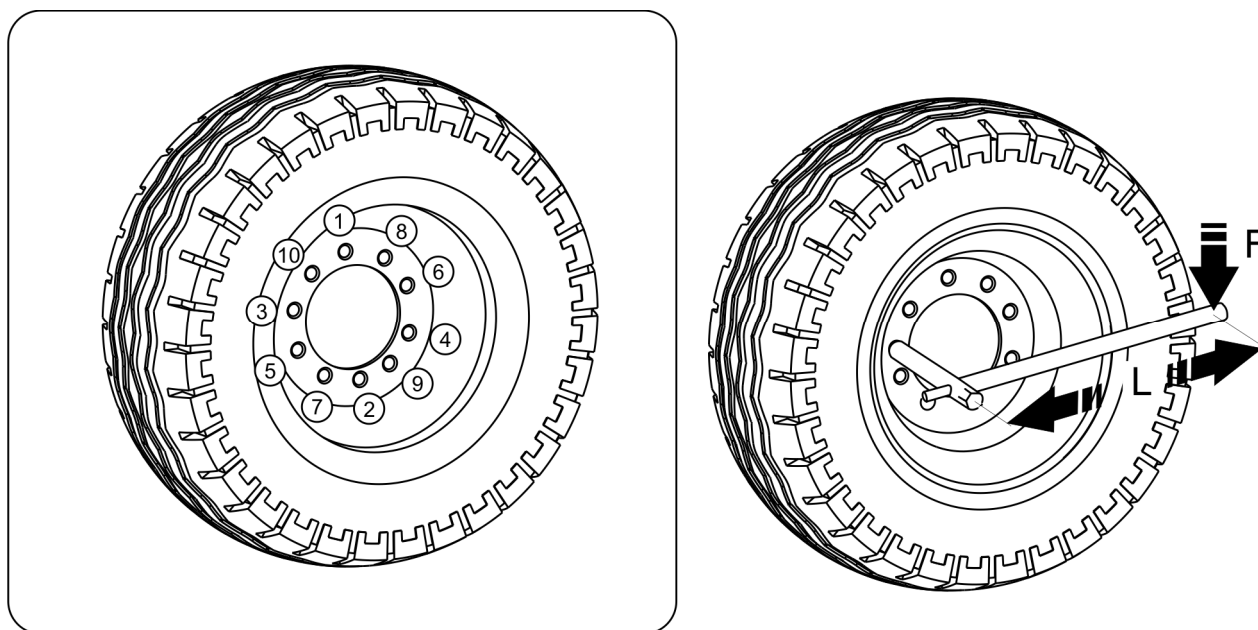
RYSUNEK 5.4 Kolejność dokręcania nakrętek, osie z 10 szpilek M22x1.5
