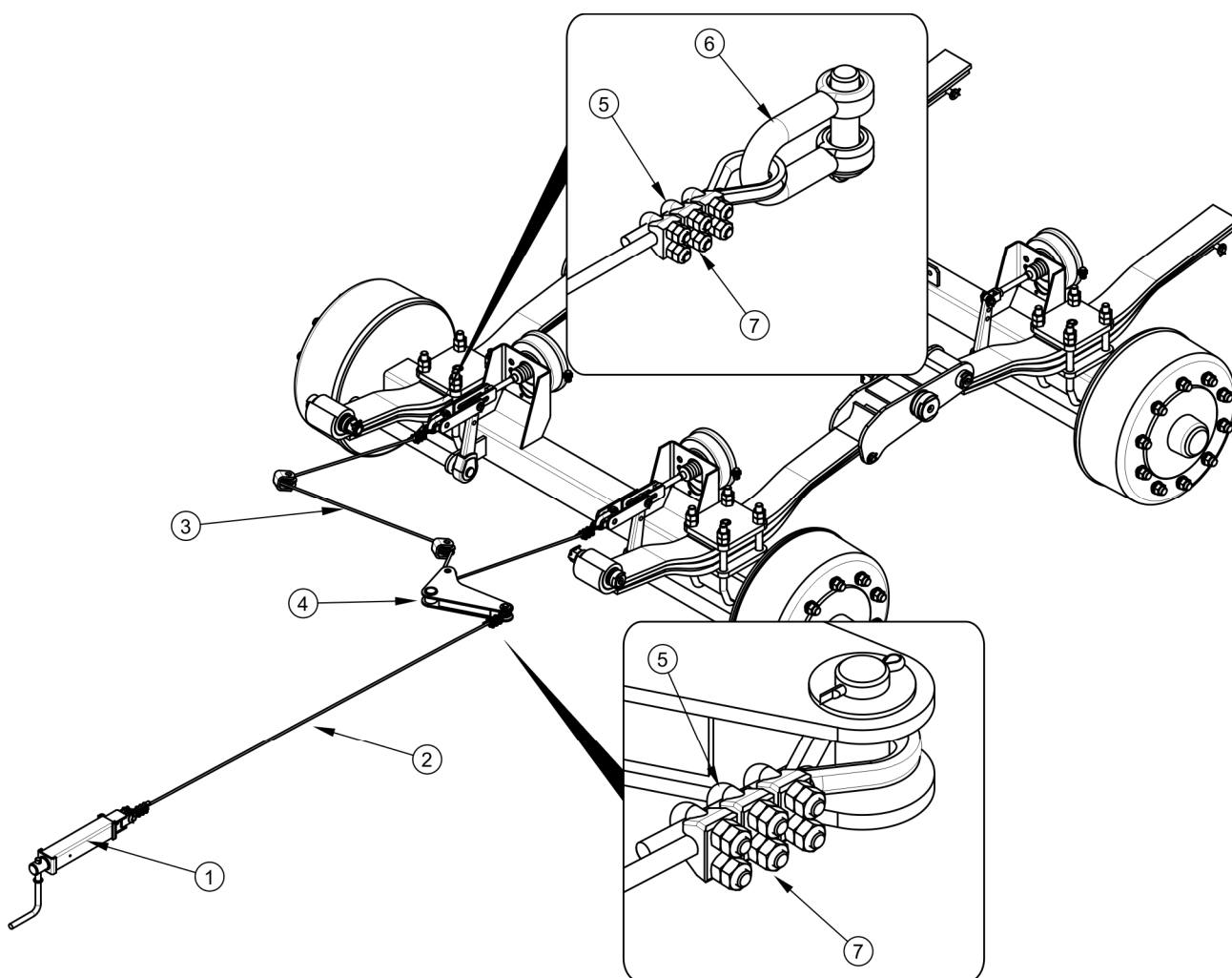
RYСУNEK 5.6 Regulacja napięcia linki hamulca postojowego
