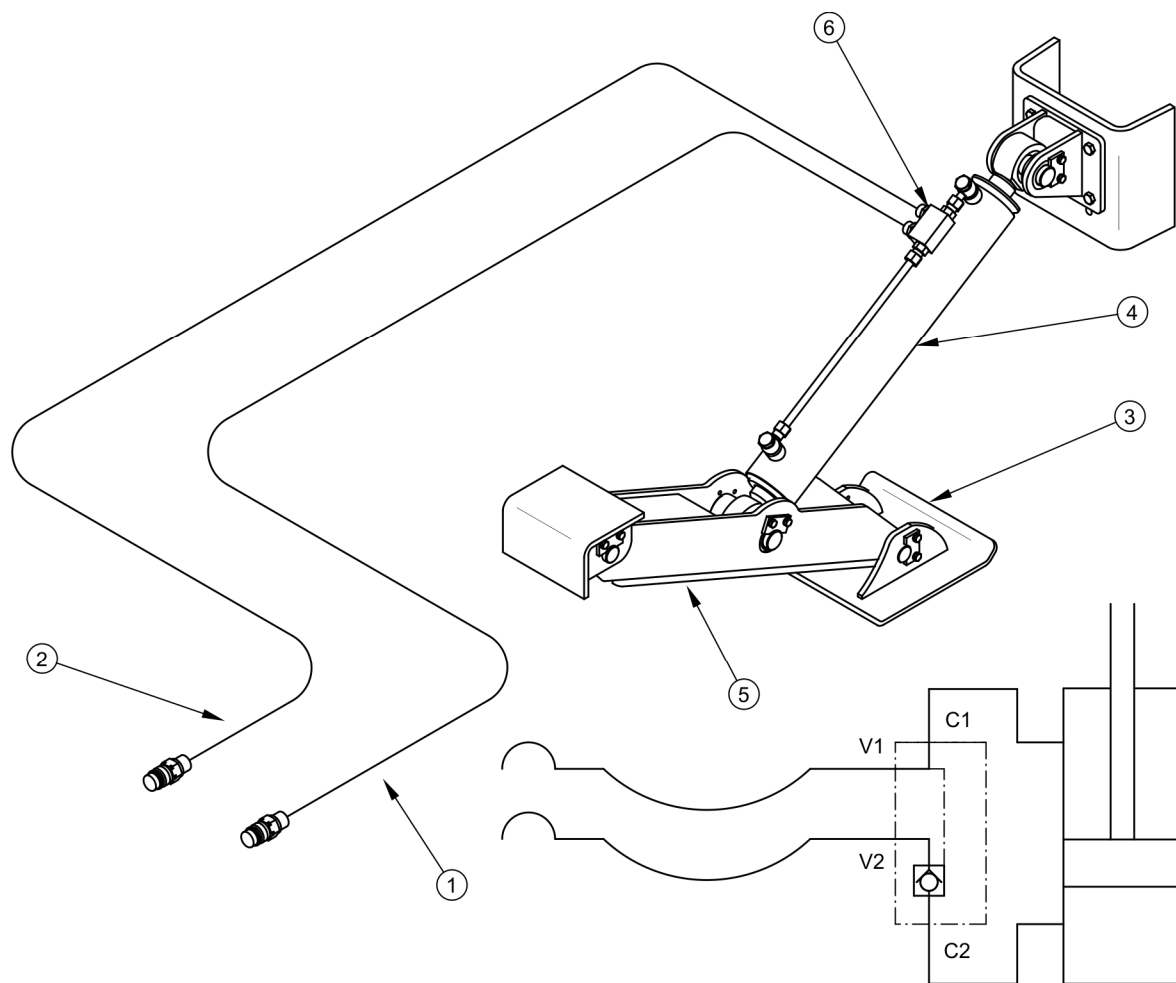
RYСУNEK 3.10 Budowa i schemat instalacji hydraulicznej podpory nożycowej
