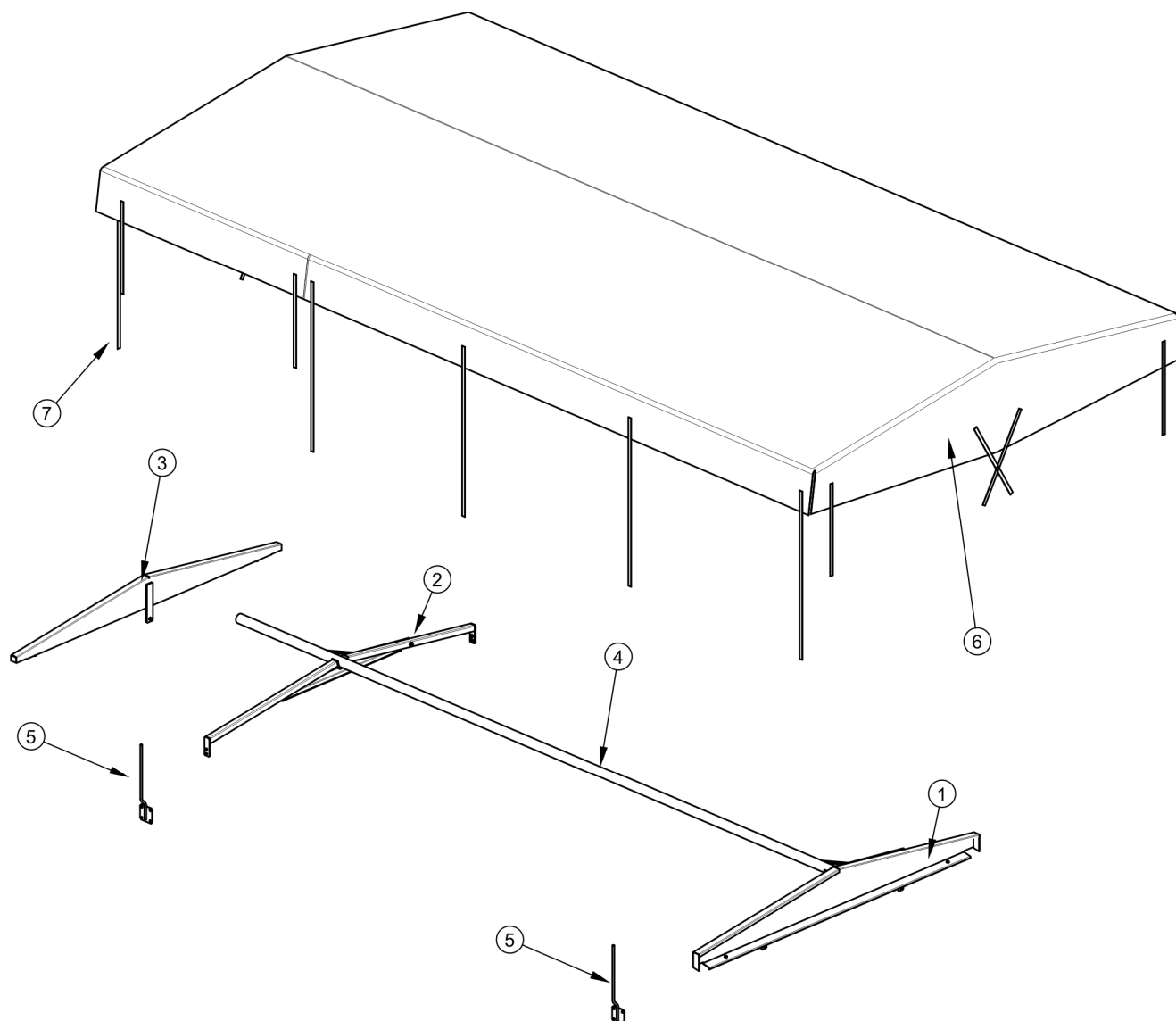
RYSUNEK 5.15 Stelaż z planeką
