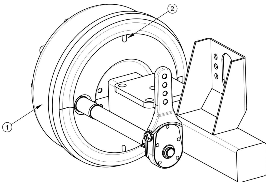
RYСУNEK 5.1 Kontrola okładzin hamulcowych
