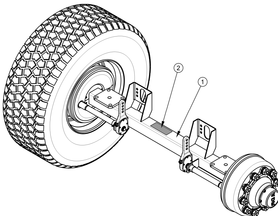
RYСУNEK 1.2 Miejsce umieszczenia tabliczki znamionowej osi jezdnej
