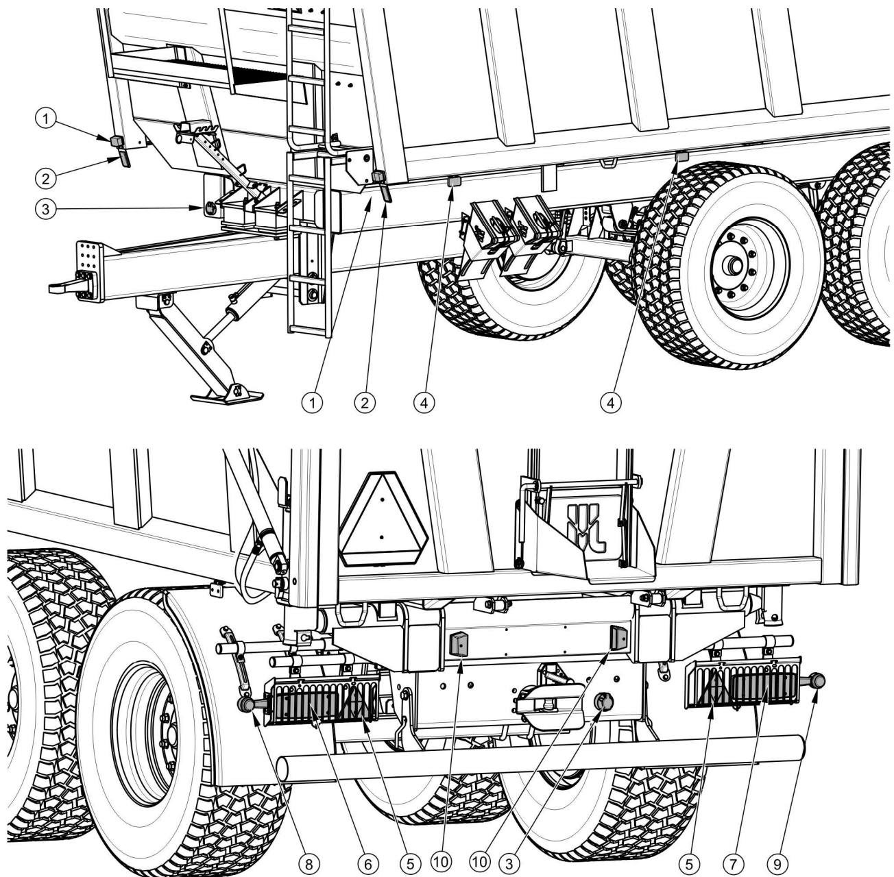
RYСУNEK 3.14 Rozmieszczenie elementów elektrycznych i odblaskowych
