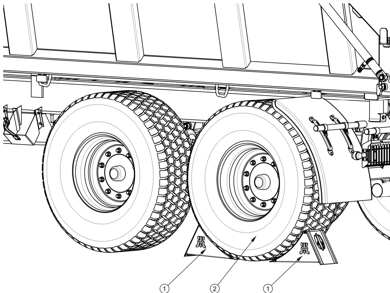
RYСУNEK 2.1 Sposób ustawiania klinów
