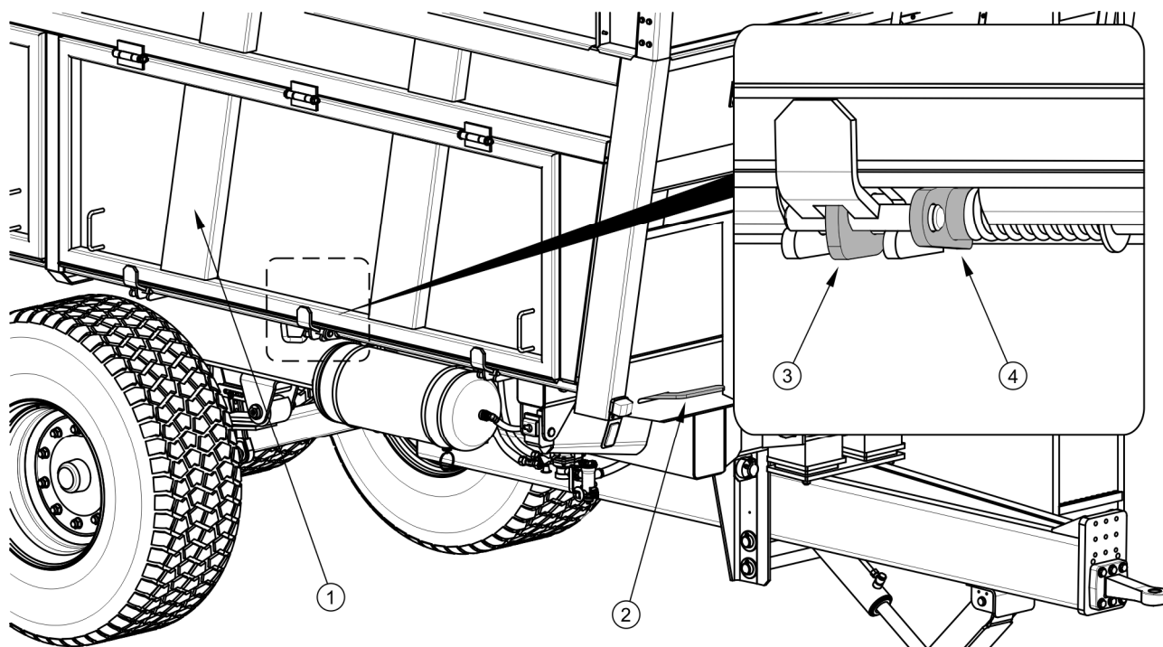
RYSUNEK 4.3 Otwieranie klap bocznych
