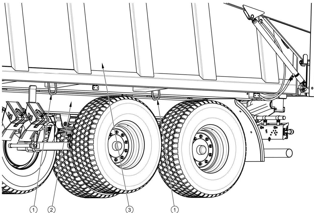
RYSUNEK 1.3 Rozmieszczenie uchwyty transportowych
