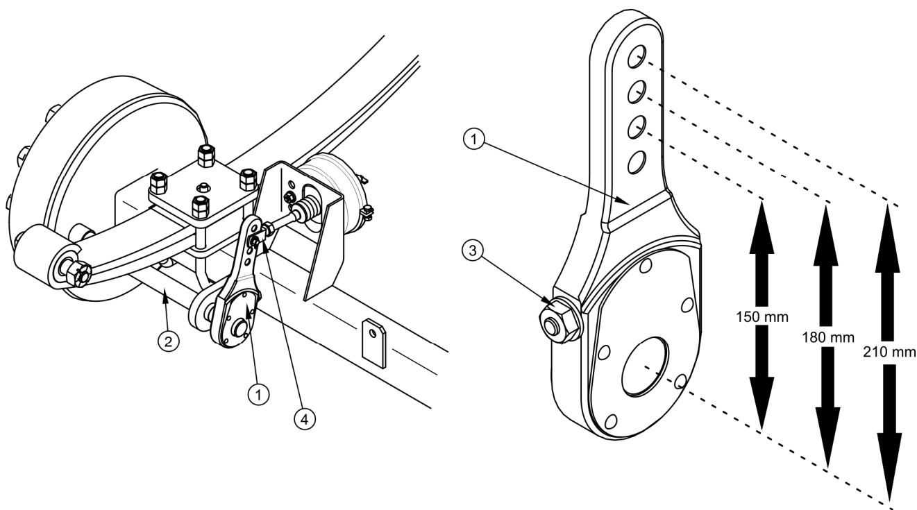
RYСУNEK 5.5 Regulacja hamulców mechanicznych osi jezdnych
