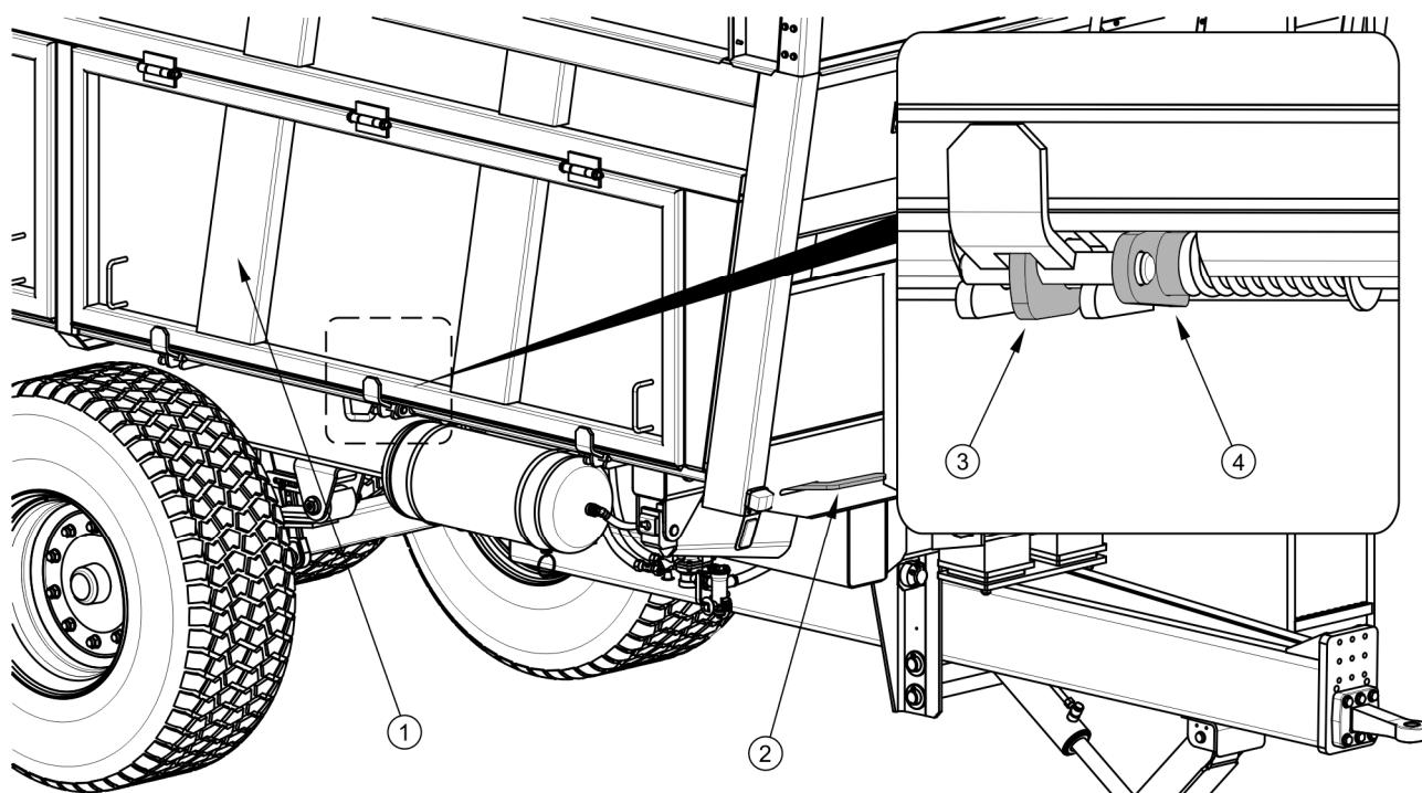
РИСУНОК 4.3 Открытие боковых бортов
