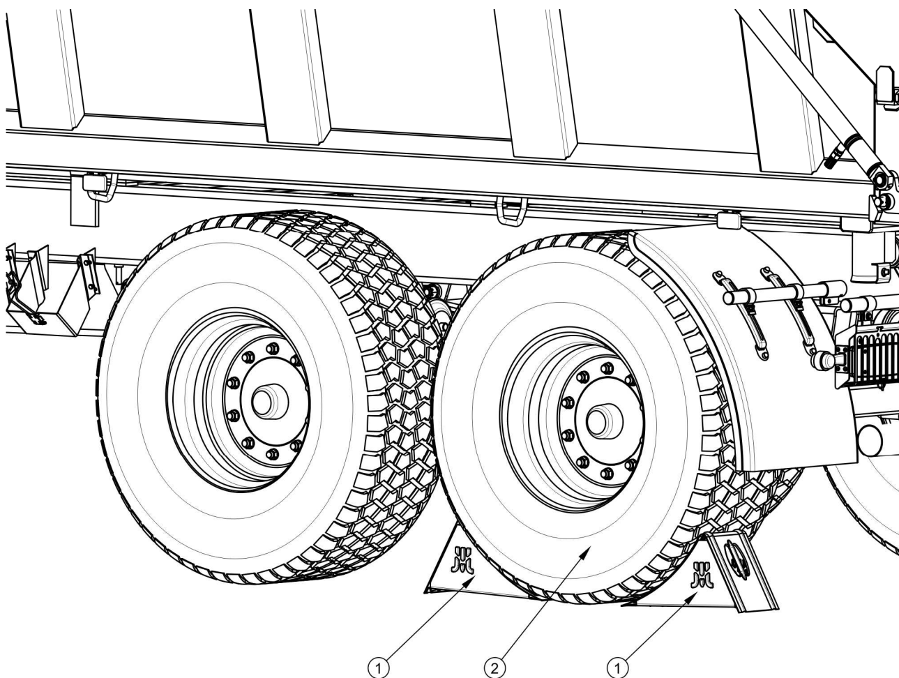
РИСУНОК 2.1 Способ установки клиньев
