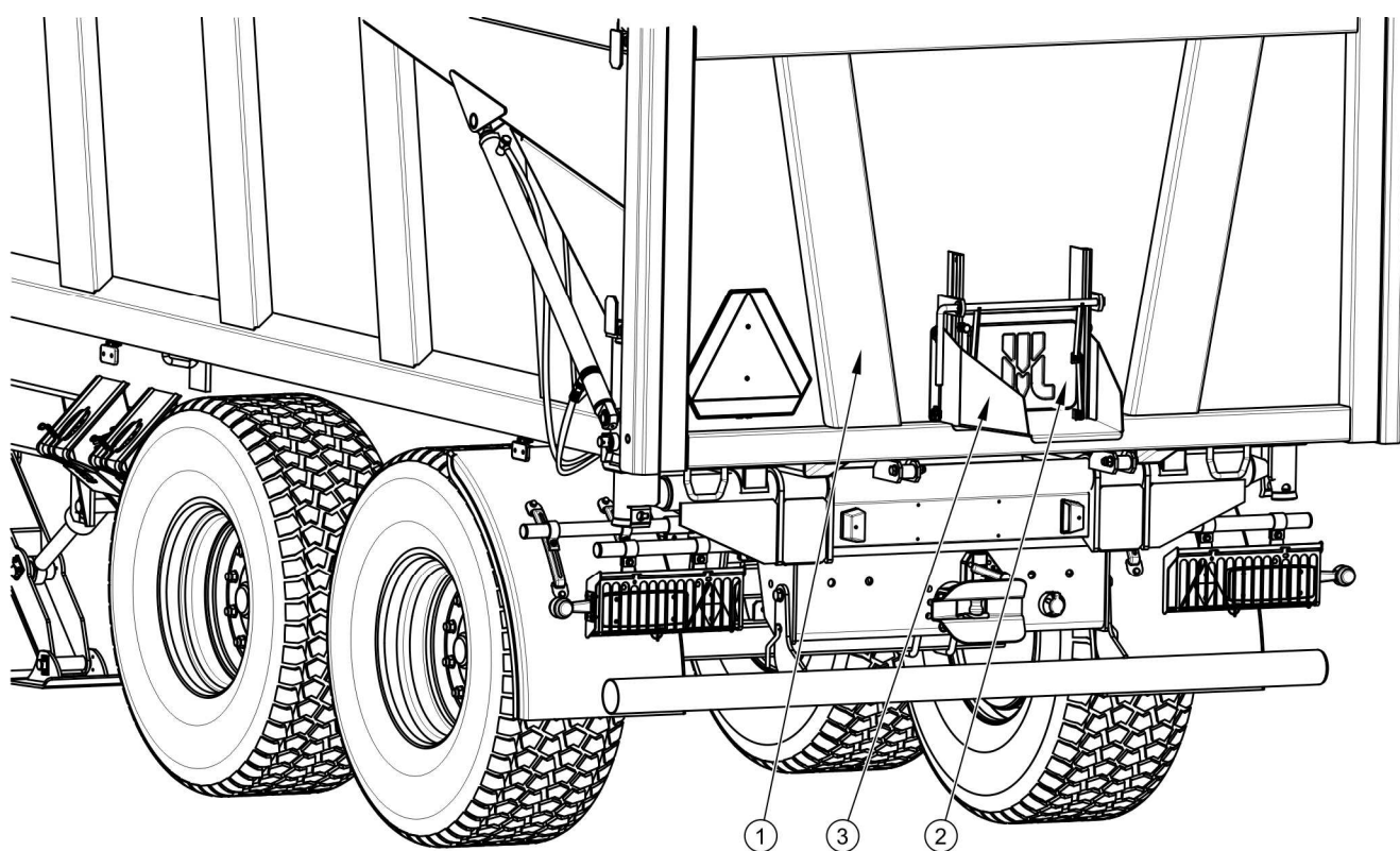
РИСУНОК 3.3 Разгрузочный люк в заднем борту
