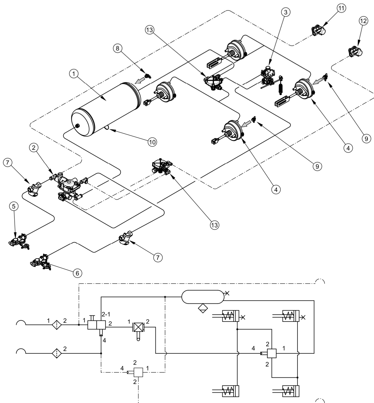
РИСУНОК 3.6 Устройство и схема пневматической двухпроводной тормозной системы с автоматическим регулятором
