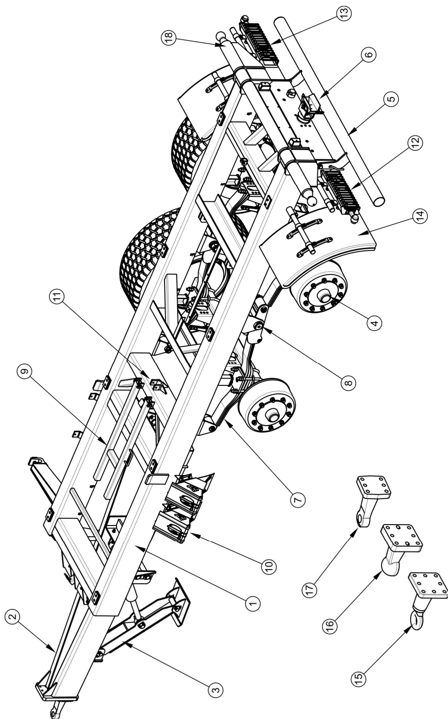
РИСУНОК 3.1 Шасси прицепа
