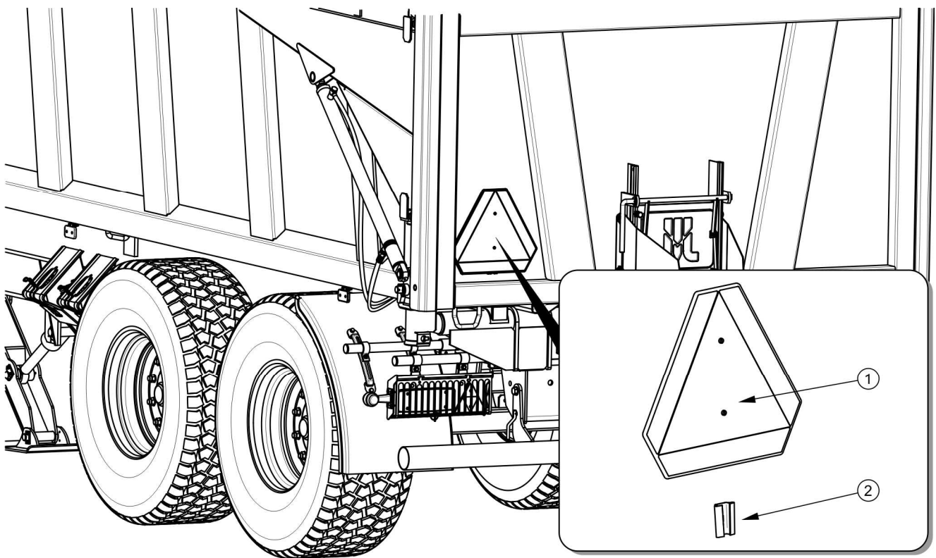
РИСУНОК 2.2 Размещение треугольного знака медленно движущегося транспортного средства.
