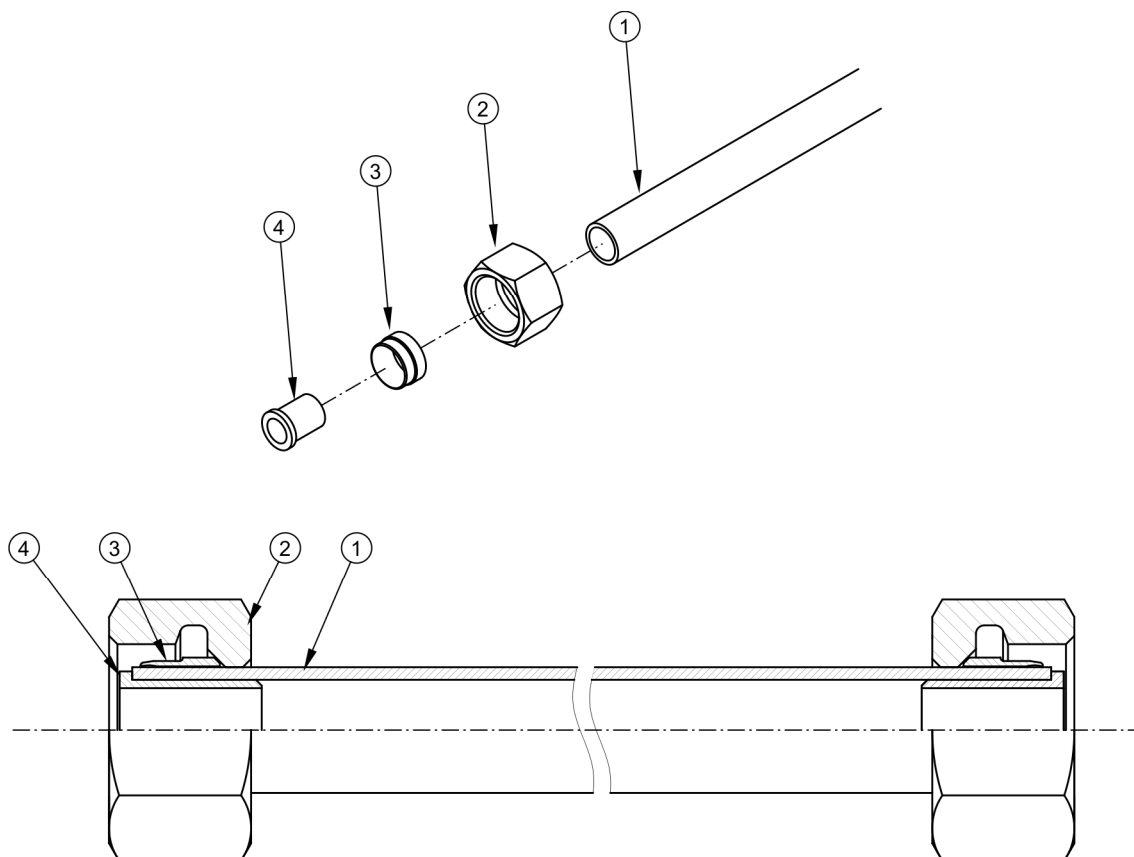
РИСУНОК 5.10 Монтаж пневмопровода
