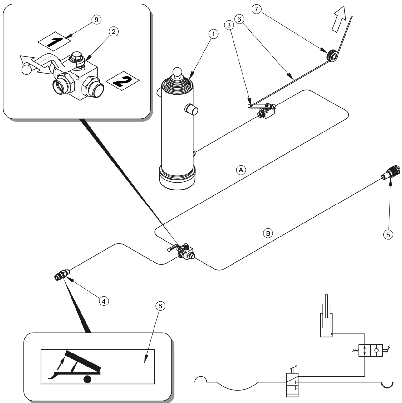
РИСУНОК 3.9 Устройство и схема гидравлической системы опрокидывания
