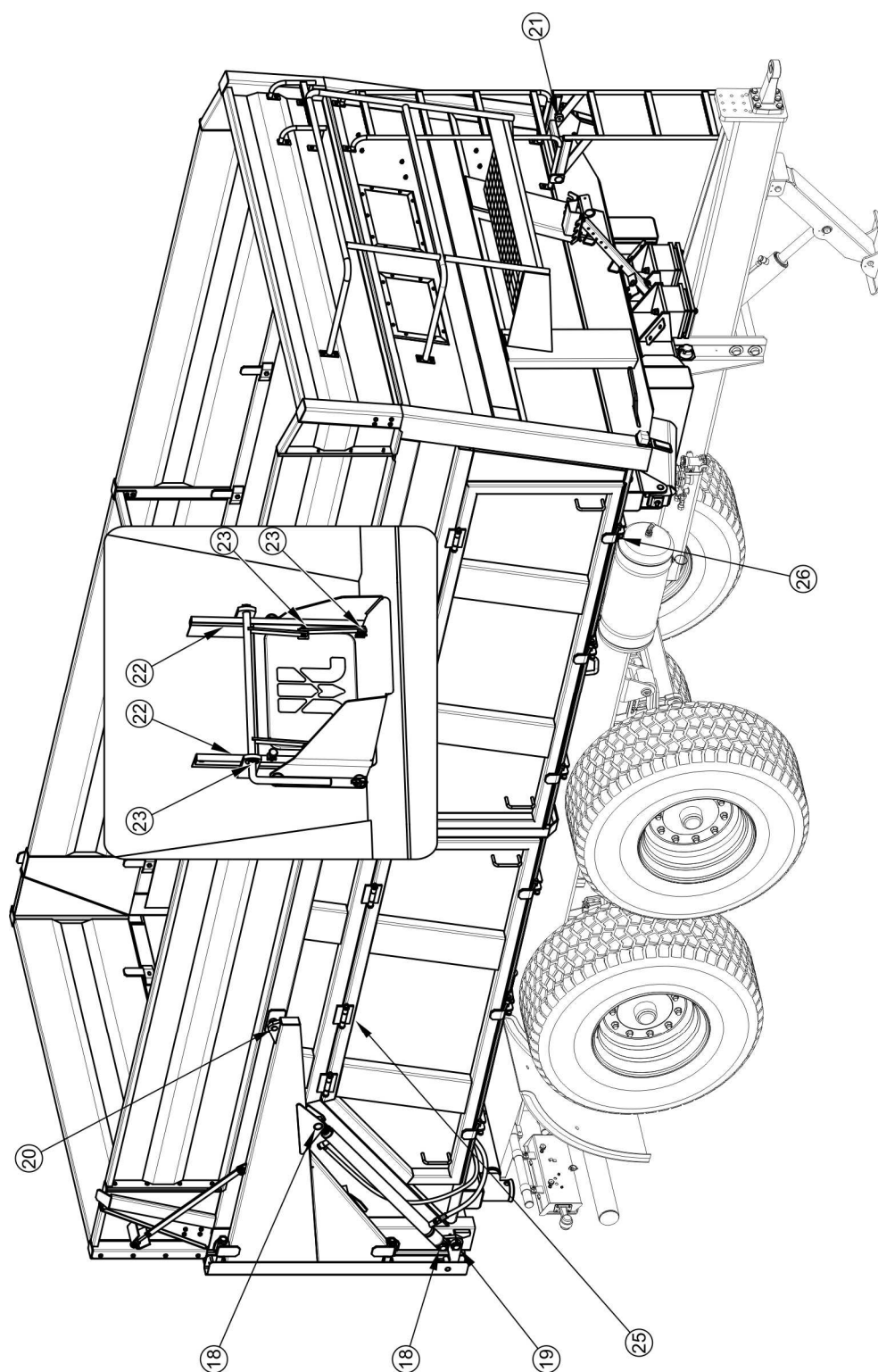
РИСУНОК 5.12 Точки смазки прицепа, часть 2
