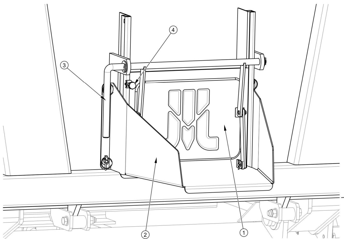
РИСУНОК 4.4 Разгрузочный люк
