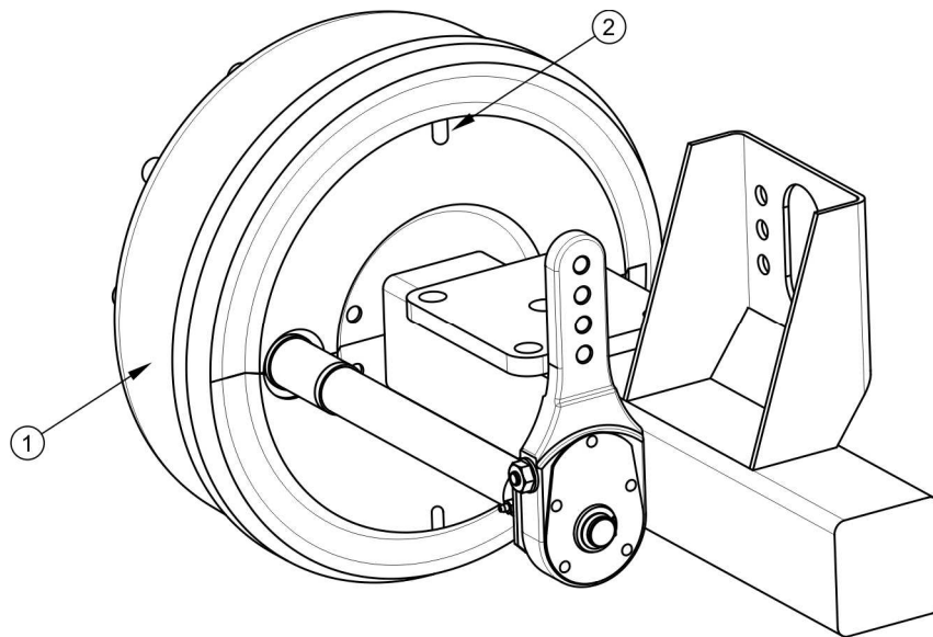
РИСУНОК 5.1 Проверка тормозных накладок
