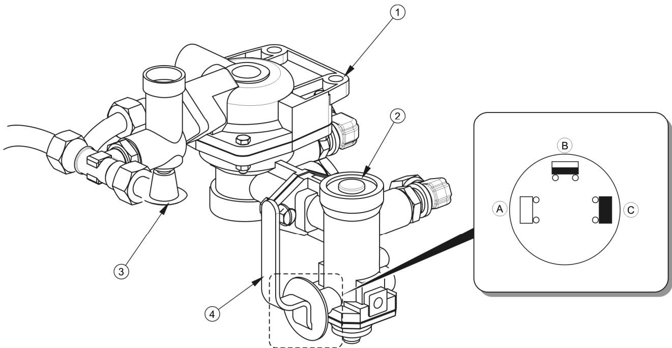
РИСУНОК 3.8 Управляющий клапан и регулятор силы торможения
