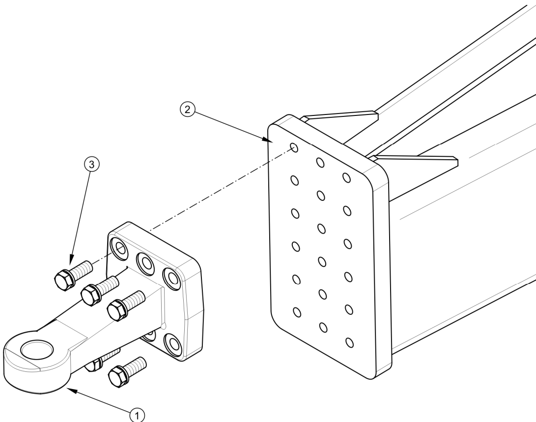
РИСУНОК 5.16 Регулирование положения дышла
