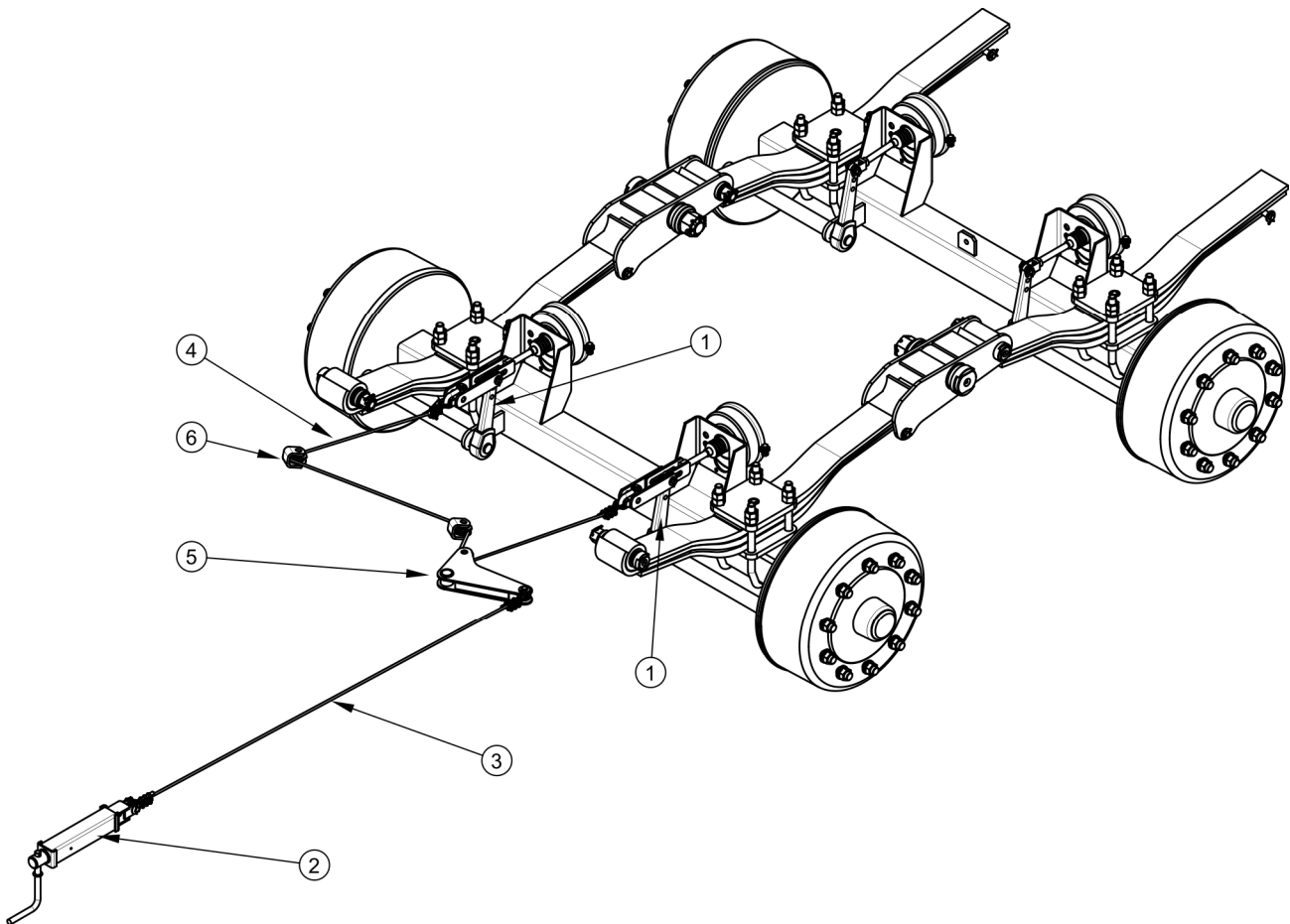
РИСУНОК 3.13 Устройство стояночного тормоза
