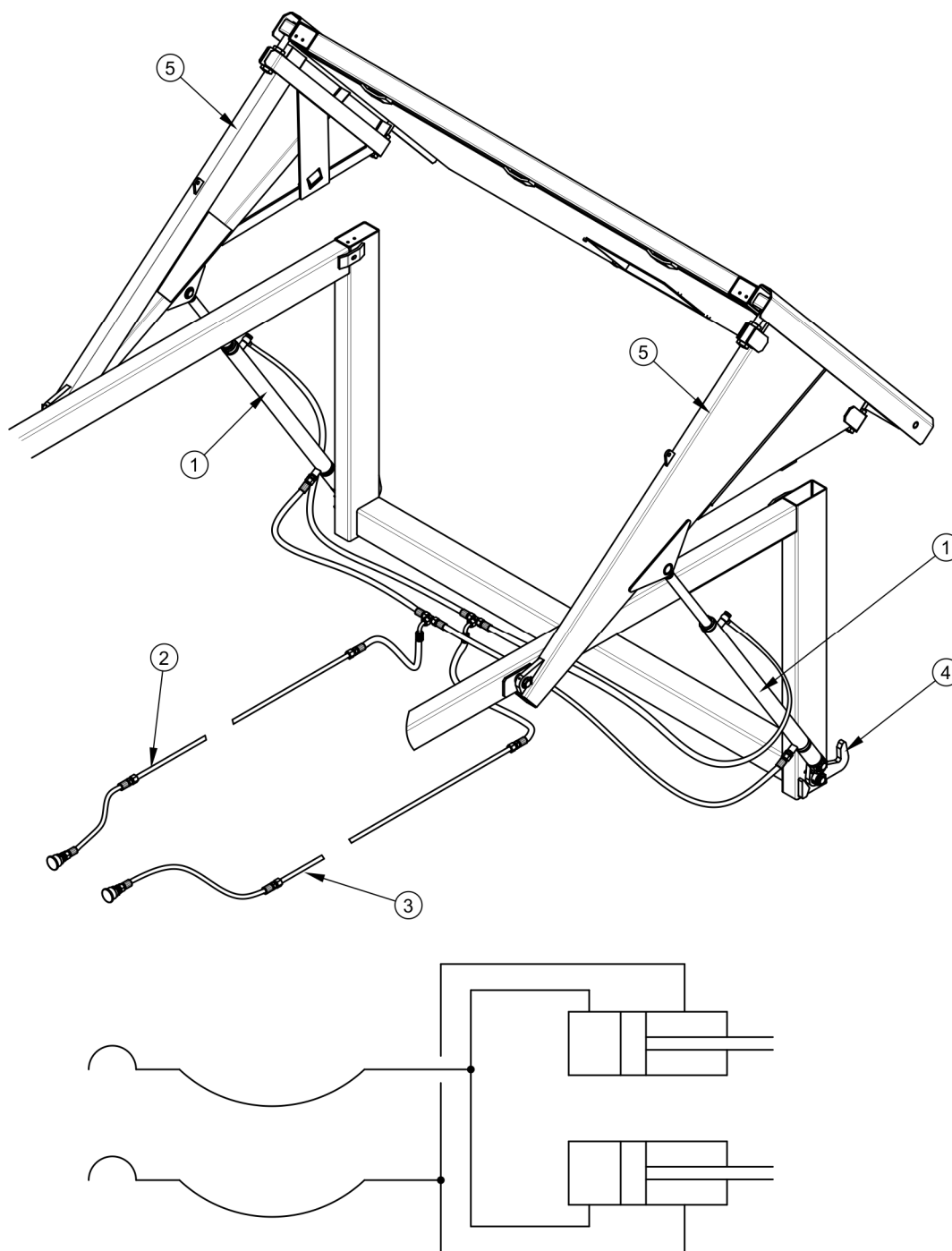
РИСУНОК 3.11 Устройство и схема гидравлической системы заднего борта
