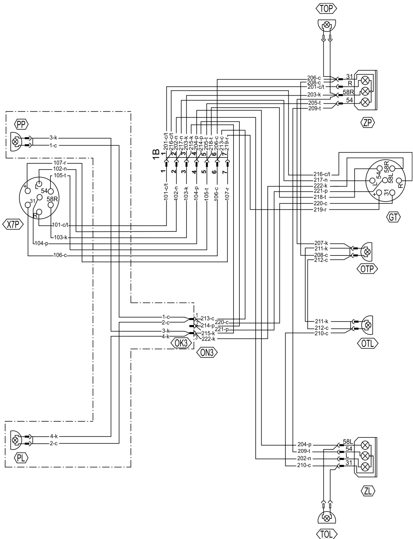
РИСУНОК 3.15 Принципиальная электрическая схема в версии без боковых фонарей
