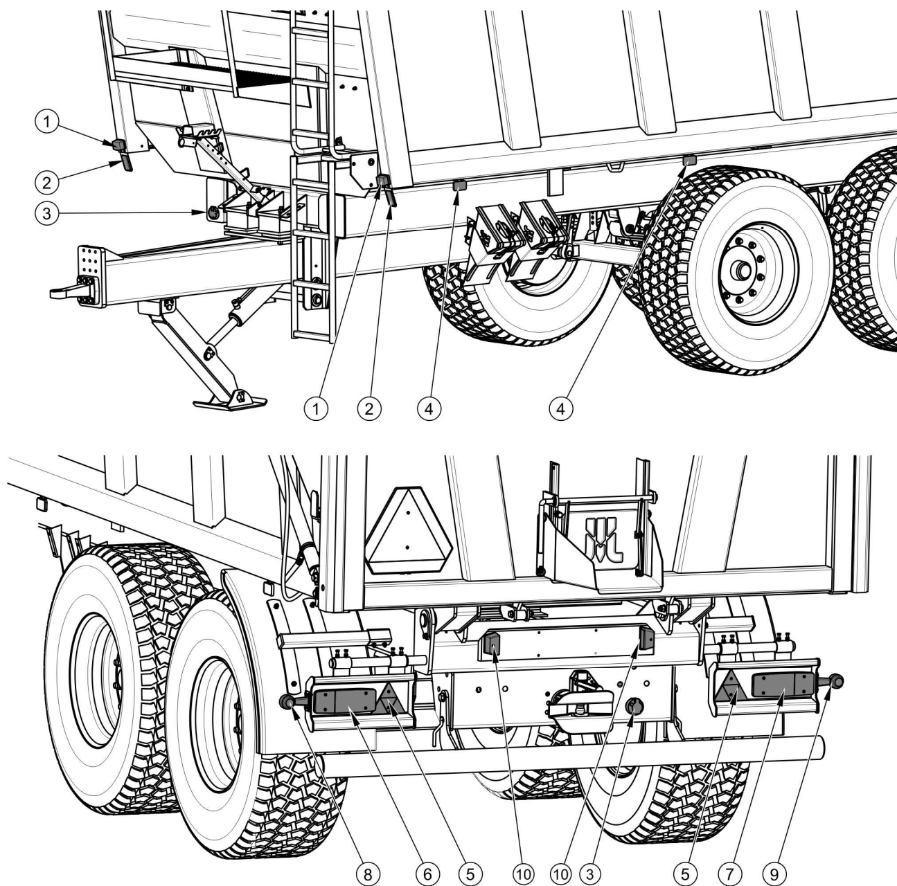
РИСУНОК 3.14 Размещение элементов электрической системы и светоотражающей сигнализации
