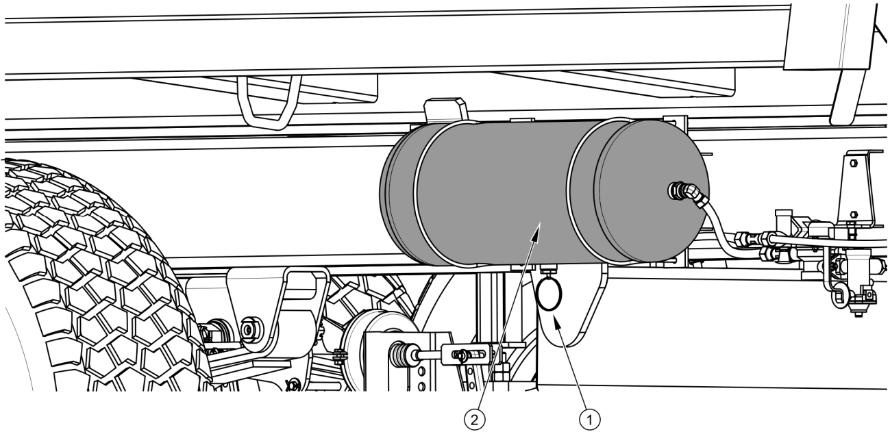
РИСУНОК 5.9 Отвод конденсата из емкости для сжатого воздуха
