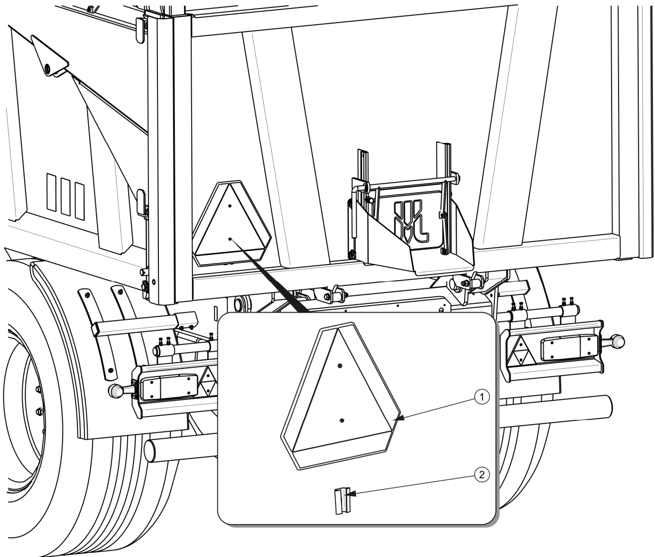
РИСУНОК 2.2 Размещение треугольного знака медленно движущегося транспортного средства.
