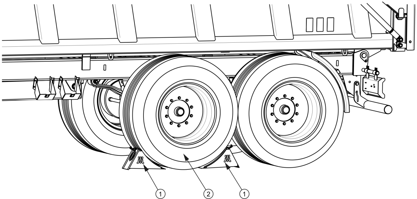
РИСУНОК 2.1 Способ установки клиньев
