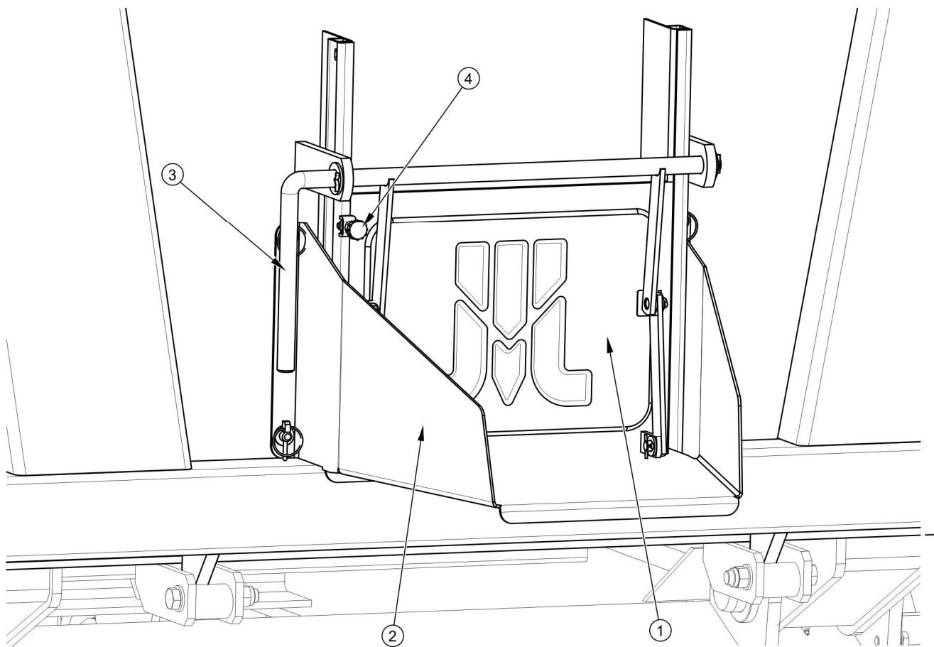
РИСУНОК 4.3 Разгрузочный люк
