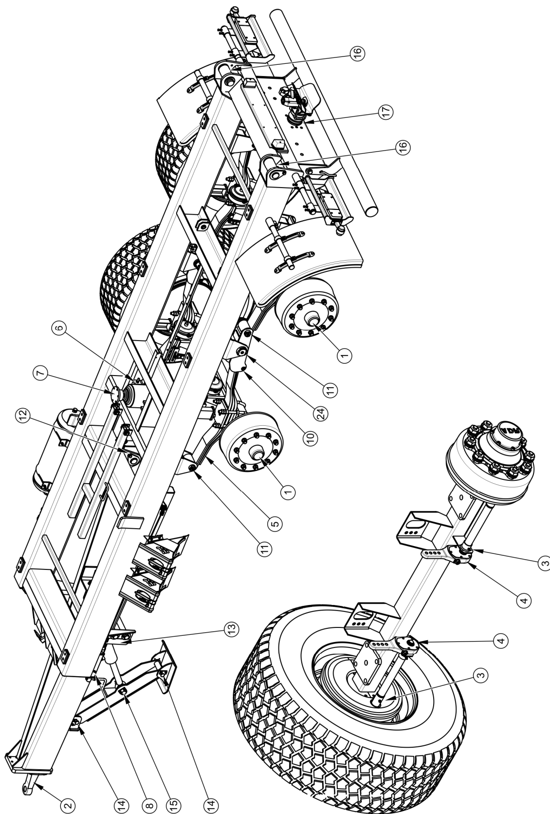
РИСУНОК 5.12 Точки смазки прицепа, часть 2
