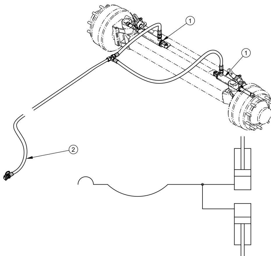
РИСУНОК 3.12 Устройство и схема гидравлического блокирования поворота
