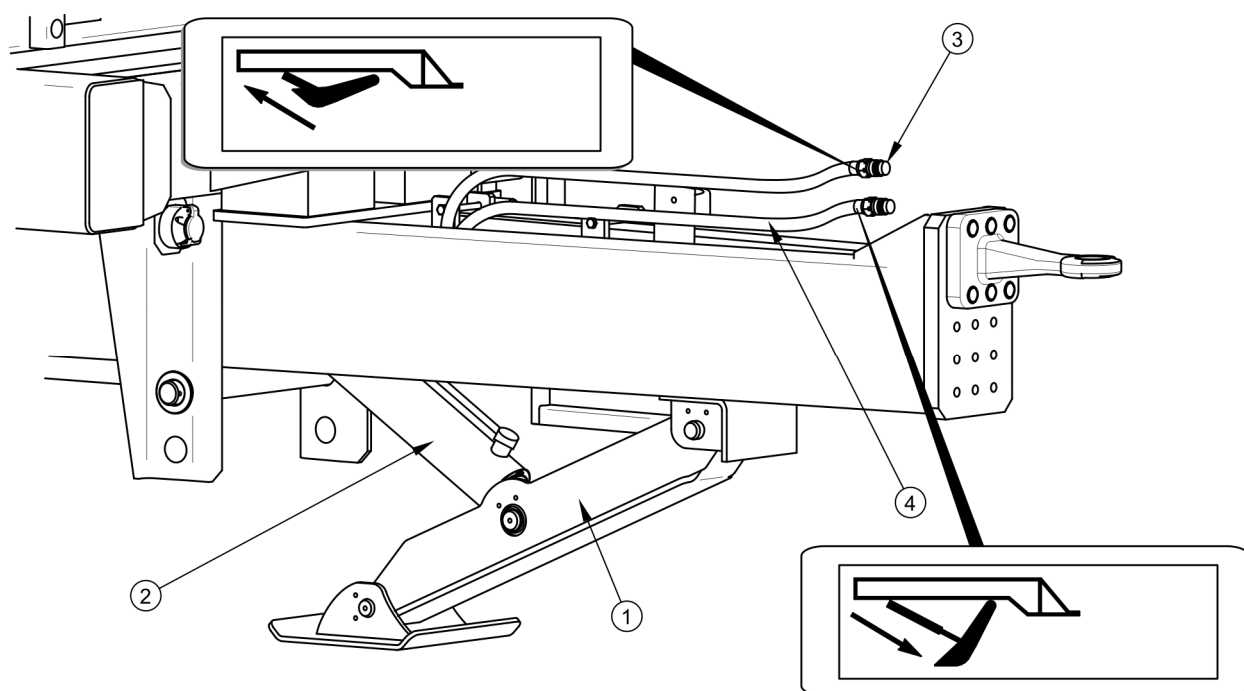
РИСУНОК 4.1 Подсоединение гидравлической ножевой опоры
