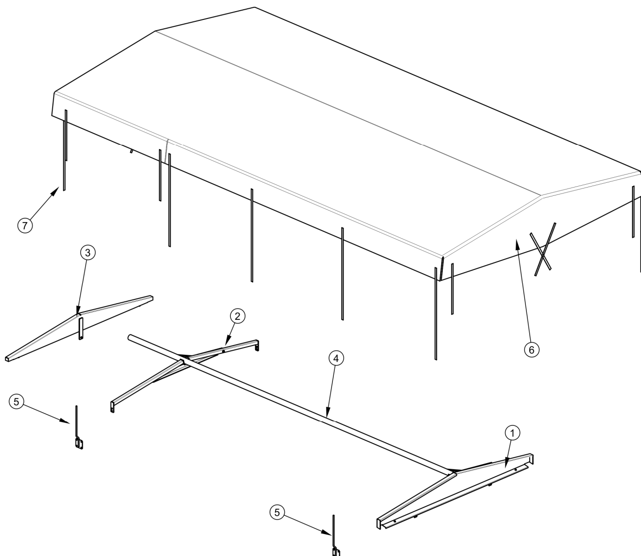
РИСУНОК 5.15 Каркас с тентом
