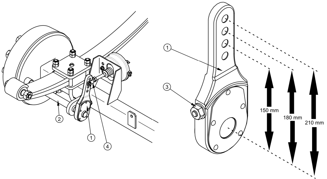
РИСУНОК 5.5 Регулирование механических тормозов ходовых осей
