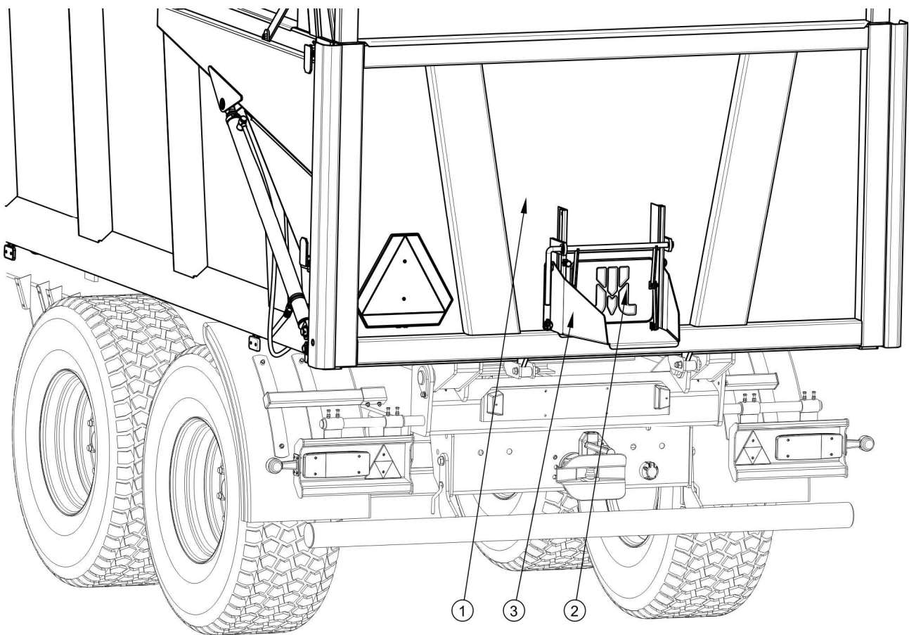
РИСУНОК 3.3 Разгрузочный люк в заднем борту
