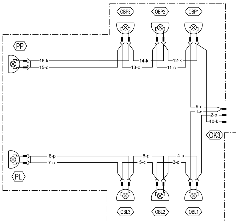
РИСУНОК 3.16 Принципиальная электрическая схема пучка боковых фонарей
