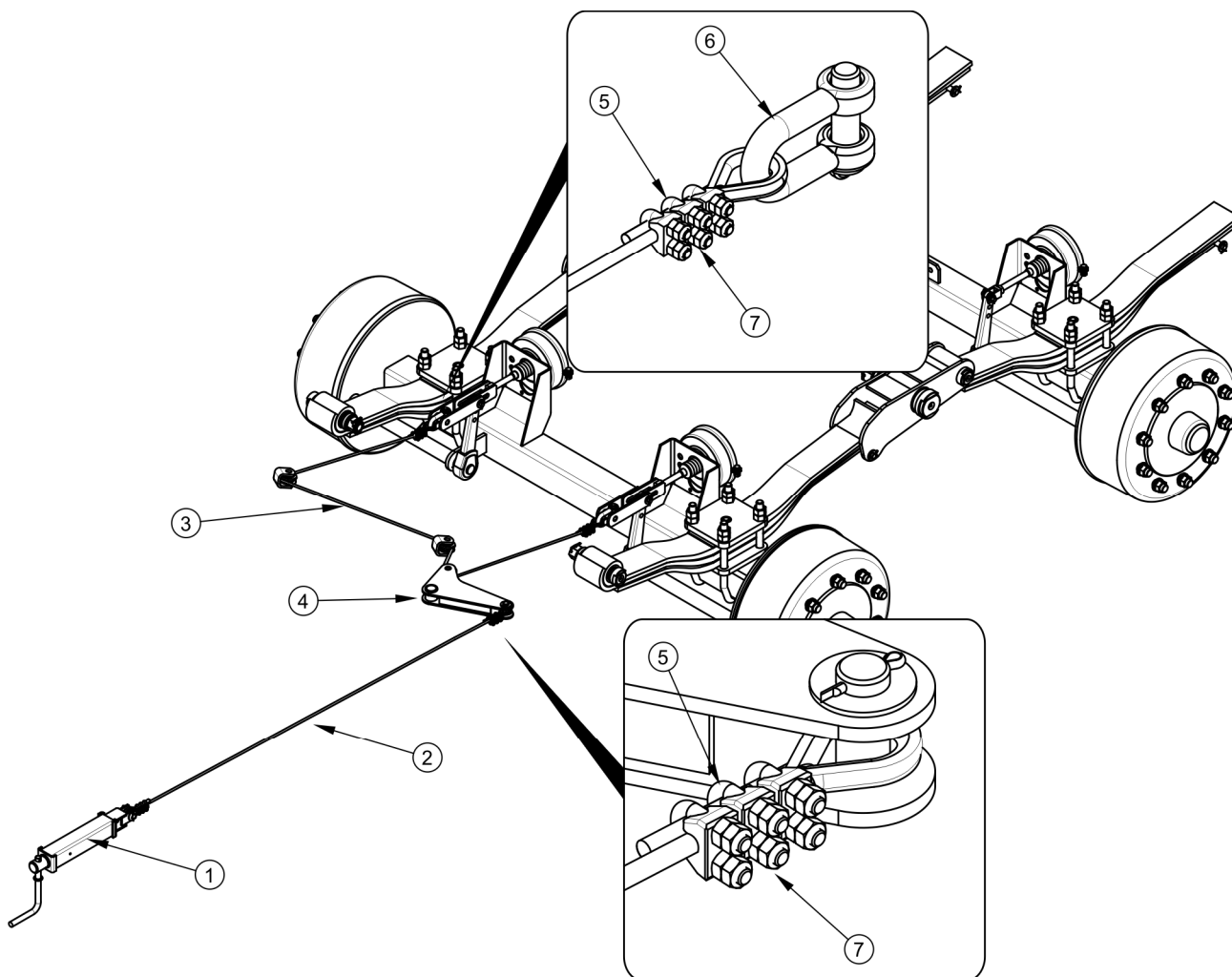
РИСУНОК 5.6 Регулирование натяжения троса стояночного тормоза
