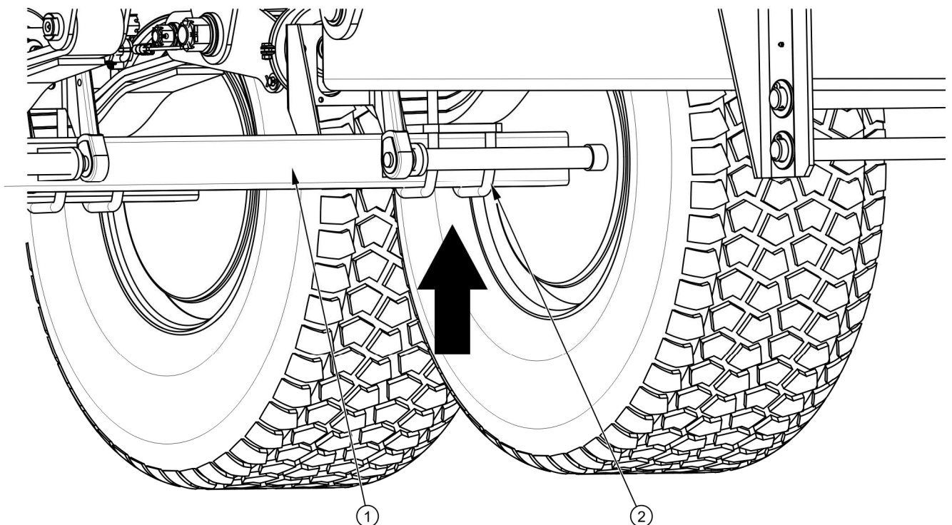
РИСУНОК 5.2 Точка поддомкрачивания
