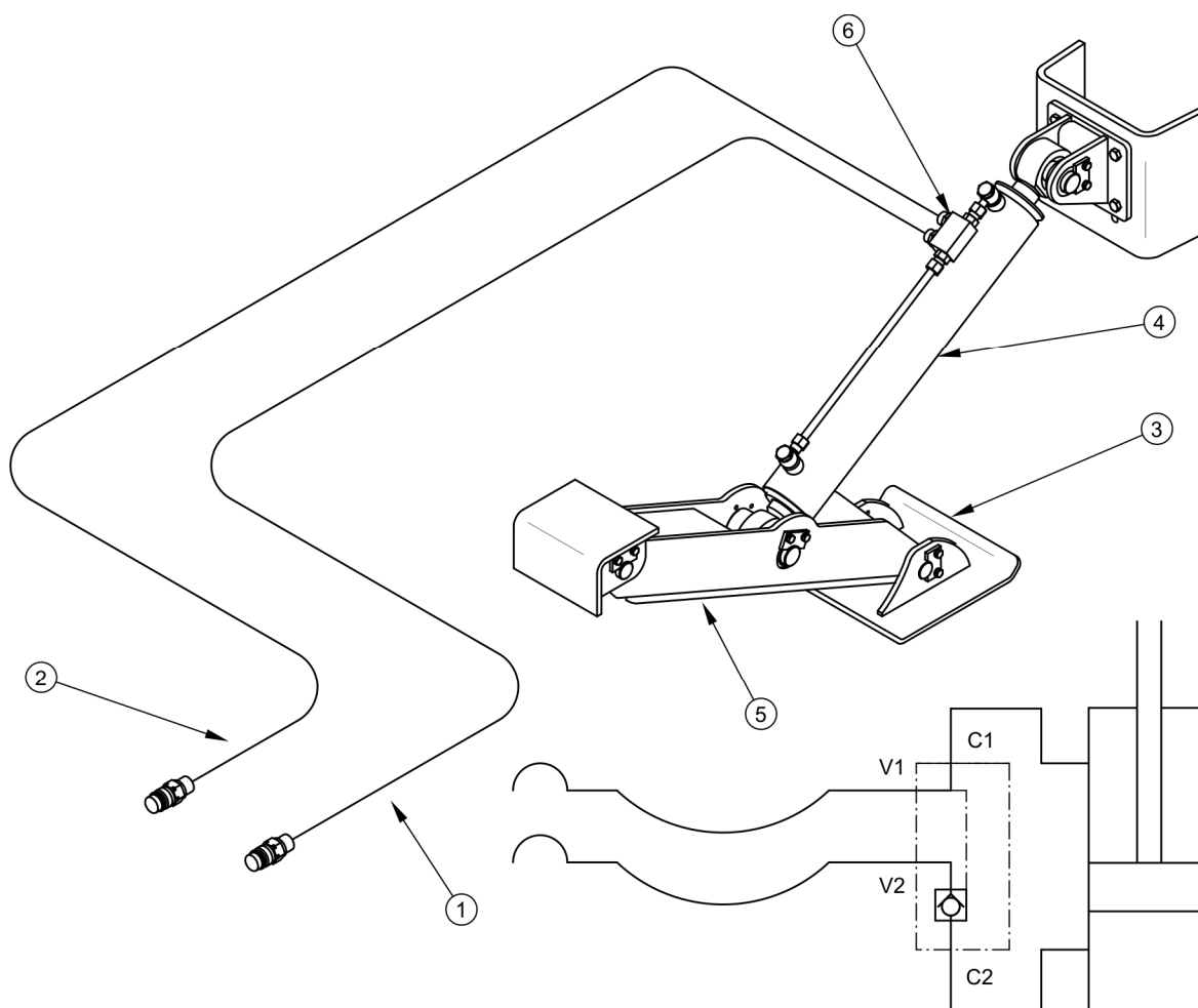
РИСУНОК 3.10 Устройство и схема гидравлической системы ножевой опоры
