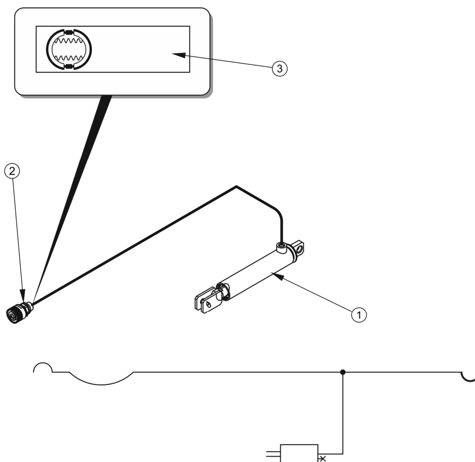
Obrázek 3.8 Konstrukce a schéma hydraulické brzdové instalace
