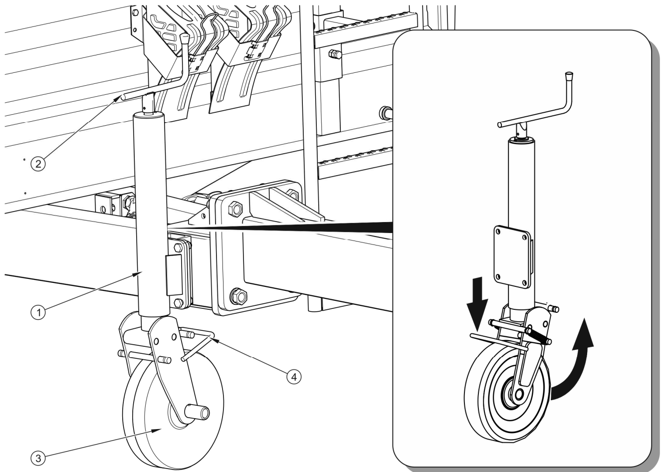
RYSUNEK 4.1 Podpěra přívěsu
