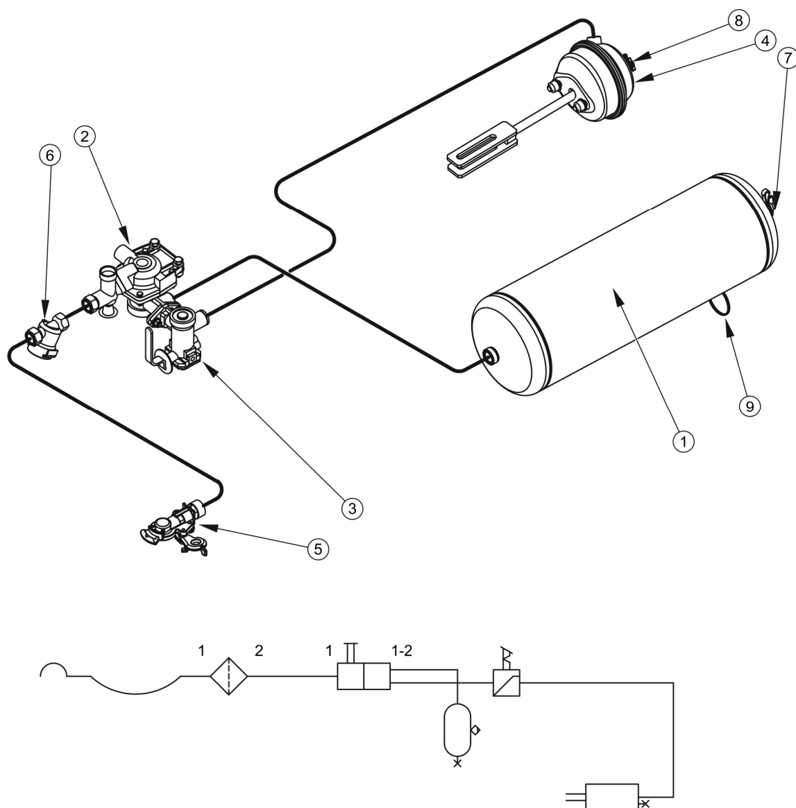
Obrázek 3.7 Konstrukce a schéma vzduchové jednohadicové brzdové instalace
