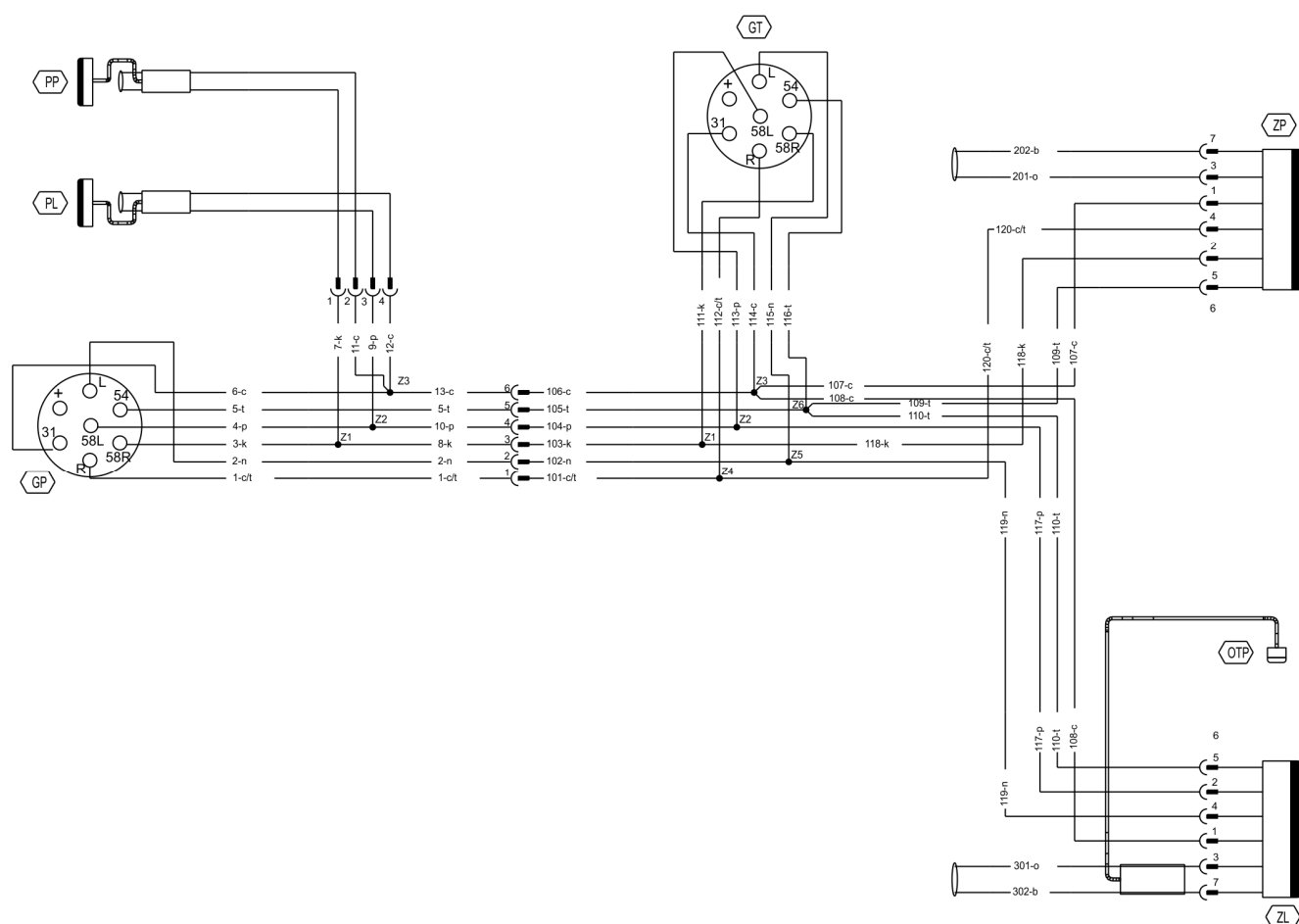
Obrázek 3.13 Ideové schéma elektroinstalace
