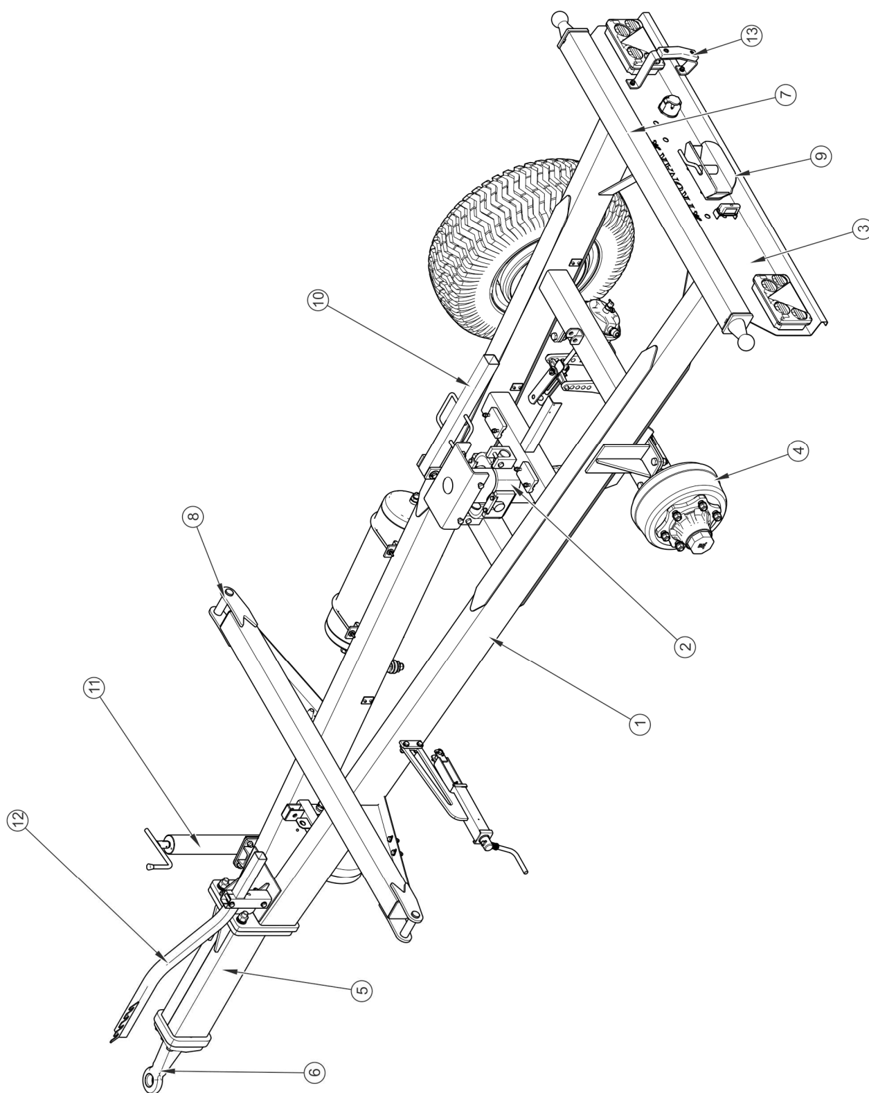
Obrázek 3.1 Podvozek přívěsu
