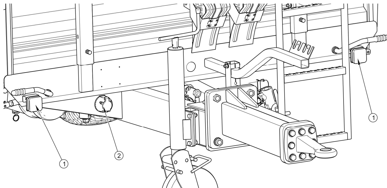
Obrázek 3.15 Rozmístění prvků světelné instalace – pohled zepředu
