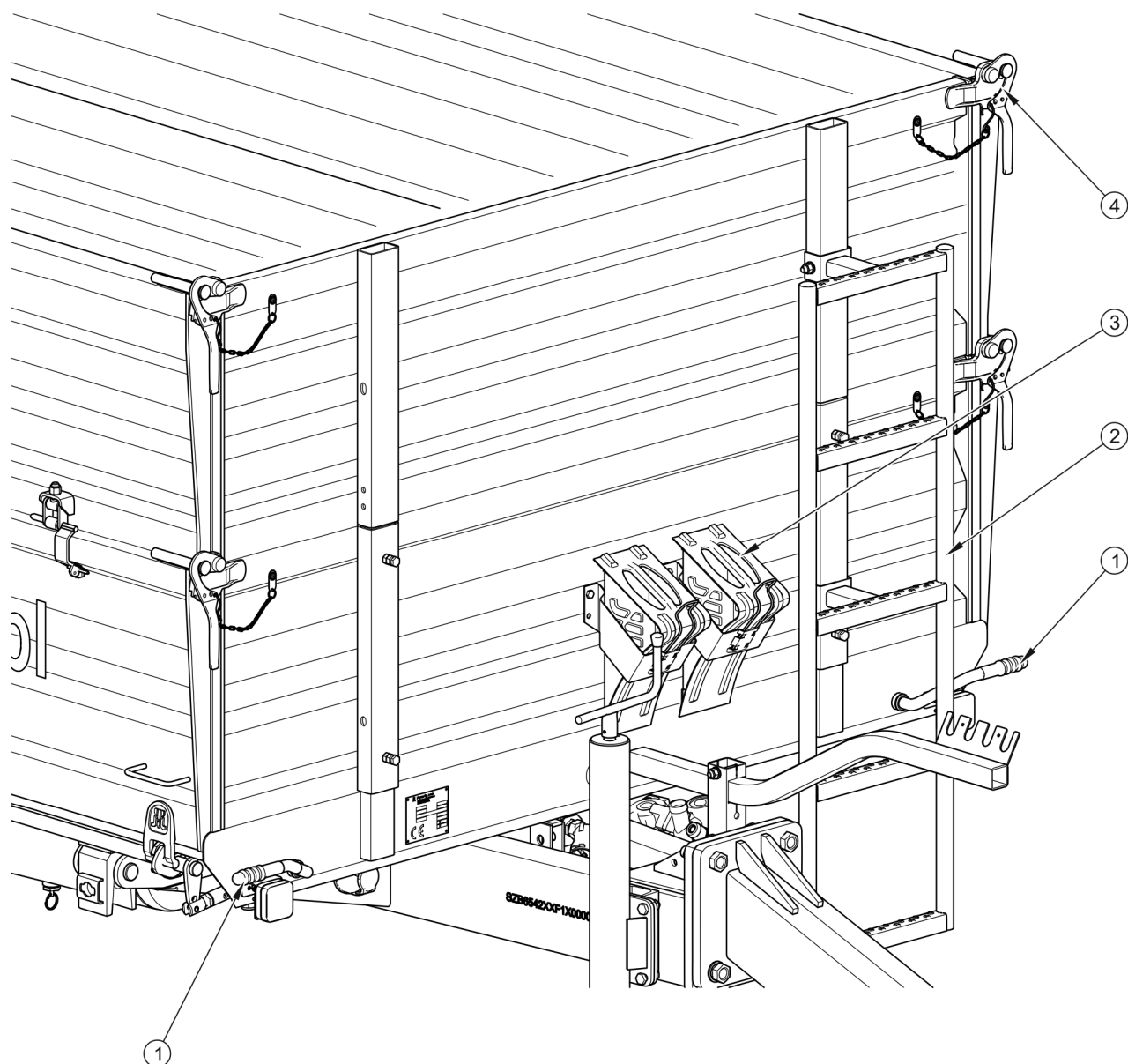
Obrázek 3.4 Korba
