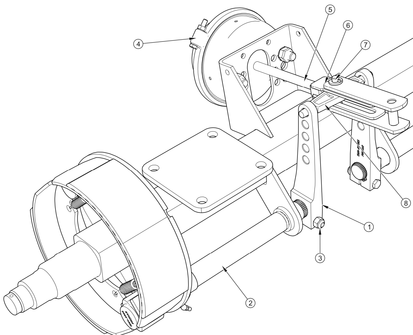
Obrázek 5.5 Konstrukce brzdy pojezdové nápravy
