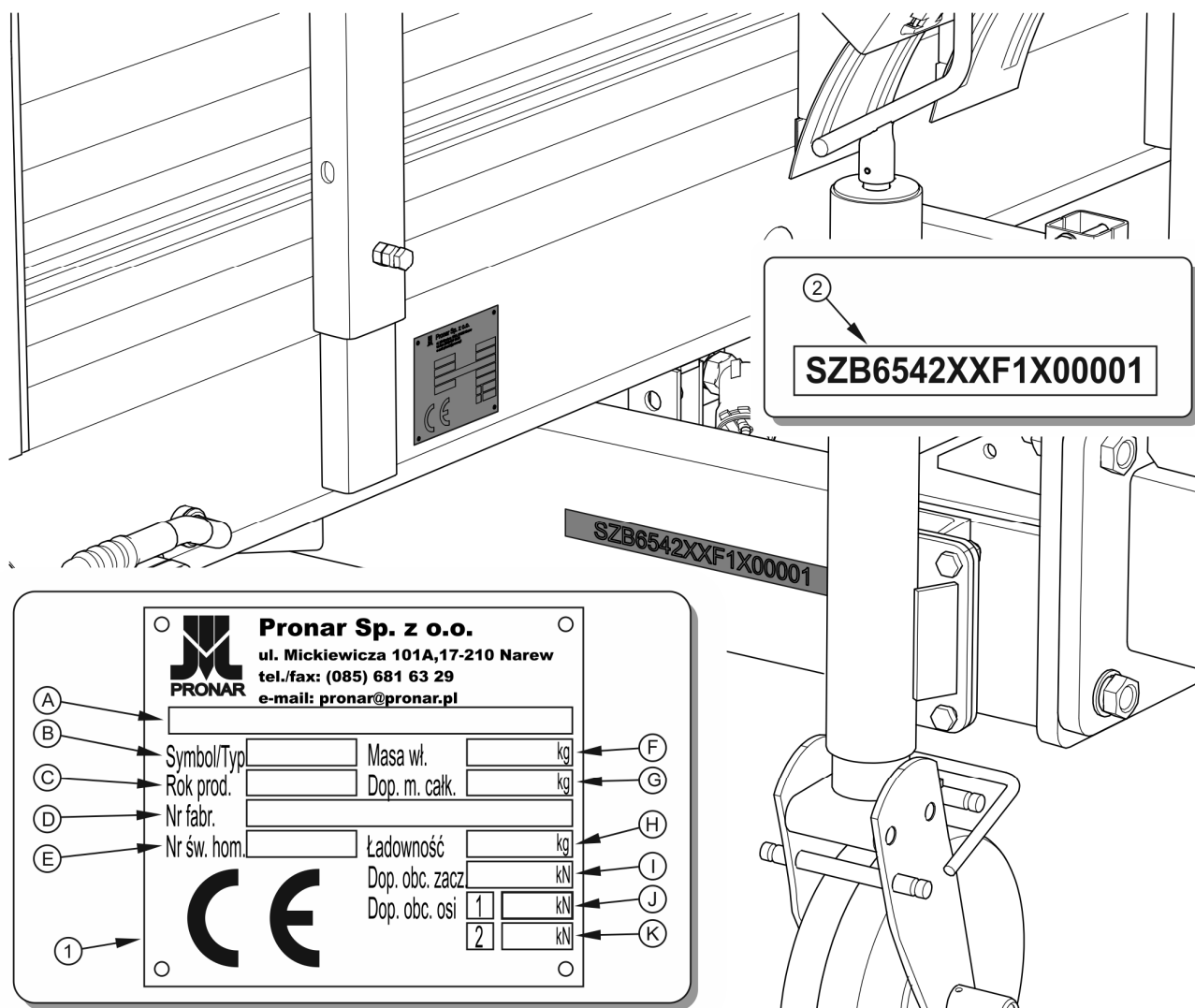
Obrázek 1.1 Místa umístění údajového štítku a vyražení výrobního čísla
