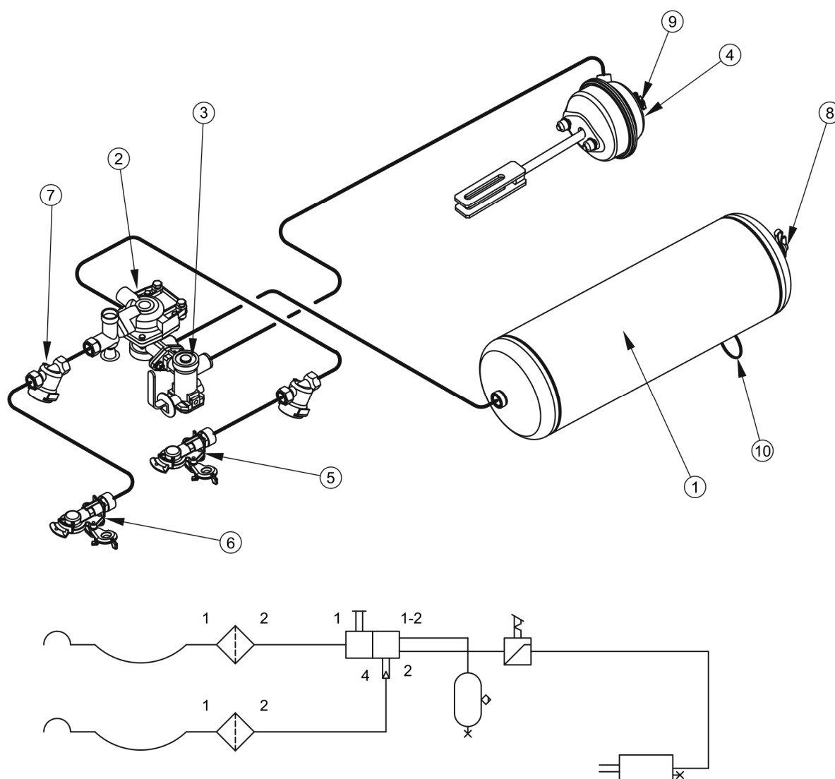
Obrázek 3.6 Konstrukce a schéma vzduchové brzdové dvouhadicové instalace
