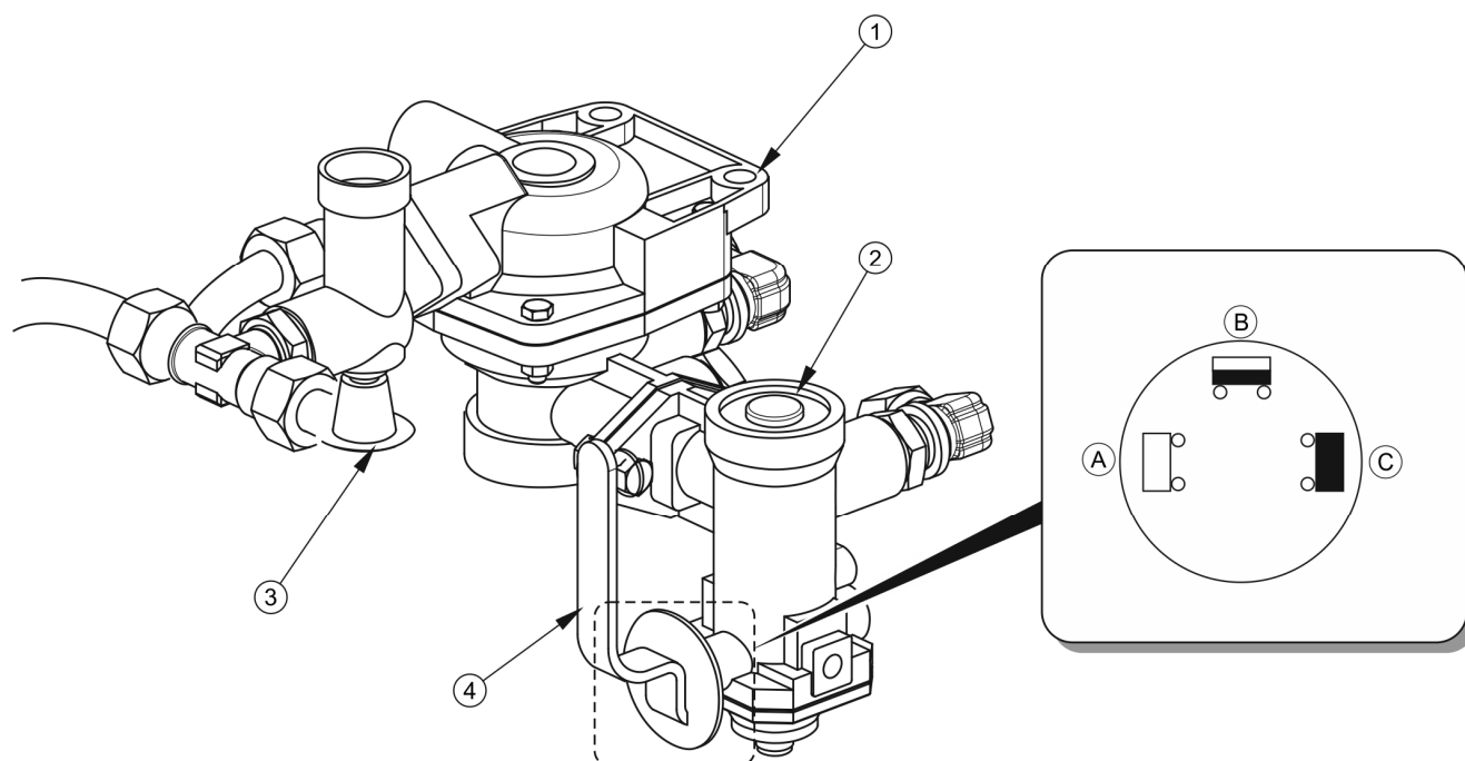
Obrázek 3.10 Ovládací ventil a regulátor brzdné síly
