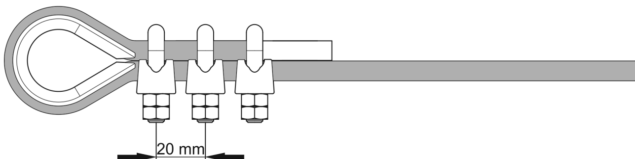
Obrázek 5.9 Montáž svorek brzdového lanka
