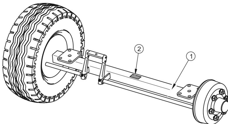
Obrázek 1.2 Místo umístění údajového štítku nápravy
