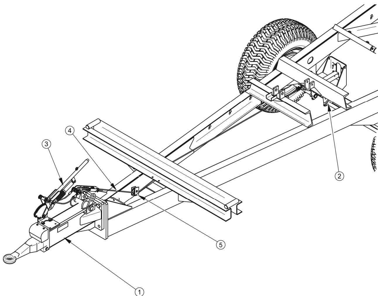
Obrázek 3.9 Nájezdová brzda
