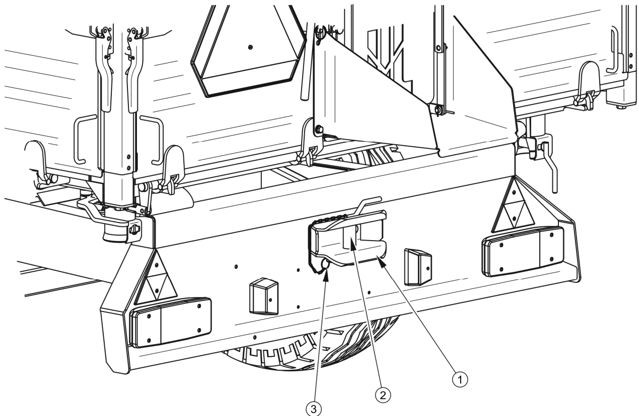
RYSUNEK 4.2 Zadní závěs
