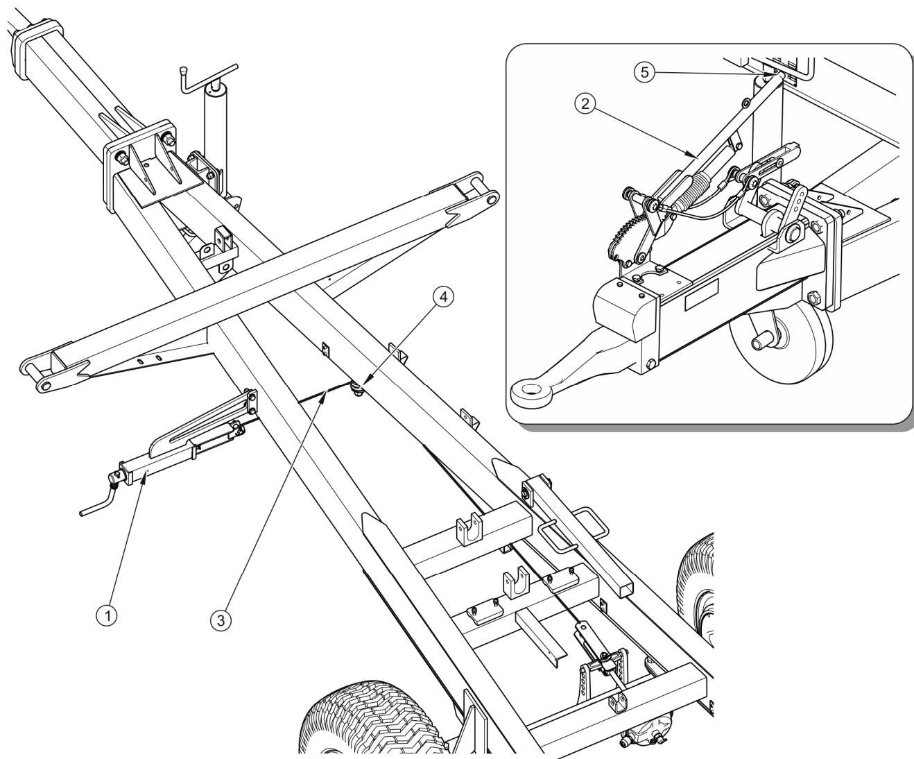
Obrázek 3.12 Konstrukce parkovací brzdy
