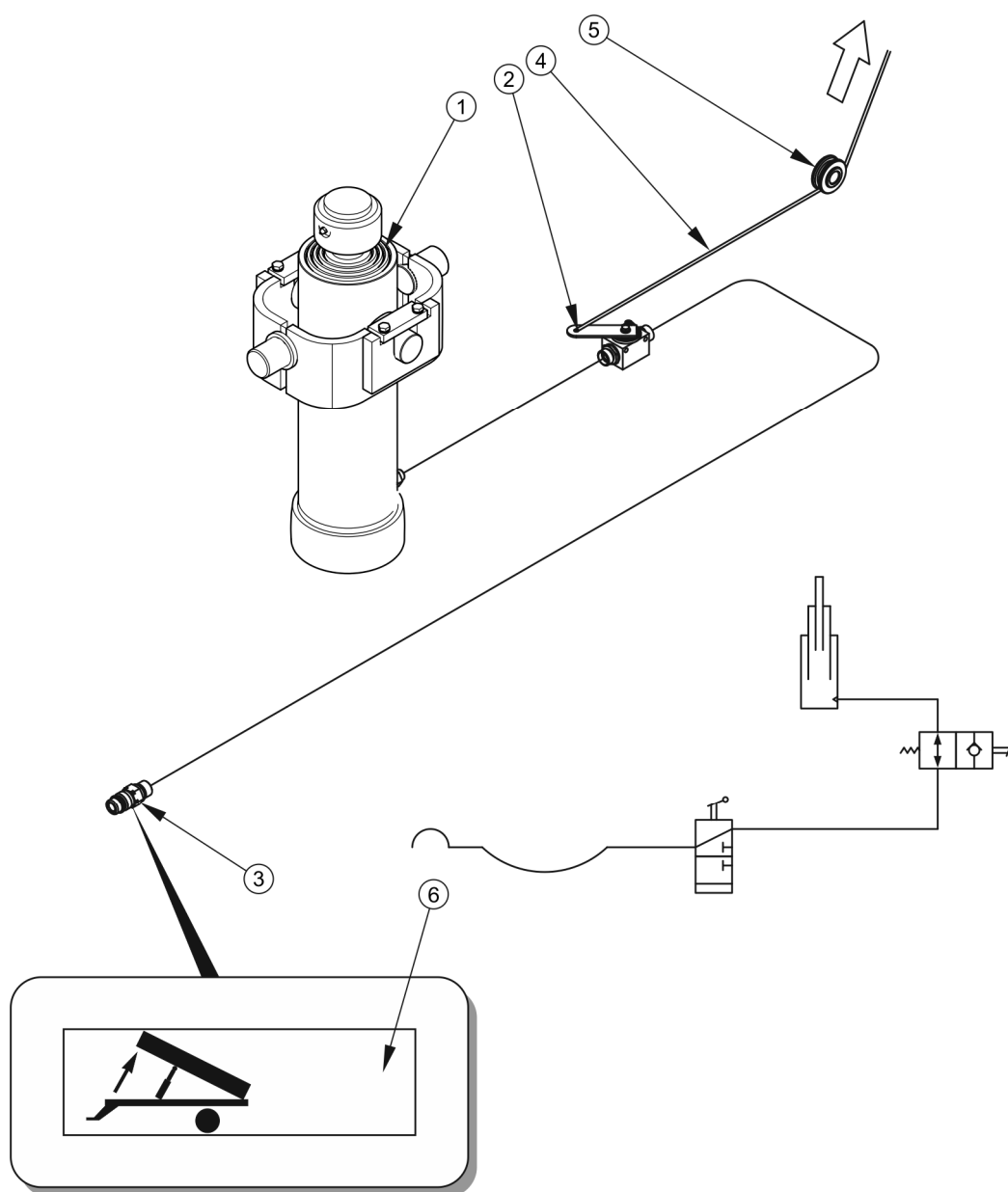
Obrázek 3.11 Konstrukce a schéma hydraulické instalace sklápění
