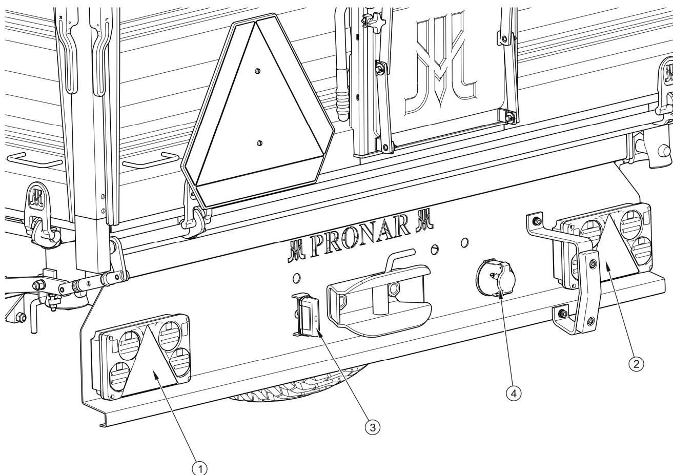
Obrázek 3.14 Rozmístění prvků světelné instalace – pohled zezadu
