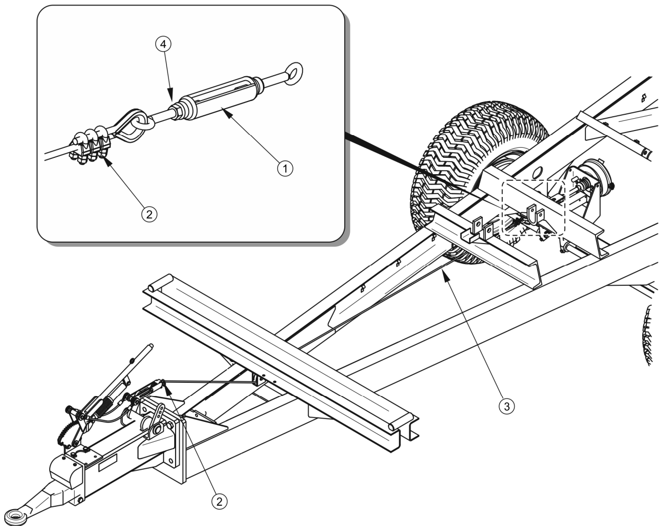
Obrázek 5.7 Seřízení napnutí lanka nájezdové brzdy
