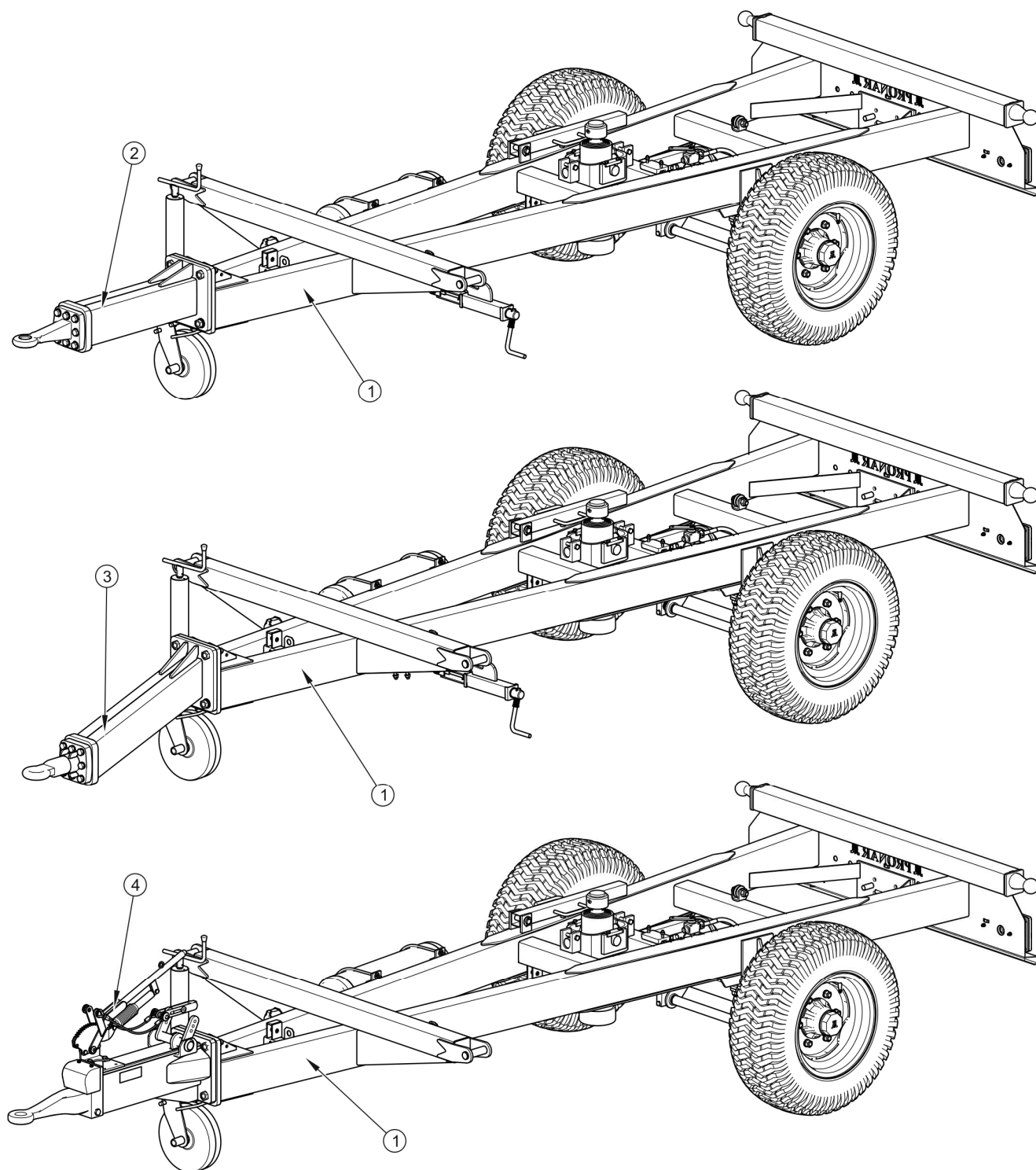
Obrázek 3.2 Podvozek přívěsu
