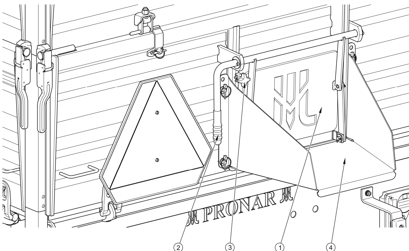
Obrázek 3.5 Dvířka zadní bočnice s blokádou a výsypkou.
