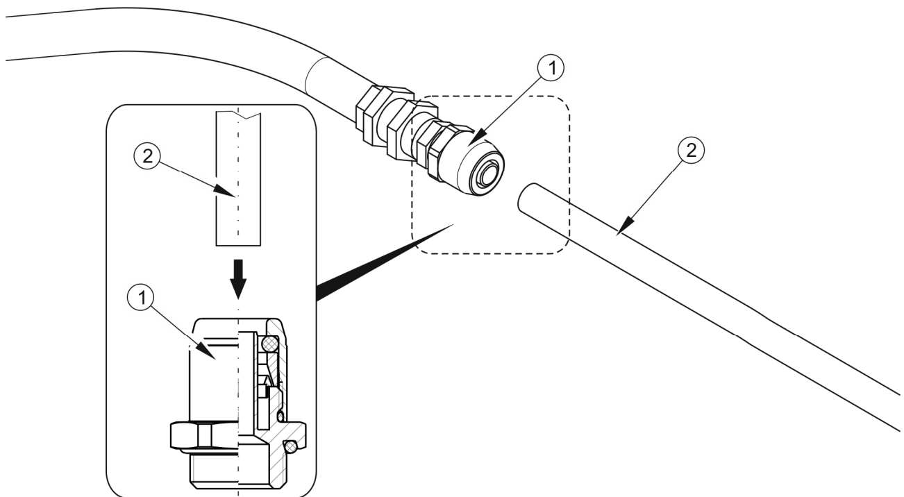
Obrázek 5.12 Montáž vzduchové hadice
