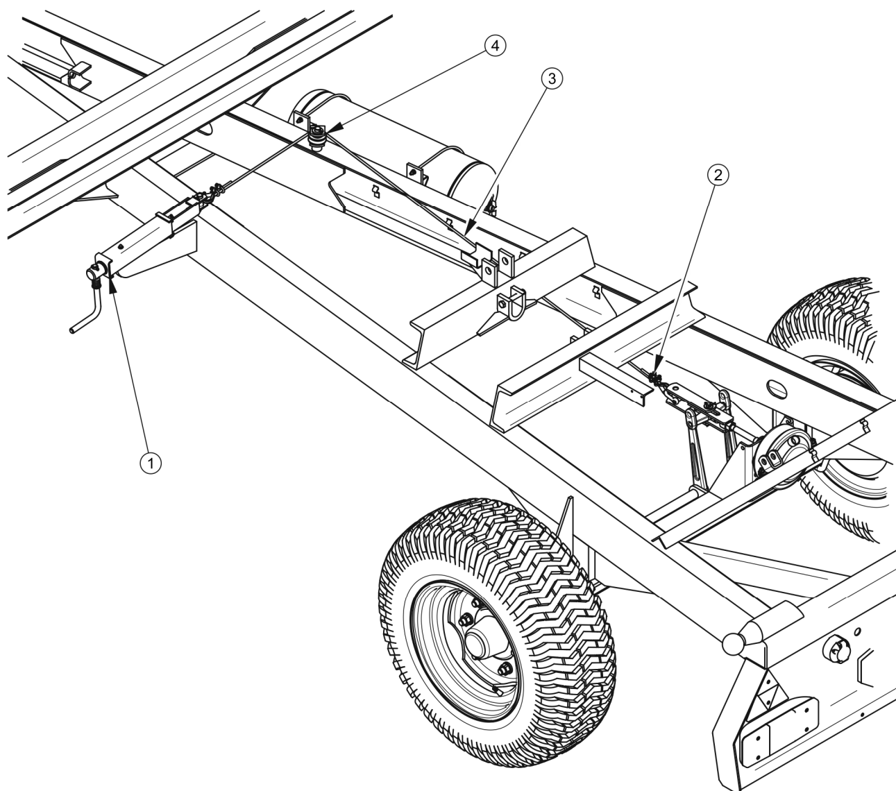
Obrázek 5.8 Regulace základní brzdy
