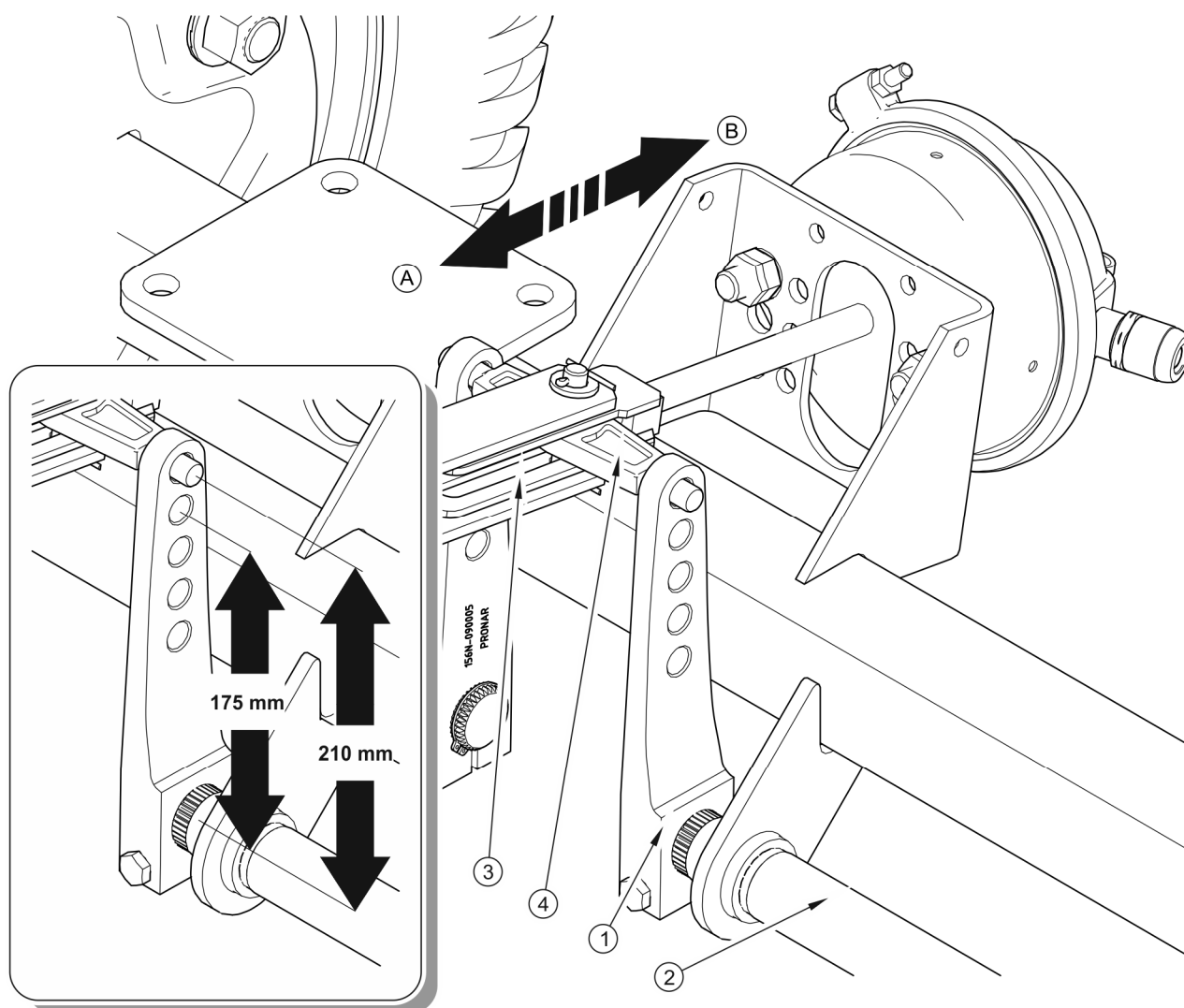
Obrázek 5.6 Zásady úpravy brzd
