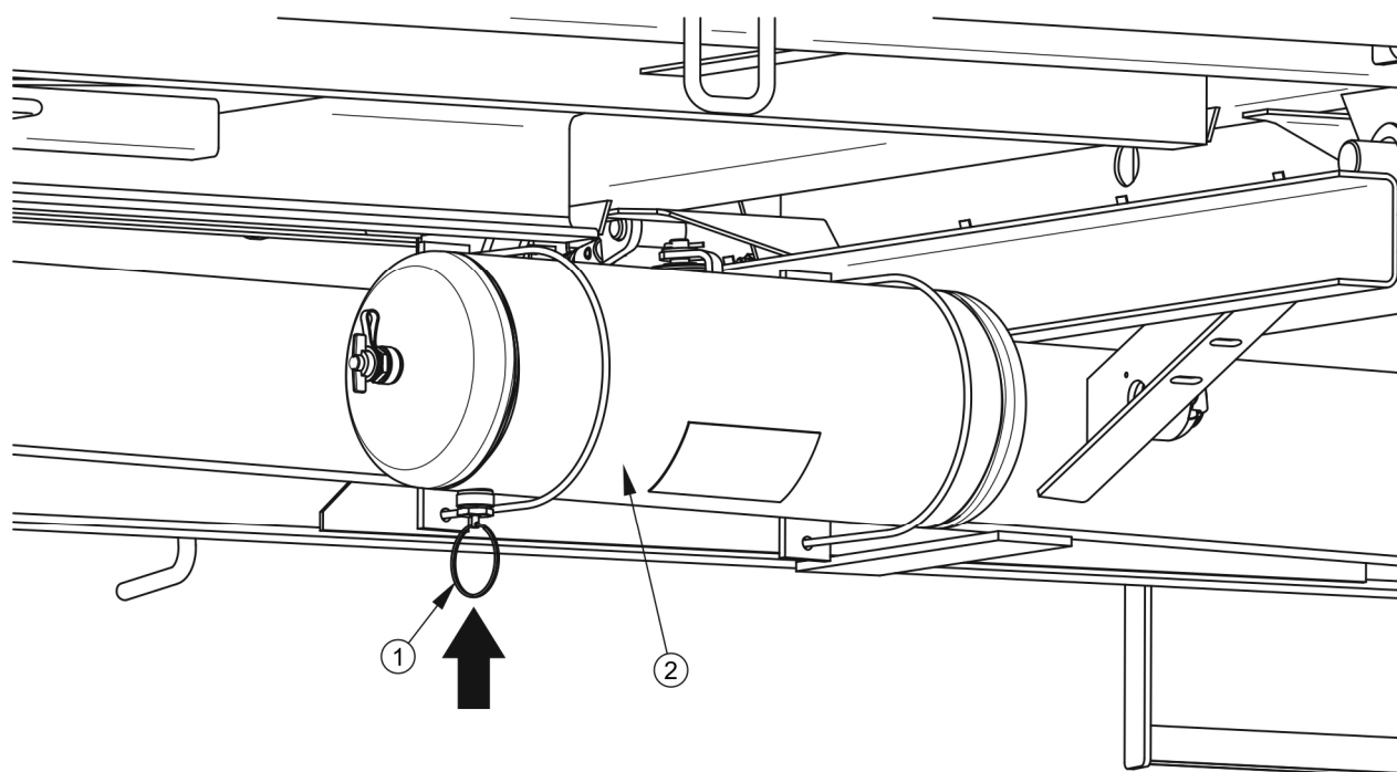
Obrázek 5.11 Odvodňování vzdušníku
