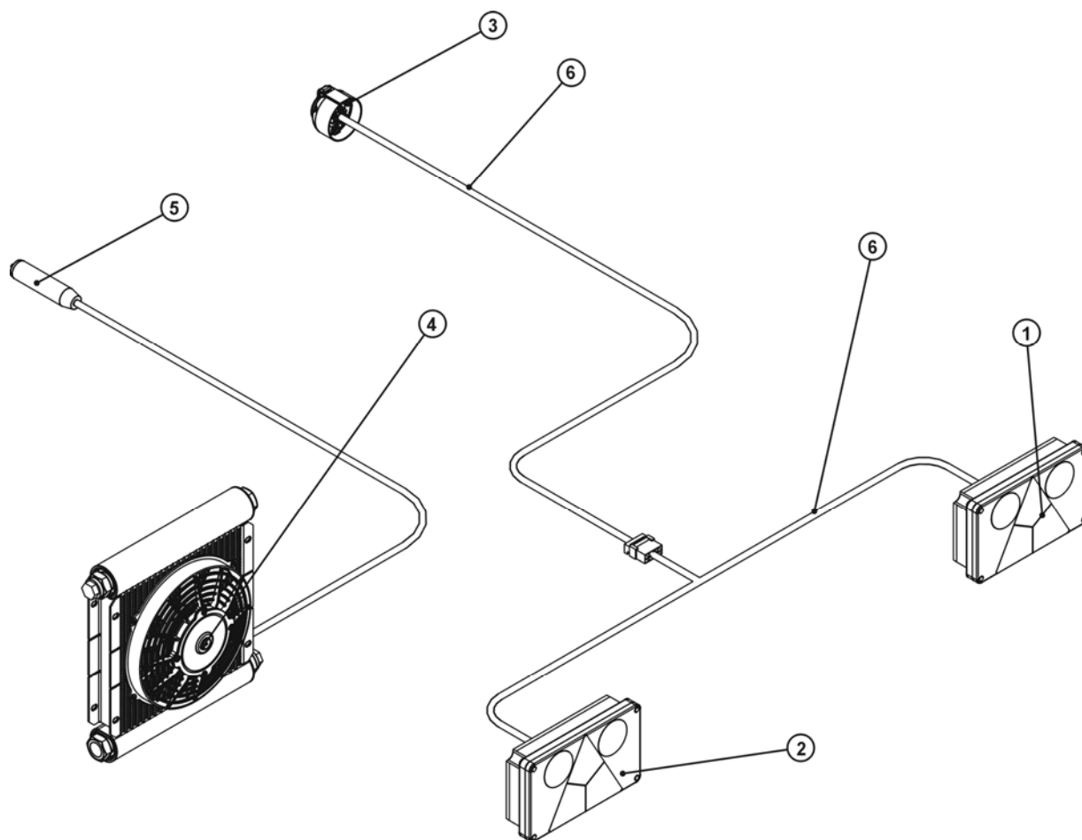
RYСУNEK 14. SCHEMAT INSTALACJI ELEKTRYCZNEJ
