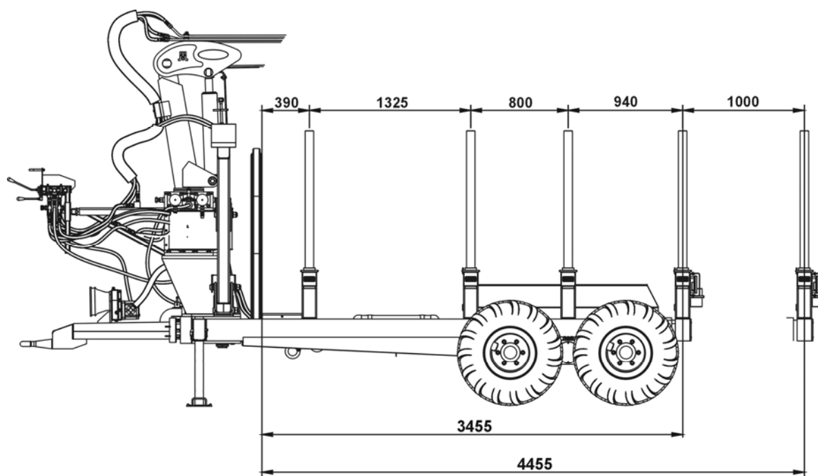
RYSUNEK 17. ROZSTAW KŁONIC
