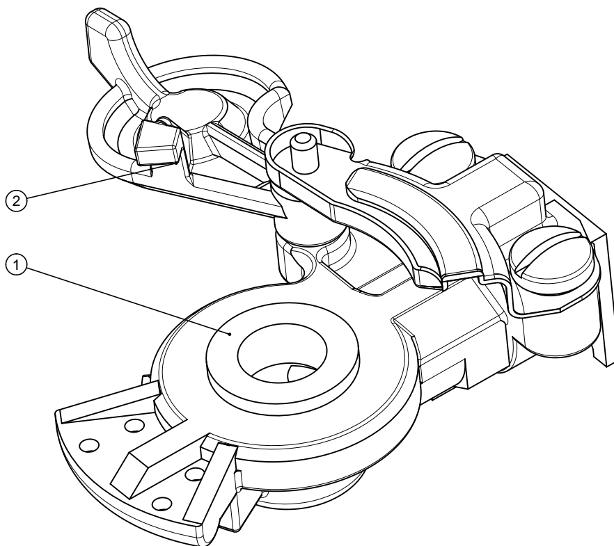
ABBILDUNG 5.5A LEITUNGSANSCHLUSSSTÜCK
