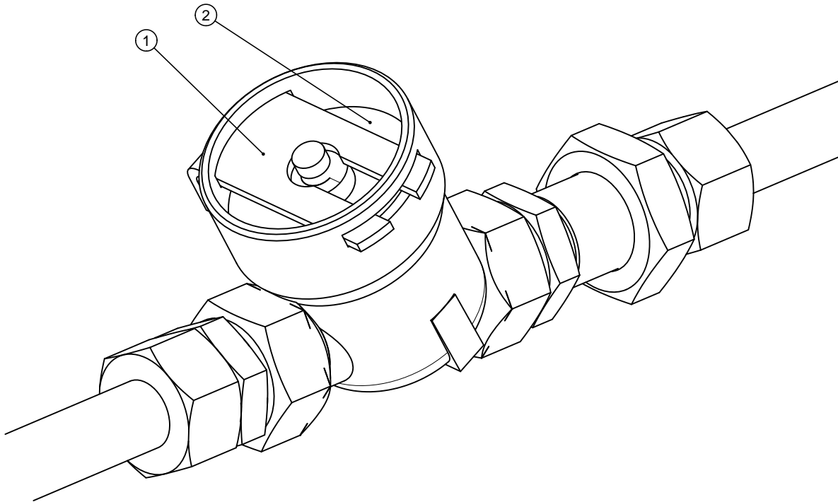
ABBILDUNG 5.4A LUFTFILTER
