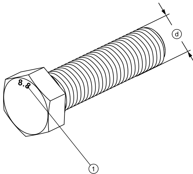
ABBILDUNG 5.10A SCHRAUBE MIT METRISCHEM GEWINDE
