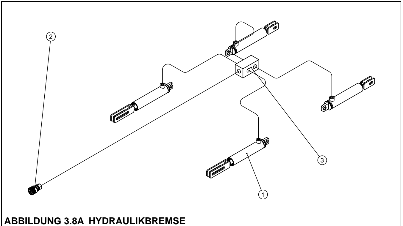
(1) hydraulischer Servomotor der Bremse, (2) Schnellkupplung, (3) Verteilerwürfel
