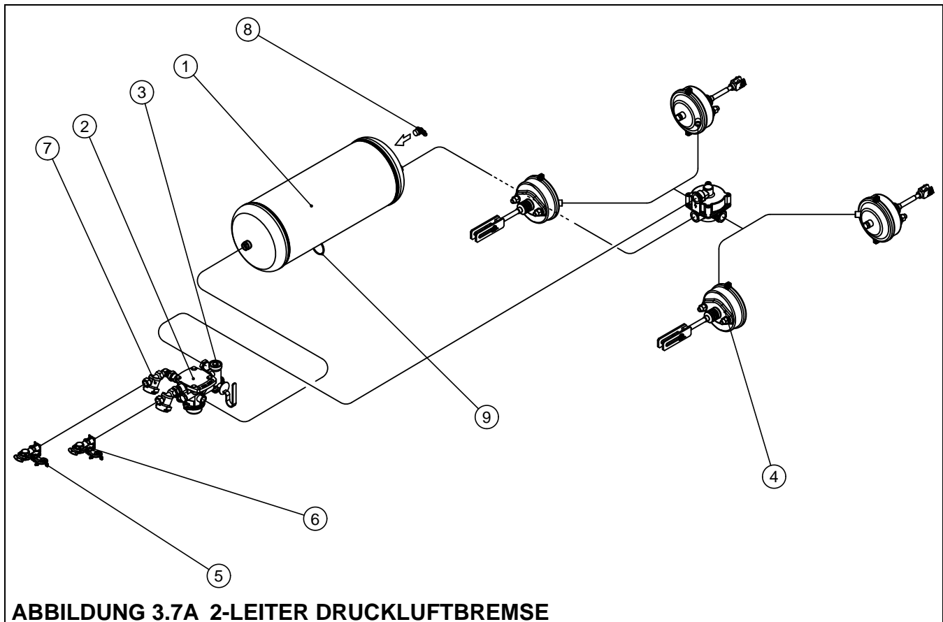
ABBILDUNG 3.7A 2-LEITER DRUCKLUFTBREMSE (1) Druckluftbehälter, (2) Steuerungsventil, (3) Bremskraftregler, (4) pneumatischer Servomotor, (5), (6) Leitungsanschlussstück, (7) Luftfilter, (8) Kontrollanschluss des Druckluftbehälters, (9) Entwässerungsventil
