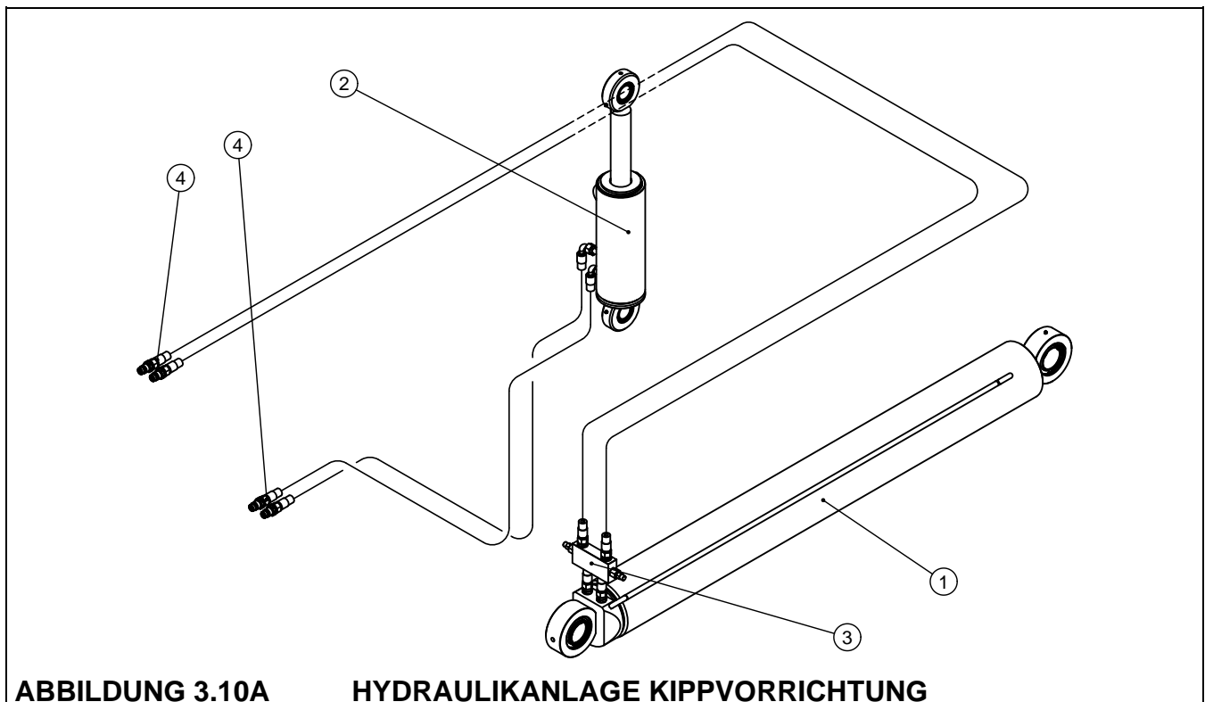
(1) Servomotor des Kipprahmens, (2) Servomotor des Hakenrahmens, (3) Ventil, (4) Leitungsanschluss
