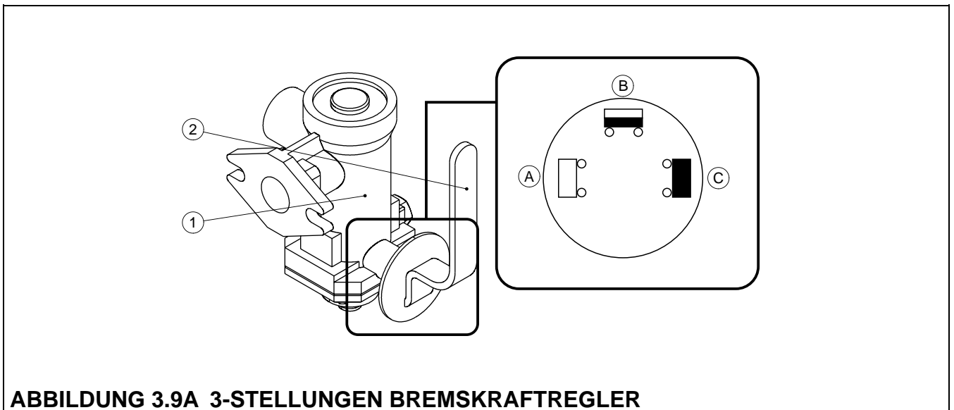
(1) 3-Stellungen Bremskraftregler, (2) Steuerhebel der Reglerarbeitsstellungen, (A), (B), (C) Reglerarbeitsstellungen
