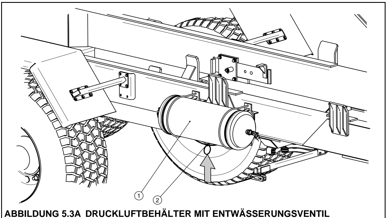
(1) Druckluftbehälter, (2) Entwässerungsventil
