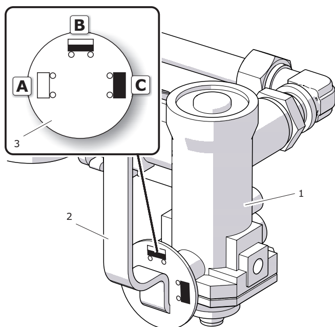
Rysunek 3.15 Trózzakresowy regulator siły hamowania
