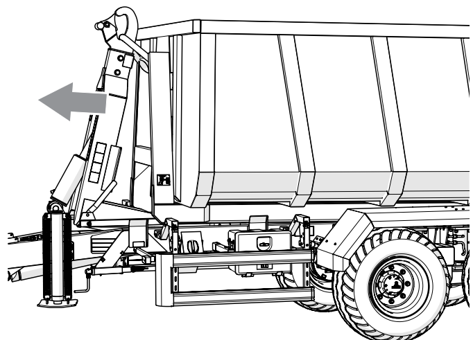
Rysunek 4.17 Wciąganie kontenera
