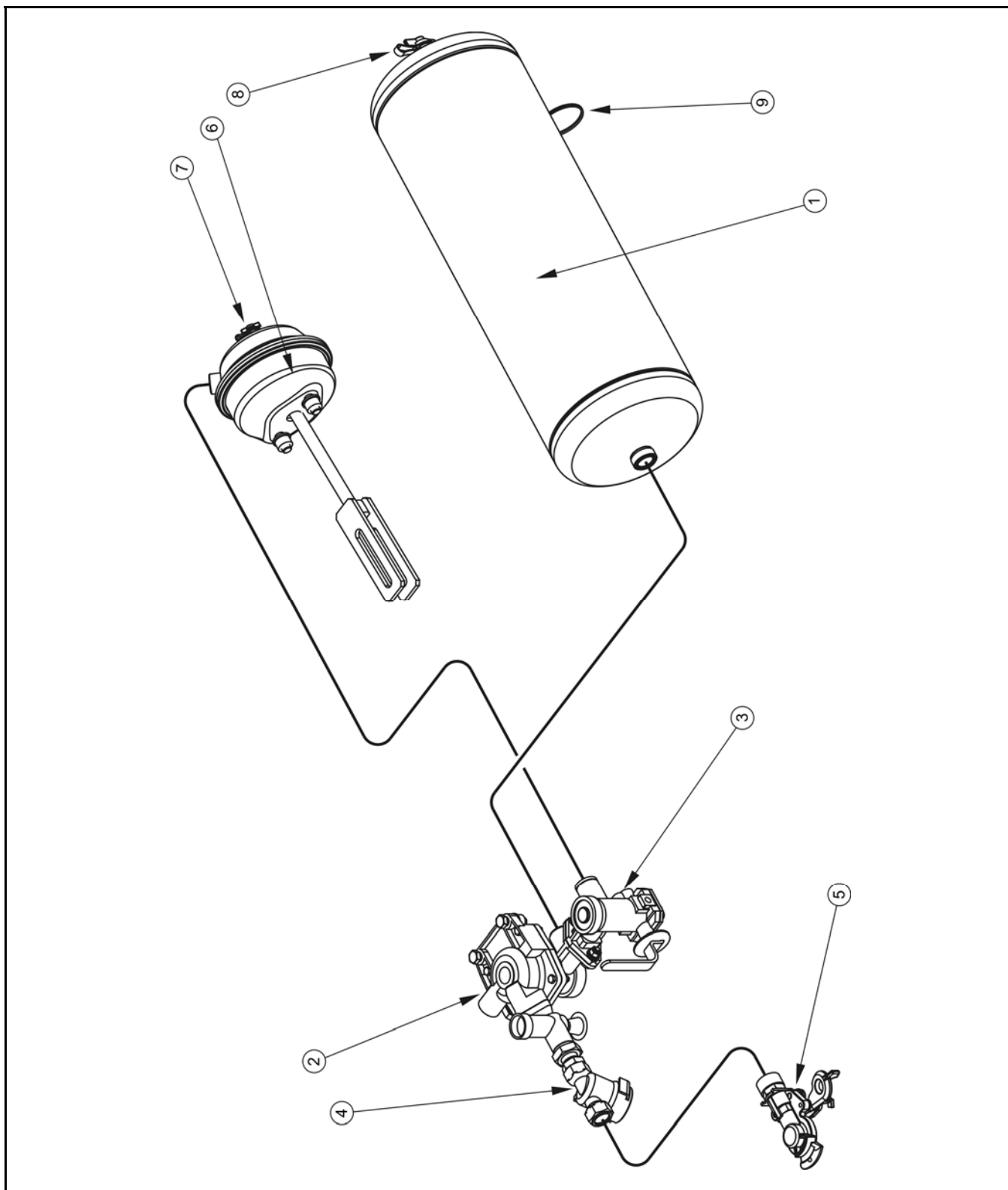
RYSUNEK 3.9A Instalacja pneumatyczna jedнопроводова
