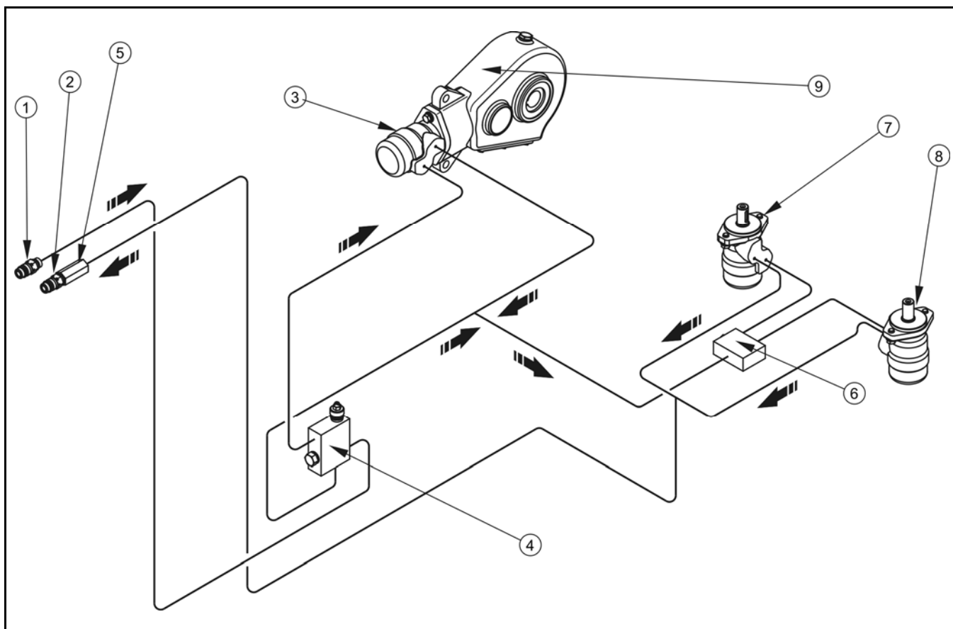
RYSUNEK 3.7A Instalacja hydrauliczna
