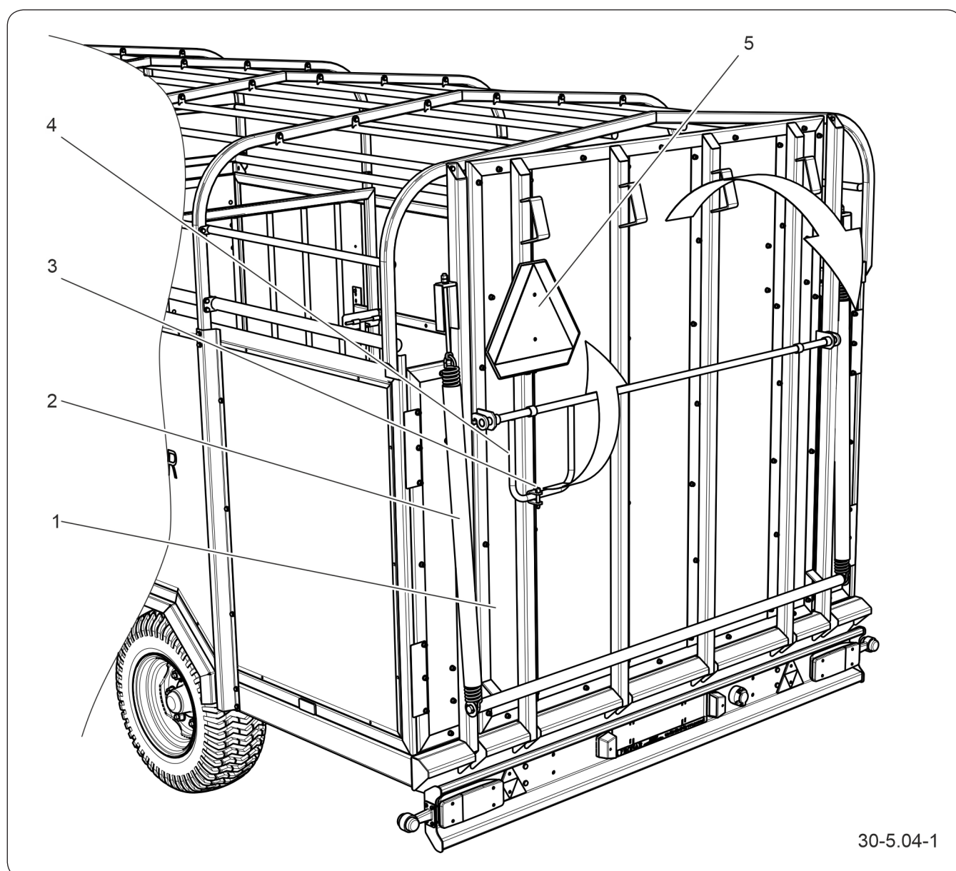
Rysunek 5.11 Kłapa tylna
