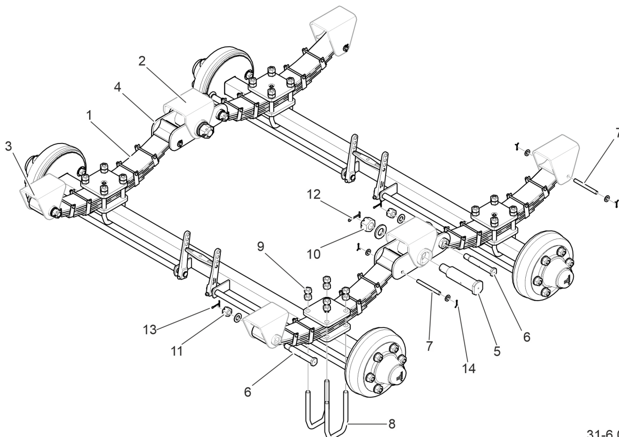
Rysunek 6.1 Obsługa zawieszenia mechanicznego
