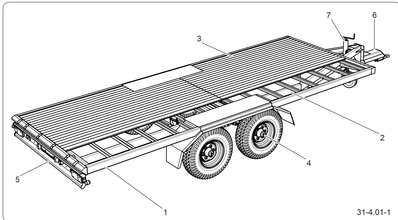
Rysunek 4.1 Podwozie
