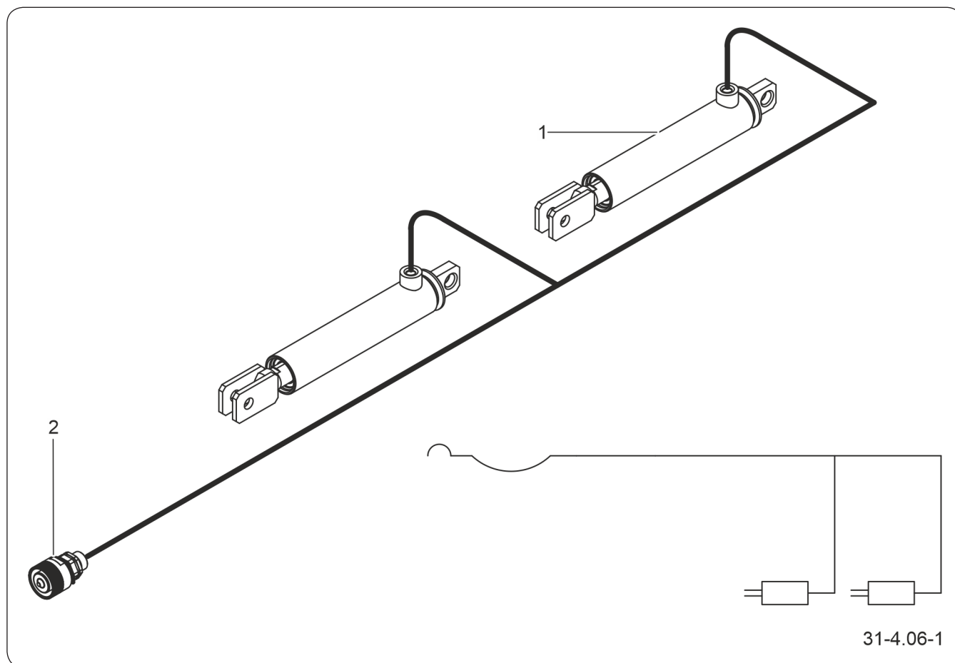
Rysunek 4.7 Budowa i schemat instalacji hydraulicznej hamulcowej
