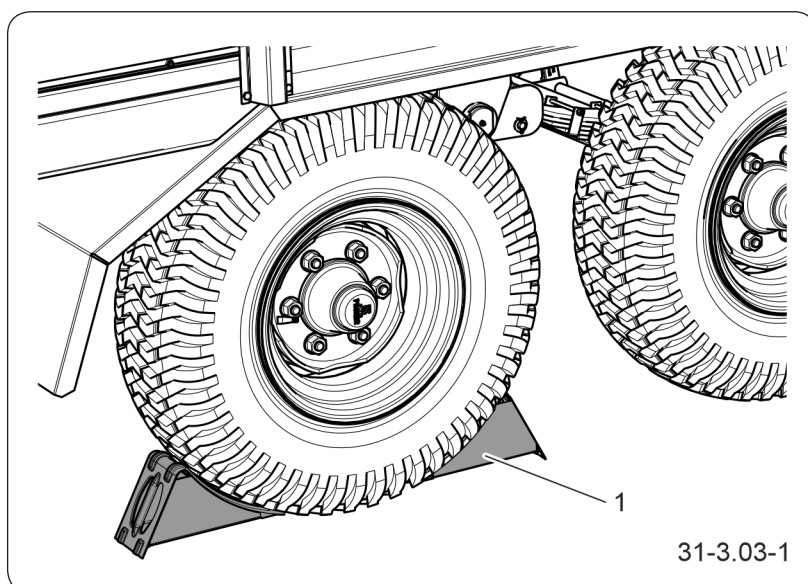
Rysunek 3.1 Ułożenie klinów blokujących (1) klin podporowy
