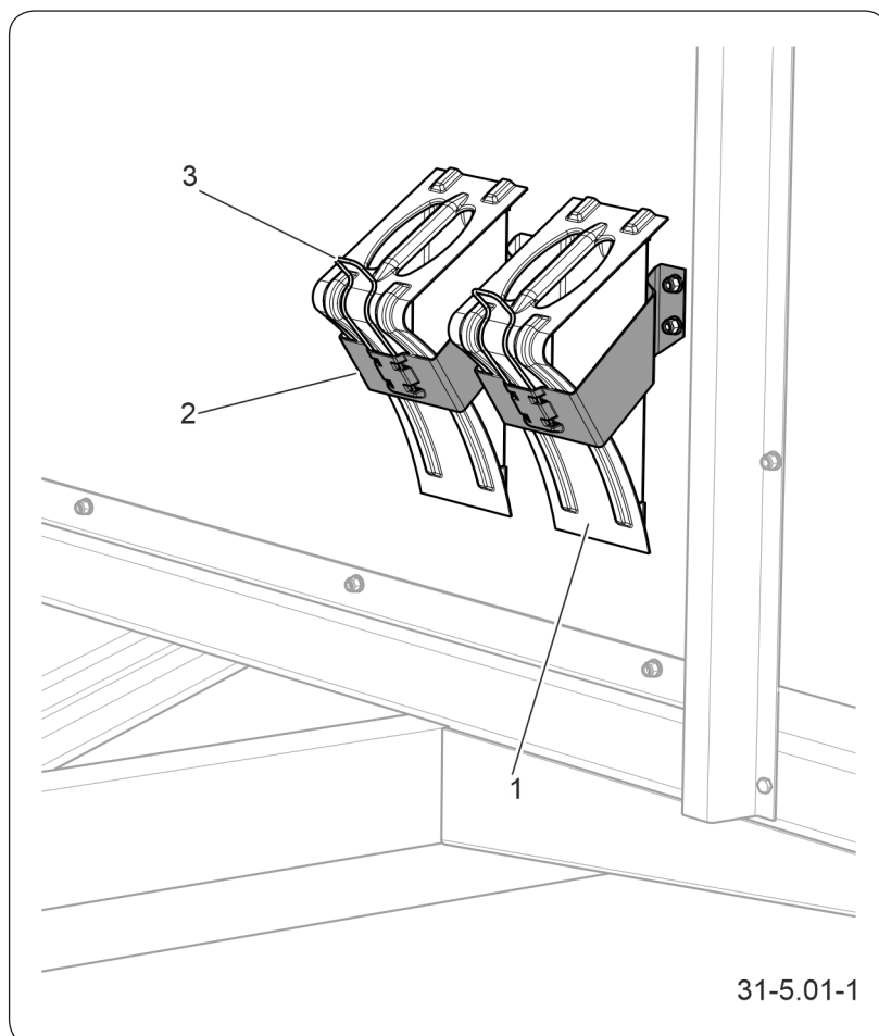
Rysunek 5.4 Umiejscowienie klinów
