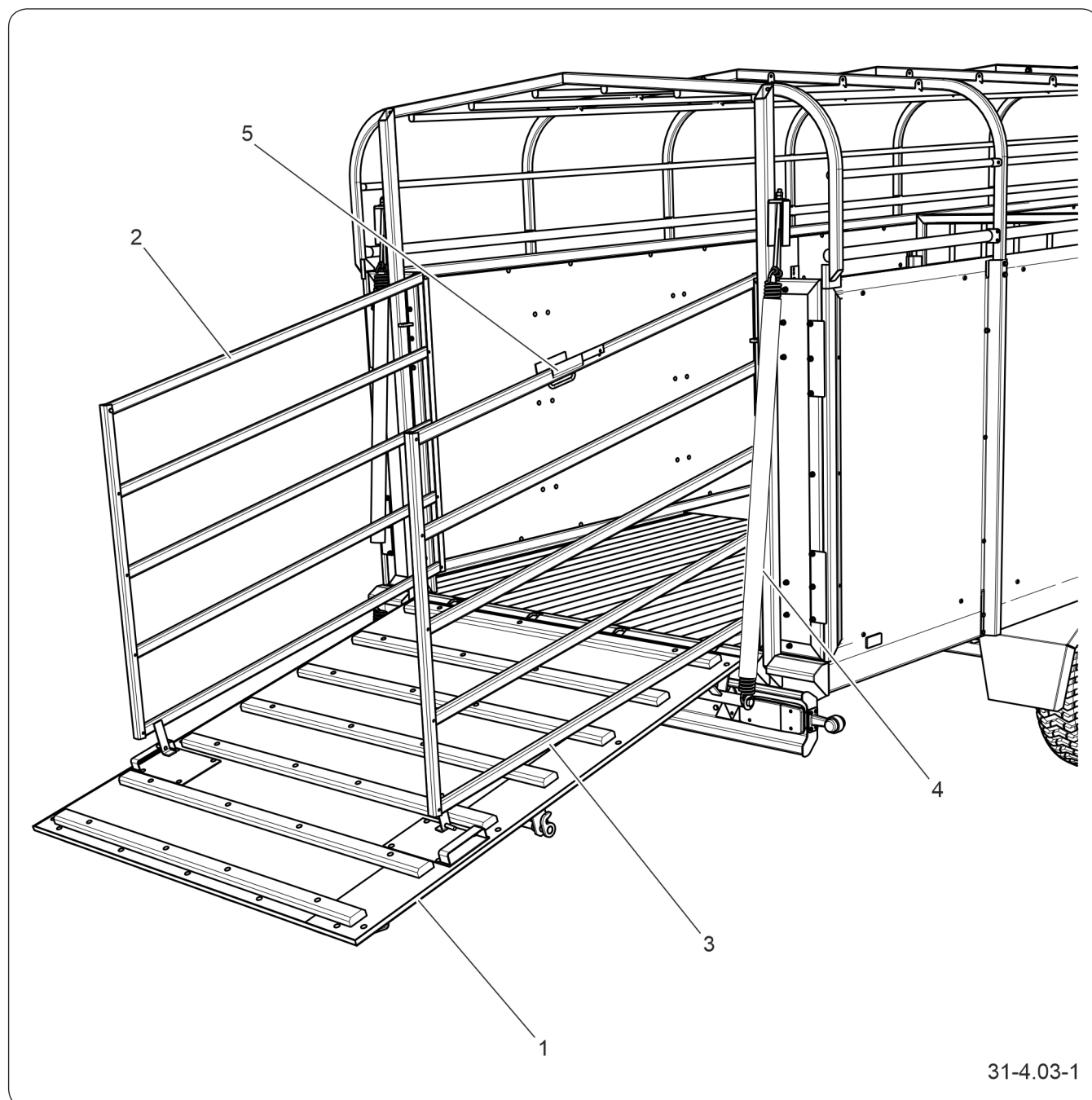
Rysunek 4.3 Kłapa i bramki tylne
