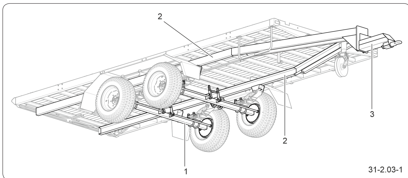
Rysunek 2.7 Punkty mocowania przyczepy
