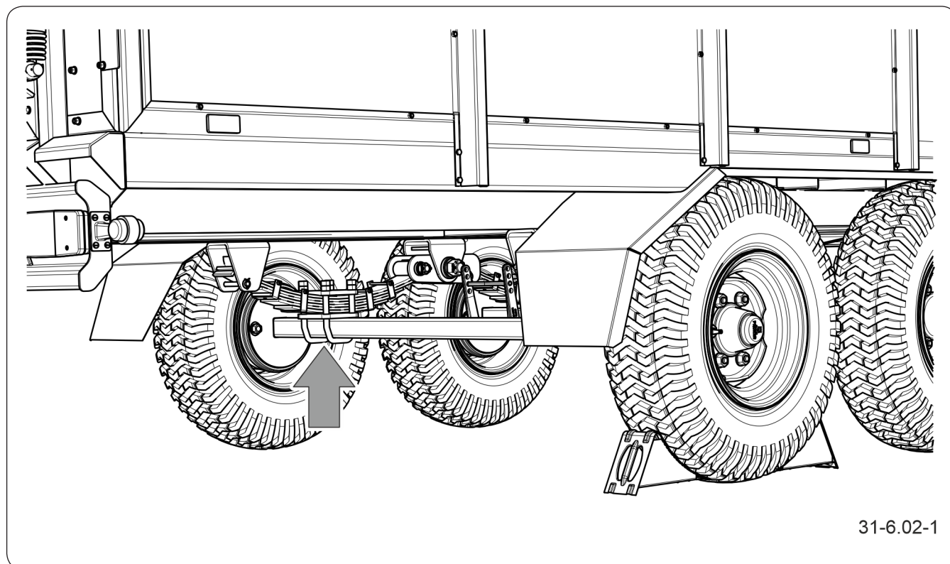
Rysunek 6.2 Zalecane punkty podparcia przyczepy
