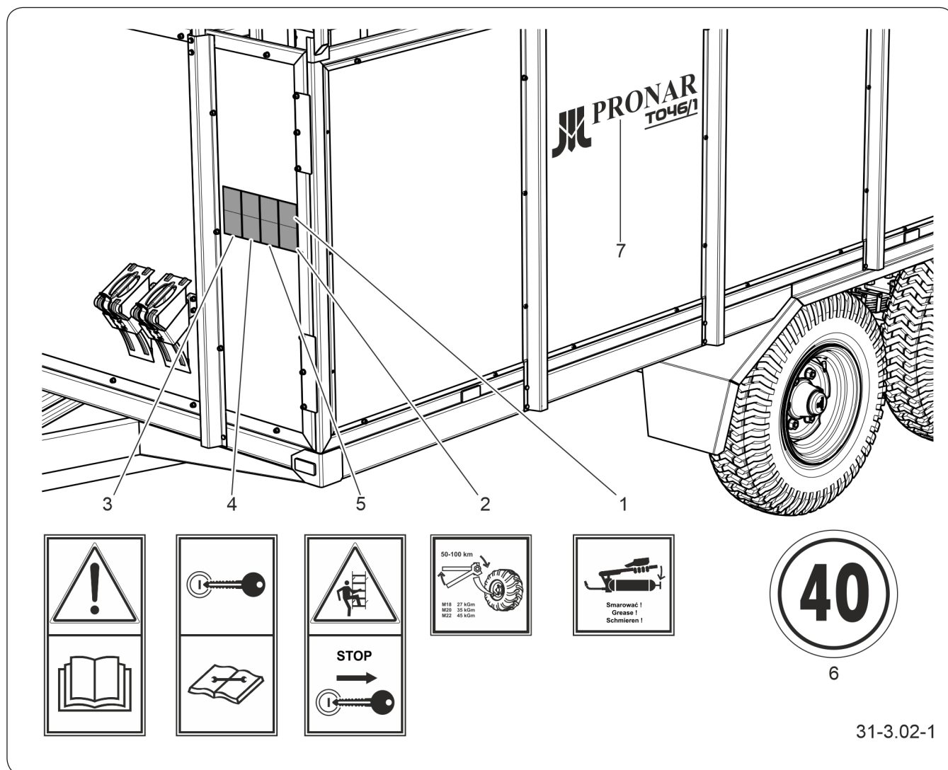
Rysunek 3.2 Rozmieszczenie nalepek informacyjnych i ostrzegawczych
