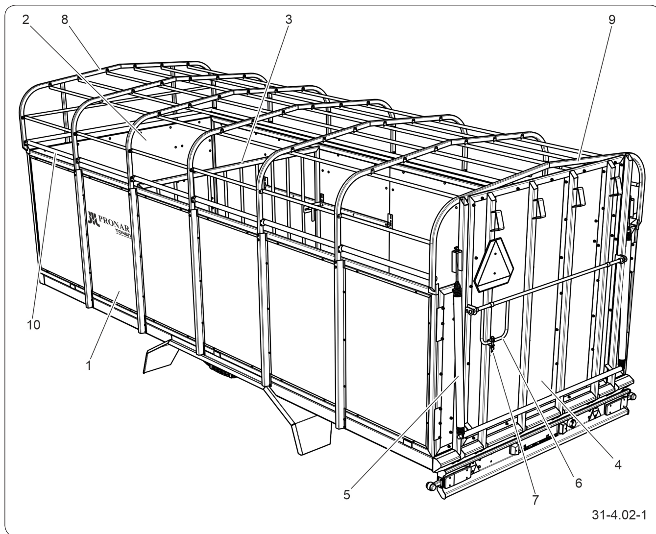
Rysunek 4.2 Skrzynia ładunkowa
