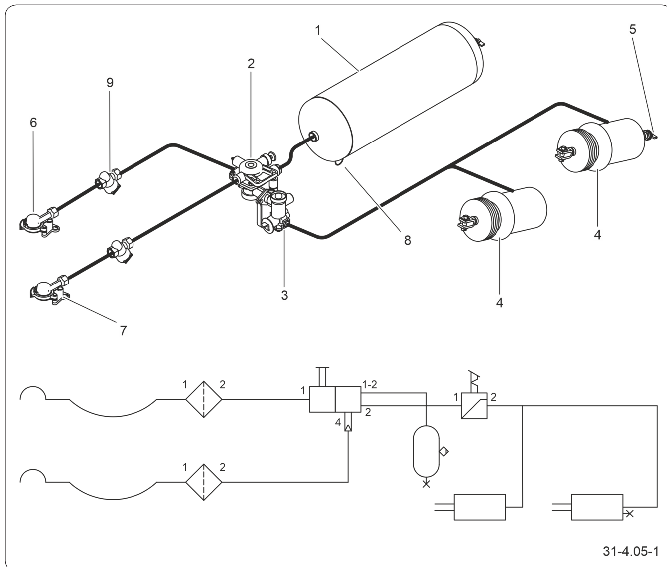
Rysunek 4.5 Budowa i schemat instalacji pneumatycznej dwuprzewodowej
