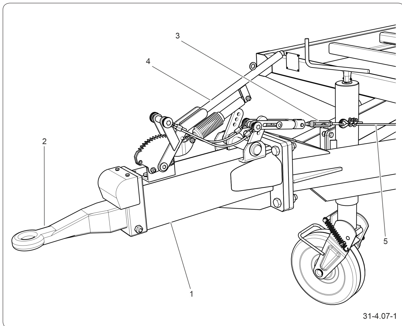
Rysunek 4.8 Budowa instalacji hamulca najazdowego
