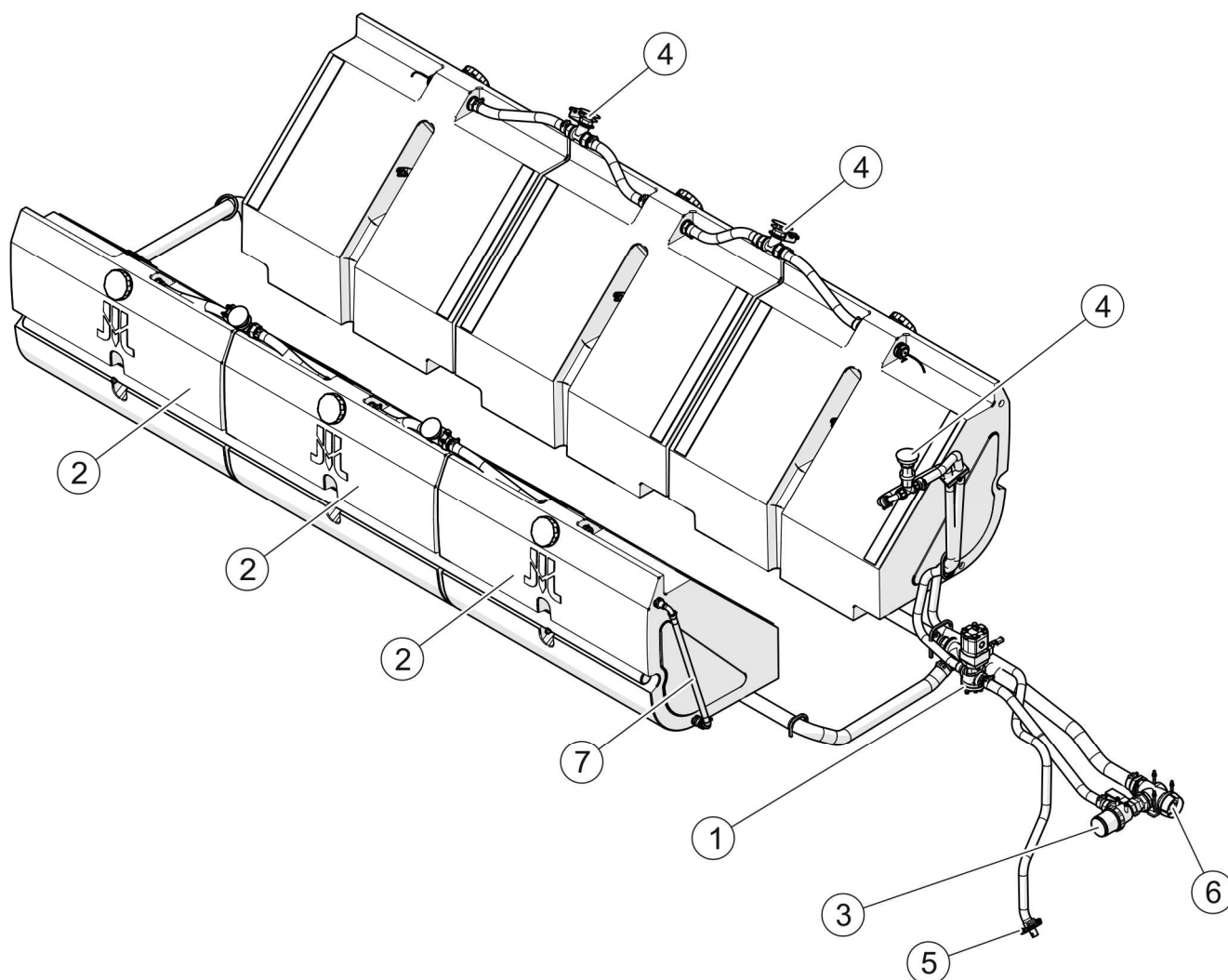
RYСУNEK 3.6 Budowa układu zraszania solanką
