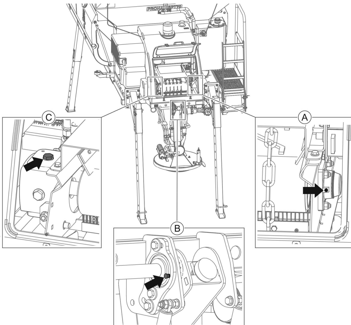
RYСУNEK 5.15 Punkty smarne
