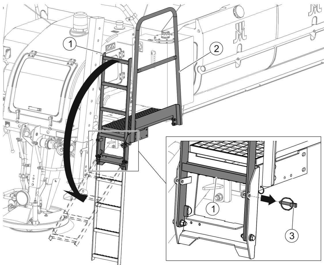
RYСУNEK 4.17 Podest z drabiną
