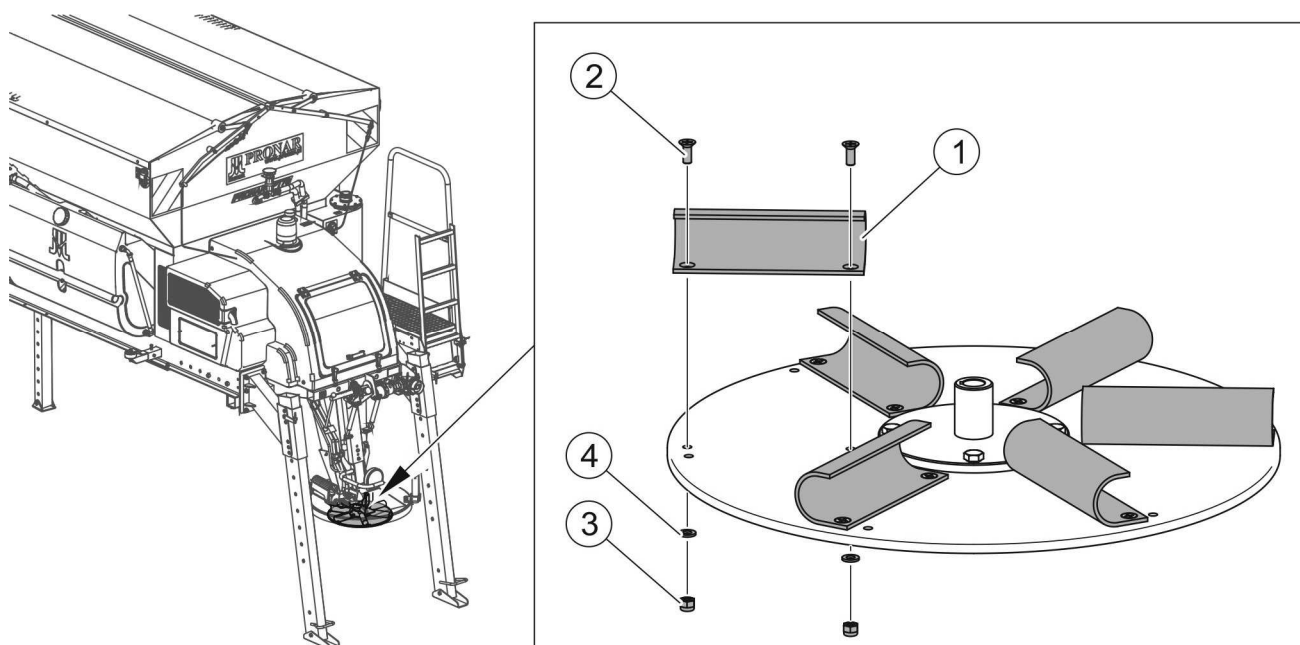
RYSUNEK 5.14 Wymiana łopatek tarczy mechanizmu wysiewającego
