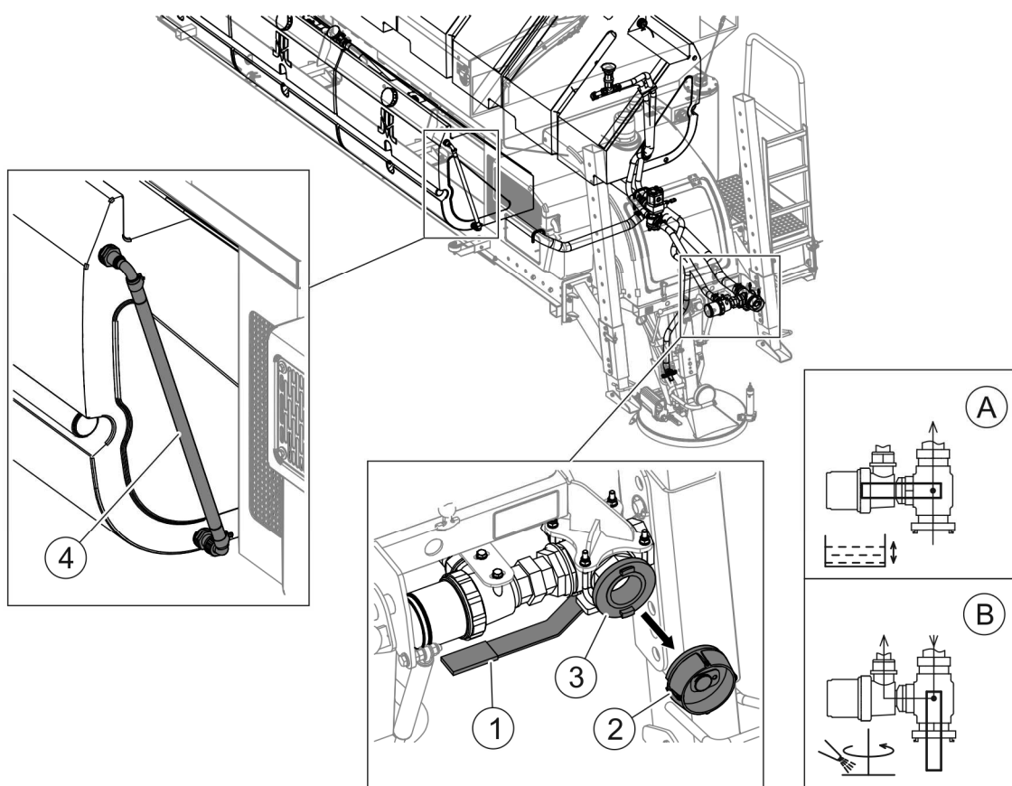
RYSUNEK 4.32 Opróżnianie zbiorników solanki
