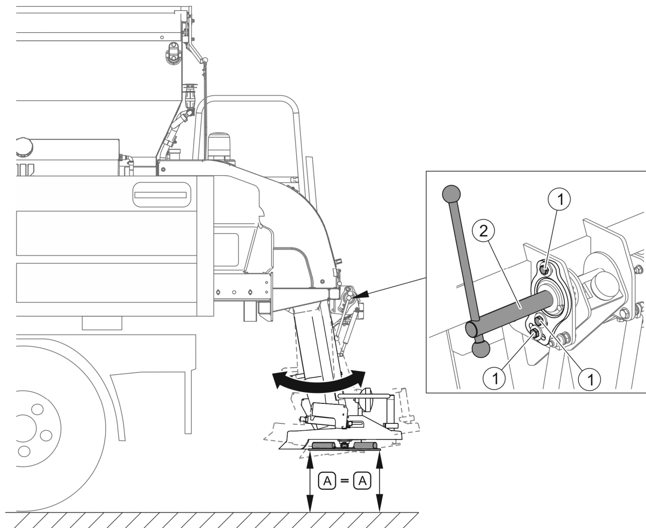
RYSUNEK 4.14 Poziomowanie tarczy rozsiewającej
