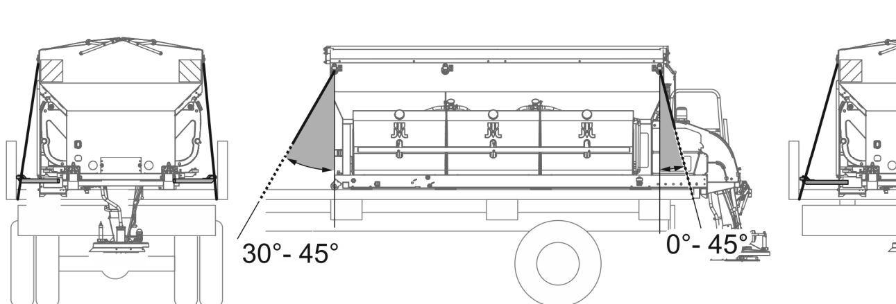
RYSUNEK 4.10 Mocowanie 2
