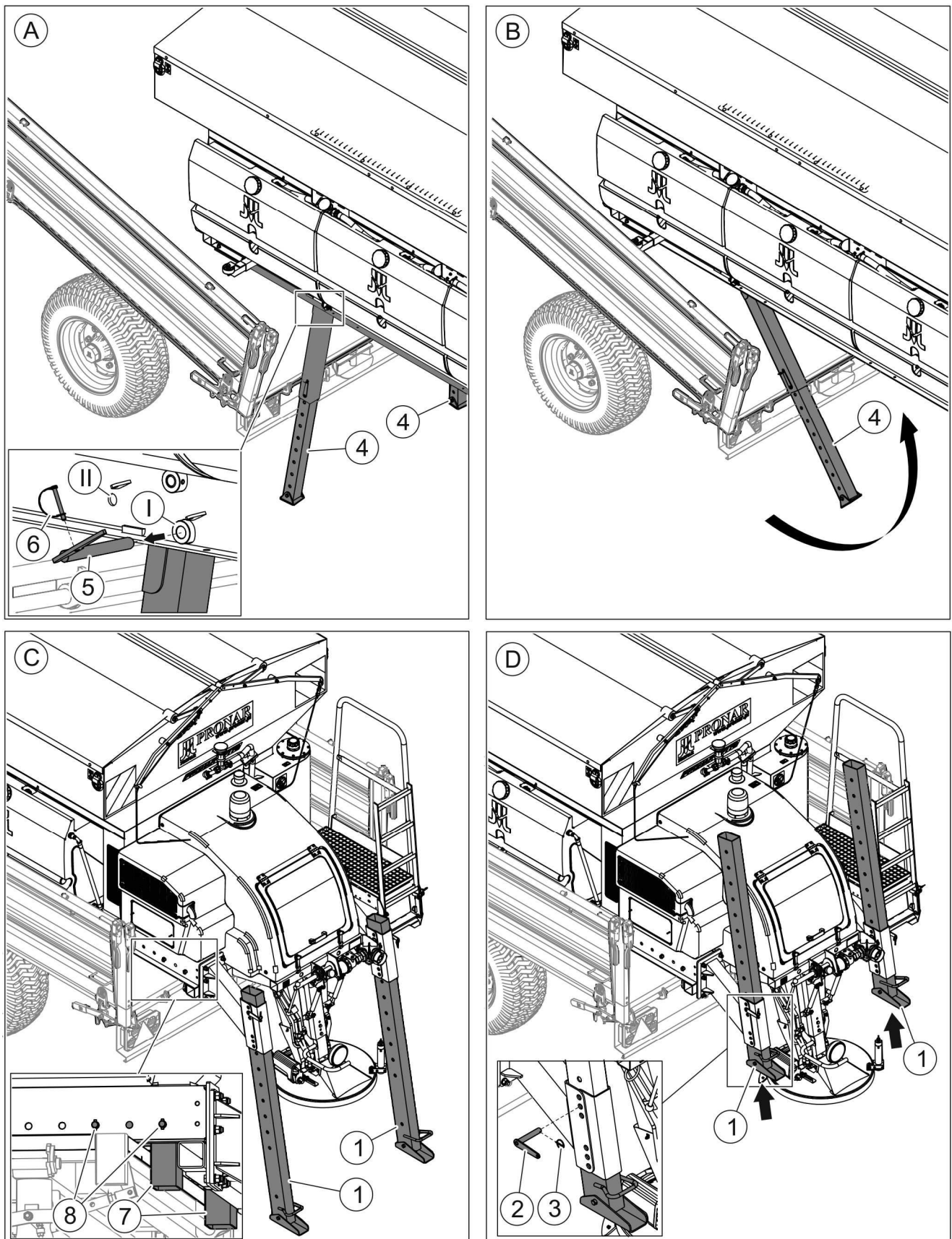
RYСУNEK 4.7 Etapy załadunku maszyny
