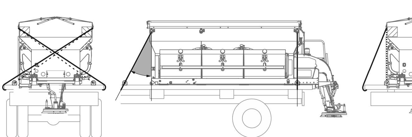
RYSUNEK 4.9 Mocowanie 1
