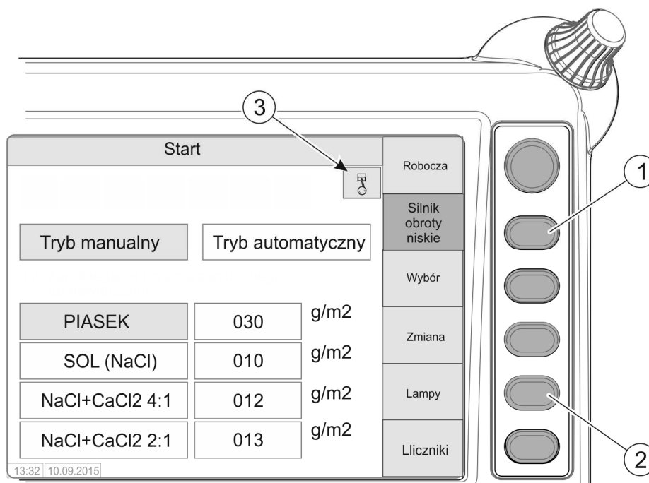
RYСУNEK 4.29 Zatrzymanie silnika
