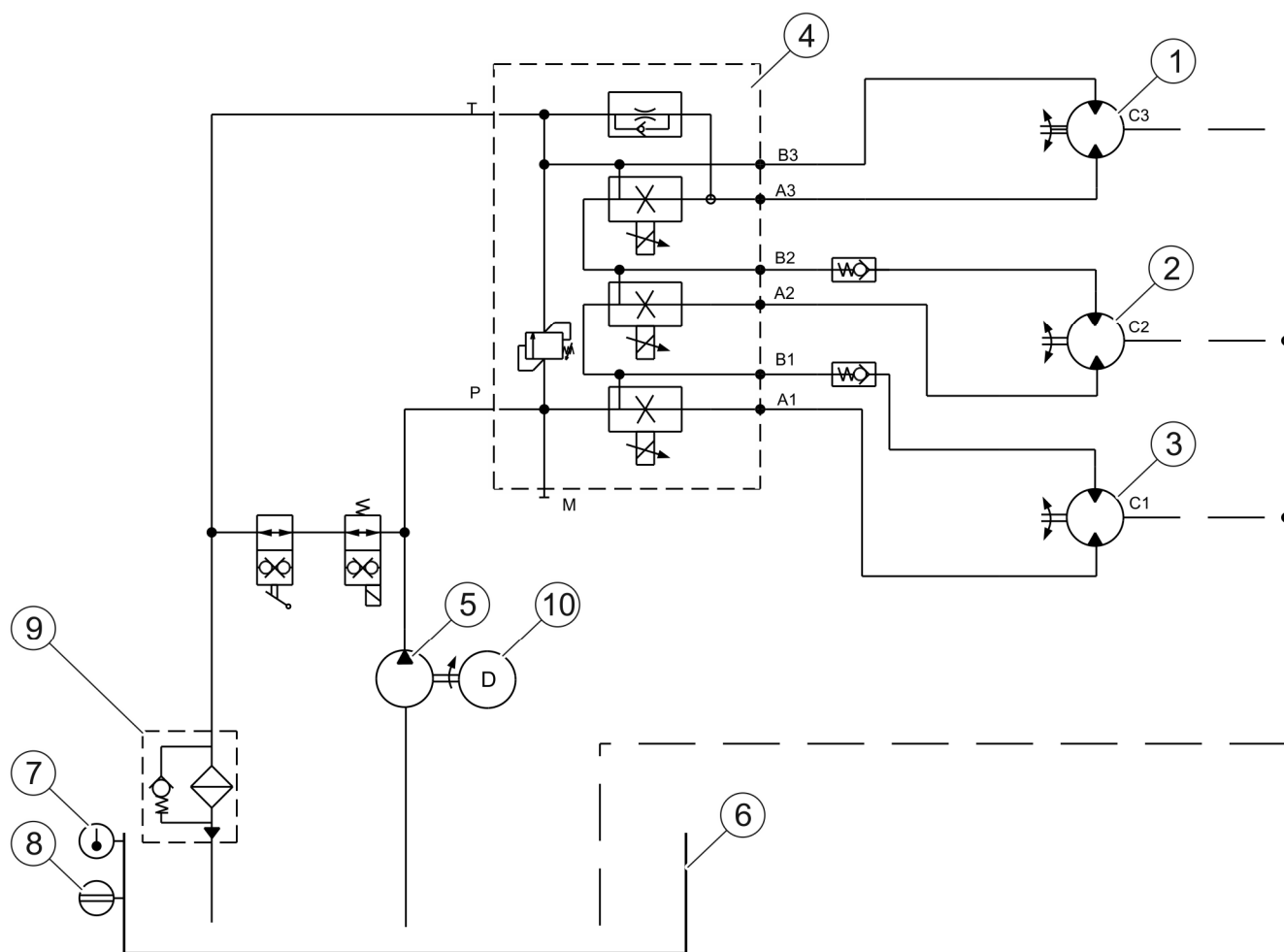
RYSUNEK 3.5 Schemat instalacji hydraulicznej
