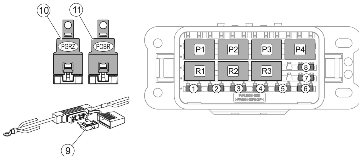
RYSUNEK 5.7 Bezpieczniki i przekaźniki
