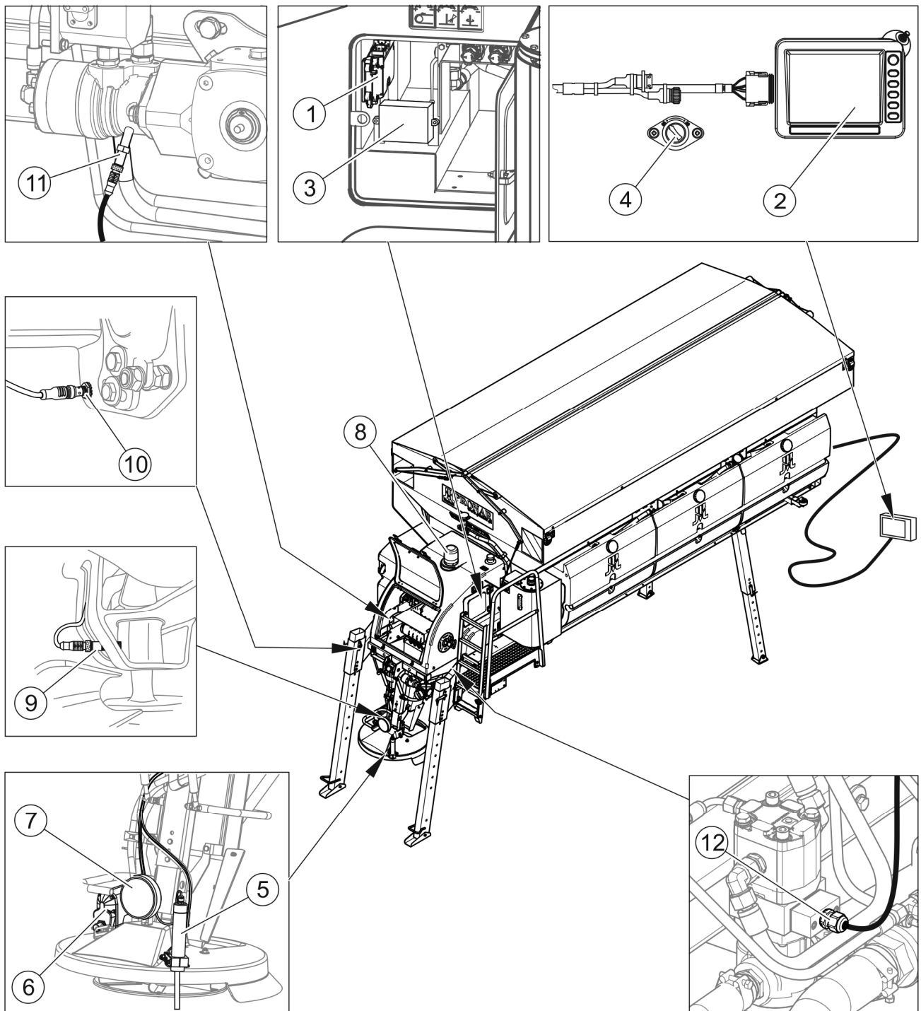
RYСУNEK 3.8 Budowa instalacji elektrycznej
