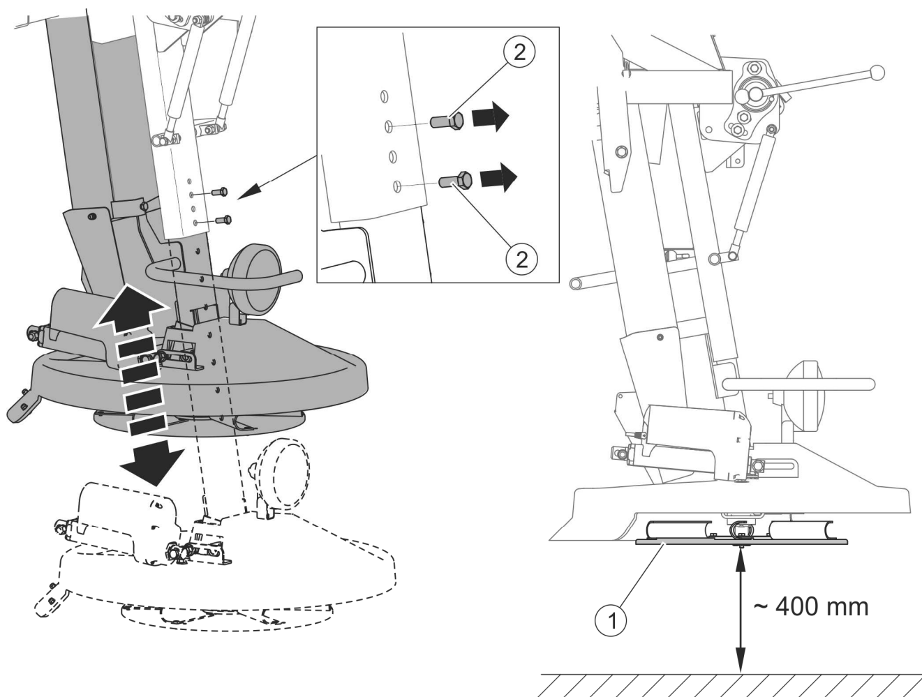
RYСУNEK 4.15 Ustawienie odległości tarczy rozsiewającej od jezdni
