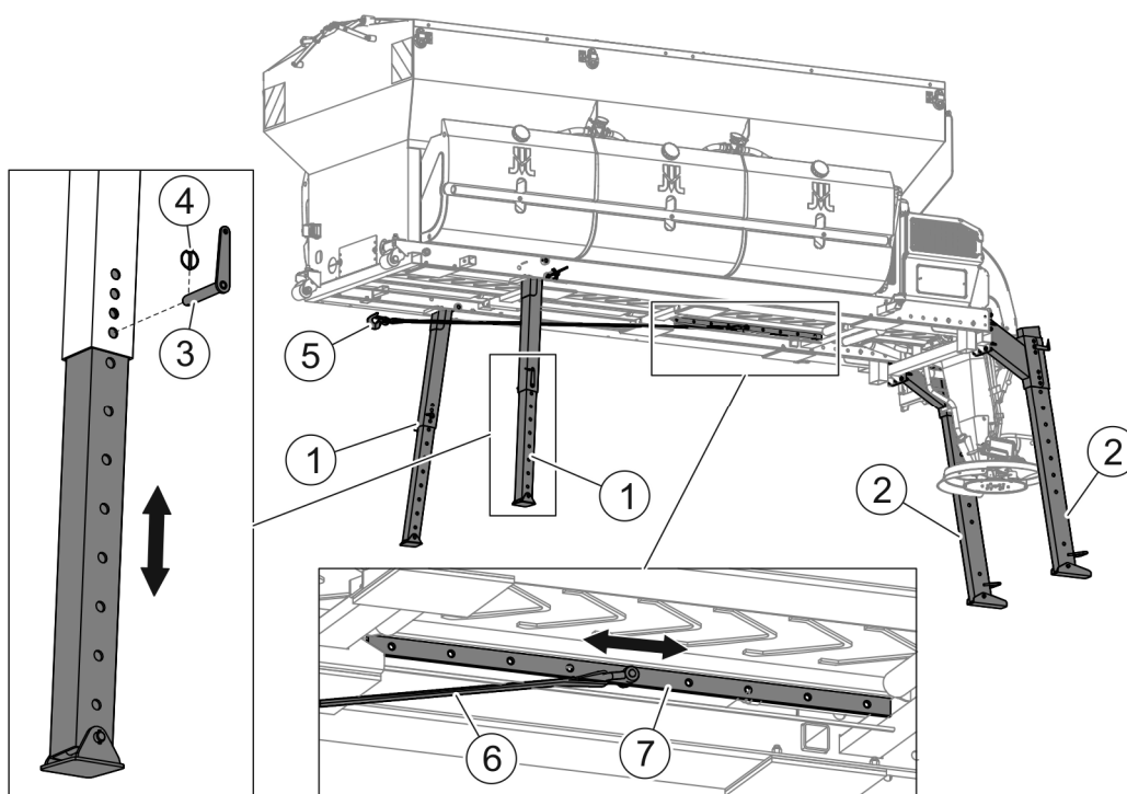
RYСУNEK 4.5 Nogi postojowe
