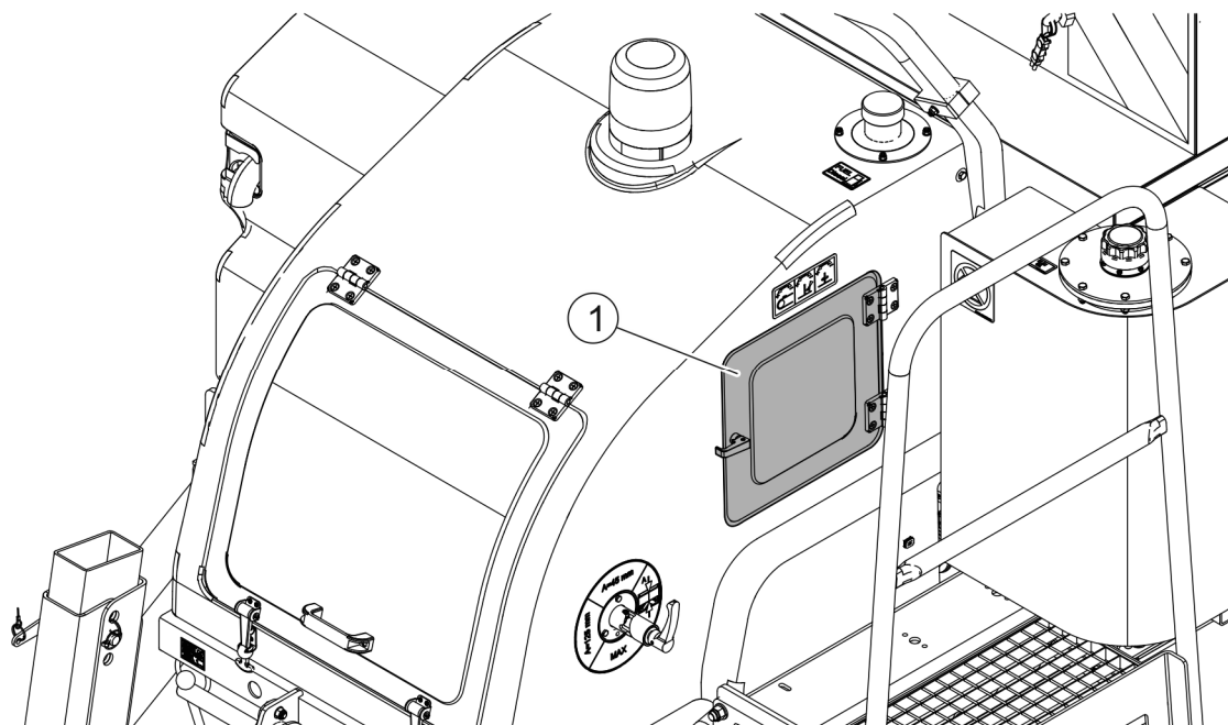
RYSUNEK 5.6 Umieszczenie skrzynki bezpiecznikowej
