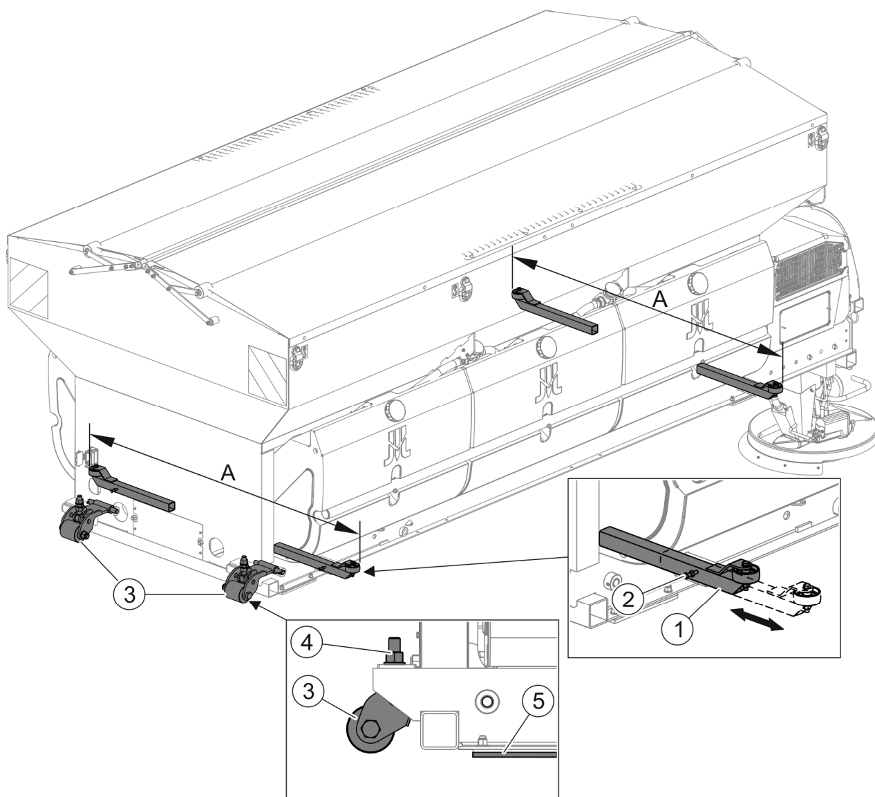
RYSUNEK 4.6 Prowadnice
