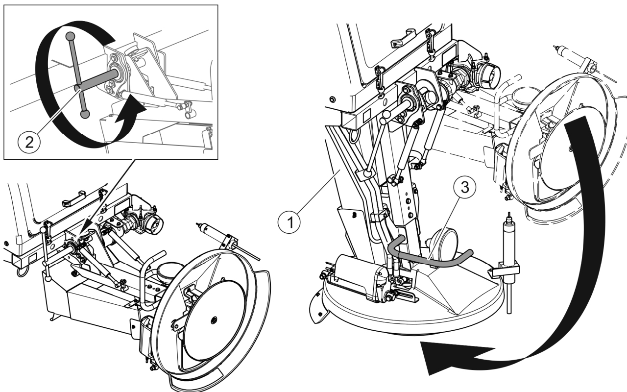
RYSUNEK 4.13 Opuszczanie mechanizmu rozsiewającego
