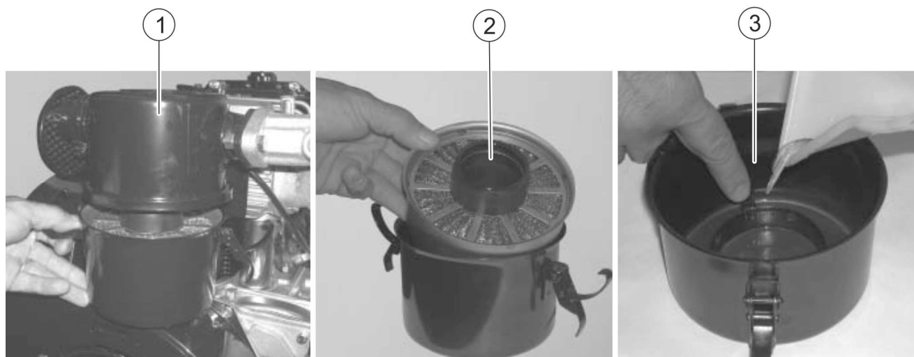
RYSUNEK 4.4 Kontrola poziomu oleju w filtrze powietrza
