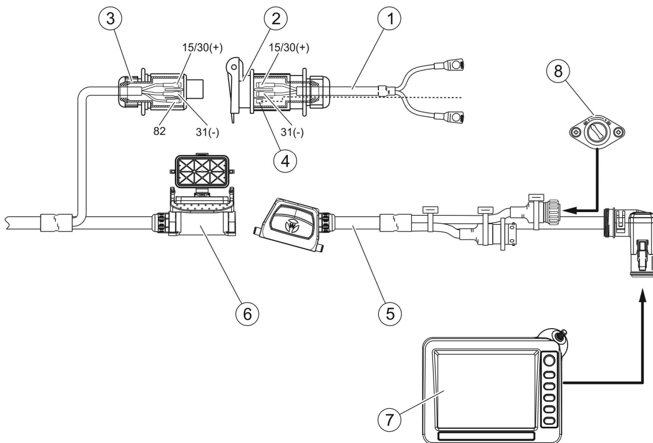
RYSUNEK 4.12 Podłączenie instalacji elektrycznej
