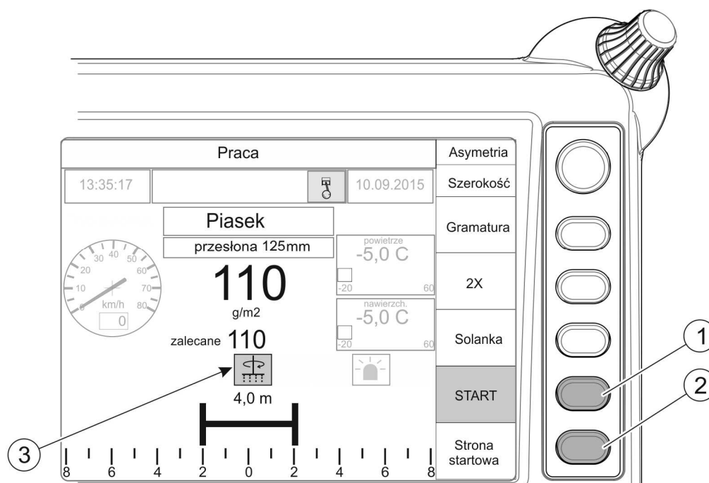
RYСУNEK 4.28 Zatrzymanie posypywania
