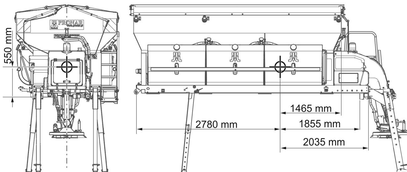
RYSUNEK 1.4 Położenie środka ciężkości (puste zbiorniki)
