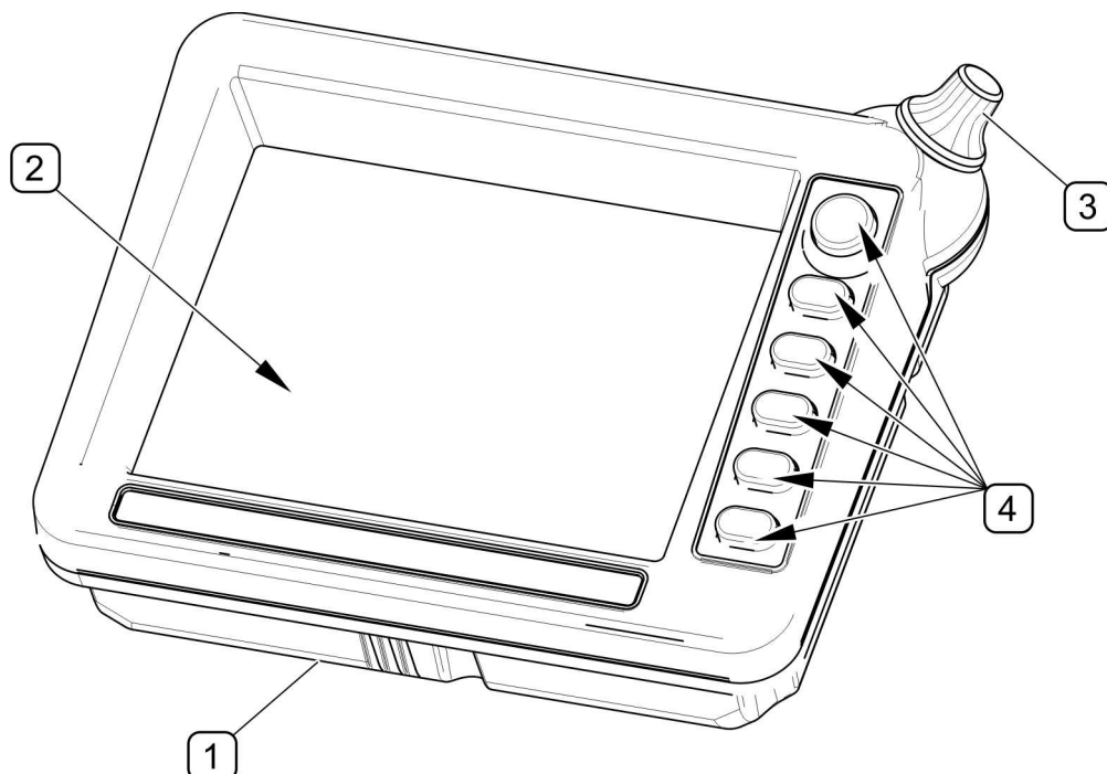
RYSUNEK 3.9 Budowa ogólna panelu sterowania
