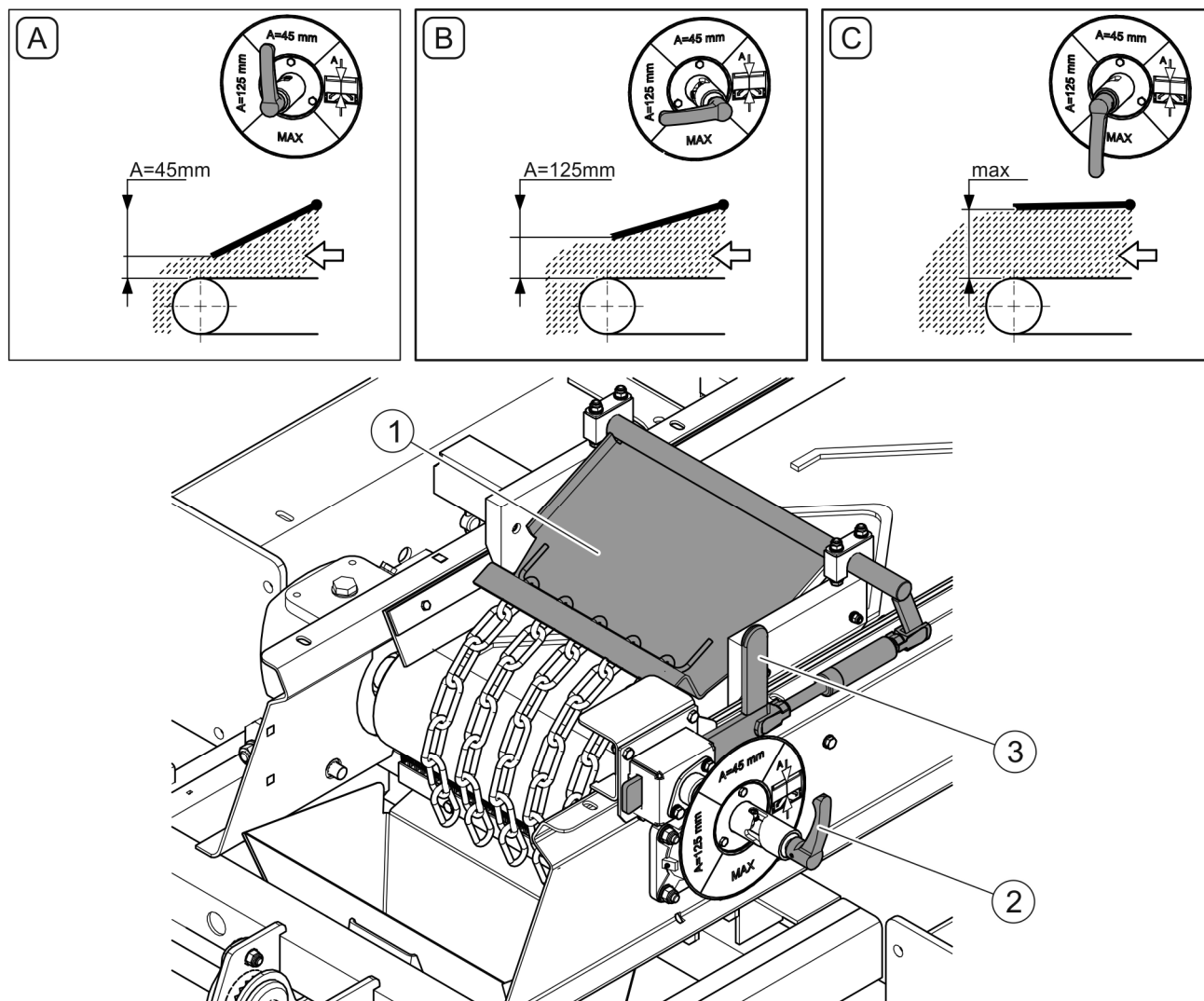
RYSUNEK 4.16 Ustawienie przesłony przenośnika taśmowego
