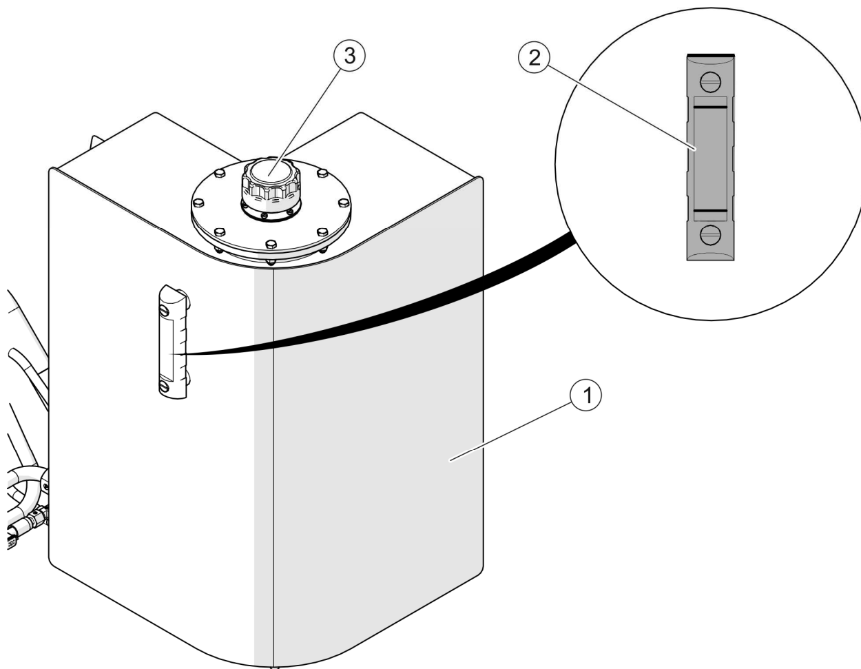
RYСУNEK 4.1 Kontrola poziomu oleju hydraulicznego
