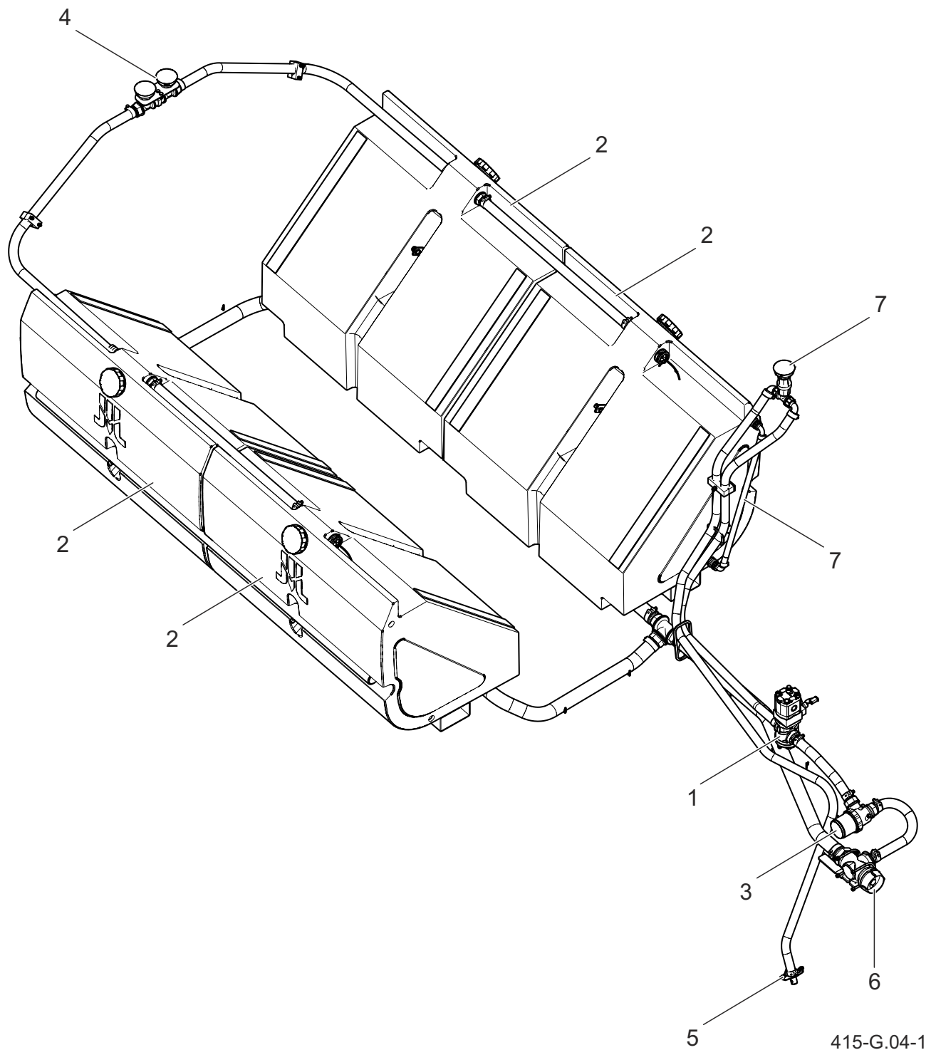
Малюнок 3.4 Конструкція системи зрошення розсолу
