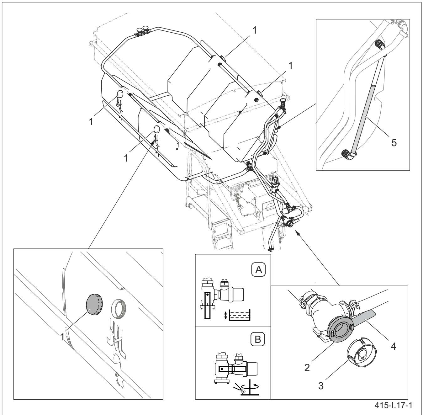
Малюнок 5.17 Наповнювання резервуарів розсолем
