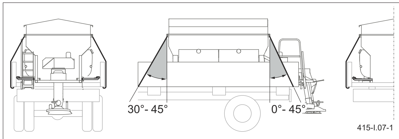
Малюнок 5.7 Кріплення 3
