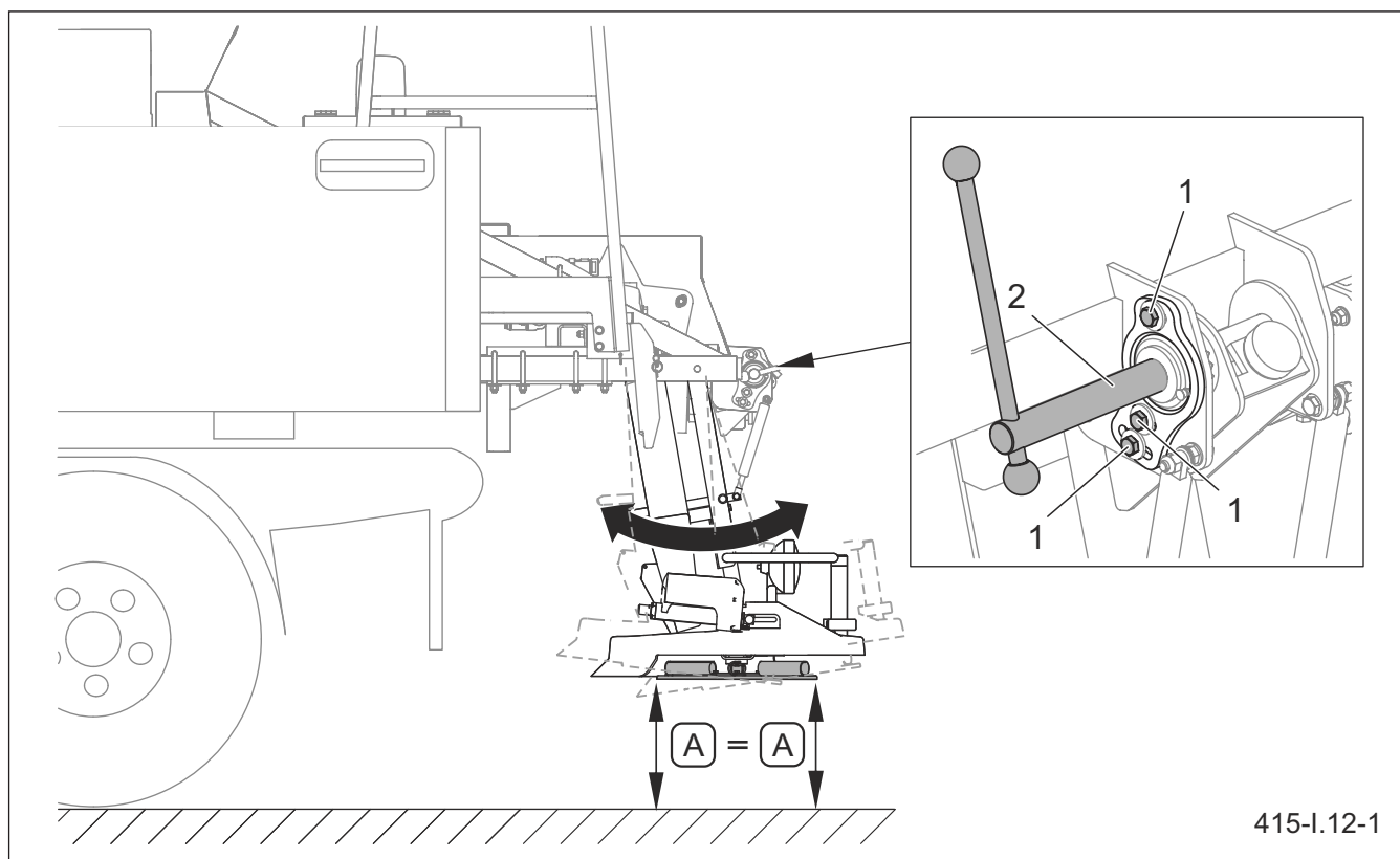
Малюнок 5.12 Вирівнювання розкидного диска (1) гвинт (2) затискний гвинт
