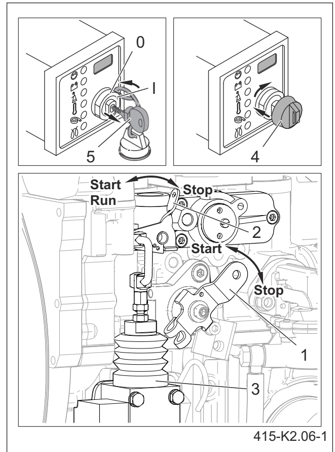
Малюнок 7.6 Зупинка двигуна
