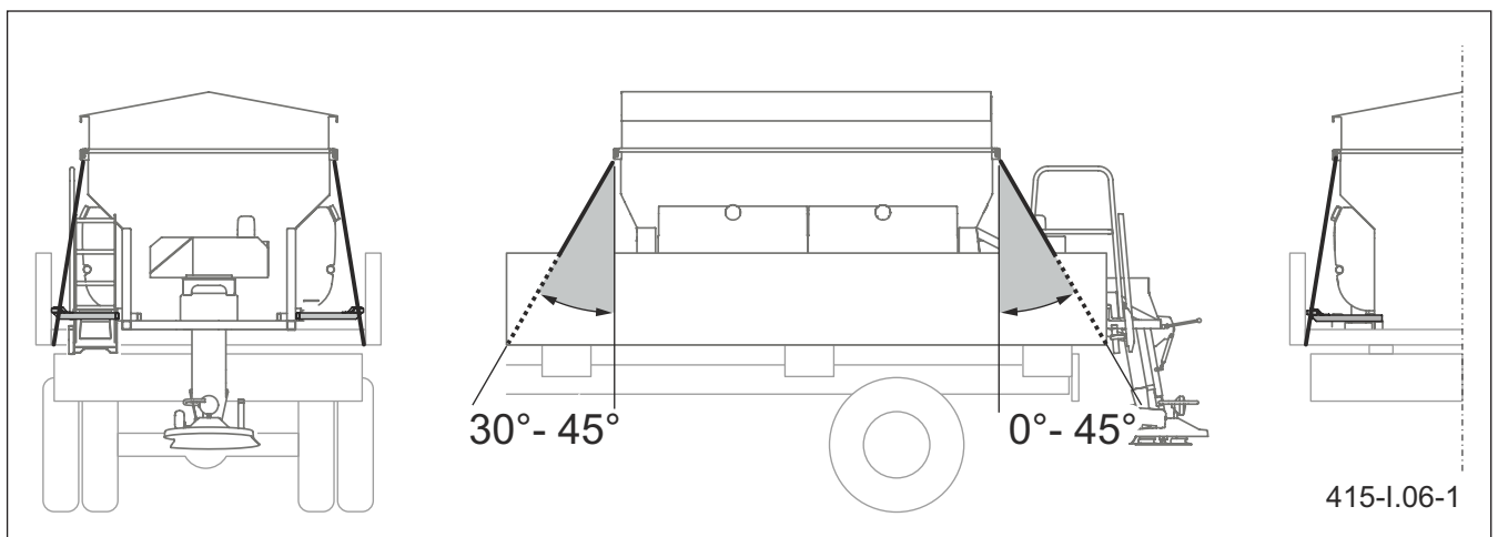
Малюнок 5.6 Кріплення 2
