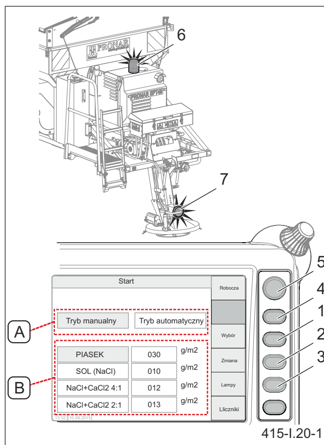
Малюнок 5.19 Включення окремих функцій на стартовій сторінці панелі (A) поле вибору режиму роботи (B) поле вибору матеріалу (1-5) функціональні кнопки (6) попереджувальна спалахова лампа (7) задня лампа
