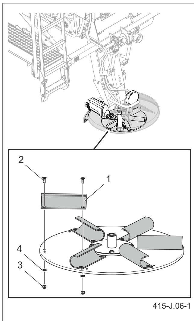
Малюнок 6.6 Заміна лопатей диска висівного механізму
