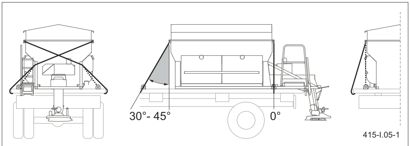
Малюнок 5.5 Кріплення 1
