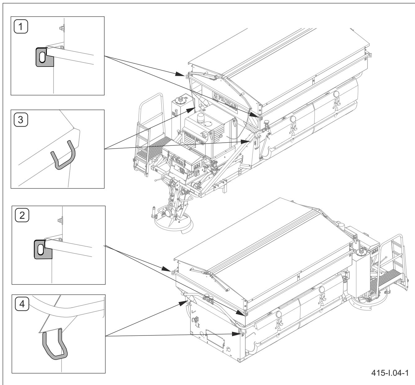
Малюнок 5.4 Точки кріплення ременів
