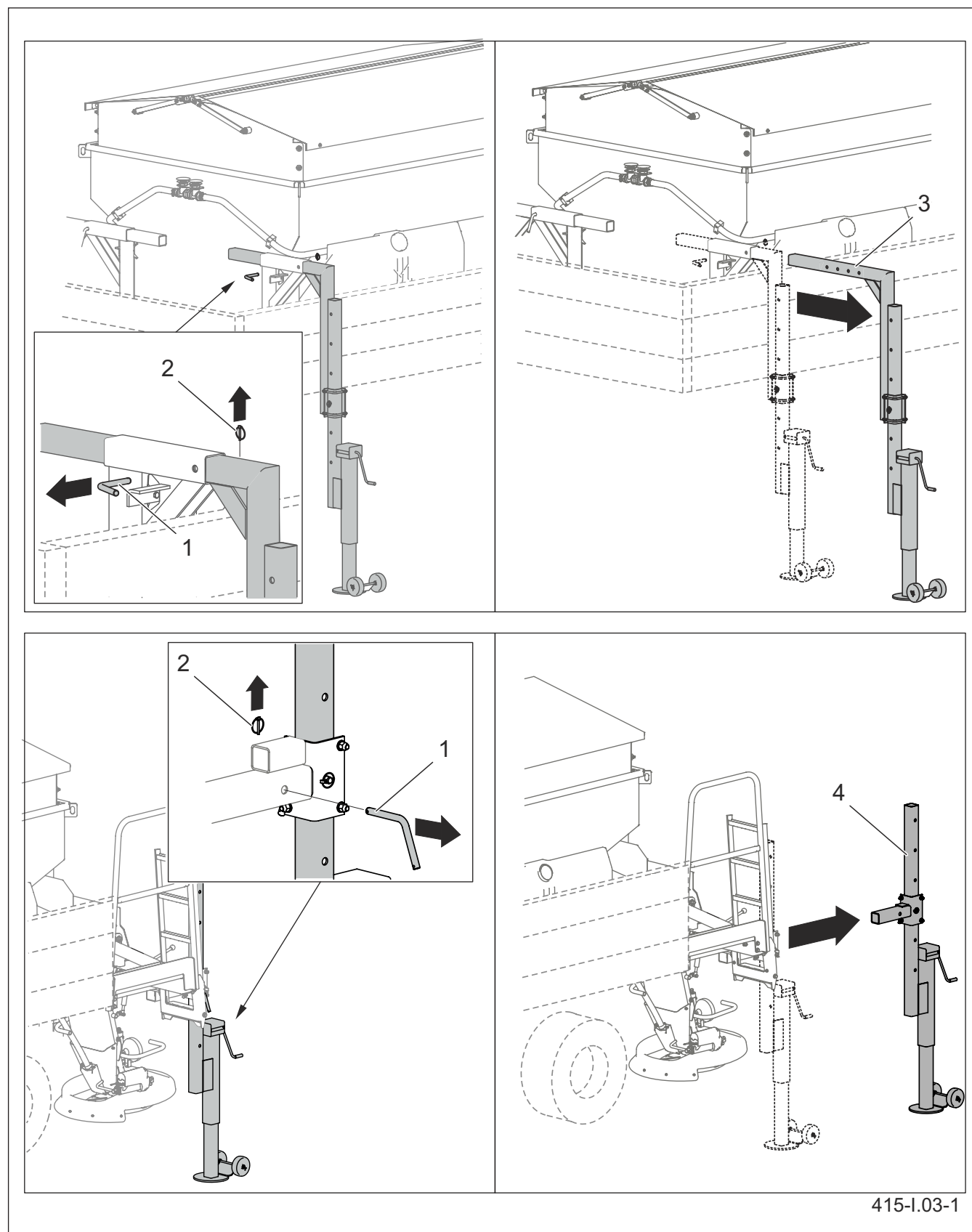
Малюнок 5.3 Демонтаж паркувальних опор
