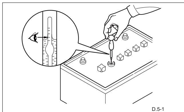
Малюнок 6.12 Вимірювання щільності електроліту
