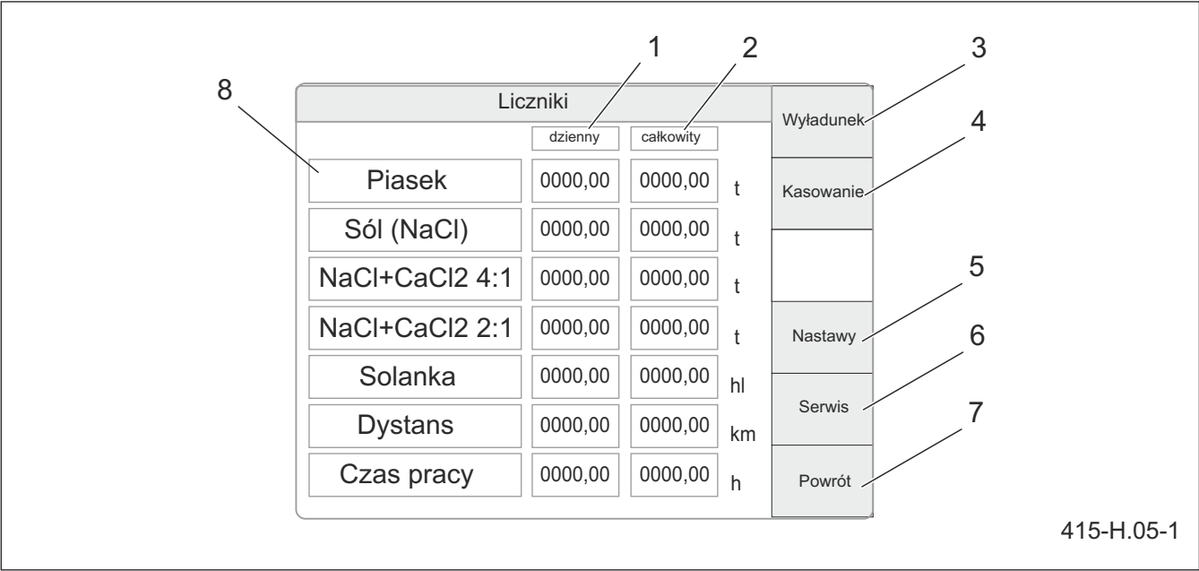
Малюнок 4.5 Сторінка лічильника дисплея панелі керування Опис значення функції сторінки лічильника представлено в ТАБЛИЦІ 4.3
