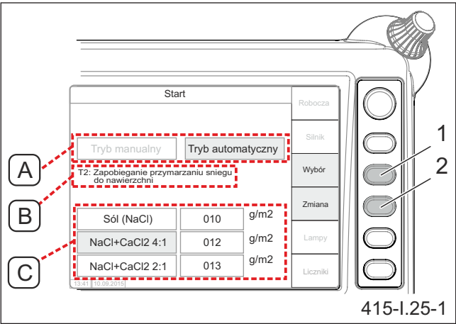
Малюнок 5.24 Зупинка автоматичного режиму (1) кнопка для вибору поля для редагування A, B або C (2) кнопка для зміни вибраного поля (A) поле для типу режиму роботи автоматичний/ручний (B) поле для вибору типу автоматичного режиму T1, T2, T3 (C) поле для вибору матеріалу для посипання
