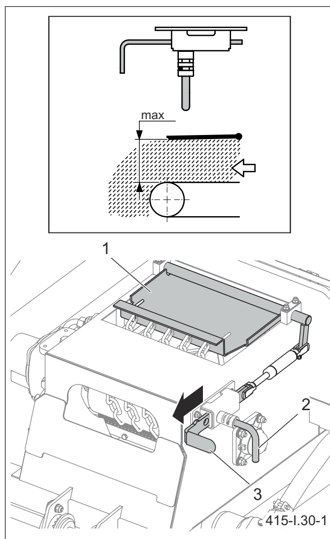
Малюнок 5.28 Постановка затвора на розвантаження (1) затвор (2) фіксуючий стрижень (3) повзунок
