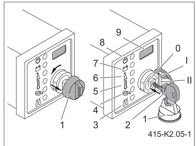
Малюнок 7.5 Стартер (1) захисний ковпачок (2) ключ запалювання (3-8) інформаційно-попереджувальні лампи (9) лічильник годин роботи - опція
