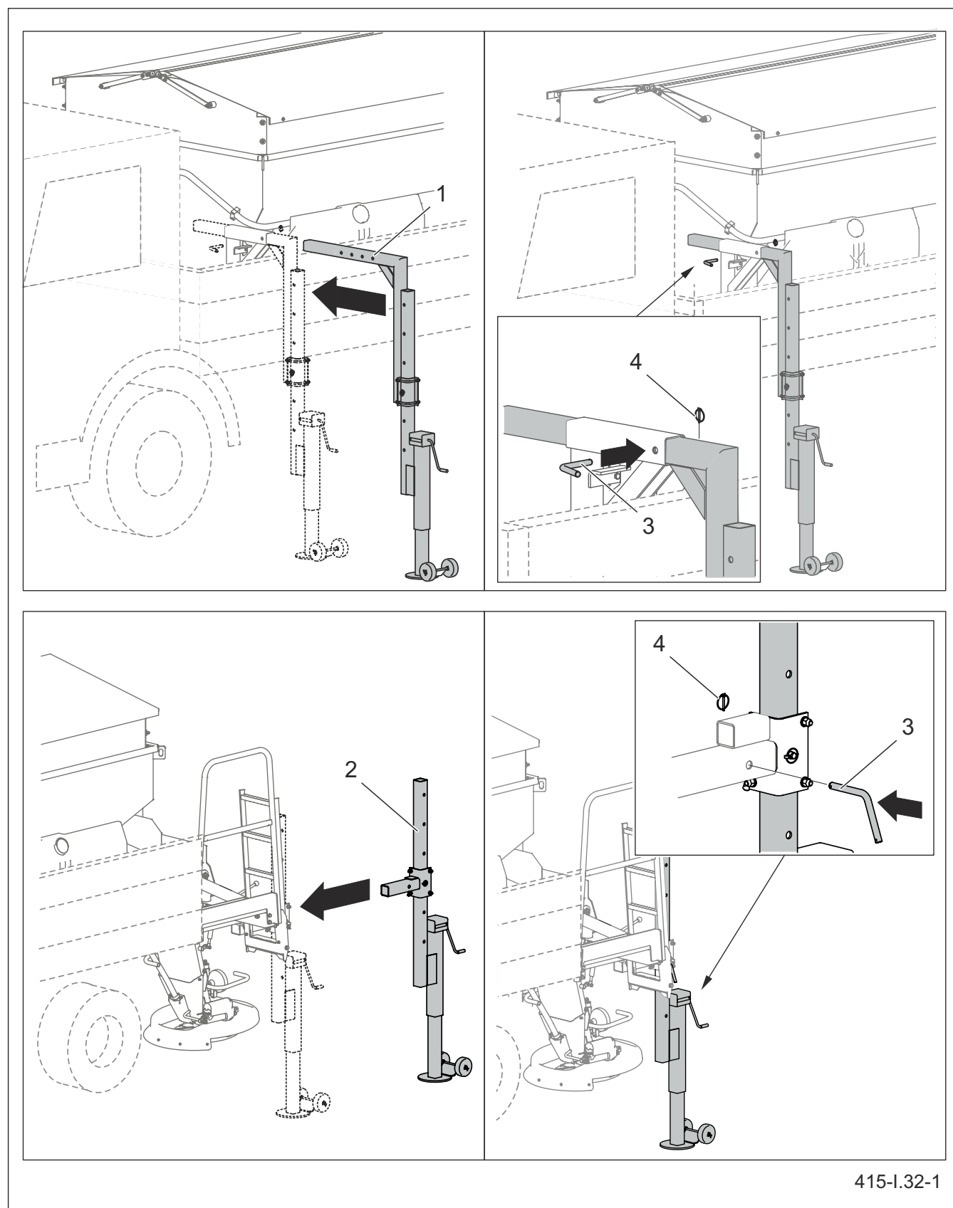
Малюнок 5.30 Монтаж паркувальних опор
