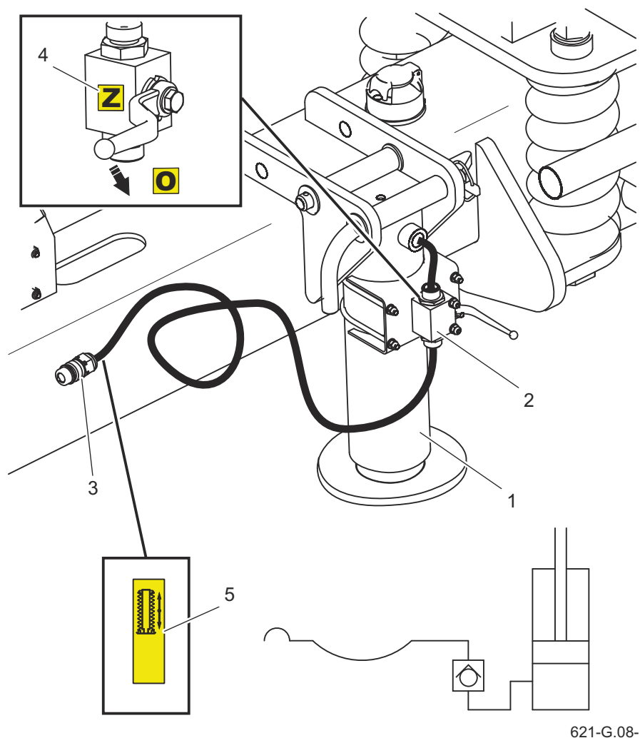
Rysunek 3.8 Budowa i schemat instalacji hydraulicznej podpory
