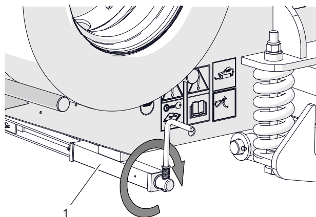
Rysunek 4.2 Hamulec postojowy (1) mechanizm hamulca
