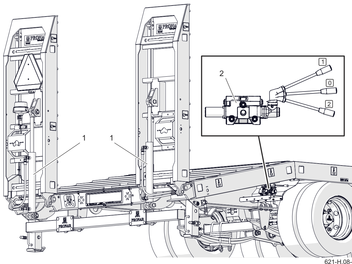
Rysunek 4.8 Najazdy hydrauliczne (1) siłownik hydrauliczny (2) rozdzielacz
