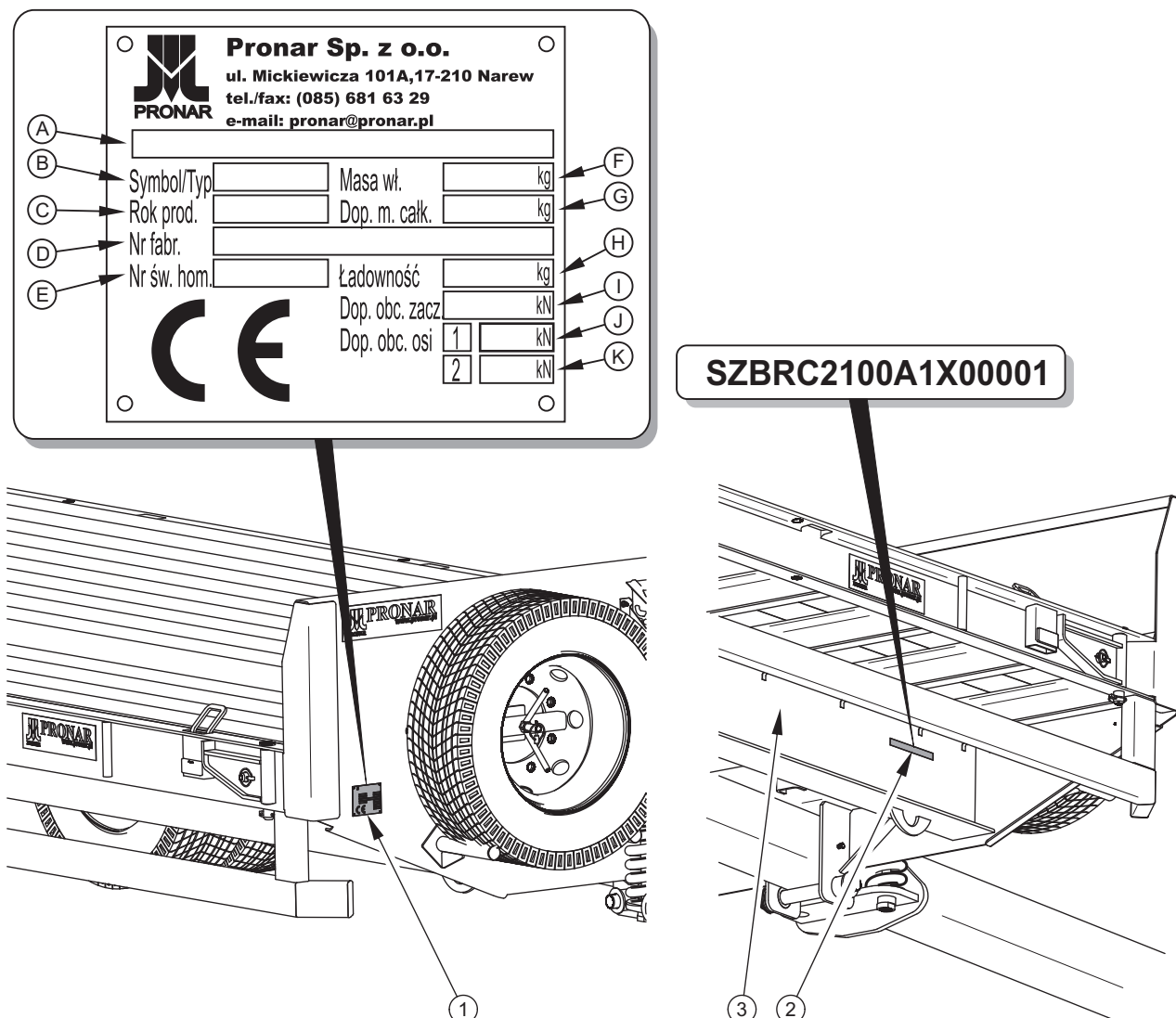
RYSUNEK 1.1 Miejsce umieszczenia tabliczki znamionowej i wybitia numeru seryjnego
