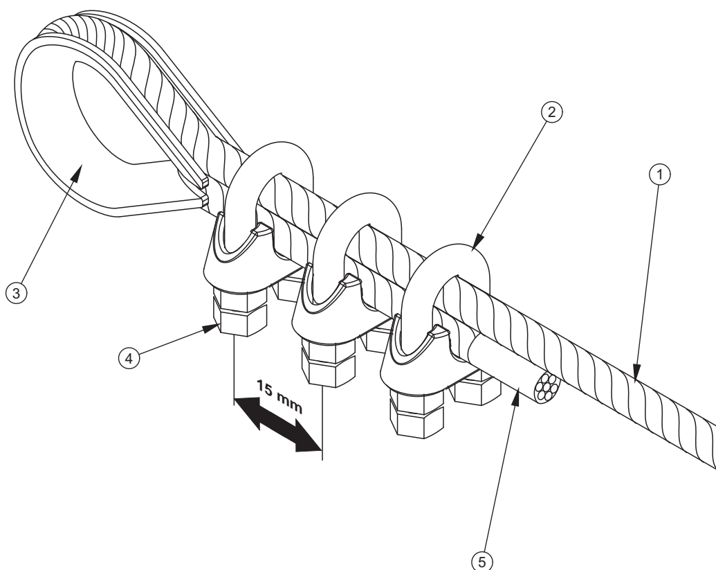
RYСУNEK 5.6 Montaż linki stalowej
