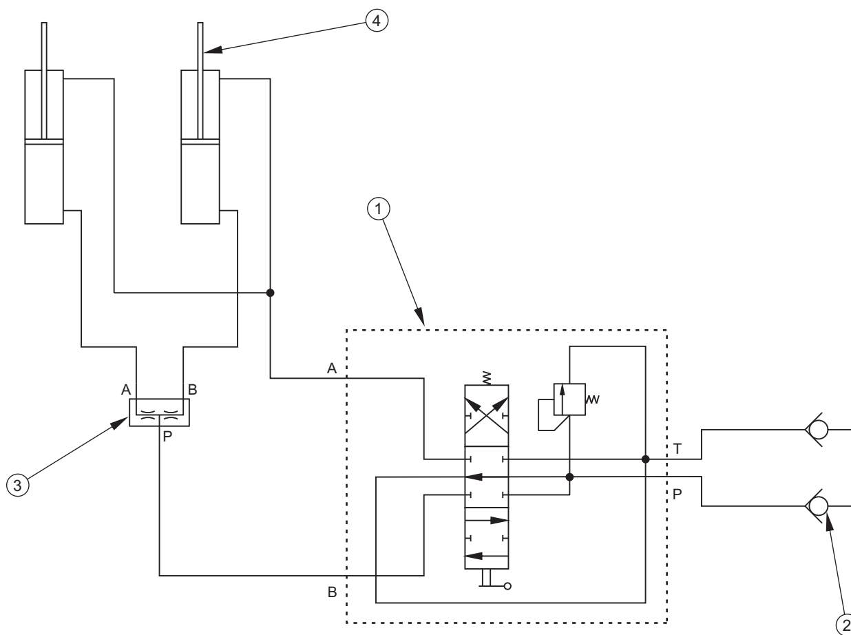
RYСУNEK 3.9 Schemat ideowy instalacji najazdów
