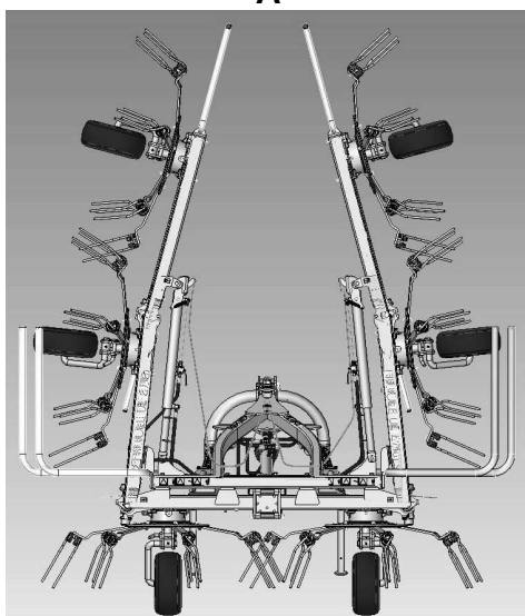
RYСУNEK 4.2A Pozycje przetrzęsacza
