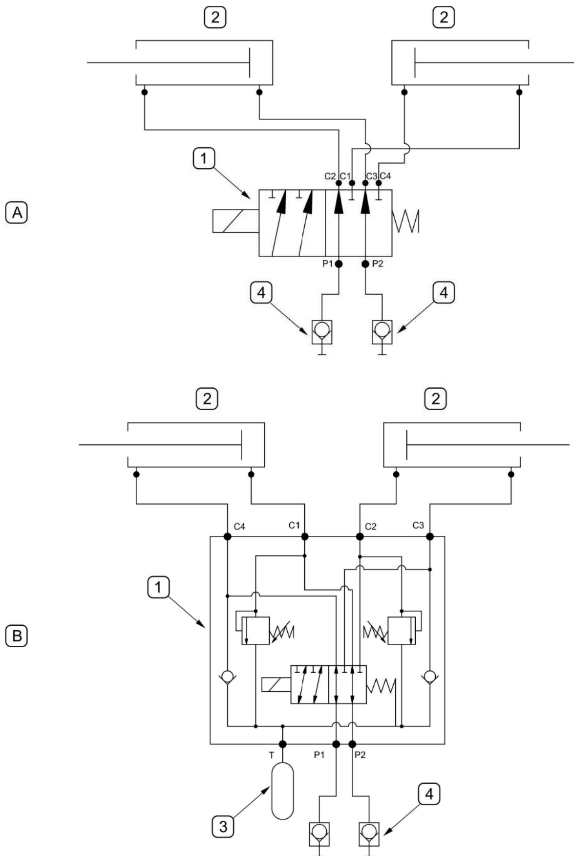
RYSUNEK 3.4 Schemat ideowy instalacji hydraulicznej
