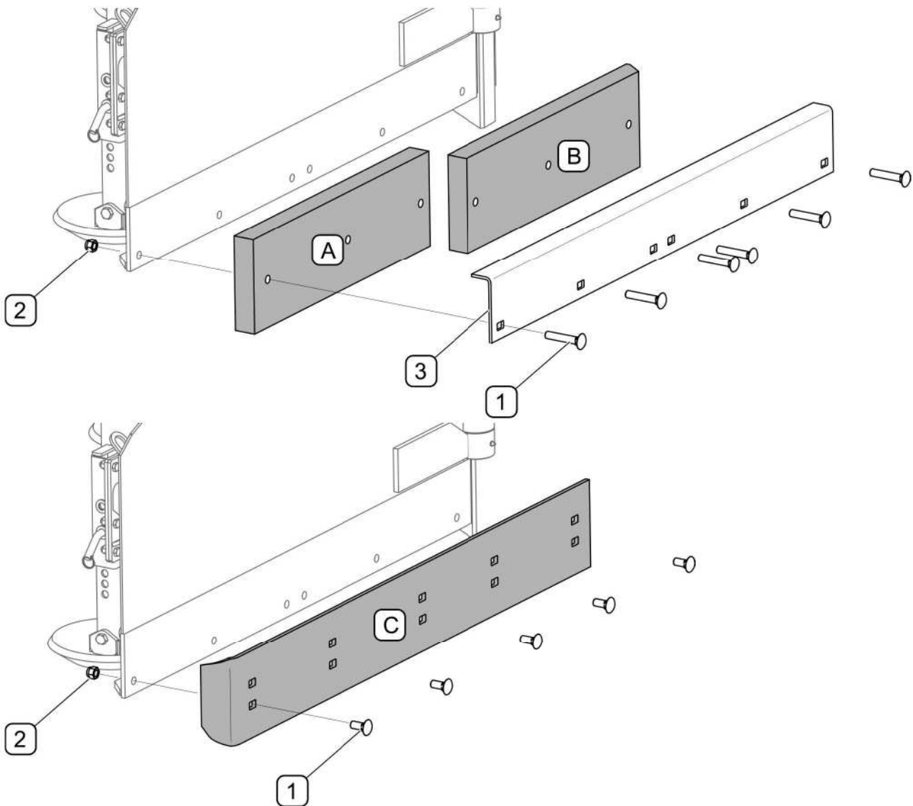
RYСУNEK 5.1 Wymiana listwy zgarniającej
