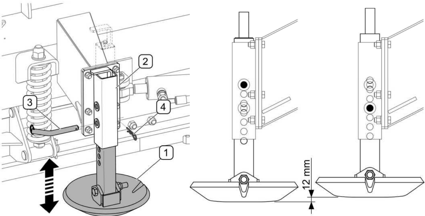
RYSUNEK 4.8 Regulacja wysokości pracy w pługach wyposażonych w ślizgi
