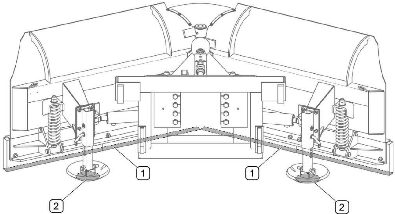
RYСУNEK 4.10 Pozycja pługa po odłączeniu od nośnika
