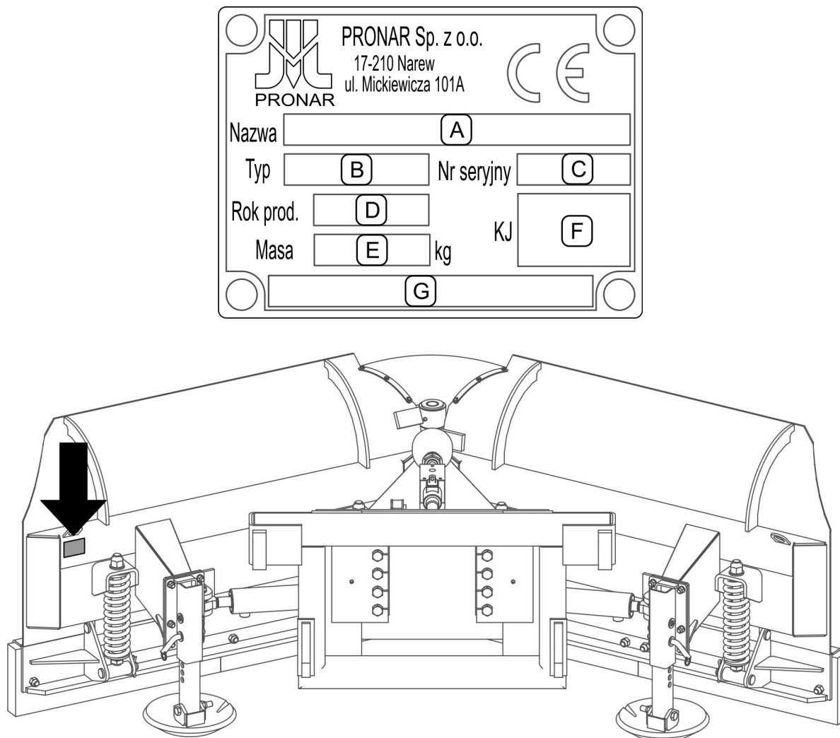
РИСУНОК 1.1 Размещение заводского щитка
