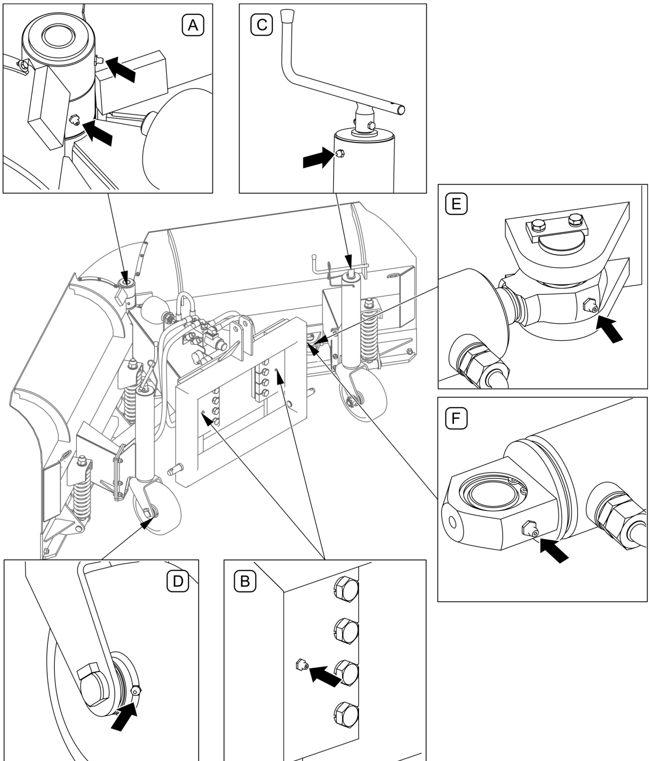
РИСУНОК 5.3 Точки смазки
