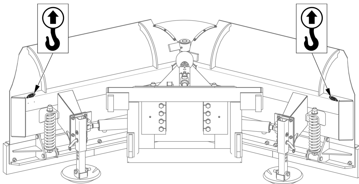
РИСУНОК 1.2 Транспортные захваты
