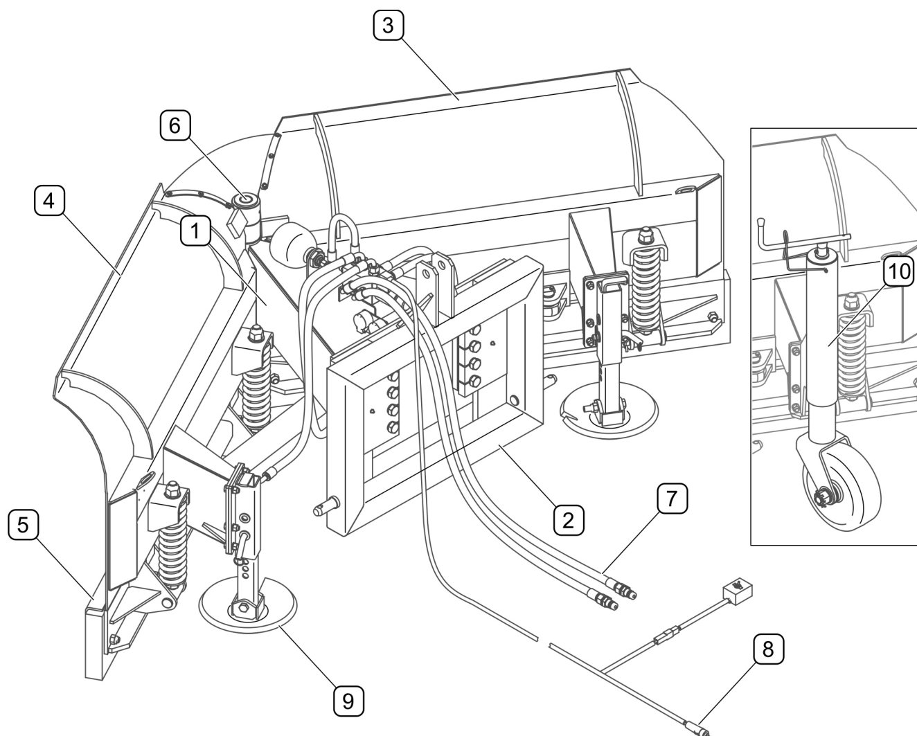
РИСУНОК 3.2 Общее устройство
