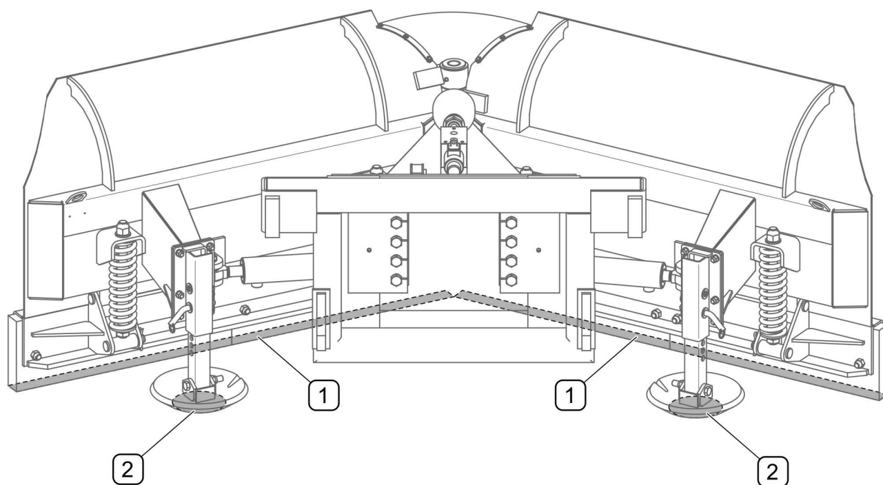
РИСУНОК 4.10 Положение плуга после отсоединения от транспортного средства
