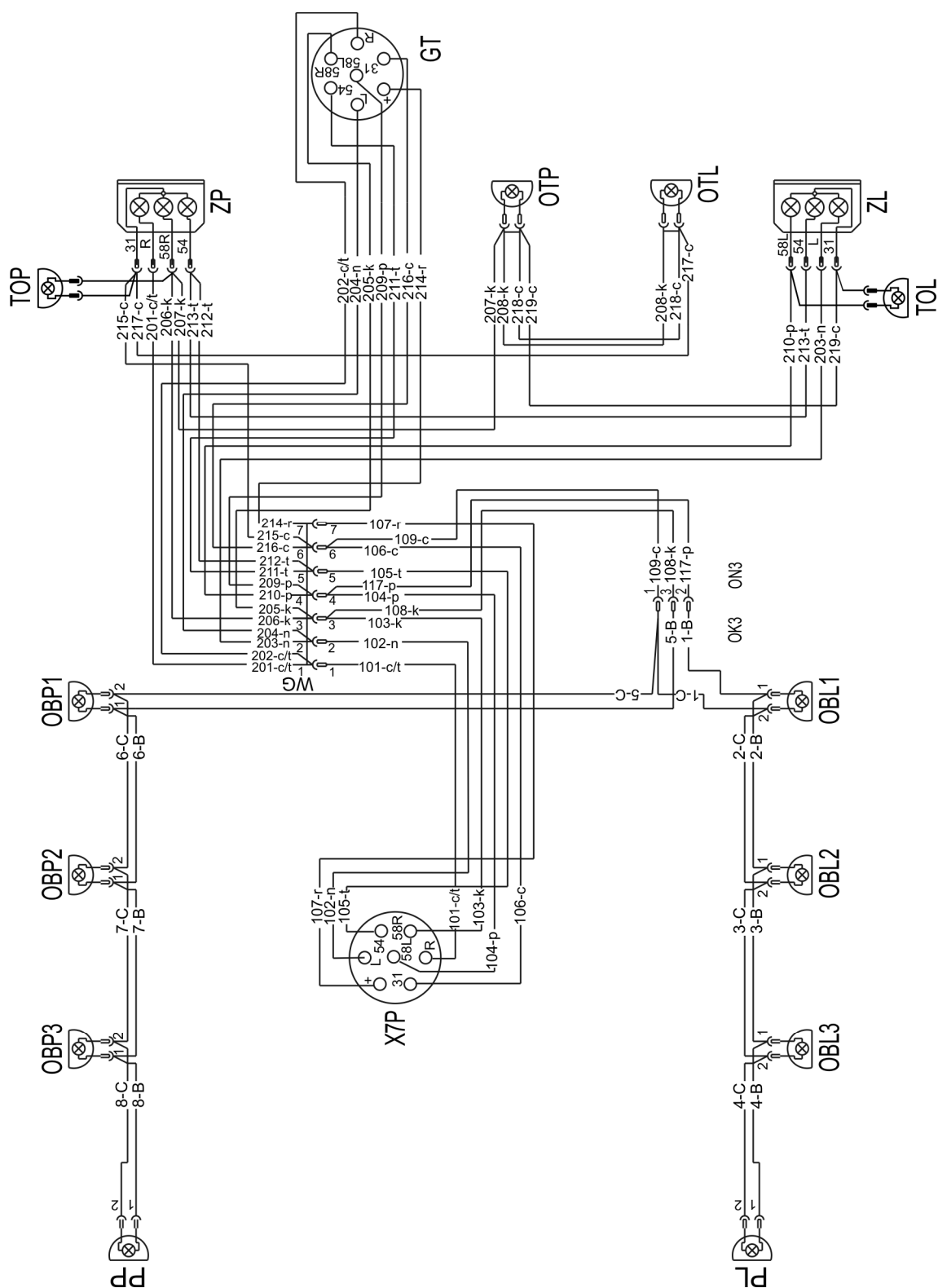
Obrázek 3.12 Ideové schéma elektroinstalace
