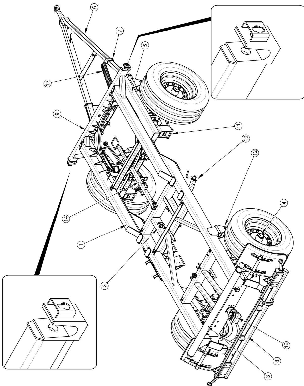
Obrázek 3.1 Podvozek přívěsu
