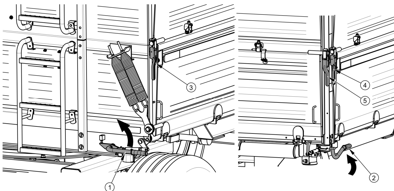
Obrázek 4.3 Otevírání bočnic
