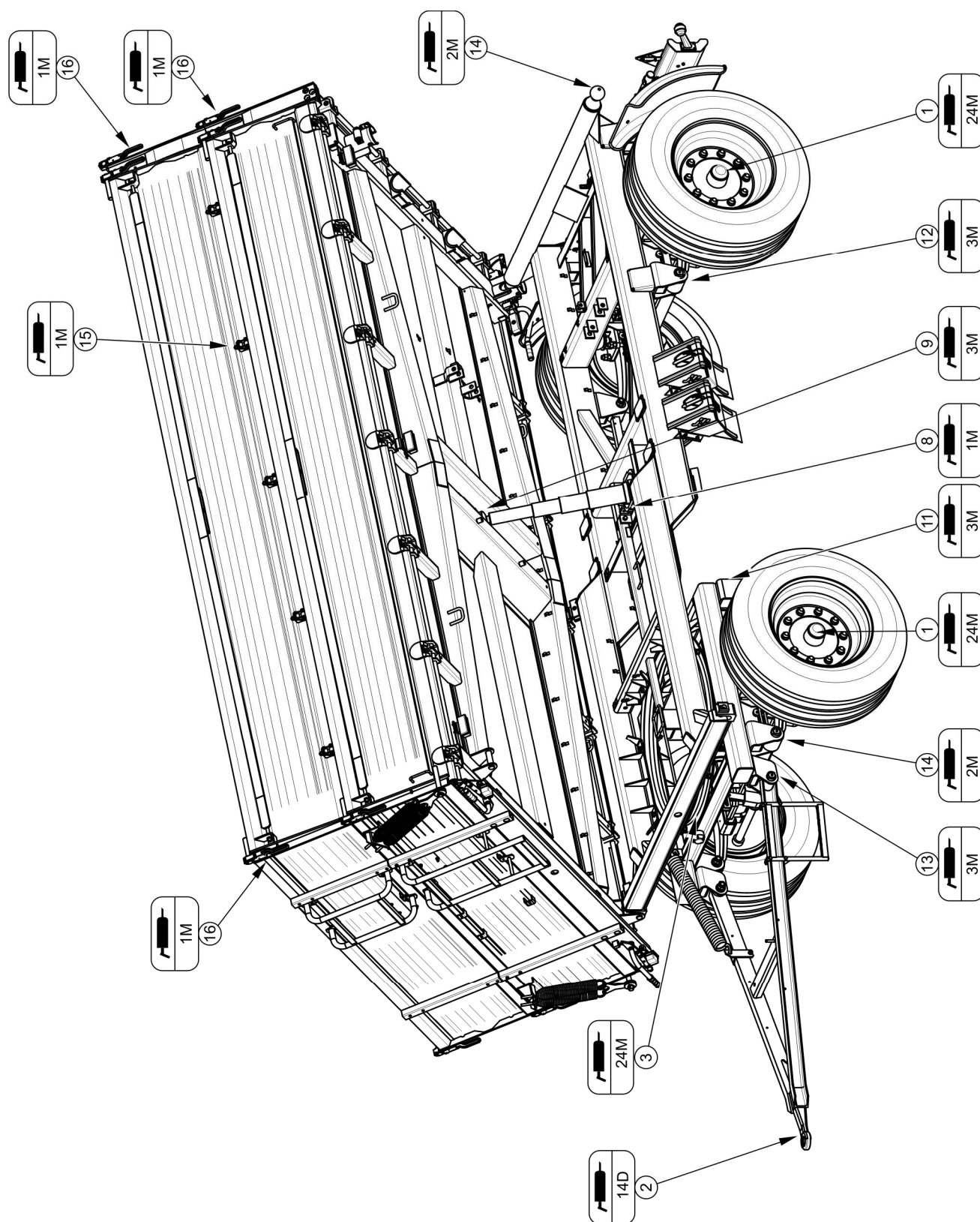
Obrázek 5.11 Mazací body přívěsu, část 1
