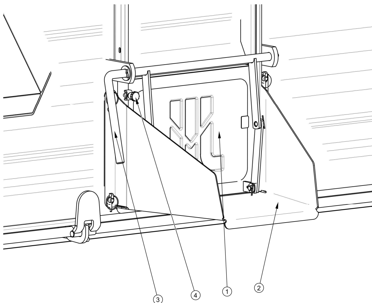
Obrázek 4.4 Skluz
