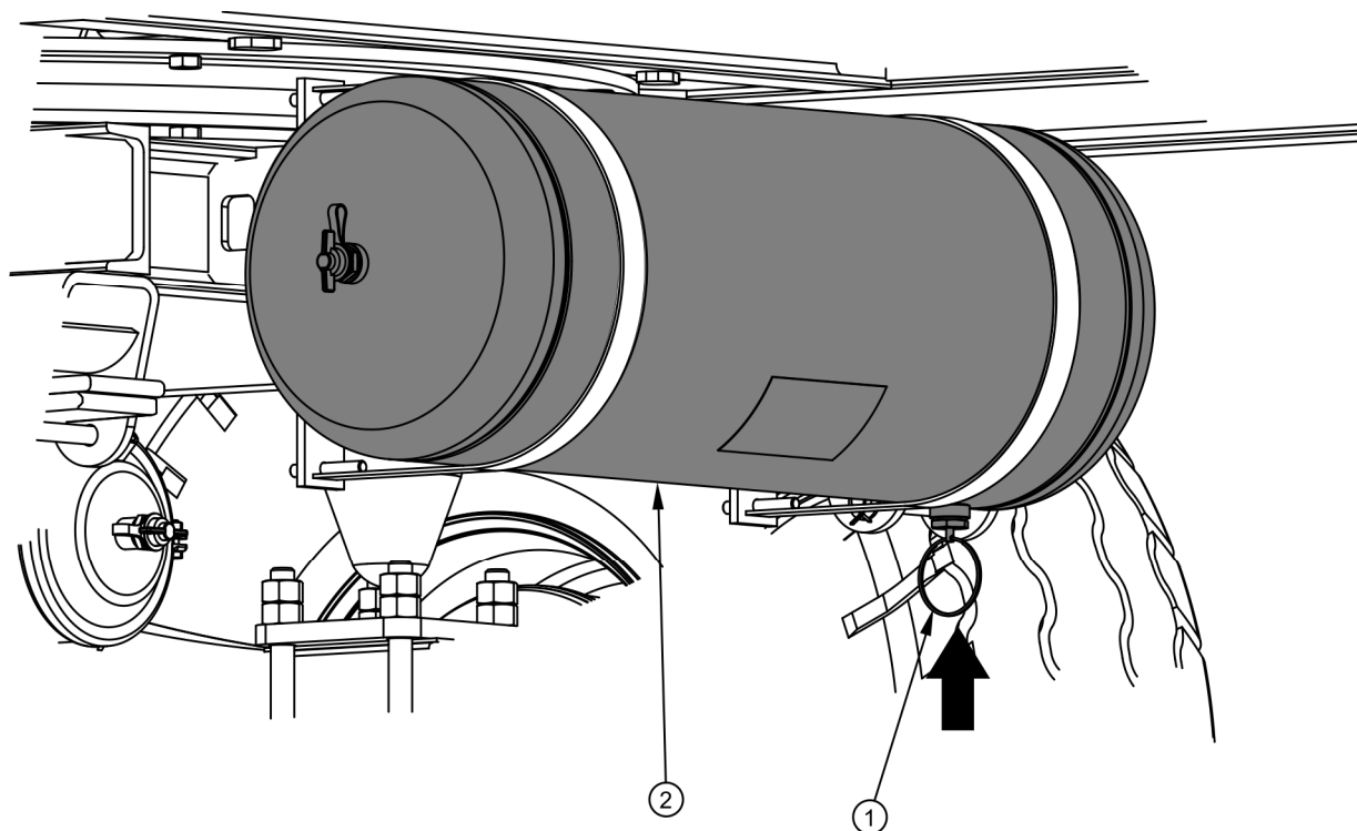
Obrázek 5.9 Odvodňování vzdušníku
