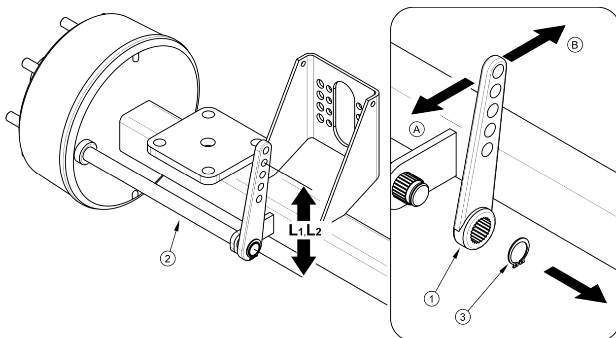
Obrázek 5.5 Seřízení mechanických brzd jezdových náprav
