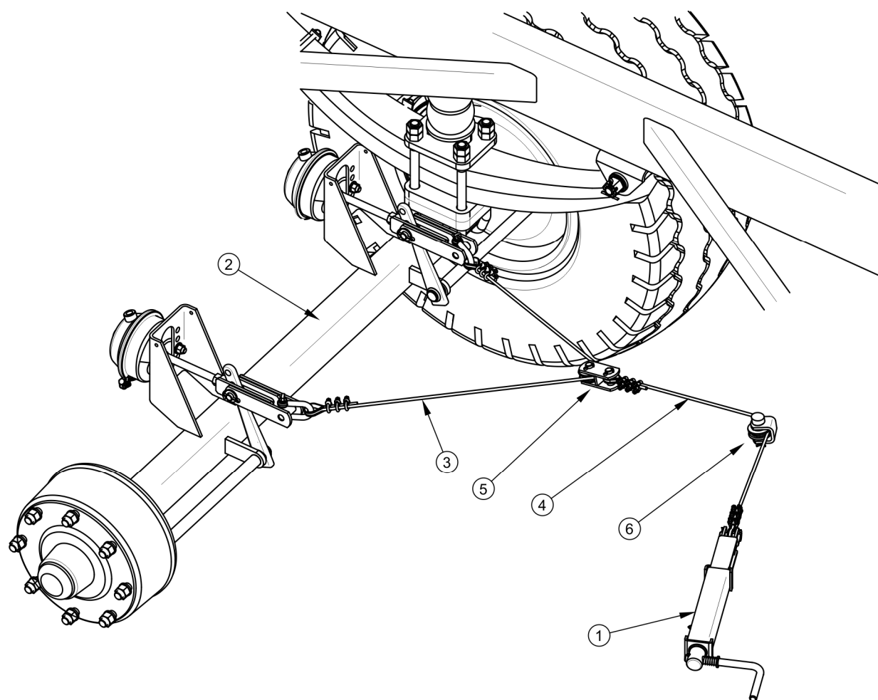
Obrázek 3.10 Konstrukce parkovací brzdy
