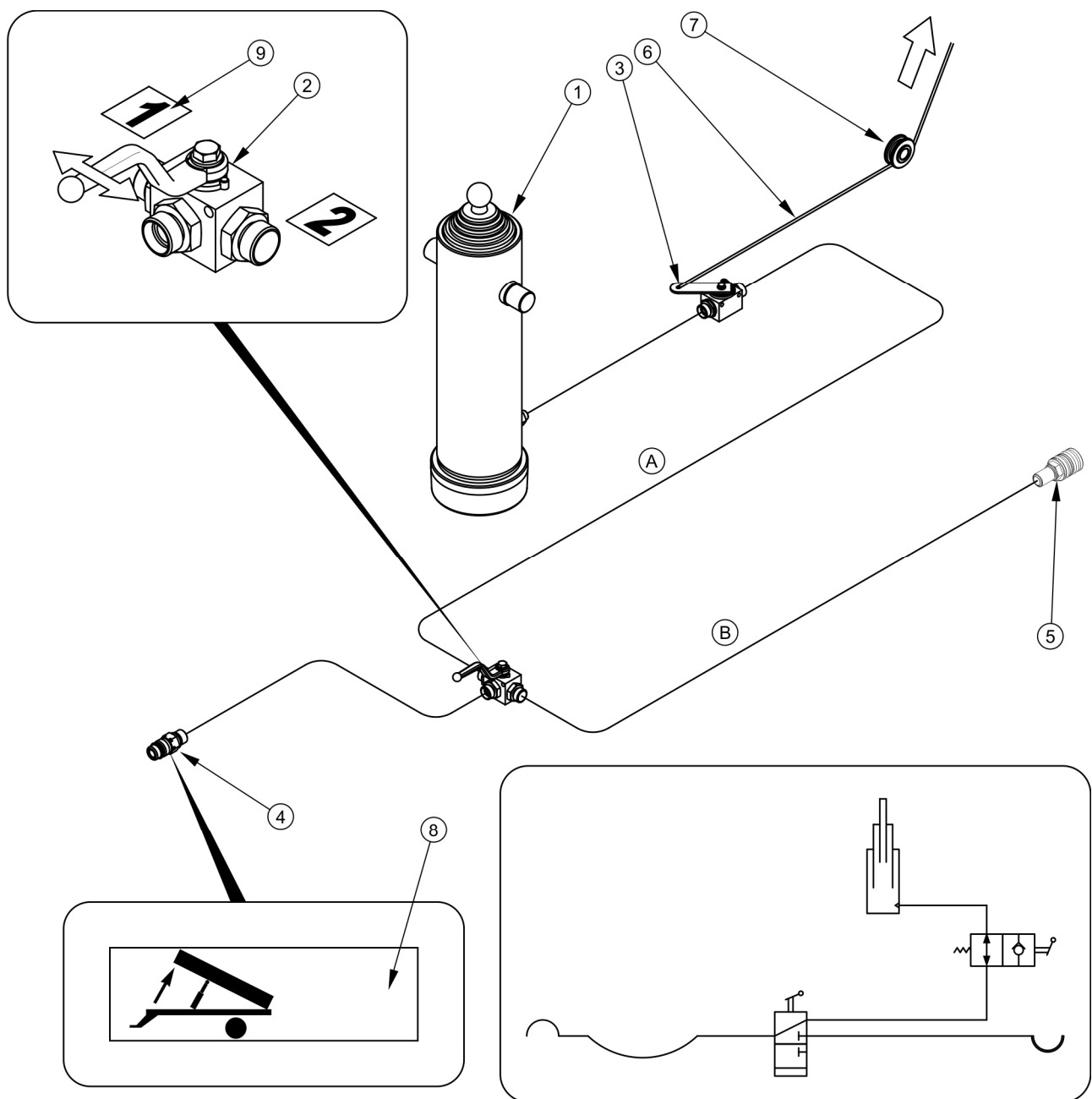
Obrázek 3.9 Konstrukce a schéma hydraulické instalace sklápění
