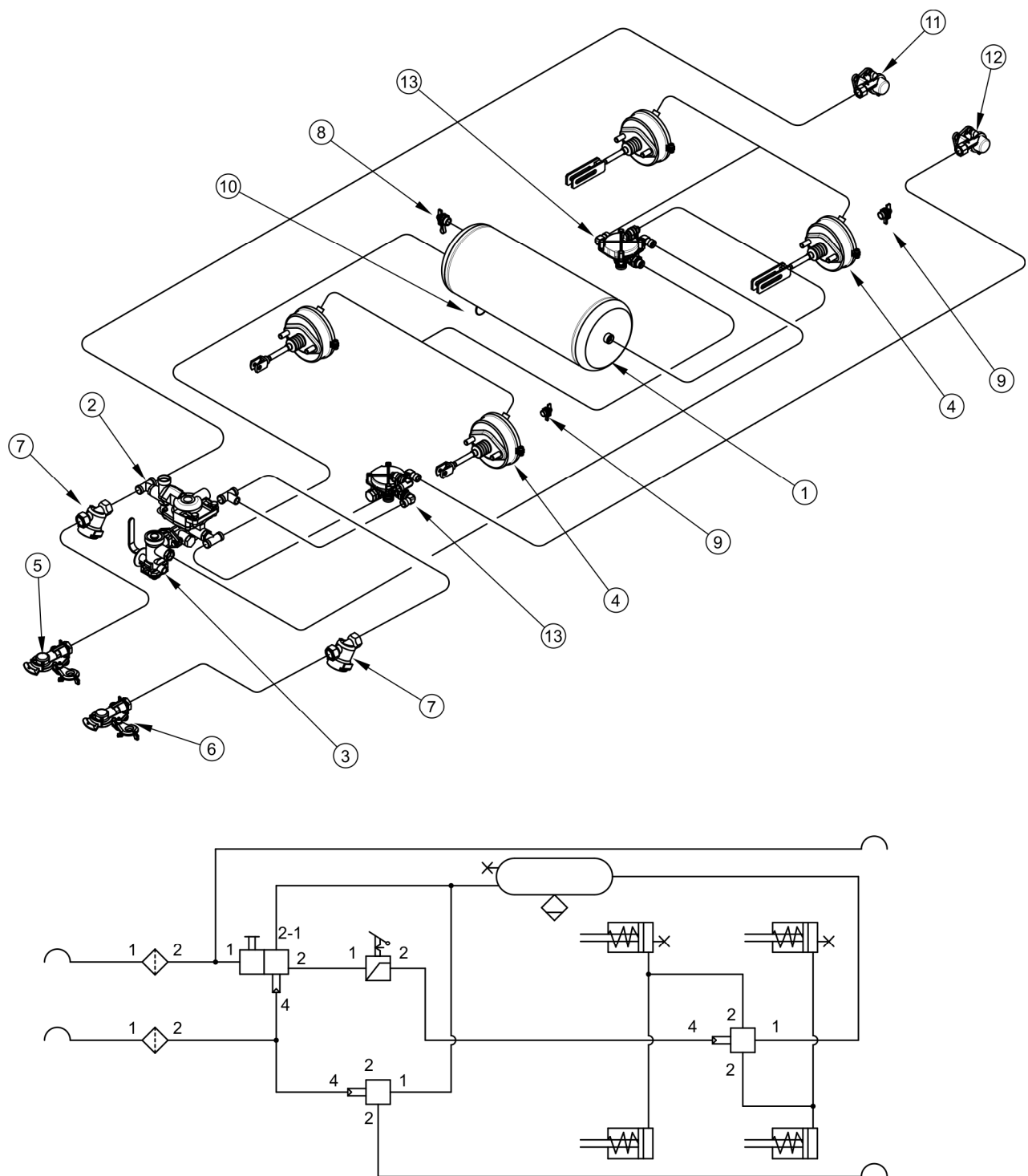
Obrázek 3.5 Konstrukce a schéma vzduchové brzdové dvouhadicové instalace
