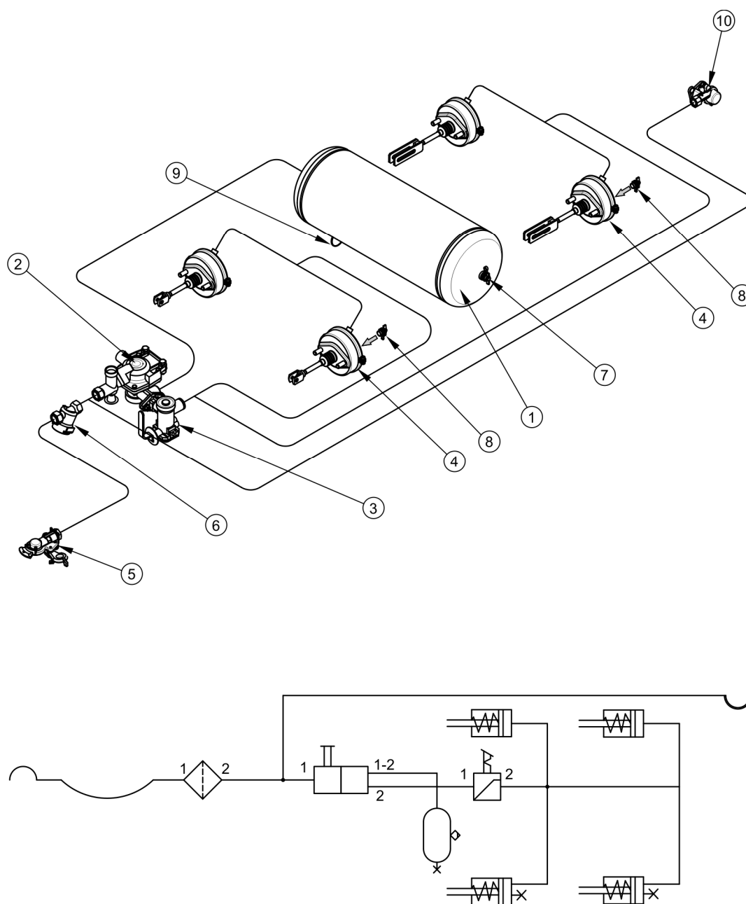
Obrázek 3.6 Konstrukce a schéma vzduchové jednohadicové brzdové instalace
