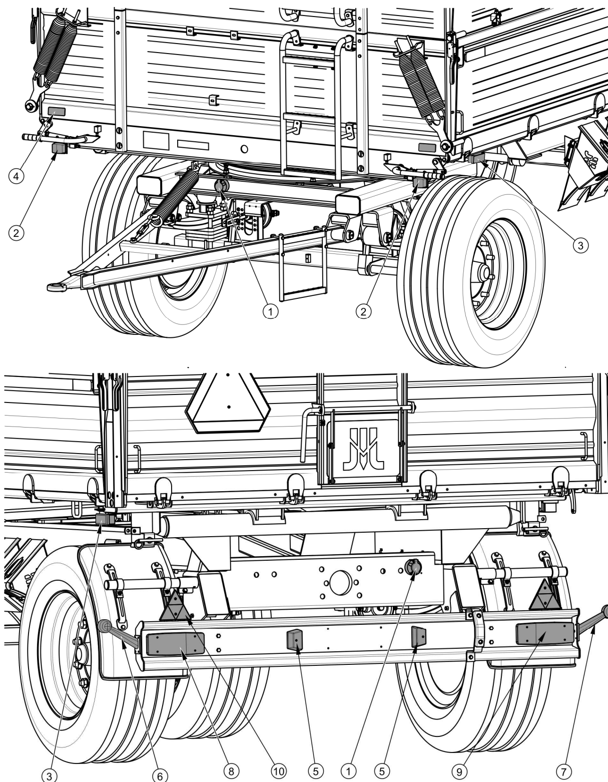
Obrázek 3.11 Rozmístění elektrických a odrazových prvků
