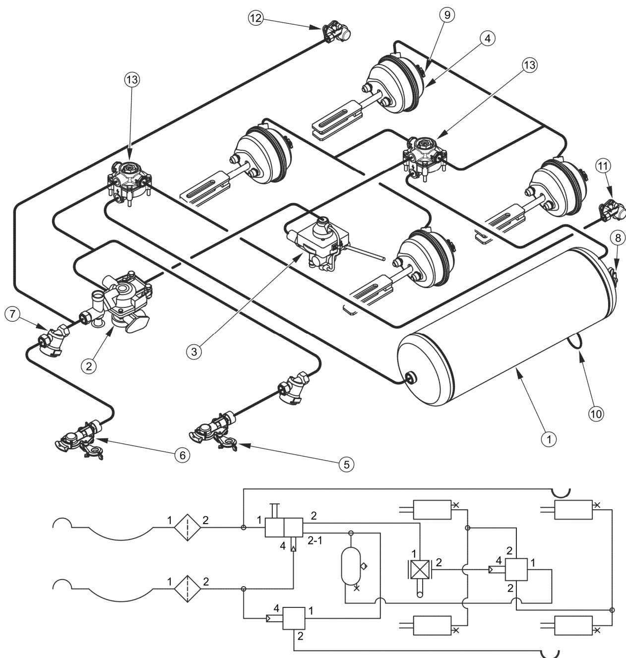
РИСУНОК 3.6 Устройство и схема двухпроводной пневматической тормозной системы с автоматическим регулятором силы торможения
