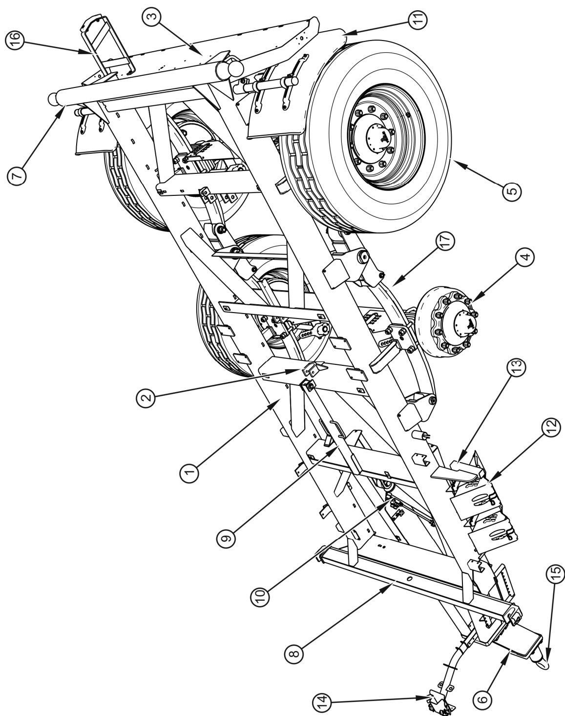
РИСУНОК 3.1 Шасси прицепа
