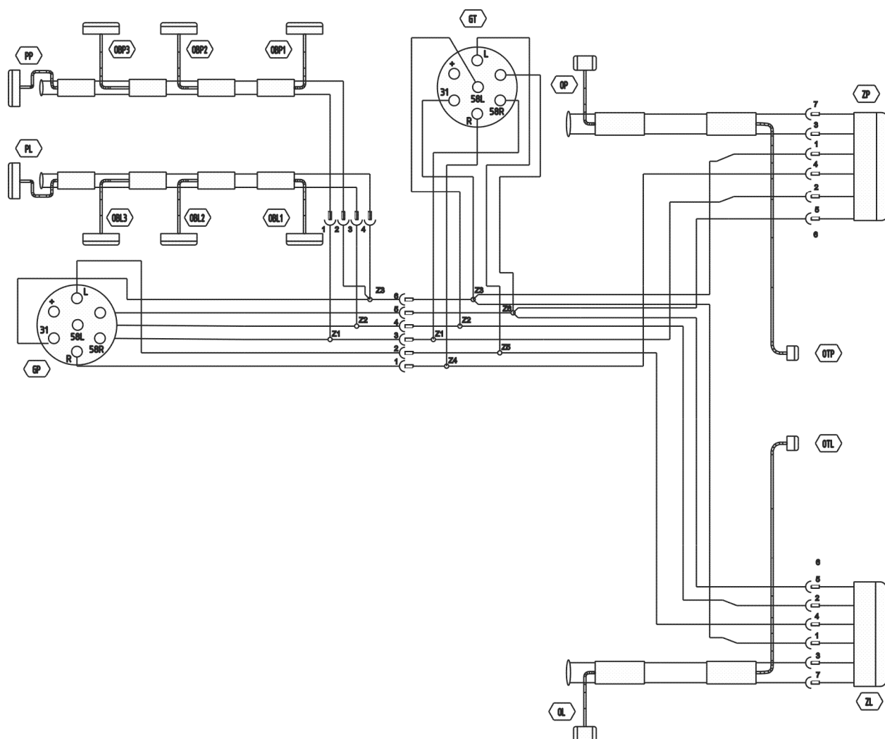
РИСУНОК 3.13 Принципиальная схема электрической системы
