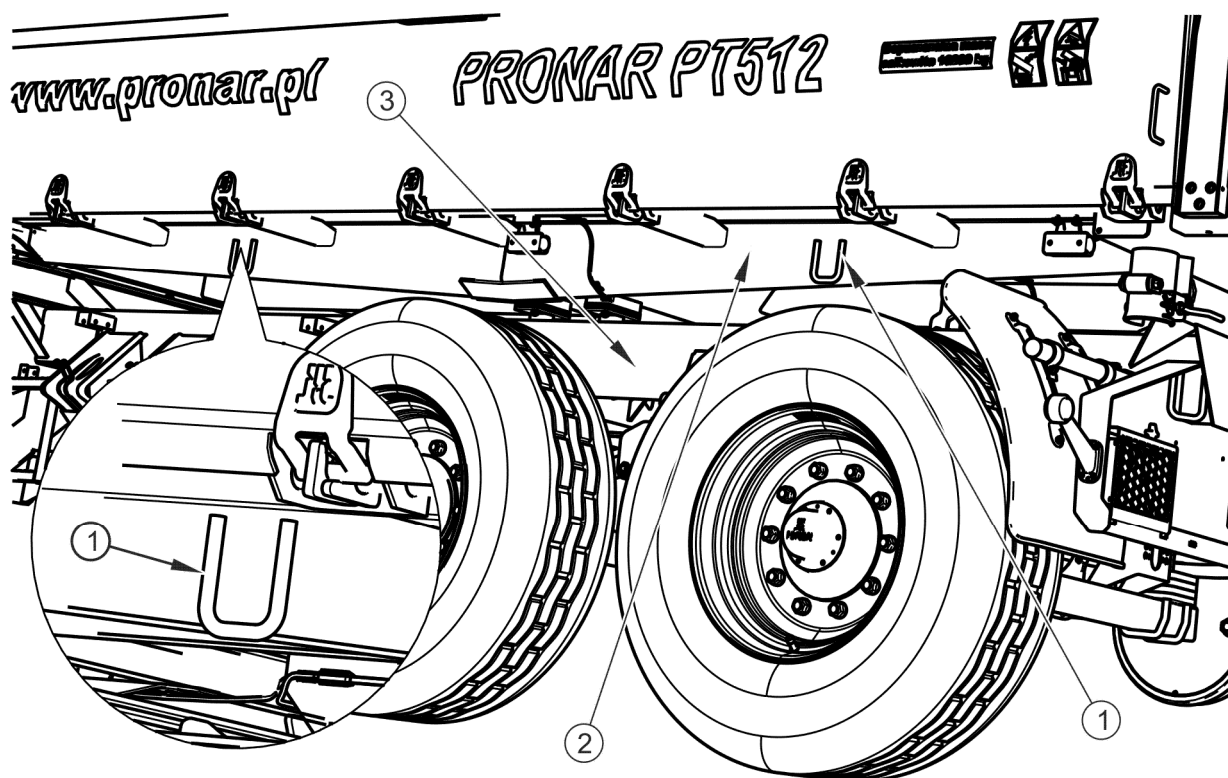
РИСУНОК 1.3 Расположение транспортных захватов
