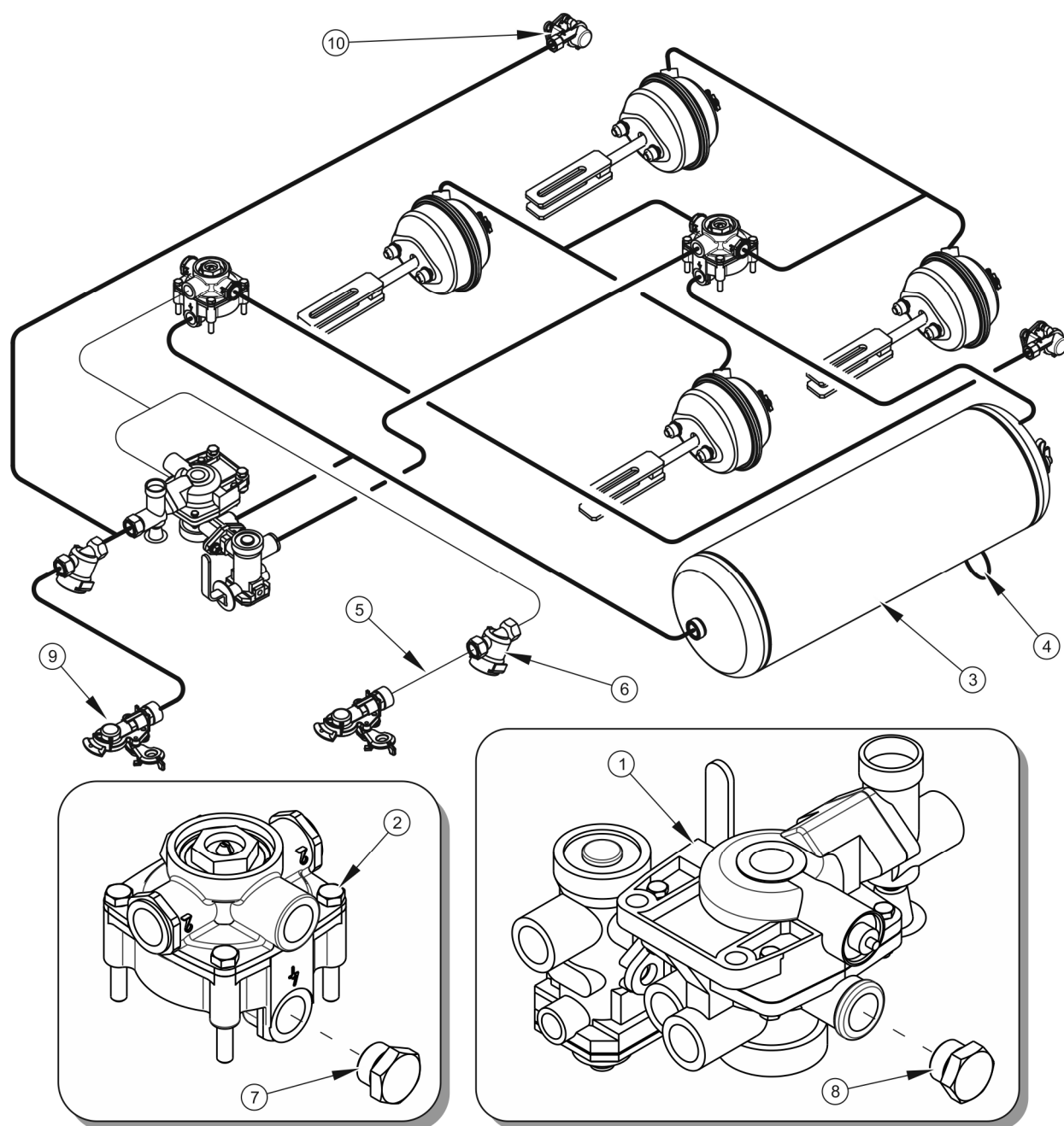
РИСУНОК 5.9 Переоснастка двухпроводной пневматической тормозной системы в однопроводную
