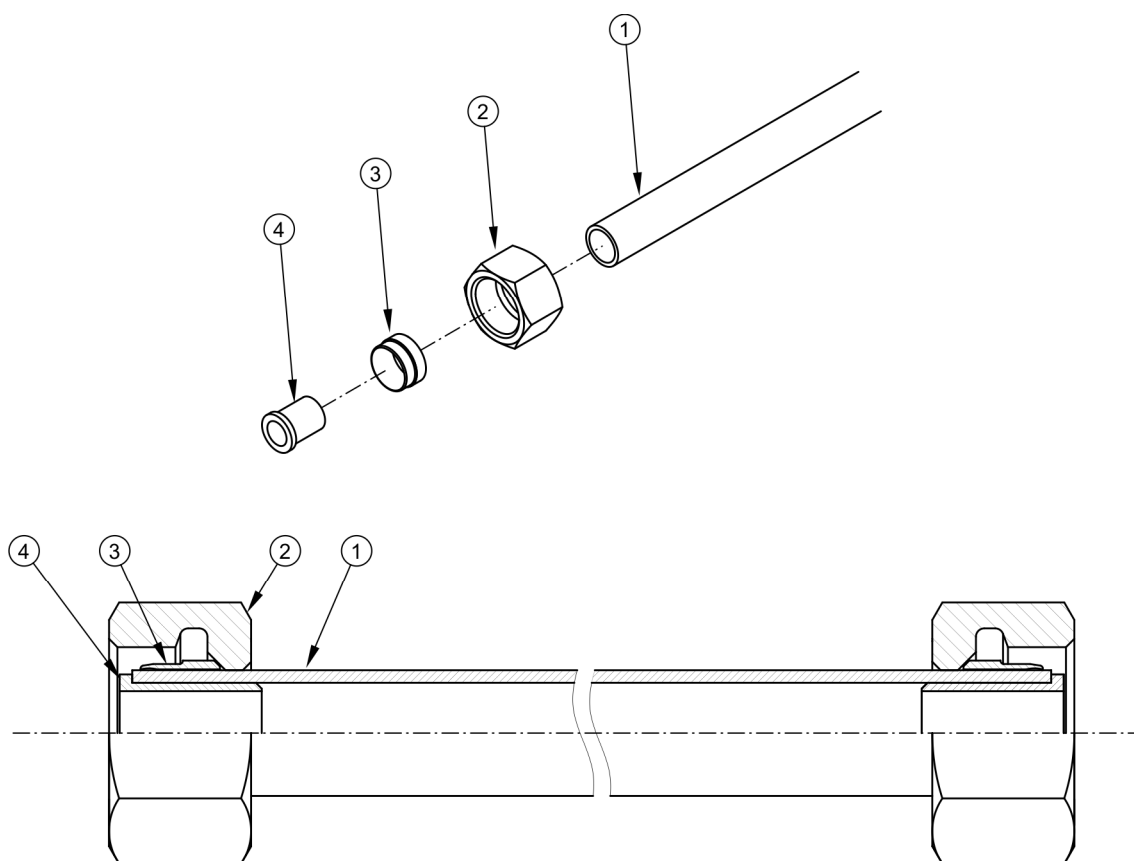
РИСУНОК 5.10 Конструкция пневмопровода
