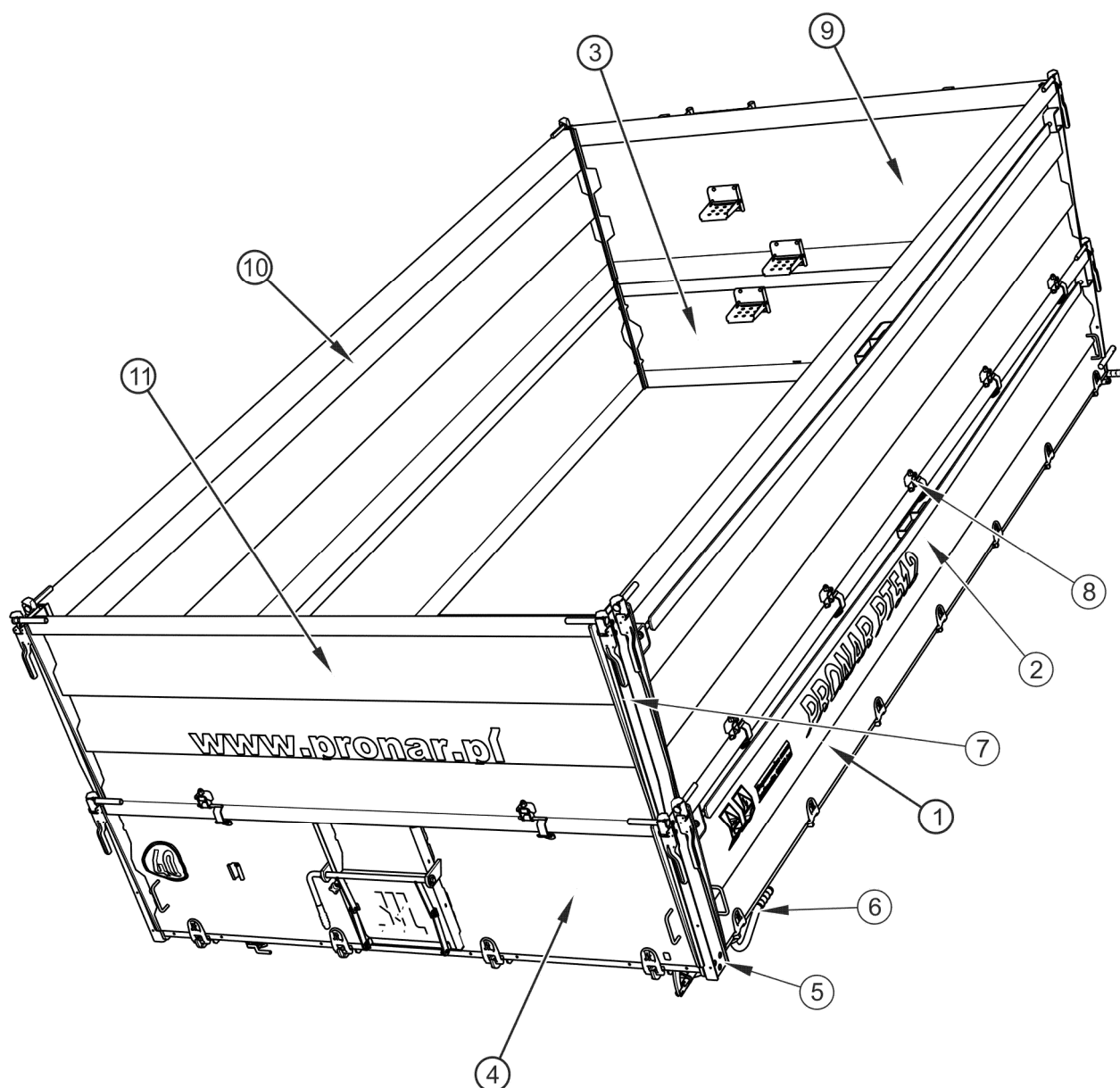
РИСУНОК 3.2 Платформа прицепа - вид сзади
