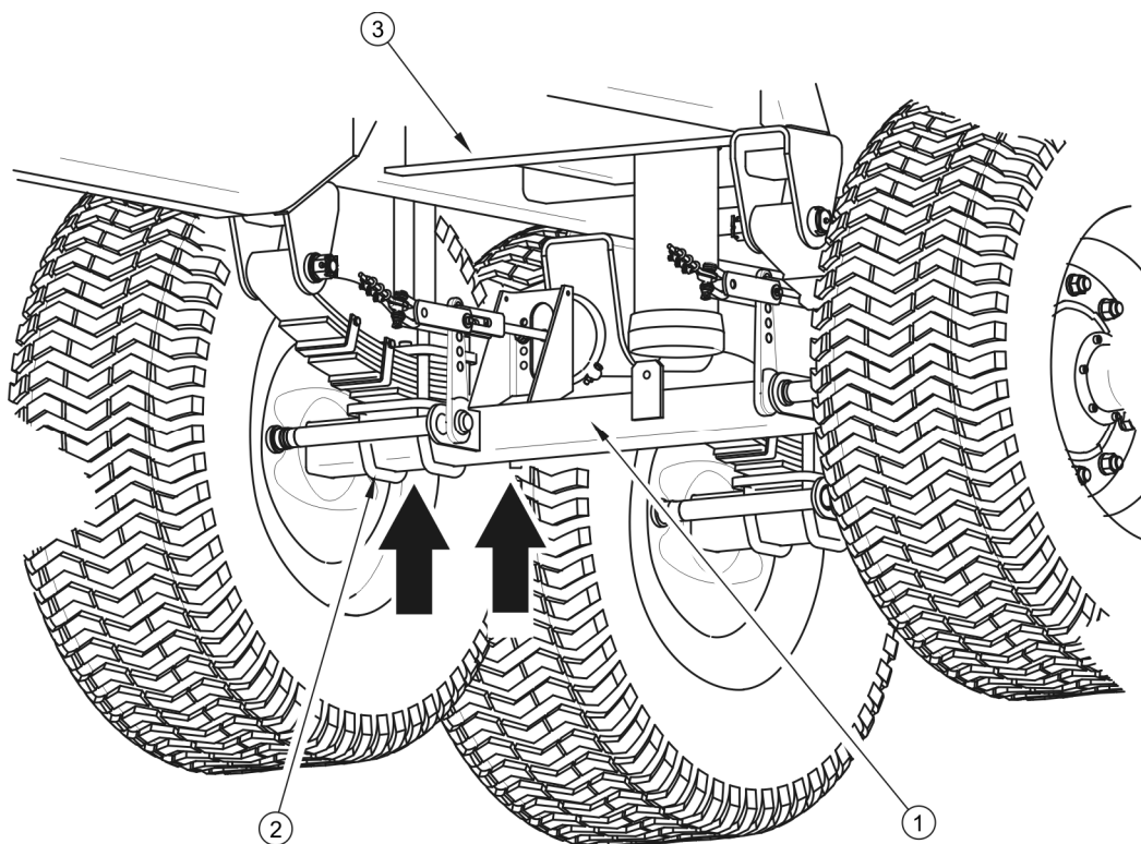
РИСУНОК 5.1 Точка поддомкрачивания
