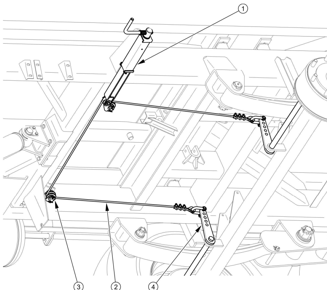
РИСУНОК 3.12 Устройство стояночного тормоза
