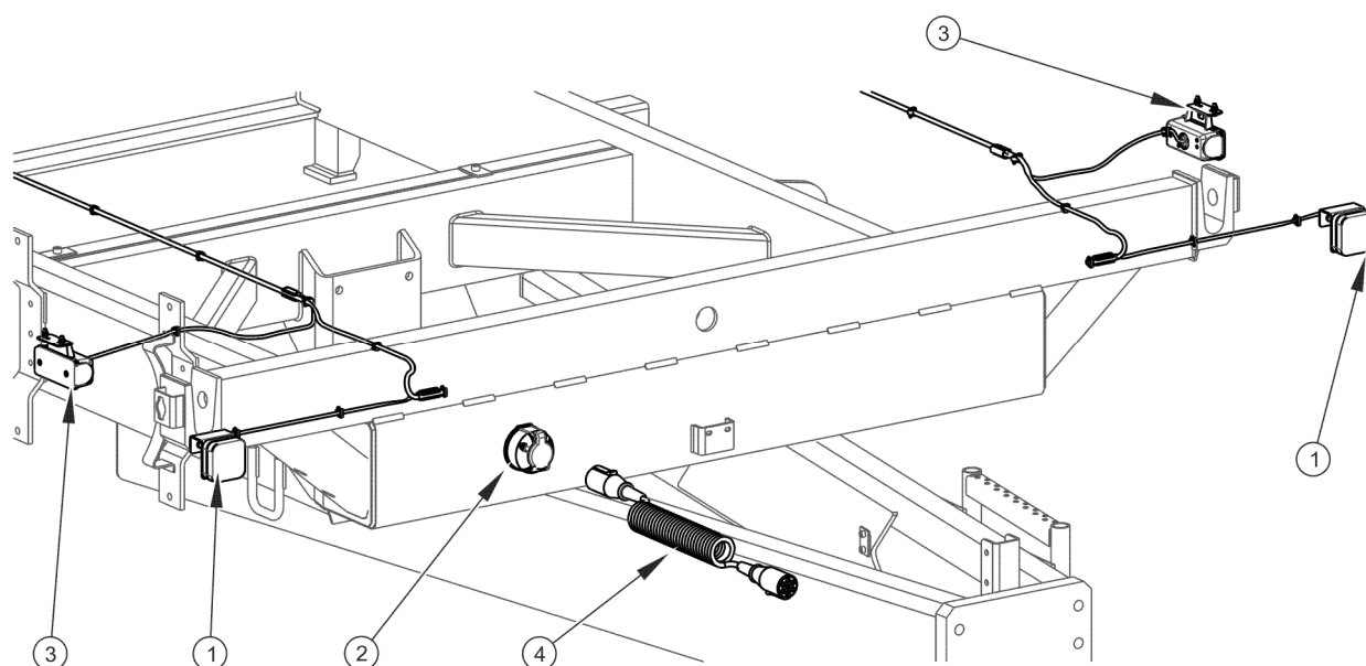
РИСУНОК 3.15 Размещение элементов системы световой сигнализации и катафотов прицепа – вид спереди
