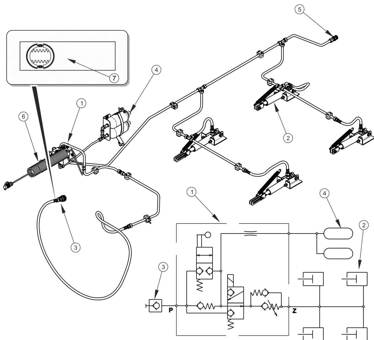
РИСУНОК 3.8 Устройство и схема гидравлической тормозной системы
