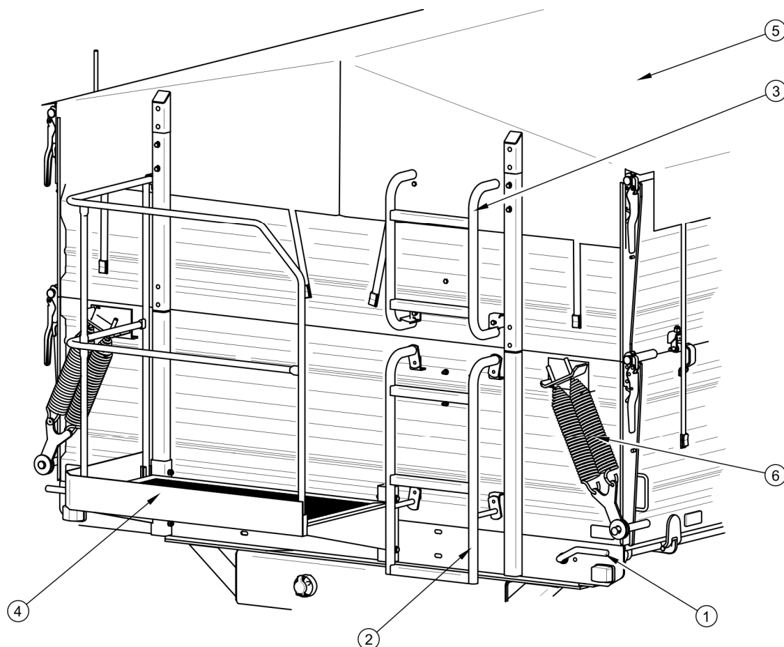
РИСУНОК 3.3 Платформа прицепа - вид спереди
