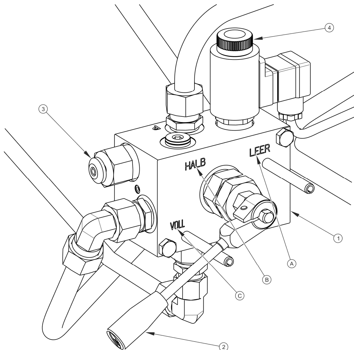
РИСУНОК 3.9 Электрогидравлический тормозной клапан
