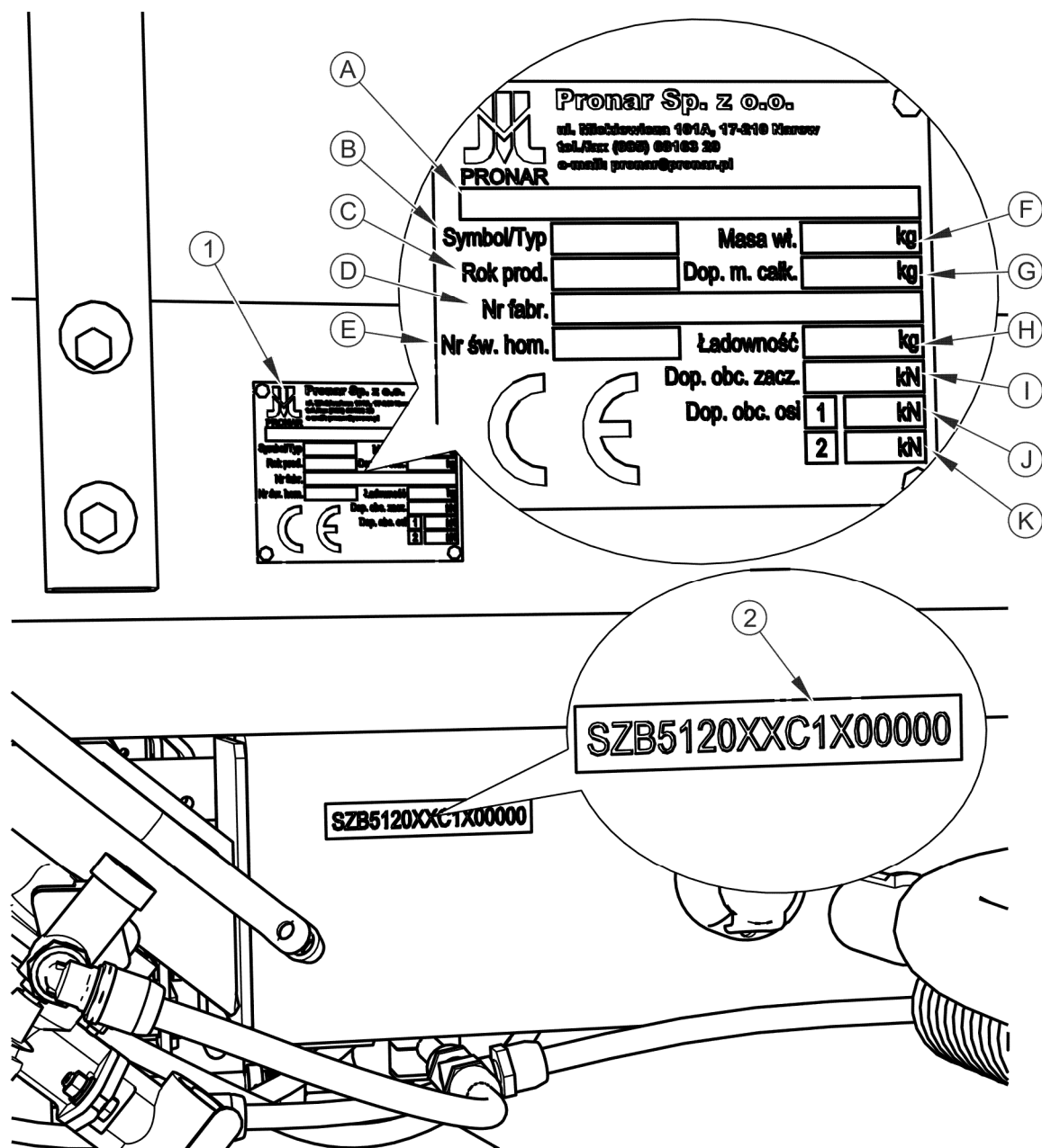
РИСУНОК 1.1 Размещение заводского щитка и заводского номера
