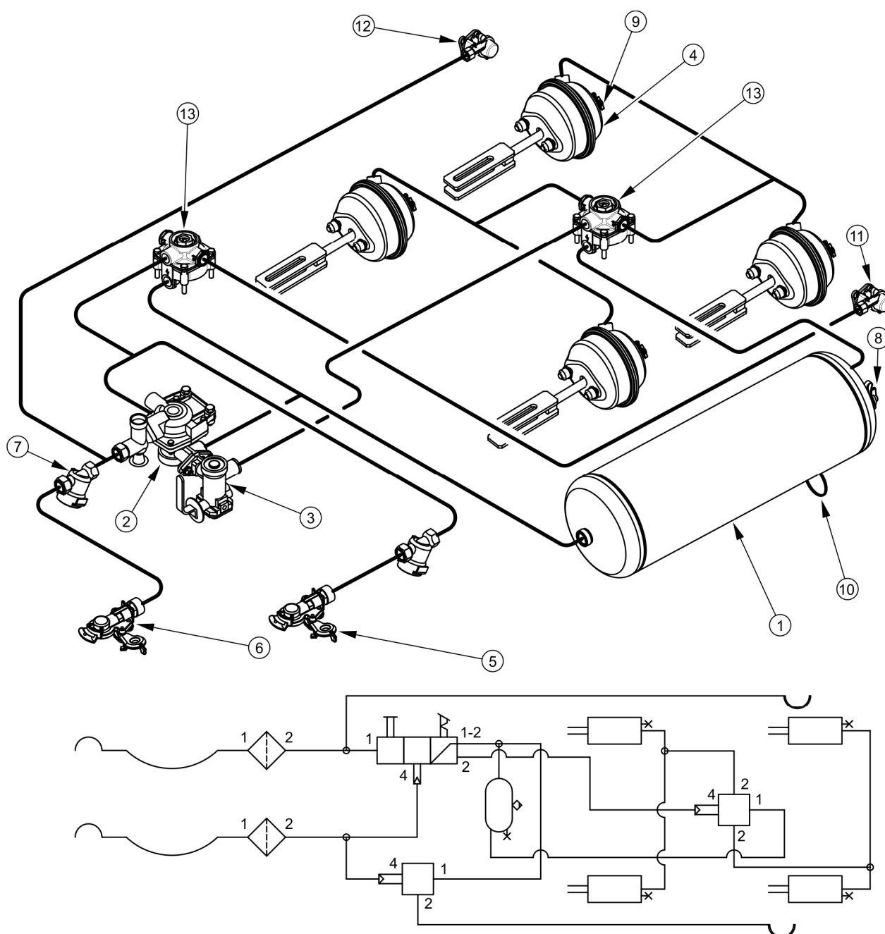
РИСУНОК 3.5 Устройство и схема одно- или двухпроводной пневматической тормозной системы с ручным регулятором силы торможения
