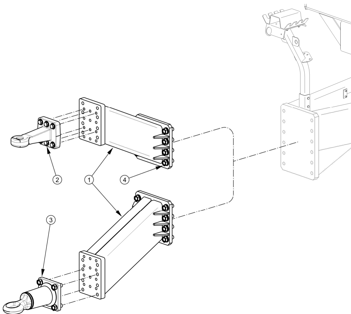
РИСУНОК 5.15 Регулирование положения дышла
