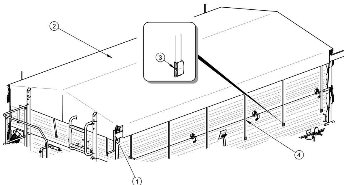
РИСУНОК 4.3 Тент
