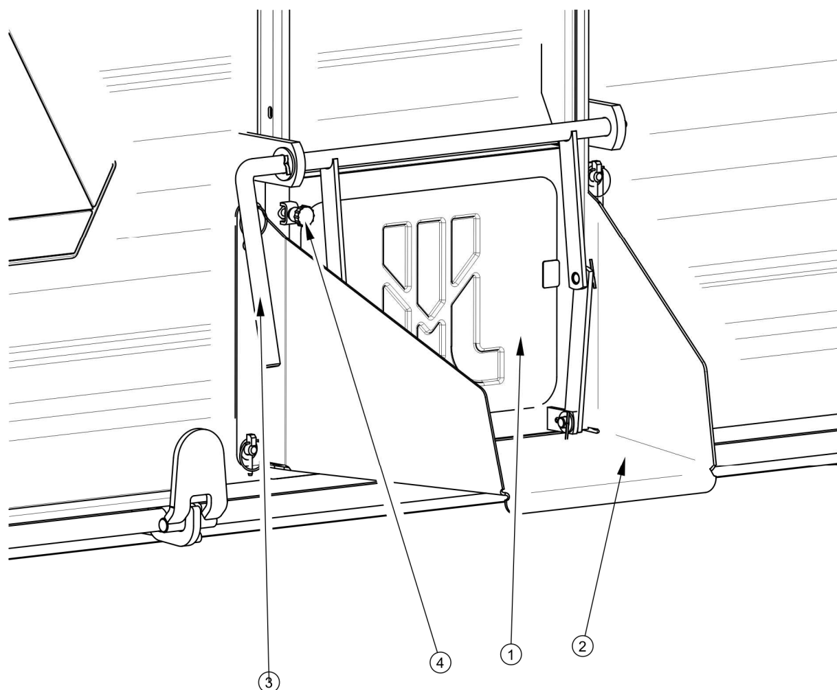
РИСУНОК 4.6 Разгрузочный люк
