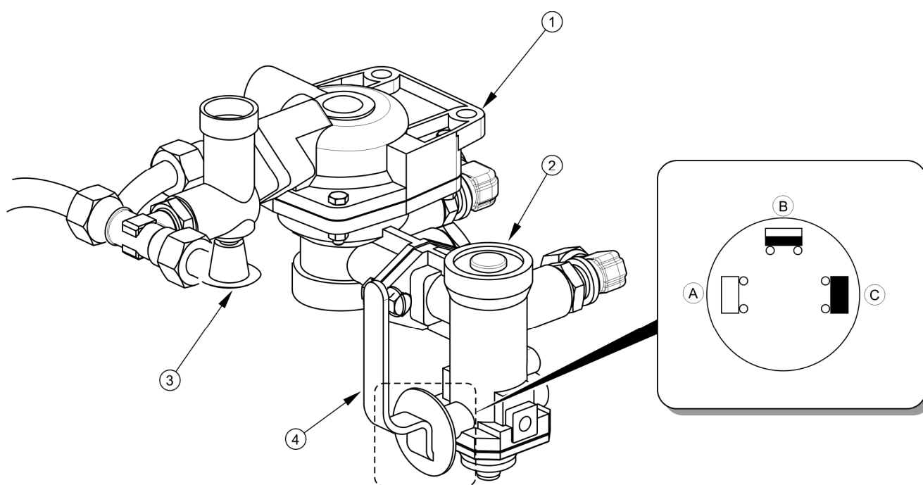
РИСУНОК 3.7 Управляющий клапан и регулятор силы торможения
