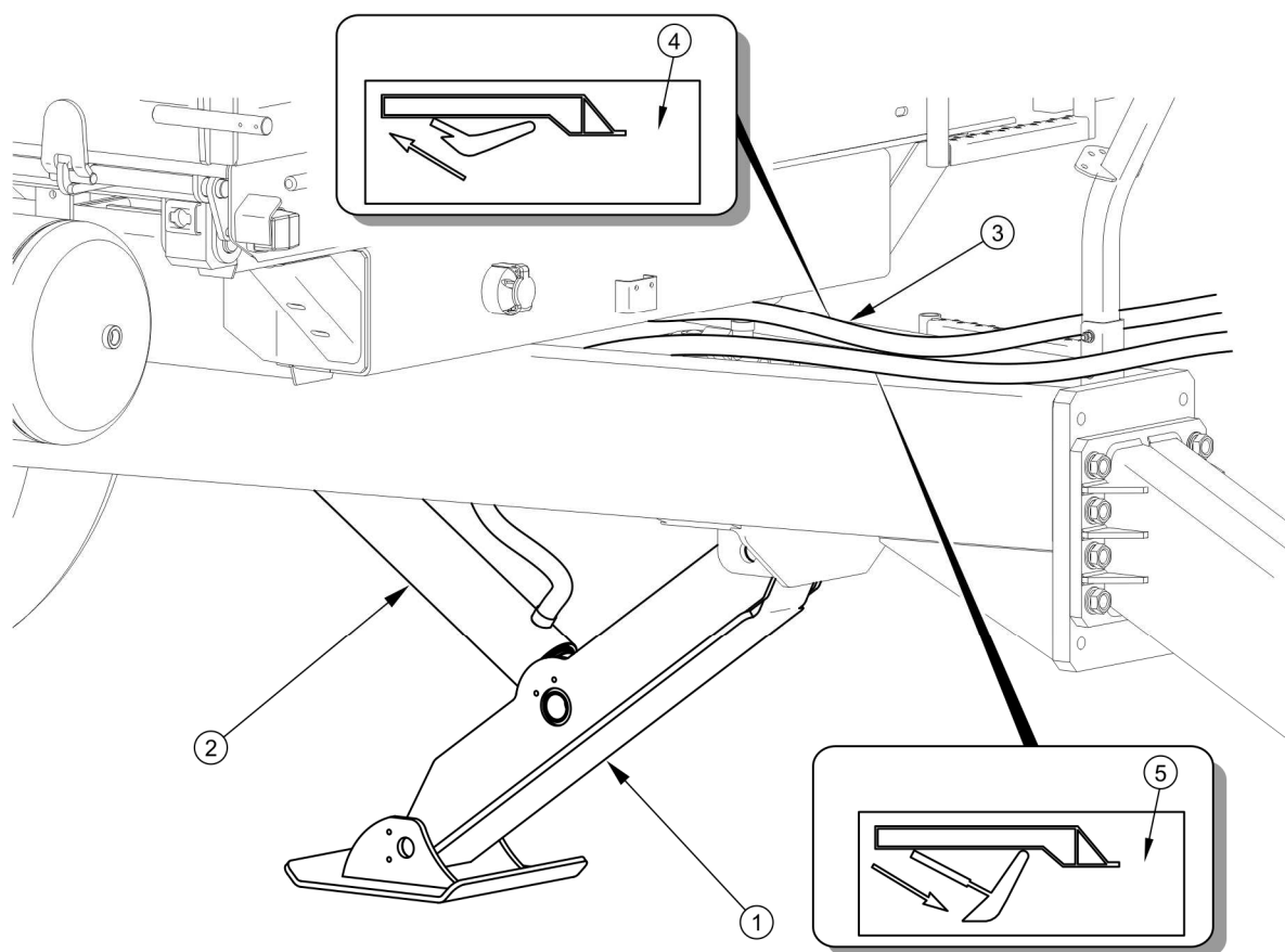
РИСУНОК 4.1 Опора прицепа
