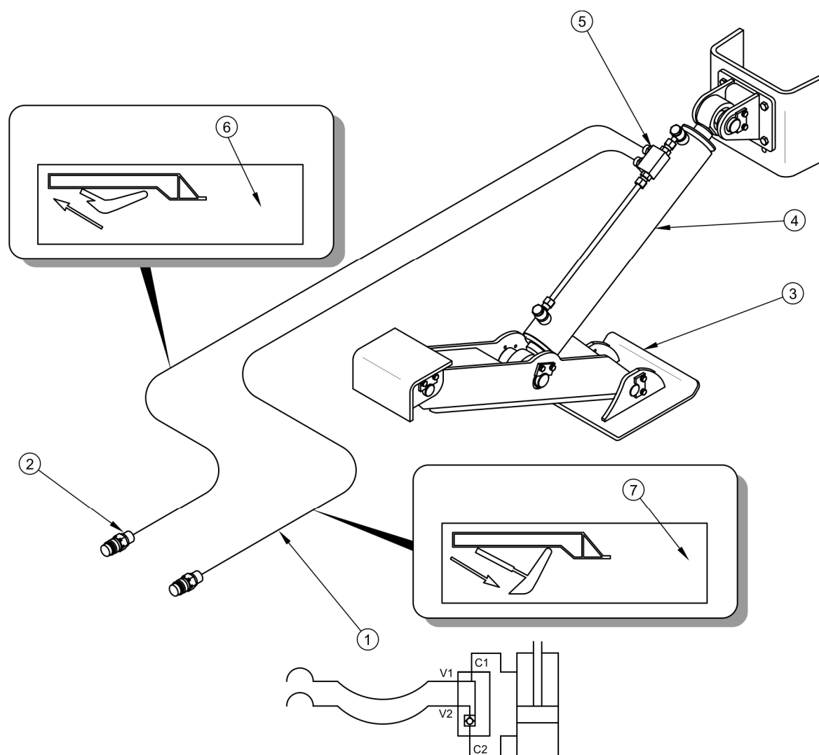
РИСУНОК 3.11 Устройство и схема гидравлической системы ножевой опоры
