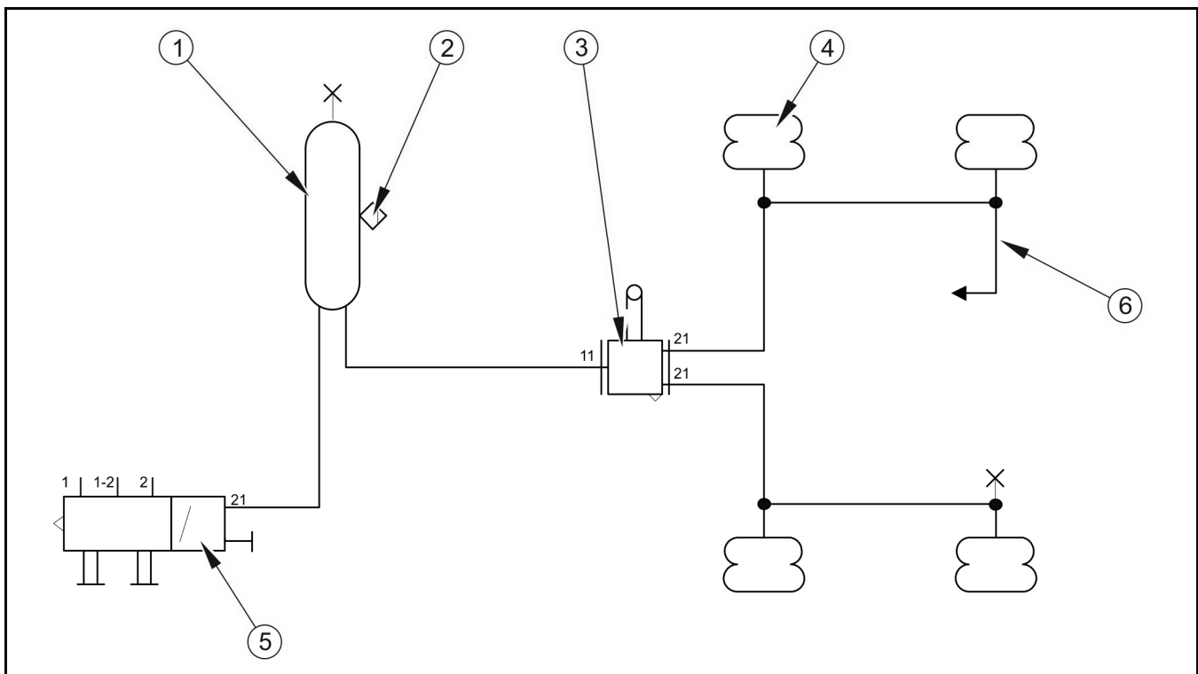
RYSUNEK 3.20 Schemat ideowy instalacji pneumatycznej zawieszania
