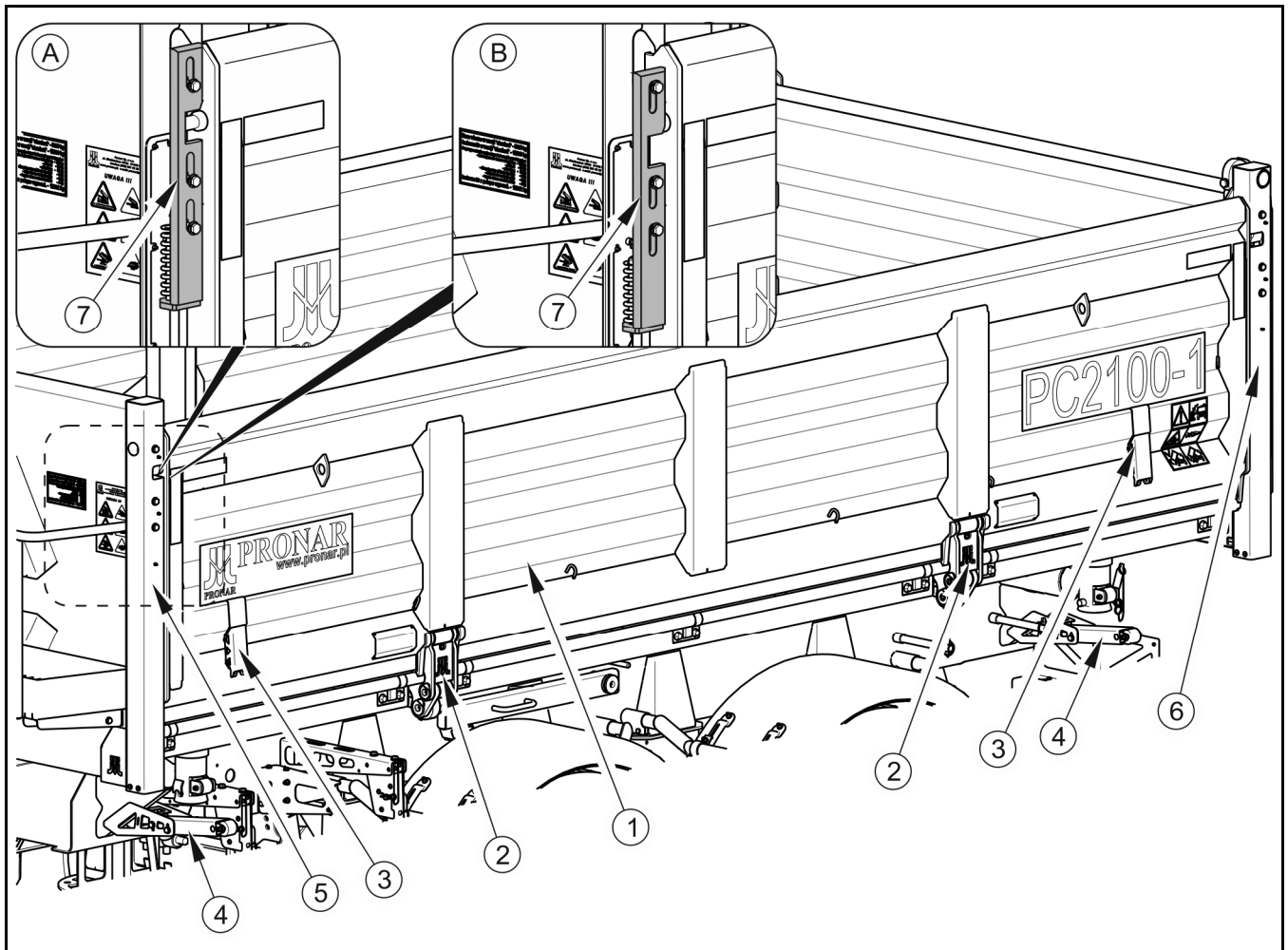
RYSUNEK 3.11 Budowa burty hydraulicznej
