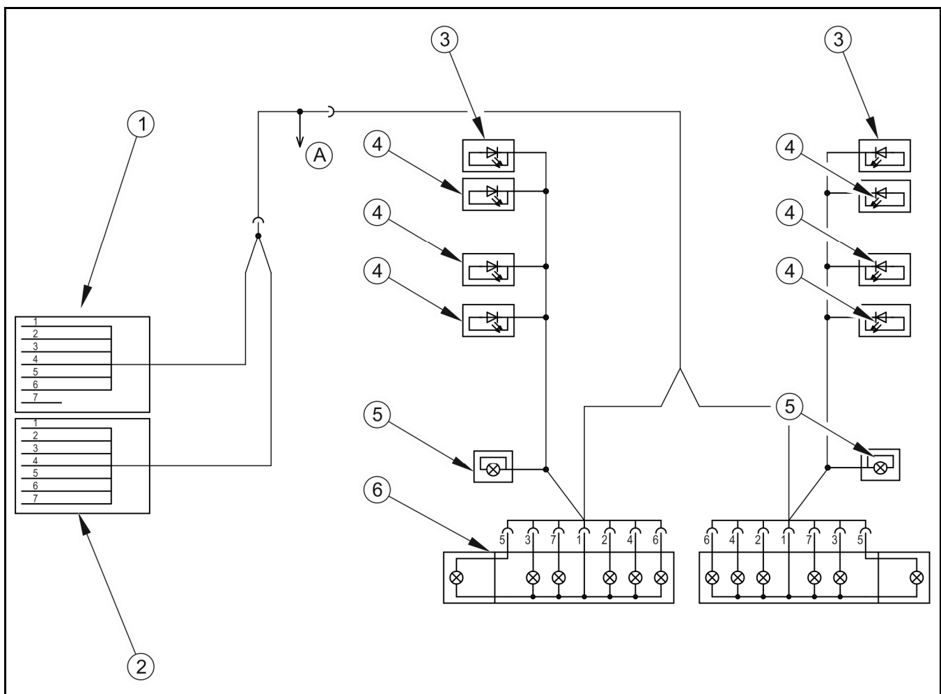
RYSUNEK 3.22 Schemat instalacji elektrycznej oświetleniowej
