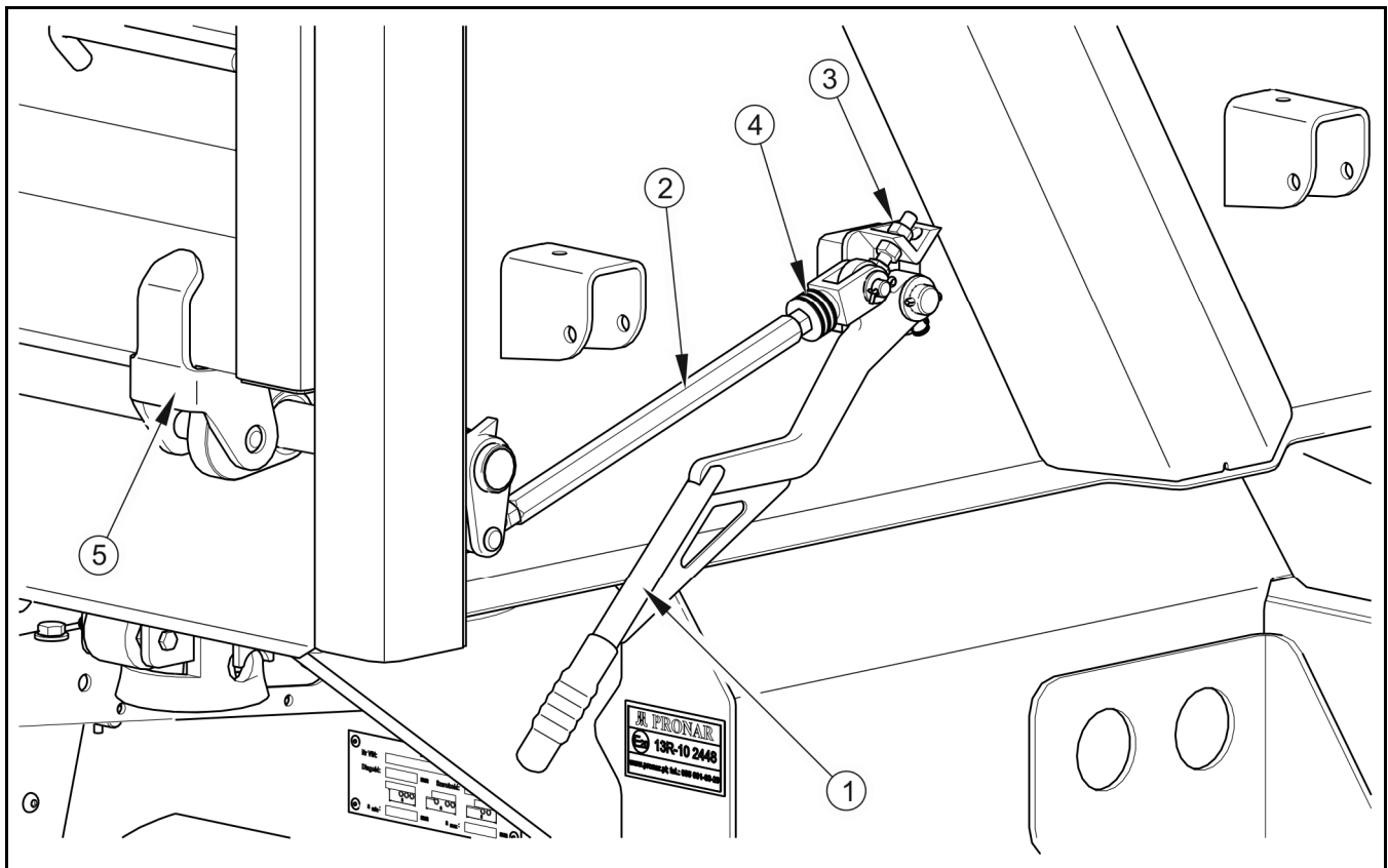
RYСУNEK 3.10 Zamknięcie boczne z prawej strony
