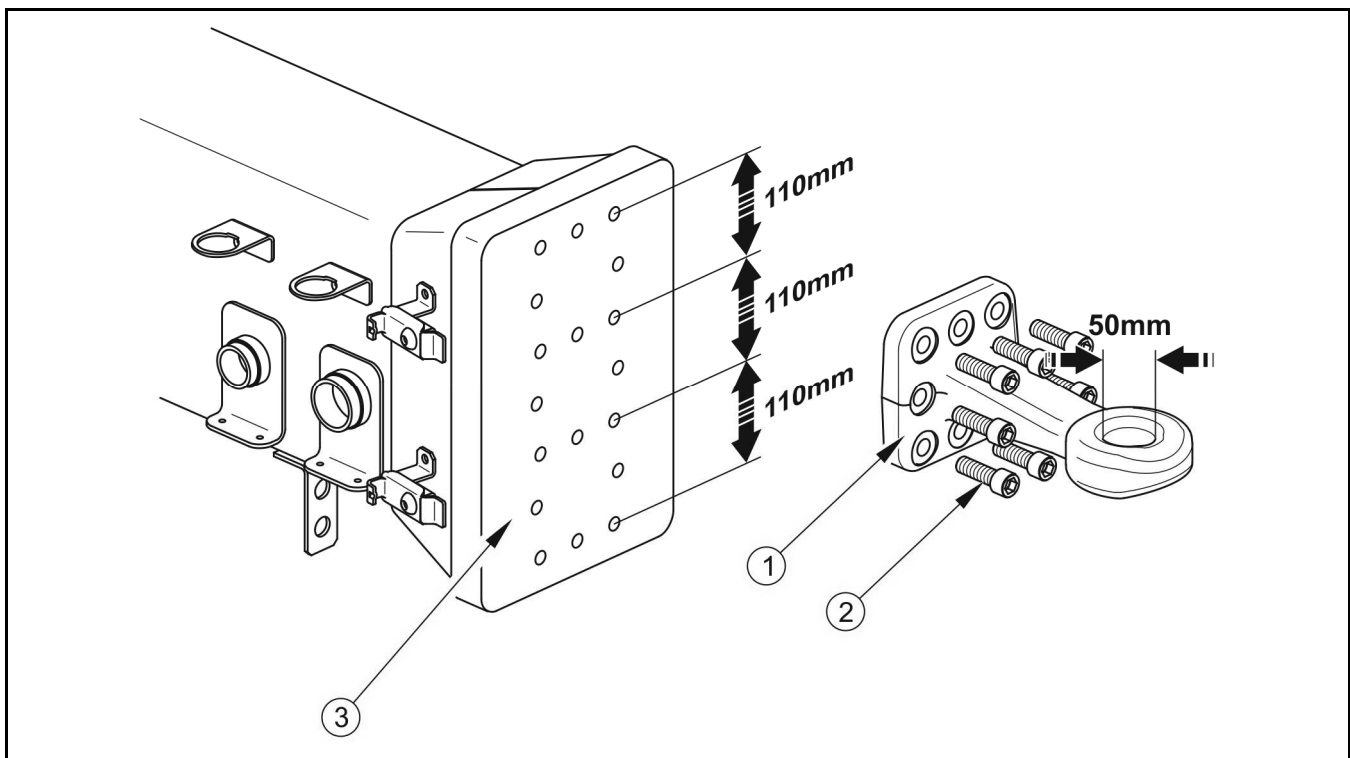
RYСУNEK 3.2 Ciągno dyszla
