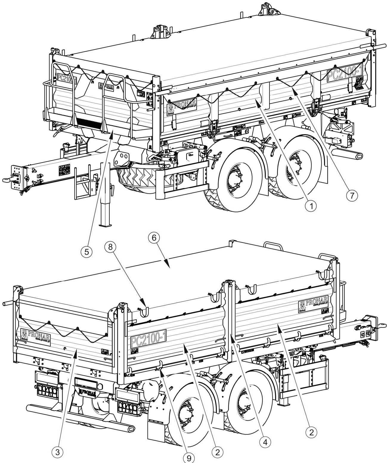
RYSUNEK 3.8 Skrzynia ładunkowa
