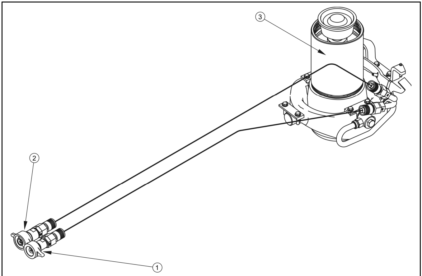
RYСУNEK 3.21 Budowa instalacji hydraulicznej wywrotu
