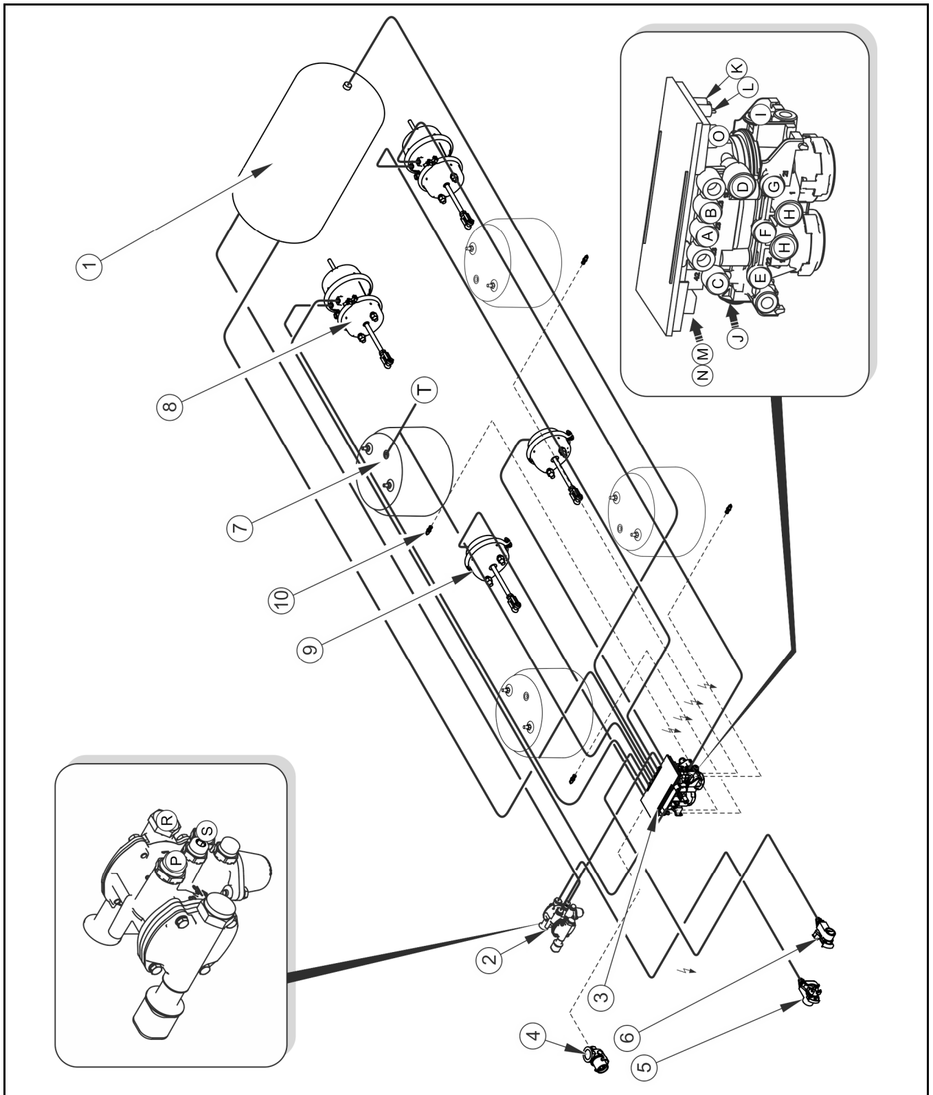
RYSUNEK 3.17 Schemat instalacji hamulcowej
