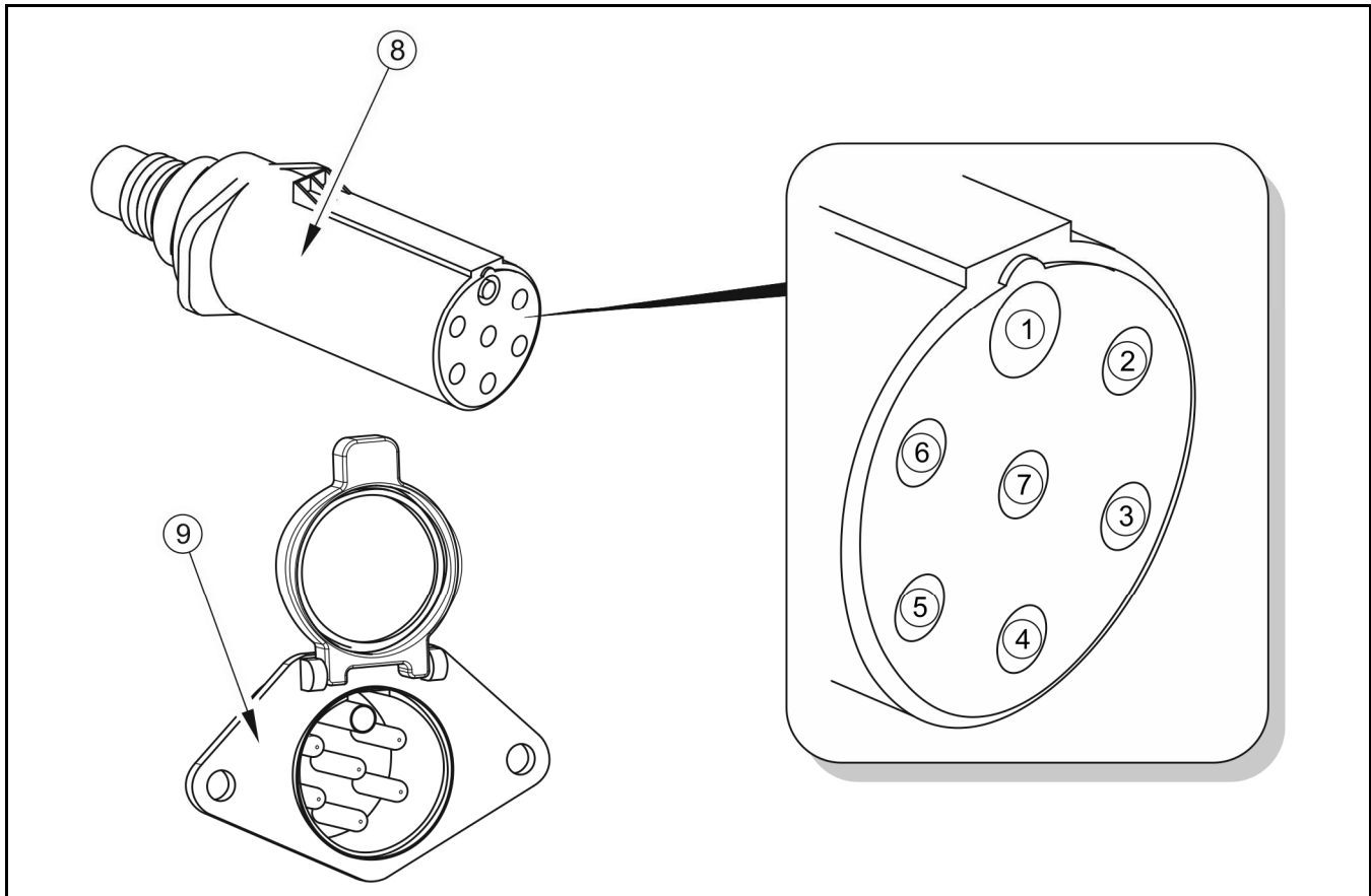
RYSUNEK 3.24 Wtyk z gniazdem 7 stykowym (ISO 3731)
