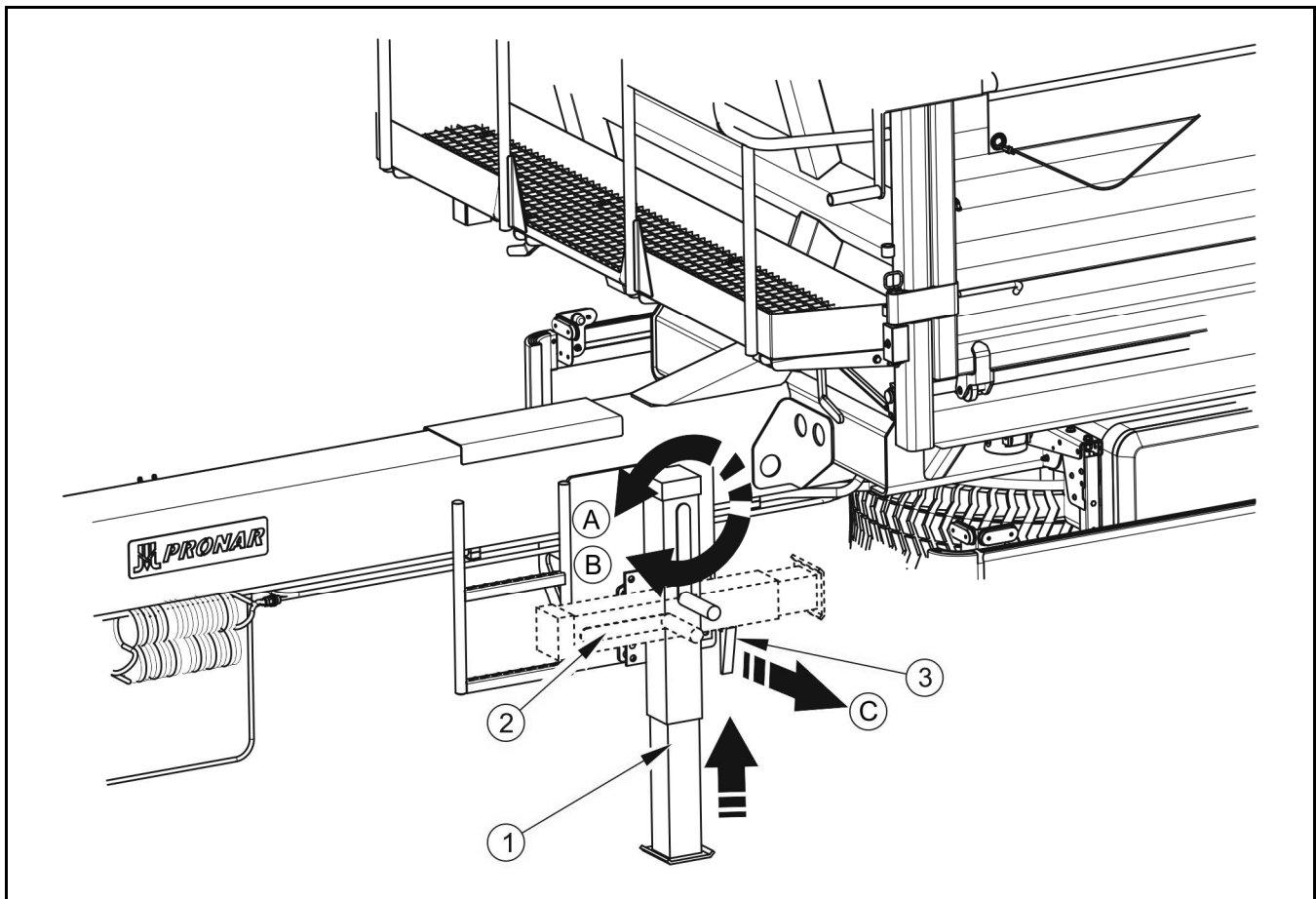
RYSUNEK 4.1 Składanie nogi podporowej przyczepy
