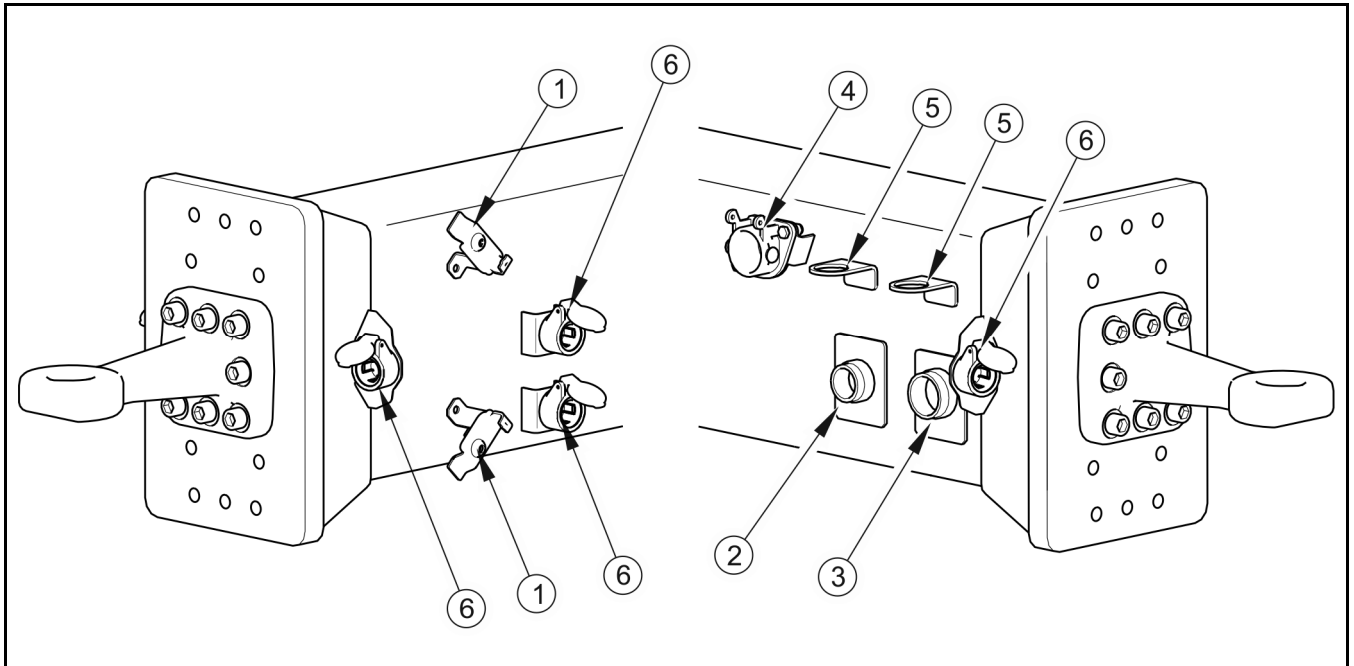
RYSUNEK 4.4 Gniazda złączy przyczepy
