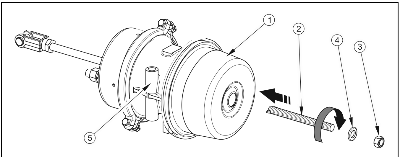
RYСУNEK 5.11 Awaryjne zwalnianie siłownika membranowego
