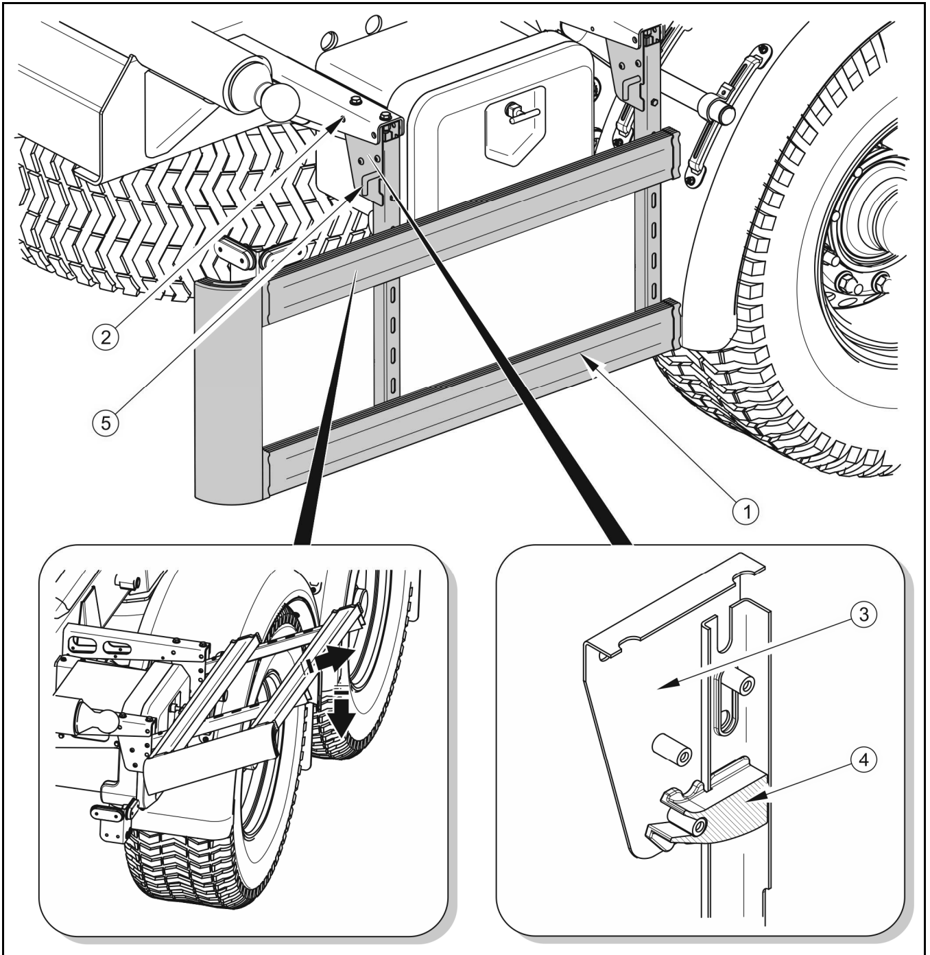
RYSUNEK 4.5 Osłona przeciwnajzdowa lewa
